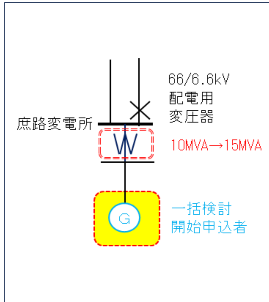
系統概略図
