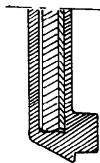
d 部縦断面図
