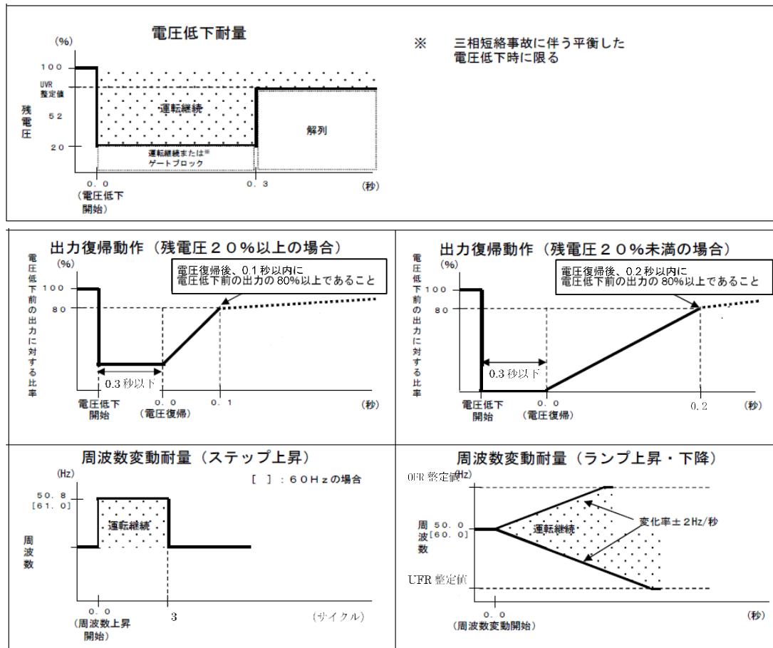
図Ⅲ－１ FRT 要件のイメージ（太陽光発電設備を例に記載）
