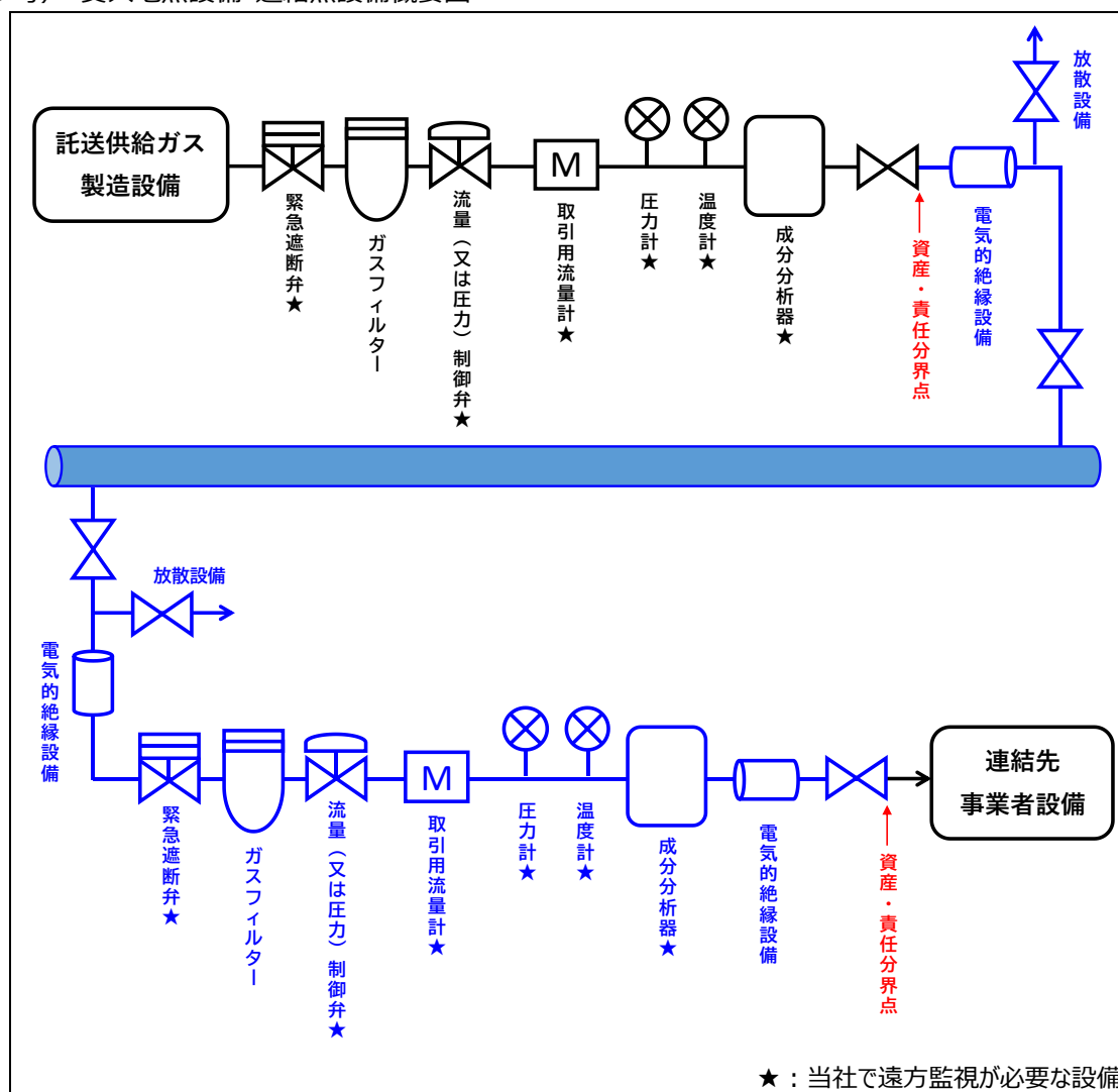
(参考) 受入地点設備・連結点設備概要図
