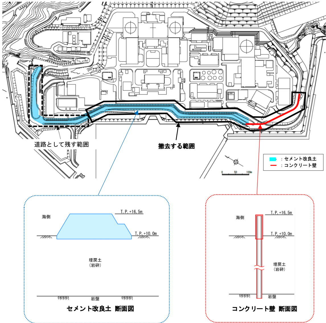
[撤去する既設防潮堤の構造]
