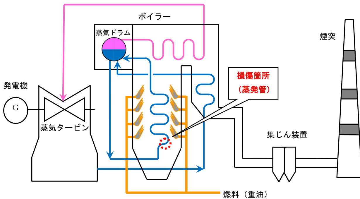
<ボイラー全体図>
