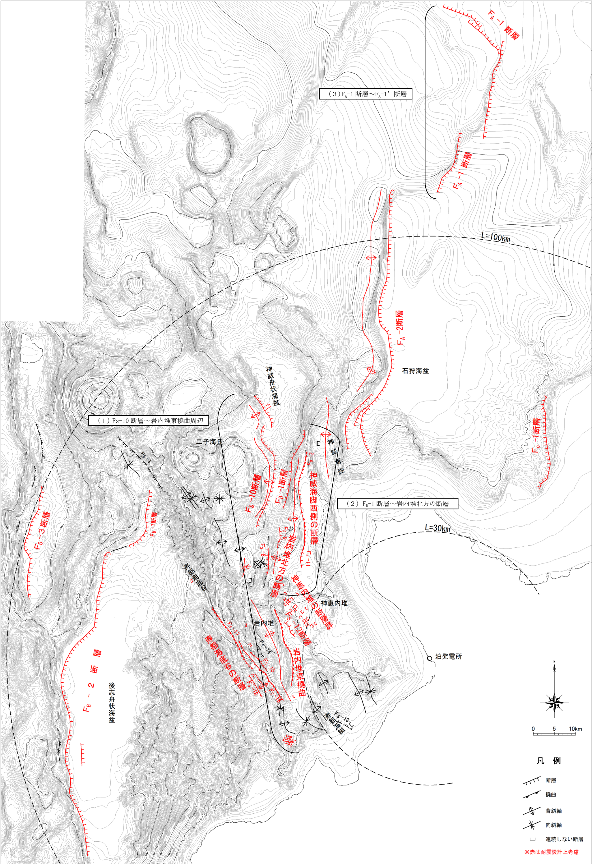
図 2 運動を考慮する活断層
