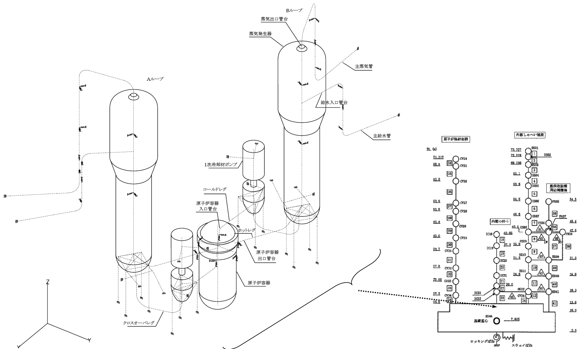
図 3-3 1 次冷却設備の建屋—機器連成解析モデル（例：水平方向）
