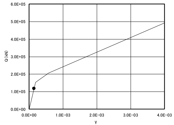
EL. 24.8m~EL. 20.0m 部材 21 (左 : E W方向、右 : N S 方向)
