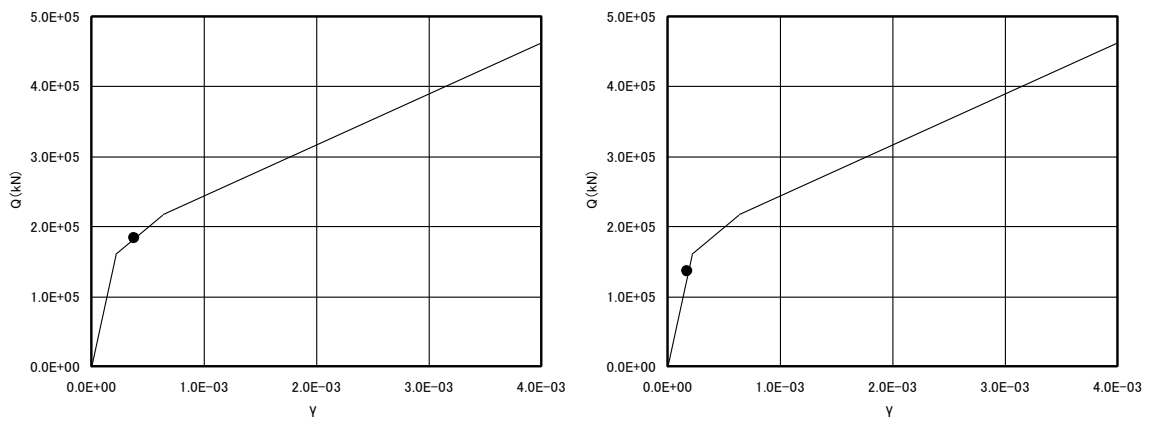
EL. 24.8m~EL. 18.3m 部材 11 (左 : E W 方向、右 : N S 方向)
