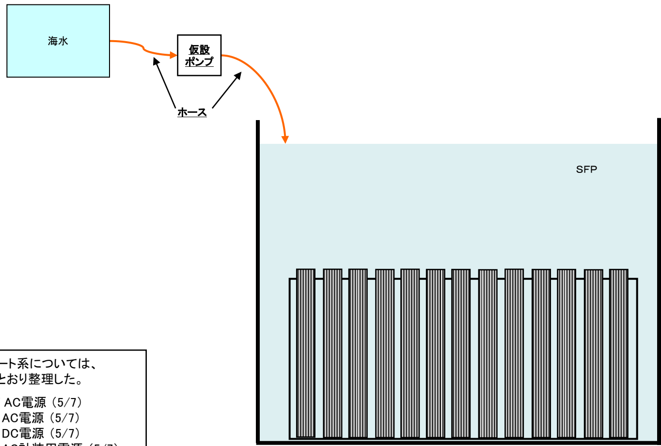
各影響緩和機能の系統図(地震:SFP燃料損傷)
