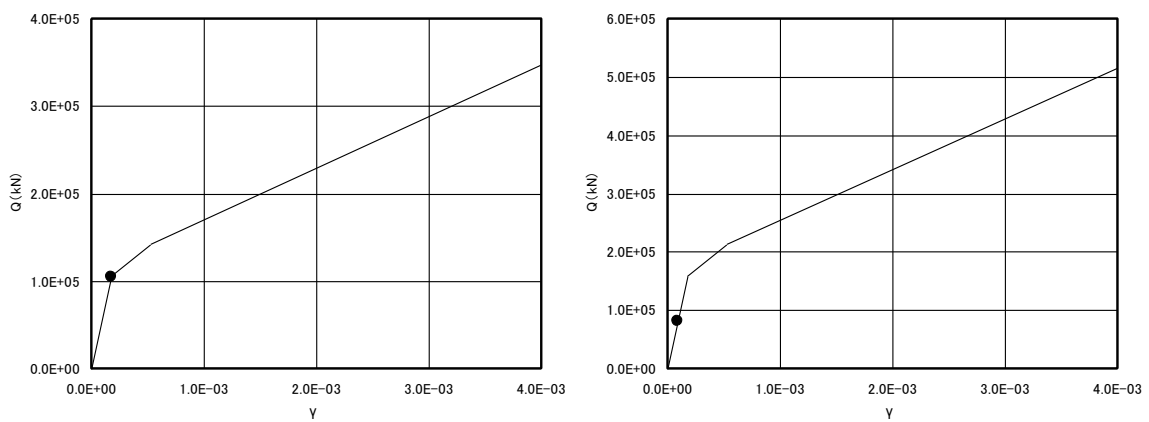
EL. 31.3m~EL. 24.8m 部材 20 (左 : E W方向、右 : N S 方向)
