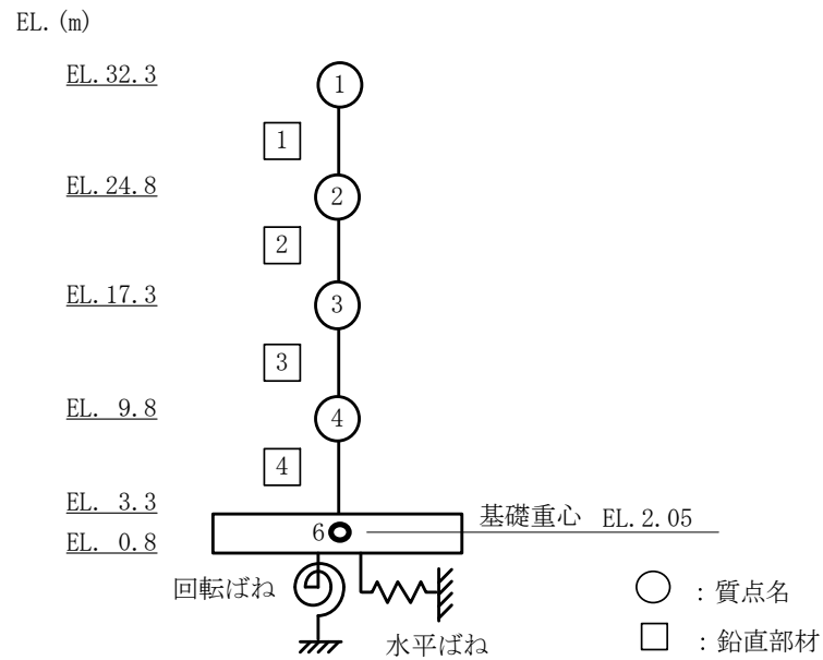
図 2-6 原子炉補助建屋の地震応答解析モデル（水平方向）
