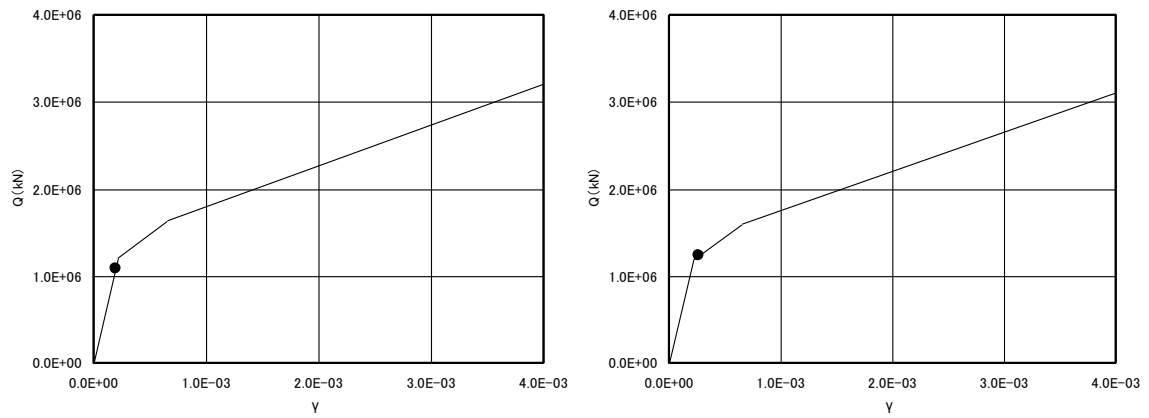
EL. 9.8m~EL. 3.3m 部材 4 (左 : E W 方向、右 : N S 方向)
