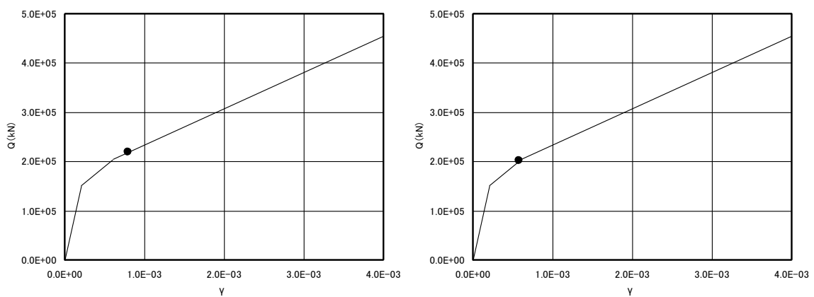
EL. 36.9m~EL. 31.3m 部材 9 (左 : E W 方向、右 : N S 方向)
