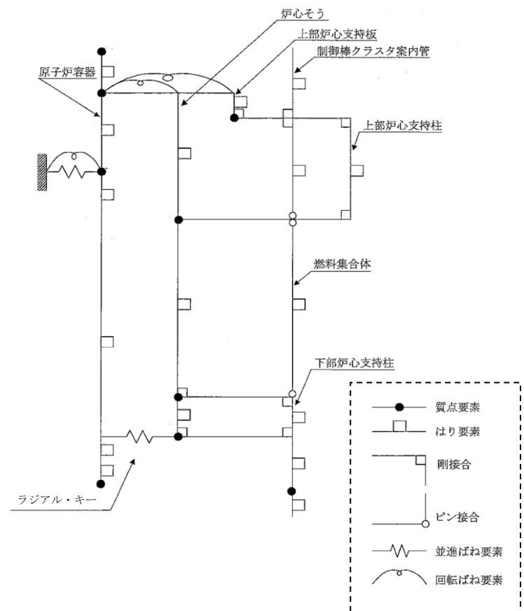
図 3-4 地震応答解析モデル（炉心支持構造物等の例）
