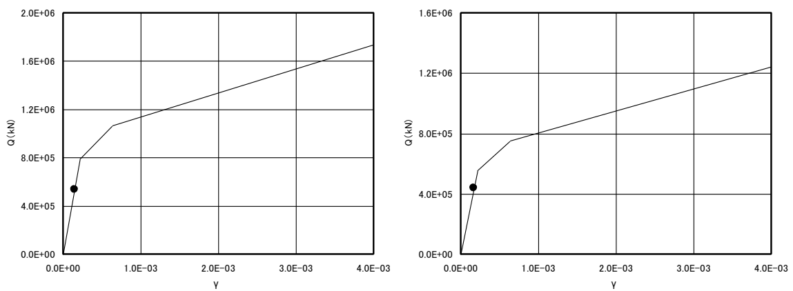
EL. 18. 3m~EL. 10. 3m 部材 41 (左 : E W方向、右 : N S 方向)
