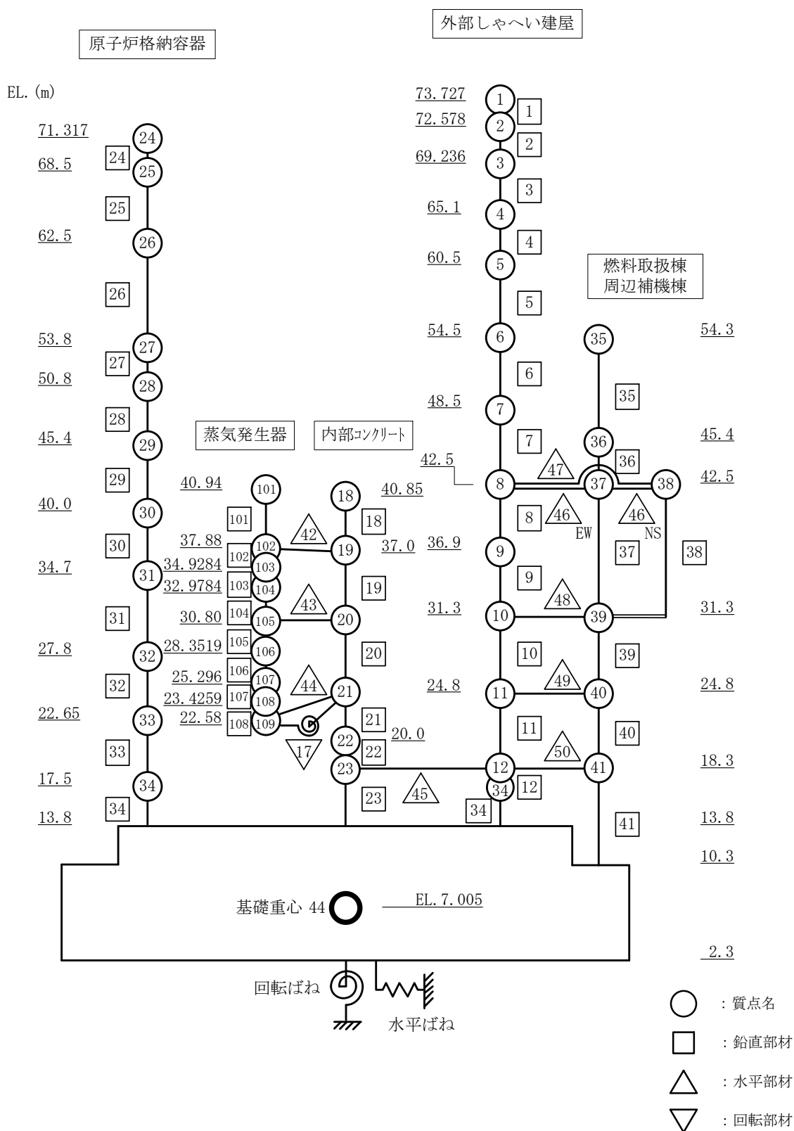
図 2-1 原子炉建屋の地震応答解析モデル（水平方向）
