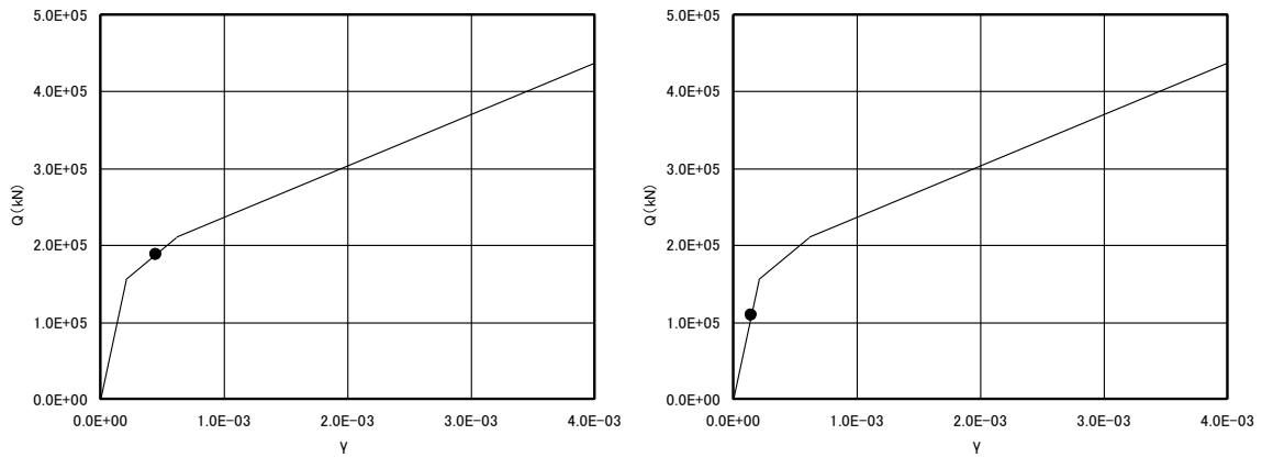
EL. 31.3m~EL. 24.8m 部材 10 (左 : E W 方向、右 : N S 方向)
