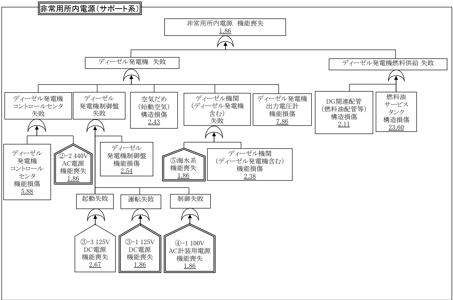
各影響緩和機能のフォールトツリー(地震:SFP燃料損傷)
