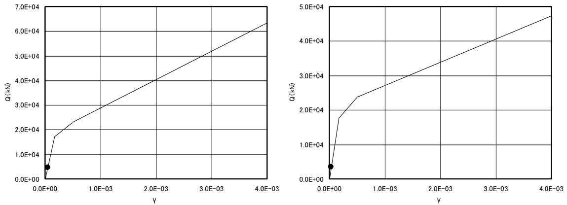
EL. 40.85m~EL. 37.0m 部材 18 (左 : E W方向、右 : N S 方向)
