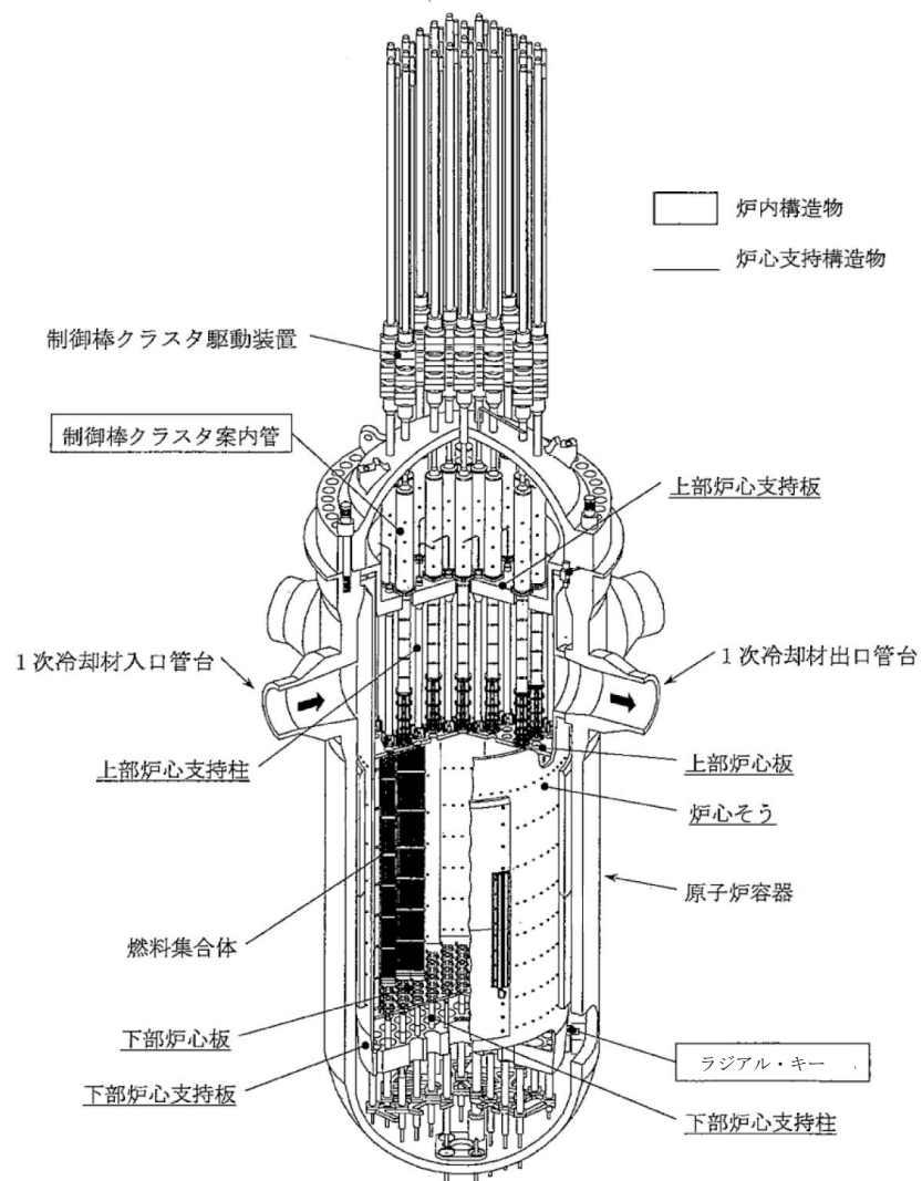
図 3-4 地震応答解析モデル（炉心支持構造物等の例）
