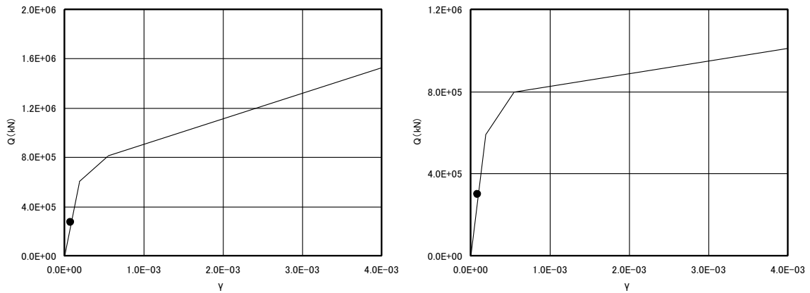
EL. 31. 3m~EL. 24. 8m 部材 39 (左 : E W方向、右 : N S 方向)
