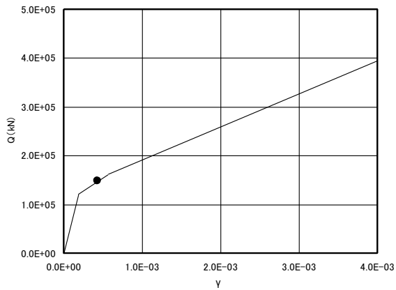
EL. 24.8m~EL. 20.0m 部材 21 (左 : E W方向、右 : N S 方向)
