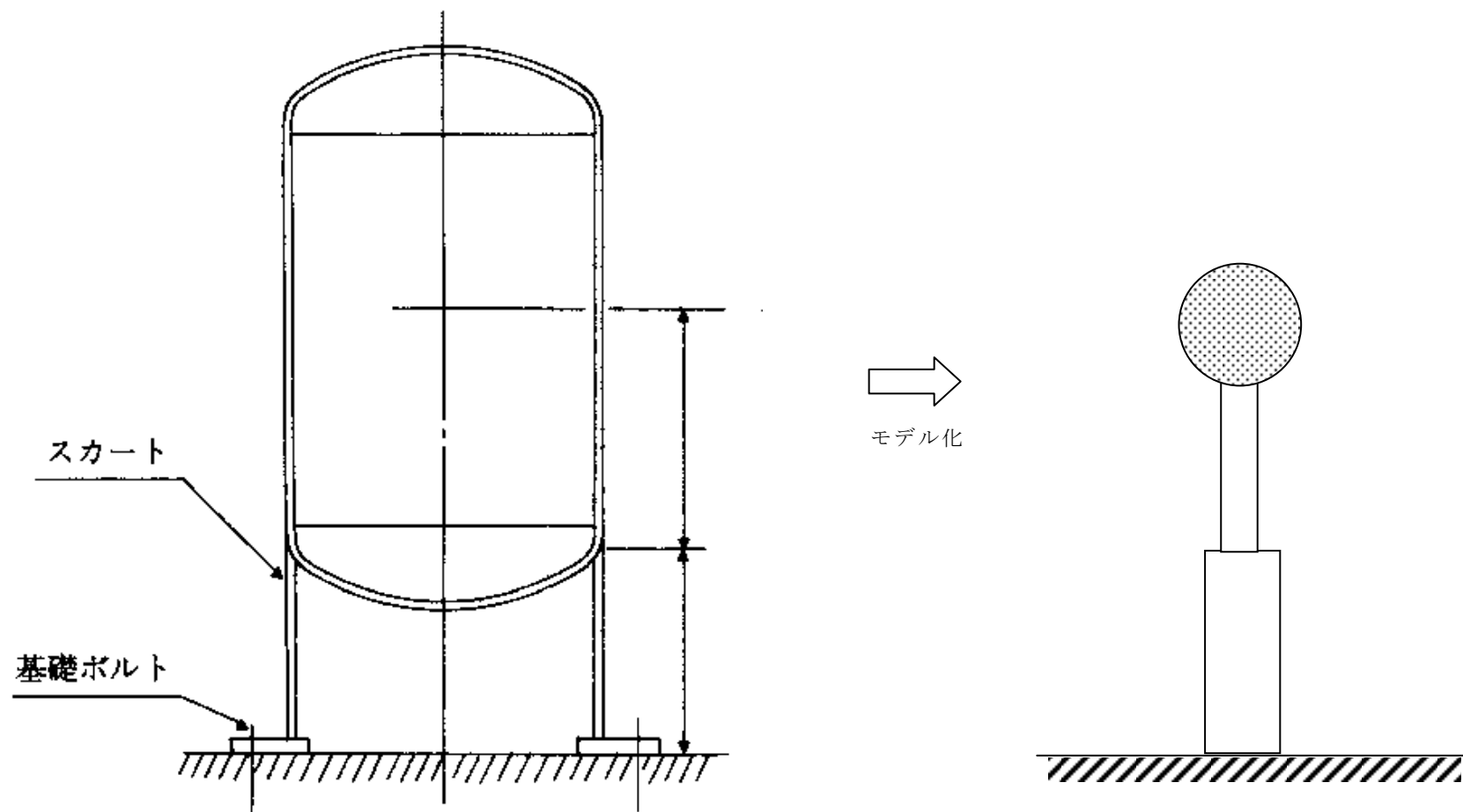
図 3-5 地震応答解析モデル（容器の例）
