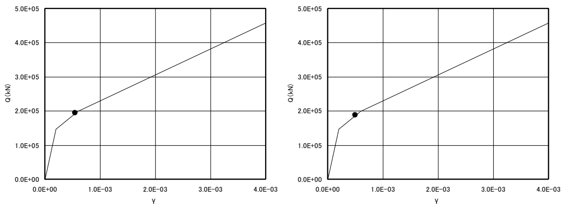
EL. 42.5m~EL. 36.9m 部材 8 (左 : E W 方向、右 : N S 方向)
