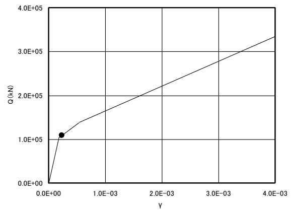
EL. 60.5m~EL. 54.5m 部材 5 (左 : E W 方向、右 : N S 方向)
