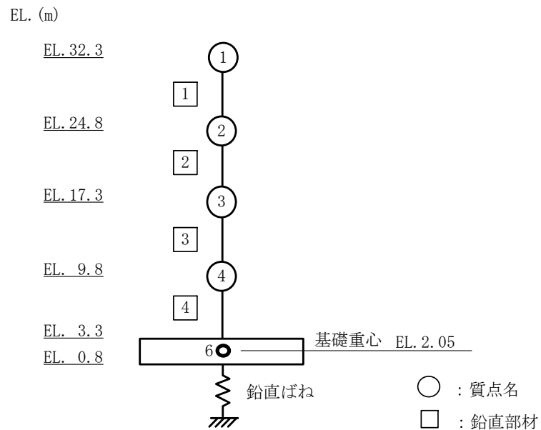
図 2-7 原子炉補助建屋の地震応答解析モデル（鉛直方向）
