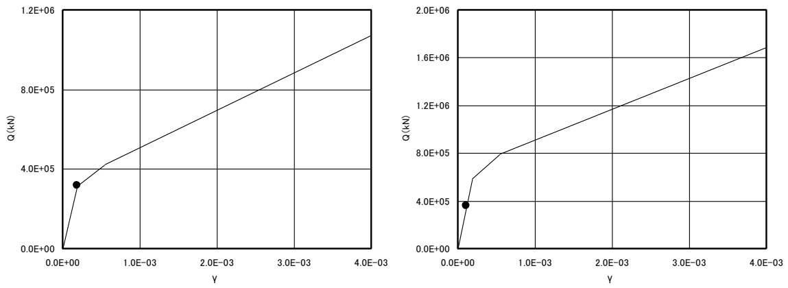
EL. 32.3m~EL. 24.8m 部材 1 (左 : E W 方向、右 : N S 方向)
