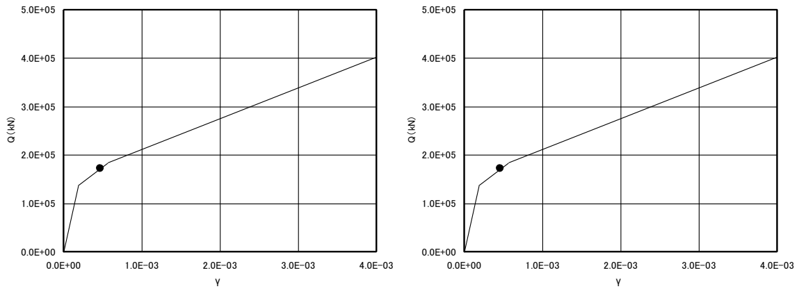
EL. 48.5m~EL. 42.5m 部材 7 (左 : E W 方向、右 : N S 方向)
