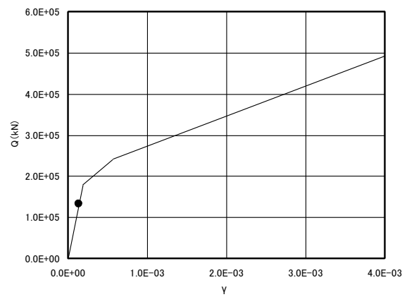
EL. 20.0m~EL. 18.3m 部材 22 (左 : E W方向、右 : N S 方向)
