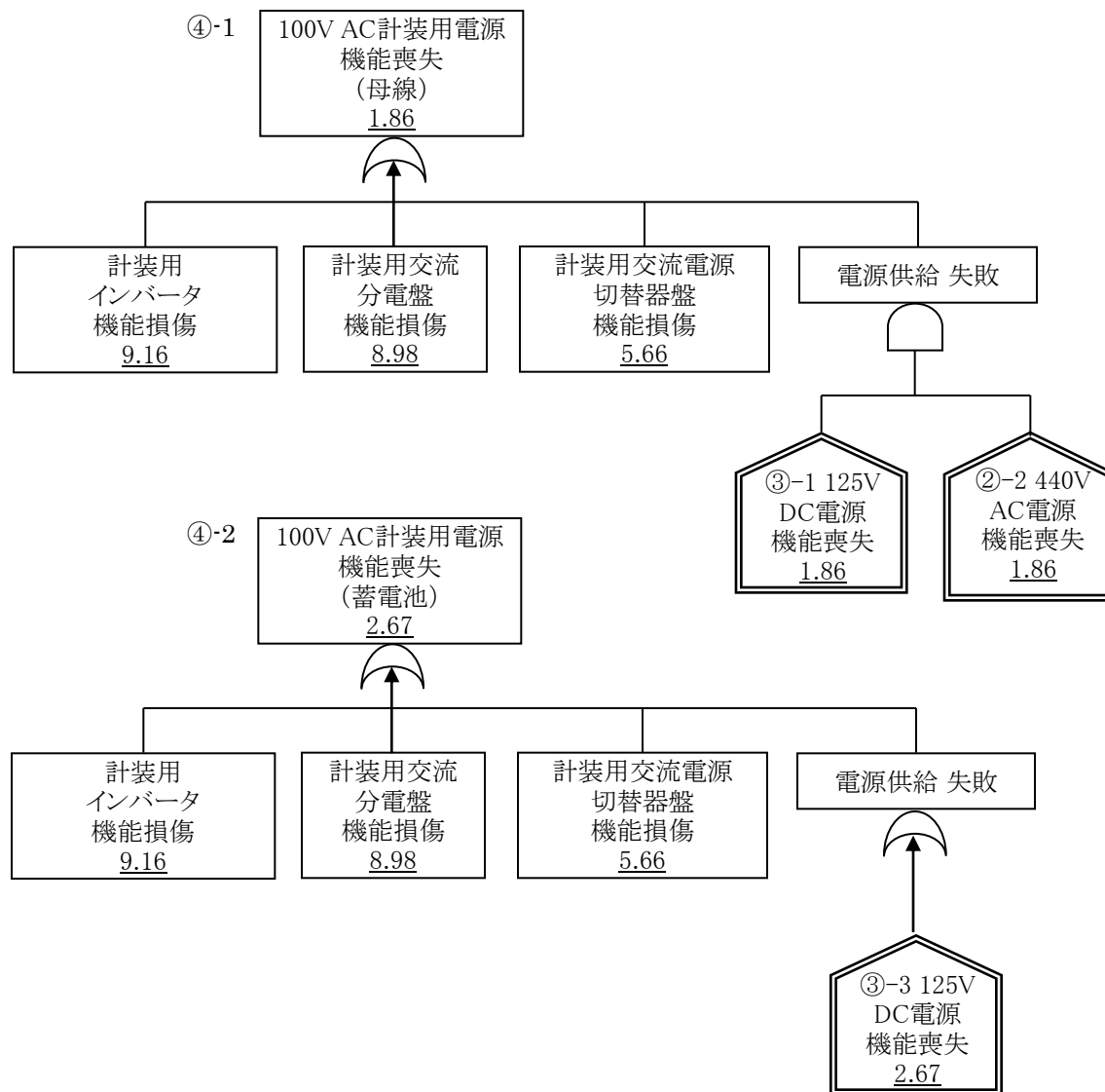
各影響緩和機能のフォールトツリー(地震:炉心損傷)
