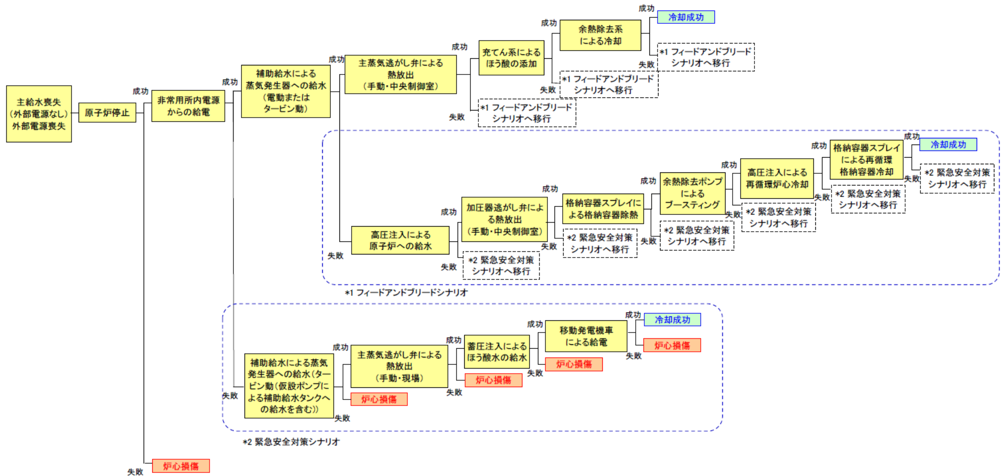
各起因事象におけるイベントツリー（地震：炉心損傷）
