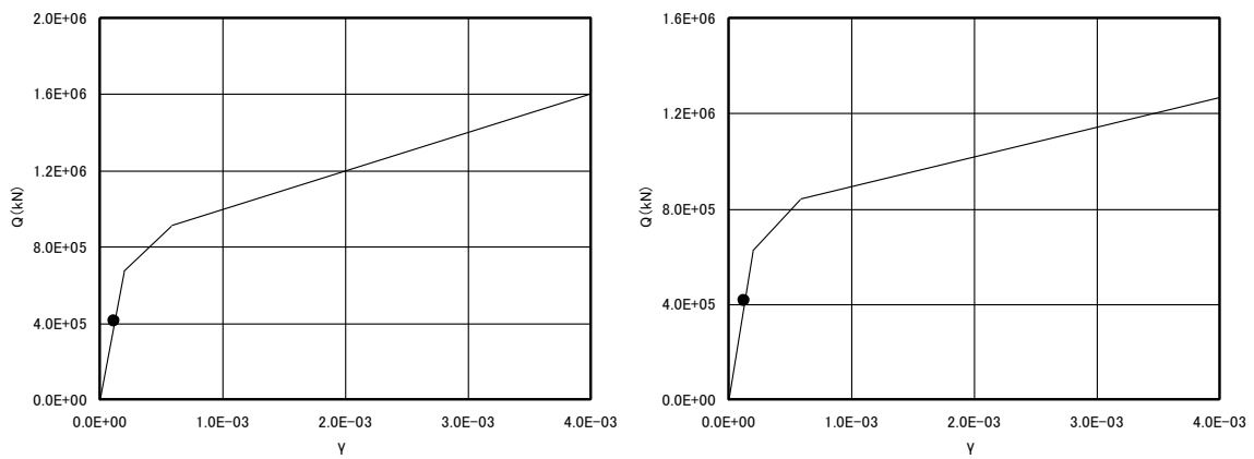
EL. 24. 8m~EL. 18. 3m 部材 40 (左 : E W方向、右 : N S 方向)
