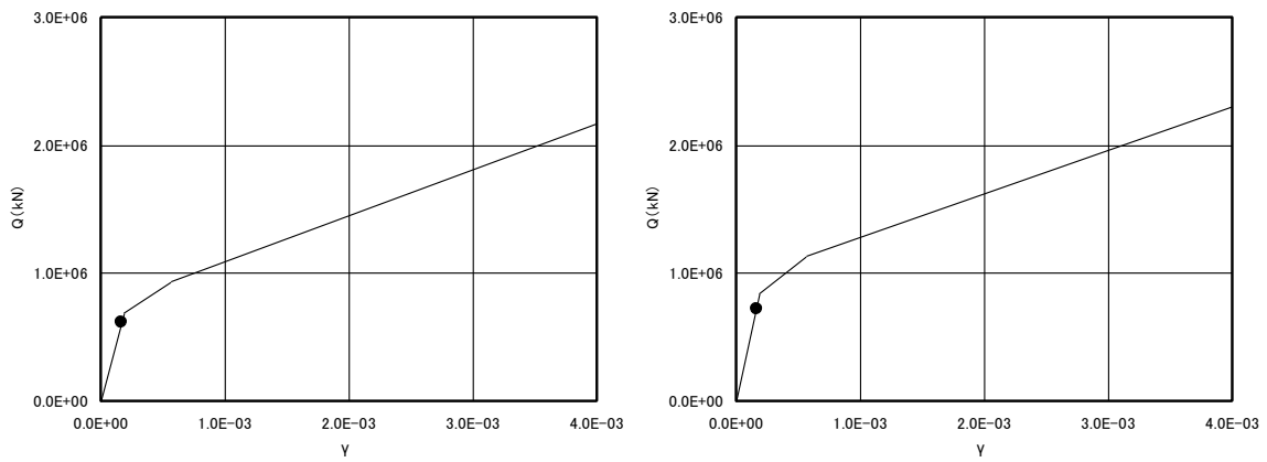
EL. 24.8m~EL. 17.3m 部材 2 (左 : E W 方向、右 : N S 方向)
