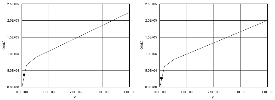
EL. 37.0m~EL. 31.3m 部材 19 (左 : E W方向、右 : N S 方向)
