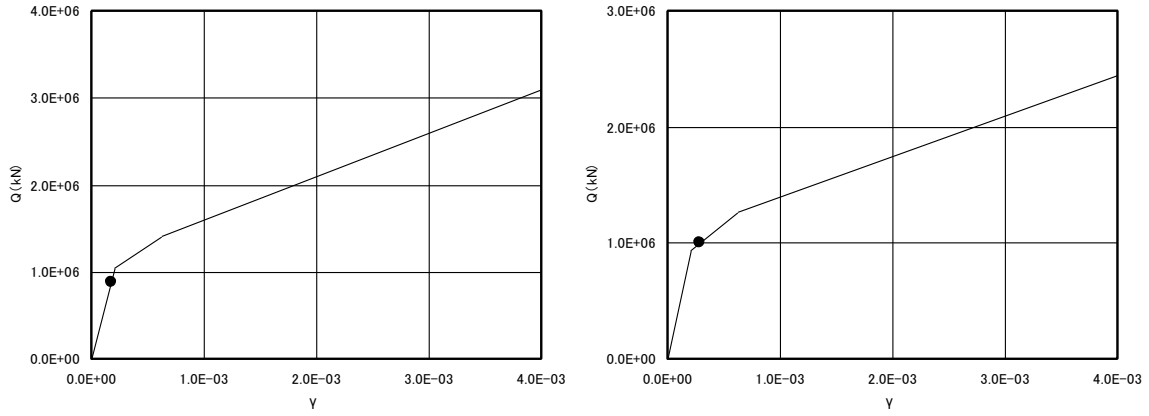
EL. 17.3m~EL. 9.8m 部材 3 (左 : E W 方向、右 : N S 方向)
