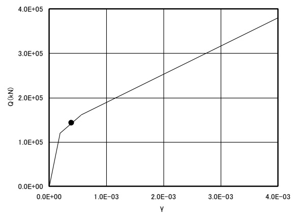
EL. 54.5m~EL. 48.5m 部材 6 (左 : E W 方向、右 : N S 方向)
