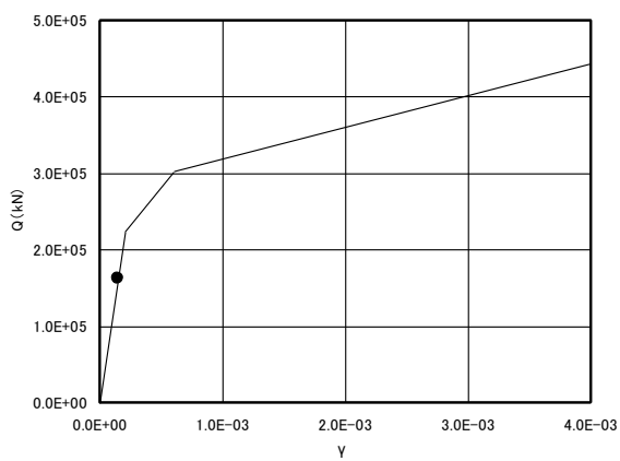
EL. 18.3m~EL. 13.8m 部材 23 (左 : E W方向、右 : N S 方向)
