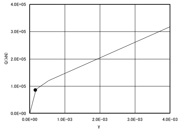
EL. 65.1m~EL. 60.5m 部材 4 (左 : E W 方向、右 : N S 方向)
