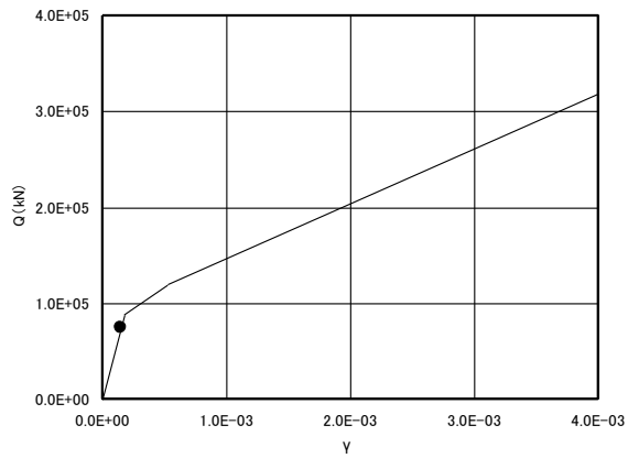
EL. 65.1m~EL. 60.5m 部材 4 (左 : E W 方向、右 : N S 方向)
