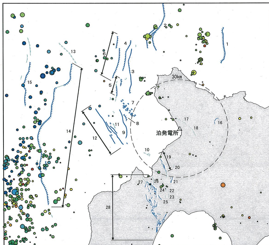
東北地方太平洋沖地震の発生前 (2010年1月1日～2011年3月11日14時45分)
