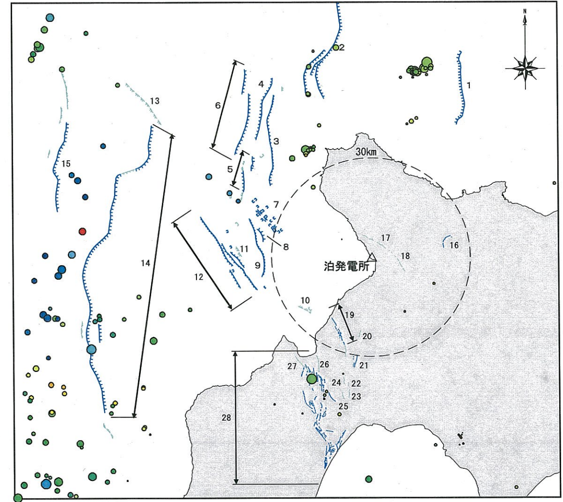
東北地方太平洋沖地震の発生後 (2011年3月11日14時46分～2011年7月31日)
