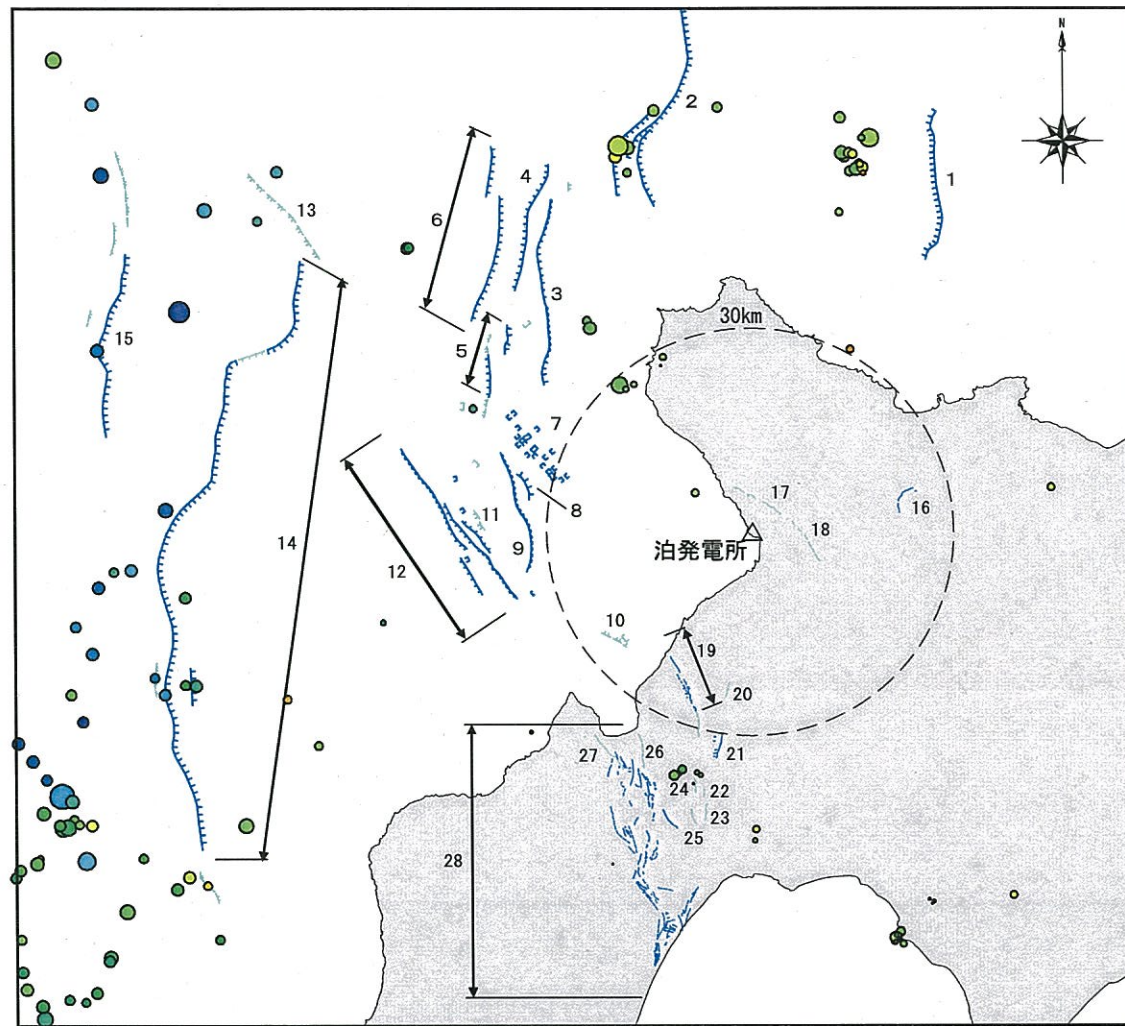
東北地方太平洋沖地震の発生前 (2010年11月1日～2011年3月11日14時45分)
