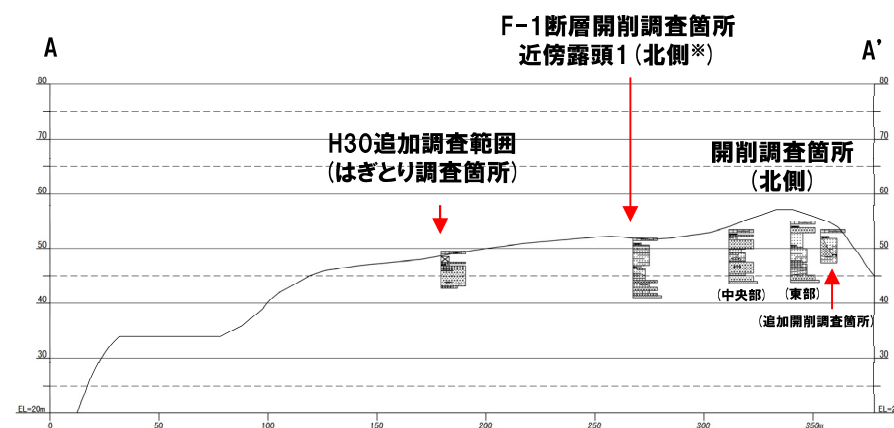
A-A' 断面図
