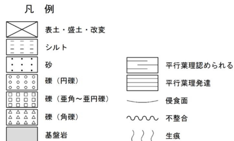
D-D'断面図
