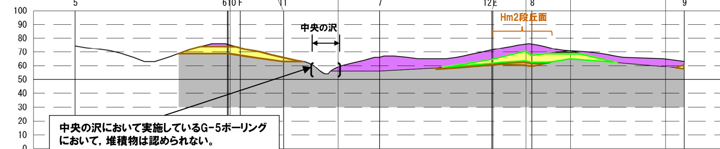
L断面図
