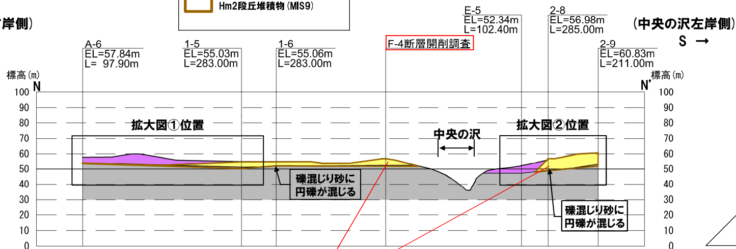
N断面図
