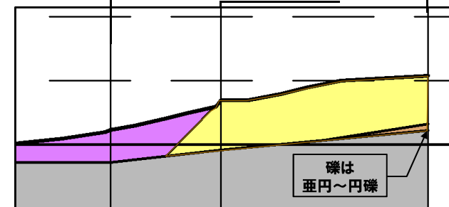
拡大図②
