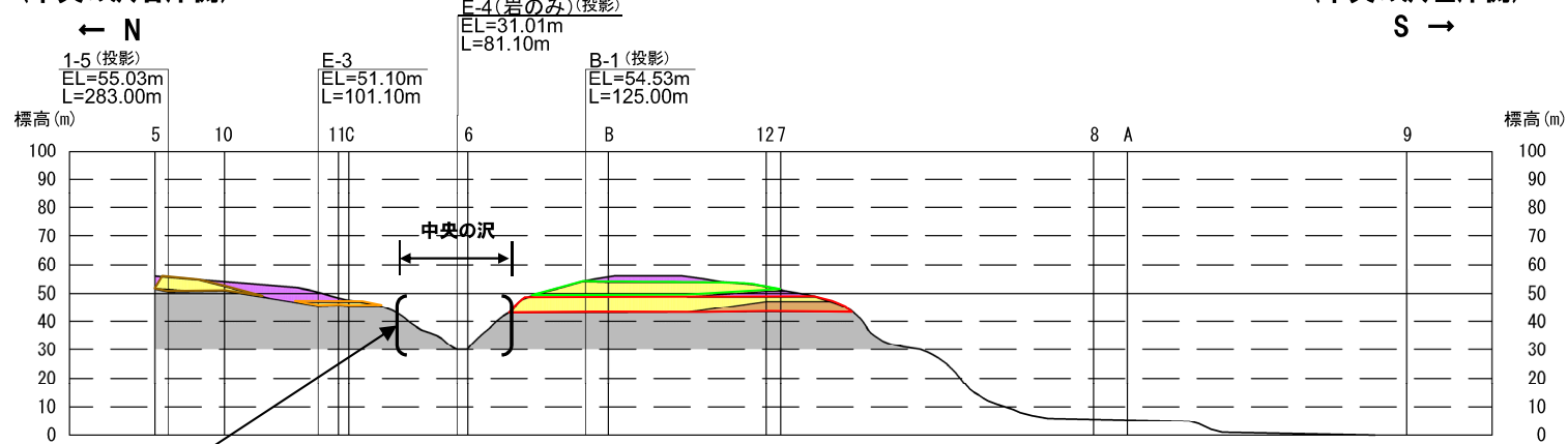
G断面図
