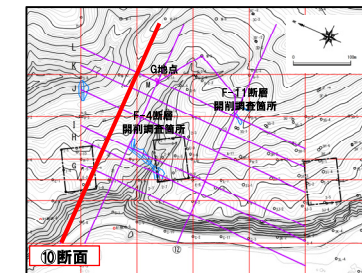
断面位置図
