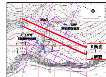
断面位置図
