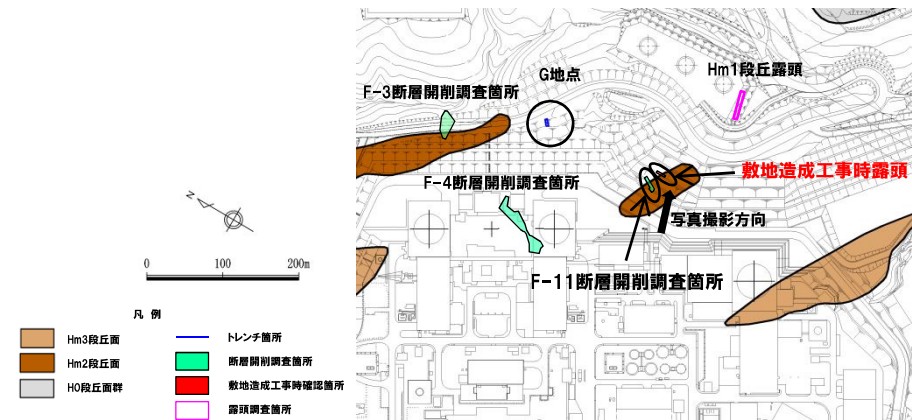
調査位置図
