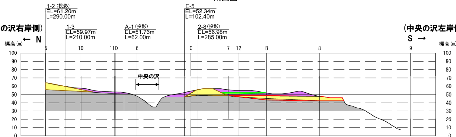
H断面図
