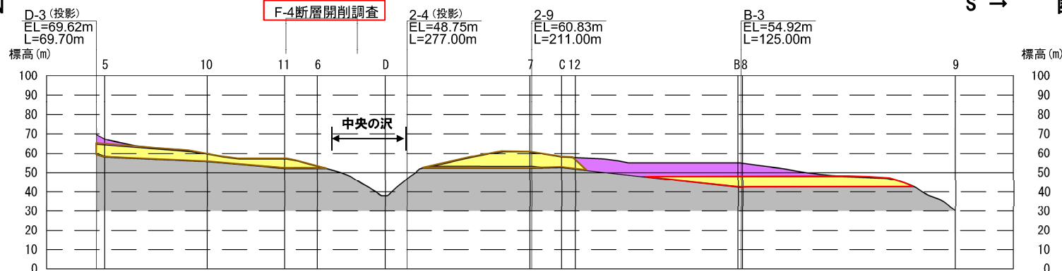
I断面図
