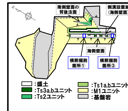
硬度測定実施箇所
