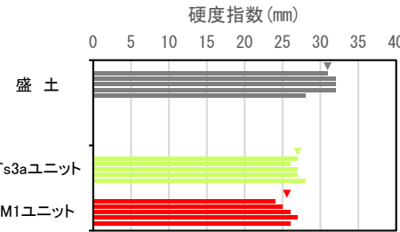
硬度測定結果 (測線:SKB-FF③)
