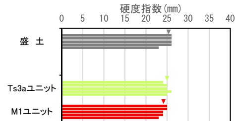
硬度測定結果 (測線:SKB-FF⑤)
