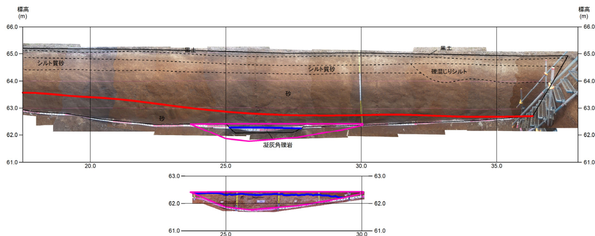
トレンチ壁面写真(A-1) (範囲B)
