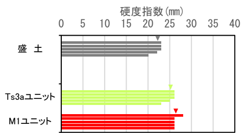
硬度測定結果 (測線:SKB-FF④)
