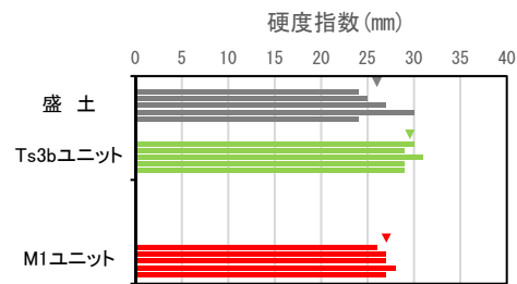
硬度測定結果 (測線:SKB-FF①)
