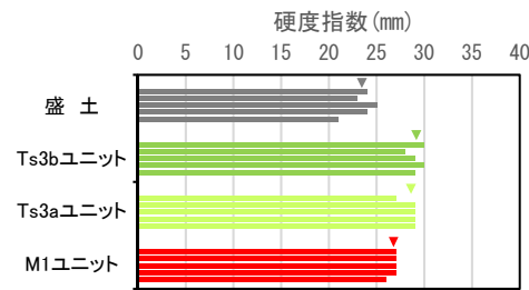
硬度測定結果 (測線:SKB-FF②)
