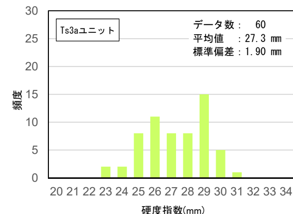
硬度指数のヒストグラム (Ts3aユニット)
