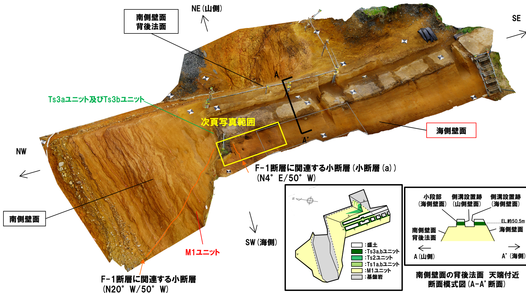
開削調査箇所(南側)露頭状況
