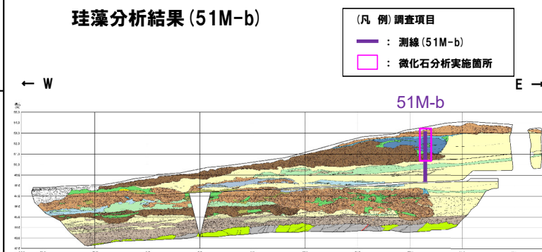
開削調査箇所(北側) 北側壁面 珪藻分析位置
