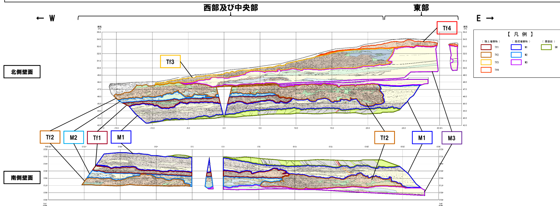
開削調査箇所(北側) 展開図
