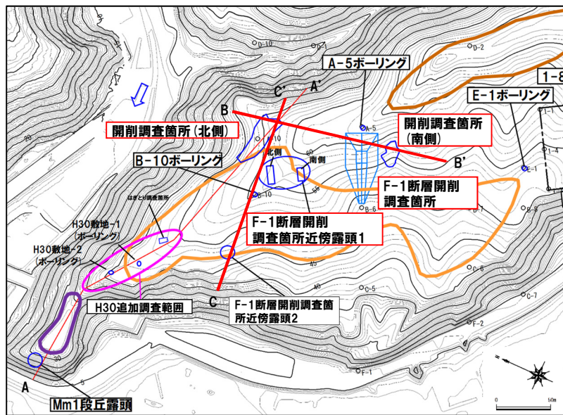
平面図(改変前の地形)
