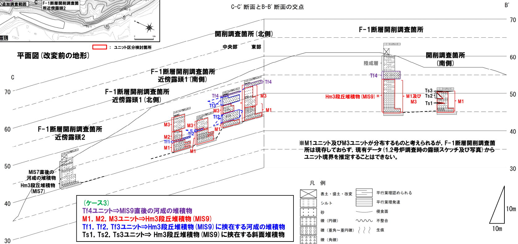
断面図 (C-B' 断面) (ケース3)
