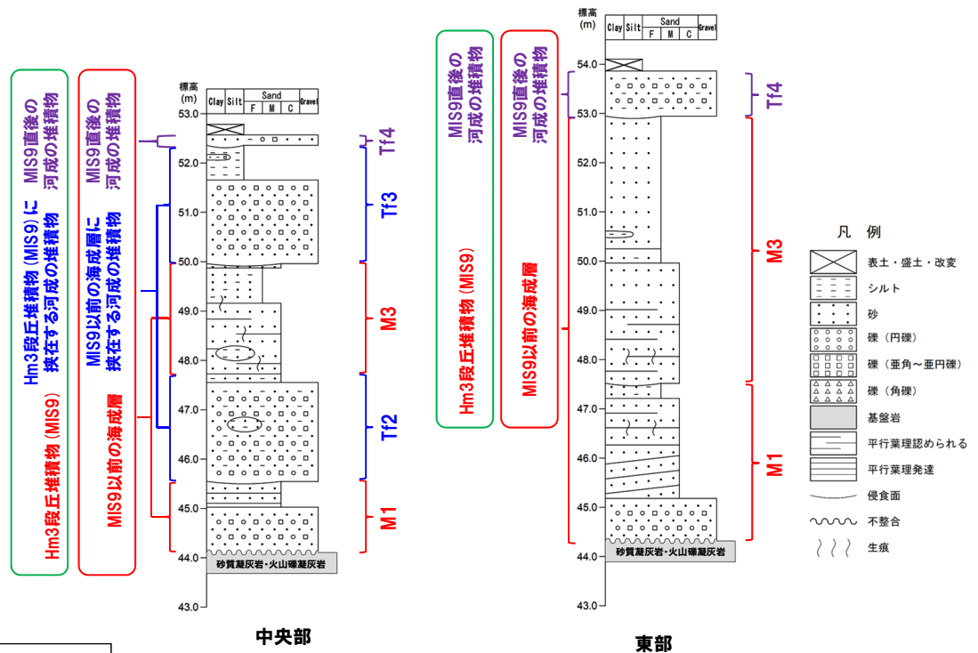
代表柱状図 (開削調査箇所(北側))
