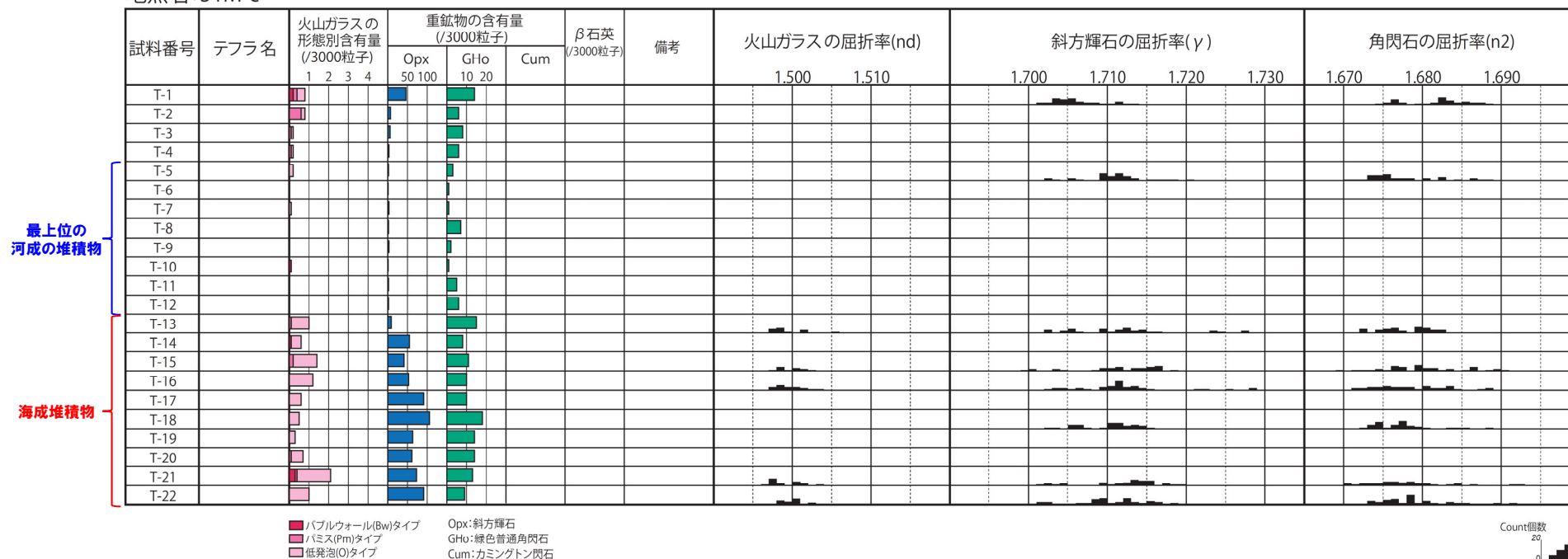
51M-c 火山灰分析結果
