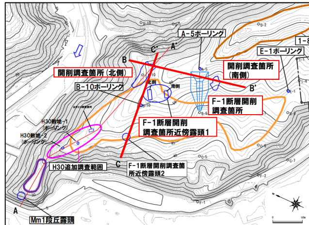
平面図 (改変前の地形)
