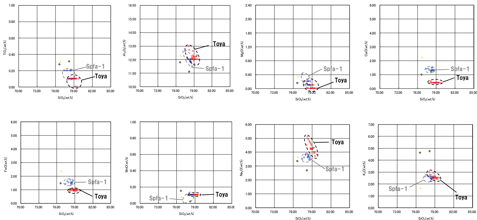
51M-c 火山ガラスの主元素組成 (ハーカー図)
