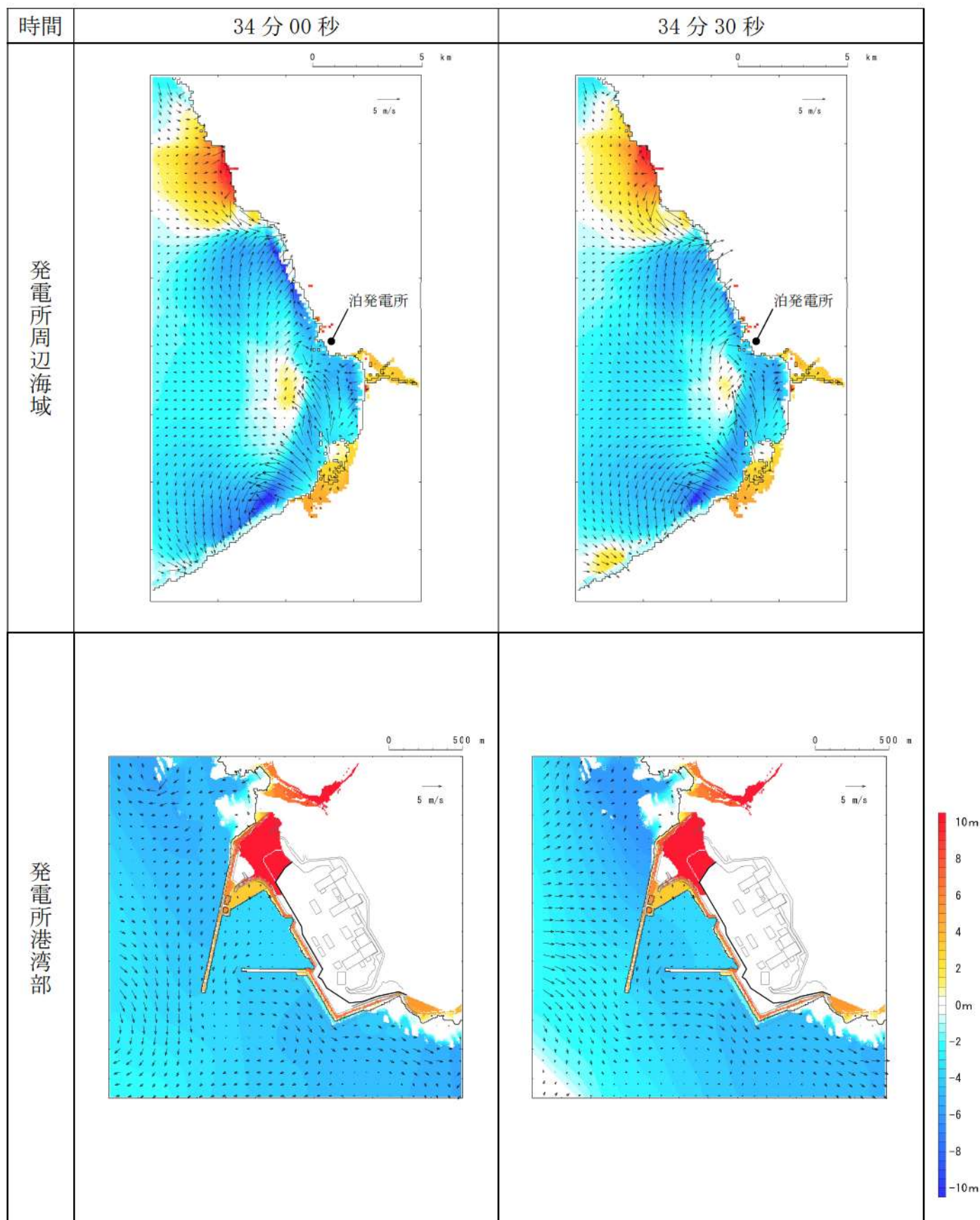
第 15 図-24 基準津波 I（防波堤損傷なし）の水位変動・流向ベクトル(24/50)
