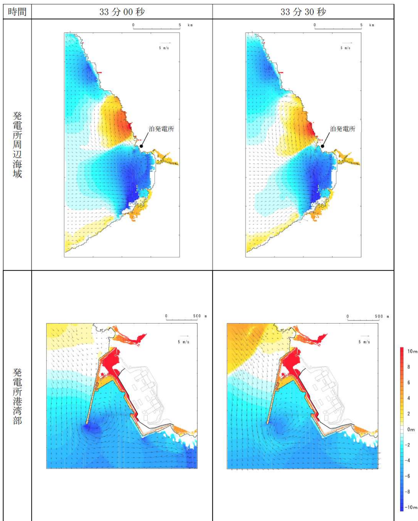
第 17 図-26 基準津波K（南防波堤損傷）の水位変動・流向ベクトル(26/53)
