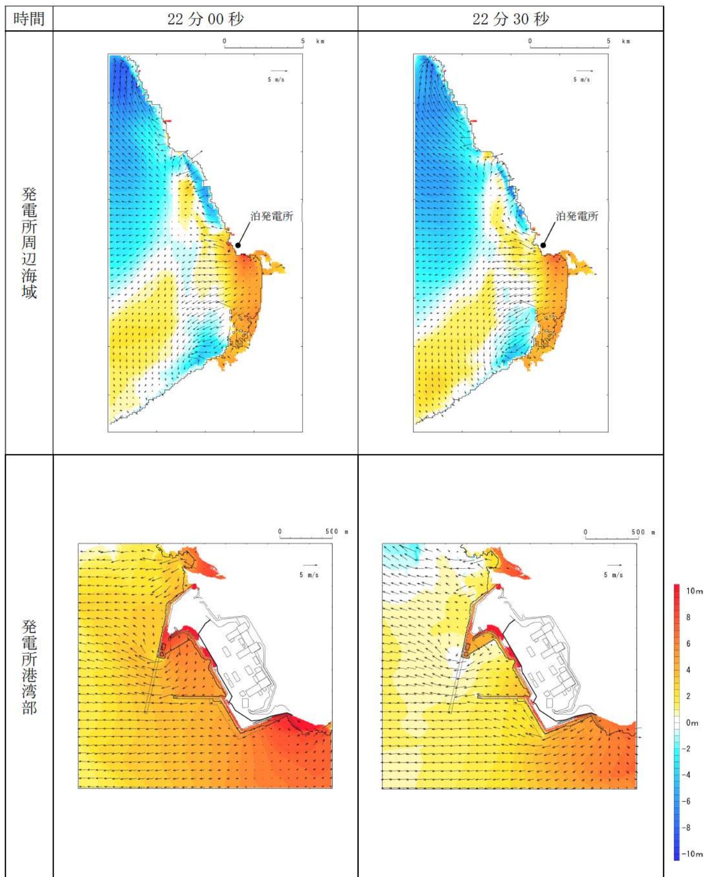
第 18 図-15 基準津波 L（北防波堤損傷）の水位変動・流向ベクトル(15/53)
