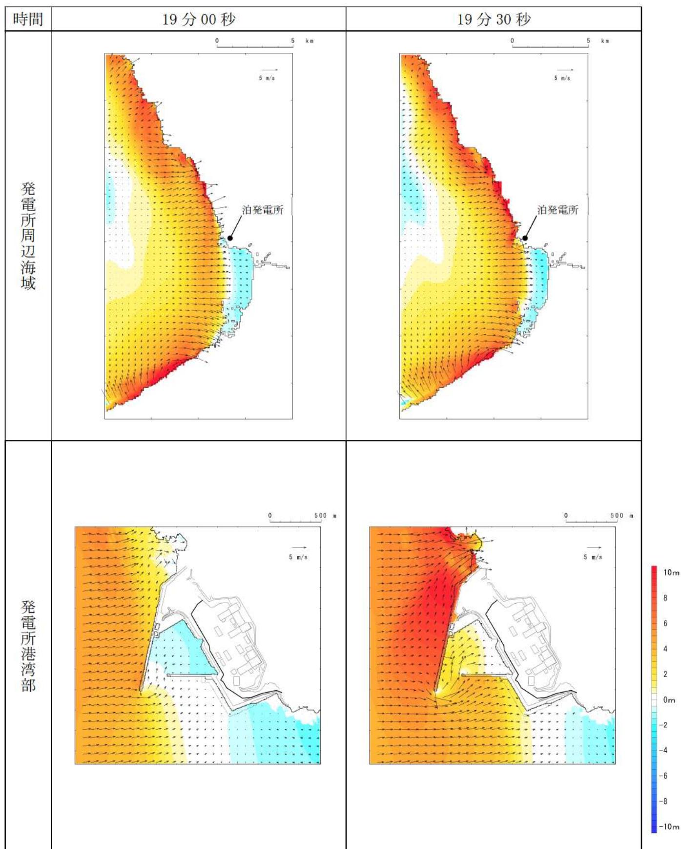
第 15 図-9 基準津波 I (防波堤損傷なし) の水位変動・流向ベクトル (9/50)
