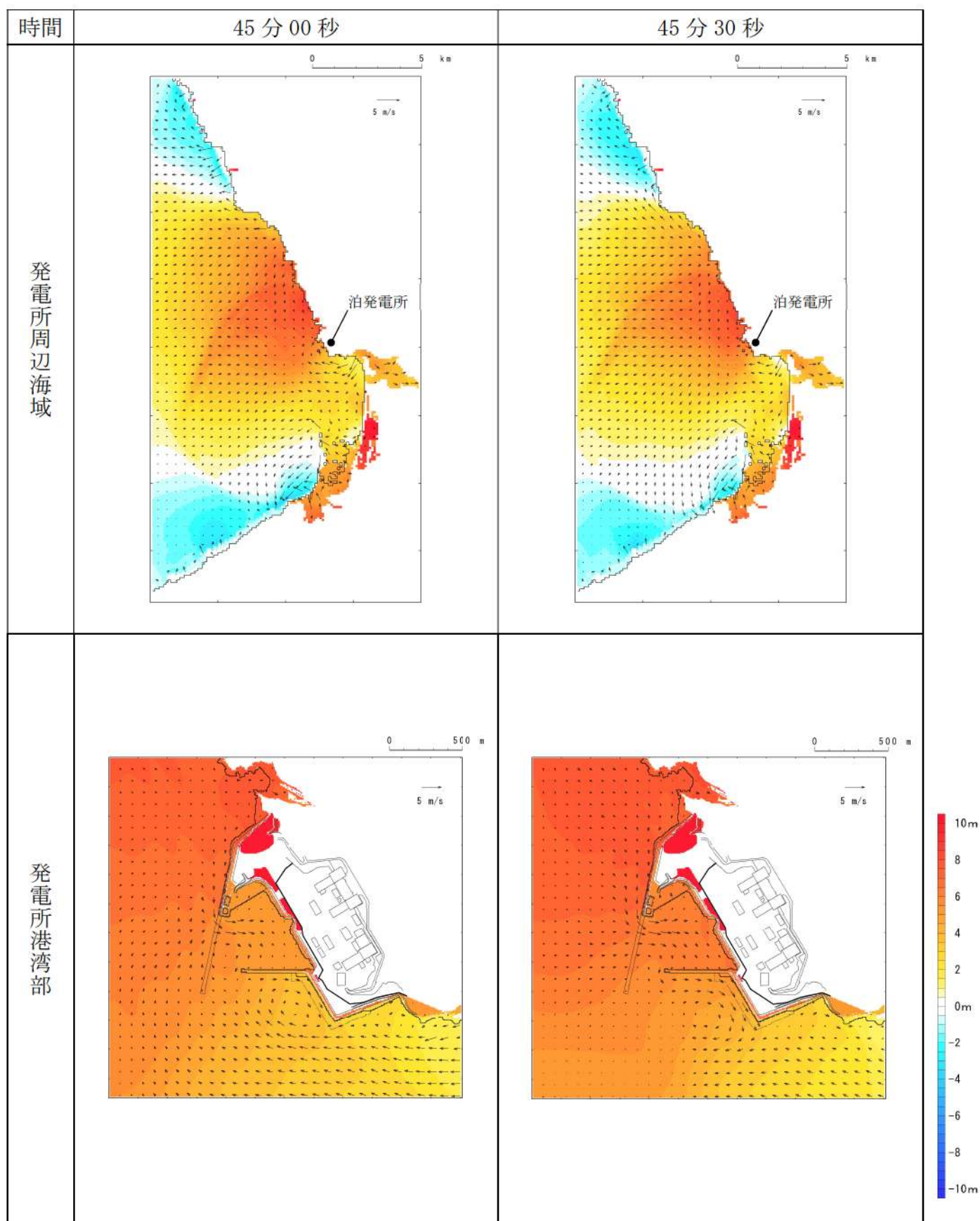
第 18 図-38 基準津波 L（北防波堤損傷）の水位変動・流向ベクトル(38/53)
