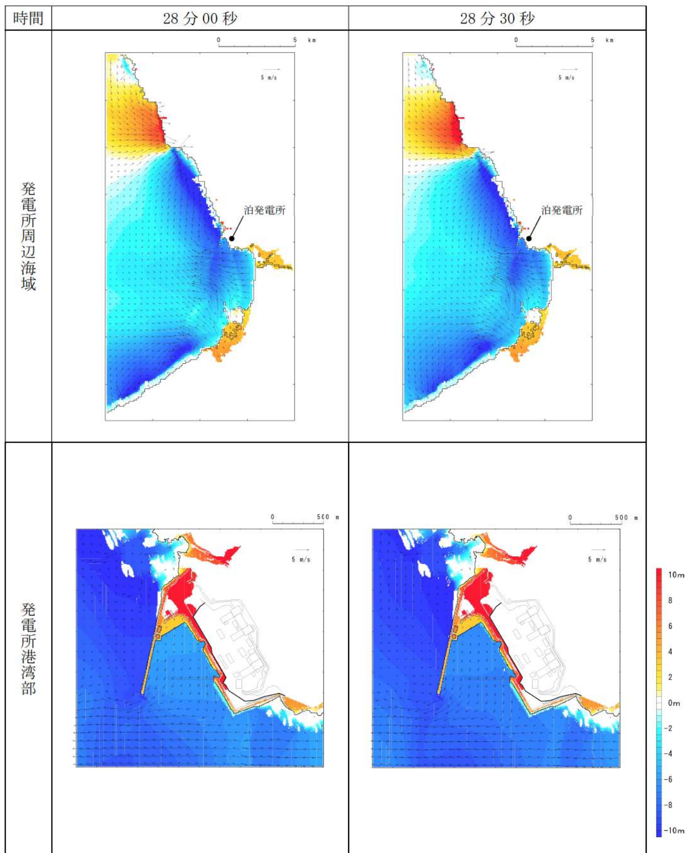
第 17 図-21 基準津波K（南防波堤損傷）の水位変動・流向ベクトル(21/53)
