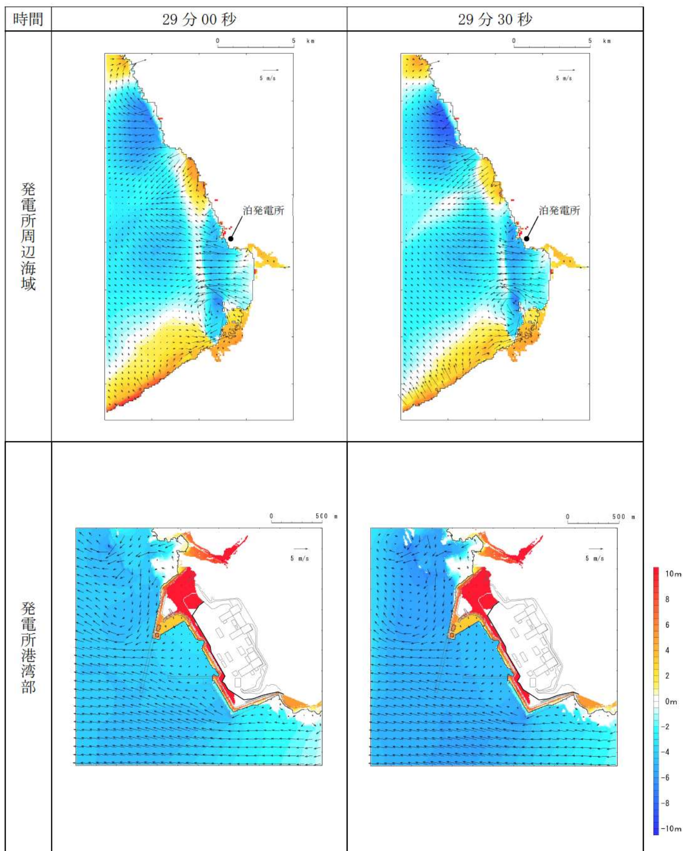
第 16 図-18 基準津波 J（北及び南防波堤損傷）の水位変動・流向ベクトル(18/49)
