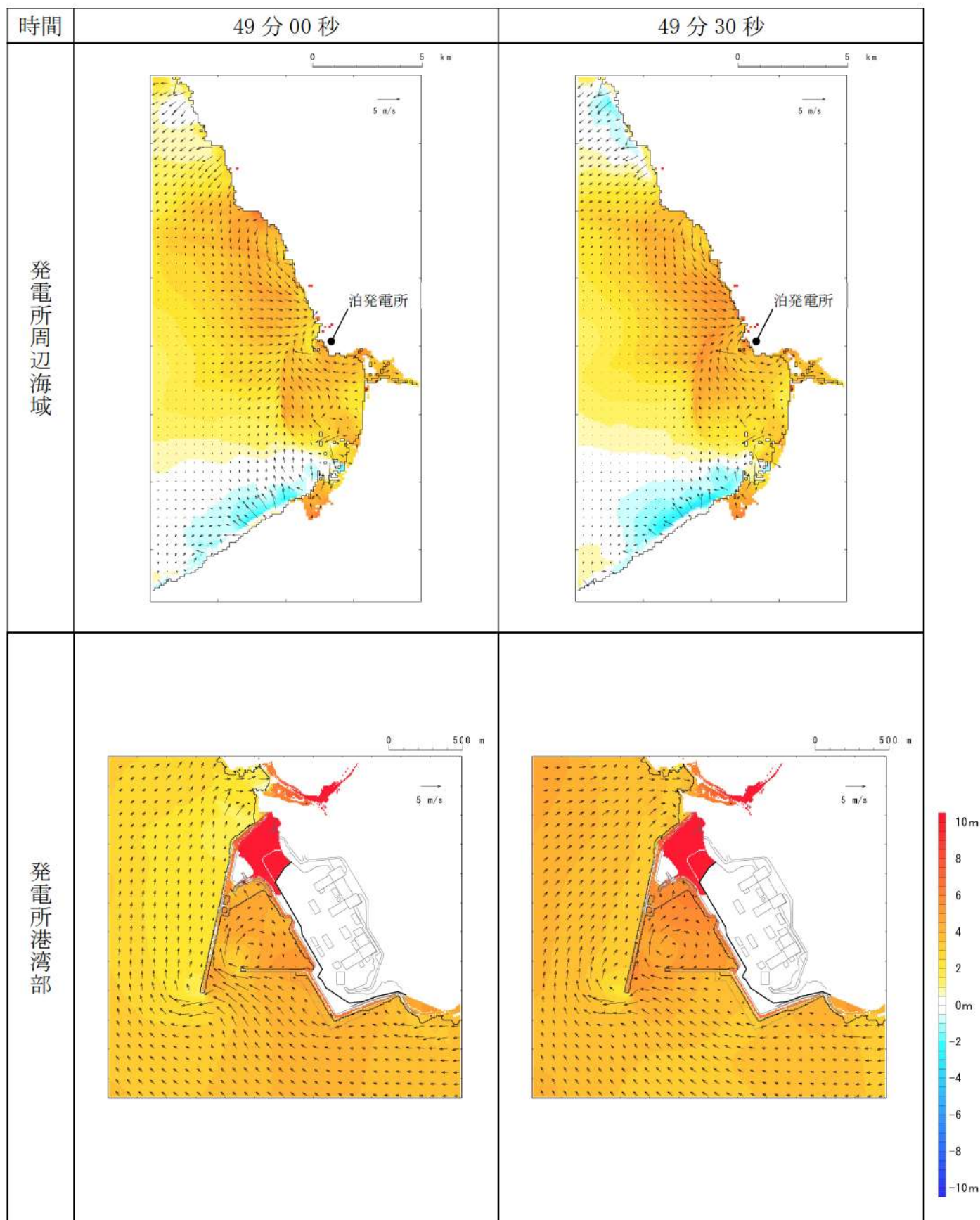
第 15 図-39 基準津波 I（防波堤損傷なし）の水位変動・流向ベクトル(39/50)
