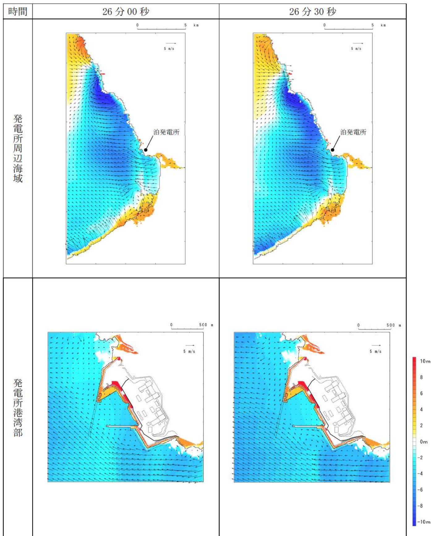
第 18 図-19 基準津波 L（北防波堤損傷）の水位変動・流向ベクトル(19/53)
