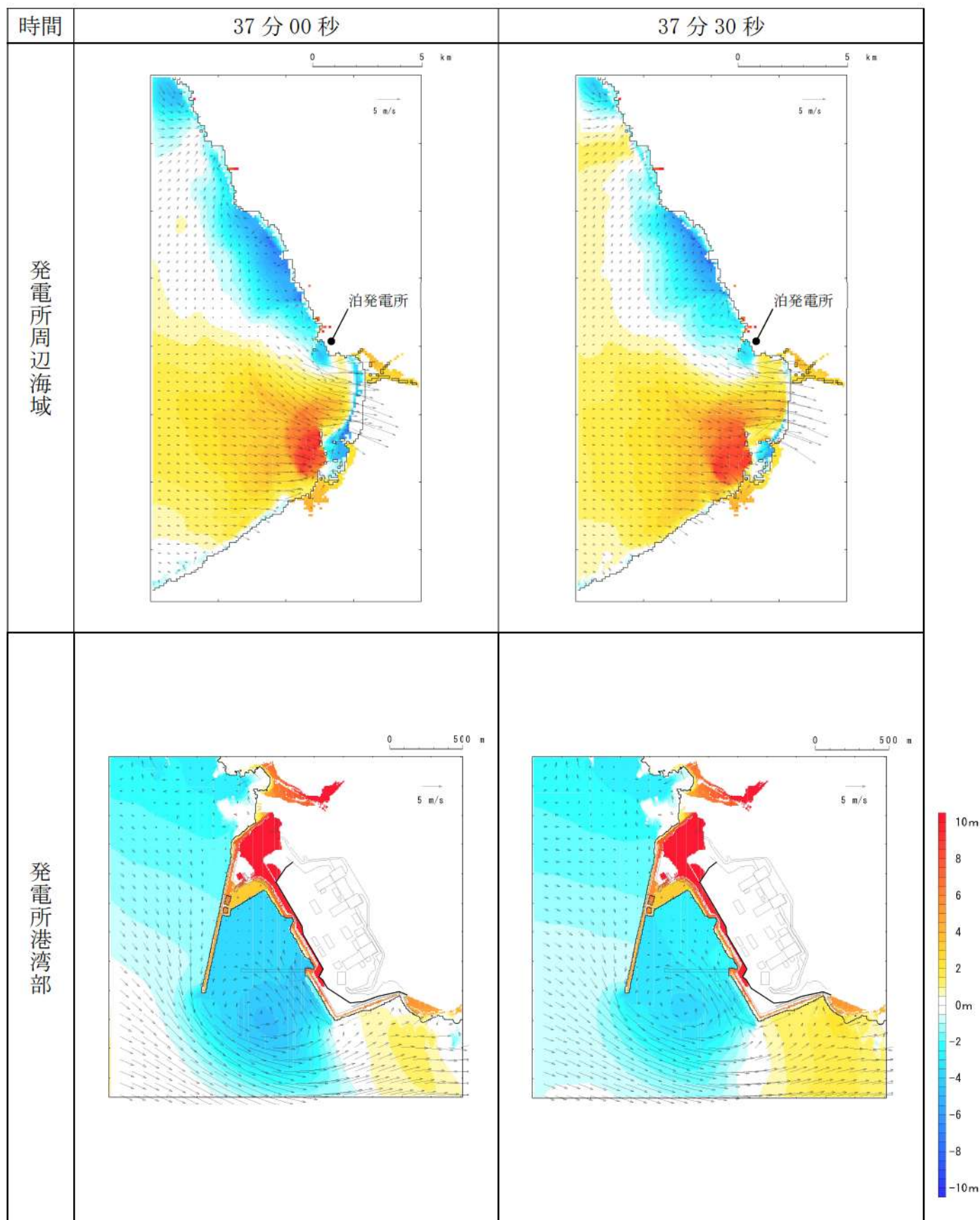
第 17 図-30 基準津波K（南防波堤損傷）の水位変動・流向ベクトル(30/53)
