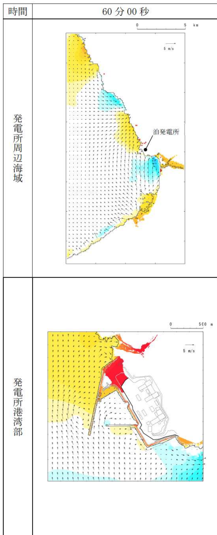
第 15 図-50 基準津波 I（防波堤損傷なし）の水位変動・流向ベクトル(50/50)
