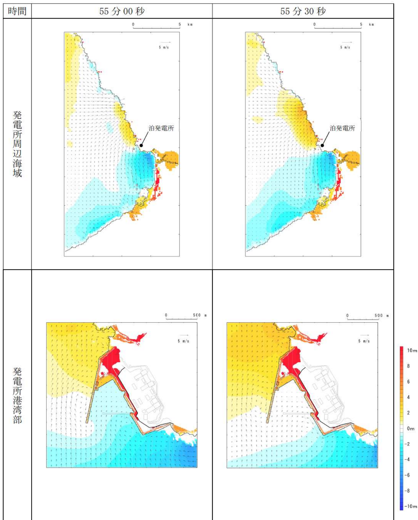
第 17 図-48 基準津波K（南防波堤損傷）の水位変動・流向ベクトル(48/53)
