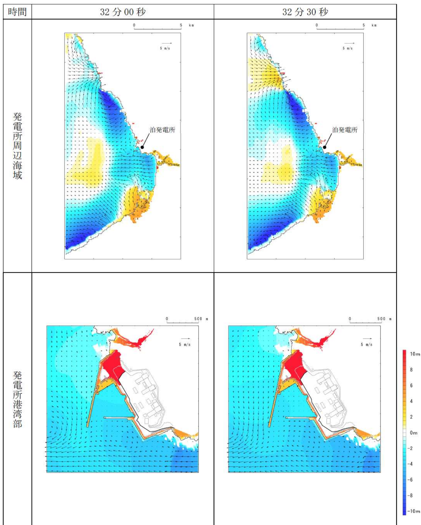
第 15 図-22 基準津波 I（防波堤損傷なし）の水位変動・流向ベクトル(22/50)
