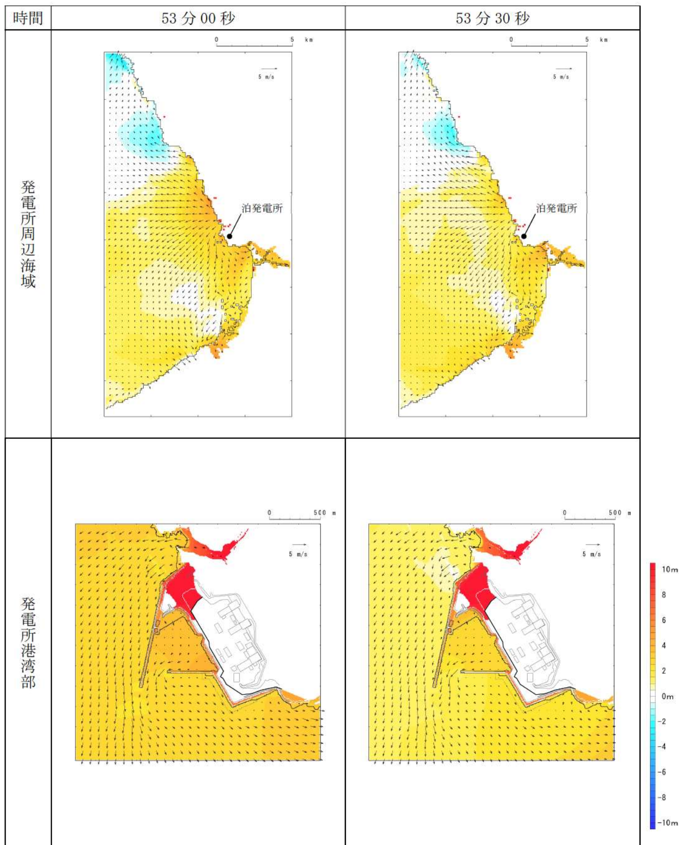
第 15 図-43 基準津波 I（防波堤損傷なし）の水位変動・流向ベクトル(43/50)
