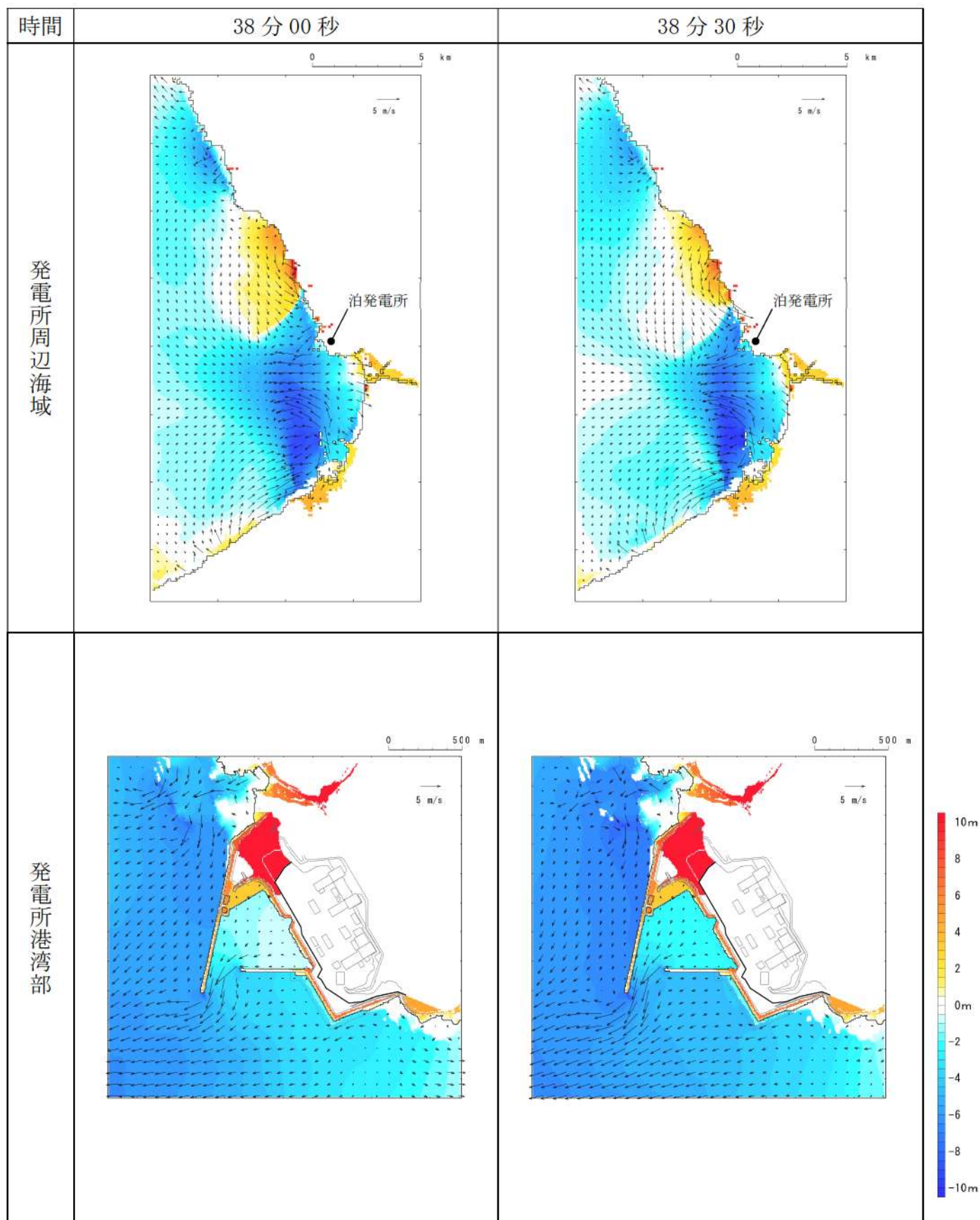
第 15 図-28 基準津波 I（防波堤損傷なし）の水位変動・流向ベクトル(28/50)
