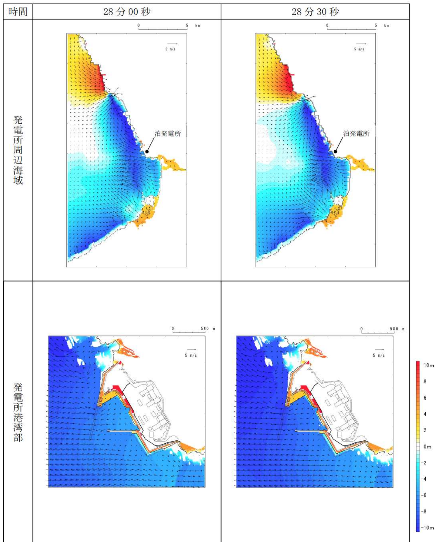
第 18 図-21 基準津波 L（北防波堤損傷）の水位変動・流向ベクトル(21/53)
