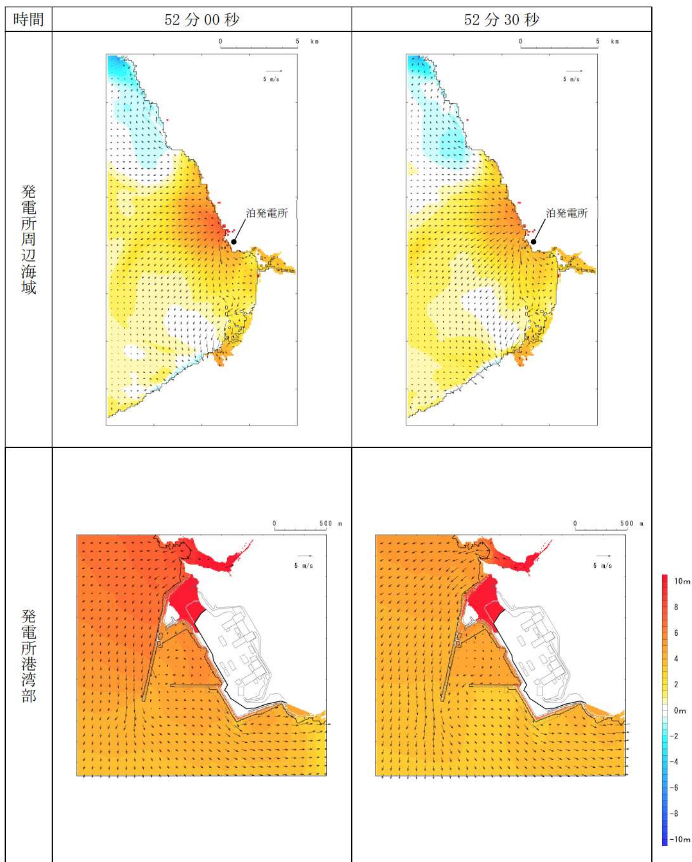
第 15 図-42 基準津波 I（防波堤損傷なし）の水位変動・流向ベクトル(42/50)
