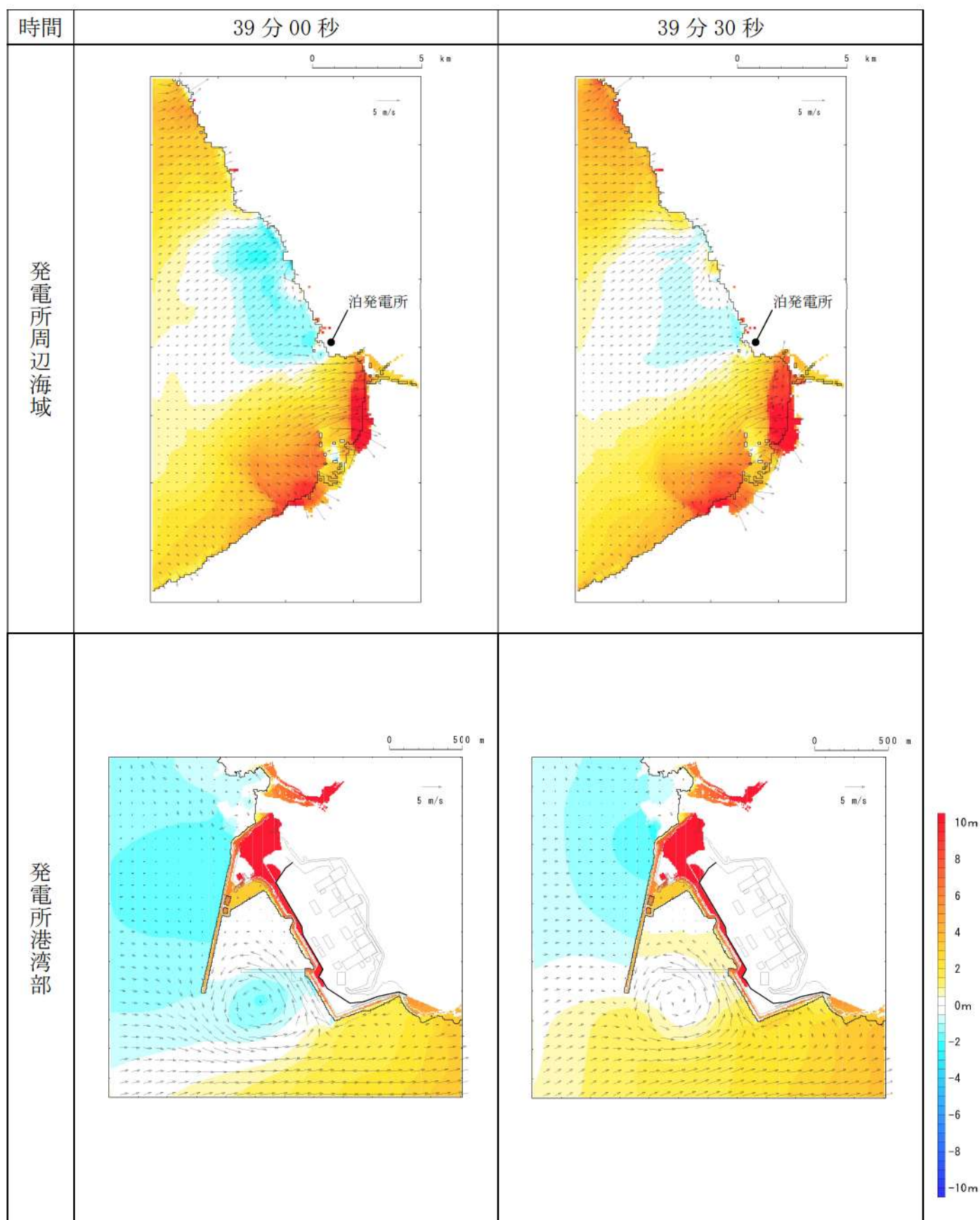
第 17 図-32 基準津波K（南防波堤損傷）の水位変動・流向ベクトル(32/53)
