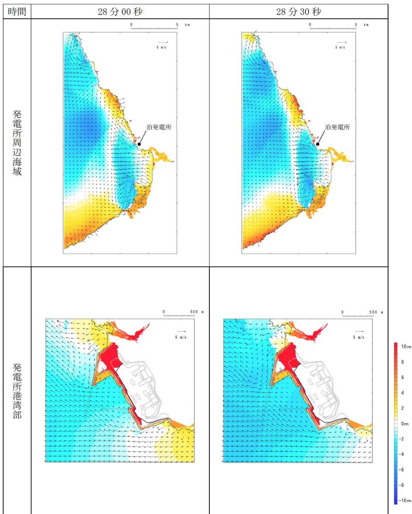
第 16 図-17 基準津波 J（北及び南防波堤損傷）の水位変動・流向ベクトル(17/49)
