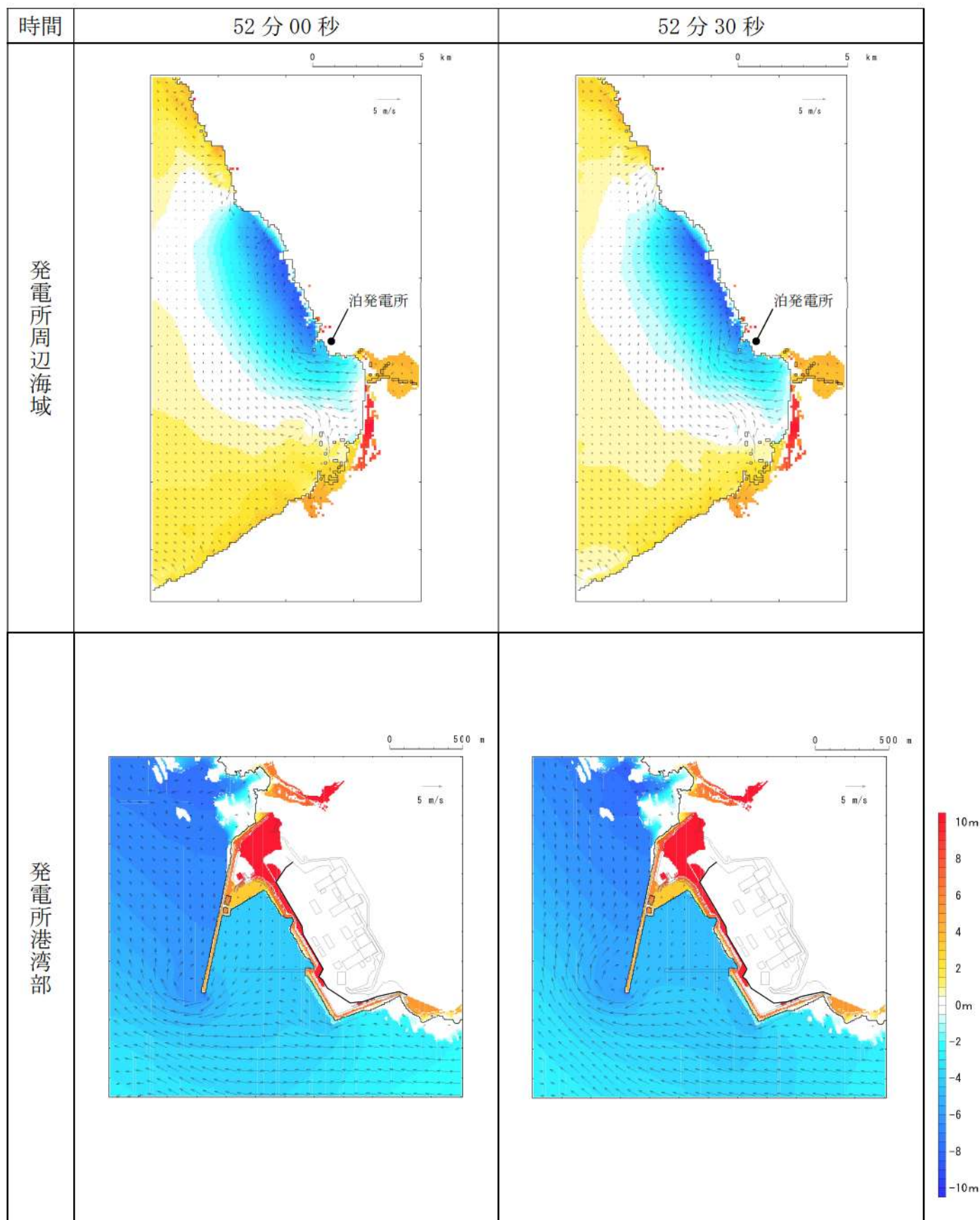
第 17 図-45 基準津波K（南防波堤損傷）の水位変動・流向ベクトル(45/53)
