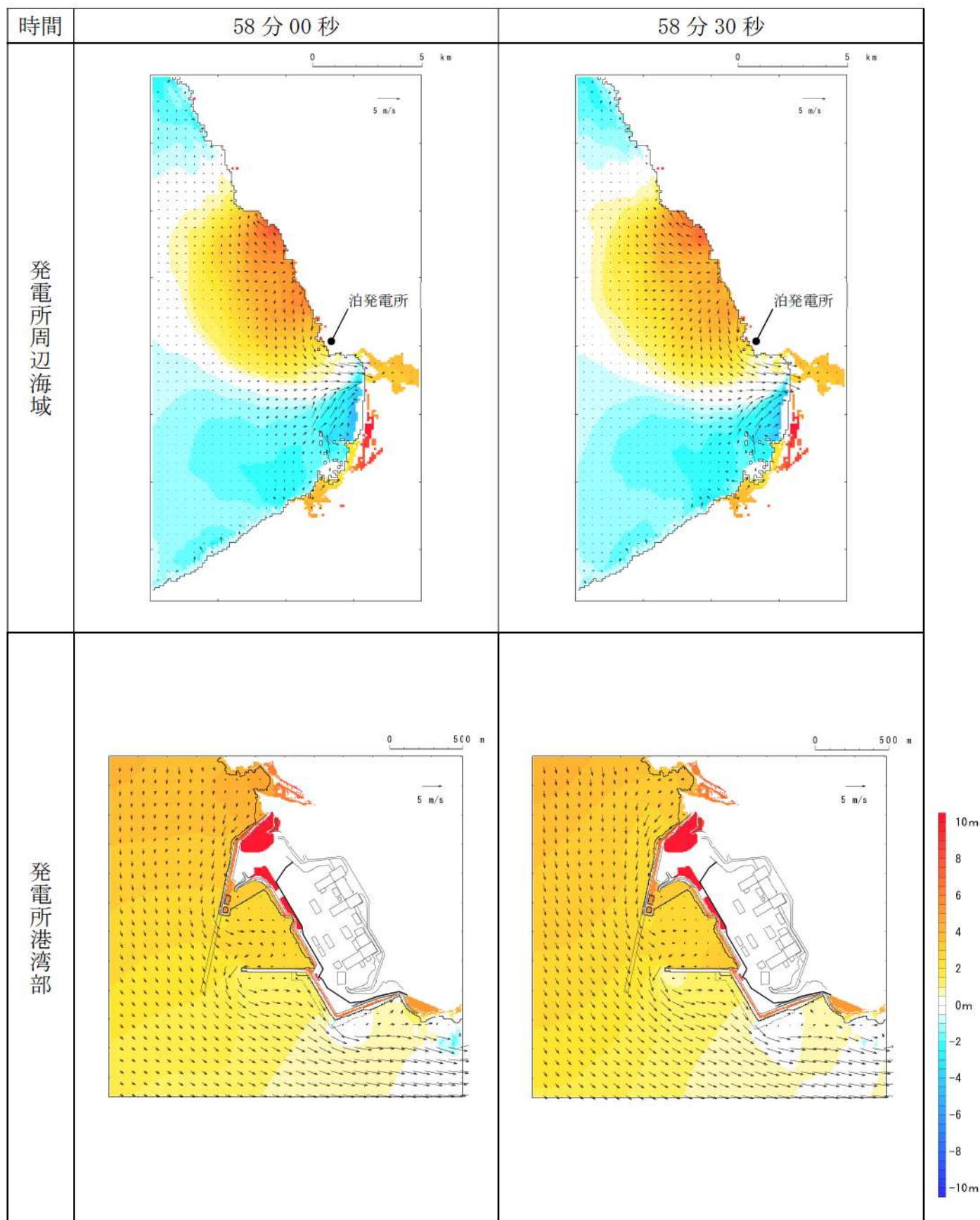
第 18 図-51 基準津波 L（北防波堤損傷）の水位変動・流向ベクトル (51/53)
