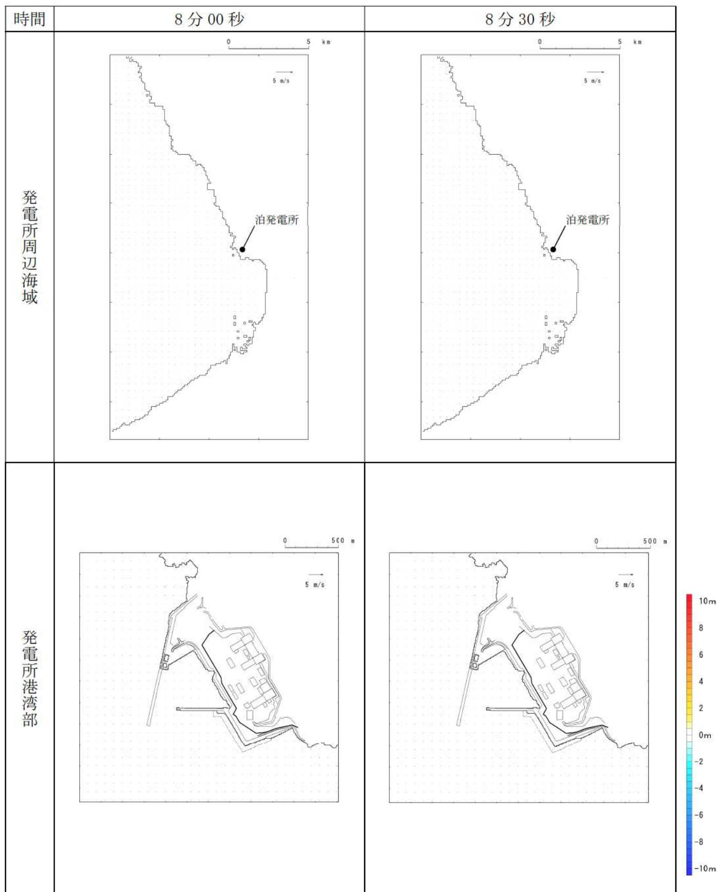
第 18 図-1 基準津波 L（北防波堤損傷）の水位変動・流向ベクトル(1/53)
