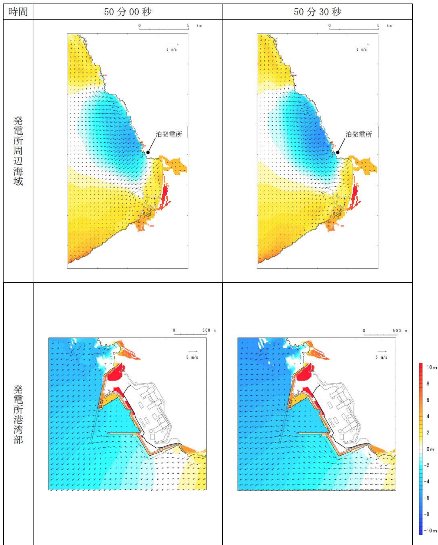
第 18 図-43 基準津波 L（北防波堤損傷）の水位変動・流向ベクトル(43/53)
