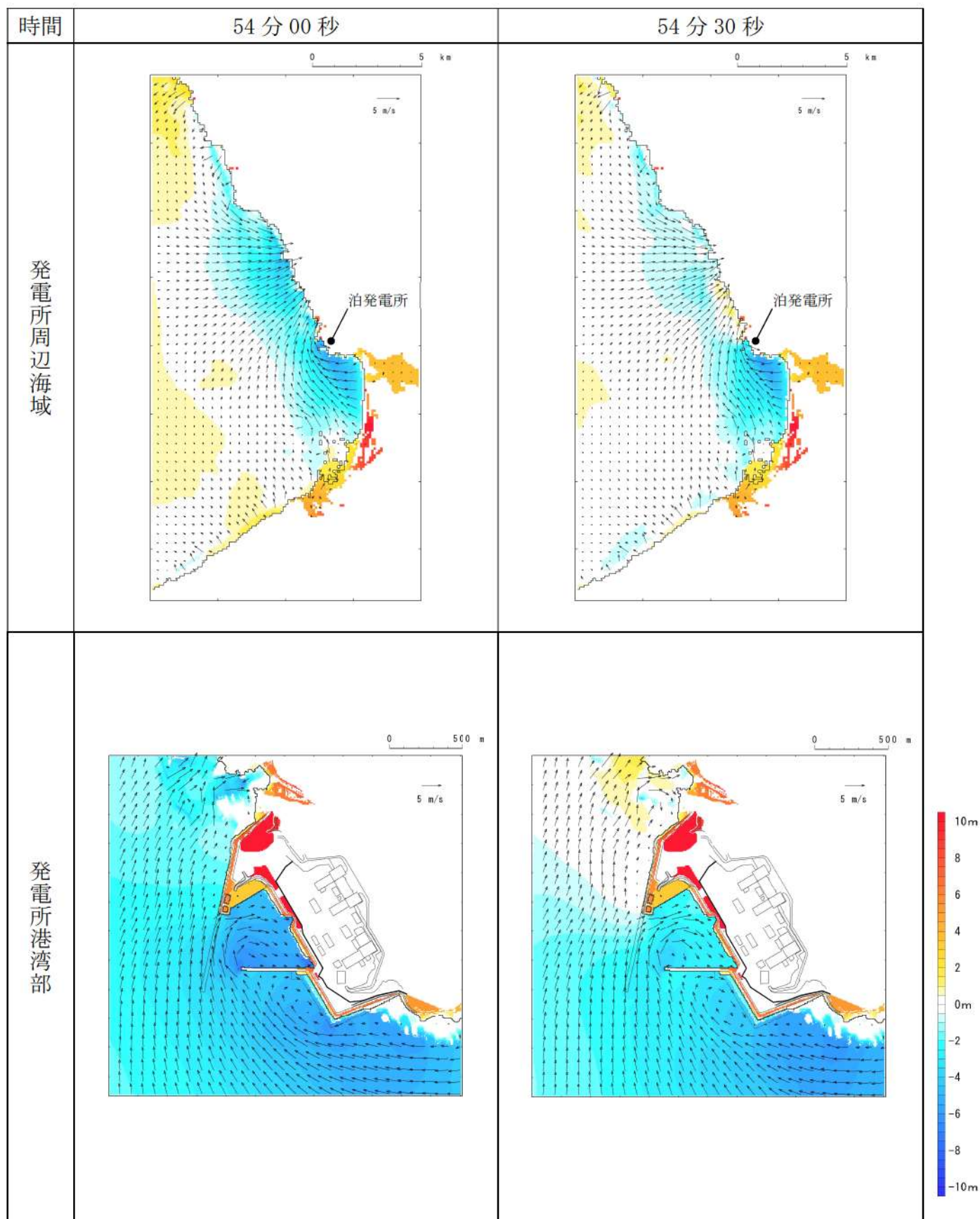
第 18 図-47 基準津波 L（北防波堤損傷）の水位変動・流向ベクトル(47/53)
