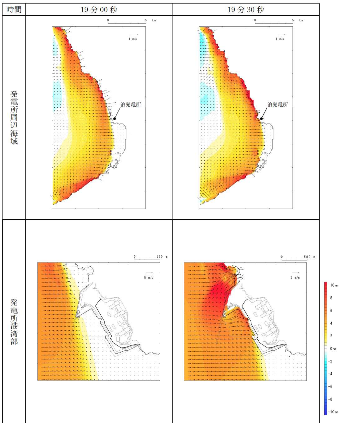
第 16 図-8 基準津波 J（北及び南防波堤損傷）の水位変動・流向ベクトル(8/49)
