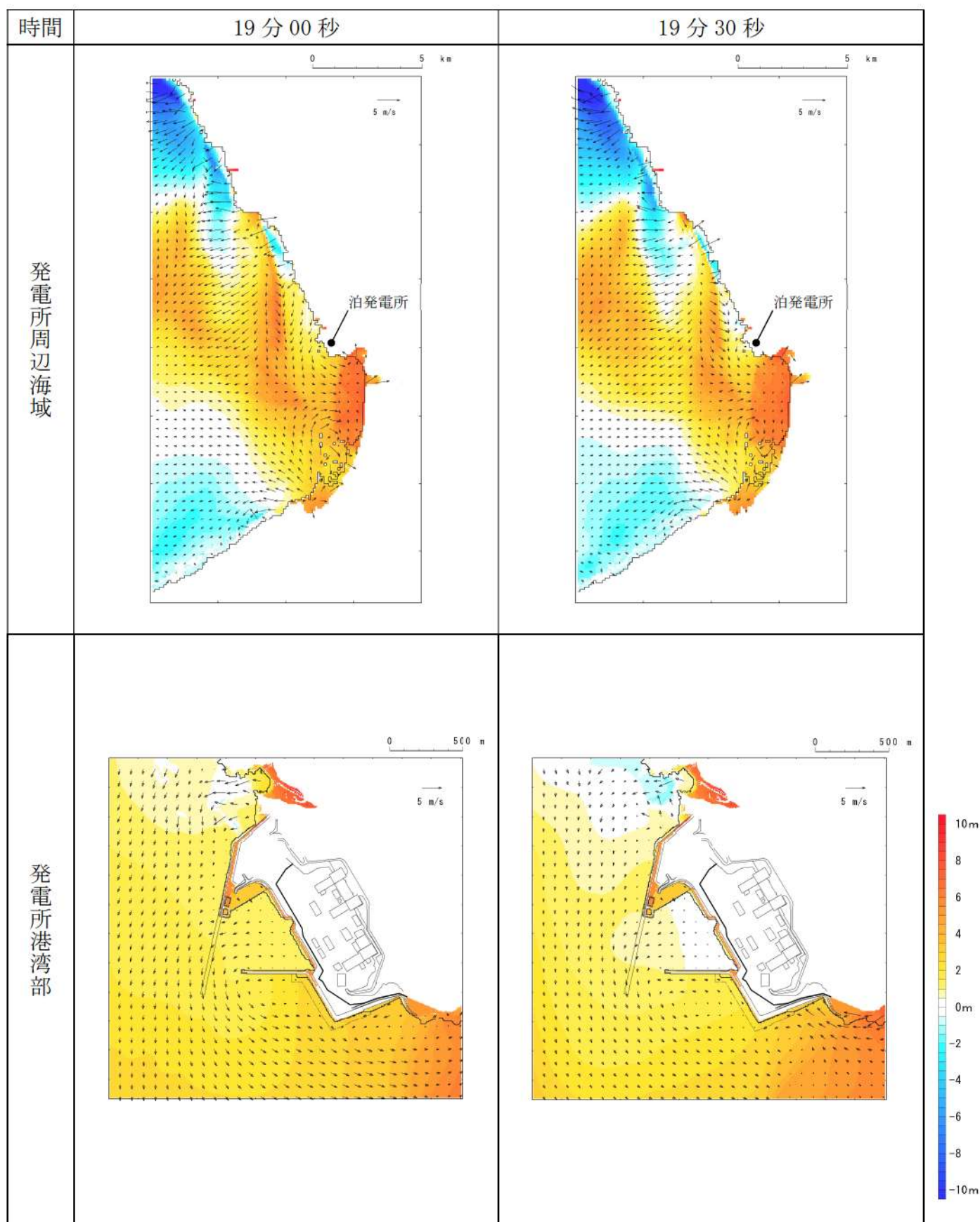
第 18 図-12 基準津波 L（北防波堤損傷）の水位変動・流向ベクトル(12/53)
