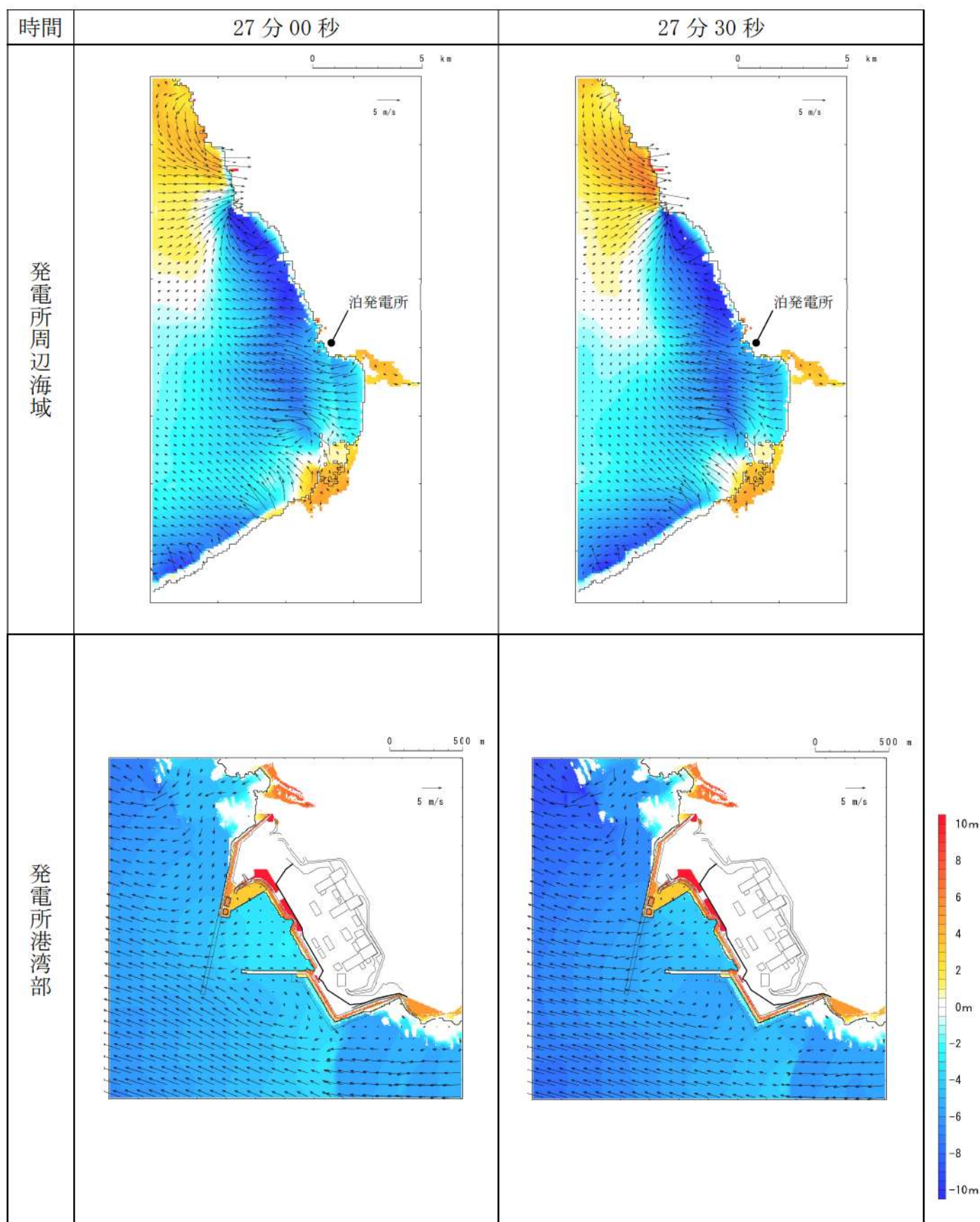
第 18 図-20 基準津波 L（北防波堤損傷）の水位変動・流向ベクトル (20/53)
