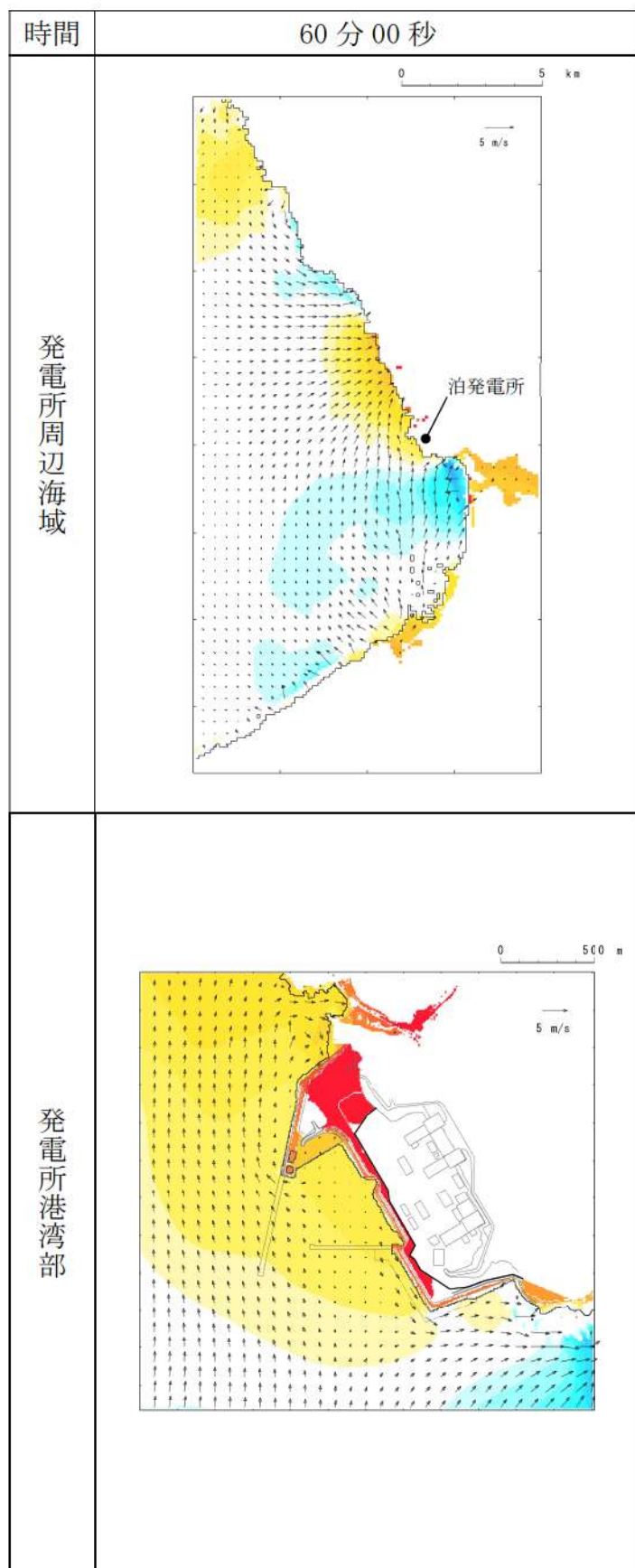
第 16 図-49 基準津波 J（北及び南防波堤損傷）の水位変動・流向ベクトル(49/49)
