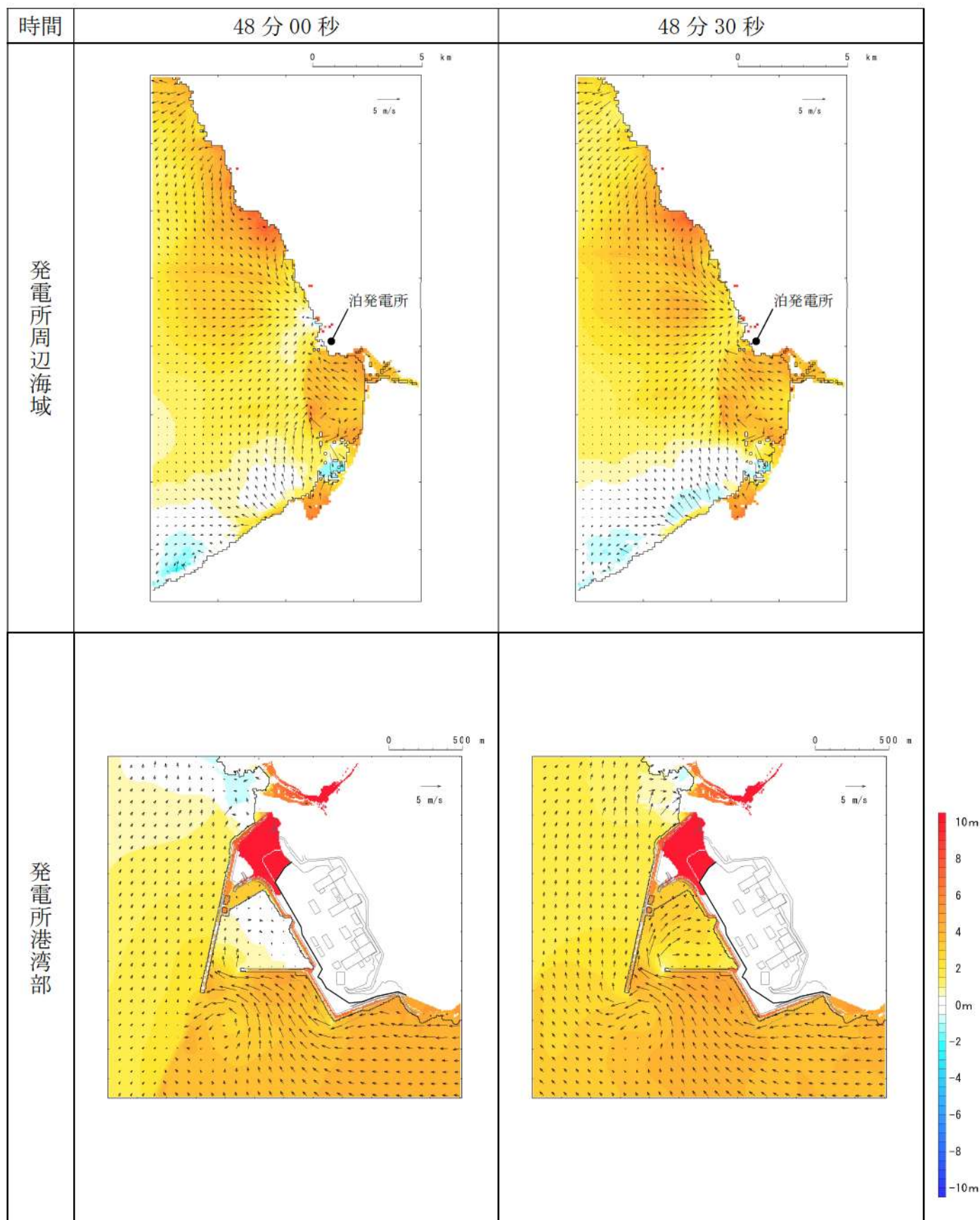
第 15 図-38 基準津波 I（防波堤損傷なし）の水位変動・流向ベクトル(38/50)
