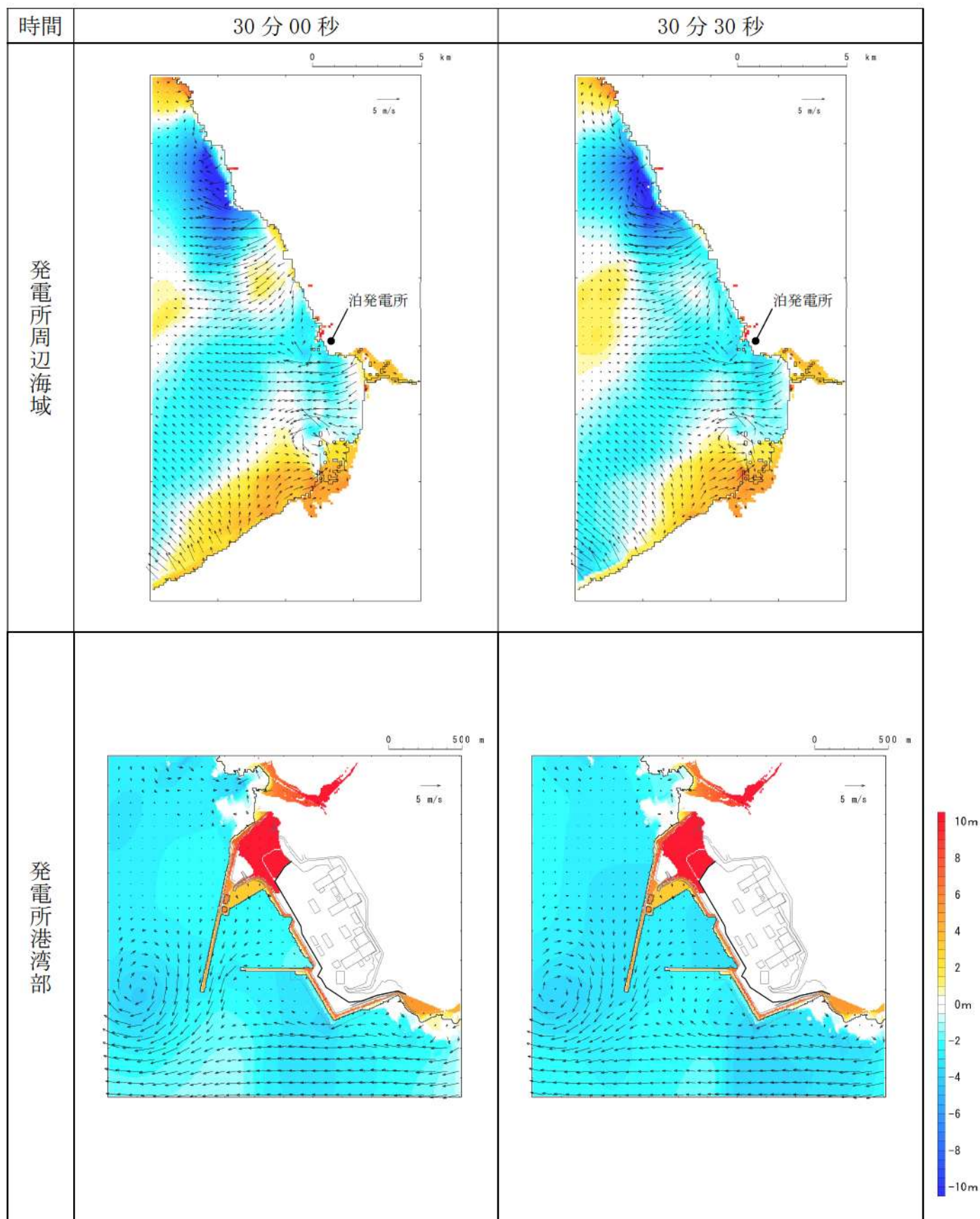
第 15 図-20 基準津波 I（防波堤損傷なし）の水位変動・流向ベクトル(20/50)
