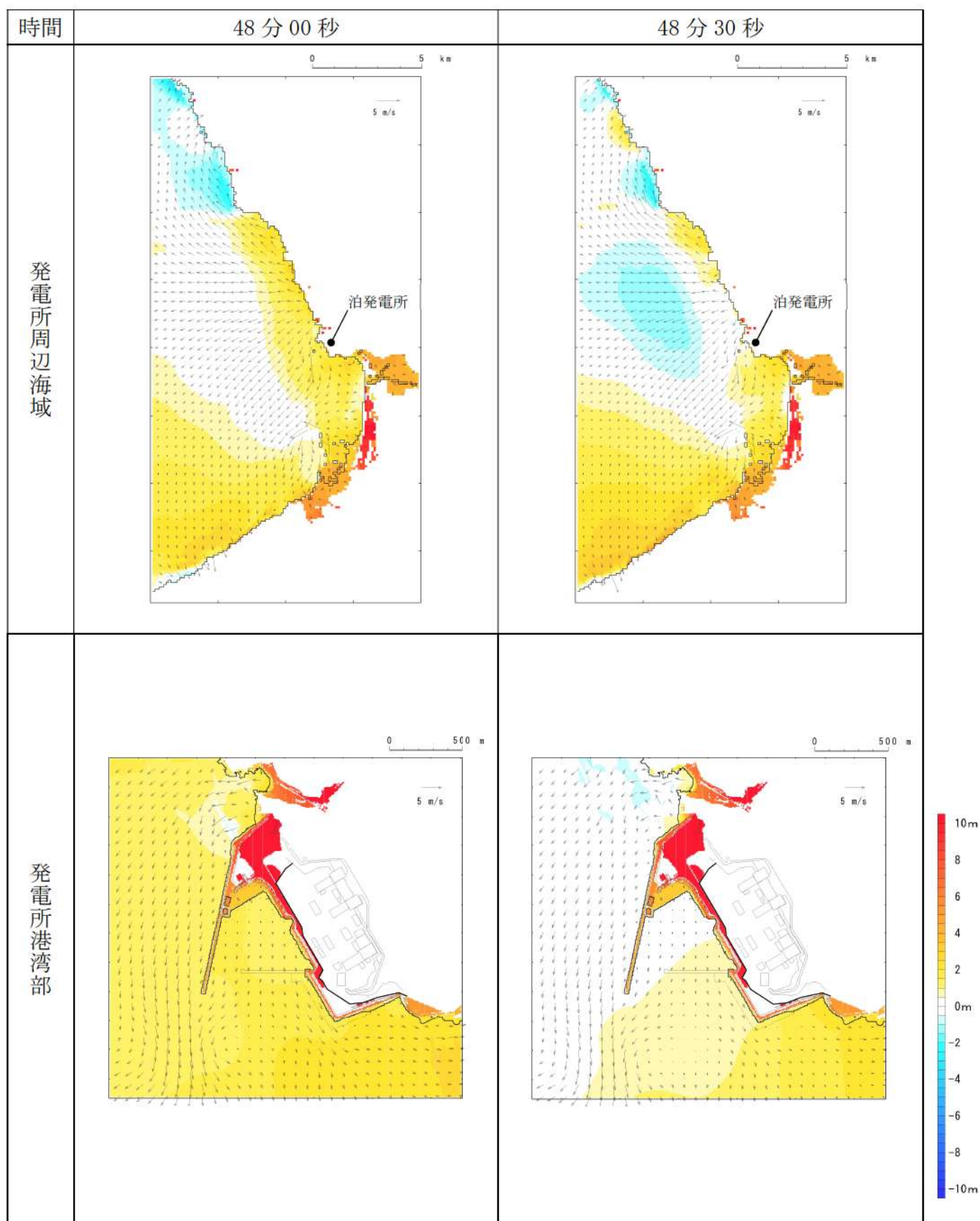
第 17 図-41 基準津波K（南防波堤損傷）の水位変動・流向ベクトル(41/53)
