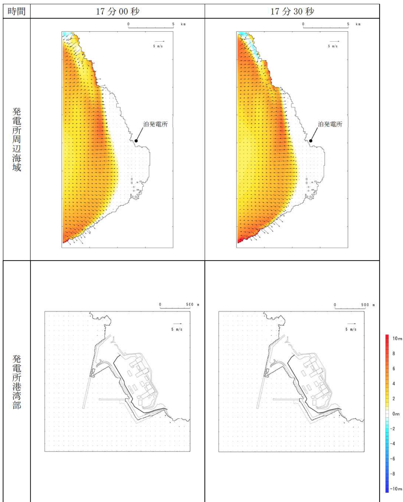
第 16 図-6 基準津波 J（北及び南防波堤損傷）の水位変動・流向ベクトル (6/49)
