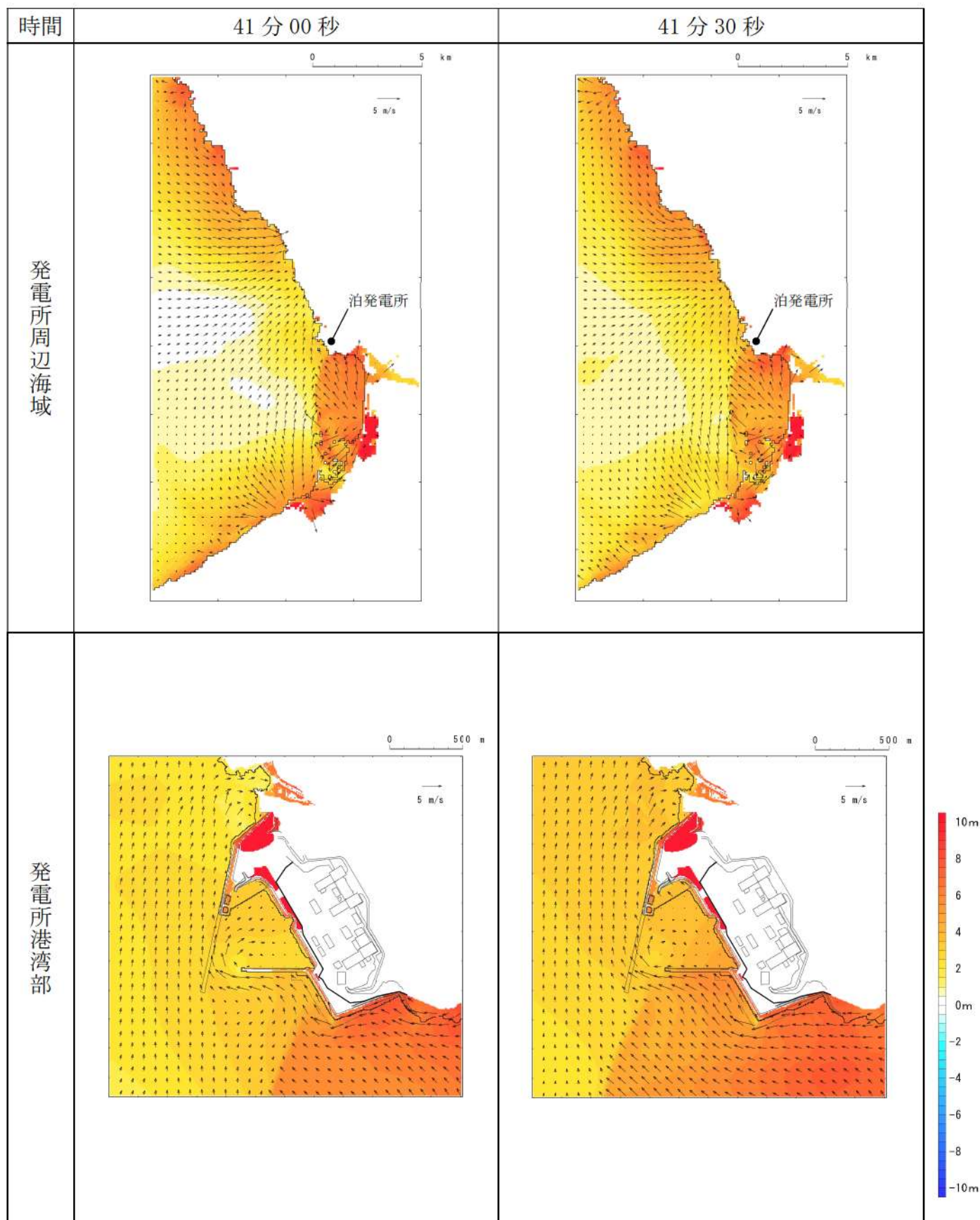
第 18 図-34 基準津波 L（北防波堤損傷）の水位変動・流向ベクトル(34/53)
