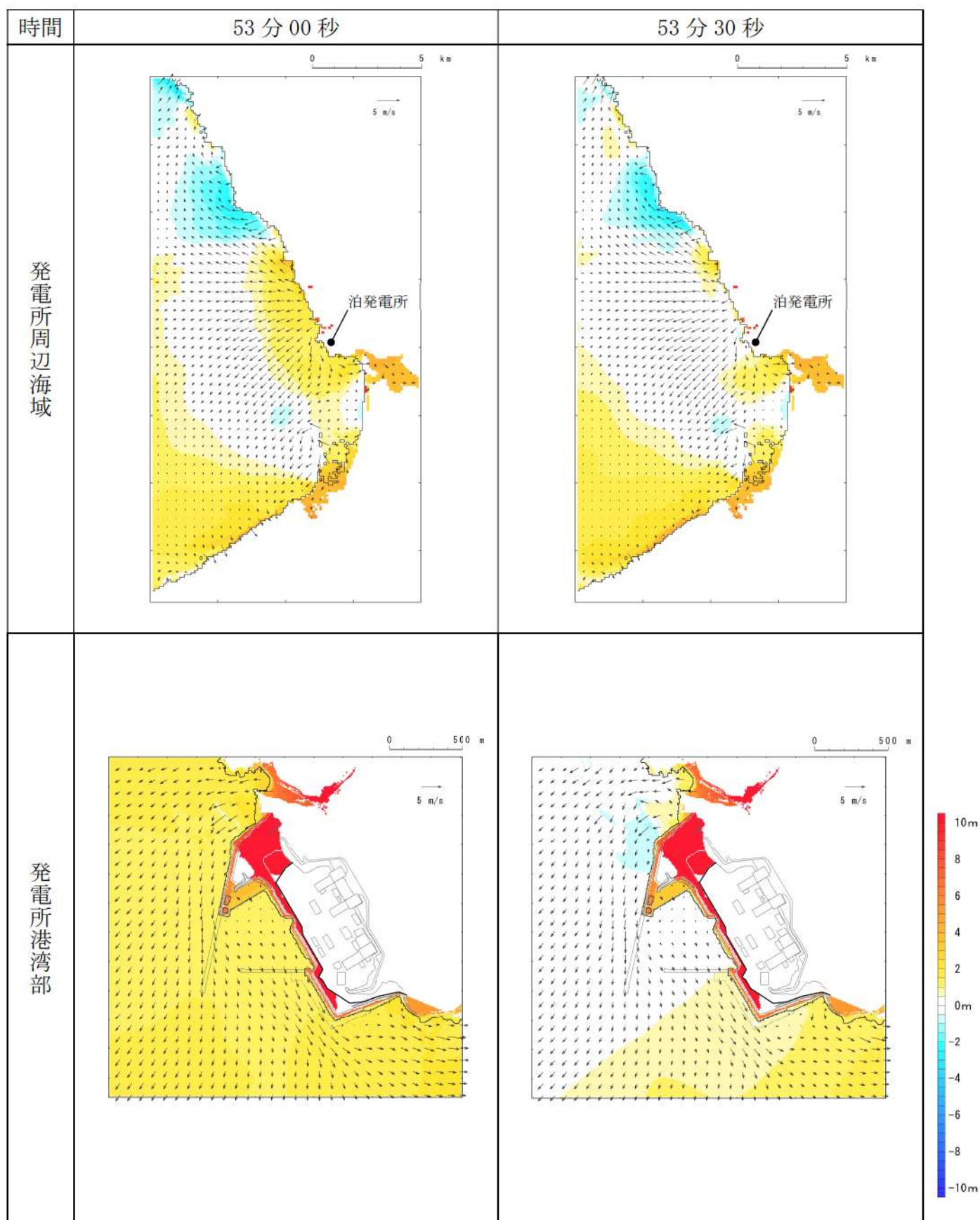
第 16 図-42 基準津波 J（北及び南防波堤損傷）の水位変動・流向ベクトル(42/49)
