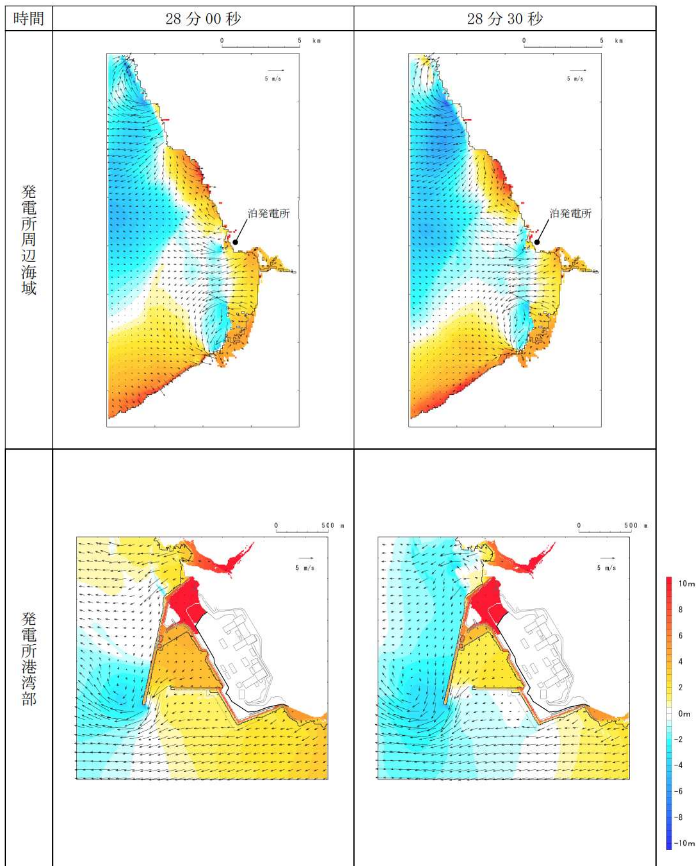
第 15 図-18 基準津波 I（防波堤損傷なし）の水位変動・流向ベクトル(18/50)
