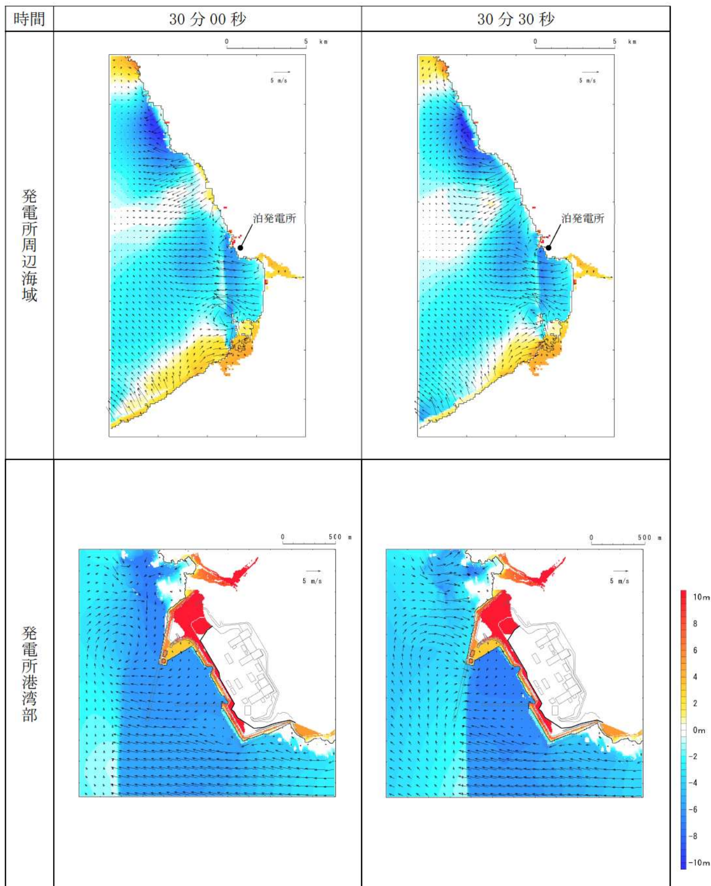
第 16 図-19 基準津波 J（北及び南防波堤損傷）の水位変動・流向ベクトル(19/49)
