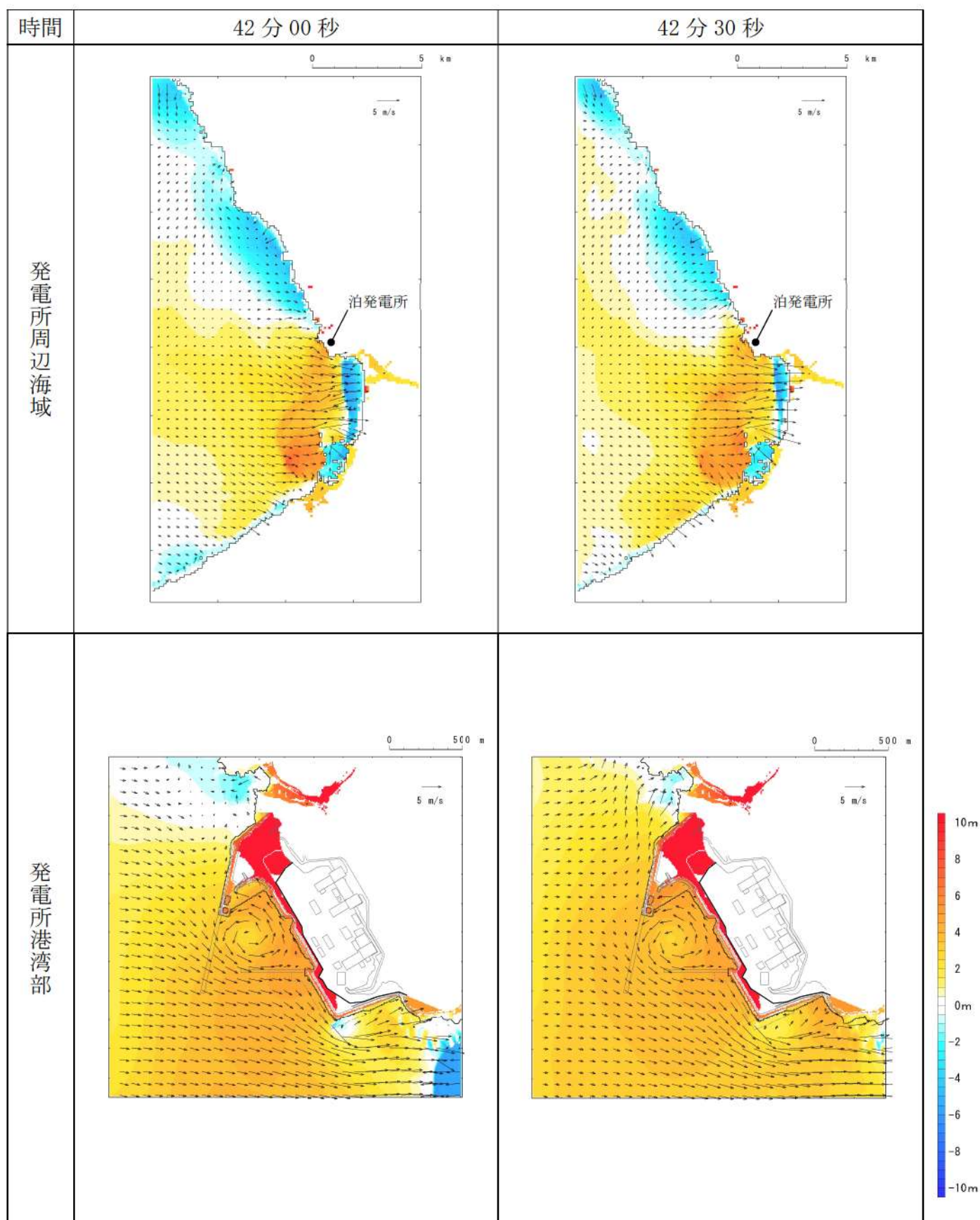
第 16 図-31 基準津波 J（北及び南防波堤損傷）の水位変動・流向ベクトル(31/49)
