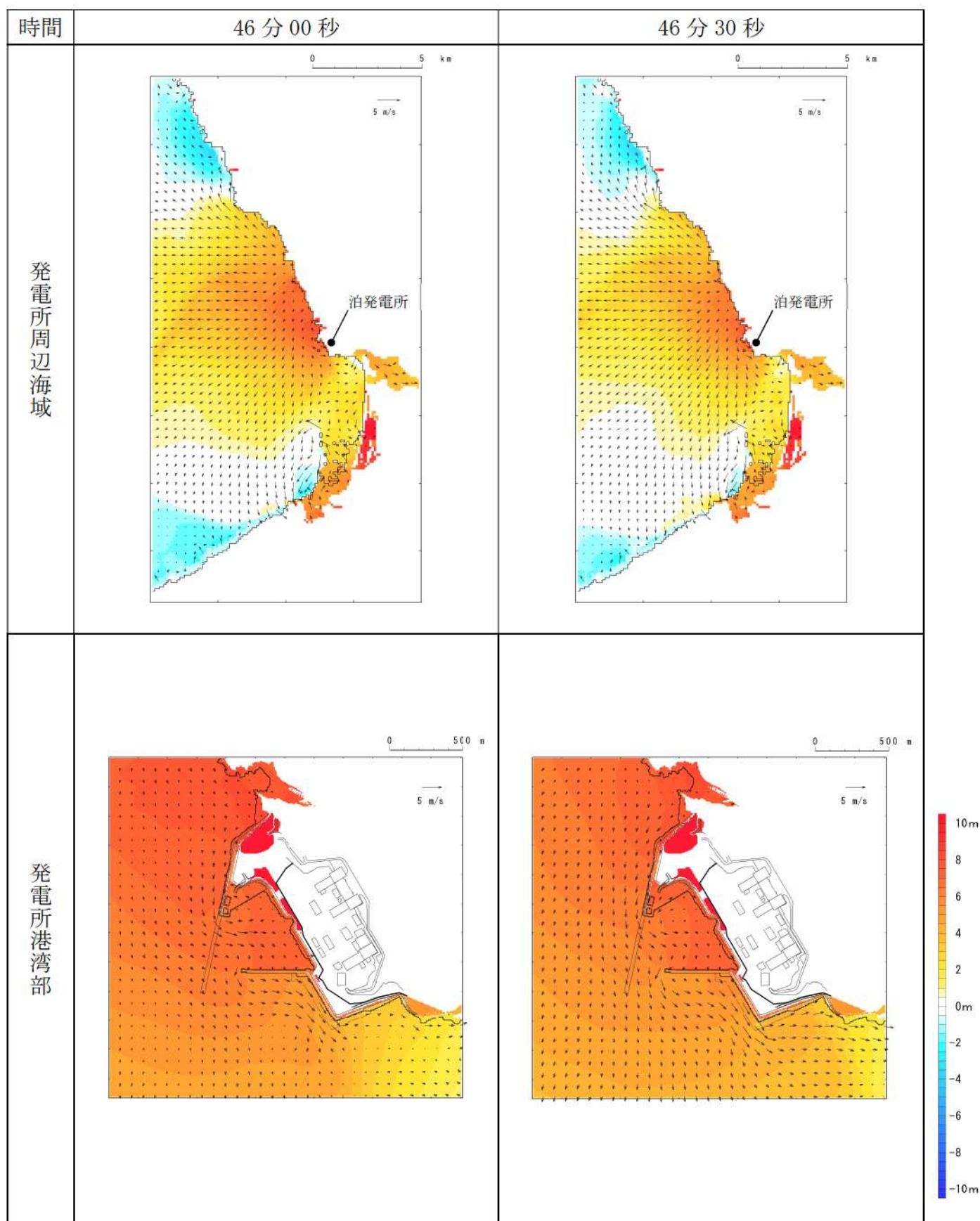
第 18 図-39 基準津波 L（北防波堤損傷）の水位変動・流向ベクトル(39/53)
