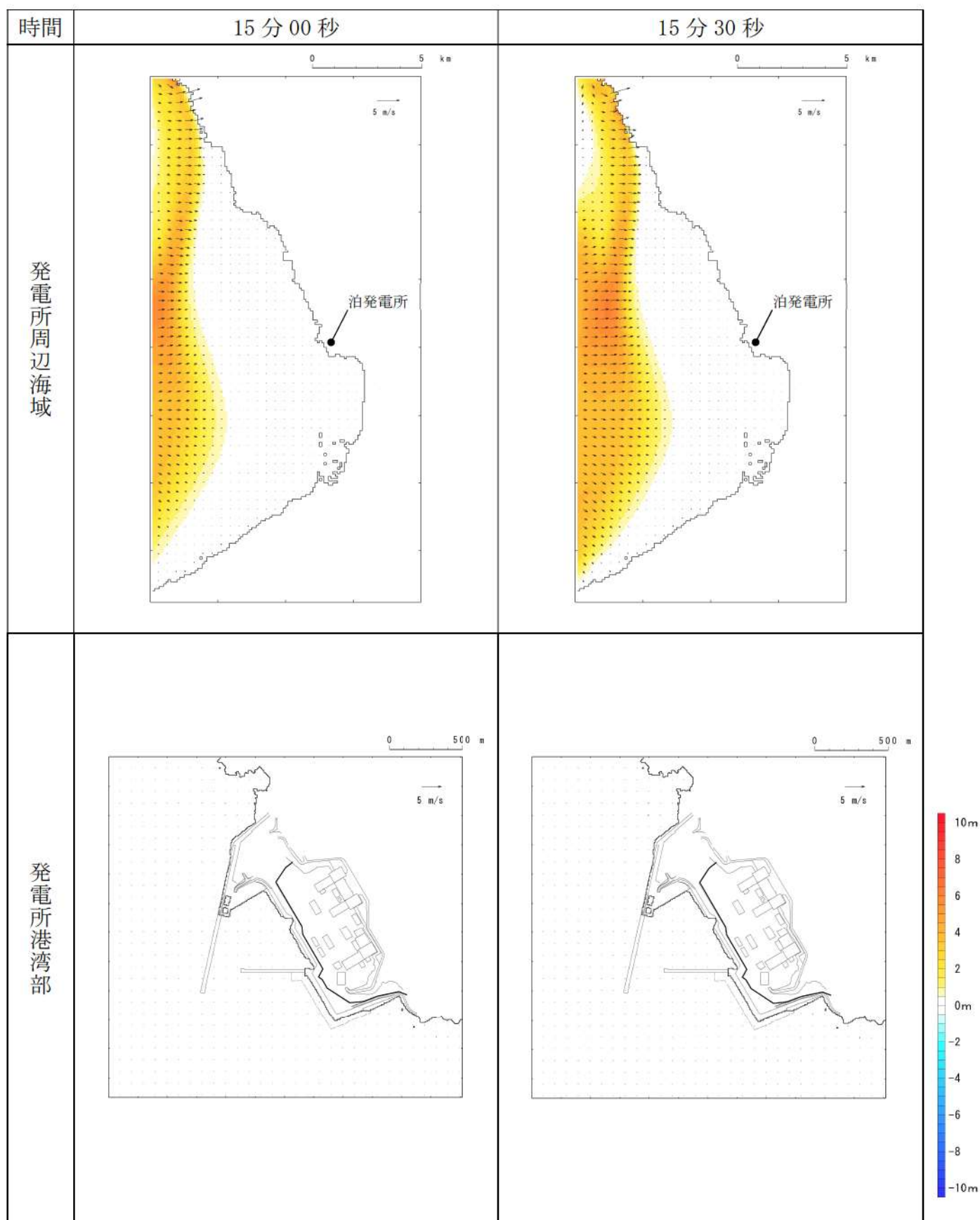
第 16 図-4 基準津波 J（北及び南防波堤損傷）の水位変動・流向ベクトル(4/49)
