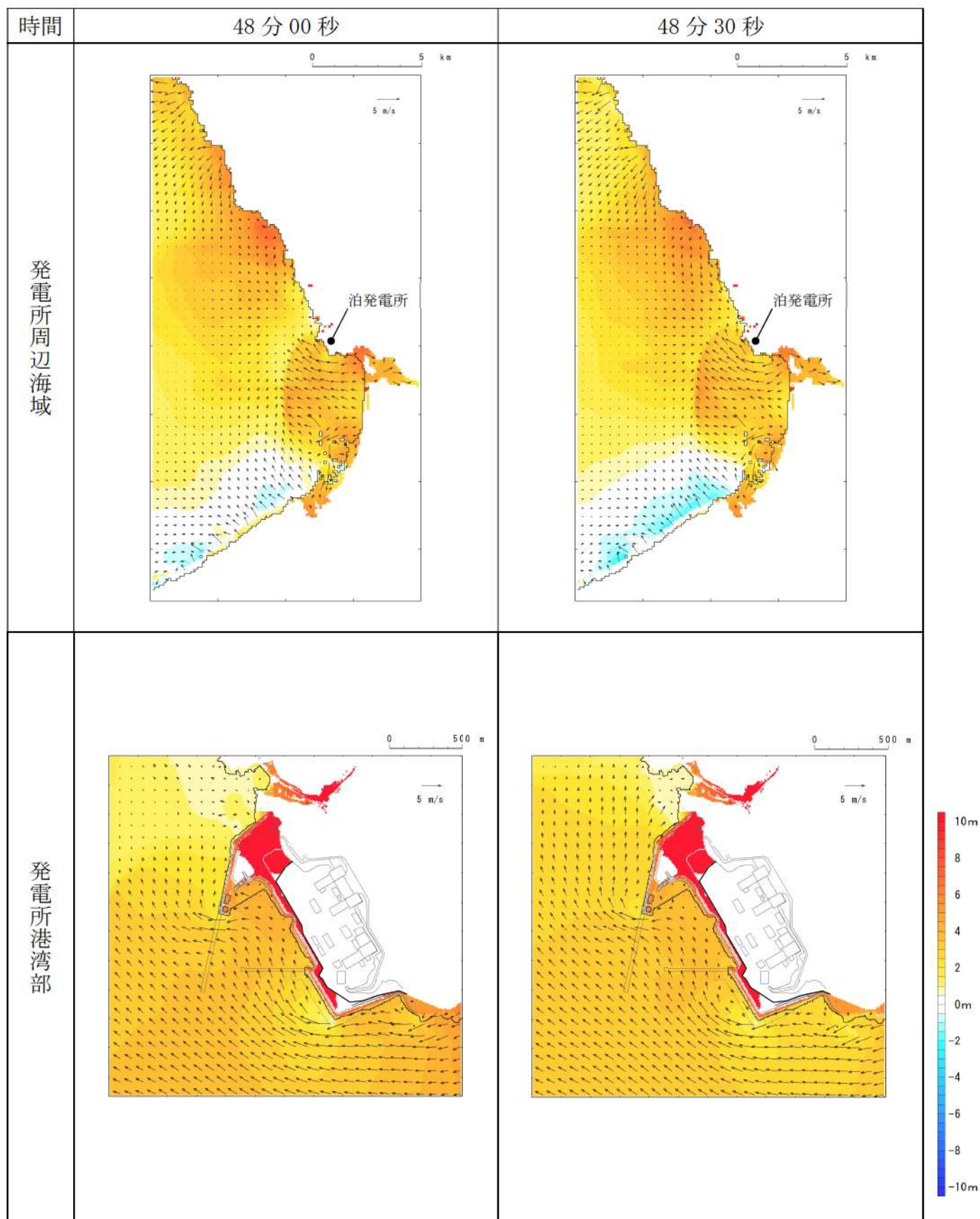
第 16 図-37 基準津波 J（北及び南防波堤損傷）の水位変動・流向ベクトル(37/49)
