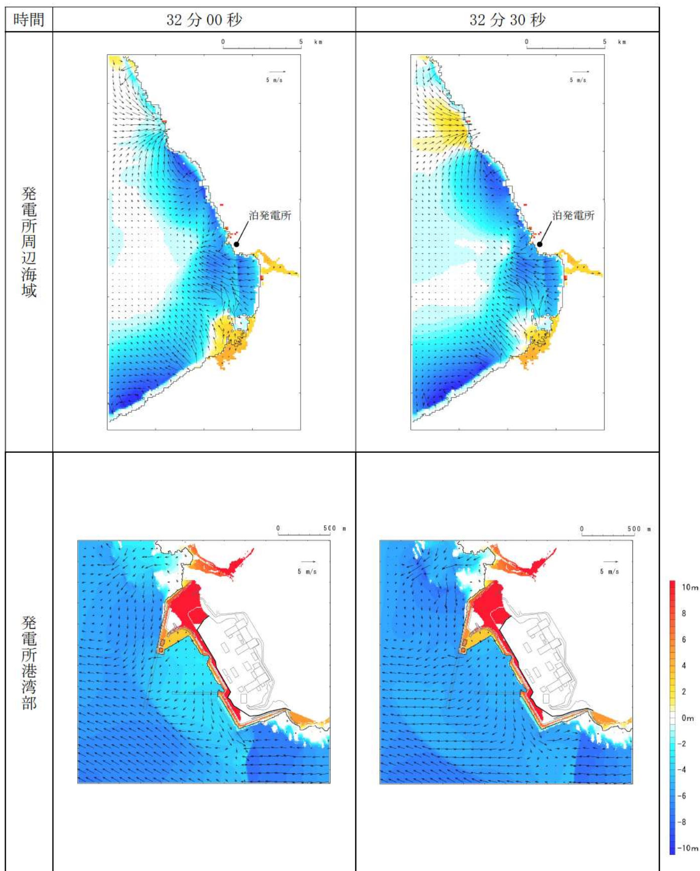
第 16 図-21 基準津波 J（北及び南防波堤損傷）の水位変動・流向ベクトル(21/49)
