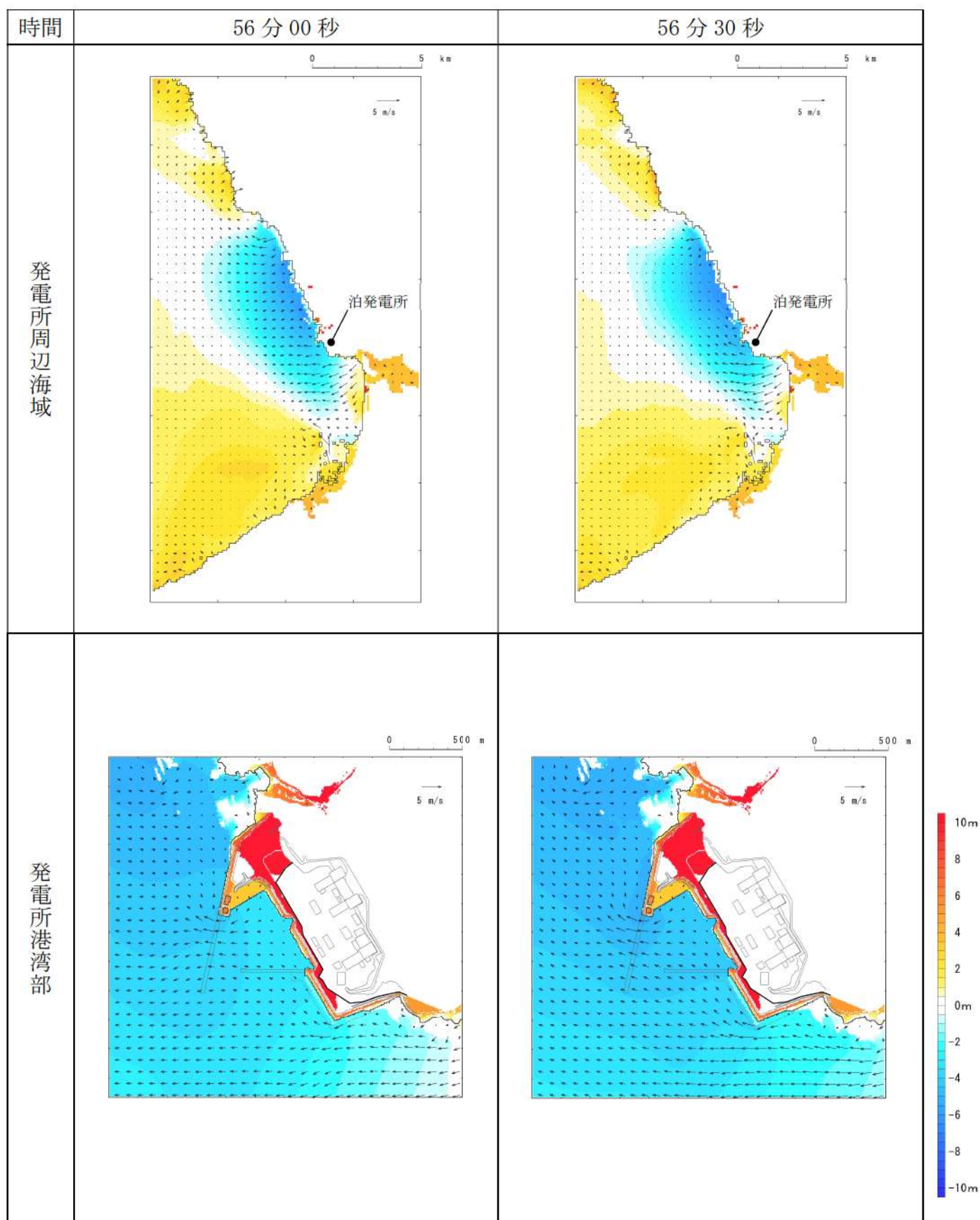
第 16 図-45 基準津波 J（北及び南防波堤損傷）の水位変動・流向ベクトル(45/49)
