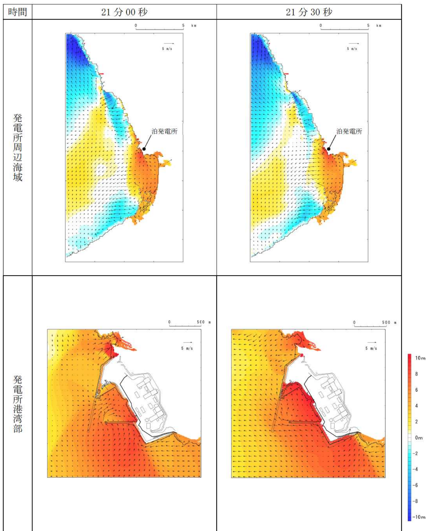
第 18 図-14 基準津波 L（北防波堤損傷）の水位変動・流向ベクトル(14/53)
