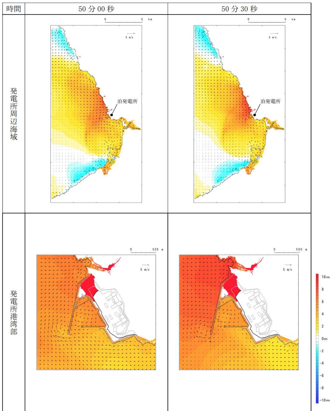
第 15 図-40 基準津波 I（防波堤損傷なし）の水位変動・流向ベクトル(40/50)
