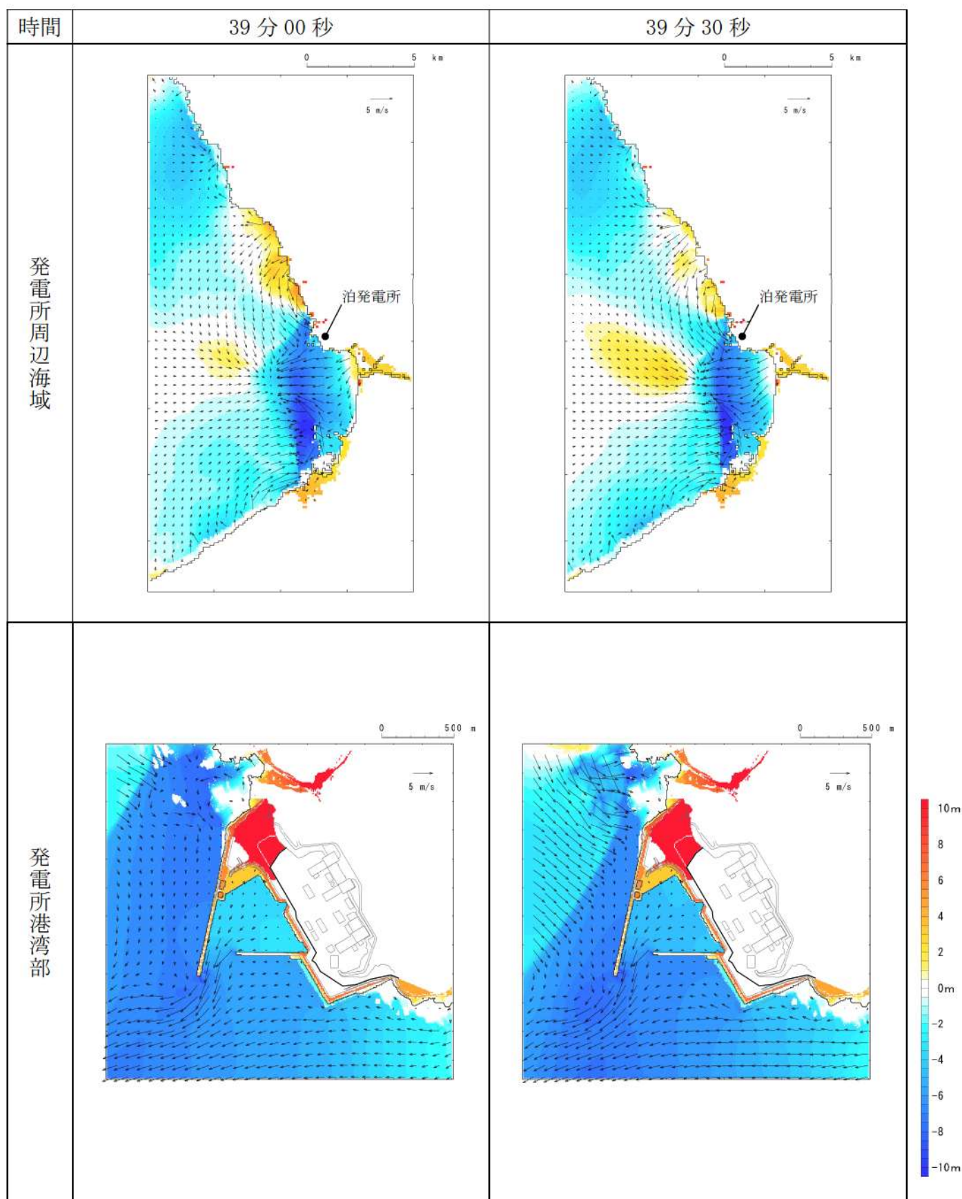
第 15 図-29 基準津波 I（防波堤損傷なし）の水位変動・流向ベクトル(29/50)
