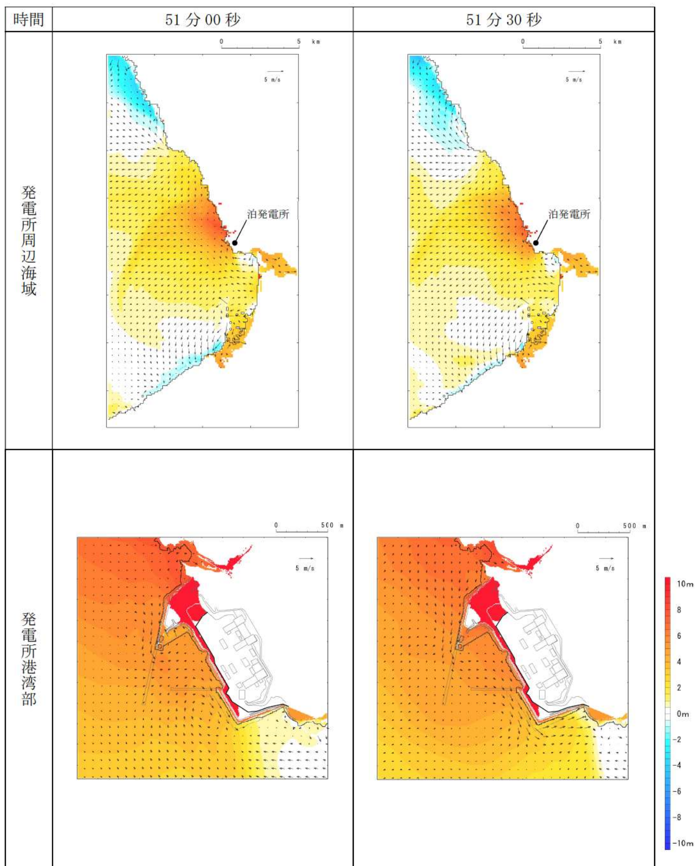
第 16 図-40 基準津波 J（北及び南防波堤損傷）の水位変動・流向ベクトル(40/49)
