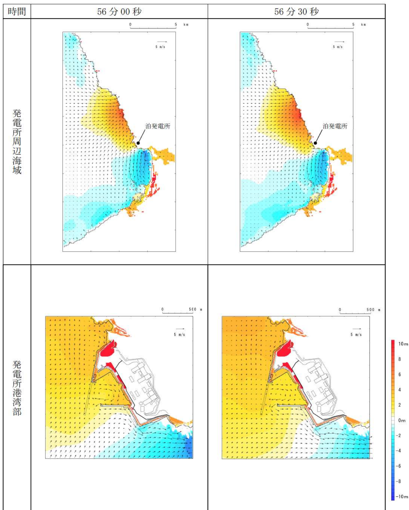
第 18 図-49 基準津波 L（北防波堤損傷）の水位変動・流向ベクトル(49/53)
