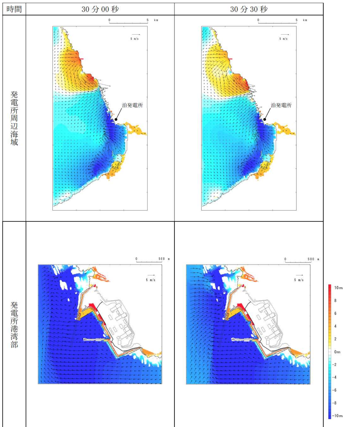
第 18 図-23 基準津波 L（北防波堤損傷）の水位変動・流向ベクトル (23/53)
