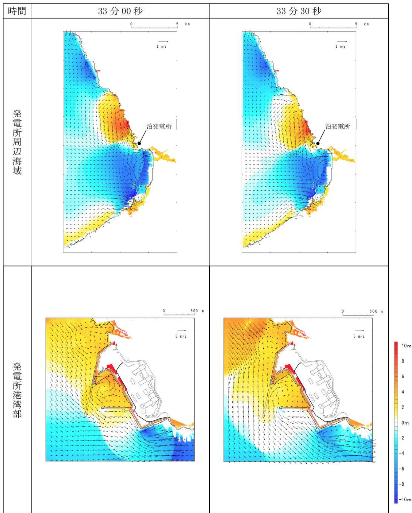
第 18 図-26 基準津波 L（北防波堤損傷）の水位変動・流向ベクトル (26/53)
