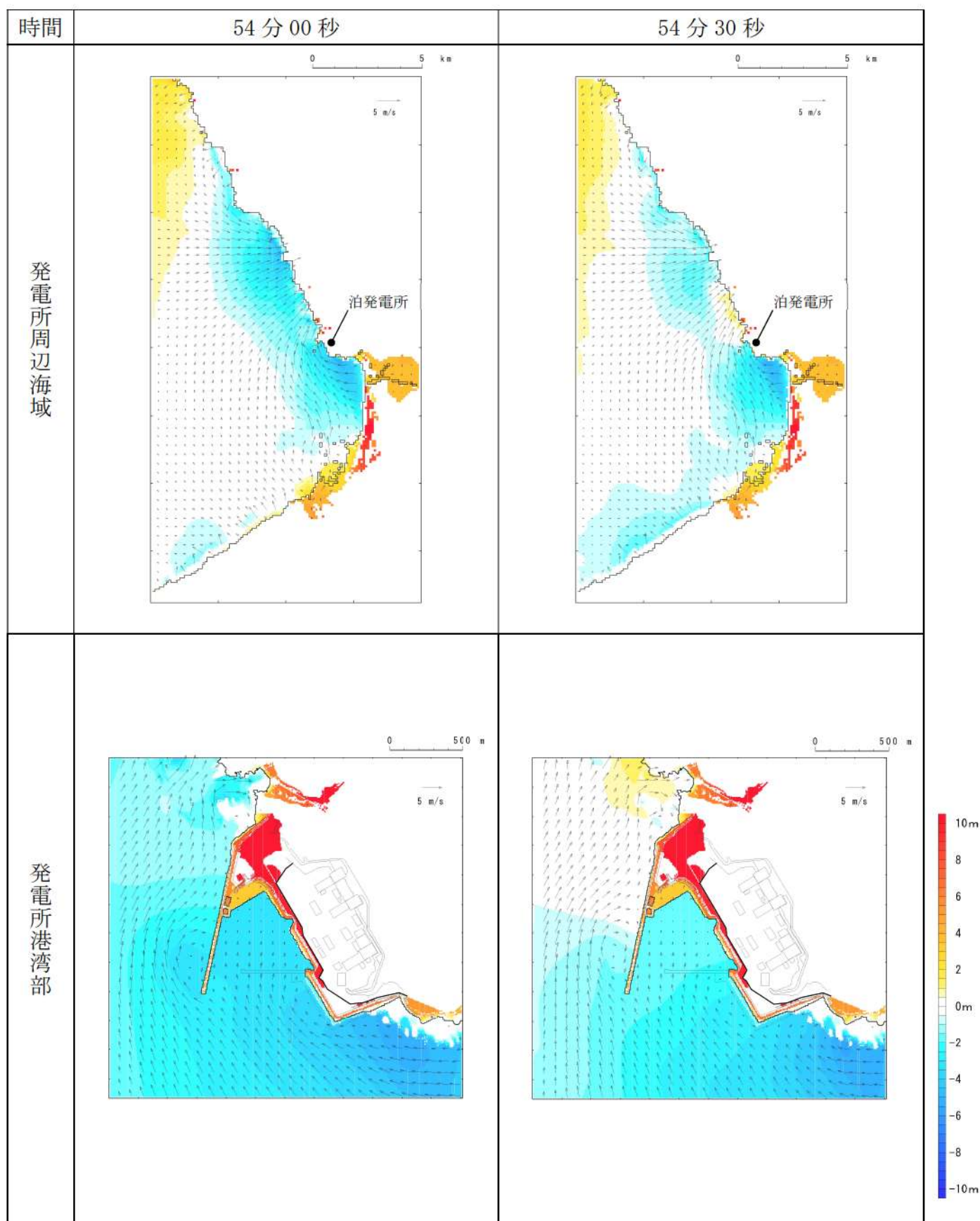
第 17 図-47 基準津波K（南防波堤損傷）の水位変動・流向ベクトル(47/53)
