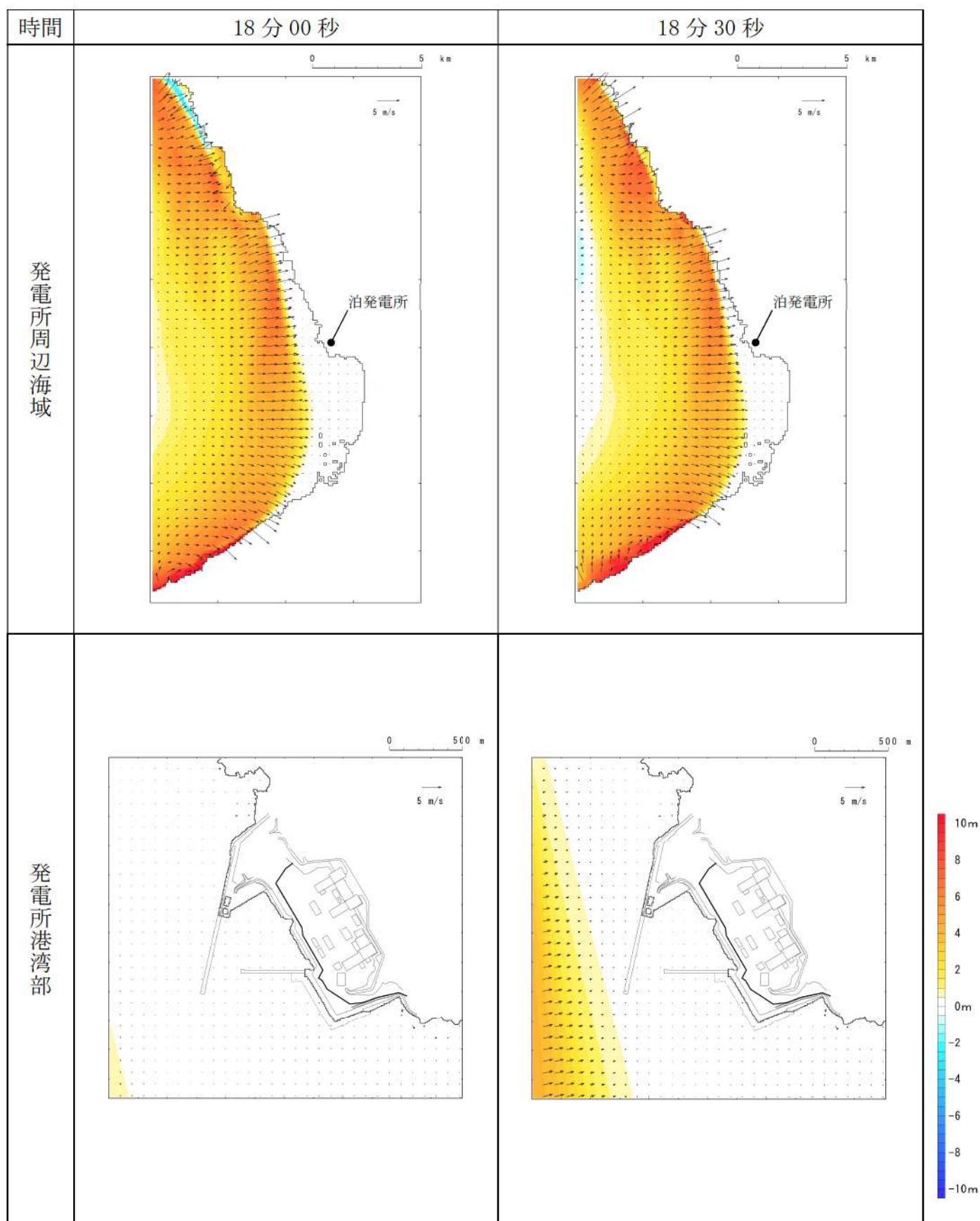
第 16 図-7 基準津波 J（北及び南防波堤損傷）の水位変動・流向ベクトル(7/49)
