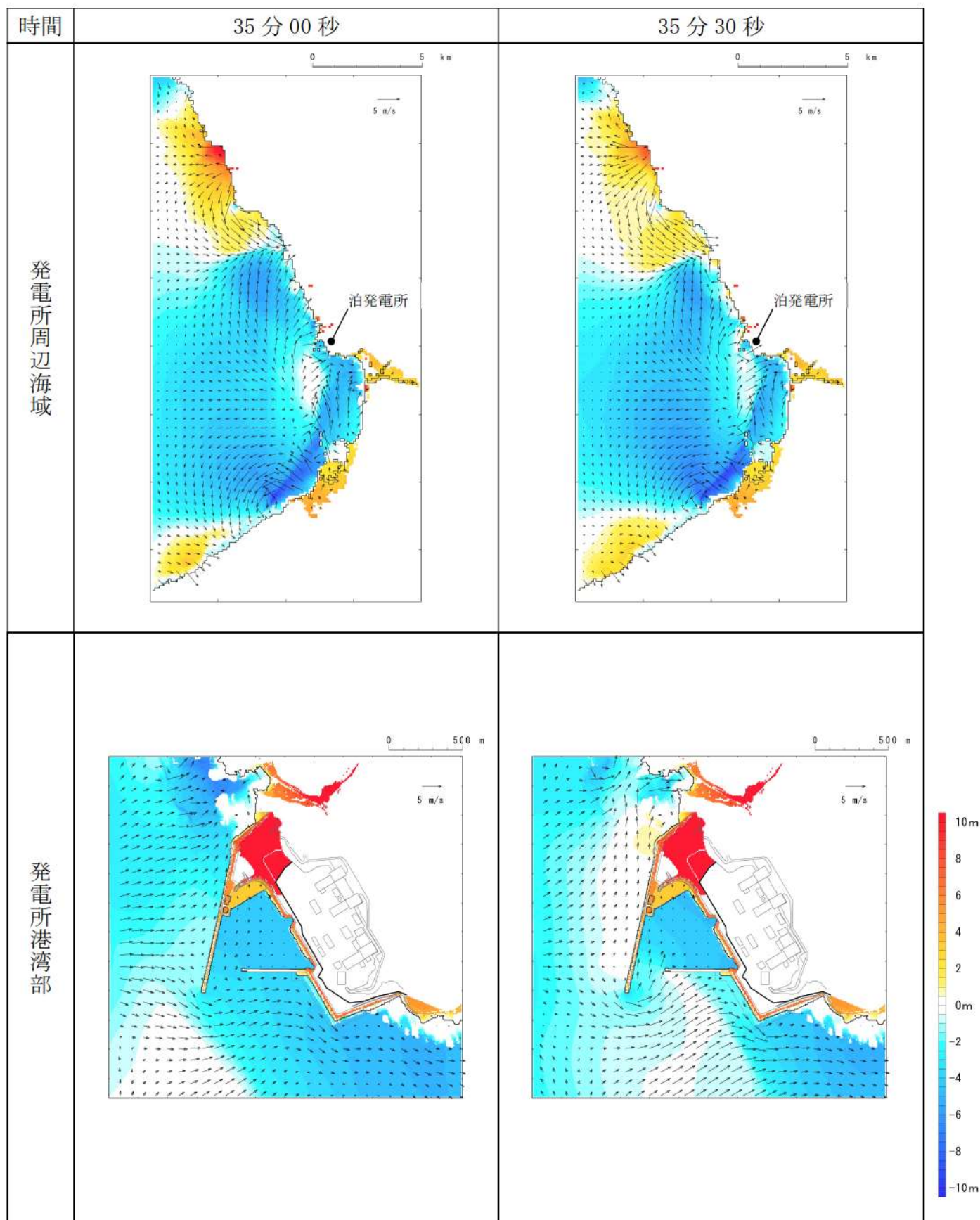
第 15 図-25 基準津波 I（防波堤損傷なし）の水位変動・流向ベクトル(25/50)
