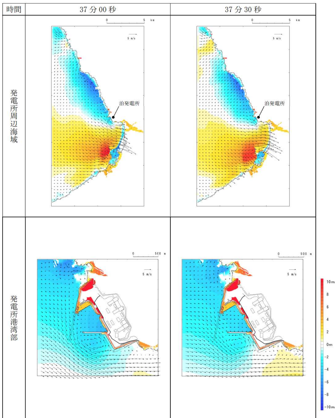
第 18 図-30 基準津波 L（北防波堤損傷）の水位変動・流向ベクトル(30/53)
