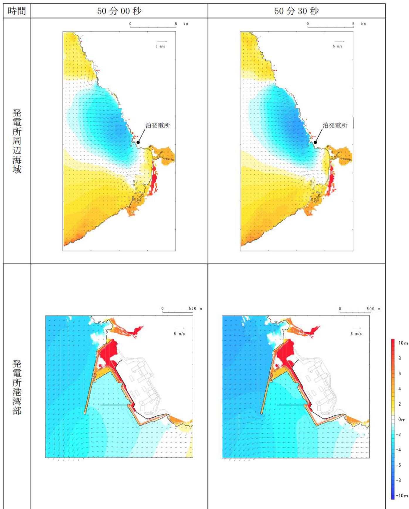
第 17 図-43 基準津波K（南防波堤損傷）の水位変動・流向ベクトル(43/53)
