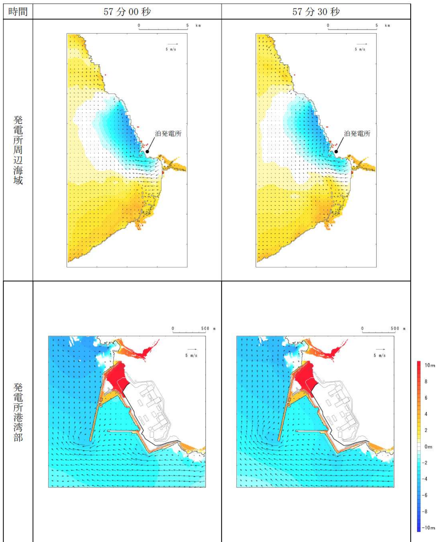
第 15 図-47 基準津波 I（防波堤損傷なし）の水位変動・流向ベクトル(47/50)
