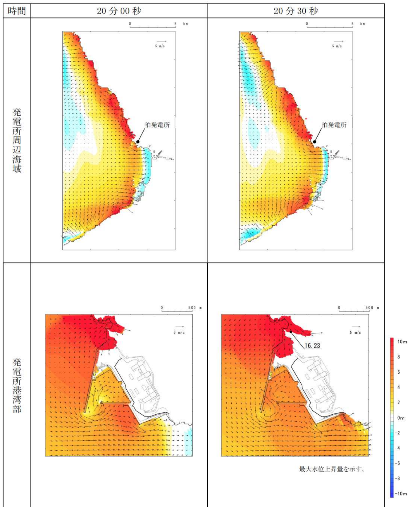
第 15 図-10 基準津波 I（防波堤損傷なし）の水位変動・流向ベクトル(10/50)
