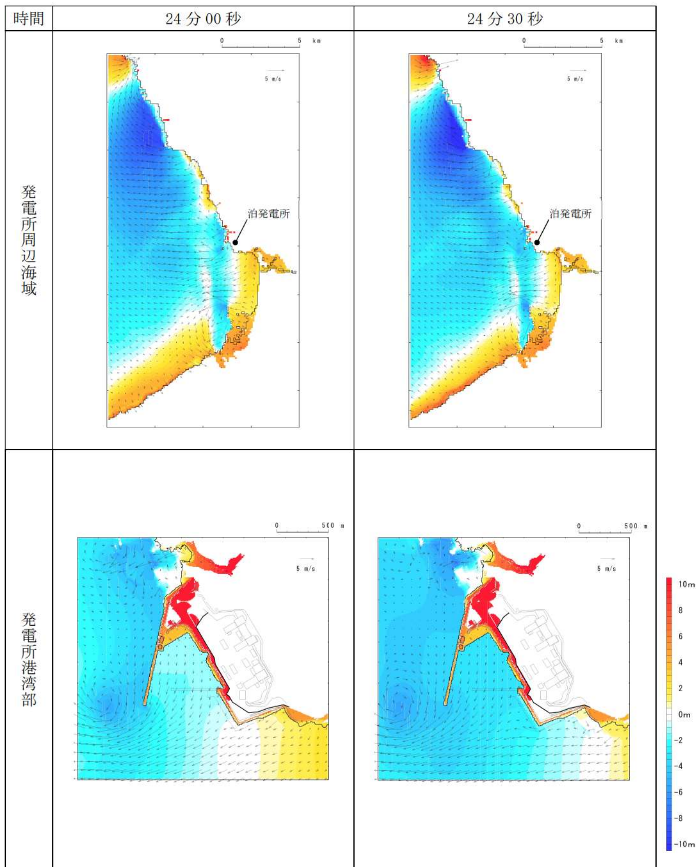
第 17 図-17 基準津波K（南防波堤損傷）の水位変動・流向ベクトル(17/53)
