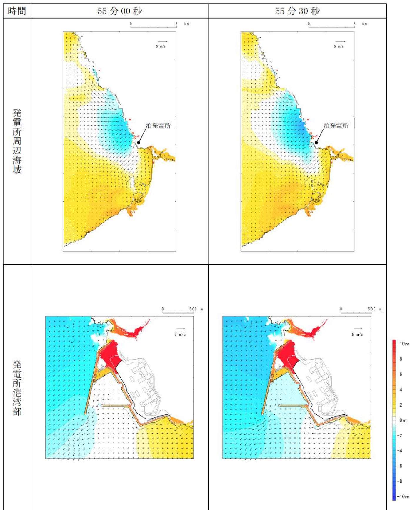
第 15 図-45 基準津波 I（防波堤損傷なし）の水位変動・流向ベクトル(45/50)
