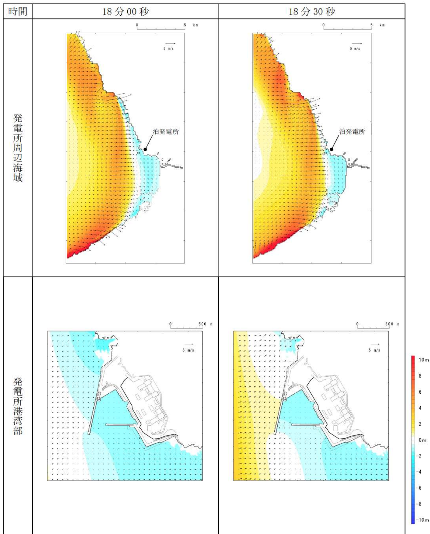
第 15 図-8 基準津波 I (防波堤損傷なし) の水位変動・流向ベクトル (8/50)
