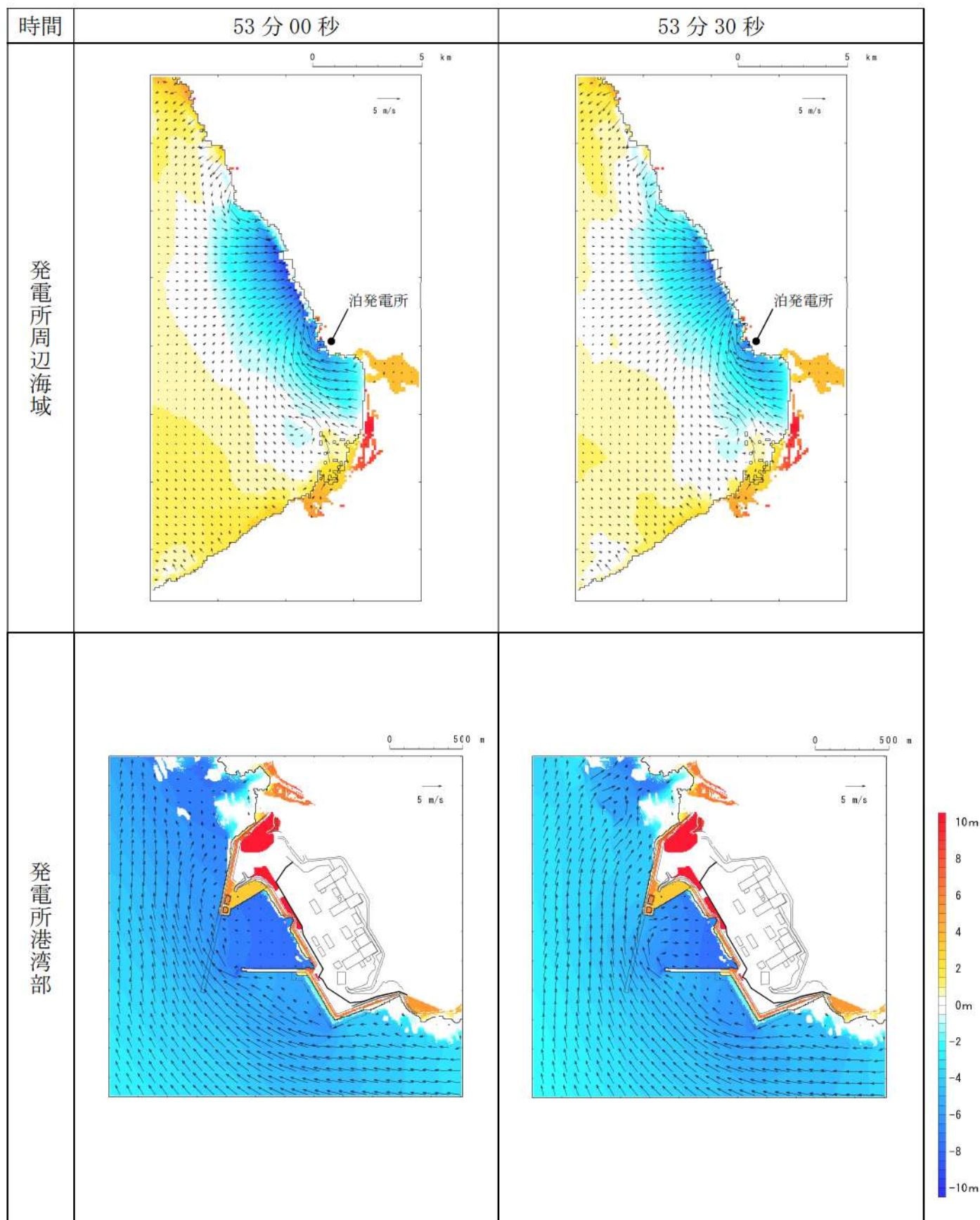
第 18 図-46 基準津波 L（北防波堤損傷）の水位変動・流向ベクトル(46/53)
