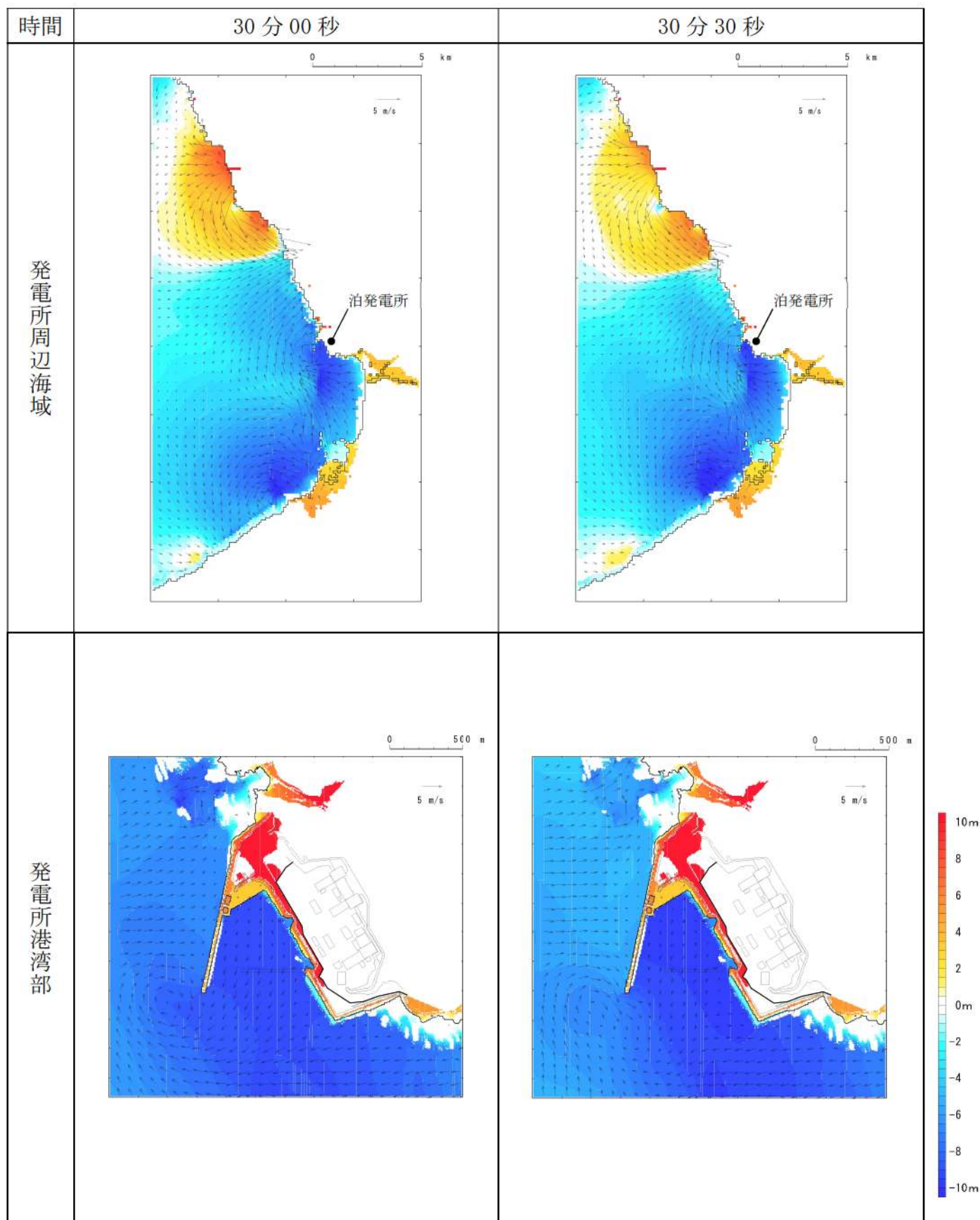
第 17 図-23 基準津波K（南防波堤損傷）の水位変動・流向ベクトル(23/53)
