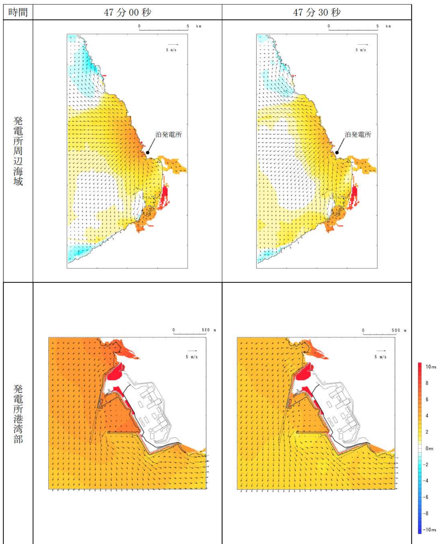
第 18 図-40 基準津波 L（北防波堤損傷）の水位変動・流向ベクトル(40/53)
