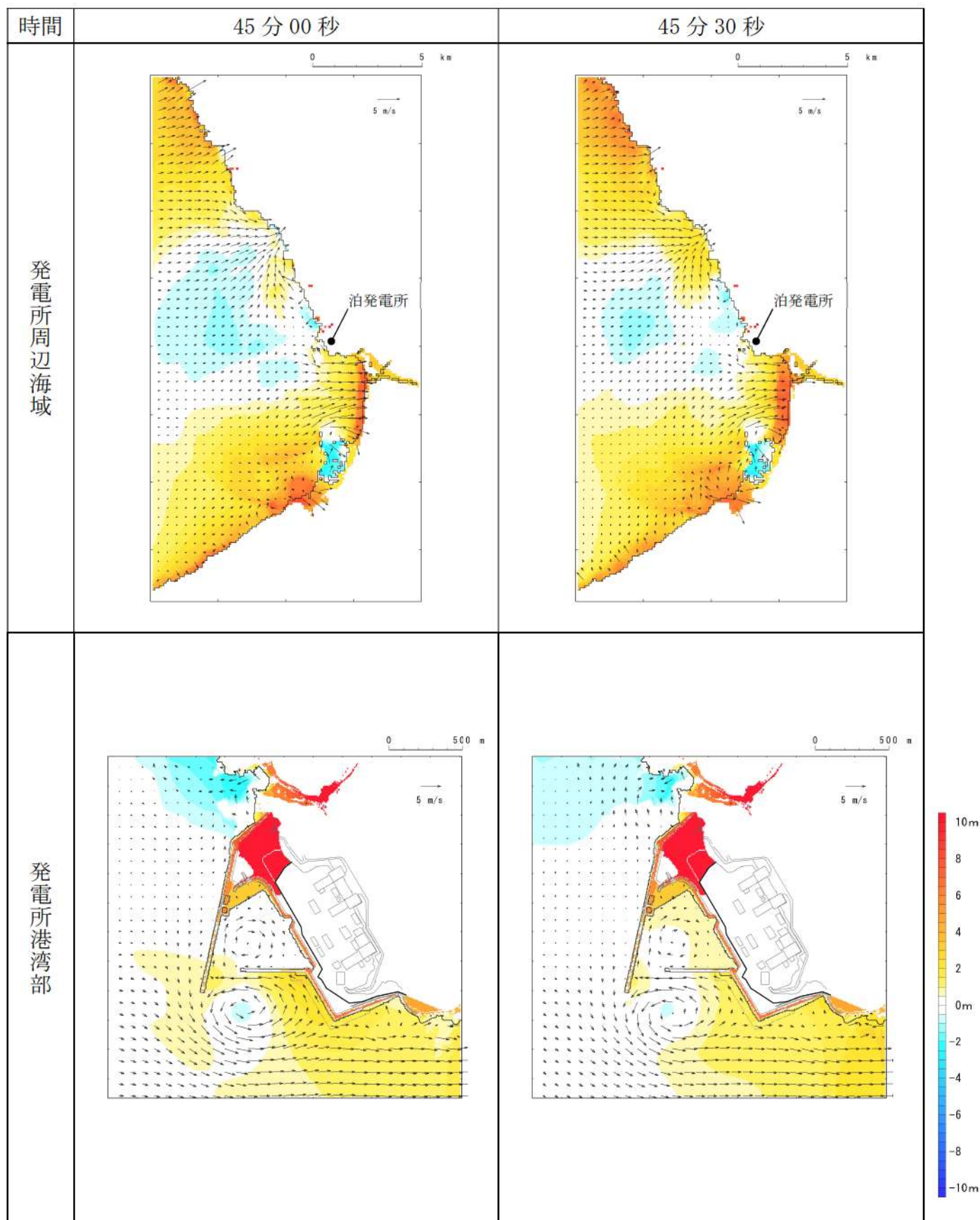
第 15 図-35 基準津波 I（防波堤損傷なし）の水位変動・流向ベクトル(35/50)
