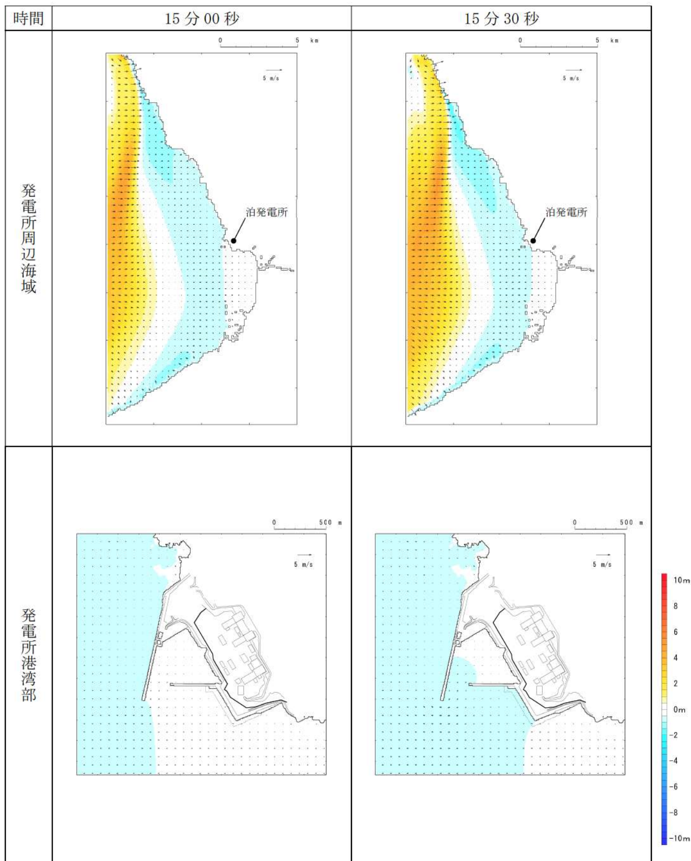
第 15 図-5 基準津波 I (防波堤損傷なし) の水位変動・流向ベクトル (5/50)
