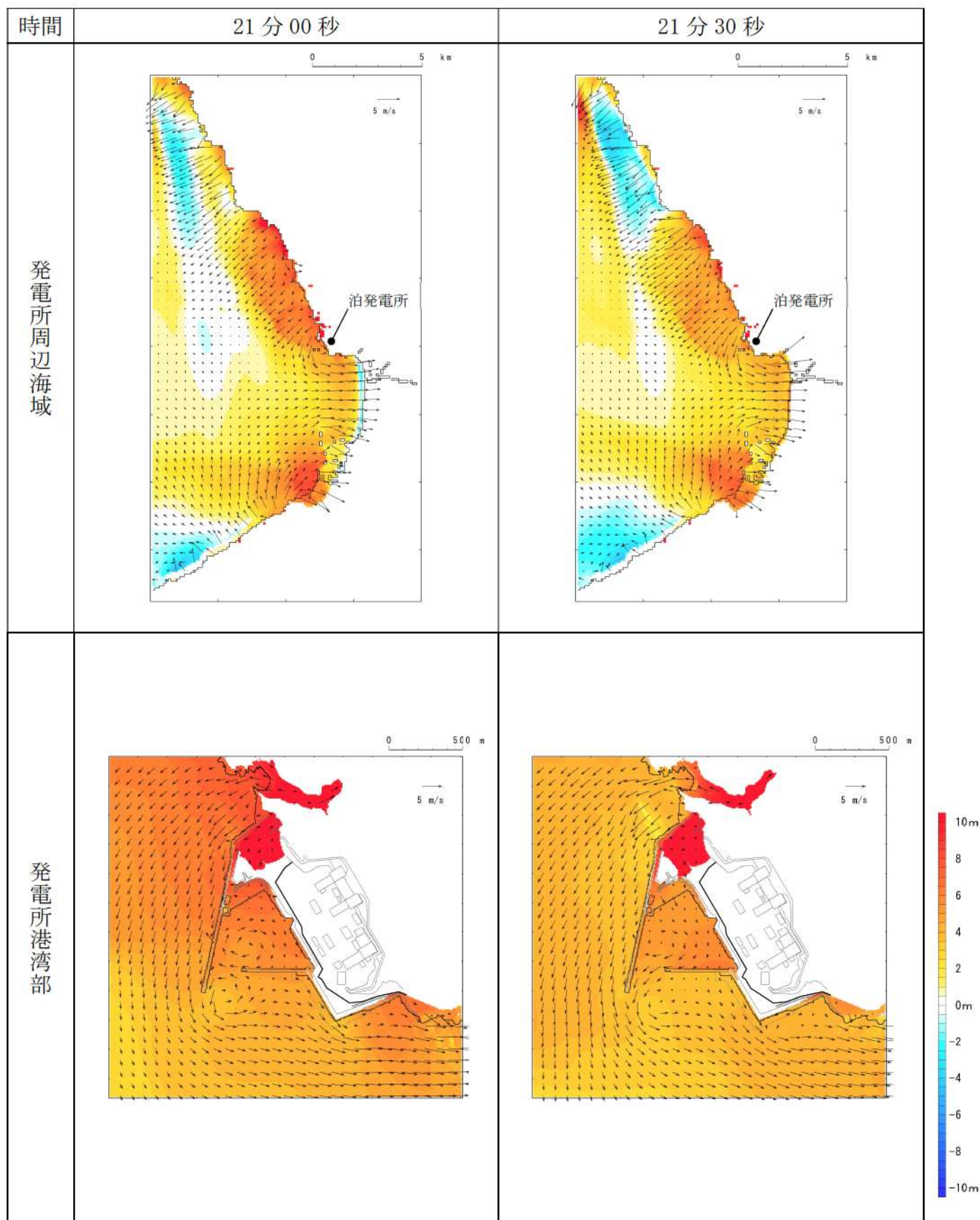
第 15 図-11 基準津波 I（防波堤損傷なし）の水位変動・流向ベクトル(11/50)
