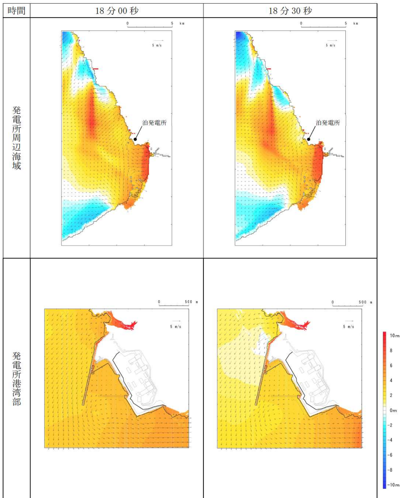
第 17 図-11 基準津波K（南防波堤損傷）の水位変動・流向ベクトル(11/53)
