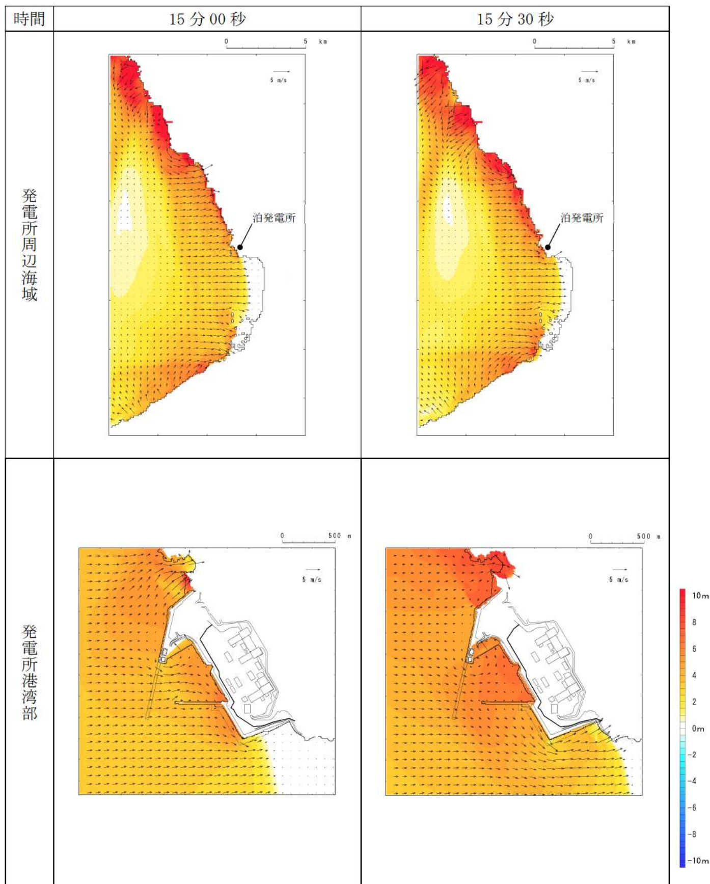
第 18 図-8 基準津波 L（北防波堤損傷）の水位変動・流向ベクトル (8/53)
