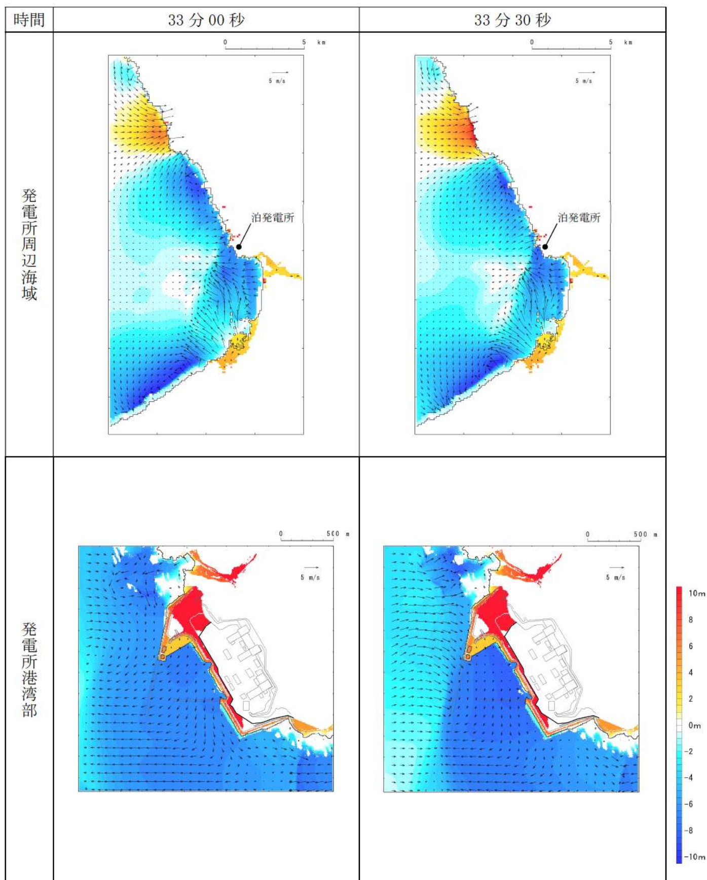
第 16 図-22 基準津波 J（北及び南防波堤損傷）の水位変動・流向ベクトル(22/49)
