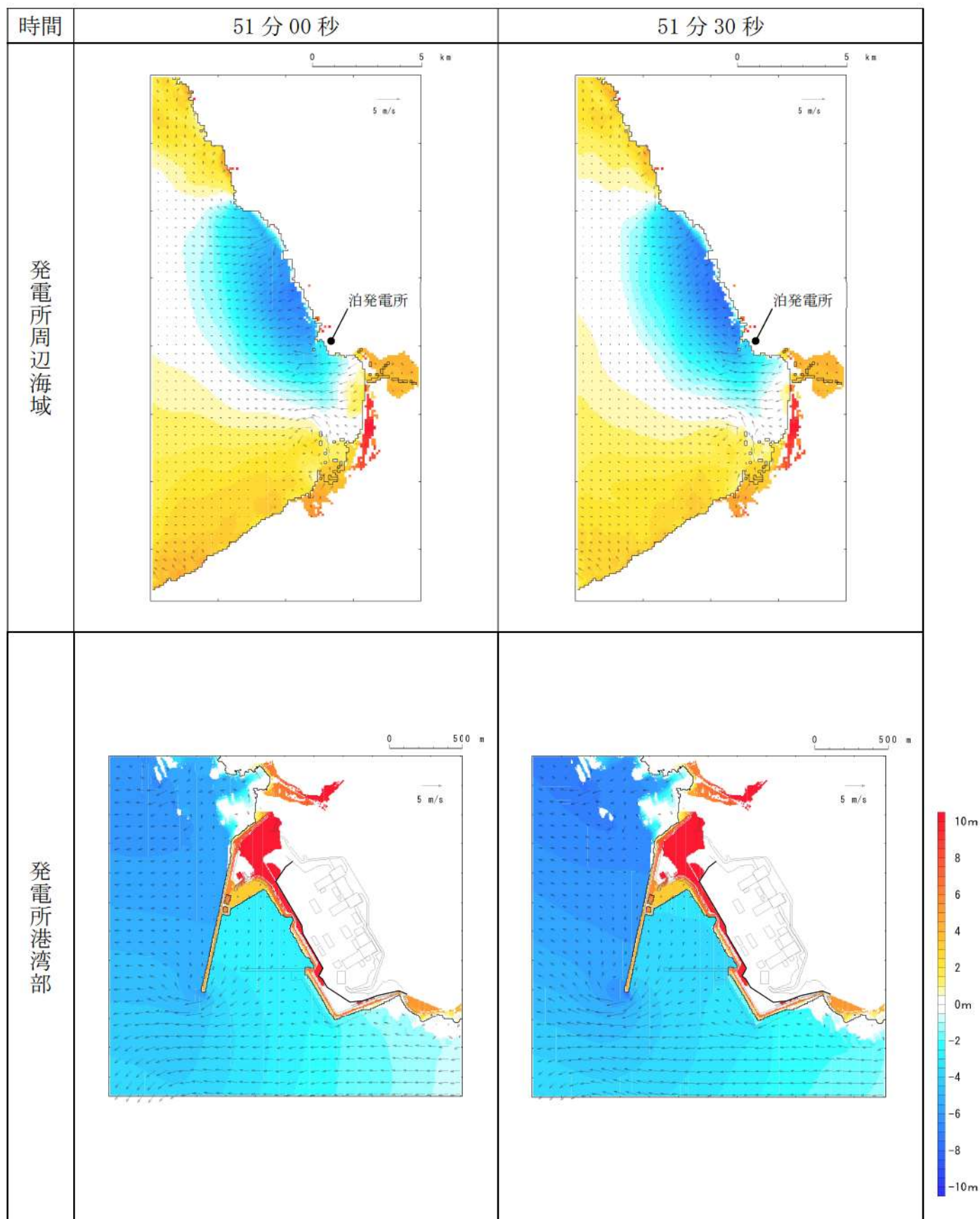
第 17 図-44 基準津波K（南防波堤損傷）の水位変動・流向ベクトル(44/53)
