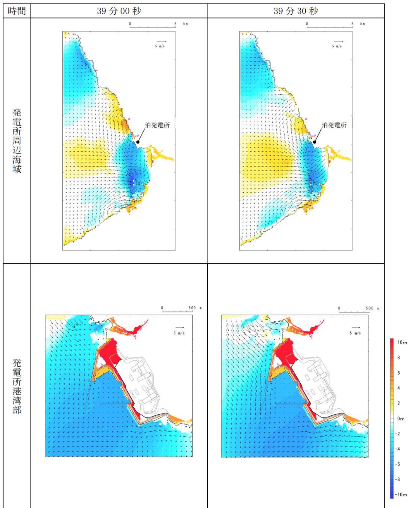
第 16 図-28 基準津波 J（北及び南防波堤損傷）の水位変動・流向ベクトル(28/49)
