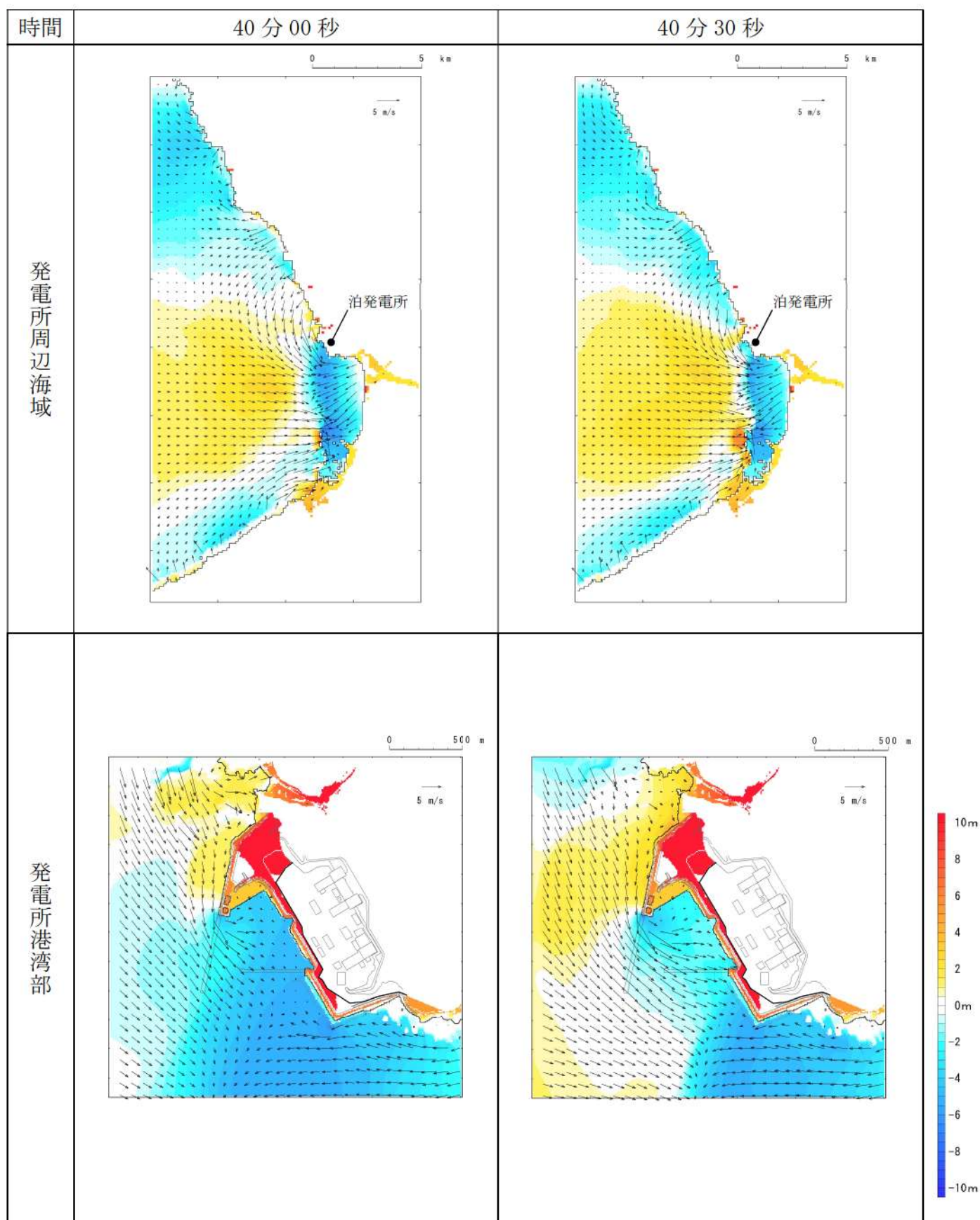
第 16 図-29 基準津波 J（北及び南防波堤損傷）の水位変動・流向ベクトル(29/49)
