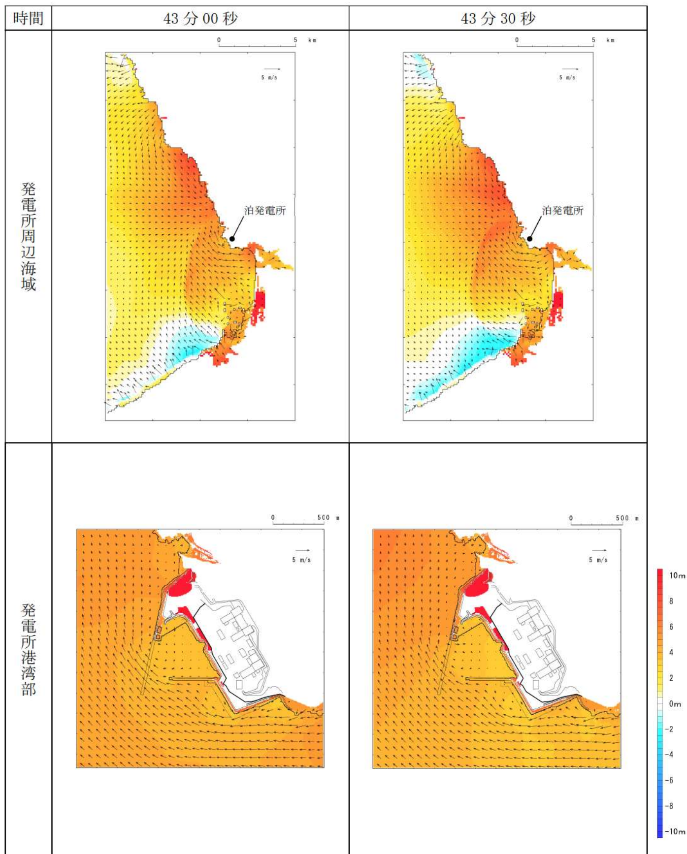
第 18 図-36 基準津波 L（北防波堤損傷）の水位変動・流向ベクトル(36/53)
