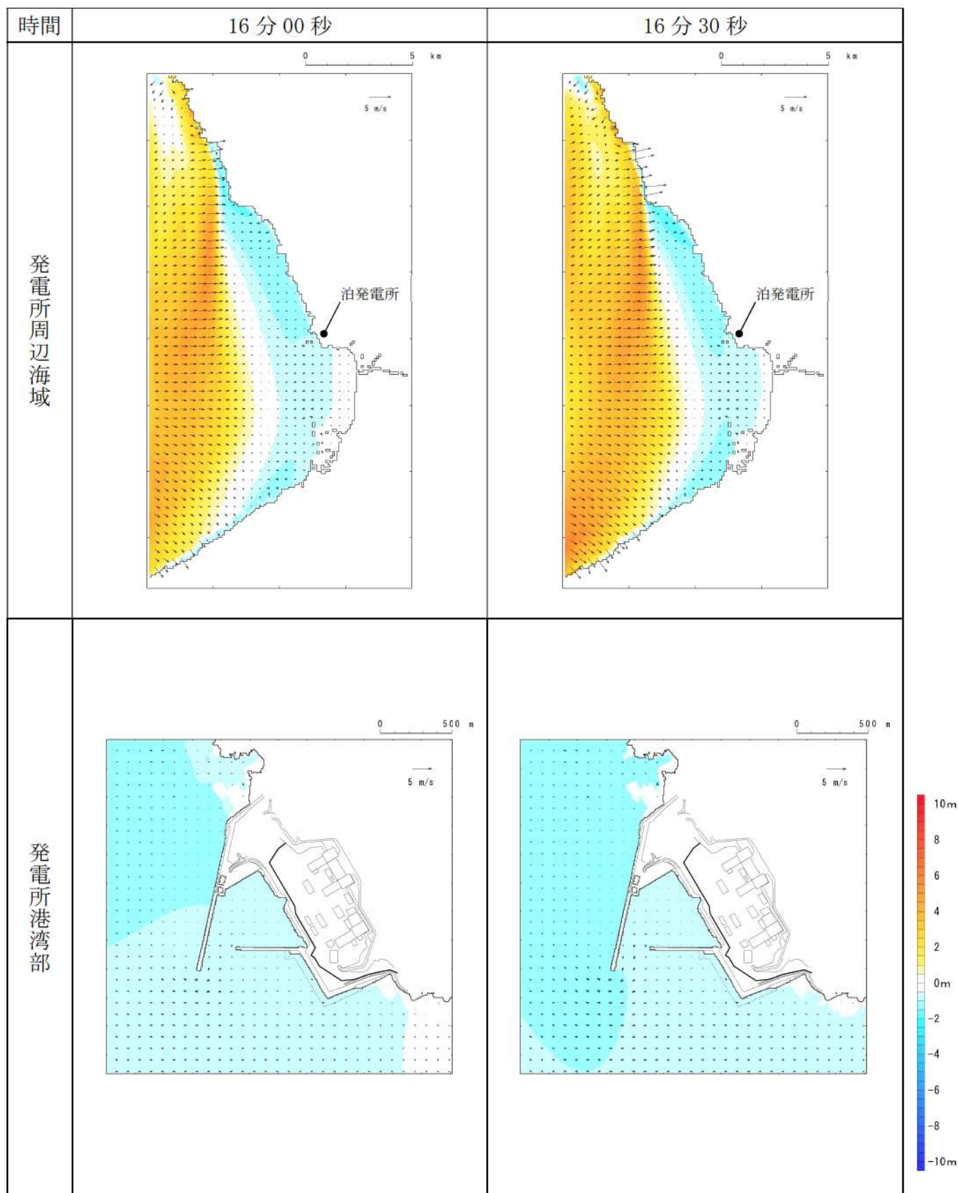
第 15 図-6 基準津波 I (防波堤損傷なし) の水位変動・流向ベクトル (6/50)
