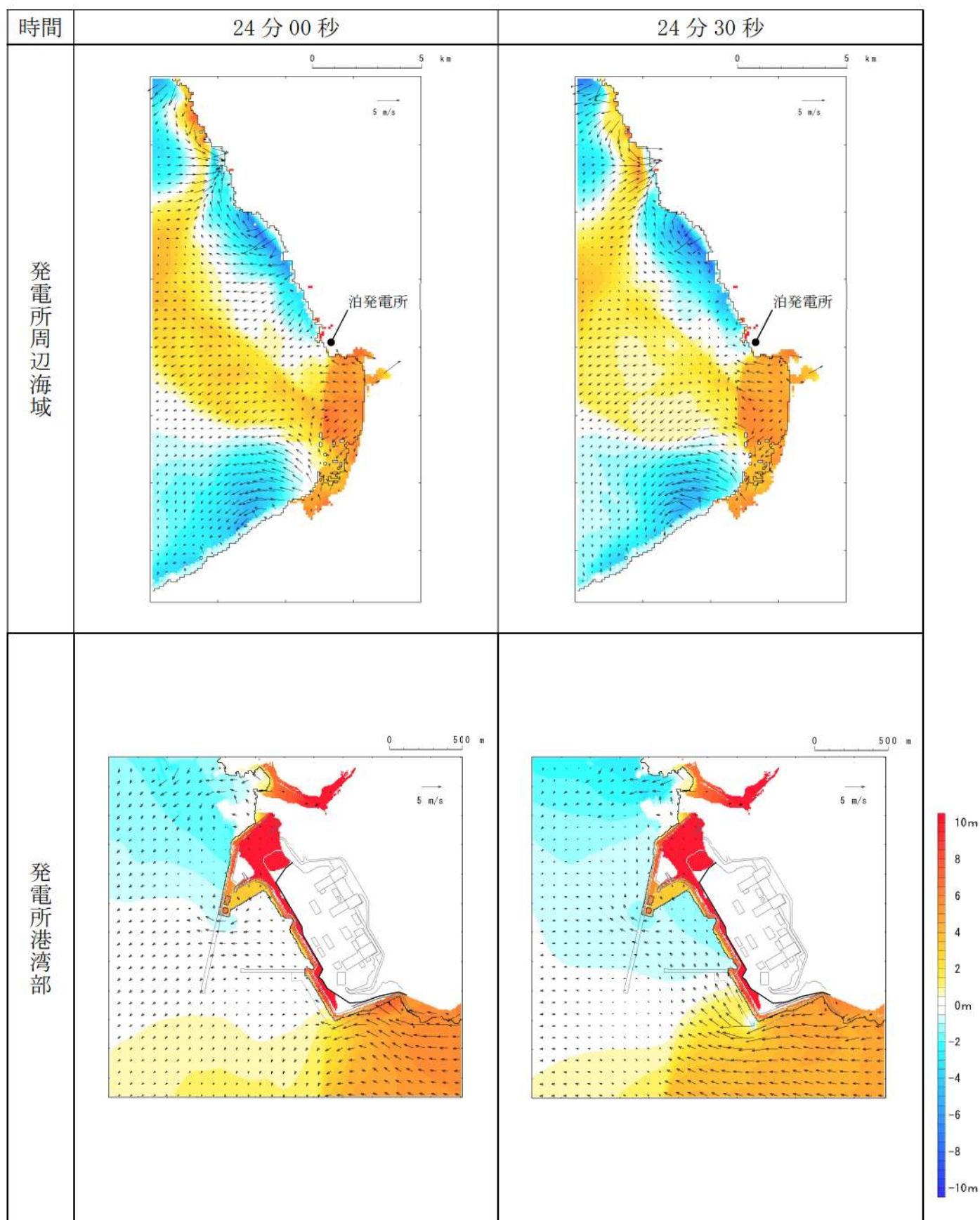
第 16 図-13 基準津波 J（北及び南防波堤損傷）の水位変動・流向ベクトル(13/49)
