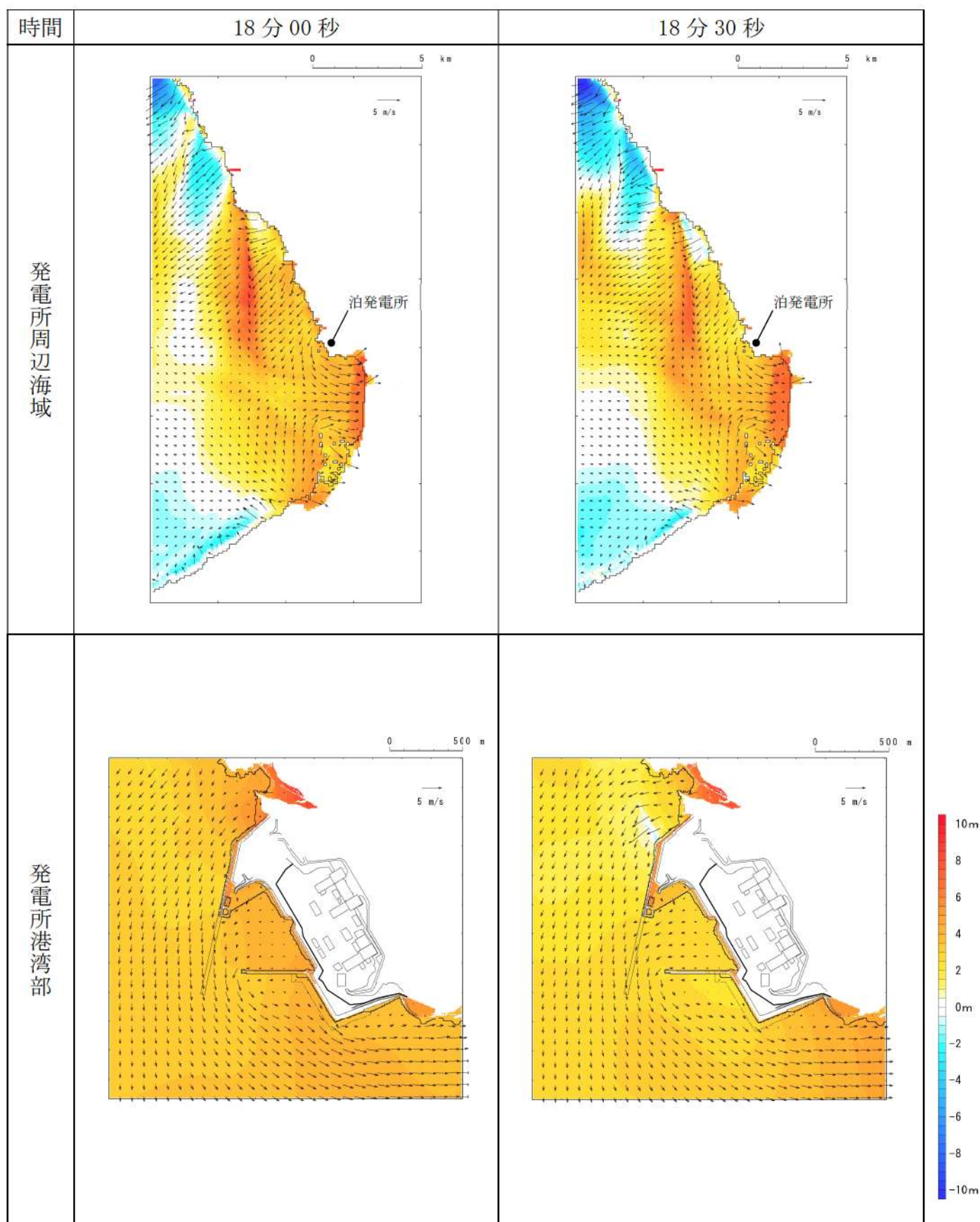
第 18 図-11 基準津波 L（北防波堤損傷）の水位変動・流向ベクトル(11/53)
