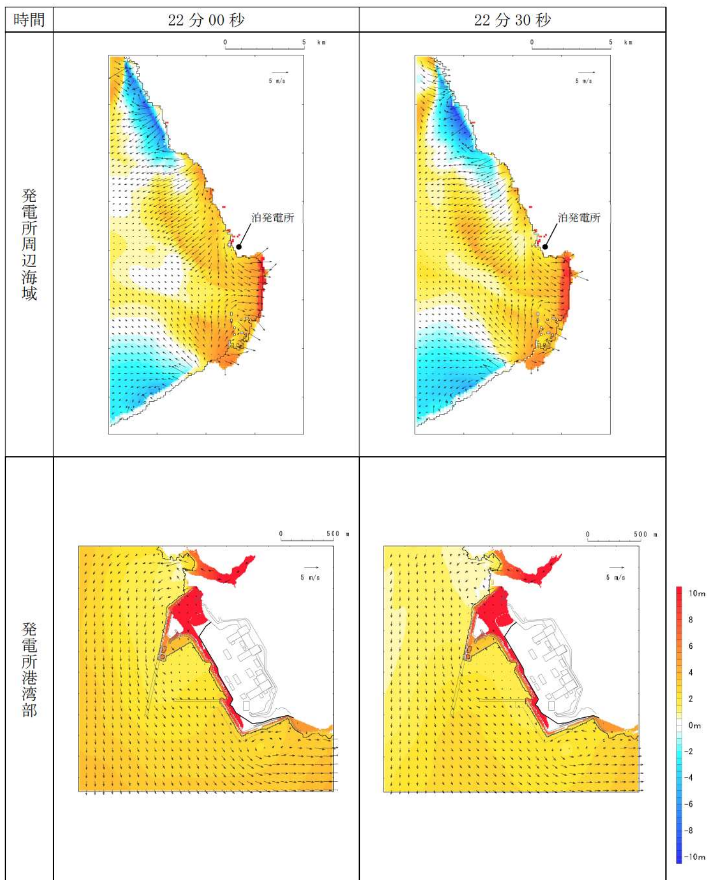
第 16 図-11 基準津波 J（北及び南防波堤損傷）の水位変動・流向ベクトル(11/49)
