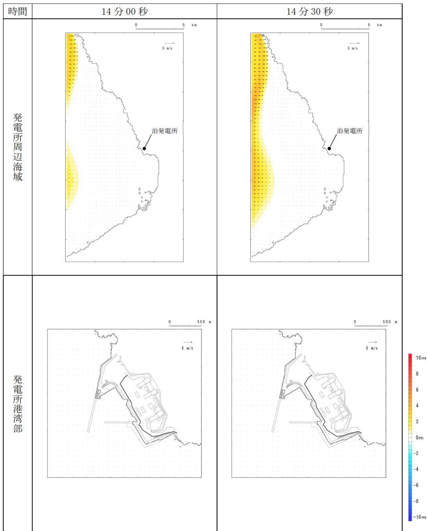
第 16 図-3 基準津波 J（北及び南防波堤損傷）の水位変動・流向ベクトル (3/49)
