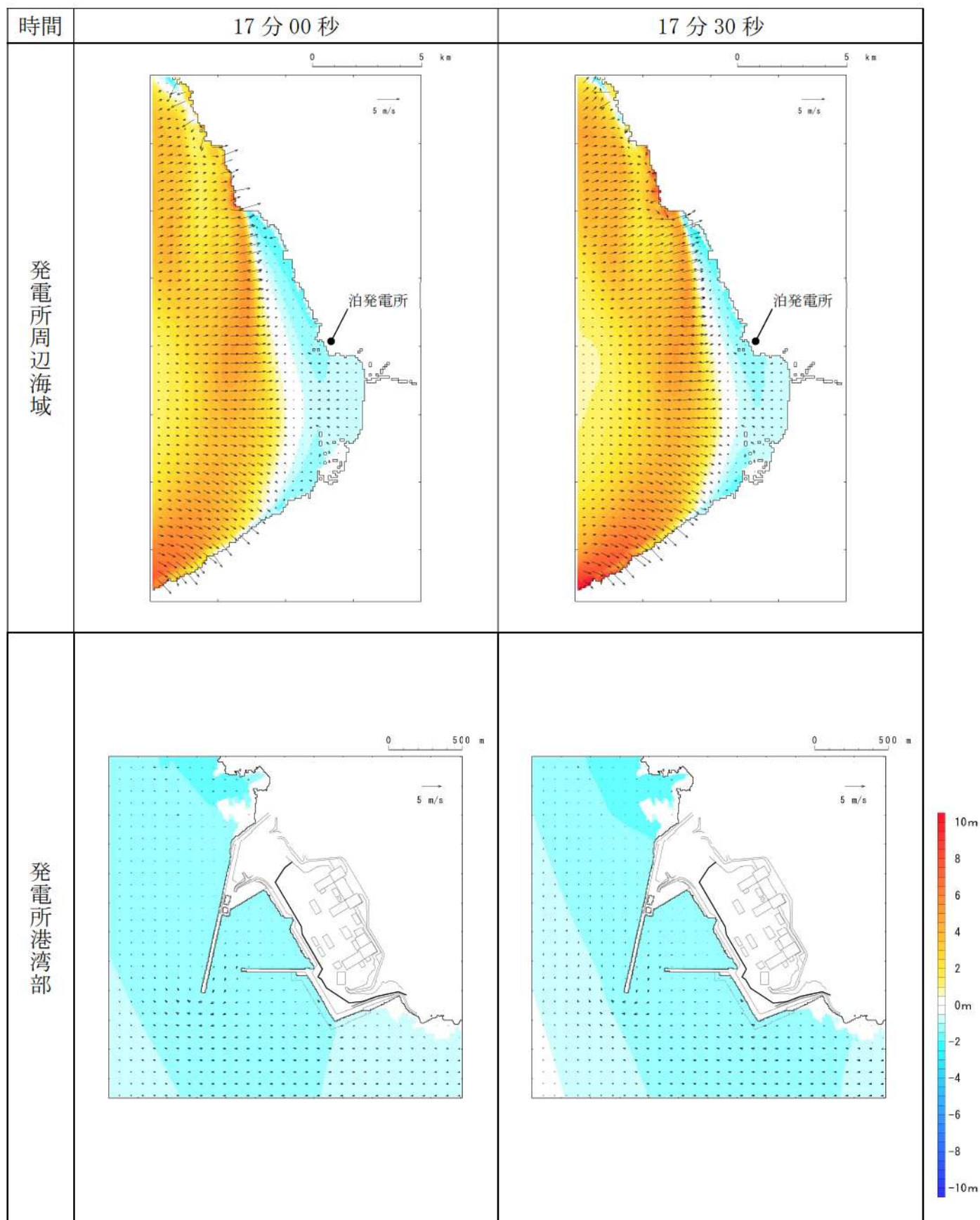
第 15 図-7 基準津波 I (防波堤損傷なし) の水位変動・流向ベクトル (7/50)
