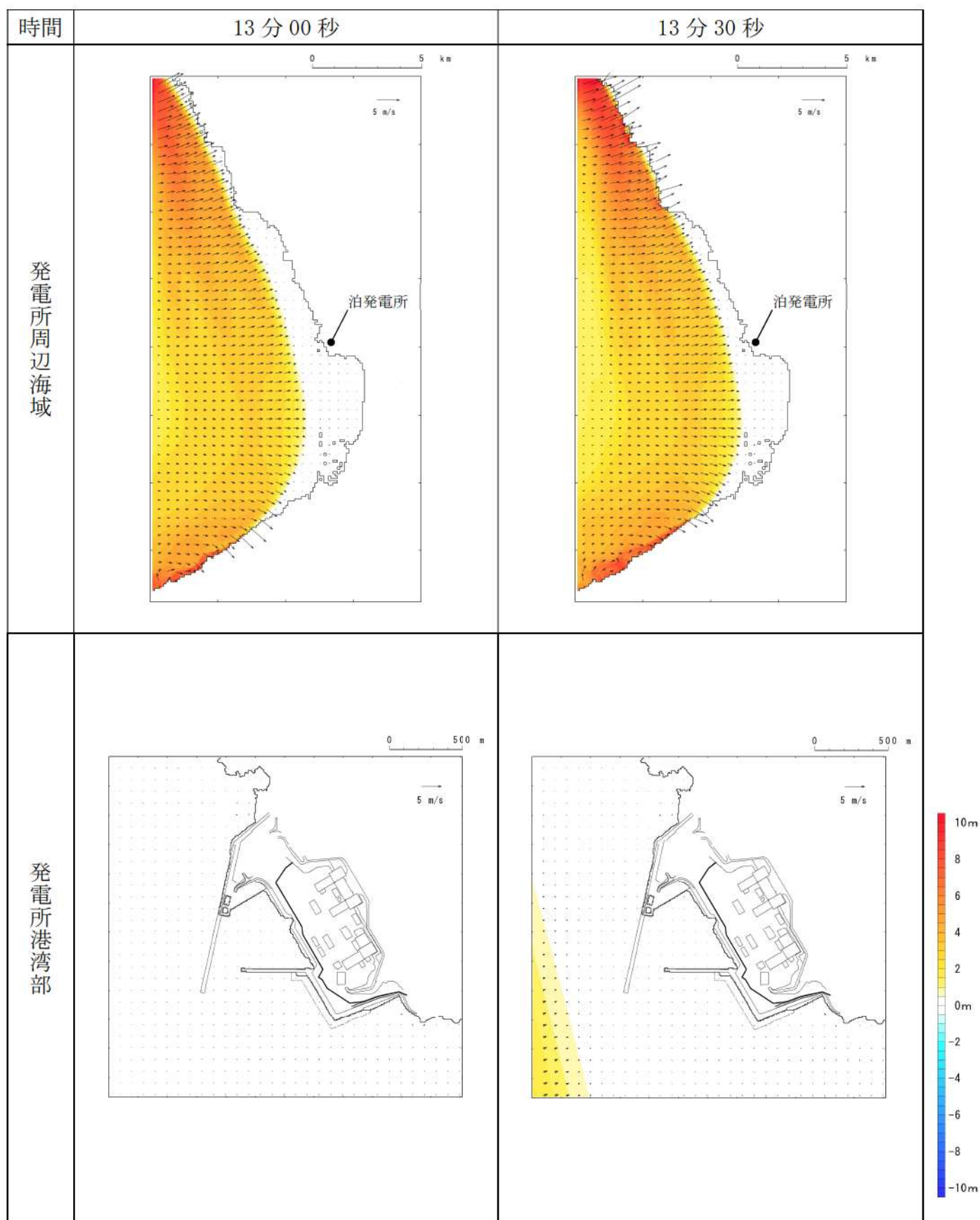
第 18 図-6 基準津波 L（北防波堤損傷）の水位変動・流向ベクトル (6/53)
