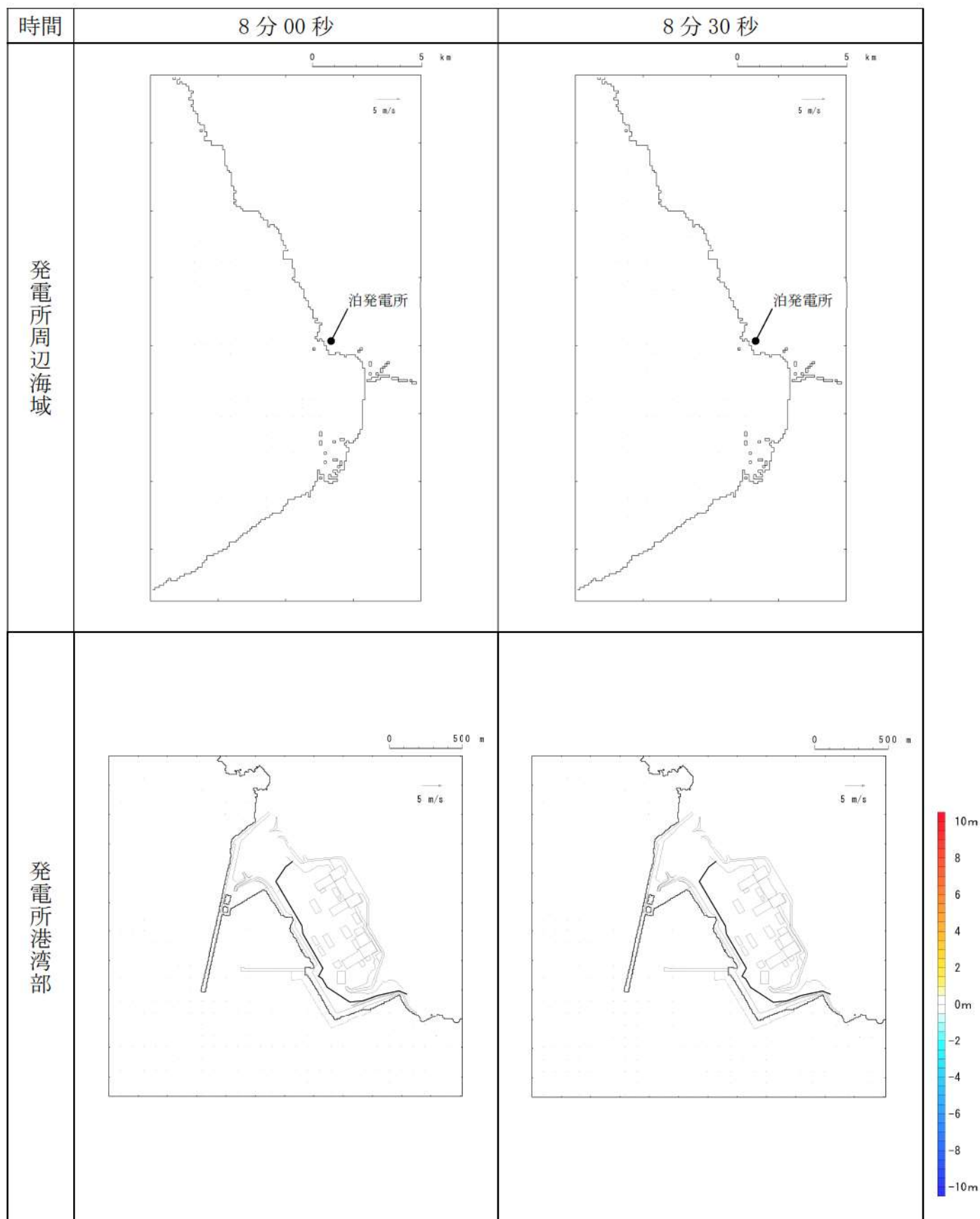
第 17 図-1 基準津波 K（南防波堤損傷）の水位変動・流向ベクトル(1/53)
