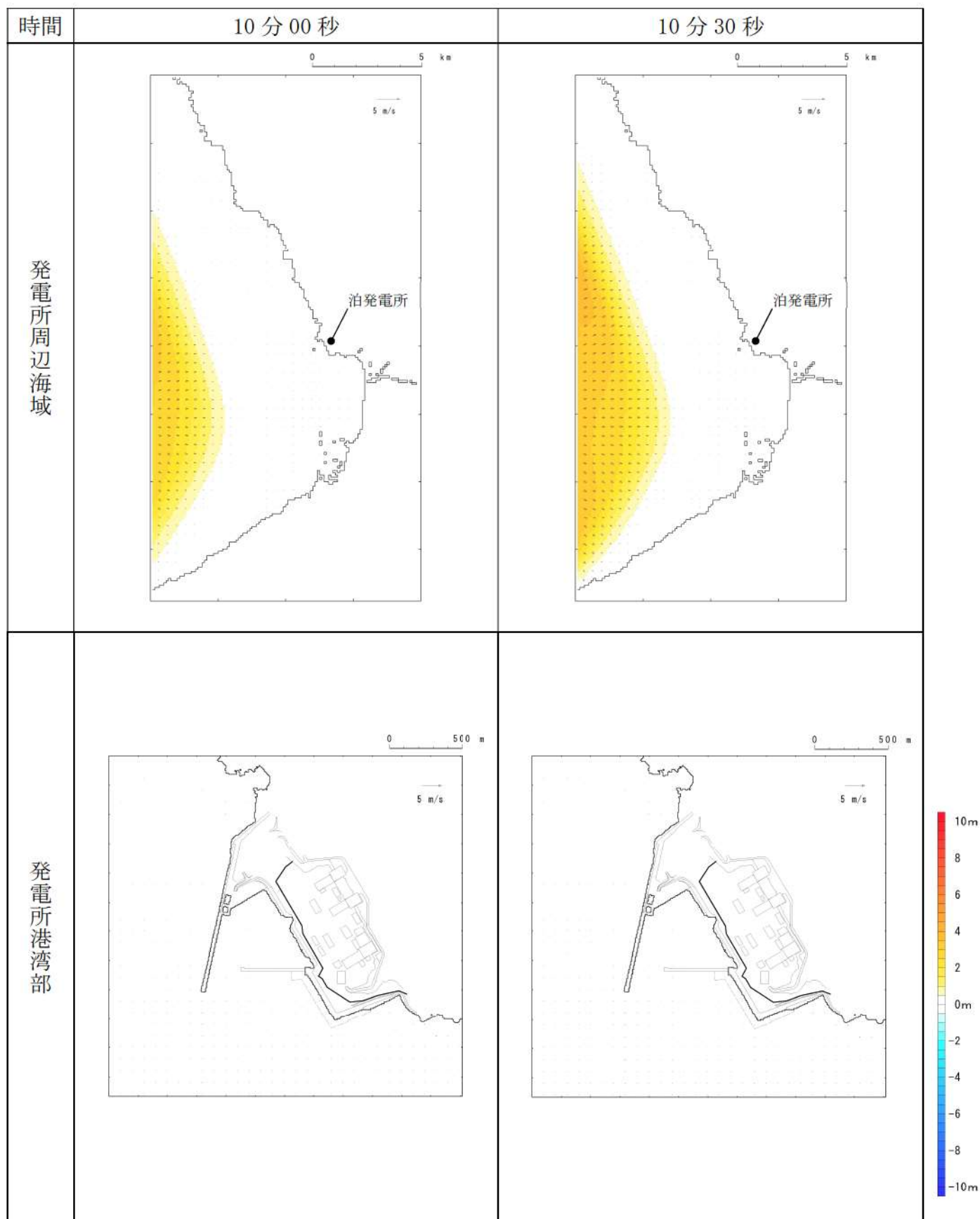
第 17 図-3 基準津波 K (南防波堤損傷) の水位変動・流向ベクトル (3/53)
