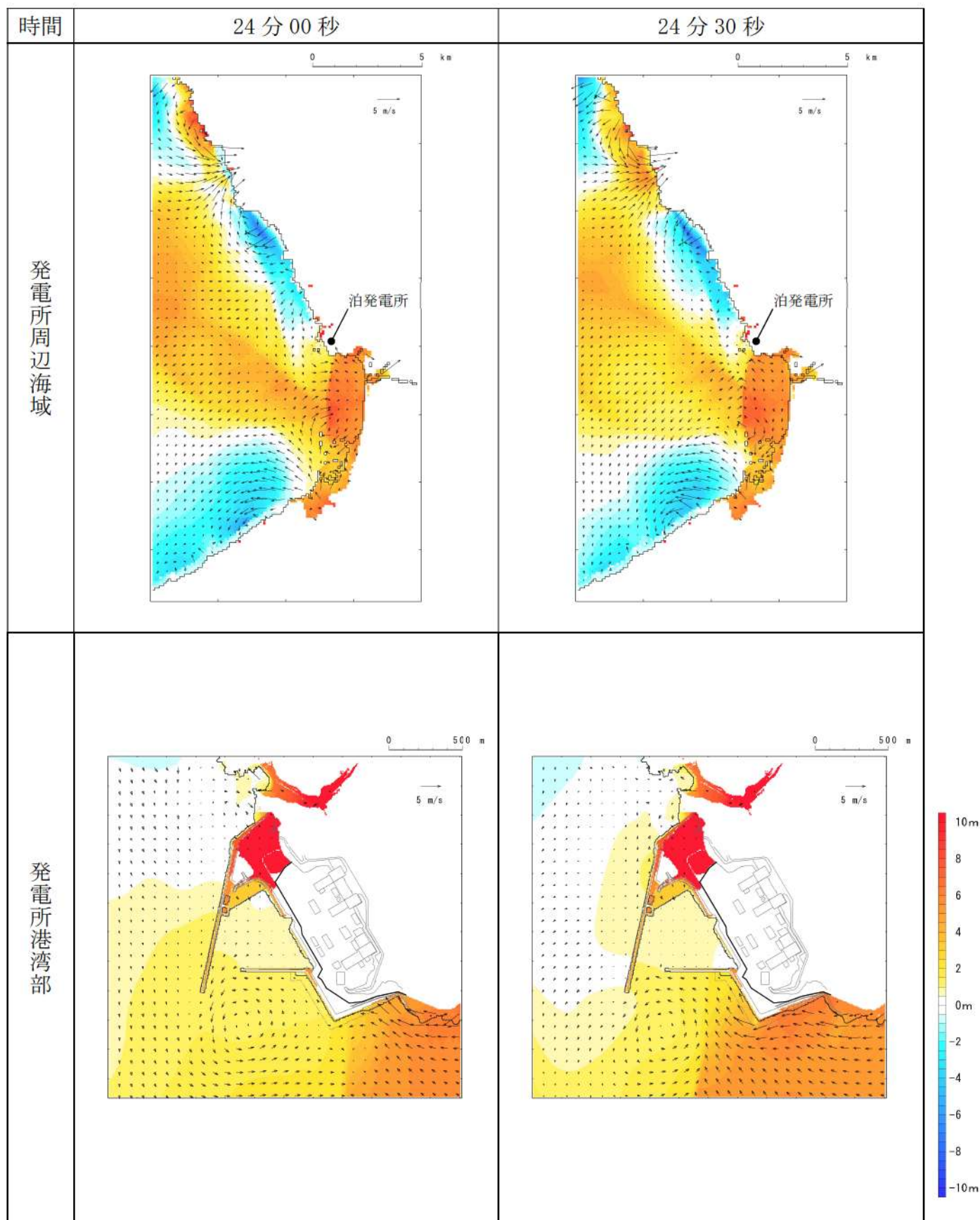
第 15 図-14 基準津波 I（防波堤損傷なし）の水位変動・流向ベクトル(14/50)
