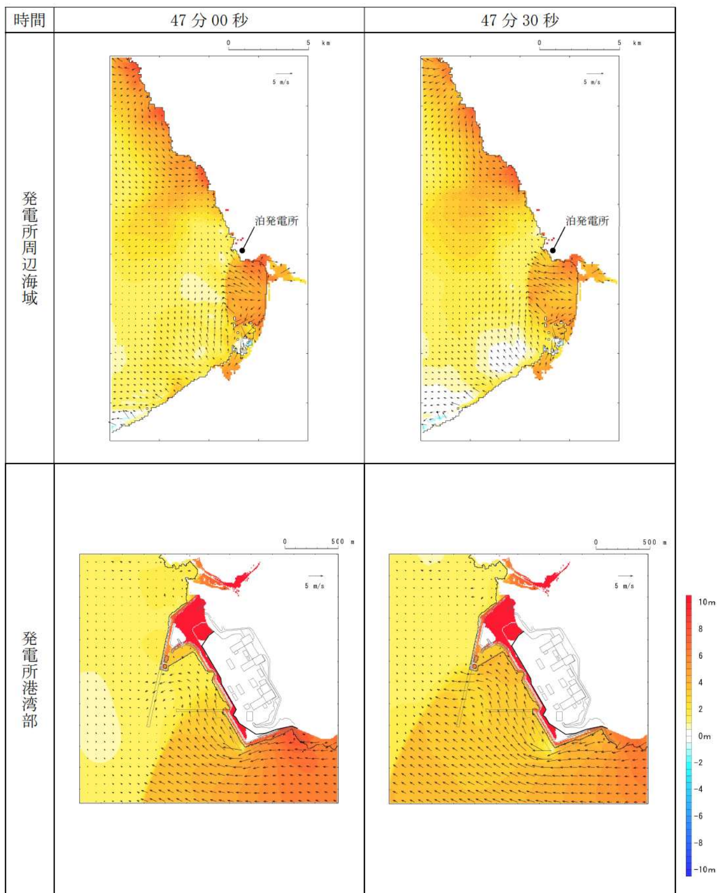
第 16 図-36 基準津波 J（北及び南防波堤損傷）の水位変動・流向ベクトル(36/49)
