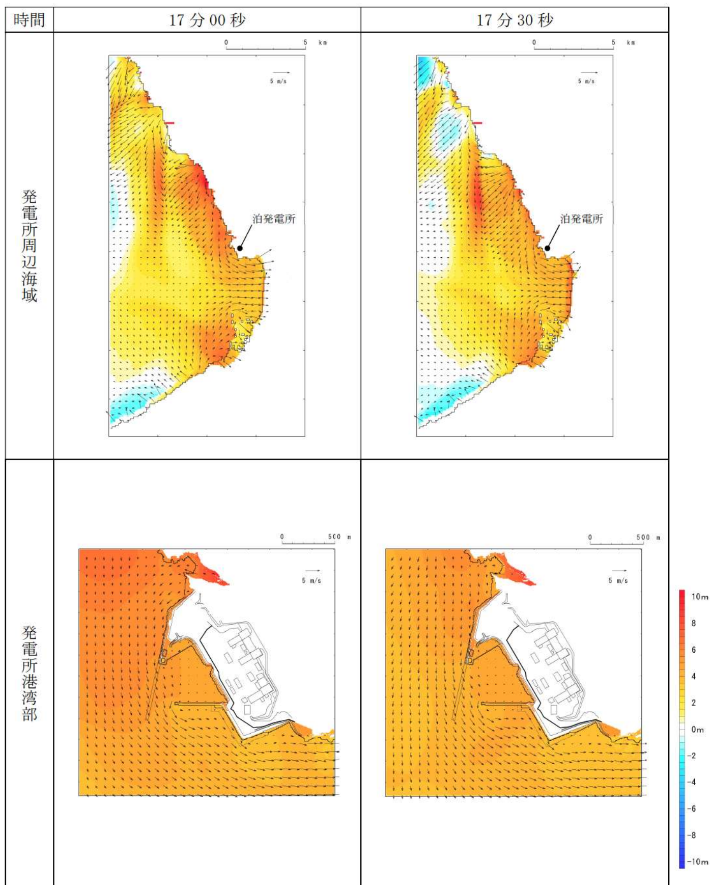
第 18 図-10 基準津波 L（北防波堤損傷）の水位変動・流向ベクトル(10/53)
