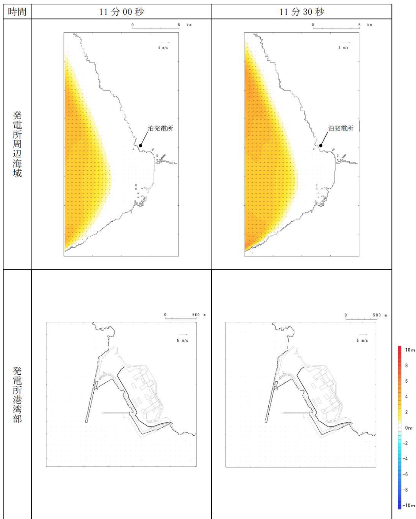
第 17 図-4 基準津波 K（南防波堤損傷）の水位変動・流向ベクトル (4/53)
