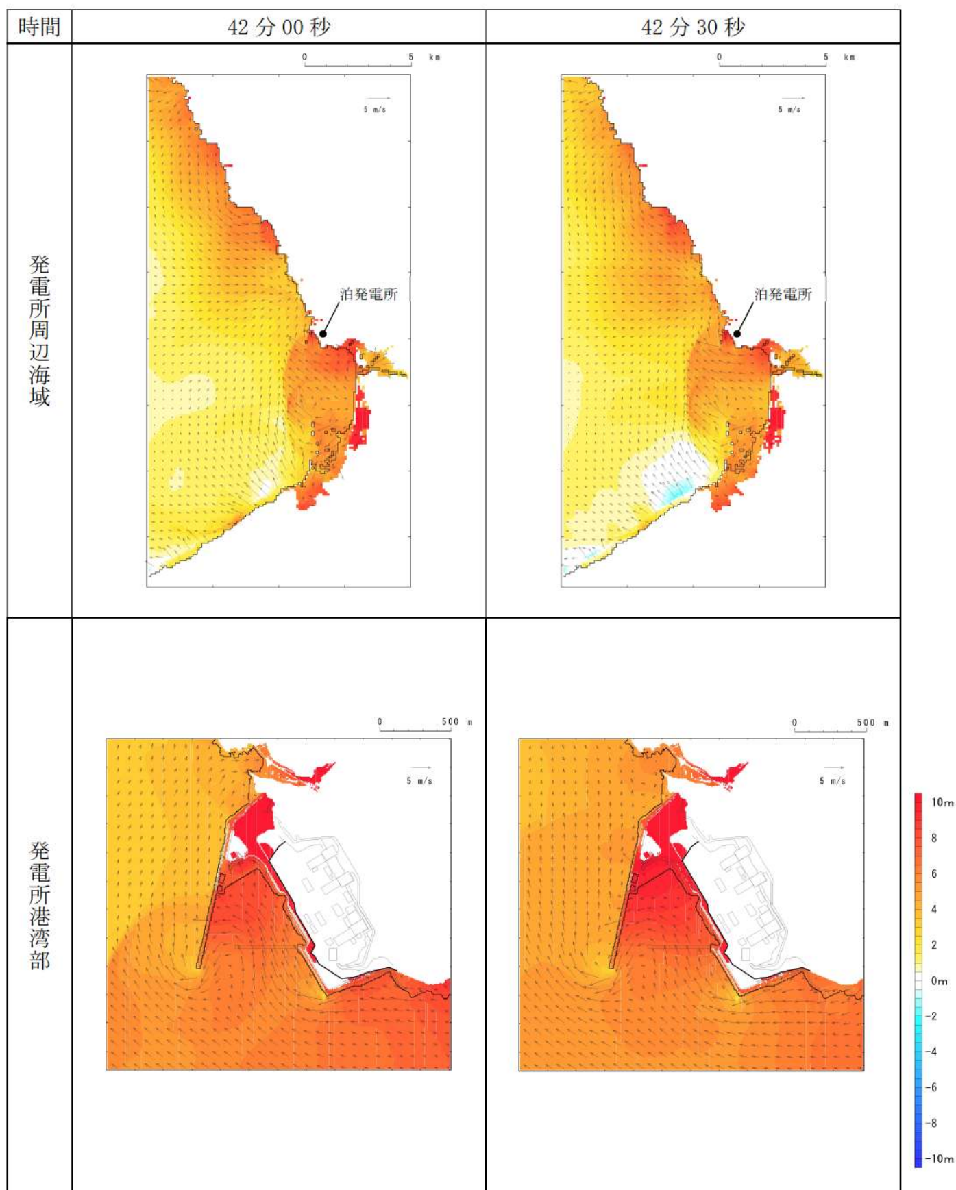
第 17 図-35 基準津波K（南防波堤損傷）の水位変動・流向ベクトル(35/53)
