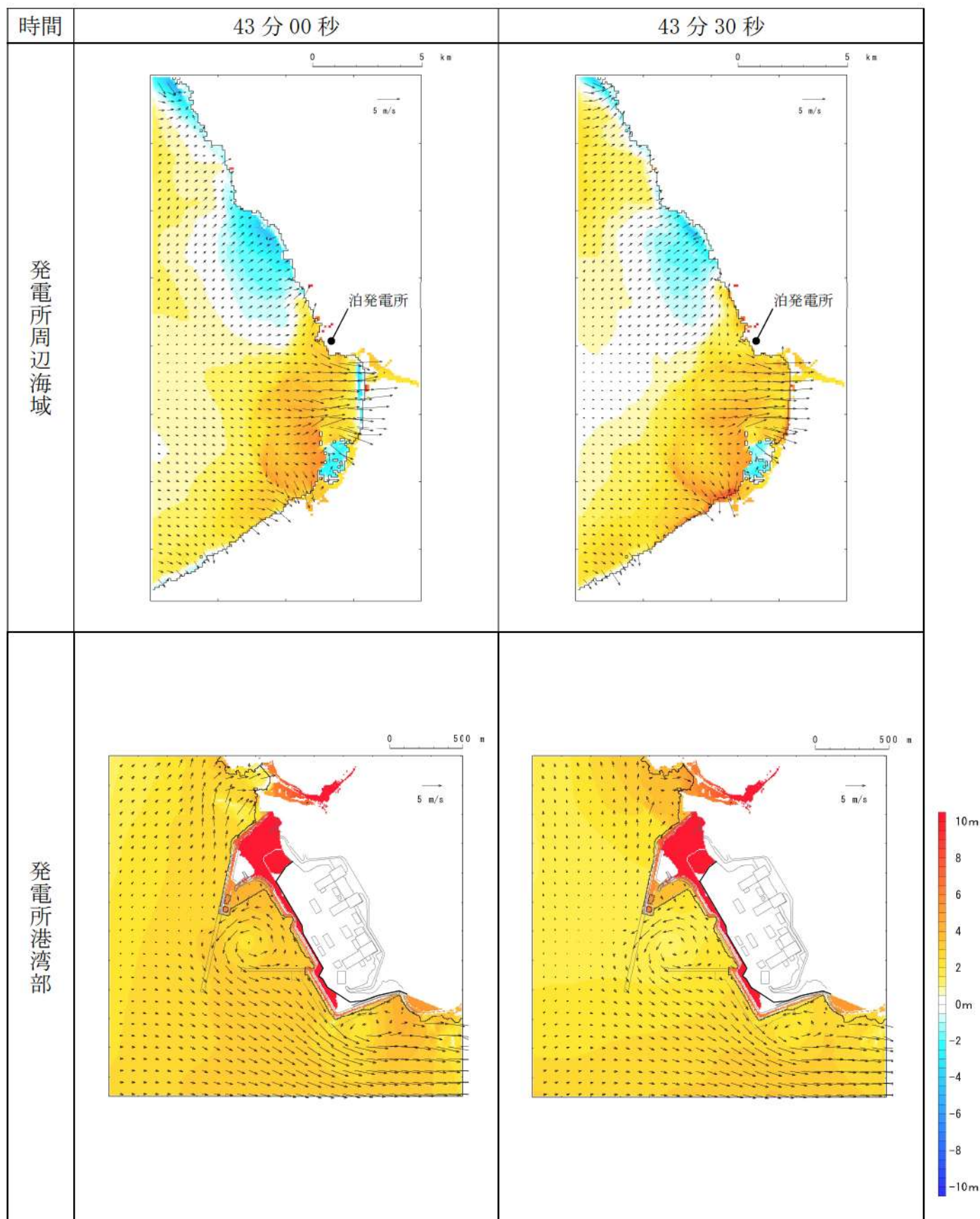
第 16 図-32 基準津波 J（北及び南防波堤損傷）の水位変動・流向ベクトル(32/49)
