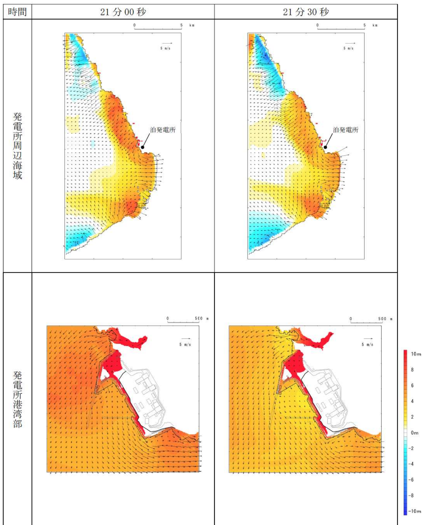
第 16 図-10 基準津波 J（北及び南防波堤損傷）の水位変動・流向ベクトル(10/49)
