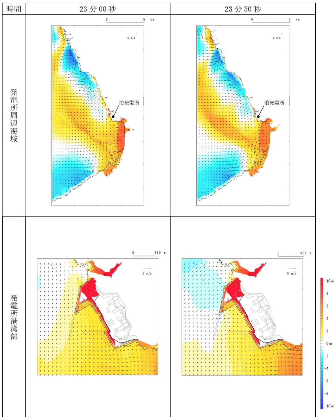
第 16 図-12 基準津波 J（北及び南防波堤損傷）の水位変動・流向ベクトル(12/49)
