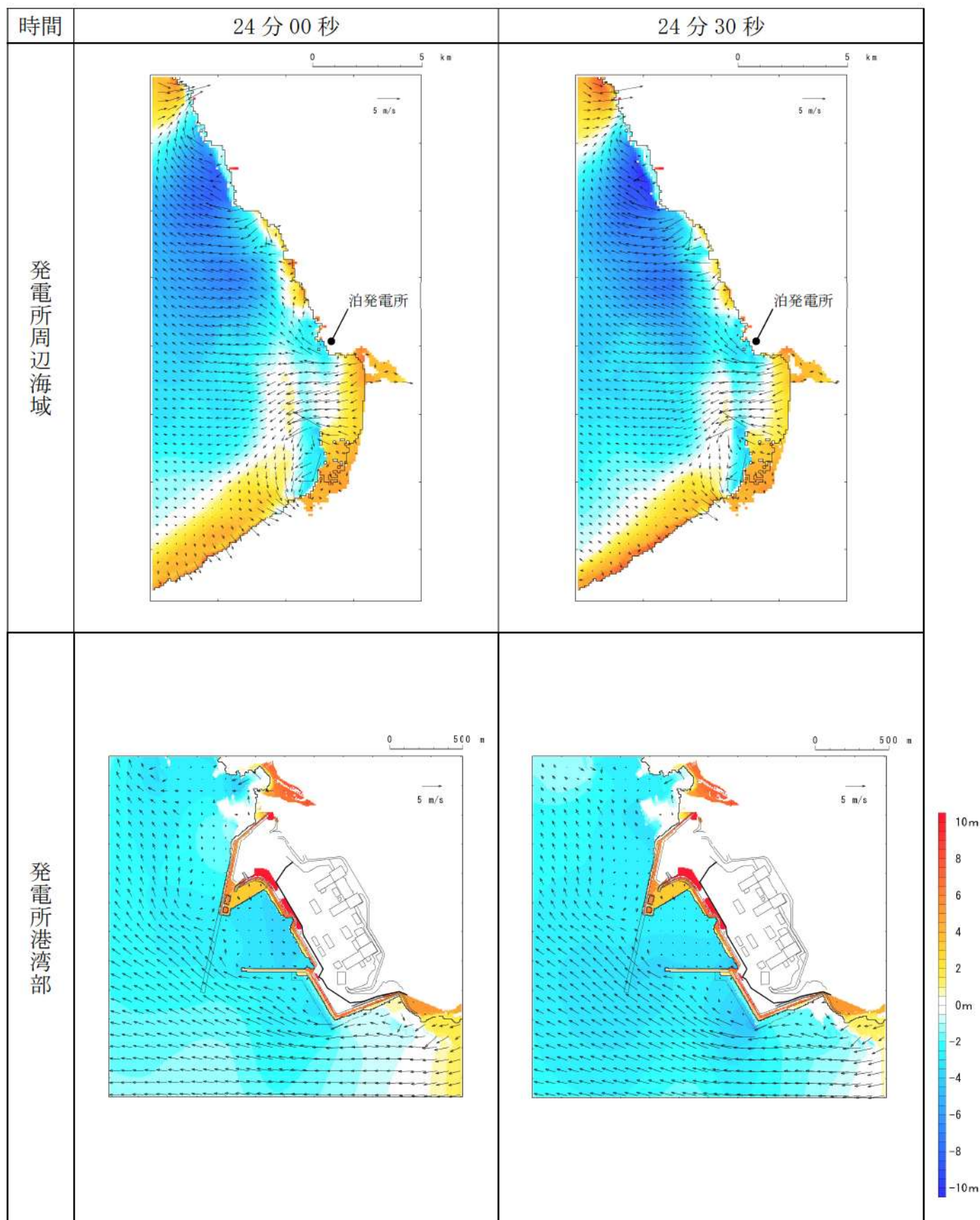
第 18 図-17 基準津波 L（北防波堤損傷）の水位変動・流向ベクトル(17/53)
