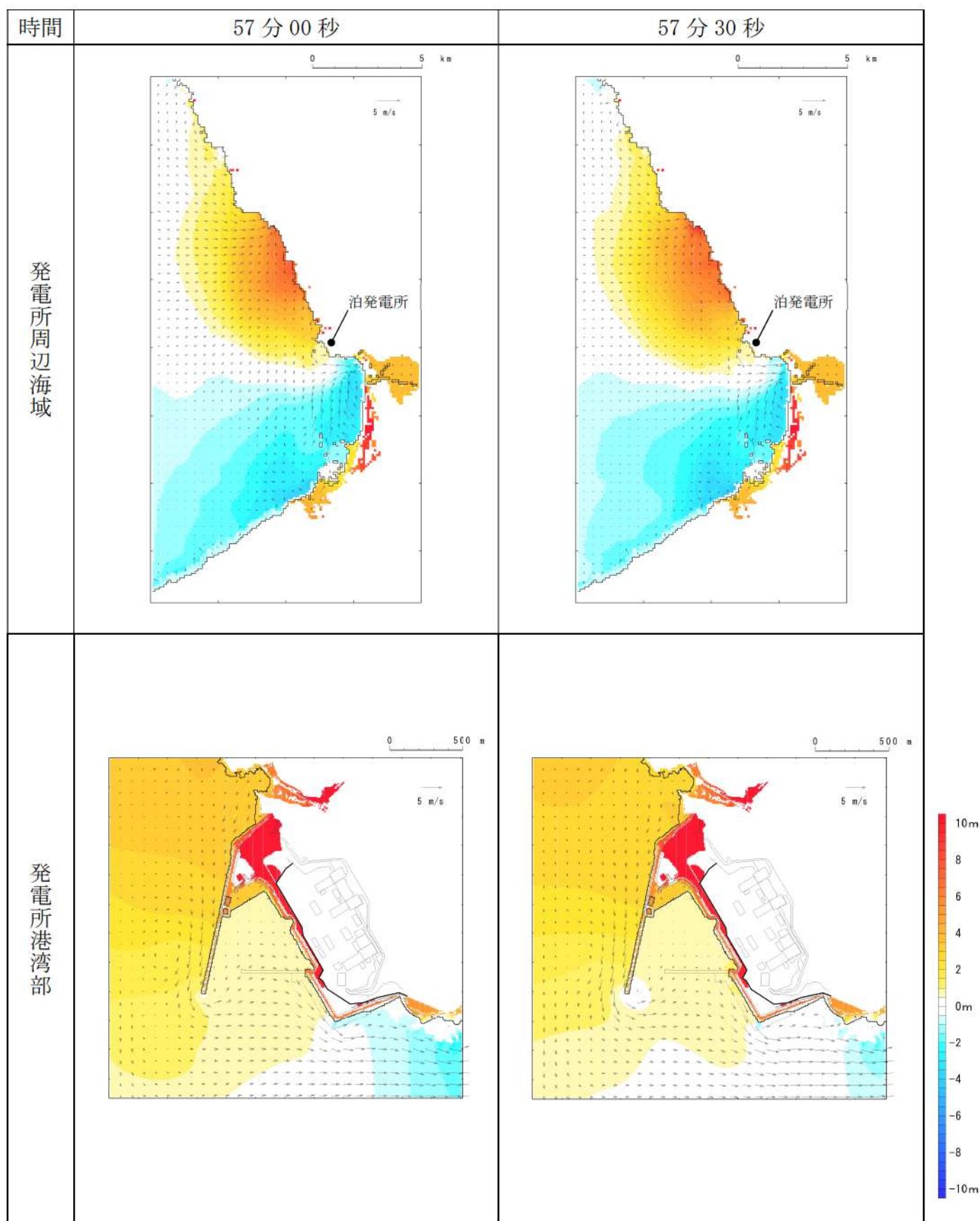
第 17 図-50 基準津波K（南防波堤損傷）の水位変動・流向ベクトル(50/53)
