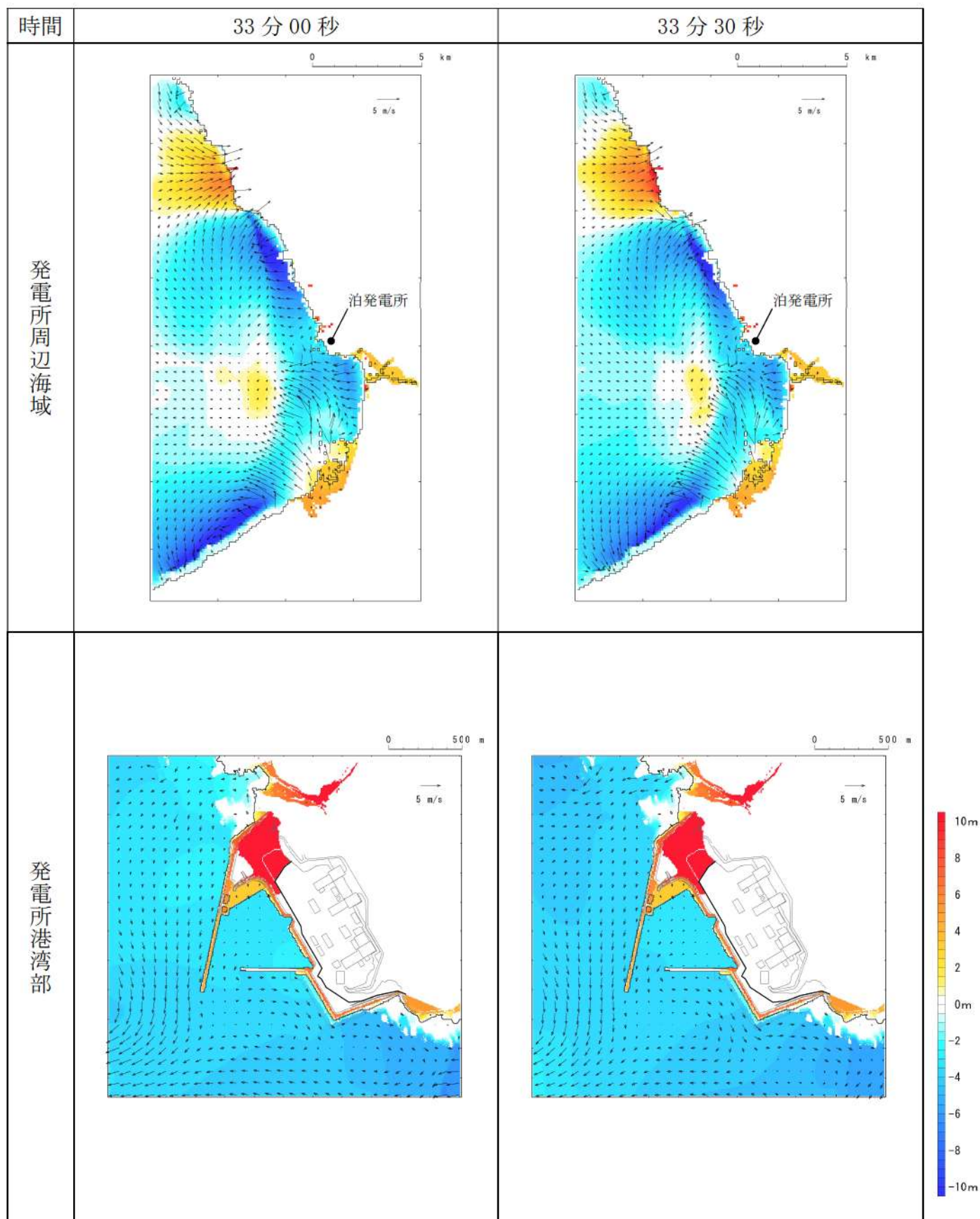
第 15 図-23 基準津波 I（防波堤損傷なし）の水位変動・流向ベクトル(23/50)
