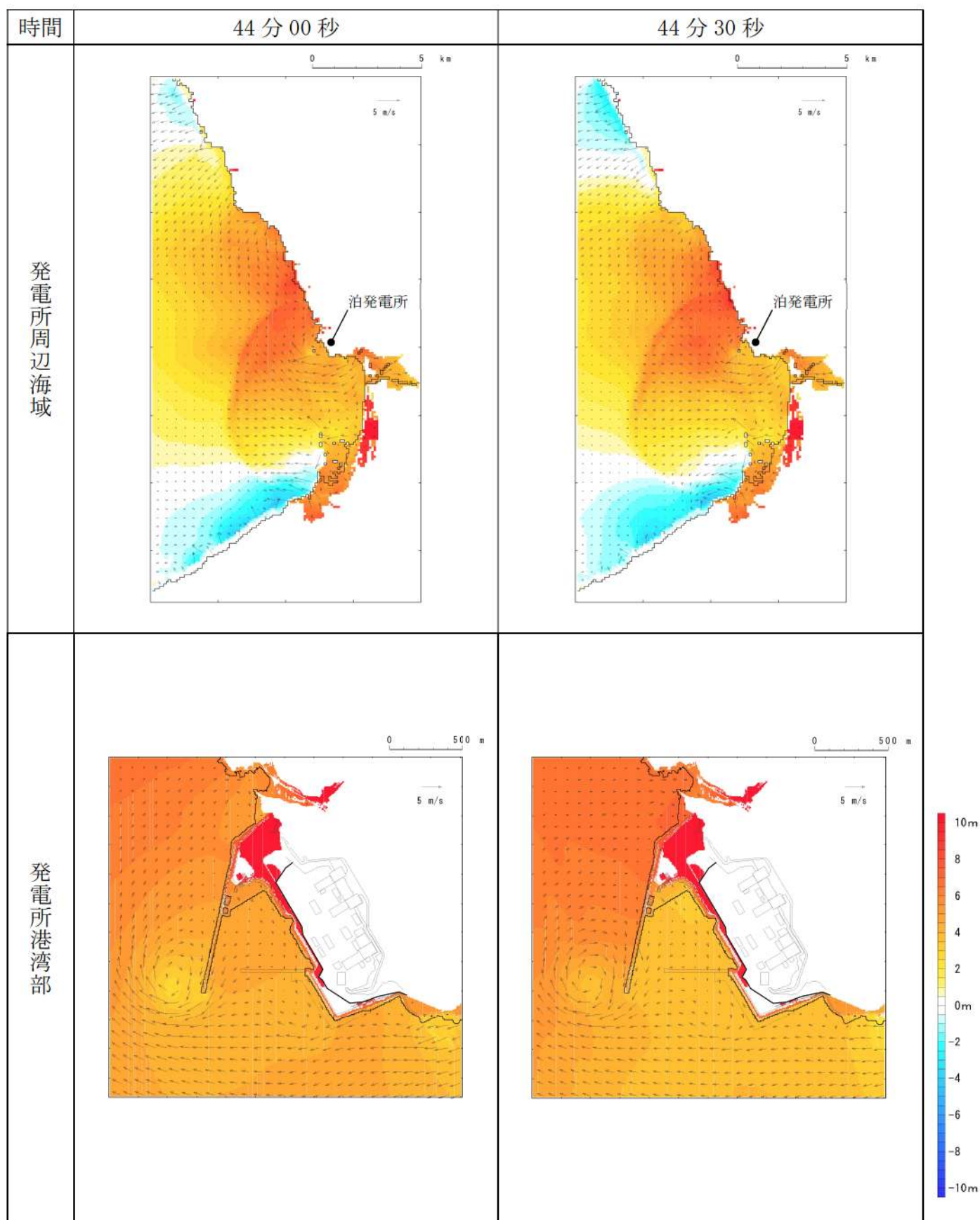
第 17 図-37 基準津波K（南防波堤損傷）の水位変動・流向ベクトル(37/53)
