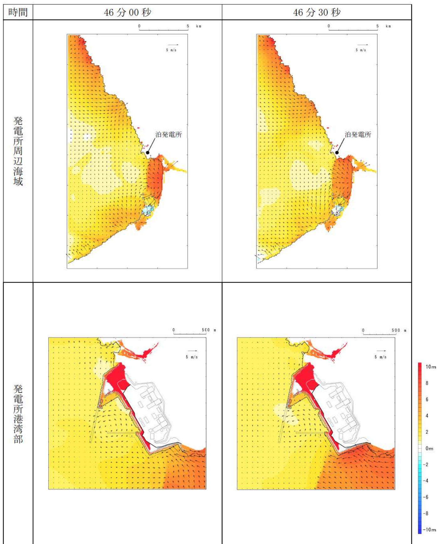
第 16 図-35 基準津波 J（北及び南防波堤損傷）の水位変動・流向ベクトル(35/49)
