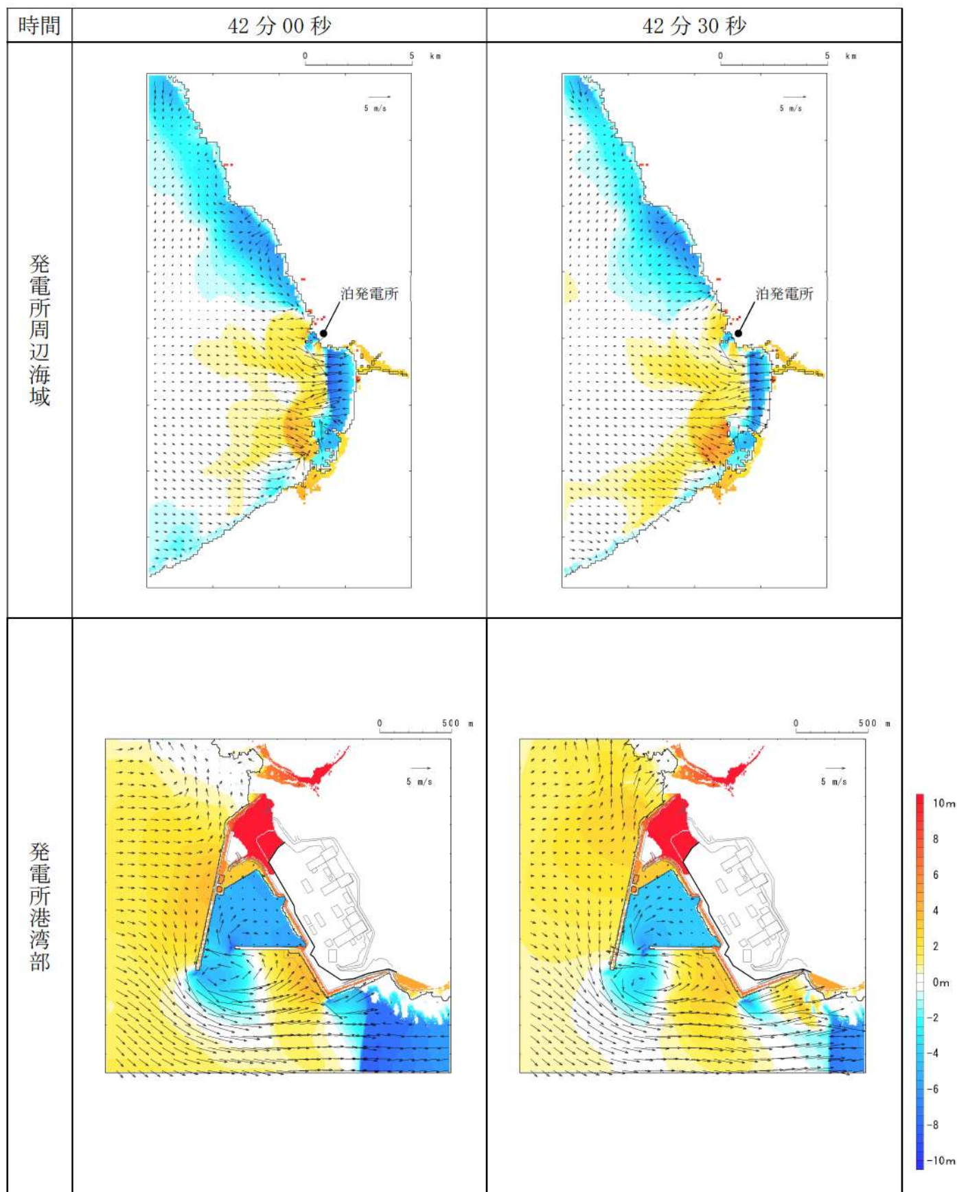
第 15 図-32 基準津波 I（防波堤損傷なし）の水位変動・流向ベクトル(32/50)
