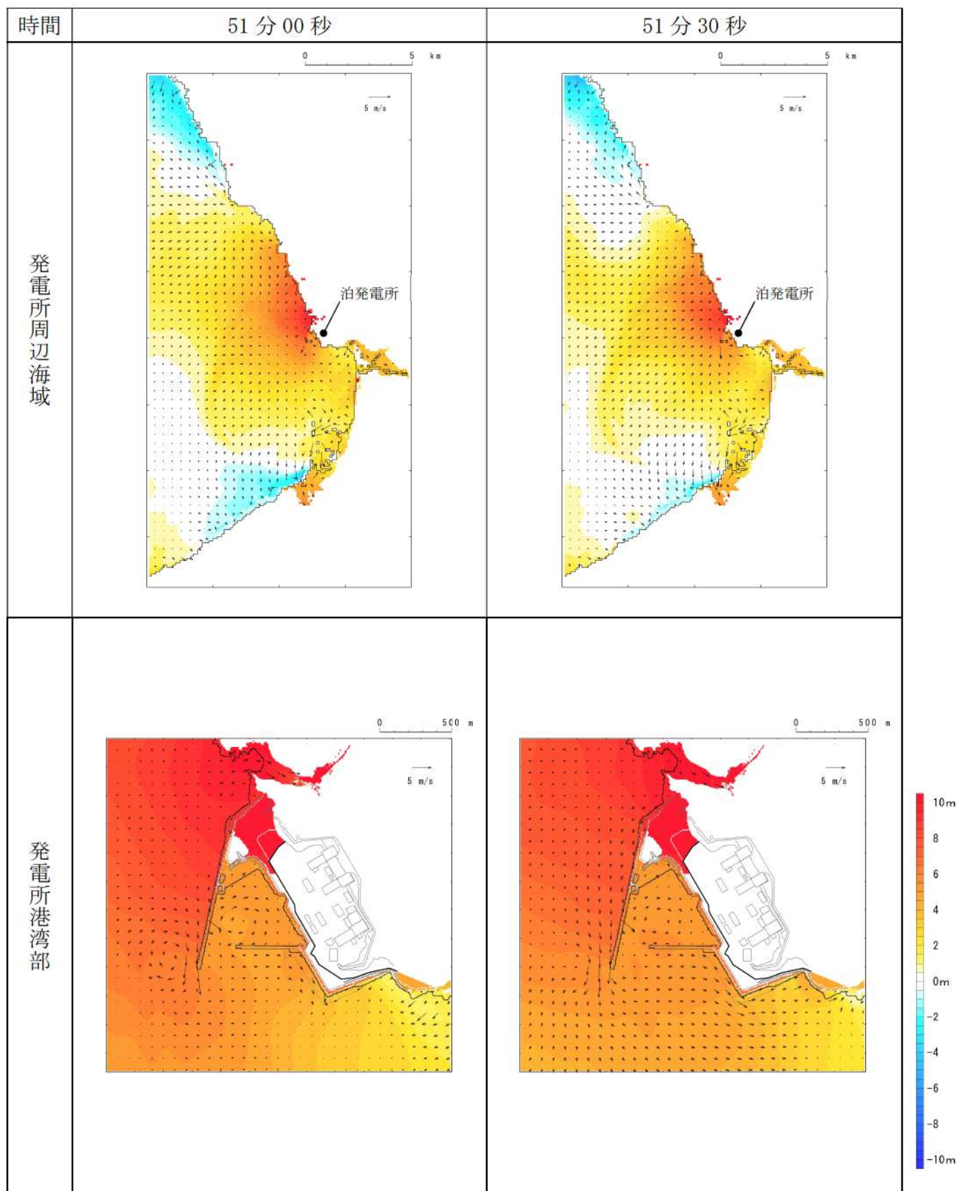
第 15 図-41 基準津波 I（防波堤損傷なし）の水位変動・流向ベクトル(41/50)
