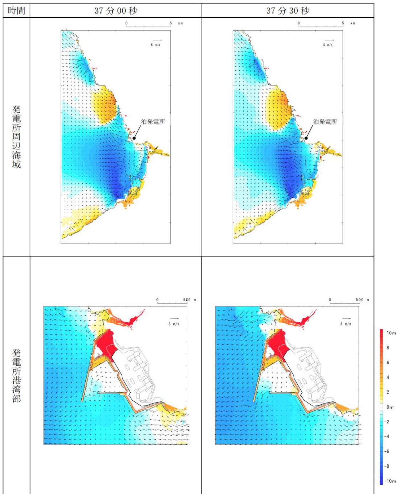
第 15 図-27 基準津波 I（防波堤損傷なし）の水位変動・流向ベクトル(27/50)
