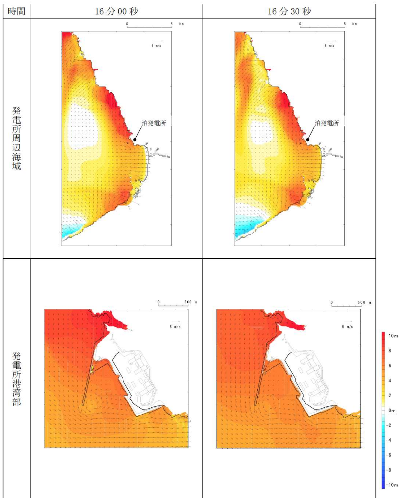
第 17 図-9 基準津波K（南防波堤損傷）の水位変動・流向ベクトル(9/53)
