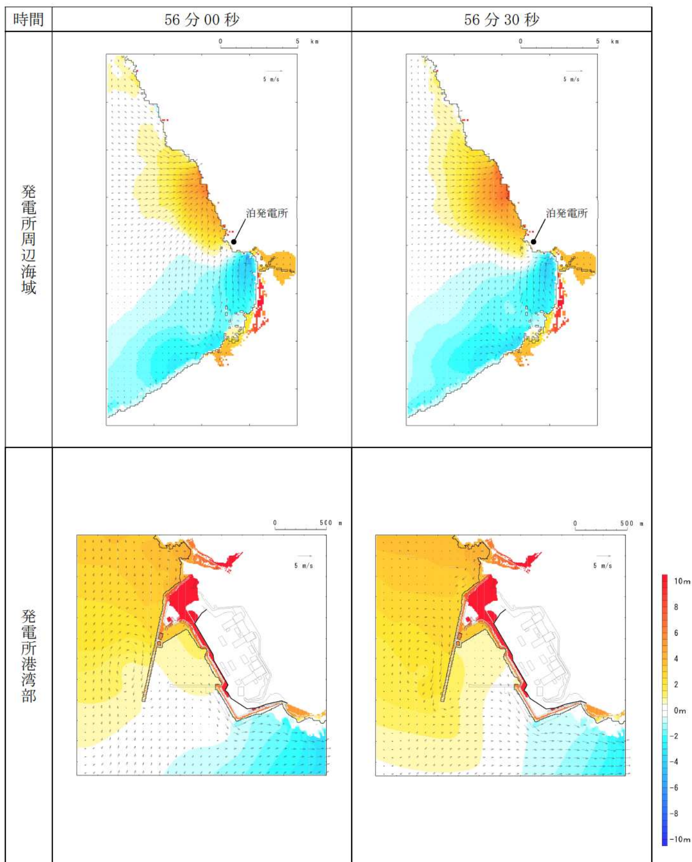
第 17 図-49 基準津波K（南防波堤損傷）の水位変動・流向ベクトル(49/53)
