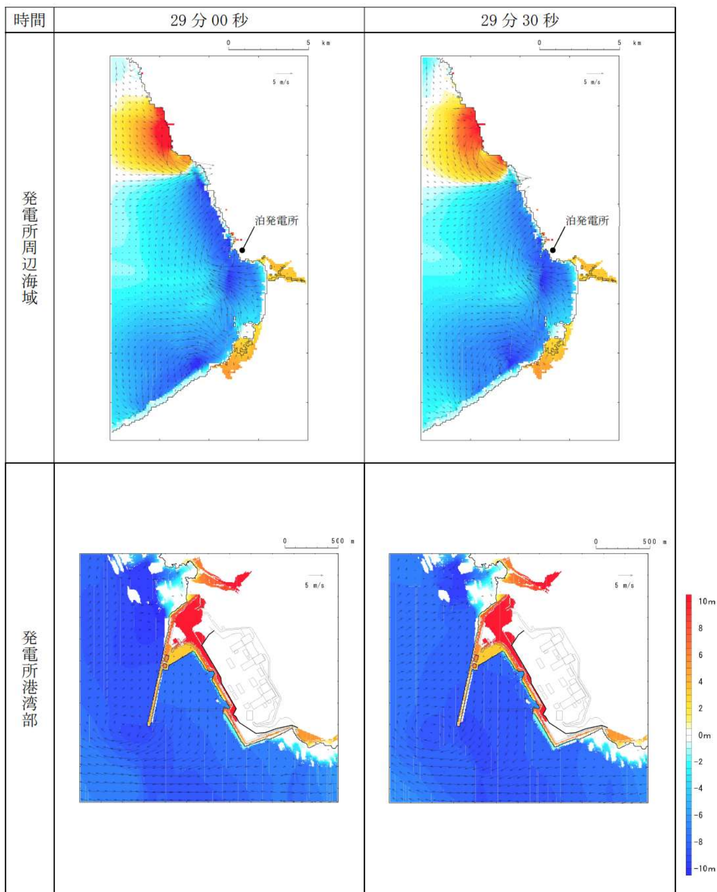
第 17 図-22 基準津波K（南防波堤損傷）の水位変動・流向ベクトル(22/53)
