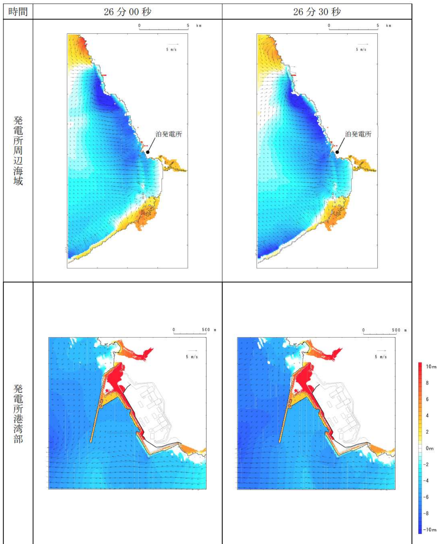
第 17 図-19 基準津波K（南防波堤損傷）の水位変動・流向ベクトル(19/53)
