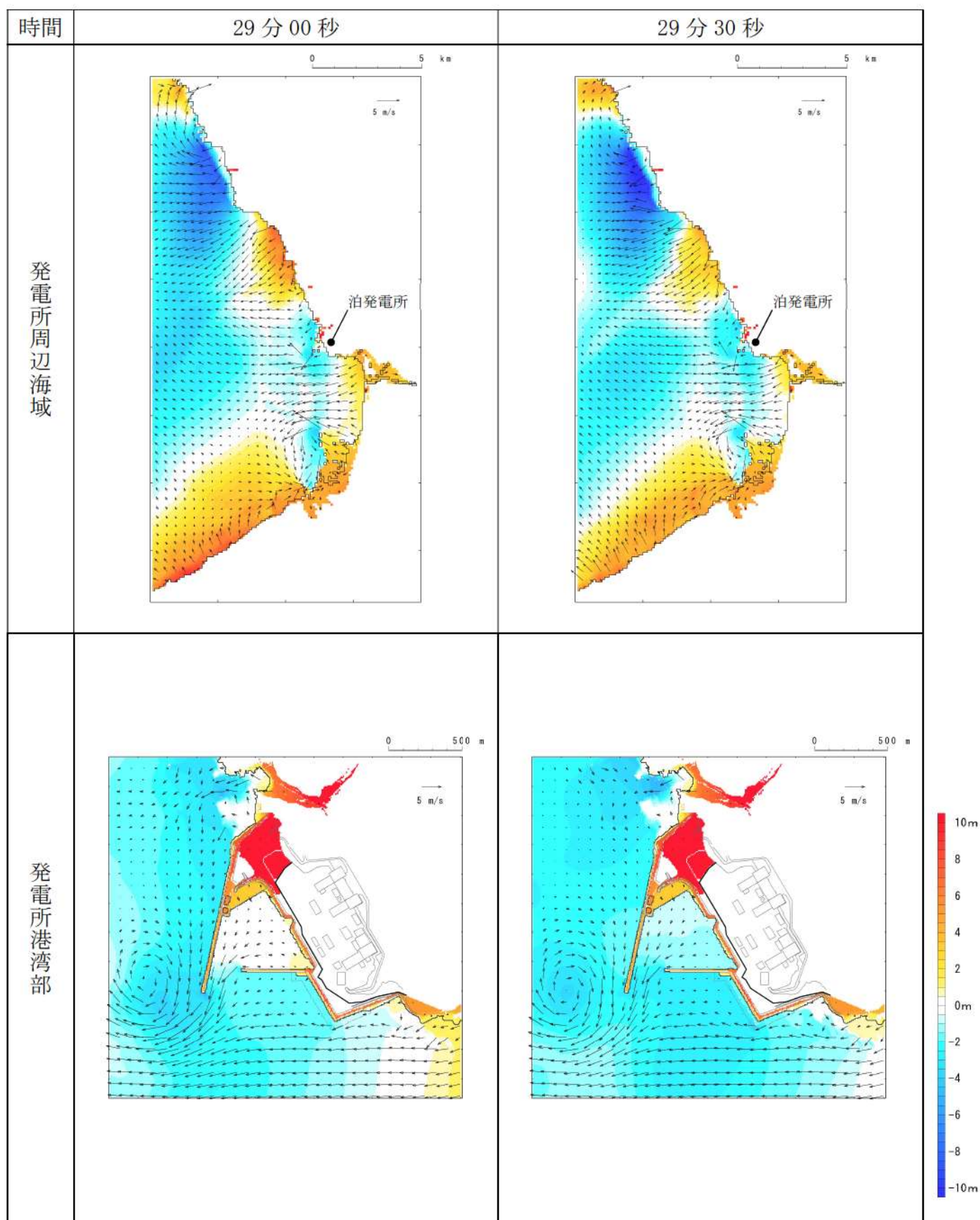
第 15 図-19 基準津波 I（防波堤損傷なし）の水位変動・流向ベクトル(19/50)
