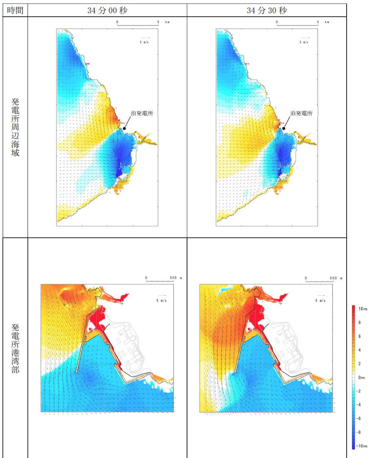
第 17 図-27 基準津波K（南防波堤損傷）の水位変動・流向ベクトル(27/53)
