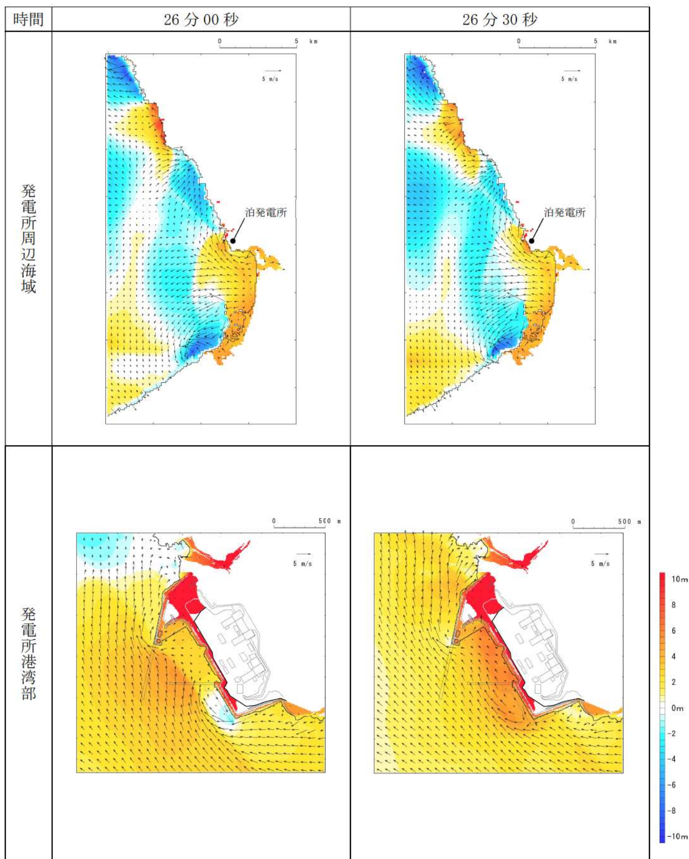
第 16 図-15 基準津波 J（北及び南防波堤損傷）の水位変動・流向ベクトル(15/49)
