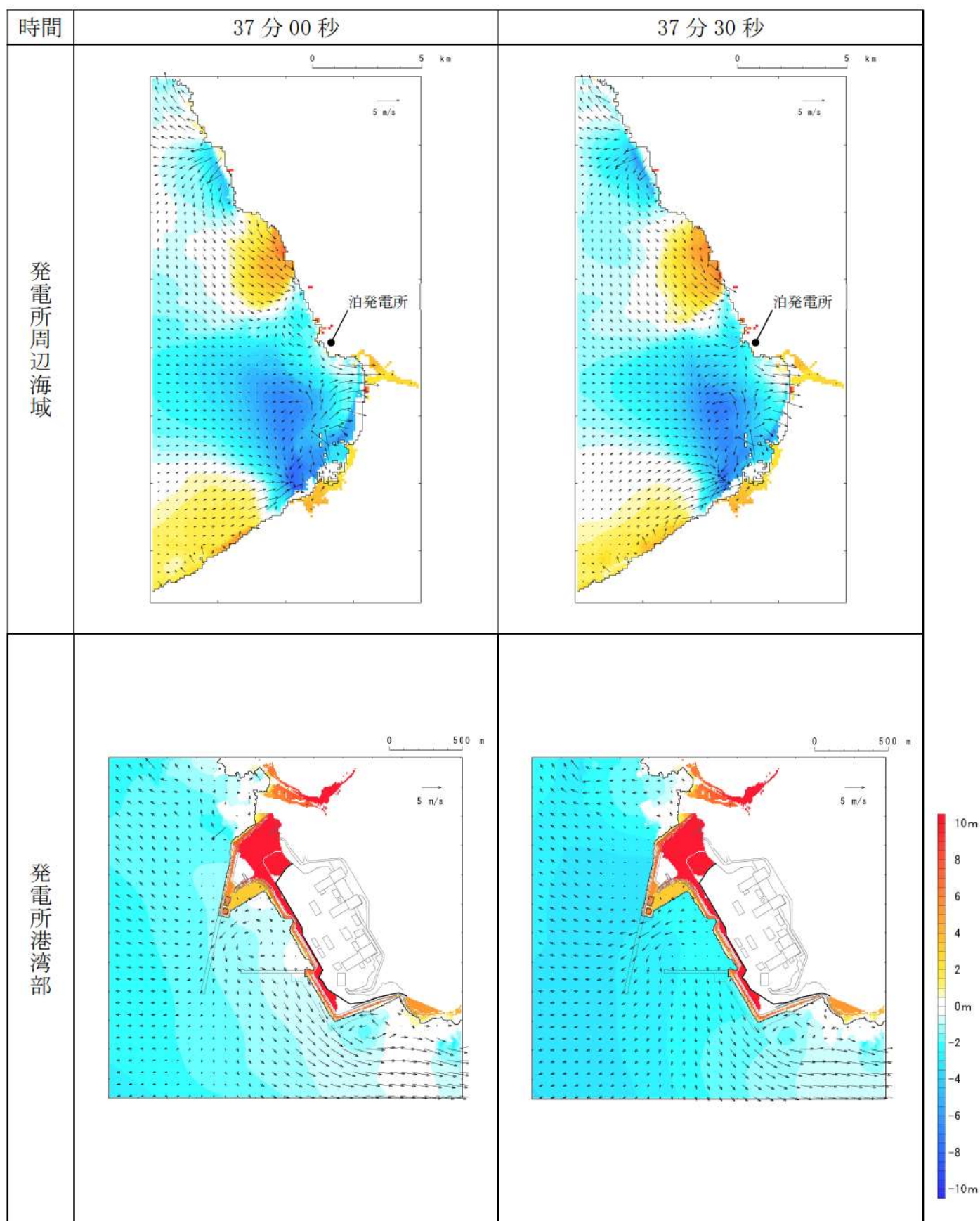
第 16 図-26 基準津波 J（北及び南防波堤損傷）の水位変動・流向ベクトル(26/49)
