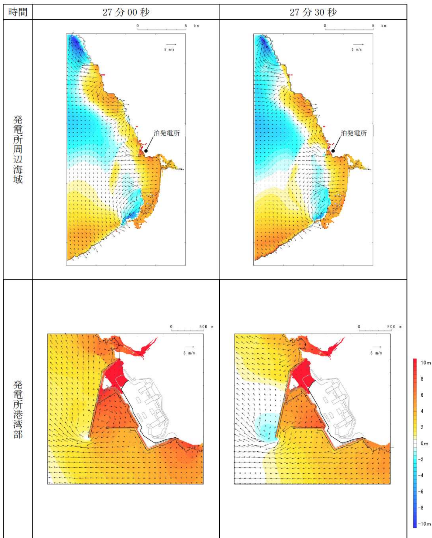
第 15 図-17 基準津波 I（防波堤損傷なし）の水位変動・流向ベクトル(17/50)
