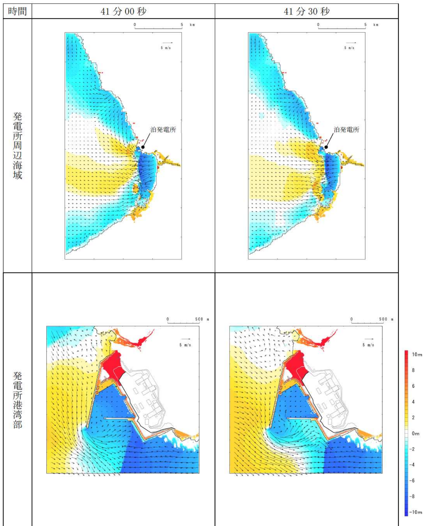
第 15 図-31 基準津波 I（防波堤損傷なし）の水位変動・流向ベクトル(31/50)
