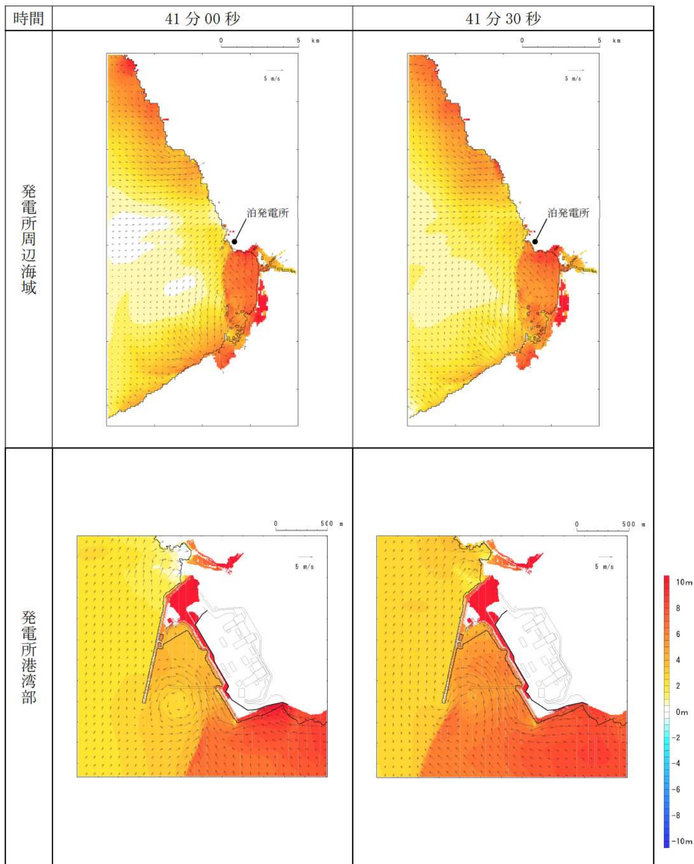
第 17 図-34 基準津波K（南防波堤損傷）の水位変動・流向ベクトル(34/53)
