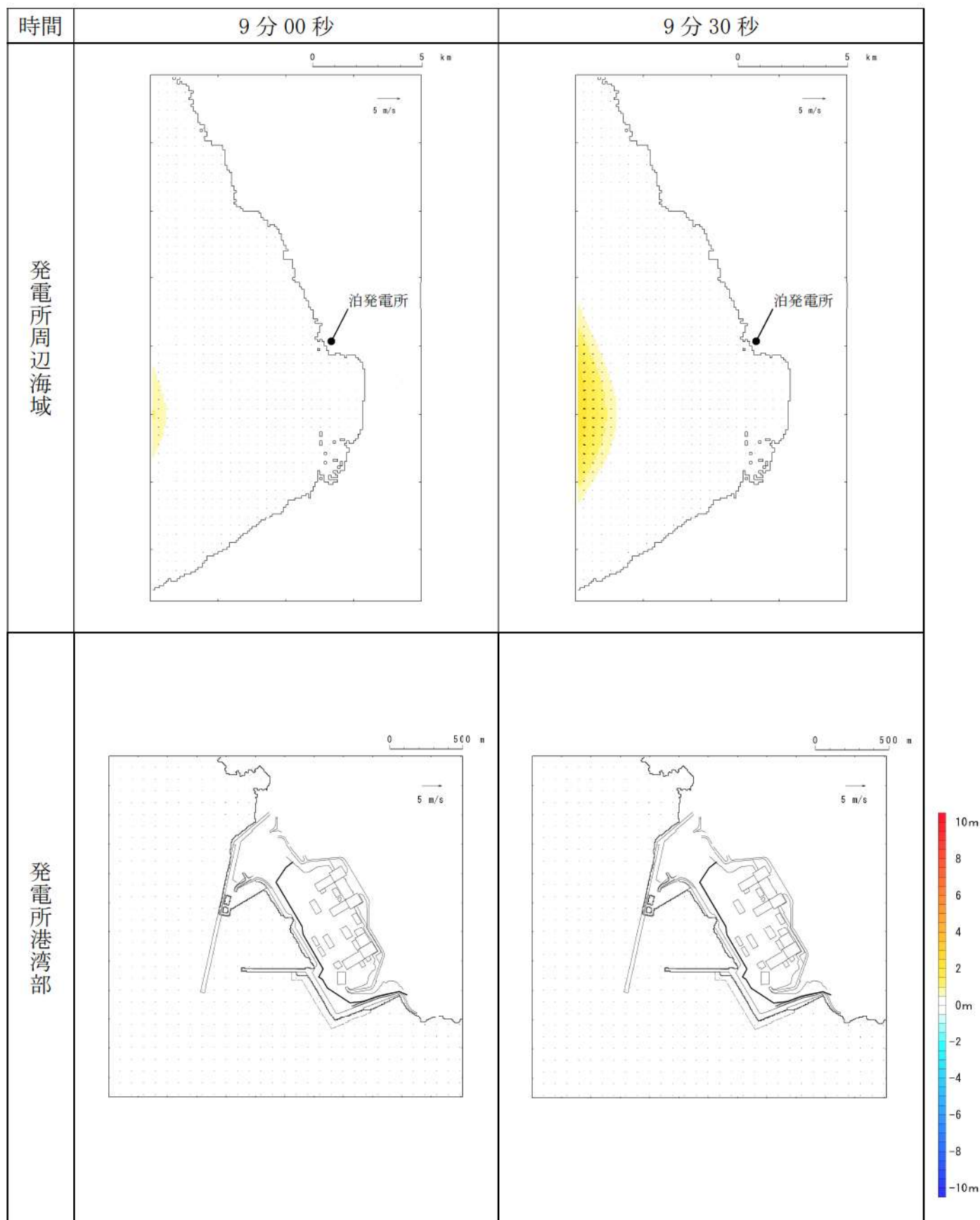
第 18 図-2 基準津波 L（北防波堤損傷）の水位変動・流向ベクトル (2/53)
