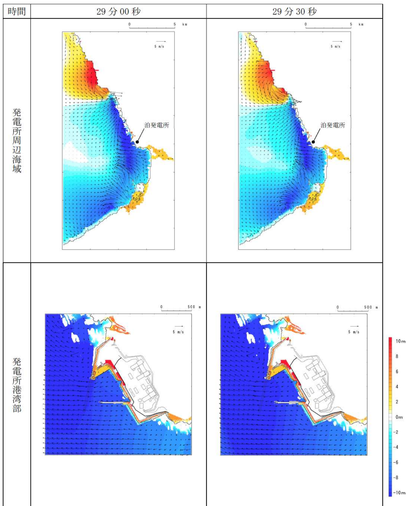
第 18 図-22 基準津波 L（北防波堤損傷）の水位変動・流向ベクトル(22/53)
