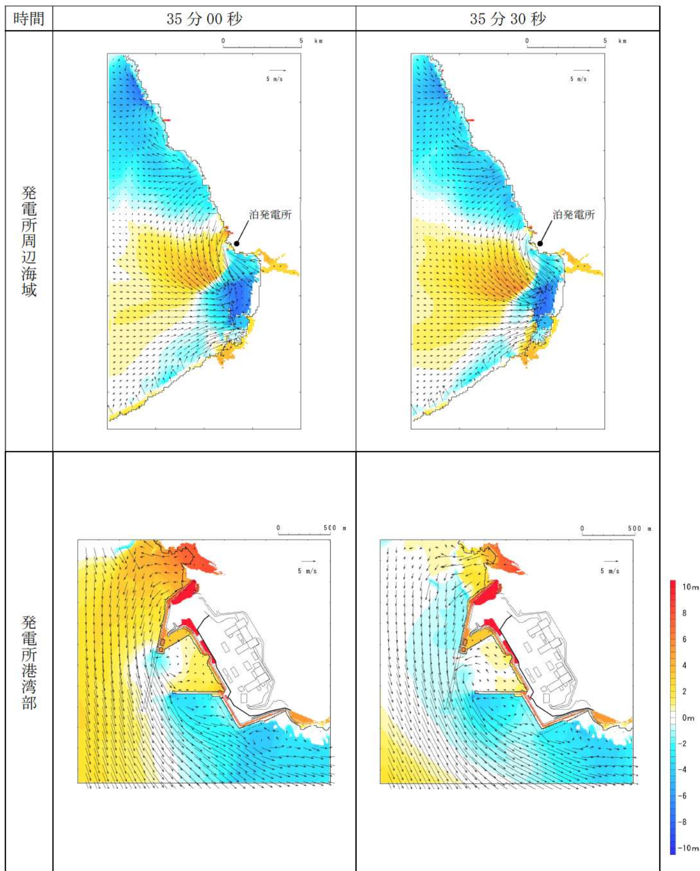
第 18 図-28 基準津波 L（北防波堤損傷）の水位変動・流向ベクトル (28/53)
