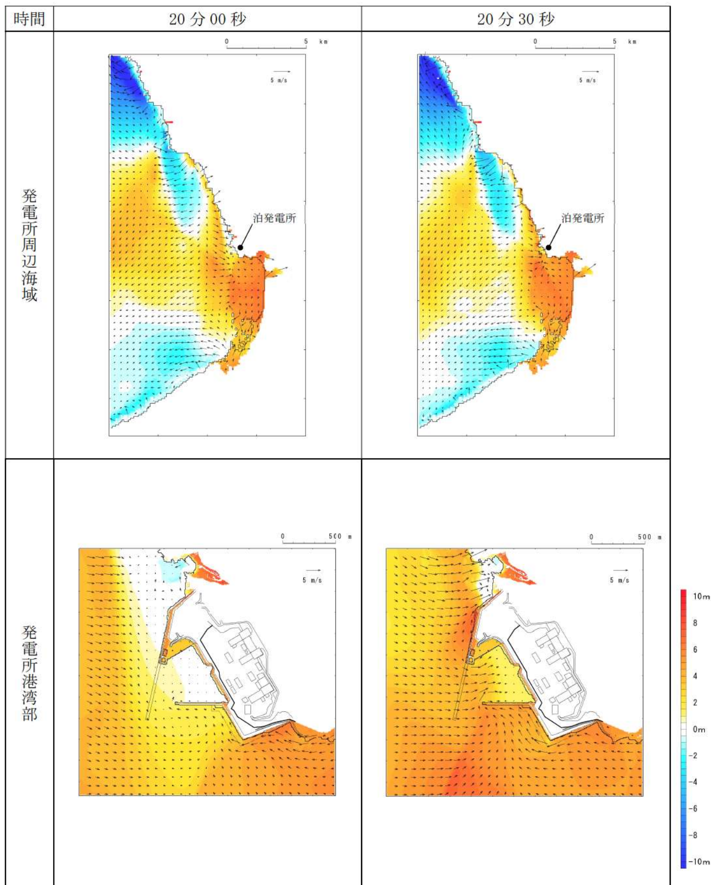
第 18 図-13 基準津波 L（北防波堤損傷）の水位変動・流向ベクトル(13/53)
