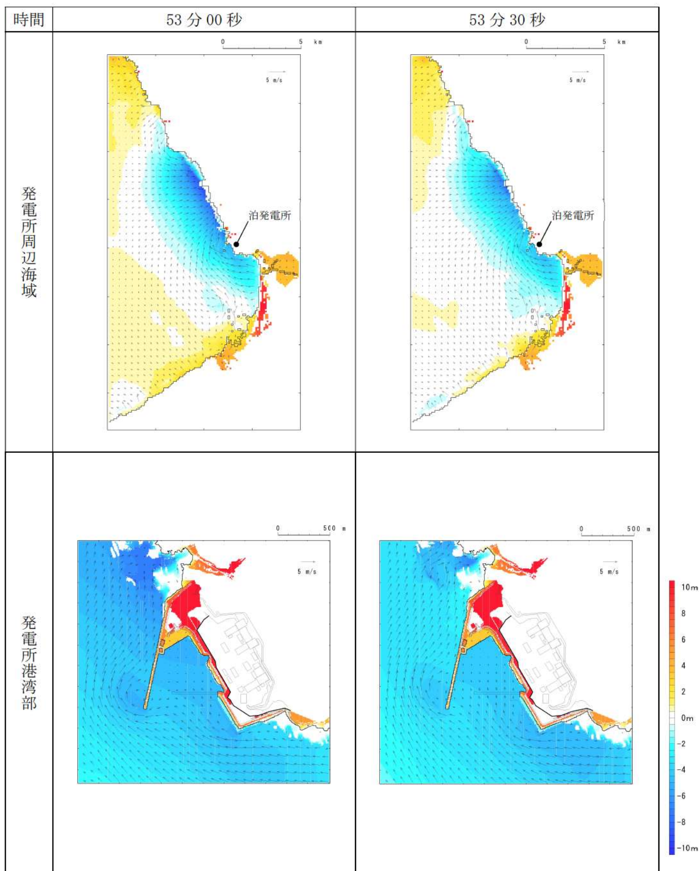
第 17 図-46 基準津波K（南防波堤損傷）の水位変動・流向ベクトル(46/53)
