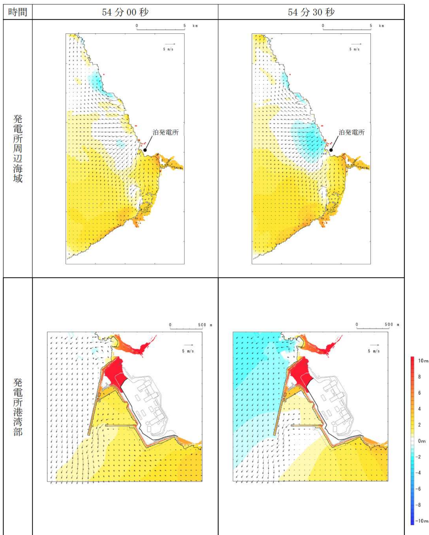
第 15 図-44 基準津波 I（防波堤損傷なし）の水位変動・流向ベクトル(44/50)
