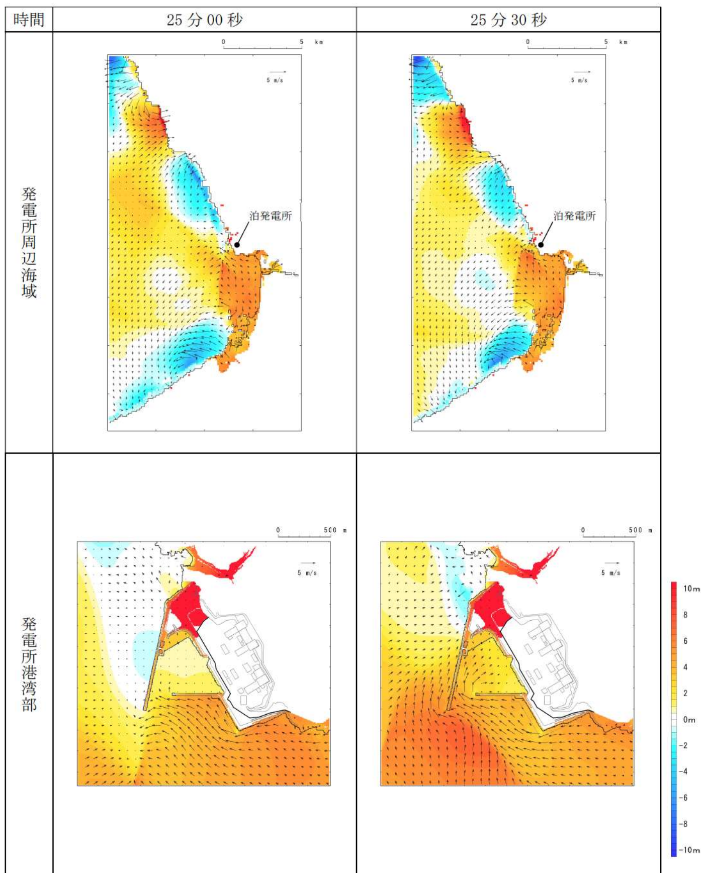
第 15 図-15 基準津波 I（防波堤損傷なし）の水位変動・流向ベクトル(15/50)
