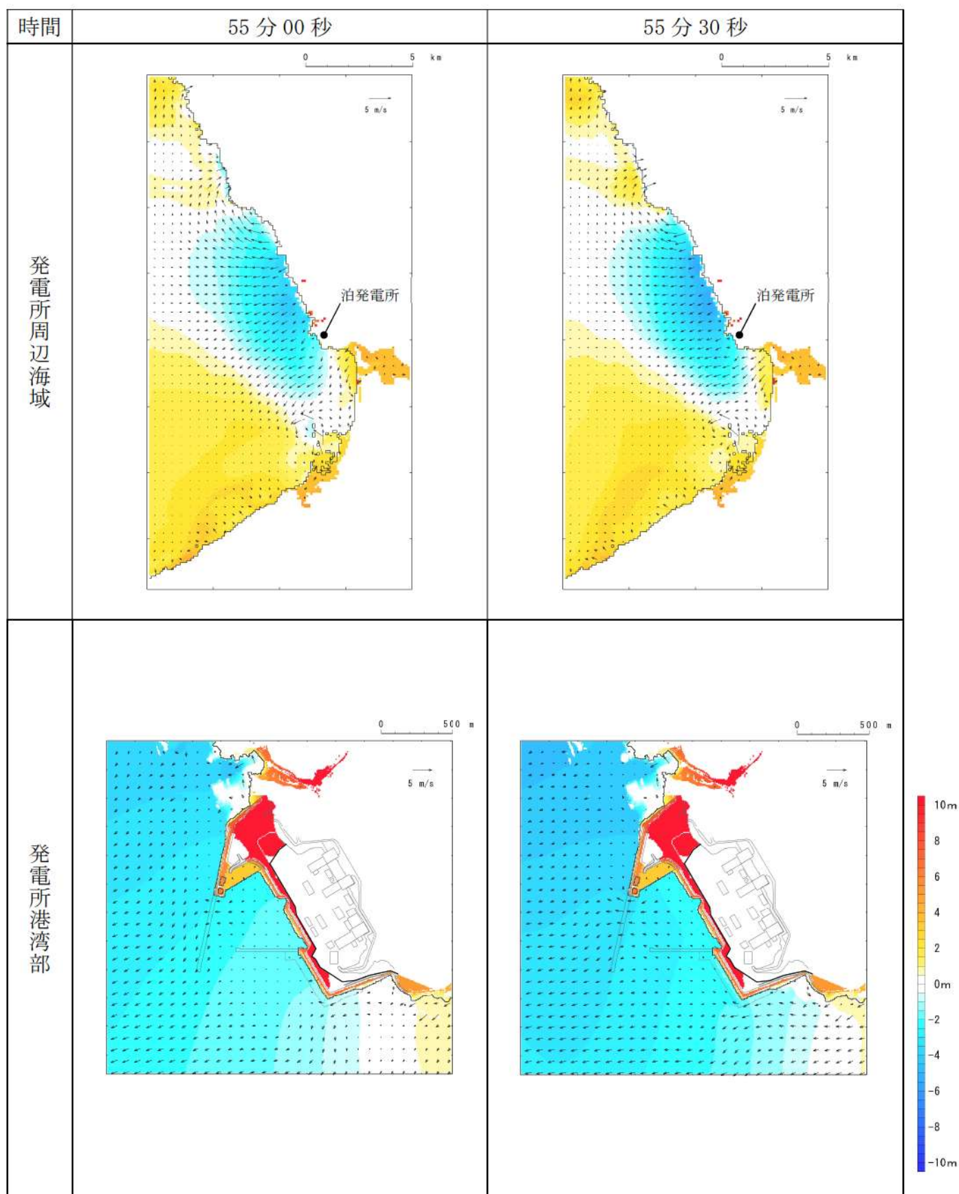
第 16 図-44 基準津波 J（北及び南防波堤損傷）の水位変動・流向ベクトル(44/49)
