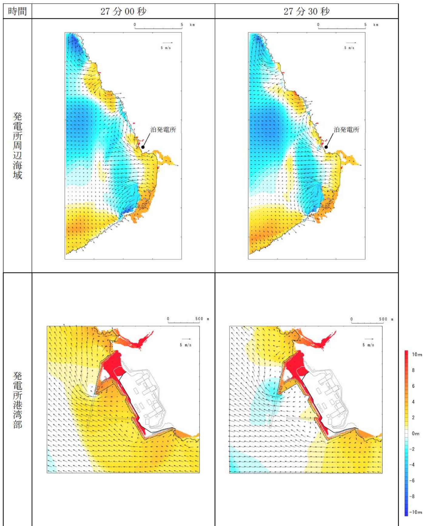
第 16 図-16 基準津波 J（北及び南防波堤損傷）の水位変動・流向ベクトル(16/49)
