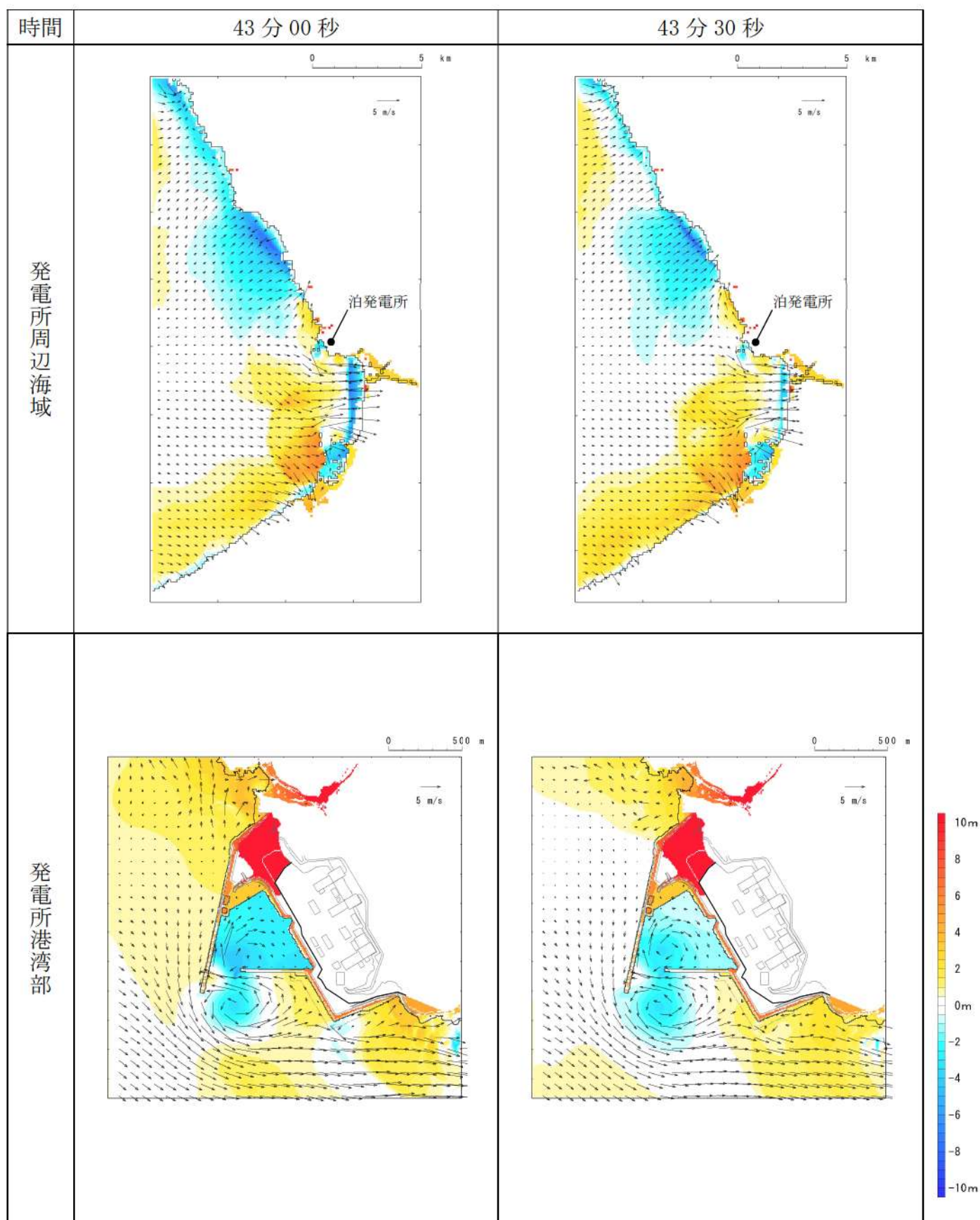
第 15 図-33 基準津波 I（防波堤損傷なし）の水位変動・流向ベクトル(33/50)
