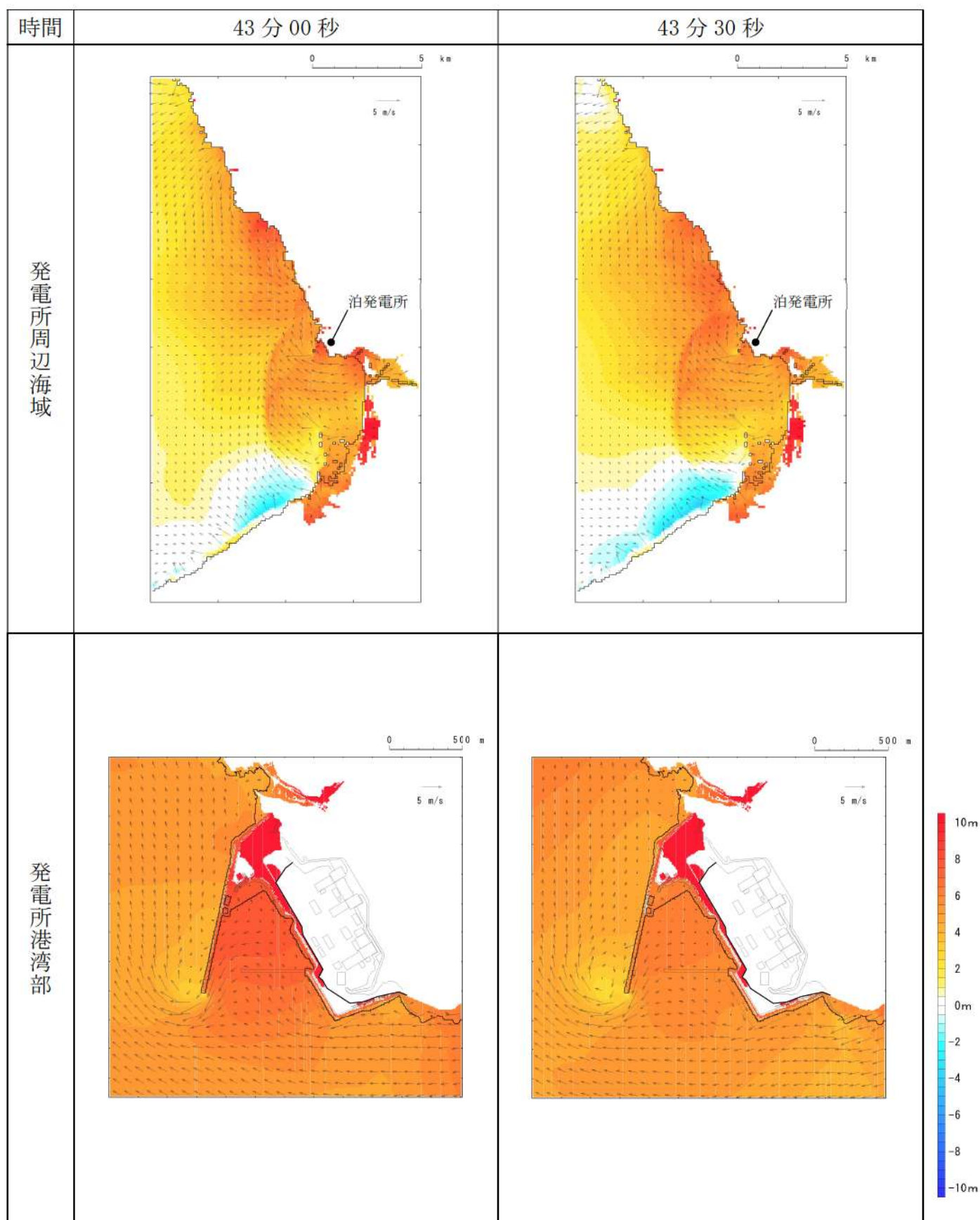
第 17 図-36 基準津波K（南防波堤損傷）の水位変動・流向ベクトル(36/53)
