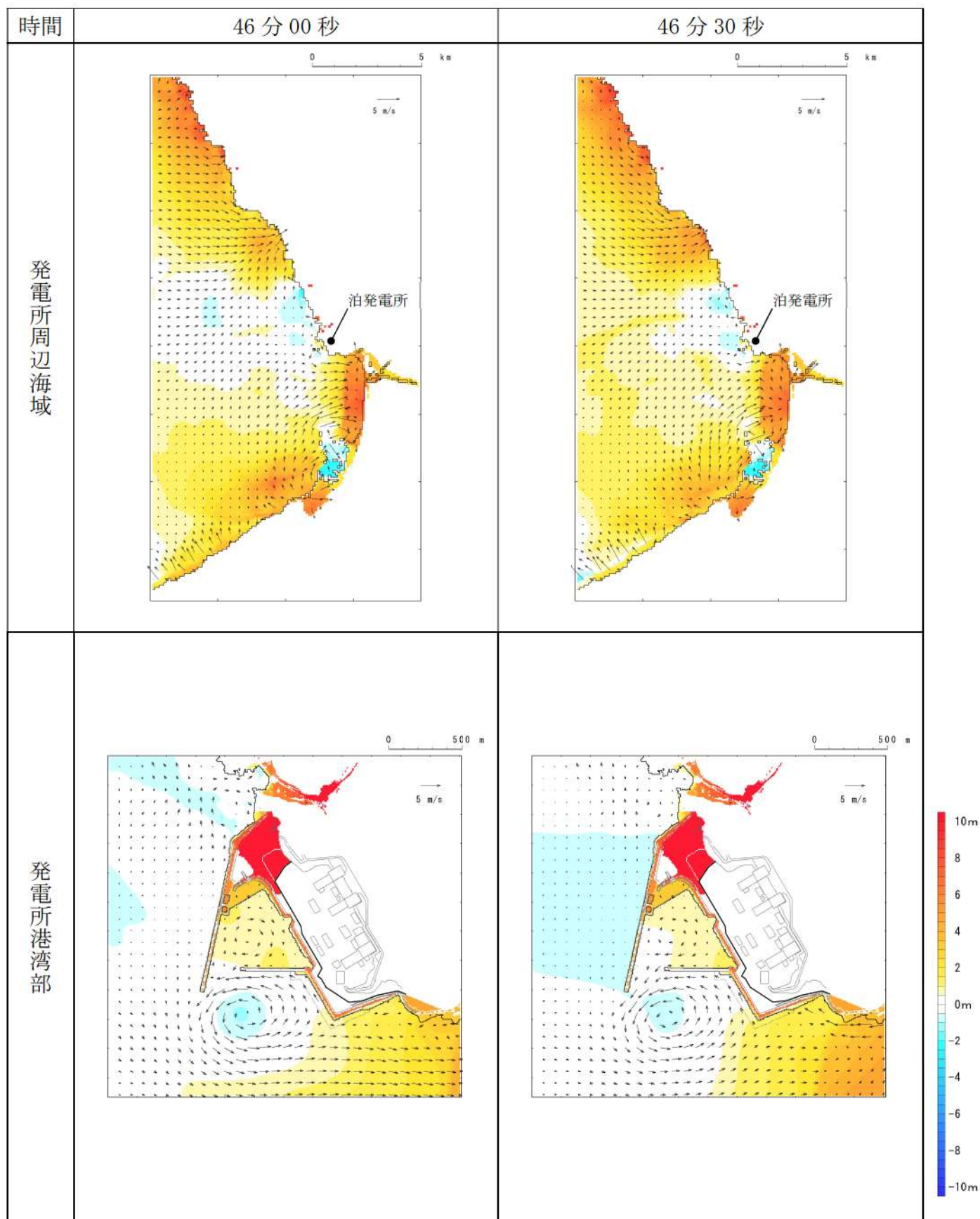
第 15 図-36 基準津波 I（防波堤損傷なし）の水位変動・流向ベクトル(36/50)
