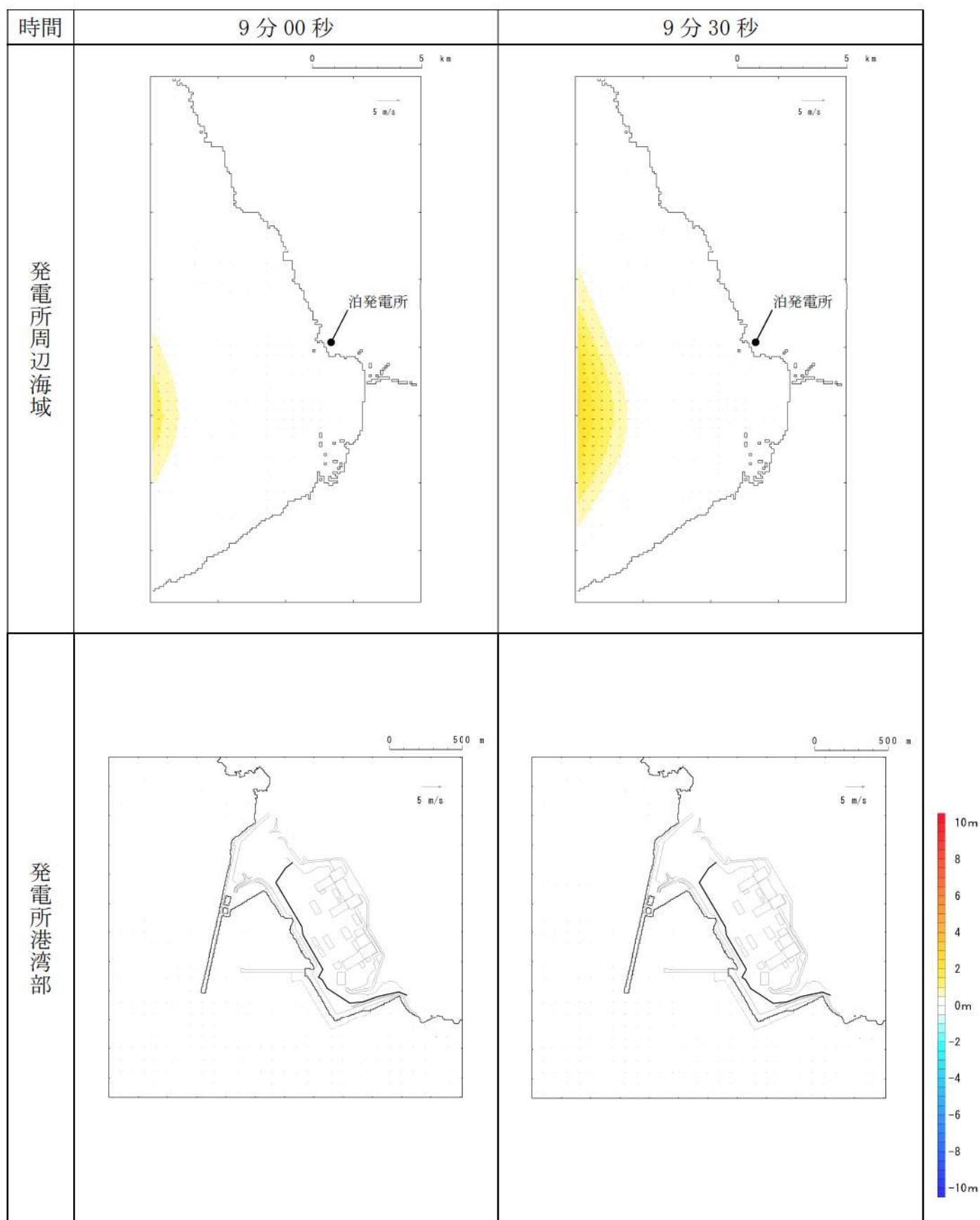
第 17 図-2 基準津波 K（南防波堤損傷）の水位変動・流向ベクトル (2/53)
