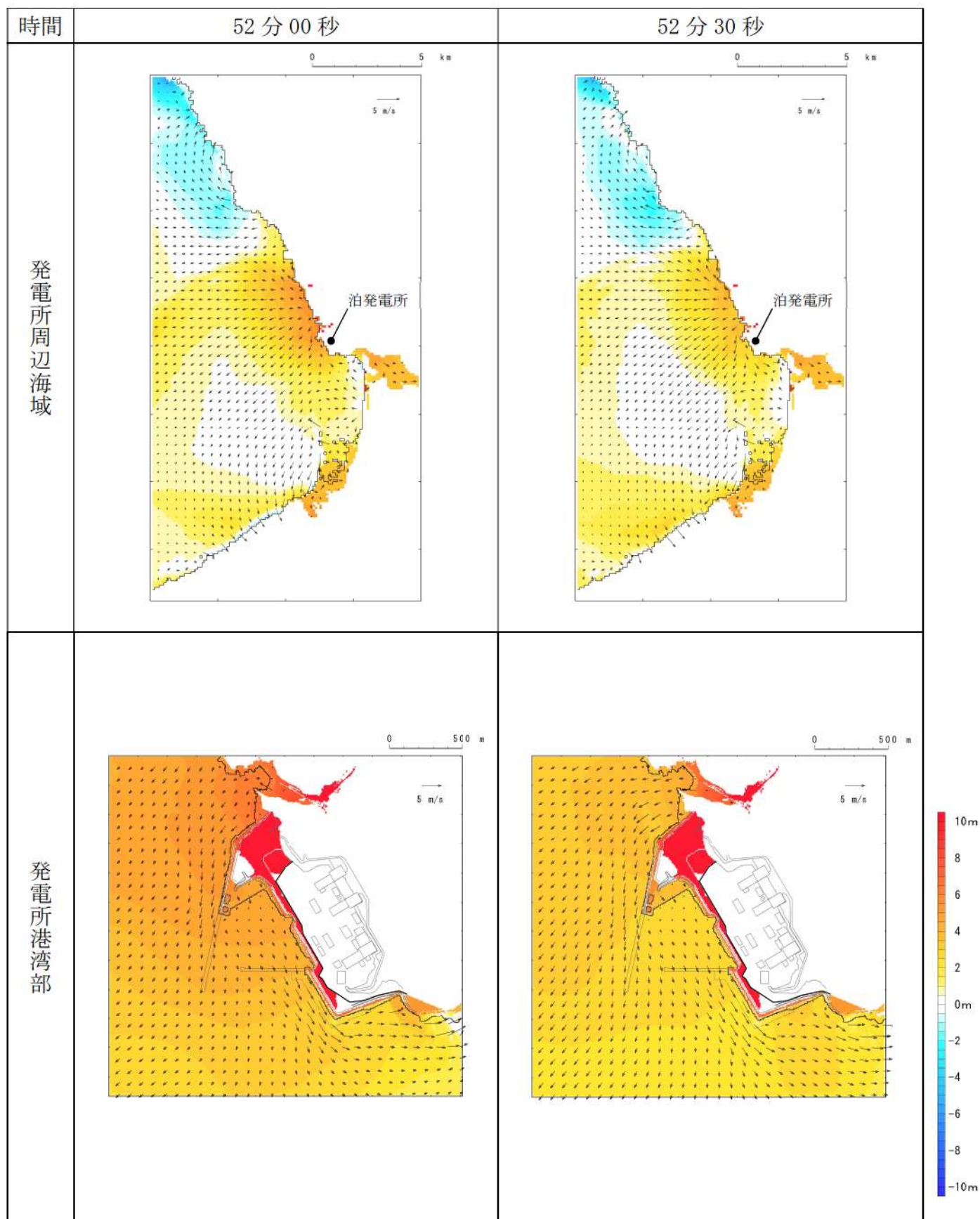
第 16 図-41 基準津波 J（北及び南防波堤損傷）の水位変動・流向ベクトル(41/49)
