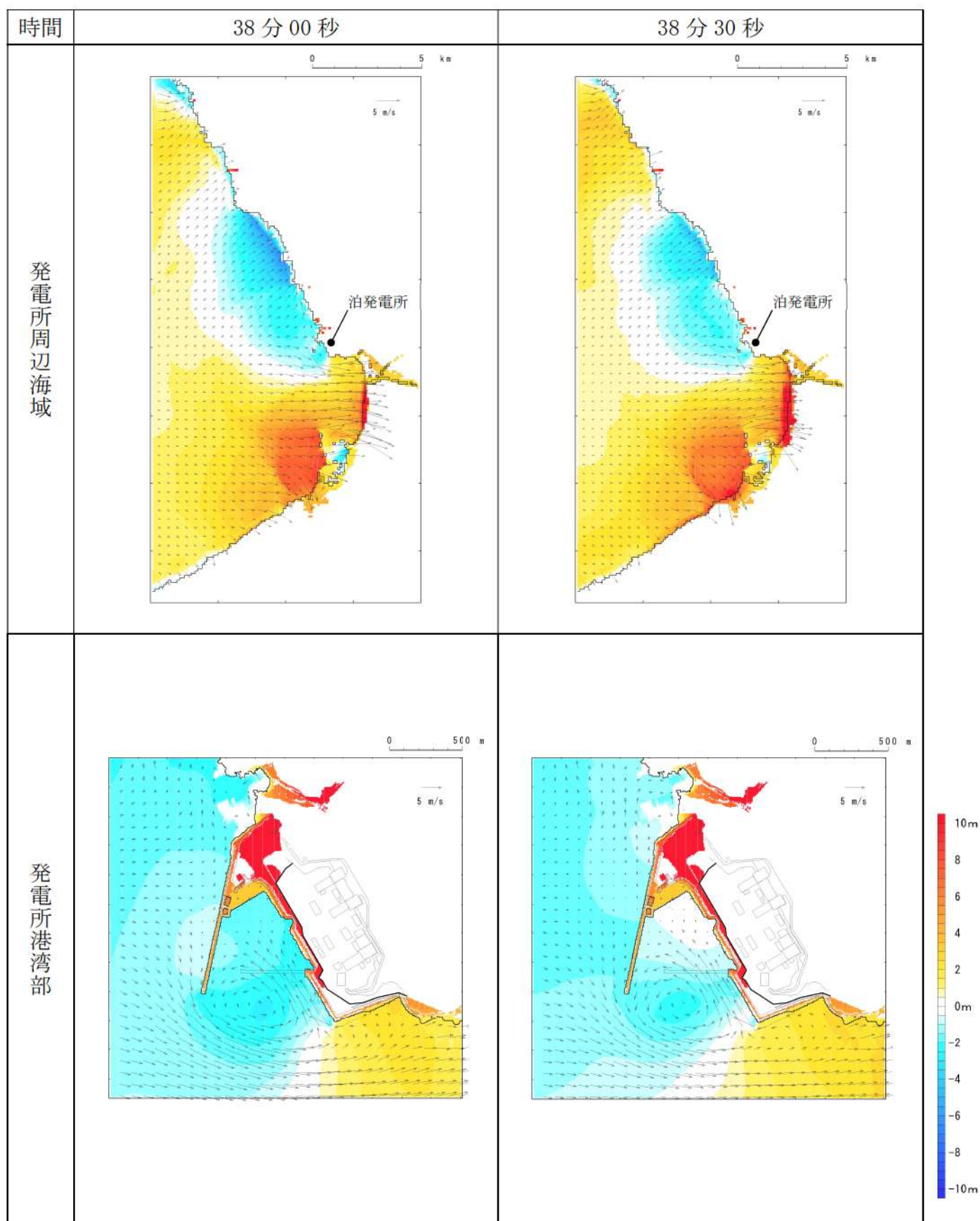
第 17 図-31 基準津波K（南防波堤損傷）の水位変動・流向ベクトル(31/53)
