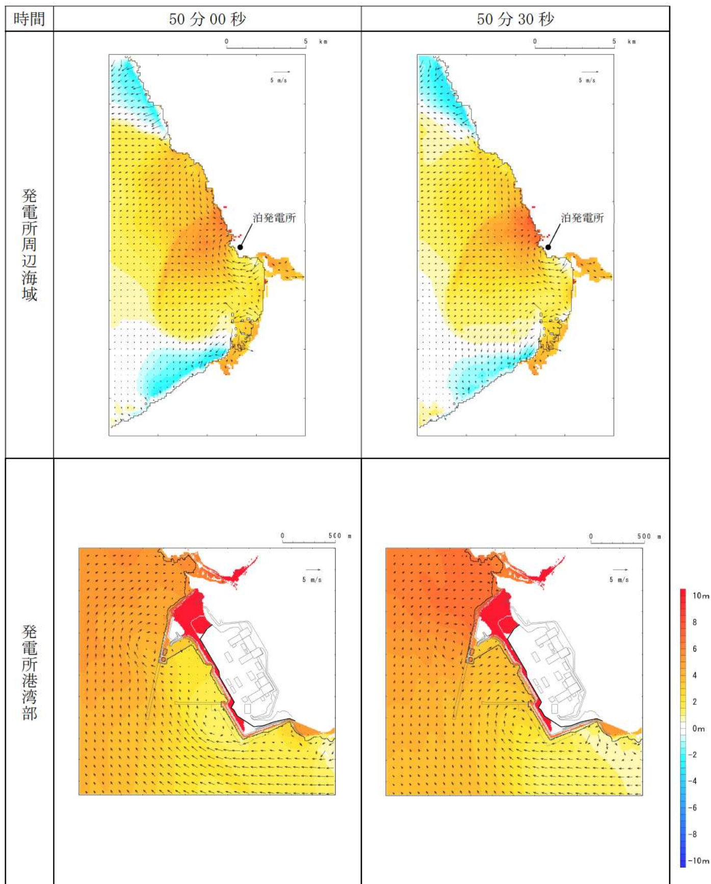
第 16 図-39 基準津波 J（北及び南防波堤損傷）の水位変動・流向ベクトル(39/49)
