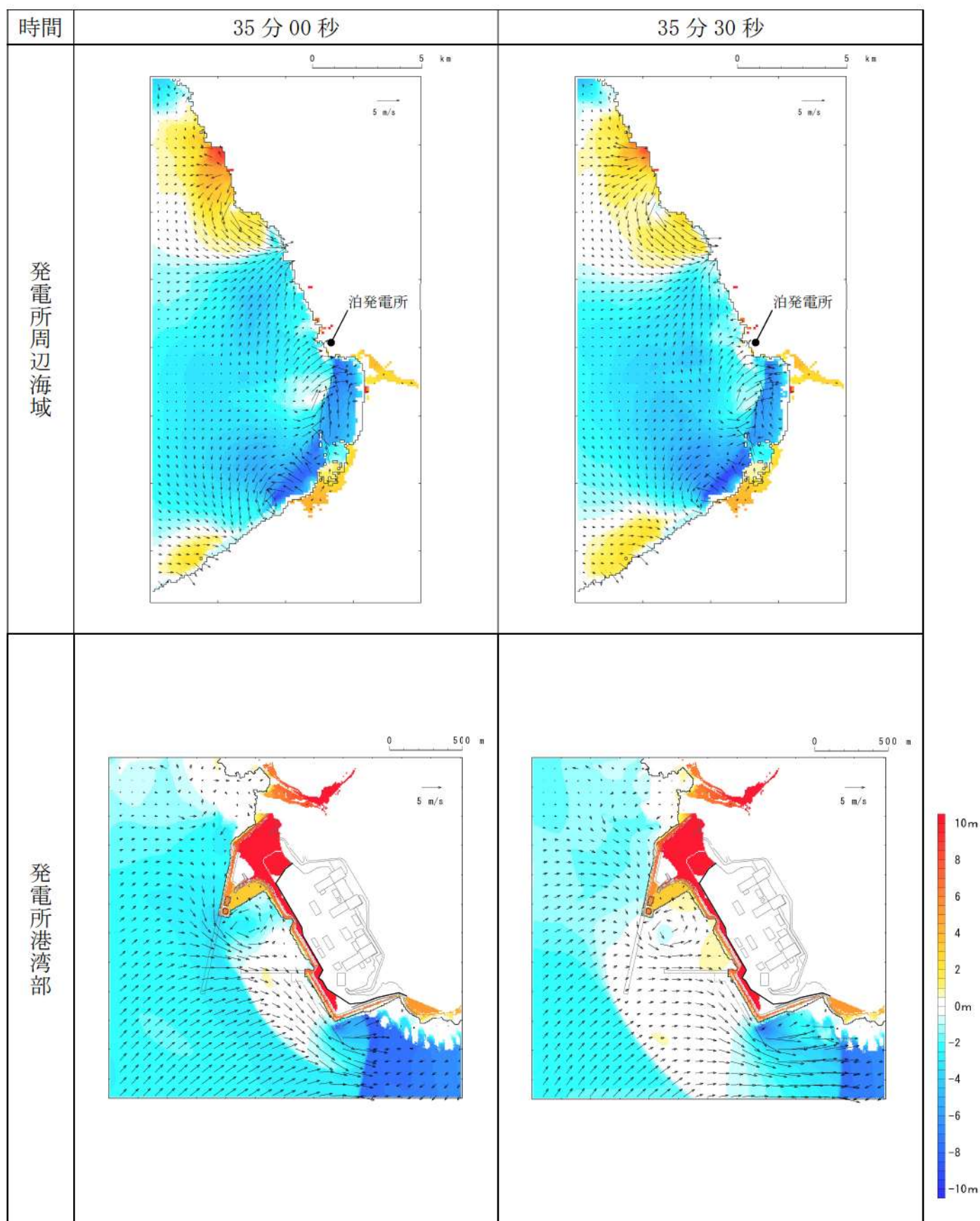
第 16 図-24 基準津波 J（北及び南防波堤損傷）の水位変動・流向ベクトル(24/49)
