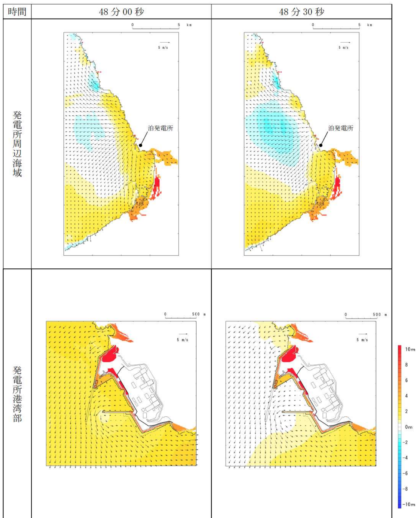
第 18 図-41 基準津波 L（北防波堤損傷）の水位変動・流向ベクトル(41/53)
