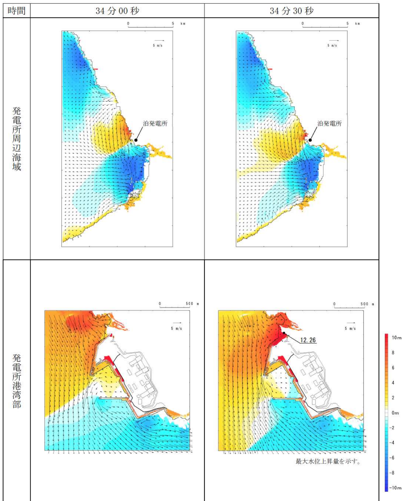
第 18 図-27 基準津波 L（北防波堤損傷）の水位変動・流向ベクトル (27/53)
