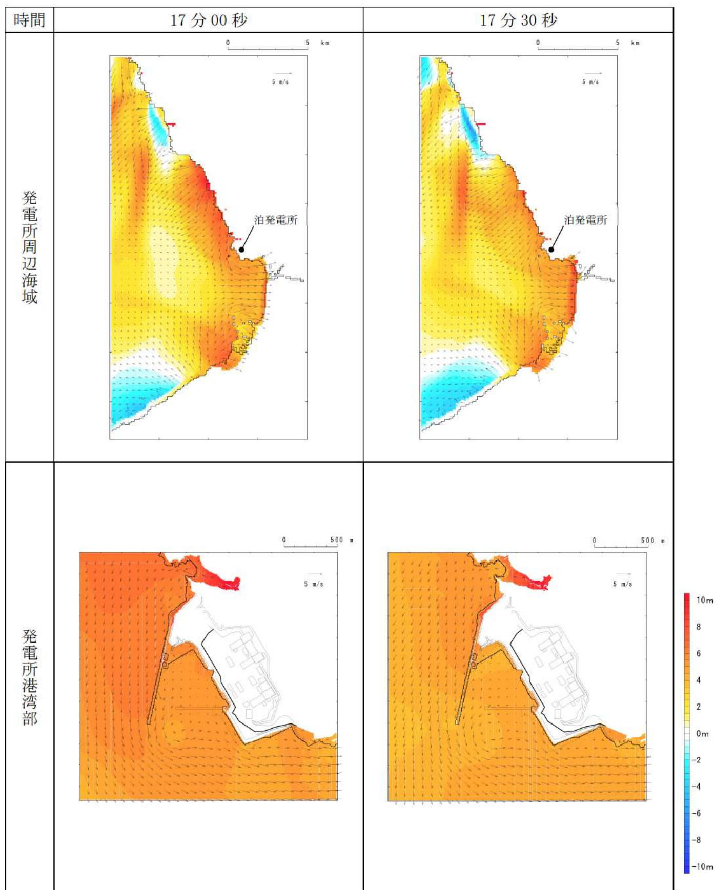
第 17 図-10 基準津波K（南防波堤損傷）の水位変動・流向ベクトル(10/53)
