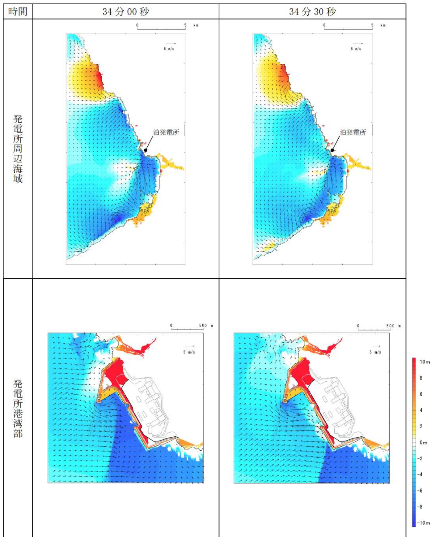
第 16 図-23 基準津波 J（北及び南防波堤損傷）の水位変動・流向ベクトル(23/49)
