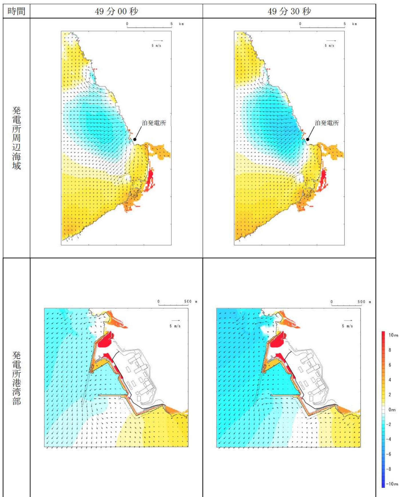
第 18 図-42 基準津波 L（北防波堤損傷）の水位変動・流向ベクトル(42/53)
