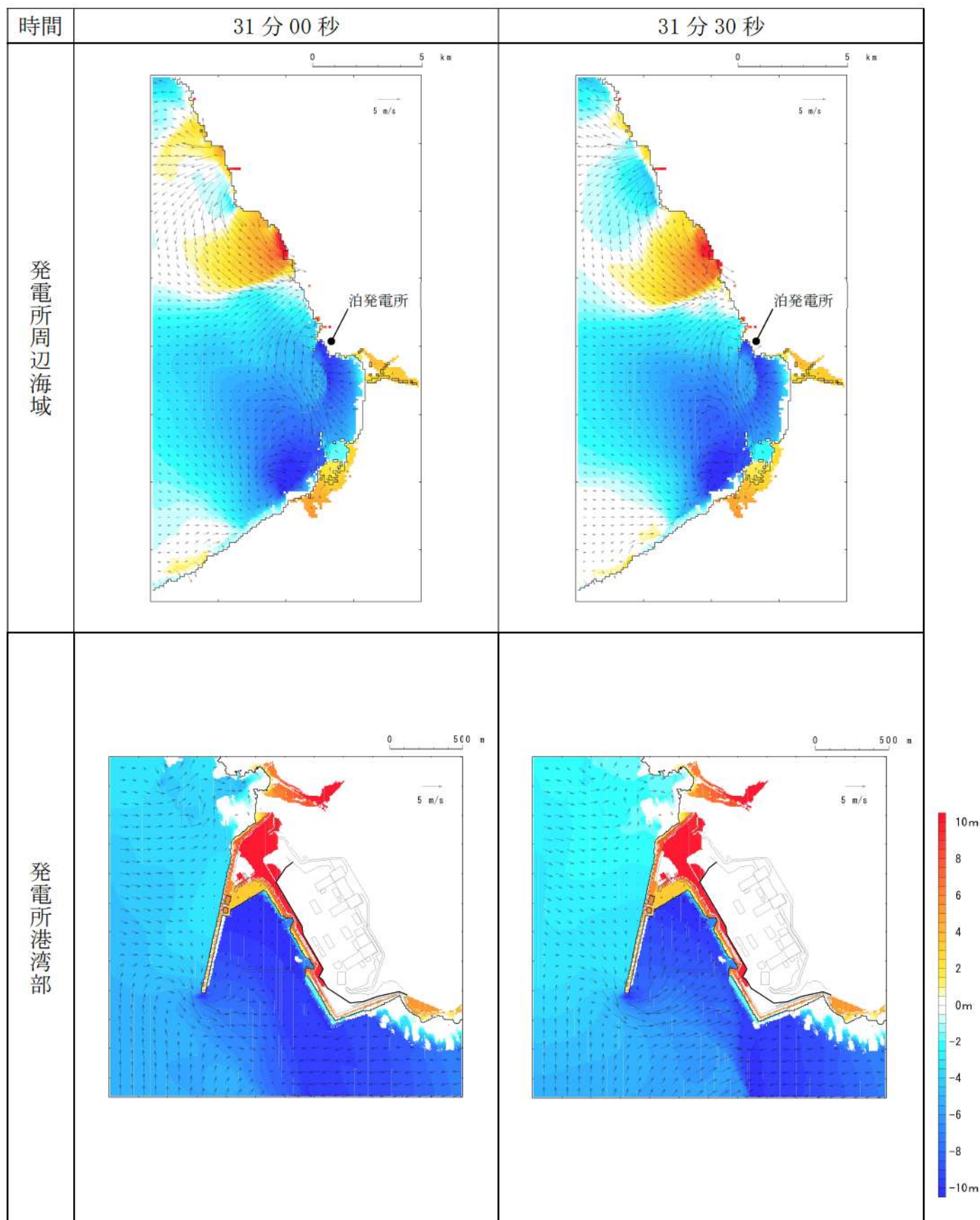
第 17 図-24 基準津波K（南防波堤損傷）の水位変動・流向ベクトル(24/53)
