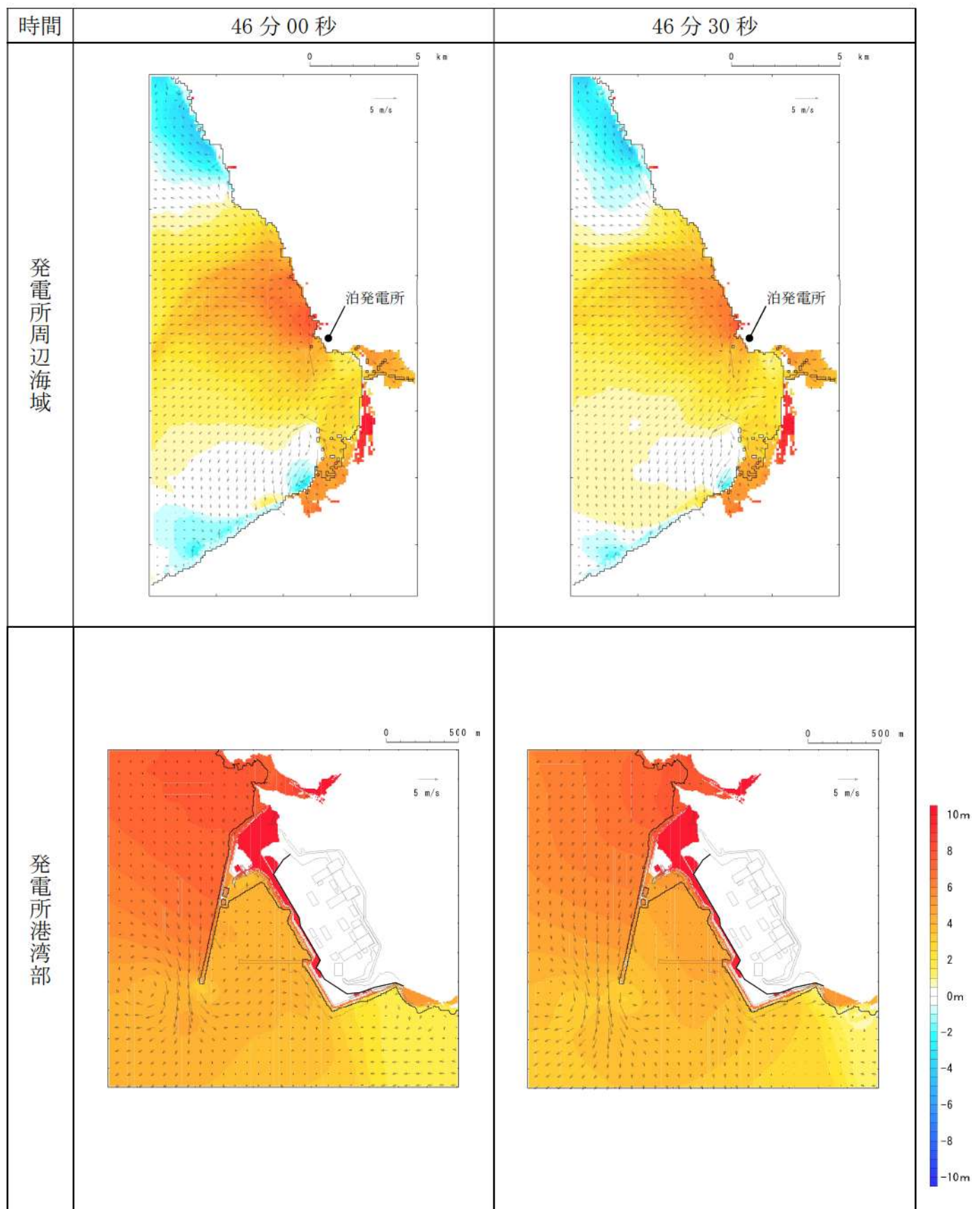
第 17 図-39 基準津波K（南防波堤損傷）の水位変動・流向ベクトル(39/53)
