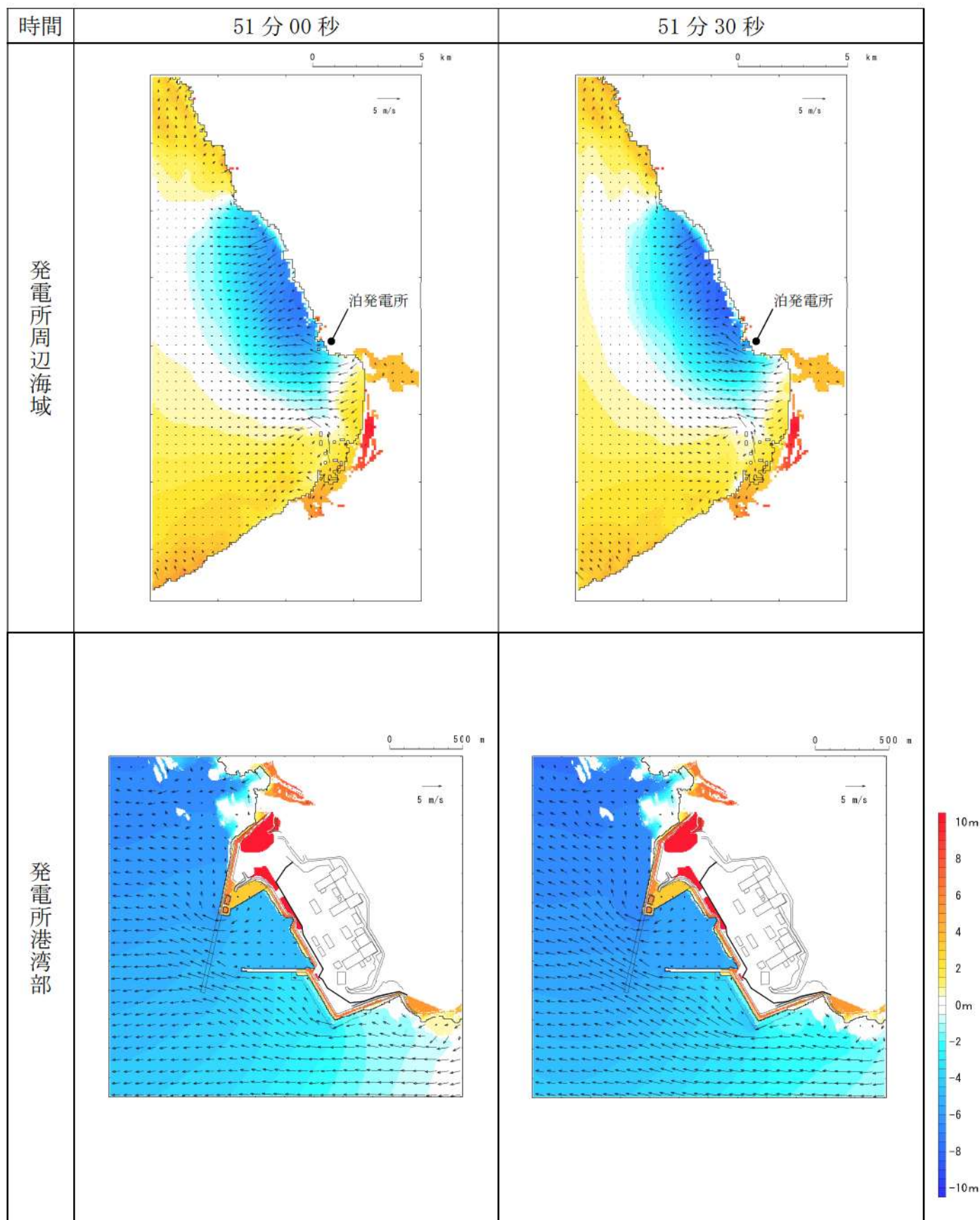
第 18 図-44 基準津波 L（北防波堤損傷）の水位変動・流向ベクトル(44/53)
