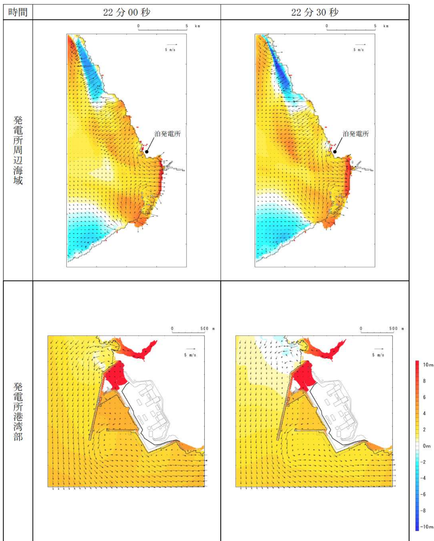
第 15 図-12 基準津波 I（防波堤損傷なし）の水位変動・流向ベクトル(12/50)
