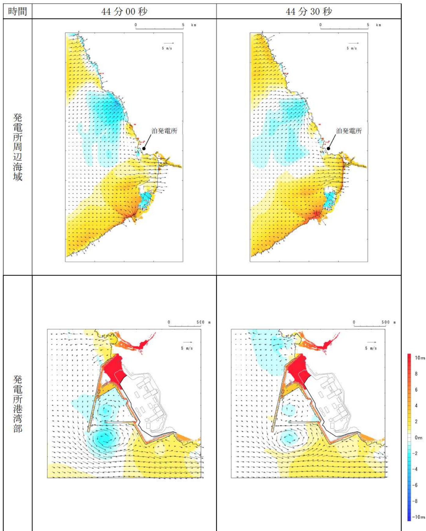
第 15 図-34 基準津波 I（防波堤損傷なし）の水位変動・流向ベクトル(34/50)
