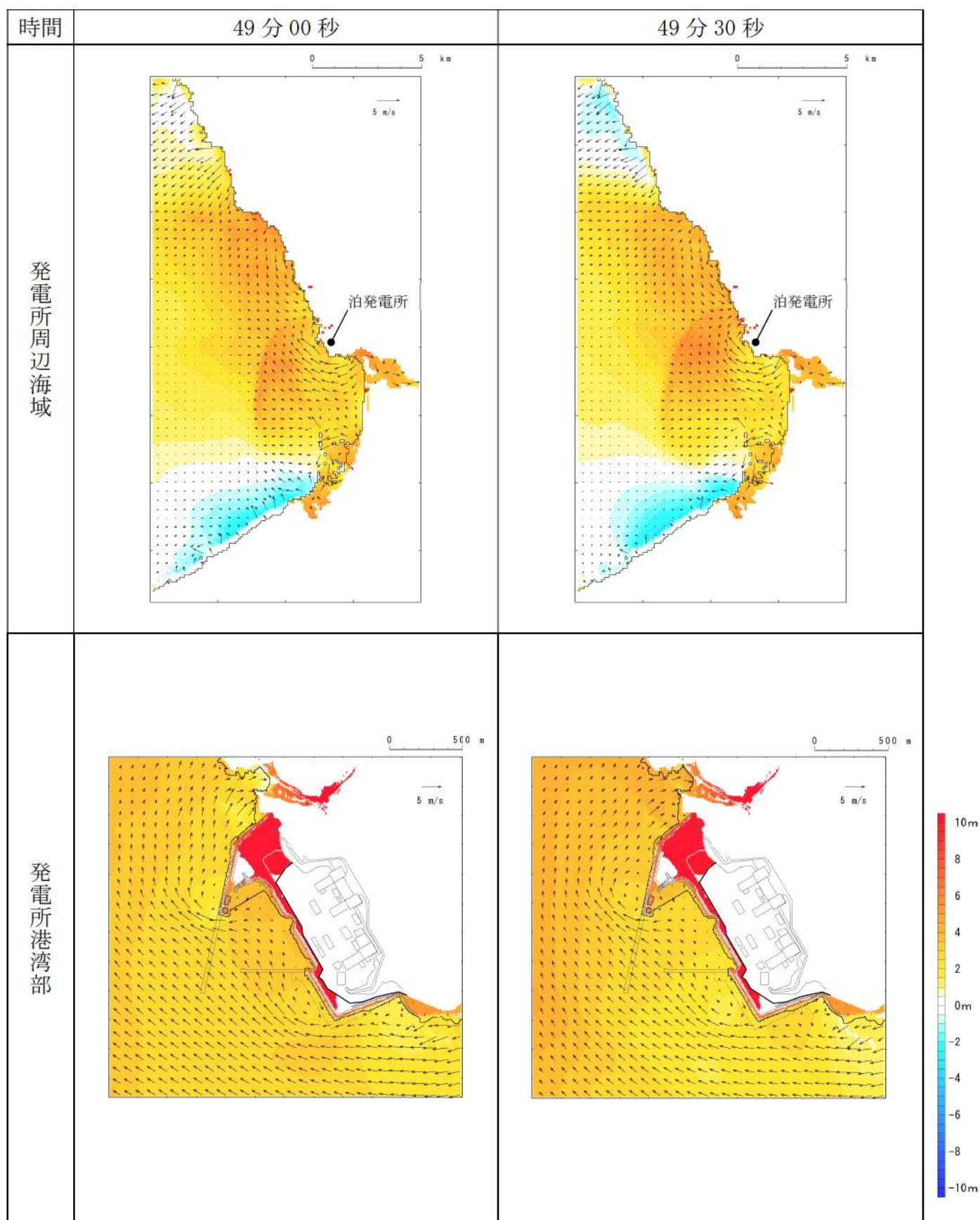
第 16 図-38 基準津波 J（北及び南防波堤損傷）の水位変動・流向ベクトル(38/49)
