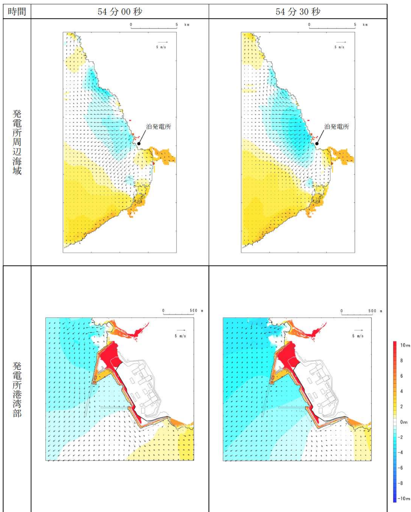
第 16 図-43 基準津波 J（北及び南防波堤損傷）の水位変動・流向ベクトル(43/49)
