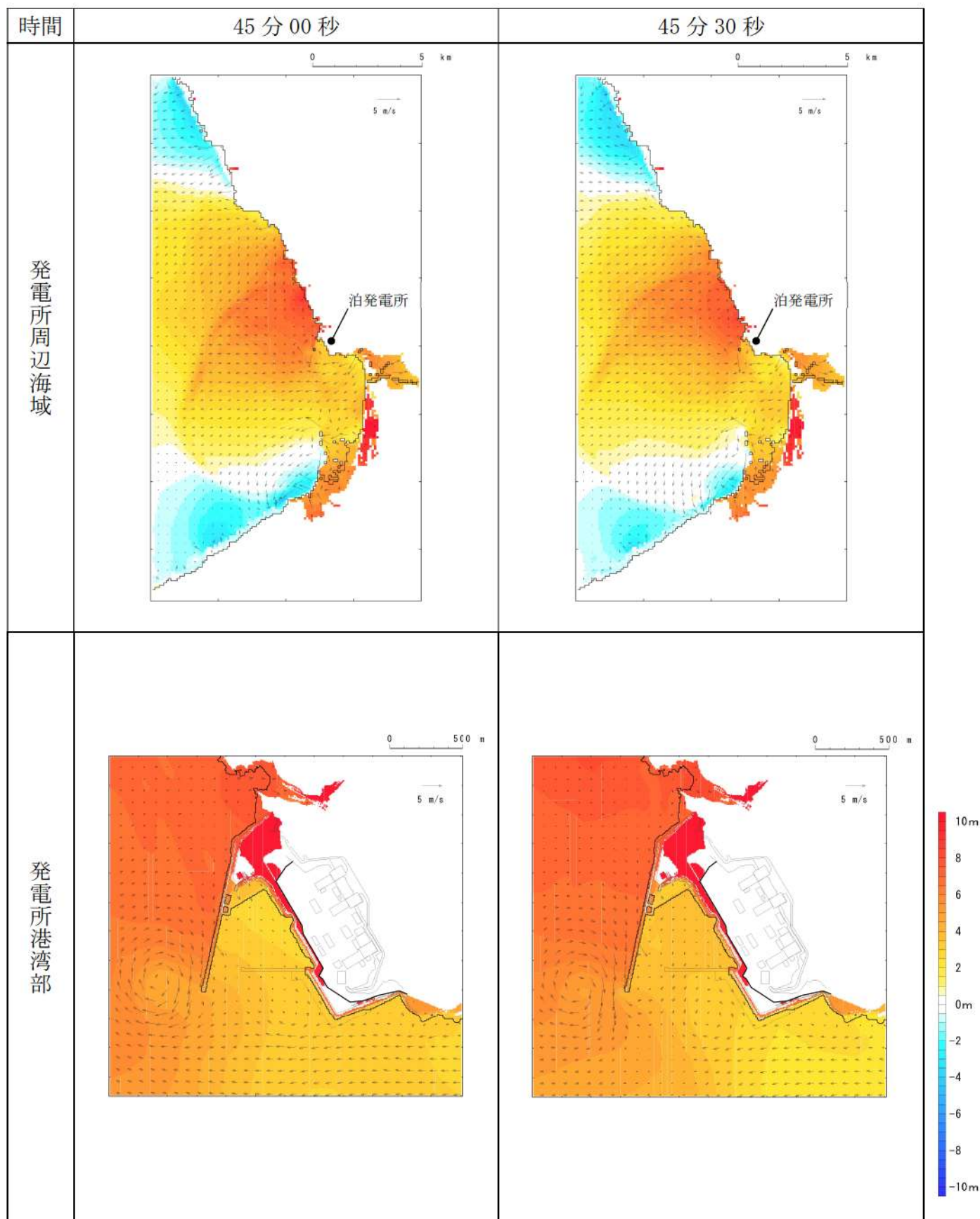
第 17 図-38 基準津波K（南防波堤損傷）の水位変動・流向ベクトル(38/53)
