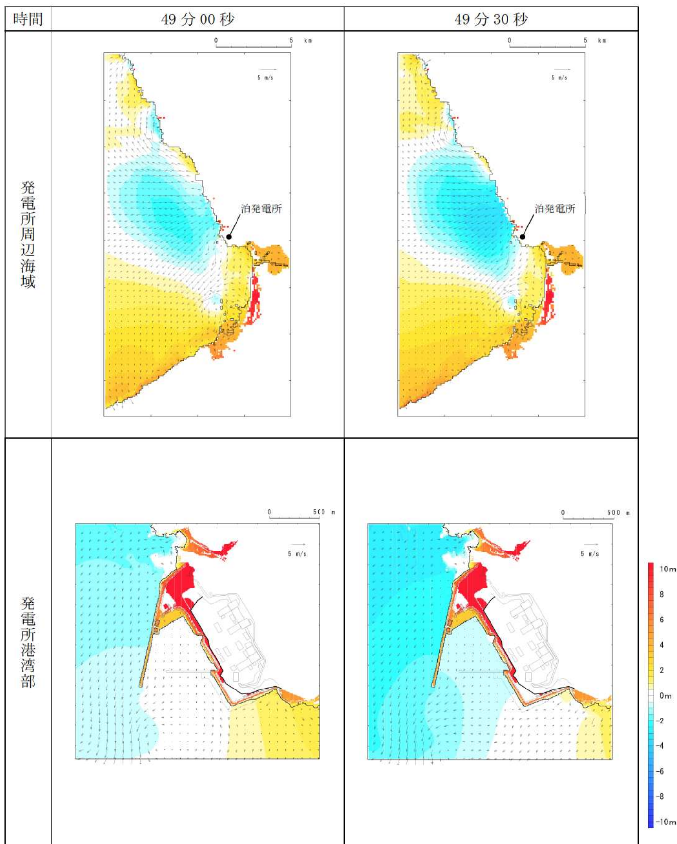
第 17 図-42 基準津波K（南防波堤損傷）の水位変動・流向ベクトル(42/53)
