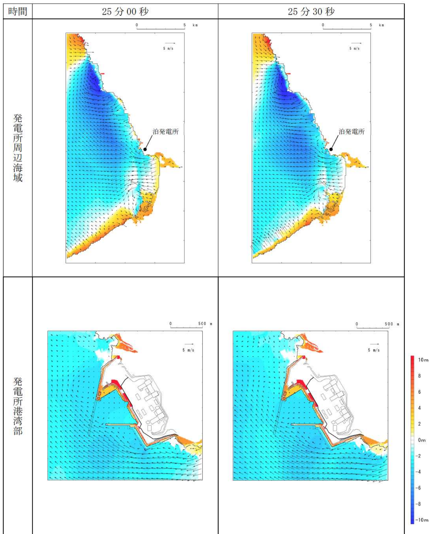
第 18 図-18 基準津波 L（北防波堤損傷）の水位変動・流向ベクトル(18/53)
