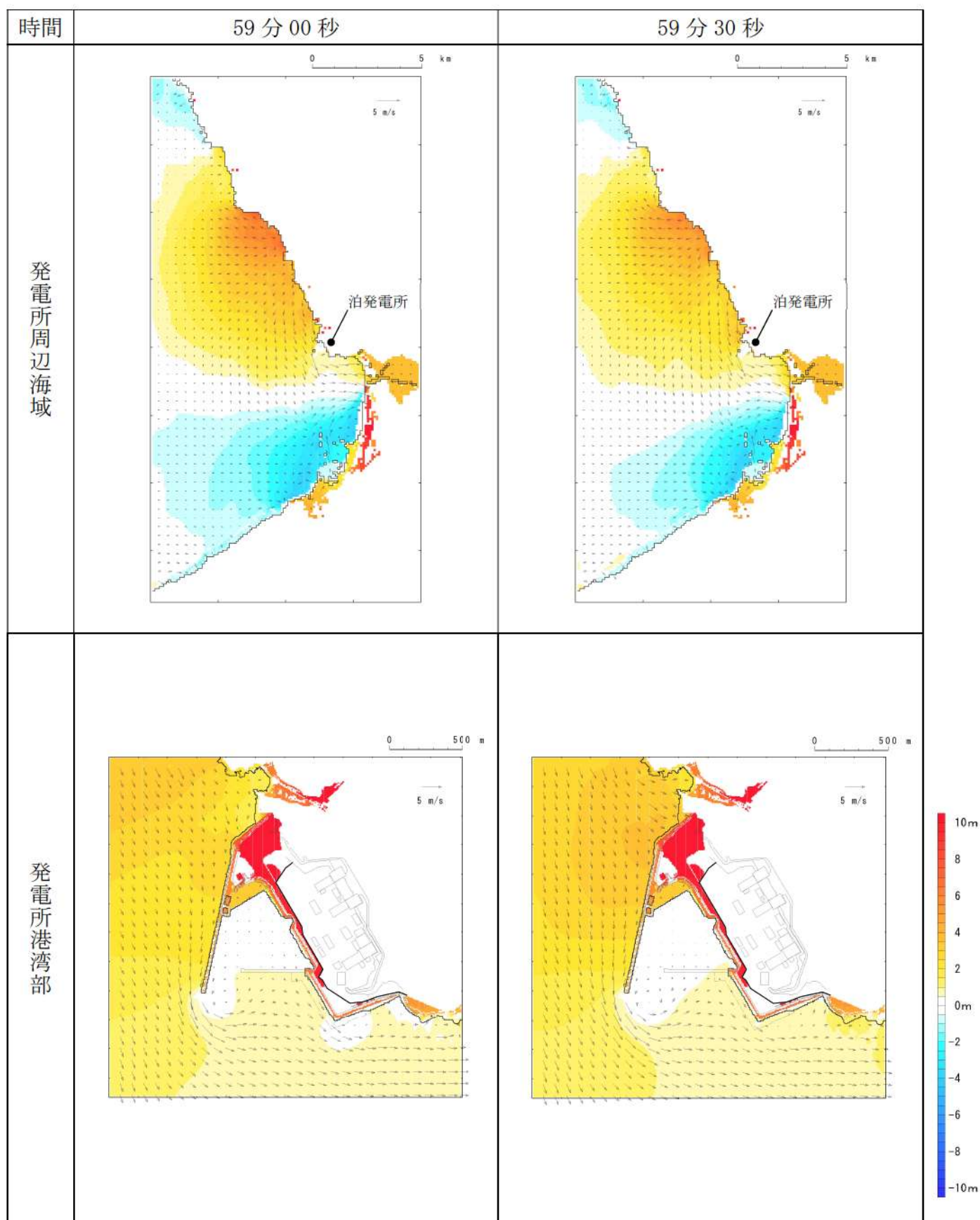
第 17 図-52 基準津波K（南防波堤損傷）の水位変動・流向ベクトル(52/53)
