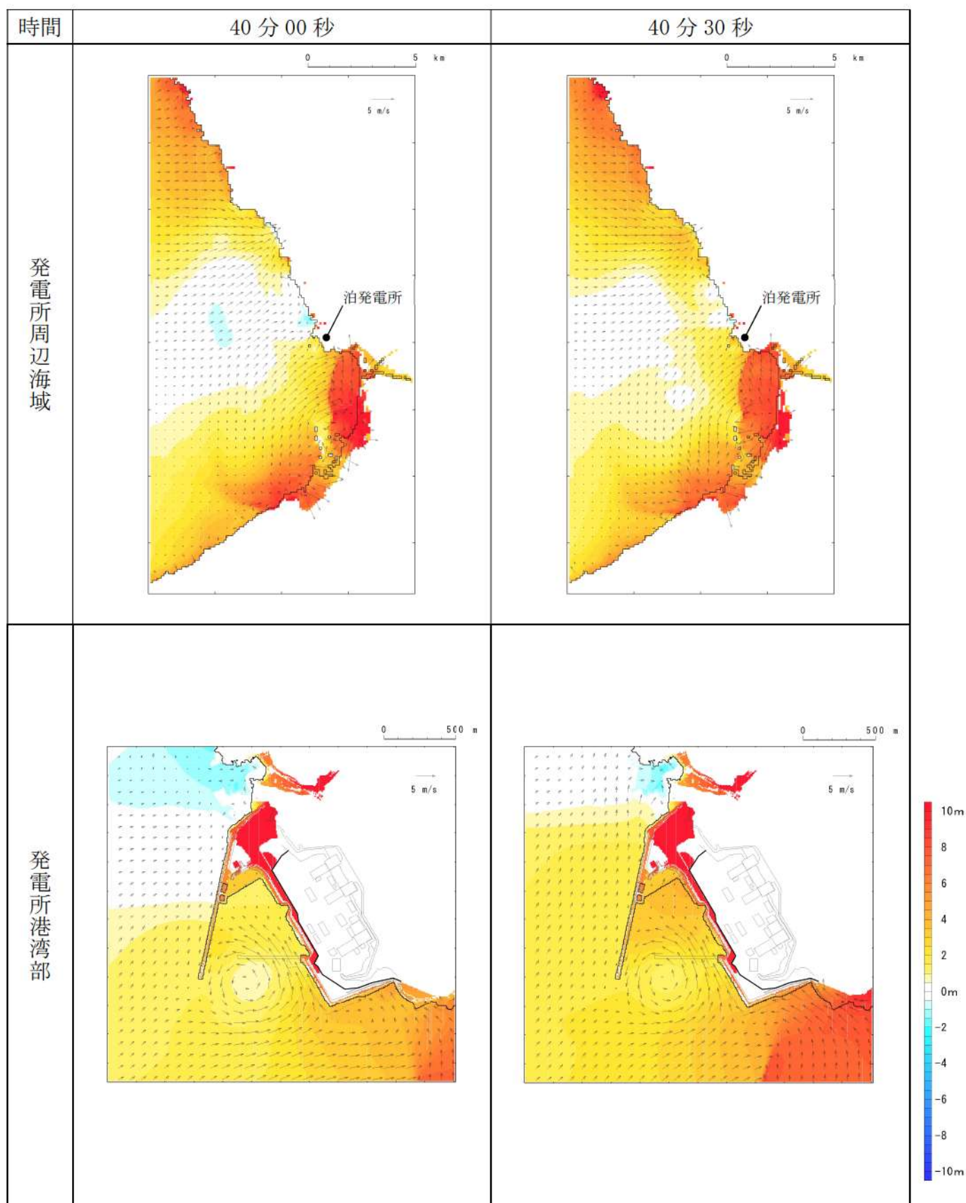
第 17 図-33 基準津波K（南防波堤損傷）の水位変動・流向ベクトル(33/53)
