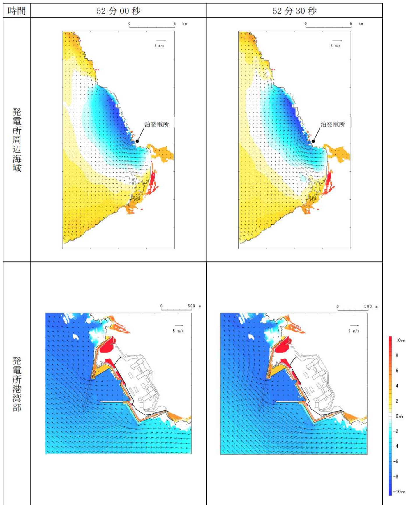
第 18 図-45 基準津波 L（北防波堤損傷）の水位変動・流向ベクトル(45/53)
