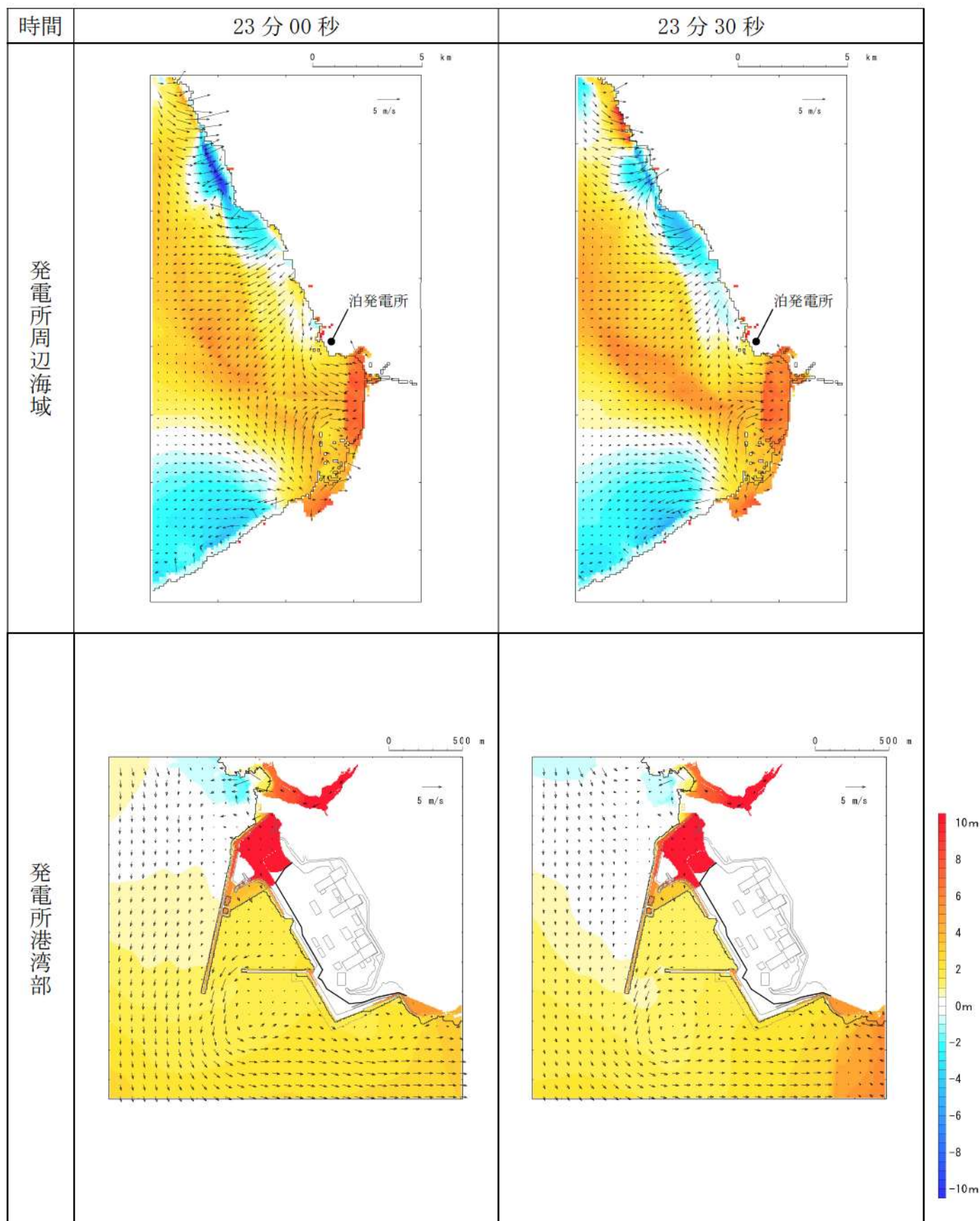
第 15 図-13 基準津波 I（防波堤損傷なし）の水位変動・流向ベクトル(13/50)
