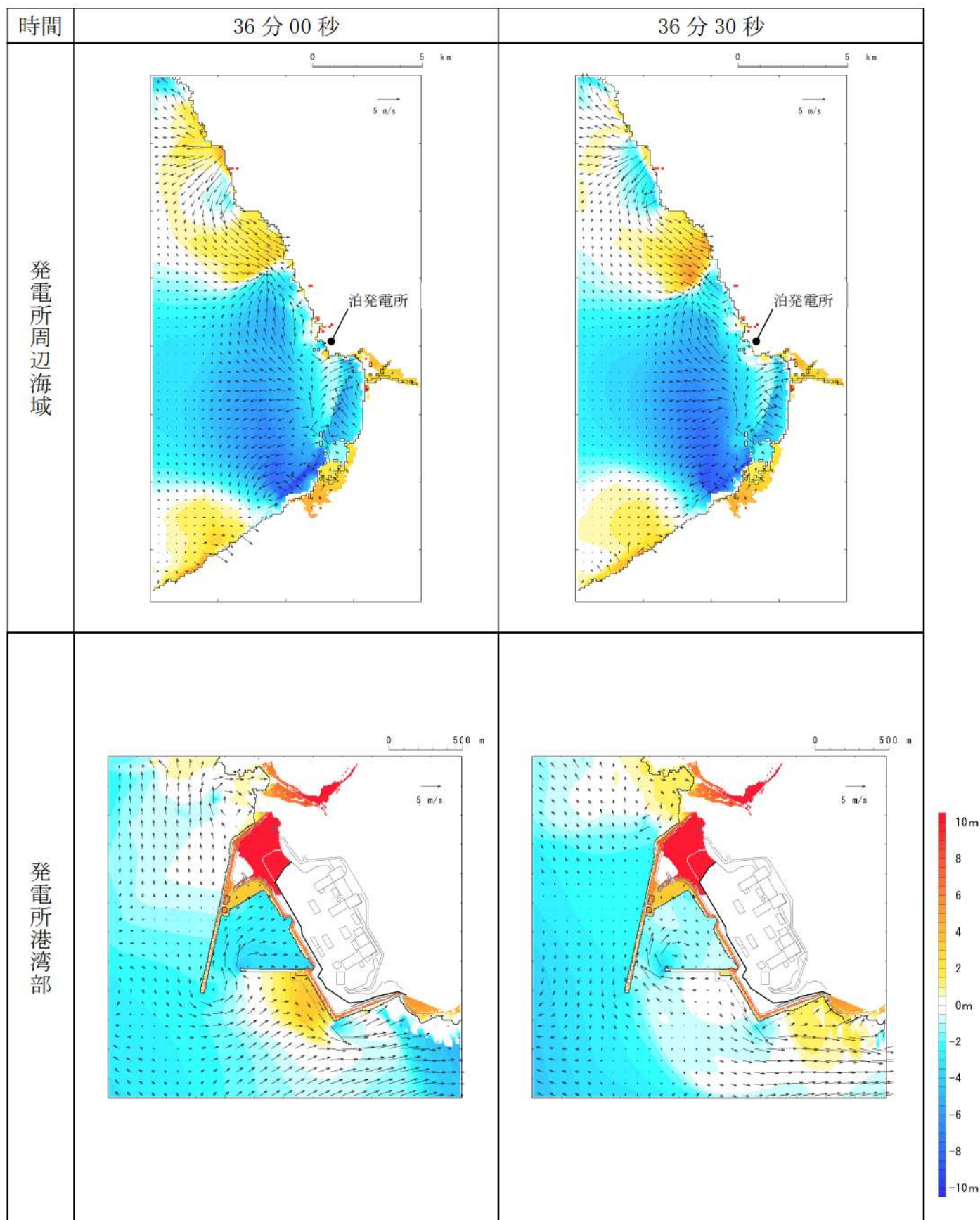
第 15 図-26 基準津波 I（防波堤損傷なし）の水位変動・流向ベクトル(26/50)
