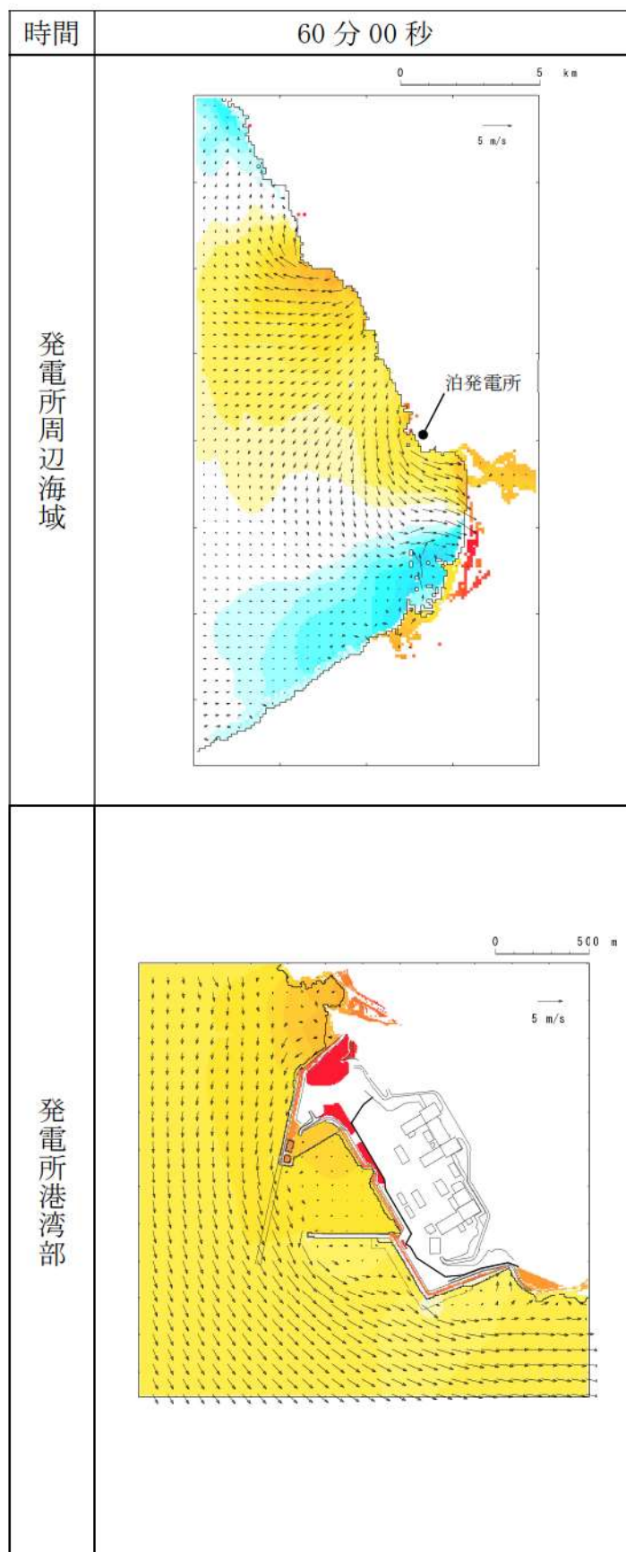
第 18 図-53 基準津波 L（北防波堤損傷）の水位変動・流向ベクトル(53/53)
