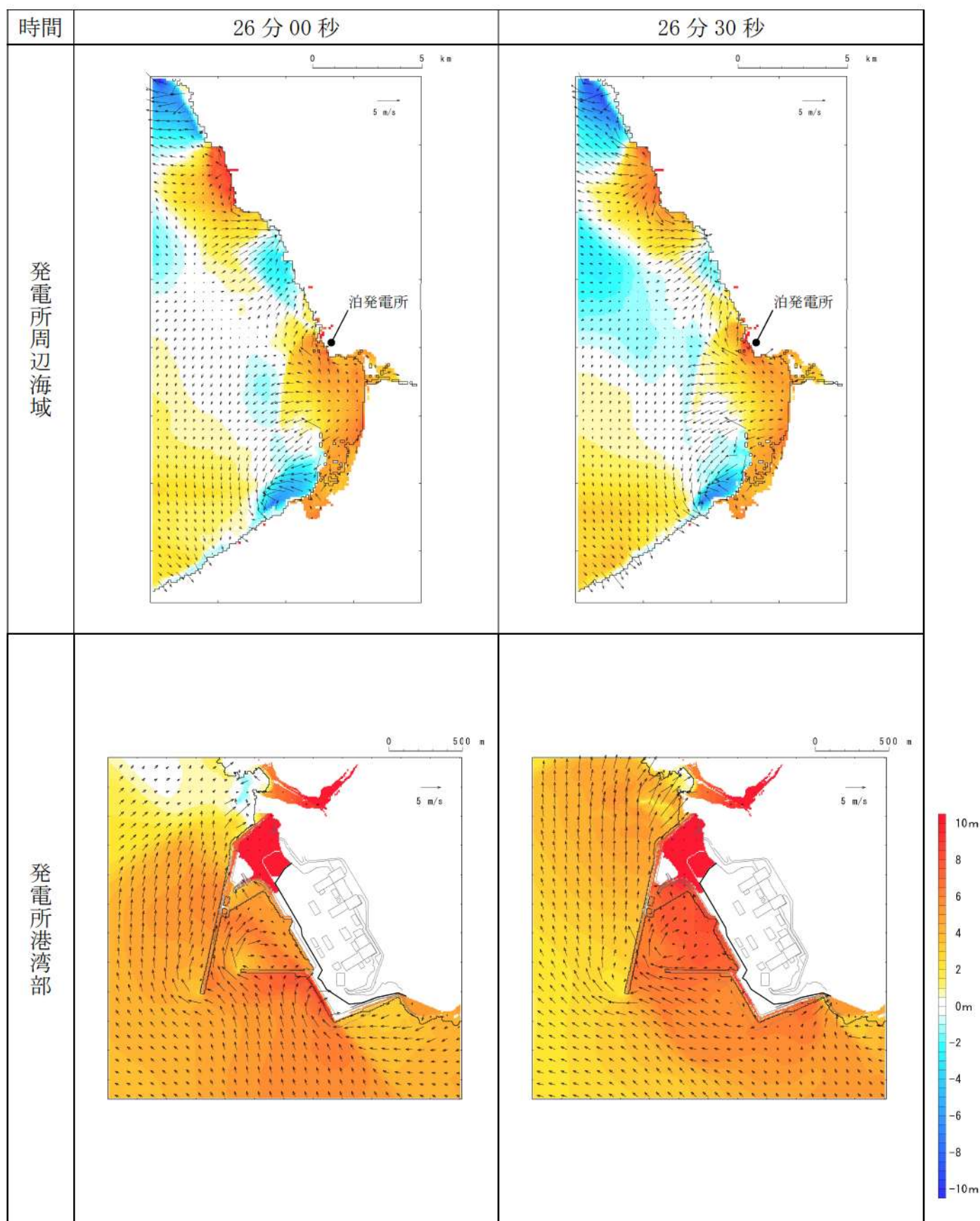
第 15 図-16 基準津波 I（防波堤損傷なし）の水位変動・流向ベクトル(16/50)
