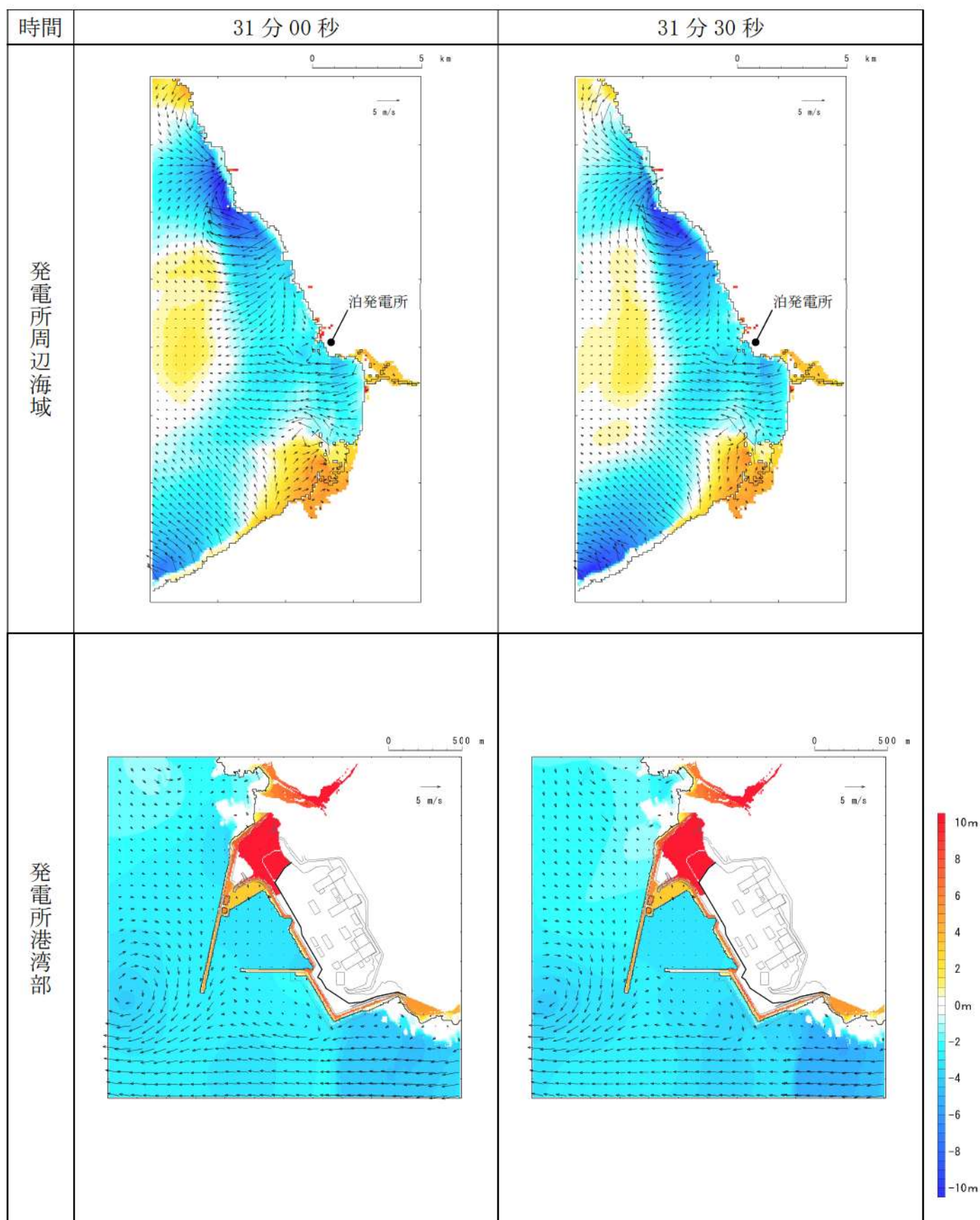
第 15 図-21 基準津波 I（防波堤損傷なし）の水位変動・流向ベクトル(21/50)
