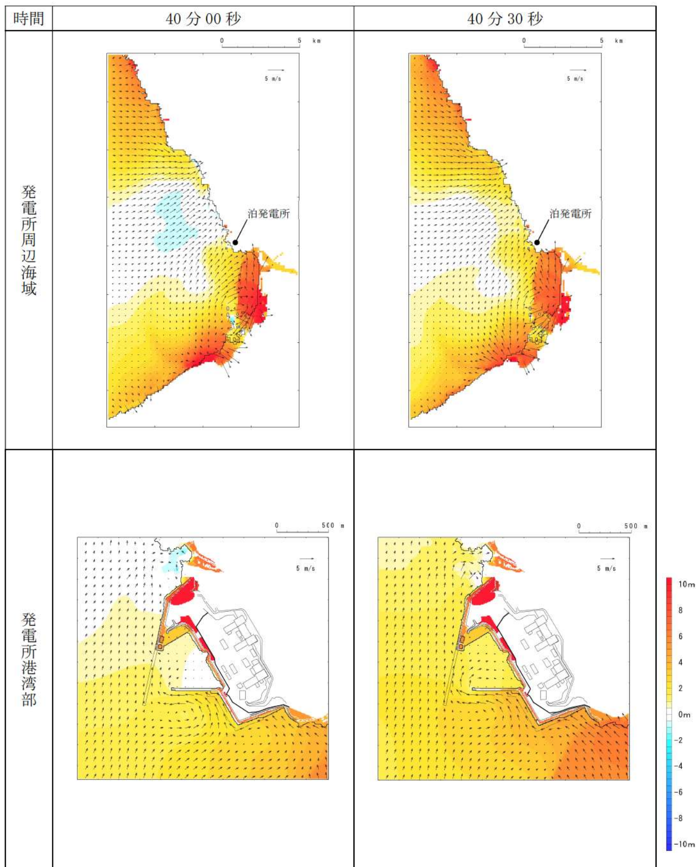
第 18 図-33 基準津波 L（北防波堤損傷）の水位変動・流向ベクトル(33/53)
