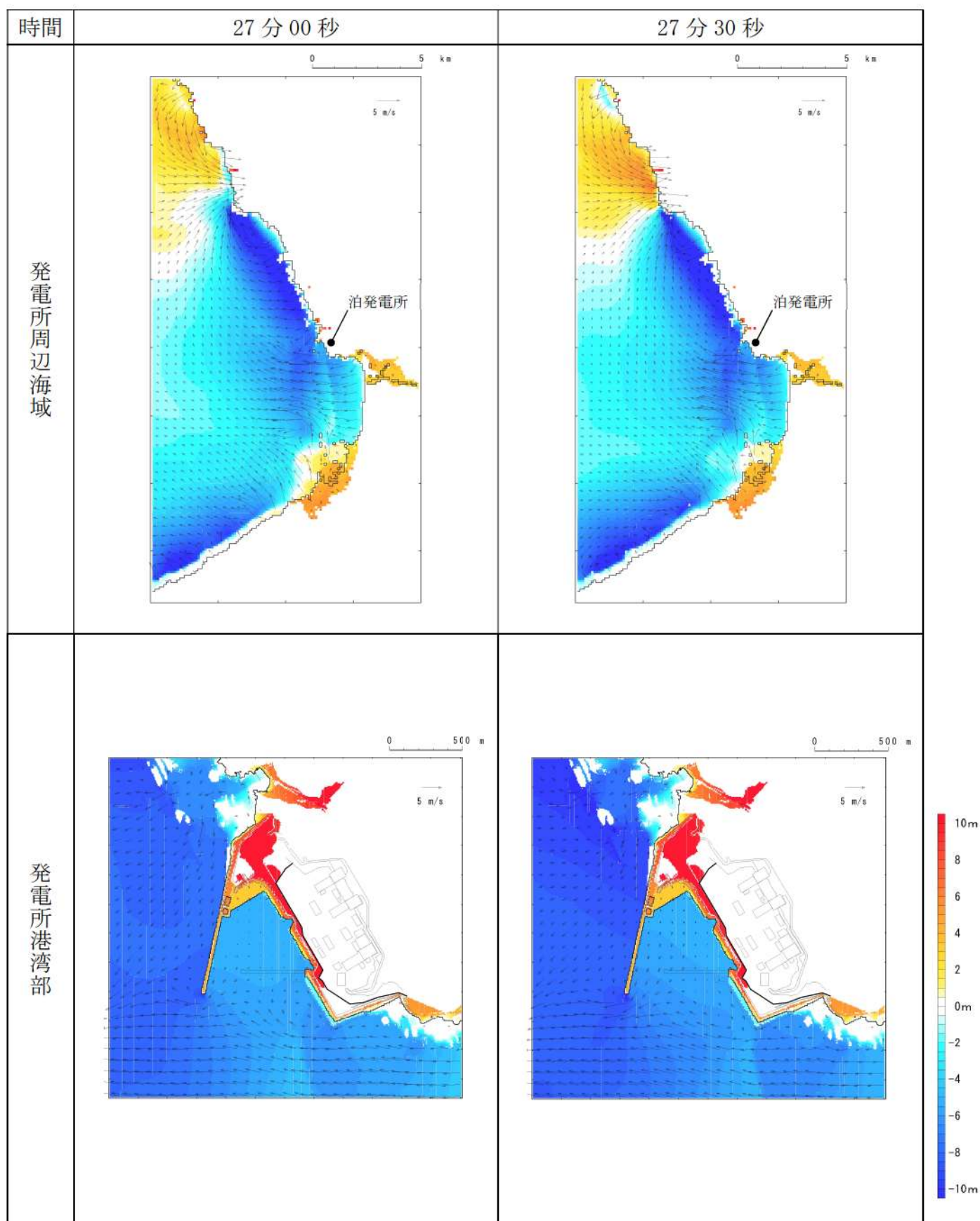
第 17 図-20 基準津波K（南防波堤損傷）の水位変動・流向ベクトル(20/53)
