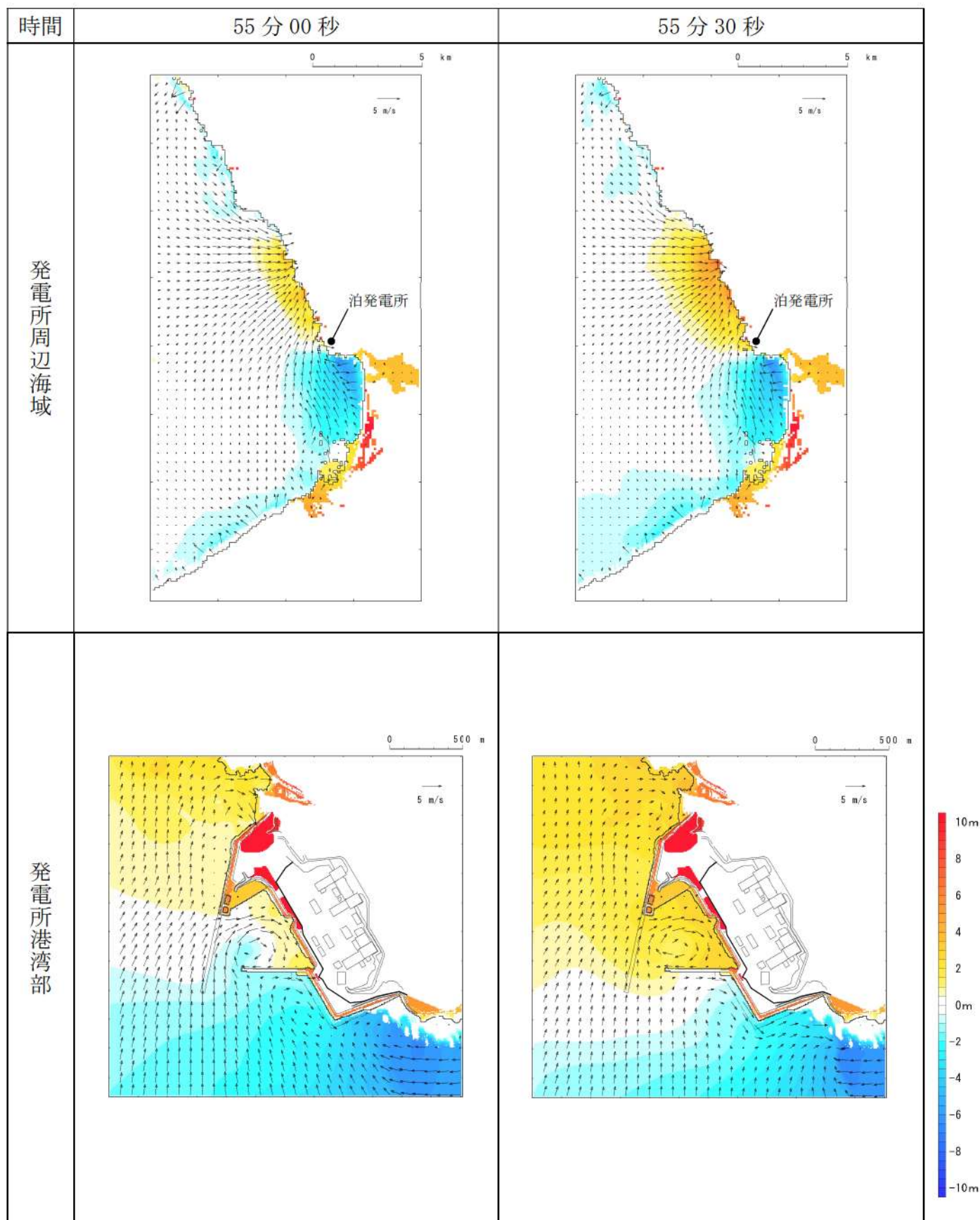
第 18 図-48 基準津波 L（北防波堤損傷）の水位変動・流向ベクトル(48/53)
