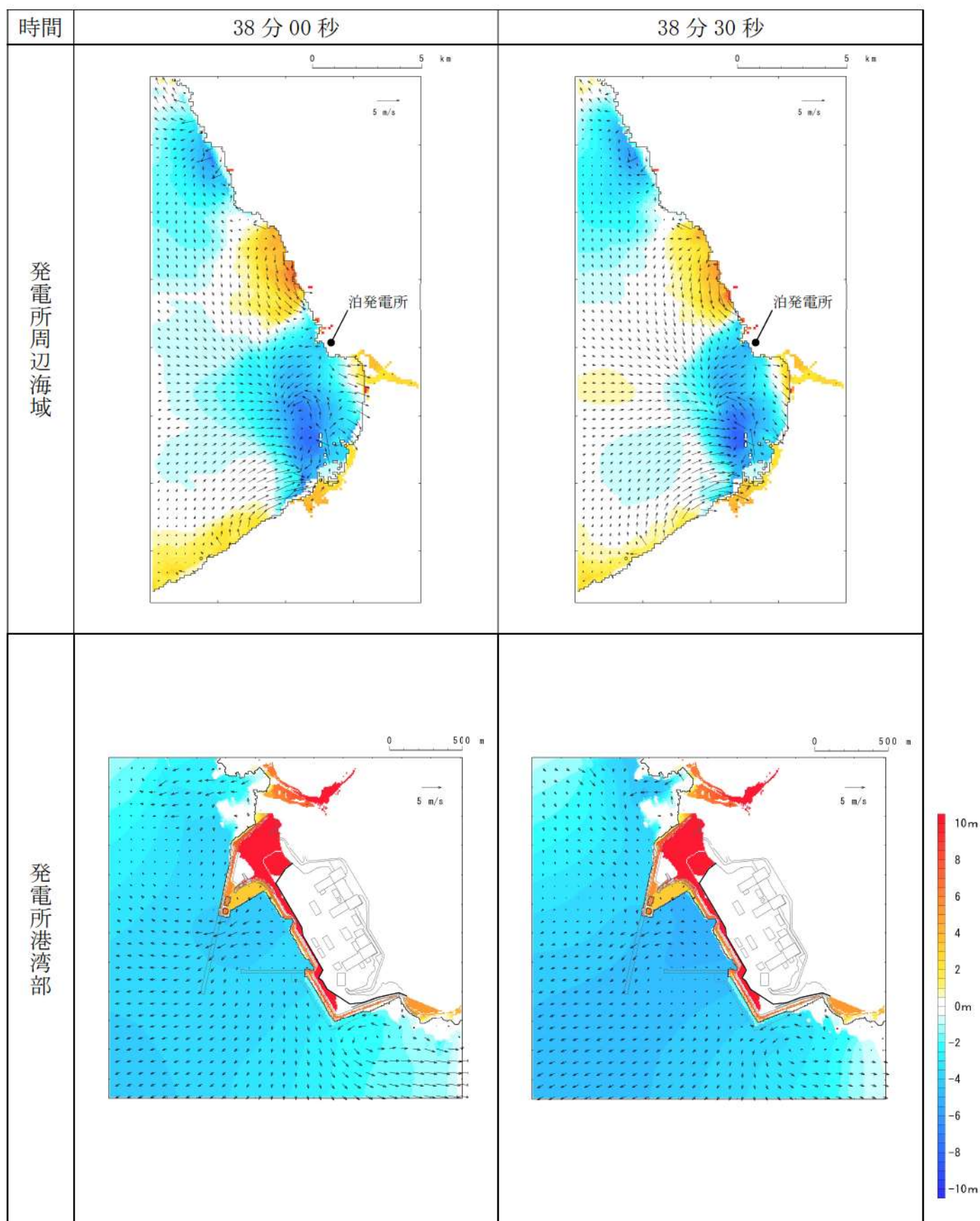
第 16 図-27 基準津波 J（北及び南防波堤損傷）の水位変動・流向ベクトル(27/49)
