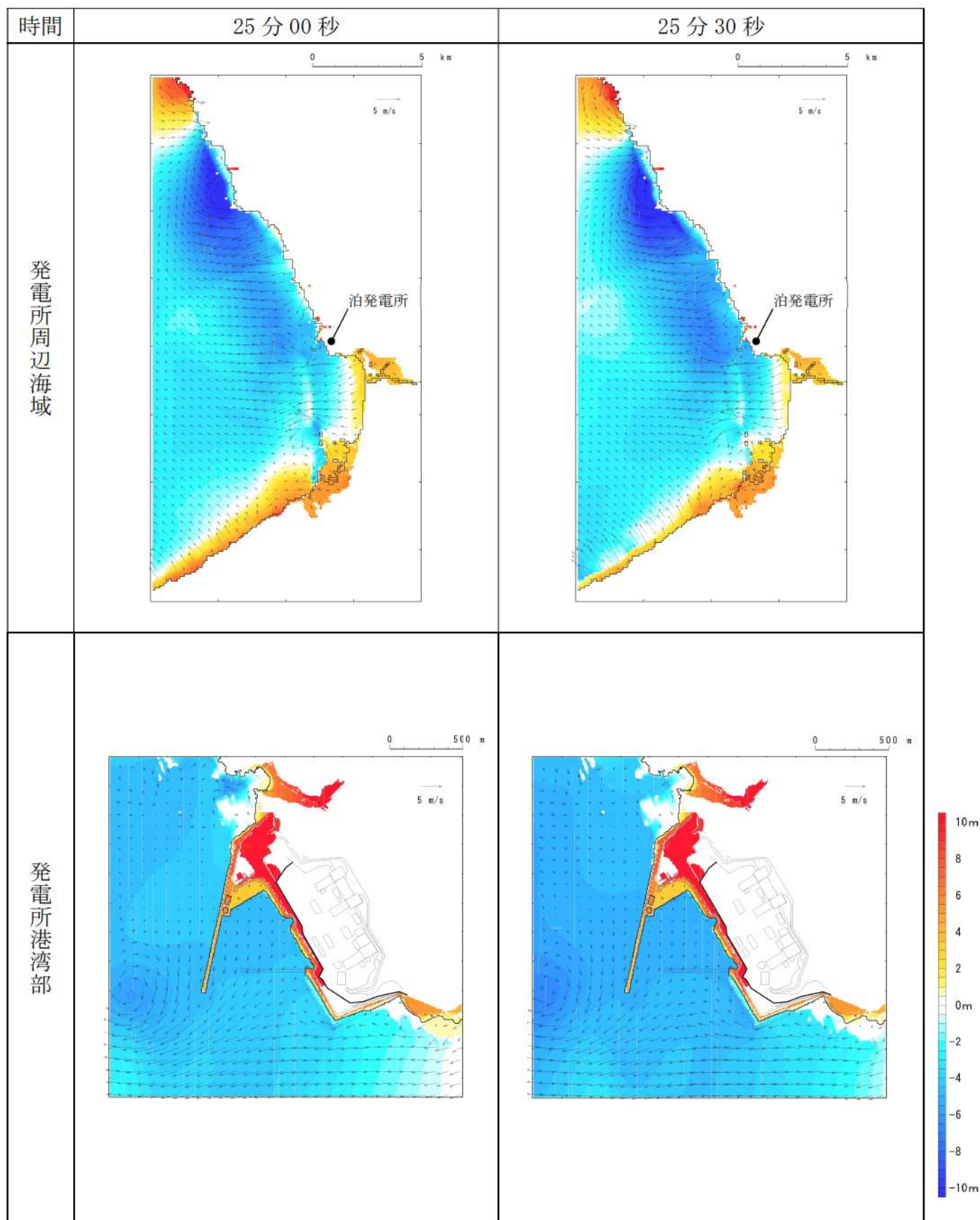
第 17 図-18 基準津波K（南防波堤損傷）の水位変動・流向ベクトル(18/53)
