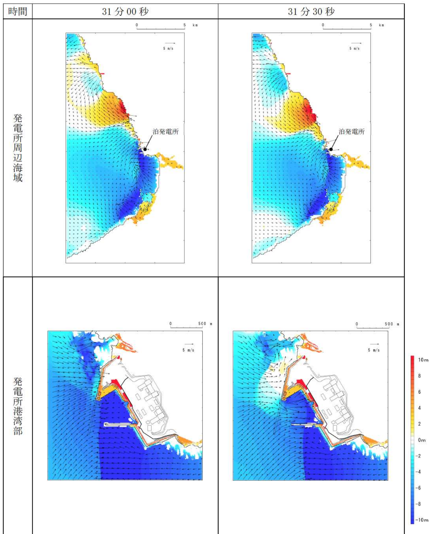
第 18 図-24 基準津波 L（北防波堤損傷）の水位変動・流向ベクトル (24/53)
