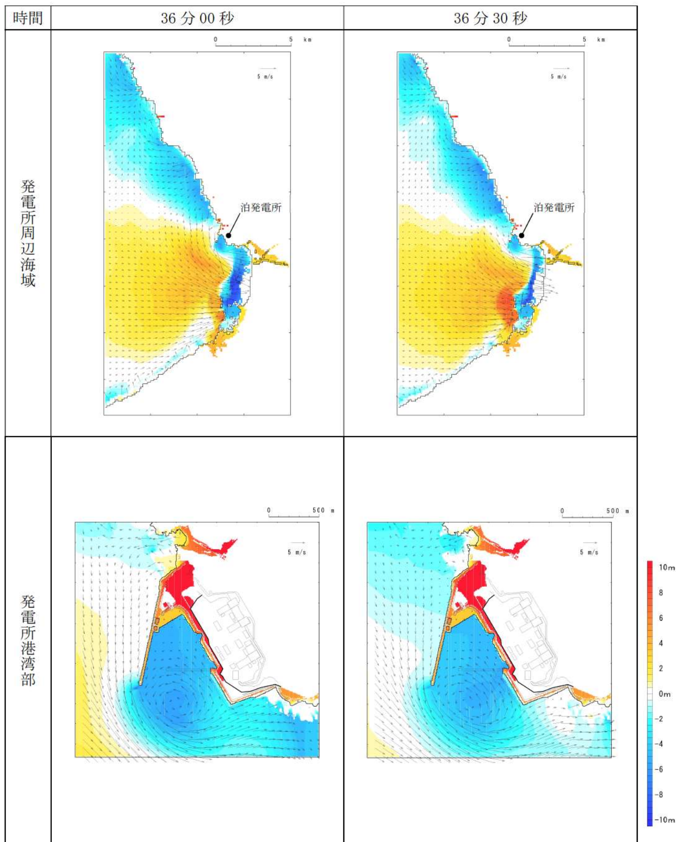
第 17 図-29 基準津波K（南防波堤損傷）の水位変動・流向ベクトル(29/53)
