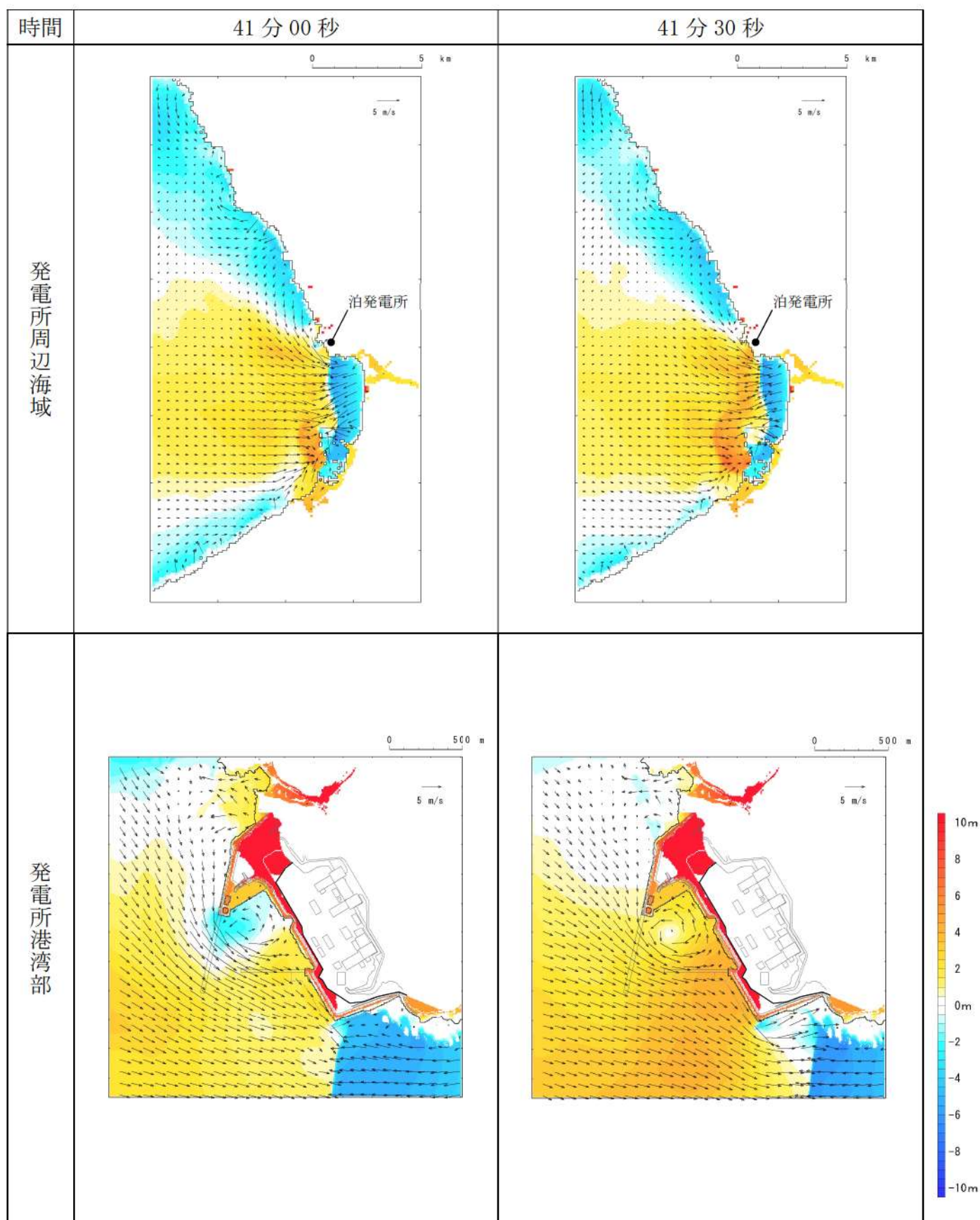
第 16 図-30 基準津波 J（北及び南防波堤損傷）の水位変動・流向ベクトル(30/49)
