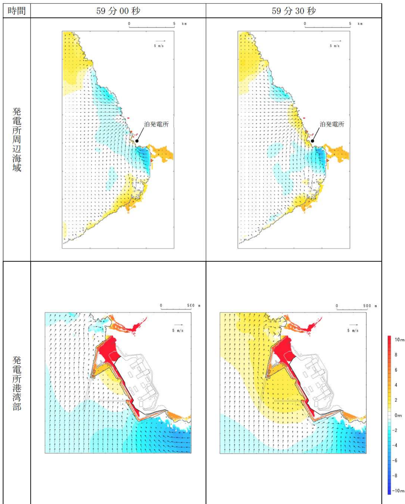
第 16 図-48 基準津波 J（北及び南防波堤損傷）の水位変動・流向ベクトル(48/49)
