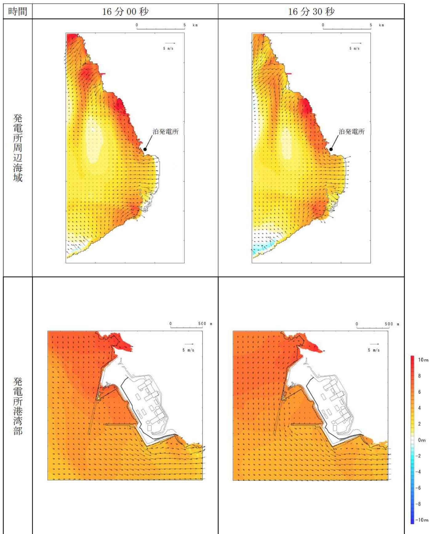
第 18 図-9 基準津波 L（北防波堤損傷）の水位変動・流向ベクトル (9/53)
