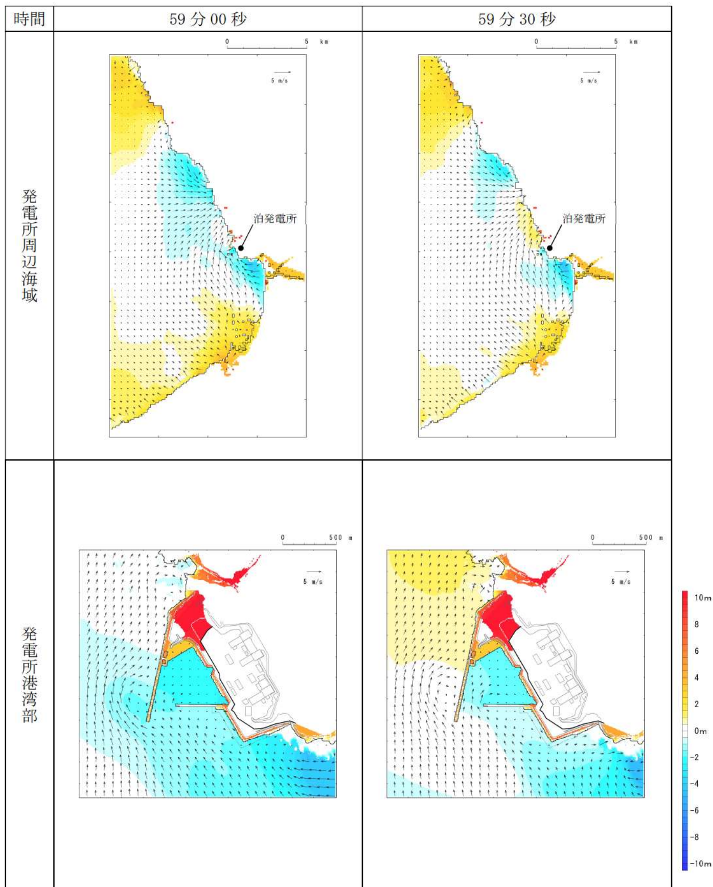
第 15 図-49 基準津波 I（防波堤損傷なし）の水位変動・流向ベクトル(49/50)
