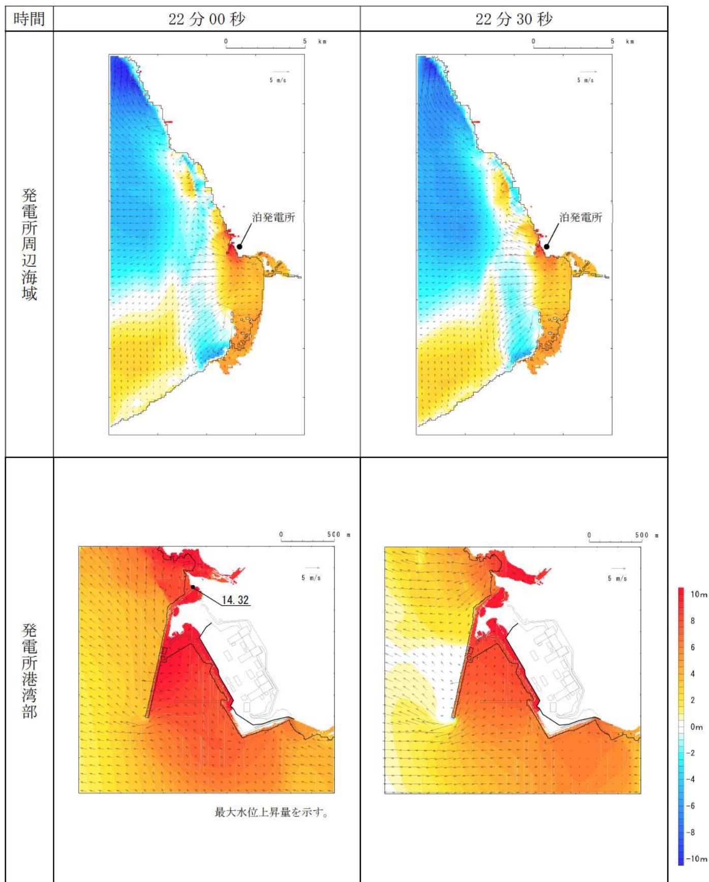
第 17 図-15 基準津波K（南防波堤損傷）の水位変動・流向ベクトル(15/53)
