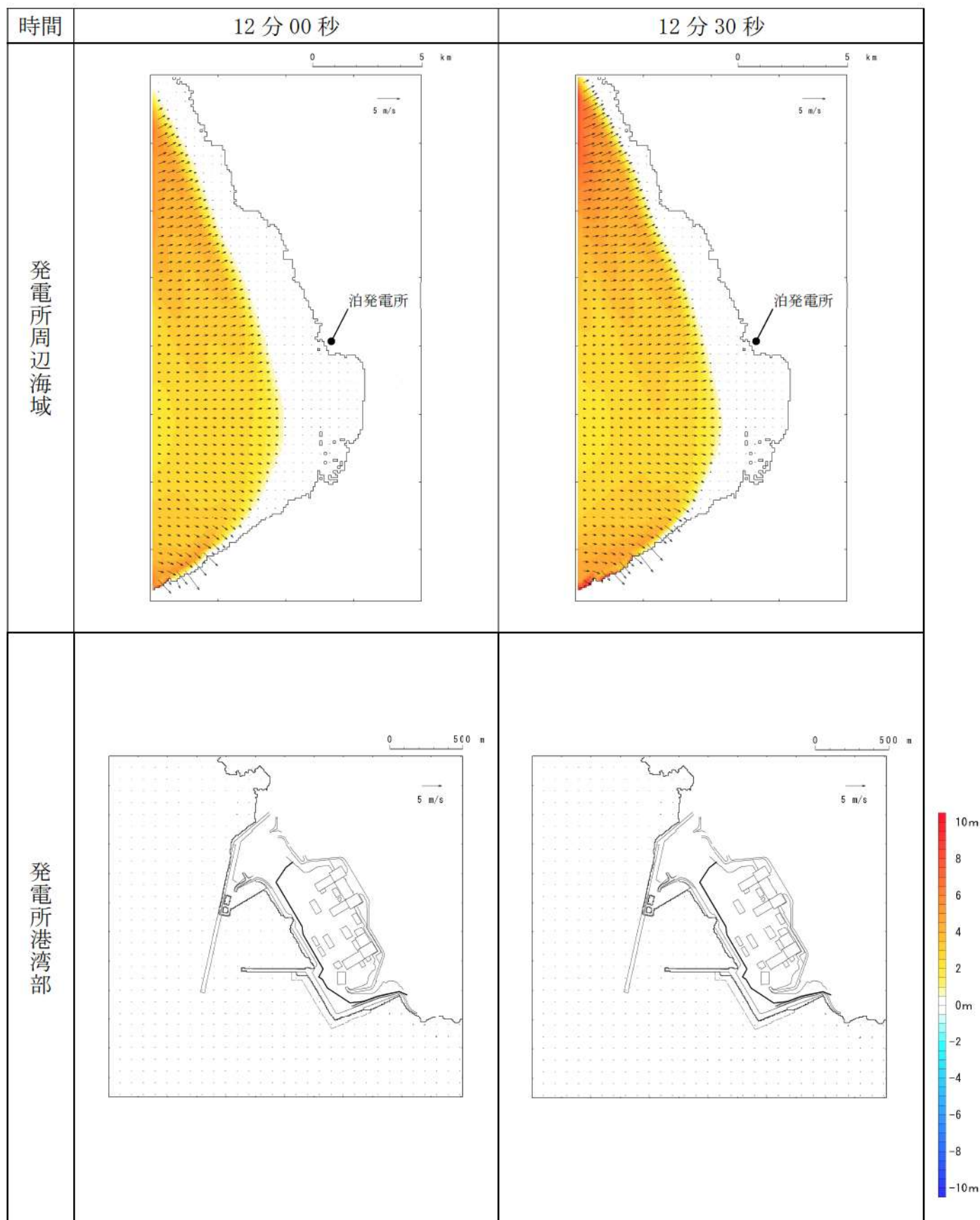
第 18 図-5 基準津波 L（北防波堤損傷）の水位変動・流向ベクトル (5/53)
