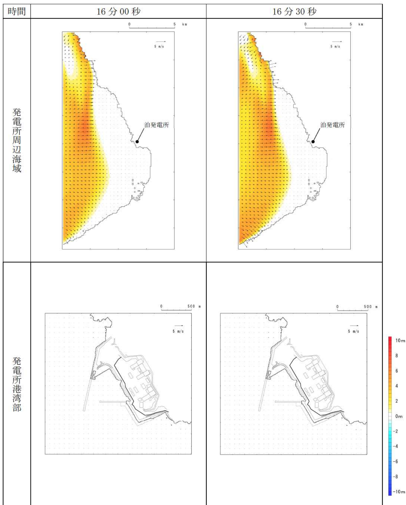
第 16 図-5 基準津波 J（北及び南防波堤損傷）の水位変動・流向ベクトル (5/49)
