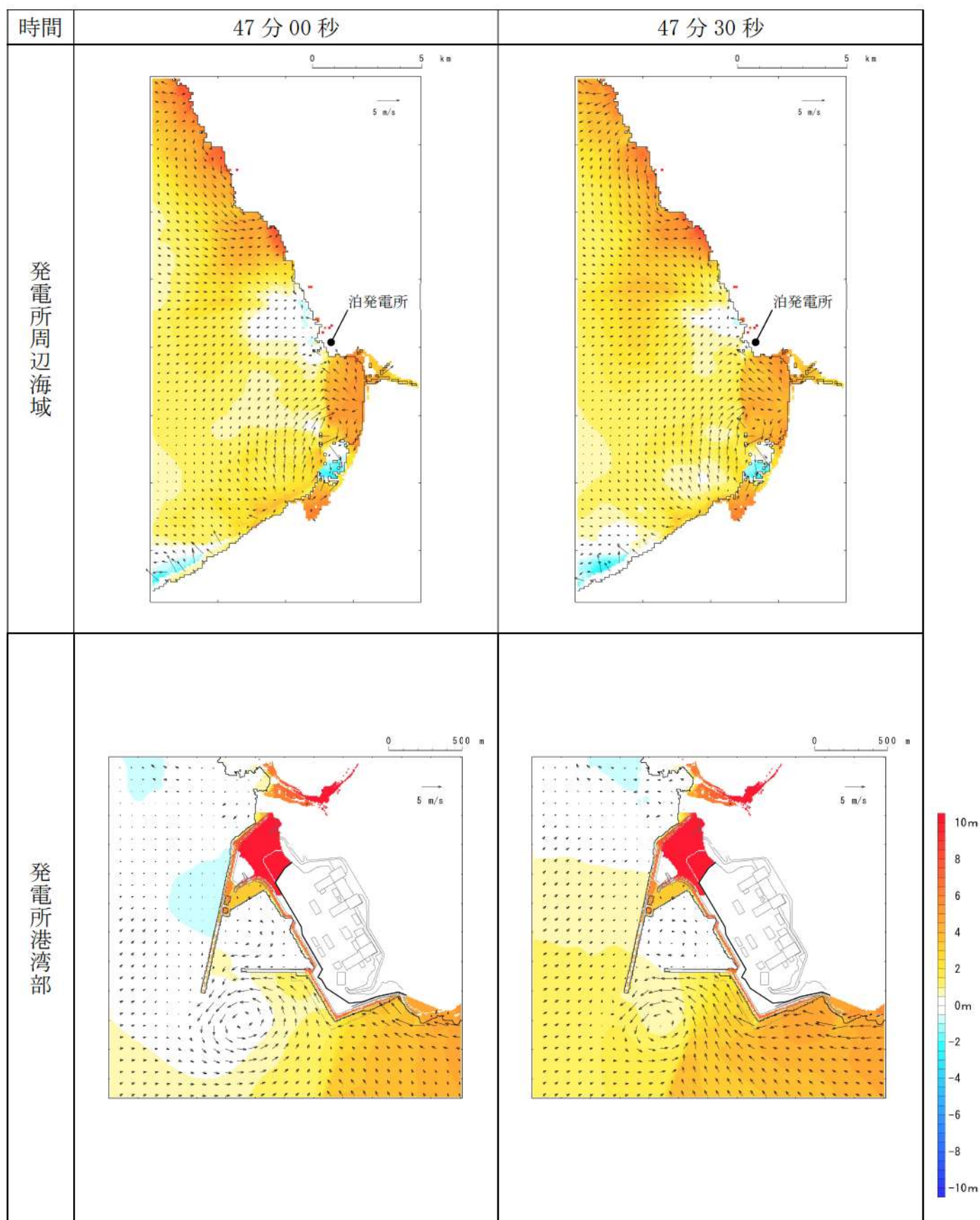
第 15 図-37 基準津波 I（防波堤損傷なし）の水位変動・流向ベクトル(37/50)
