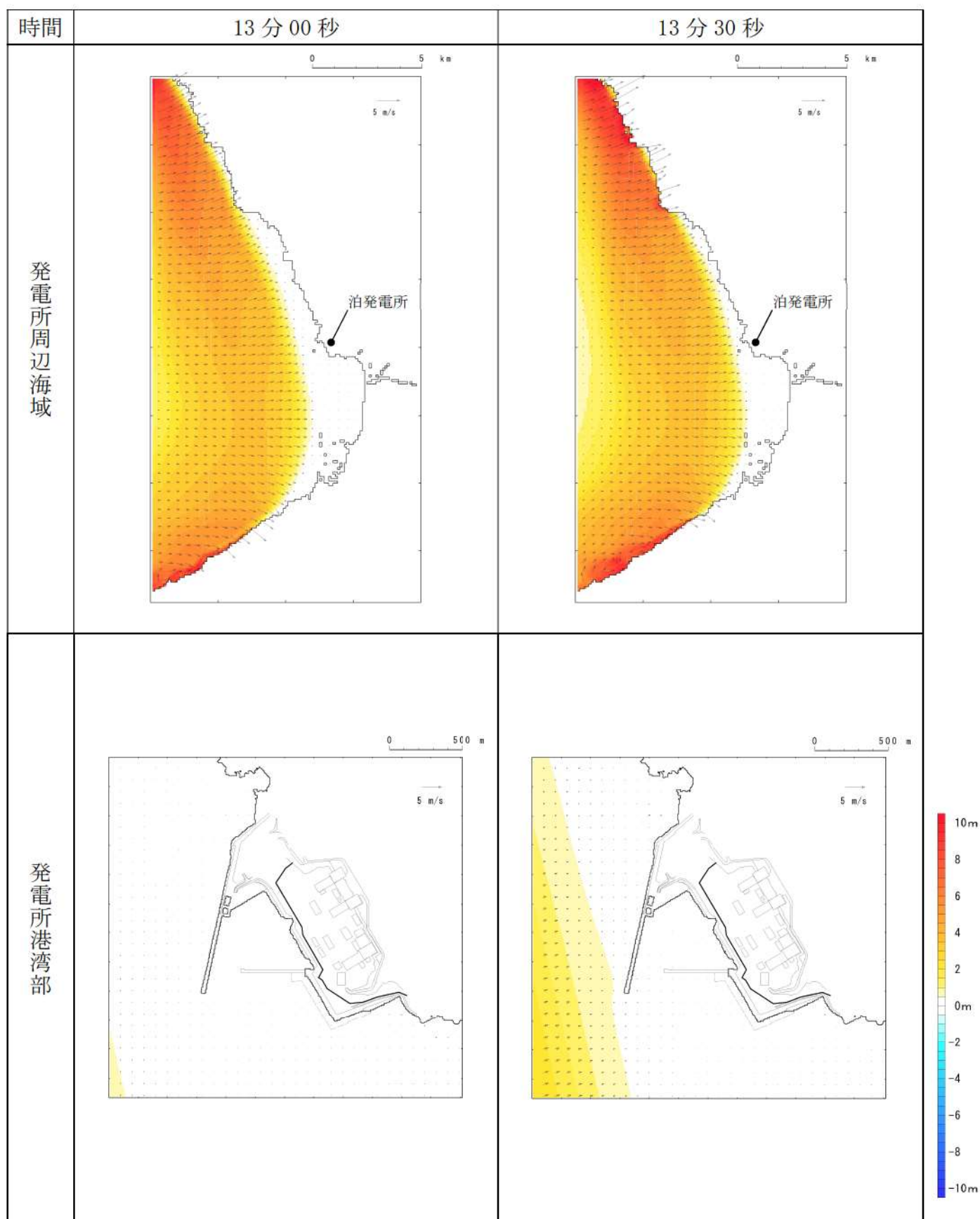
第 17 図-6 基準津波 K (南防波堤損傷) の水位変動・流向ベクトル (6/53)
