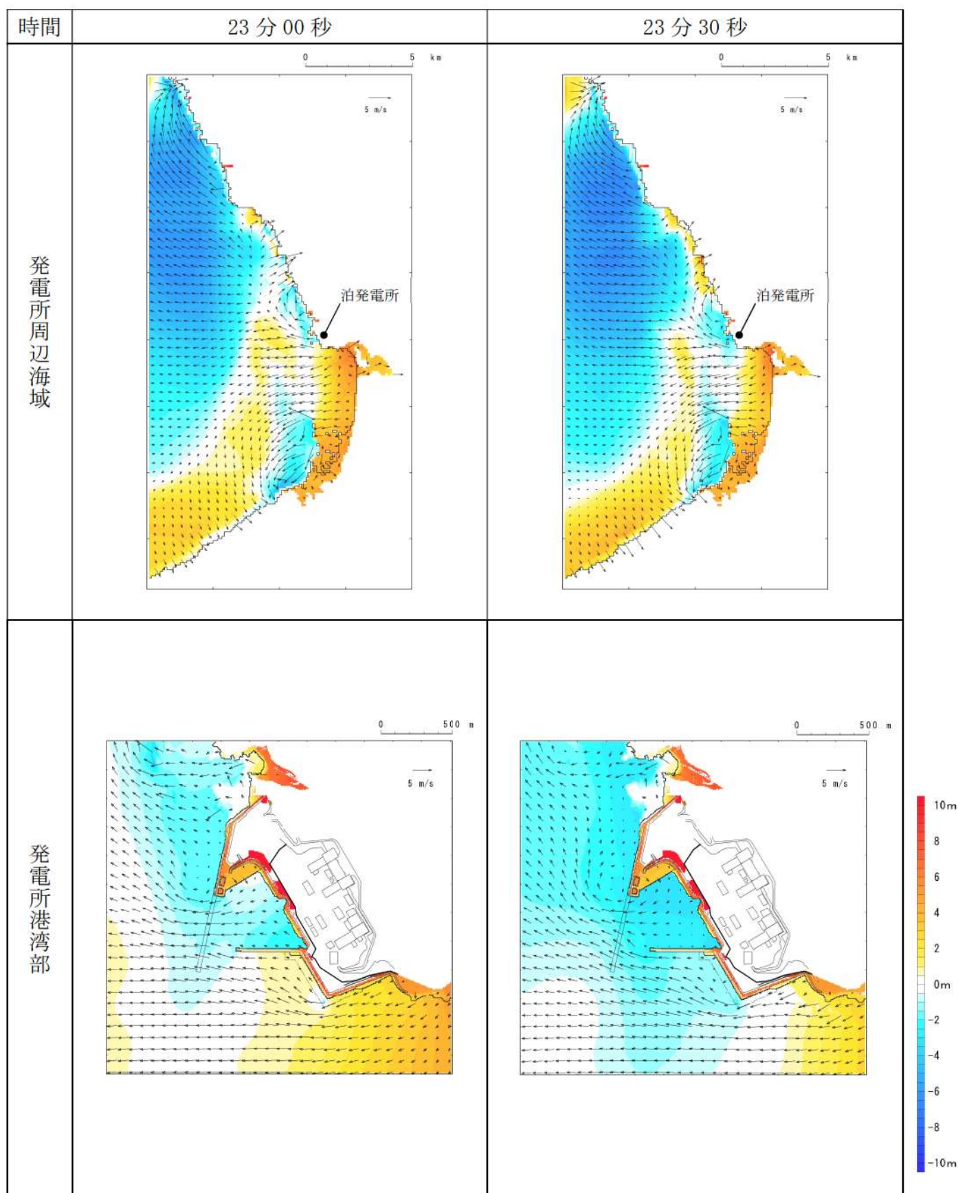
第 18 図-16 基準津波 L（北防波堤損傷）の水位変動・流向ベクトル(16/53)
