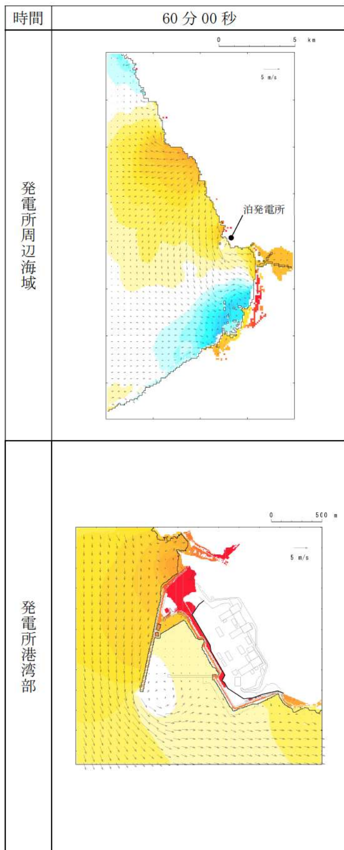
第 17 図-53 基準津波K（南防波堤損傷）の水位変動・流向ベクトル(53/53)
