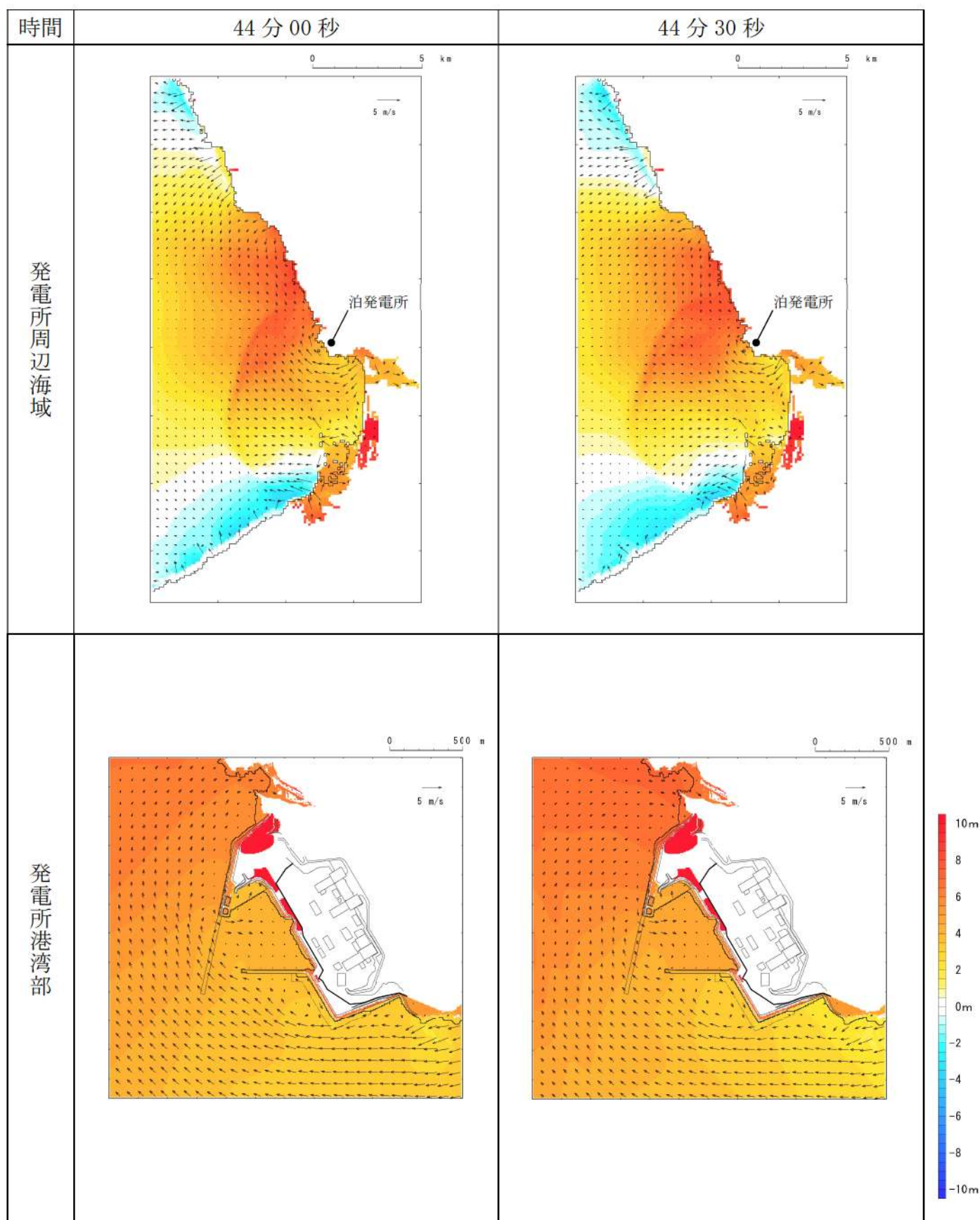
第 18 図-37 基準津波 L（北防波堤損傷）の水位変動・流向ベクトル(37/53)
