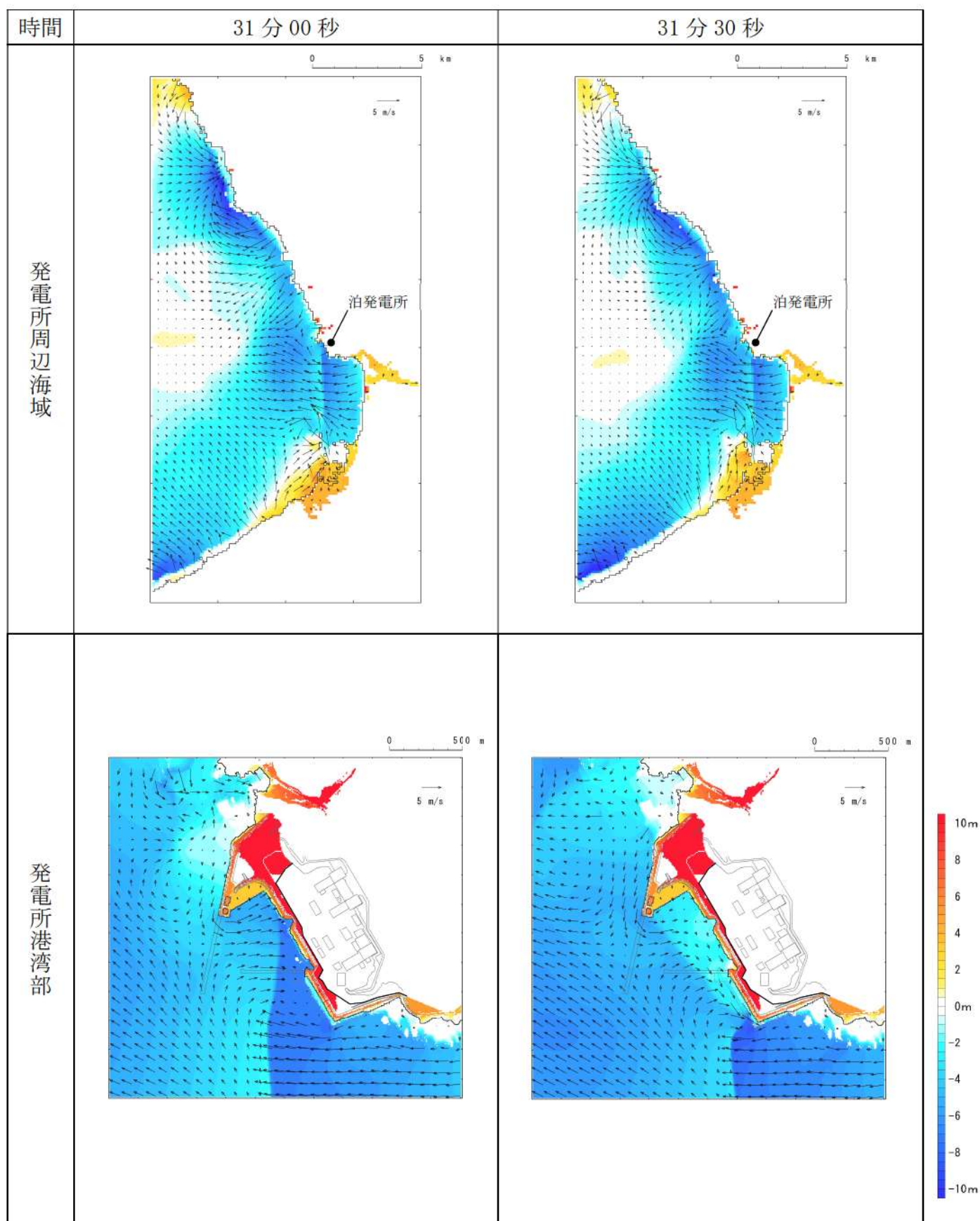
第 16 図-20 基準津波 J（北及び南防波堤損傷）の水位変動・流向ベクトル(20/49)
