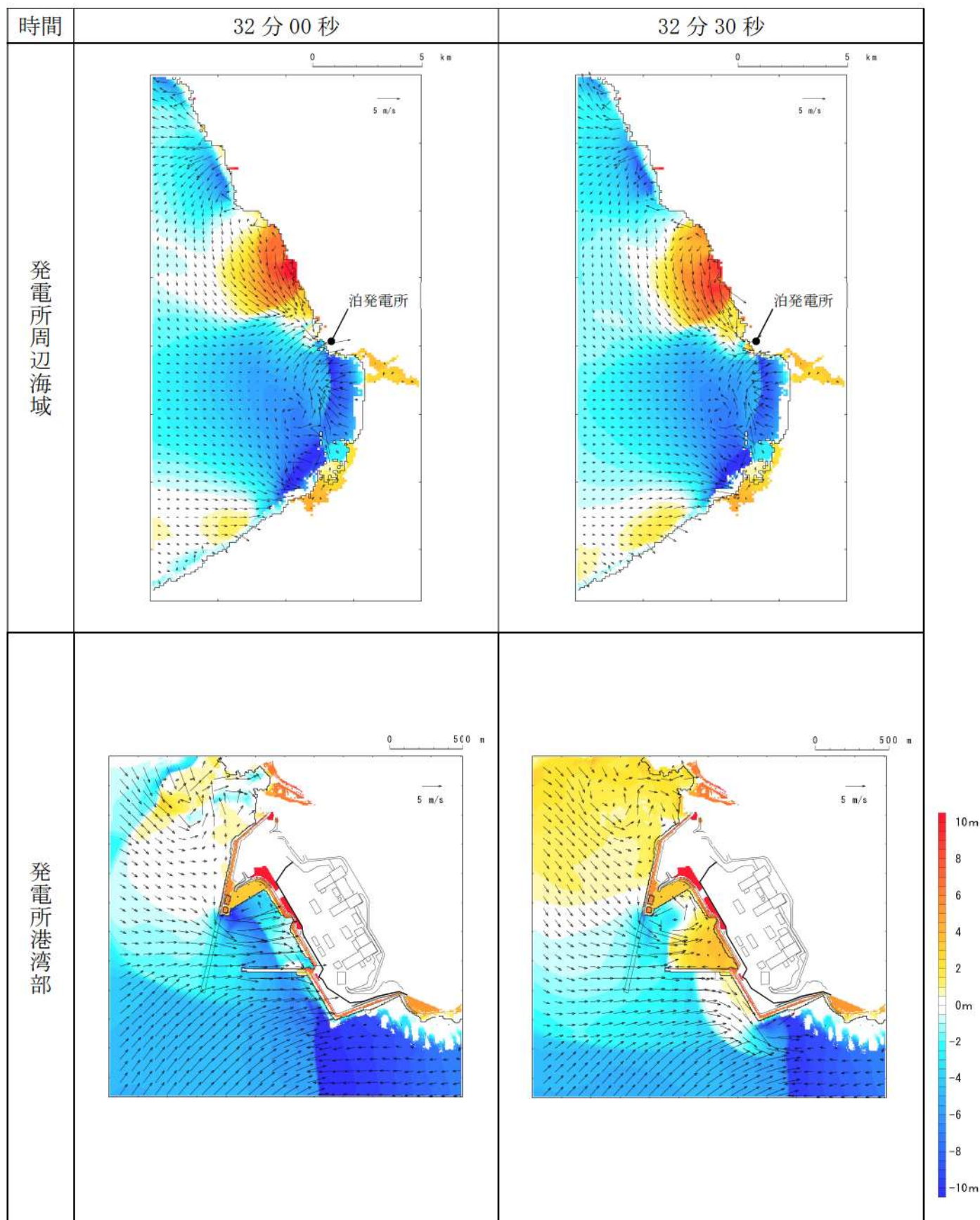
第 18 図-25 基準津波 L（北防波堤損傷）の水位変動・流向ベクトル (25/53)
