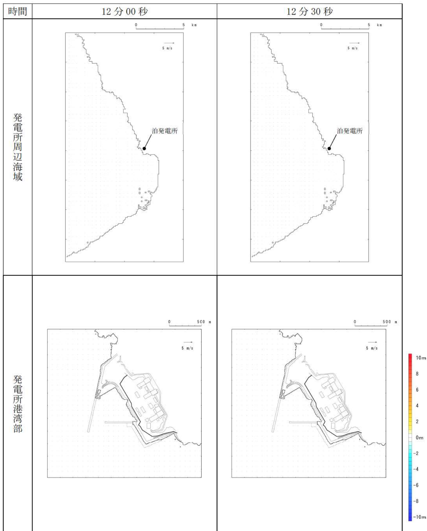
第 16 図-1 基準津波 J（北及び南防波堤損傷）の水位変動・流向ベクトル(1/49)
