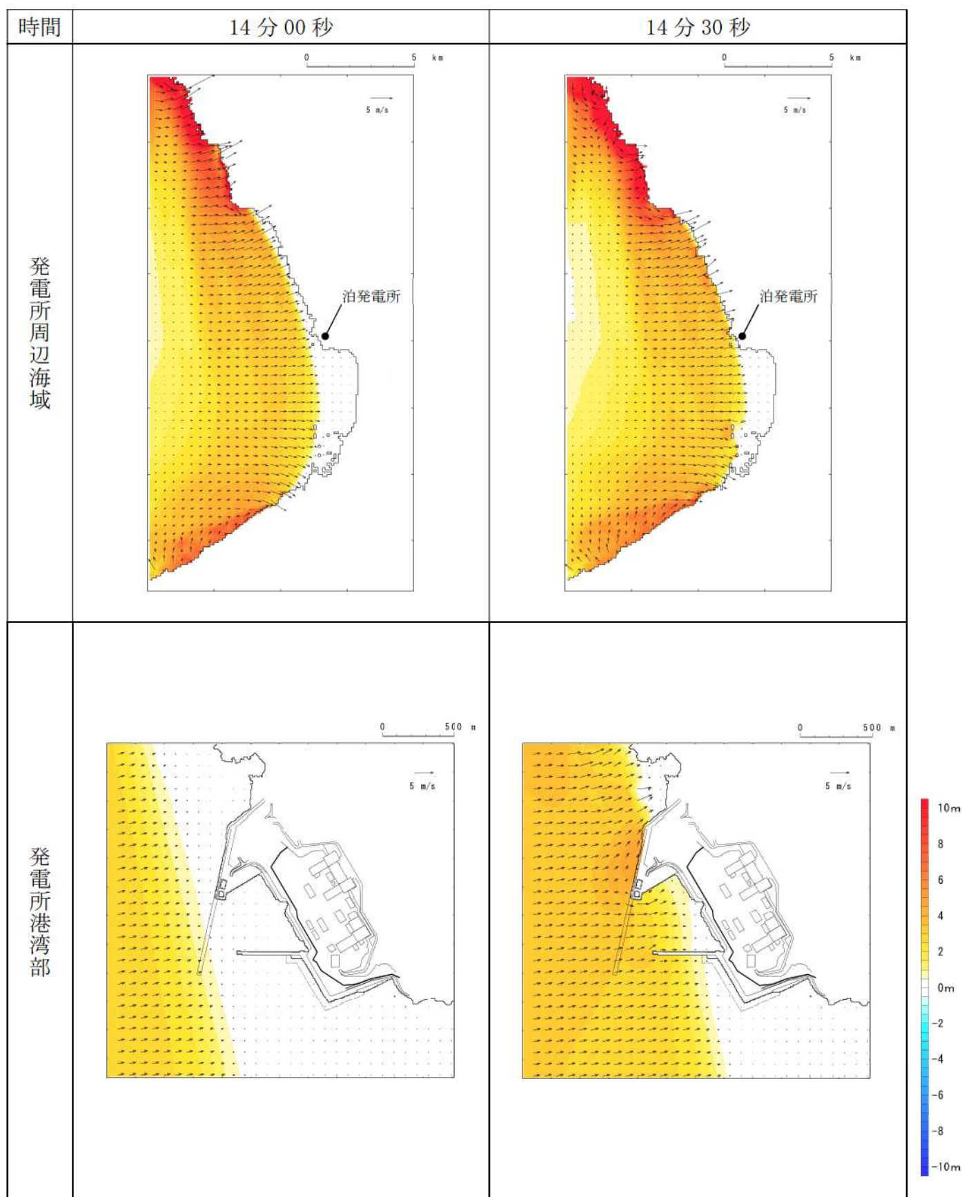
第 18 図-7 基準津波 L（北防波堤損傷）の水位変動・流向ベクトル (7/53)
