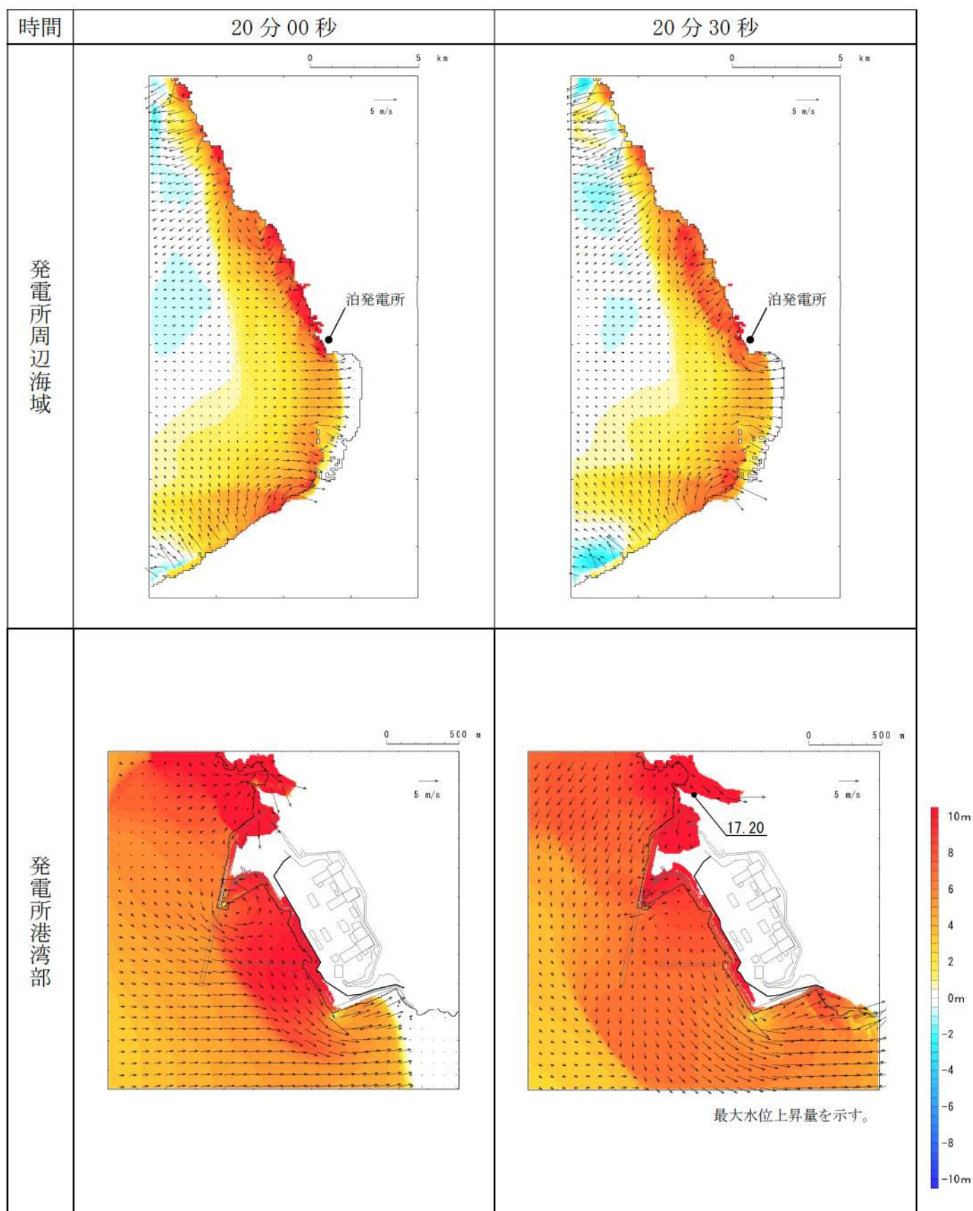
第 16 図-9 基準津波 J（北及び南防波堤損傷）の水位変動・流向ベクトル (9/49)
