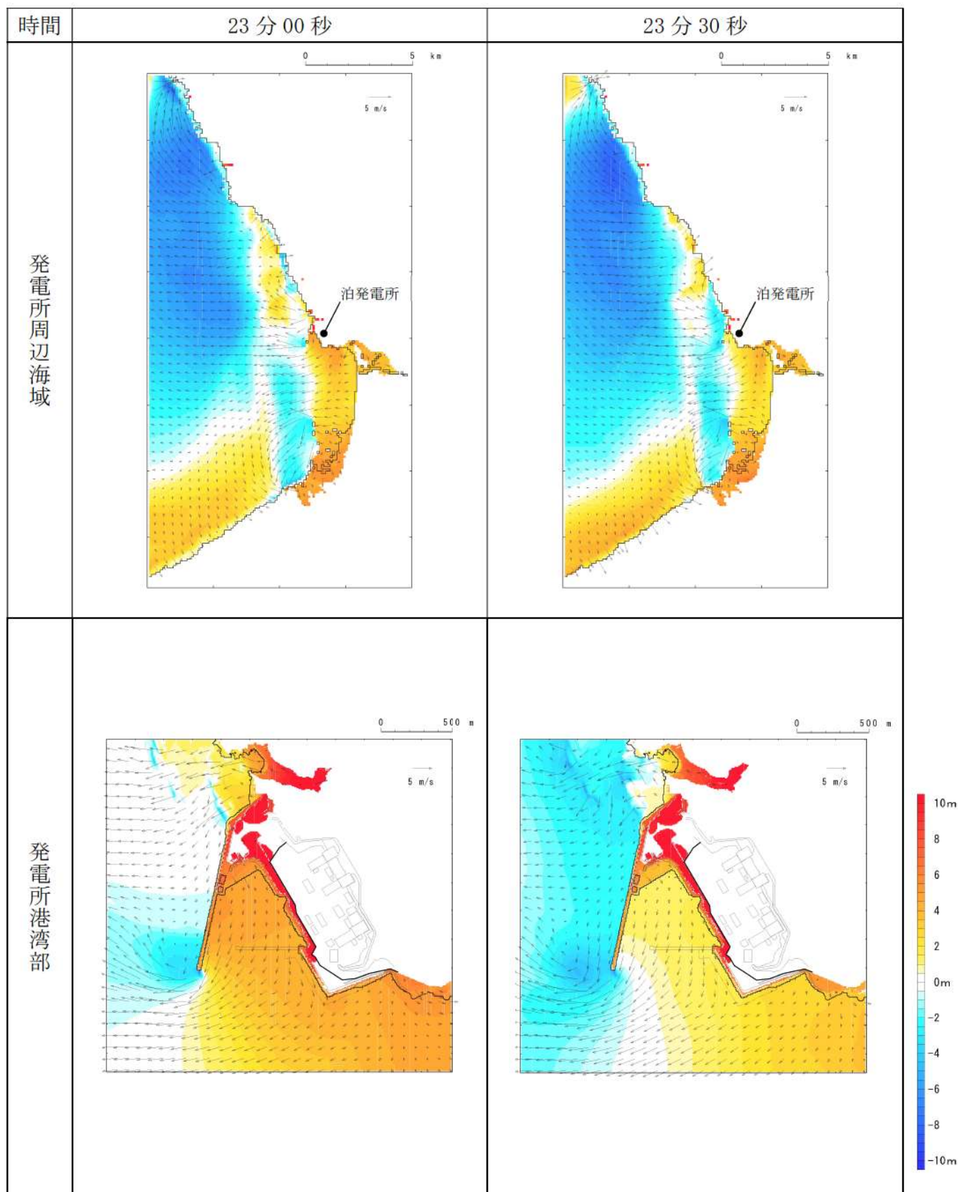
第 17 図-16 基準津波K（南防波堤損傷）の水位変動・流向ベクトル(16/53)
