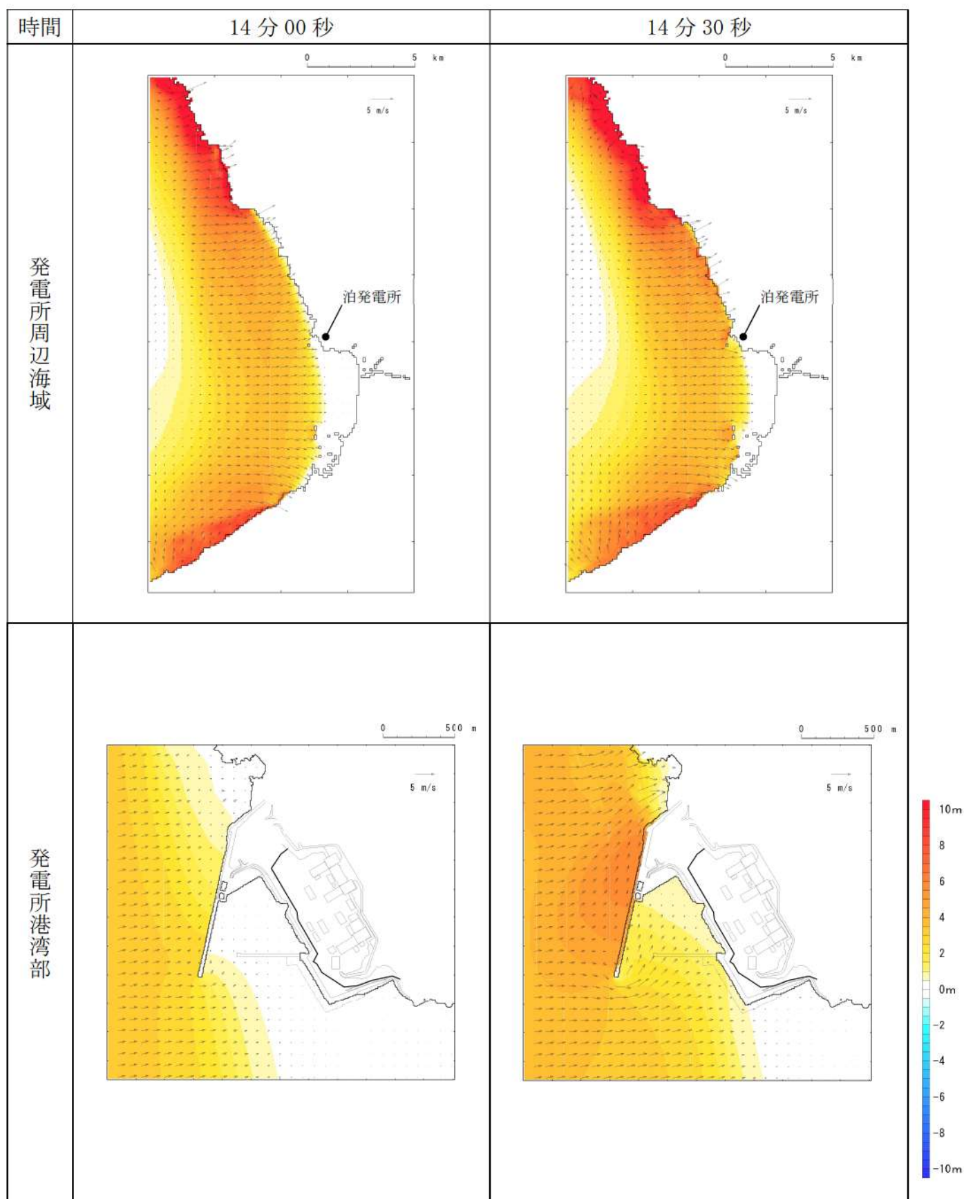
第 17 図-7 基準津波K（南防波堤損傷）の水位変動・流向ベクトル(7/53)
