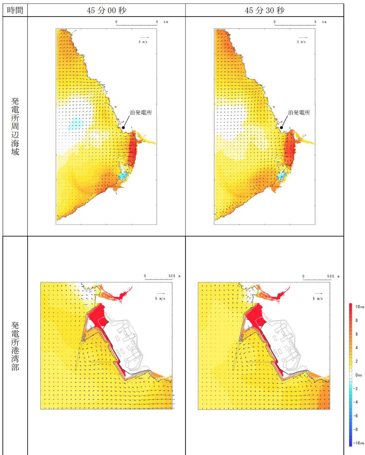
第 16 図-34 基準津波 J（北及び南防波堤損傷）の水位変動・流向ベクトル(34/49)
