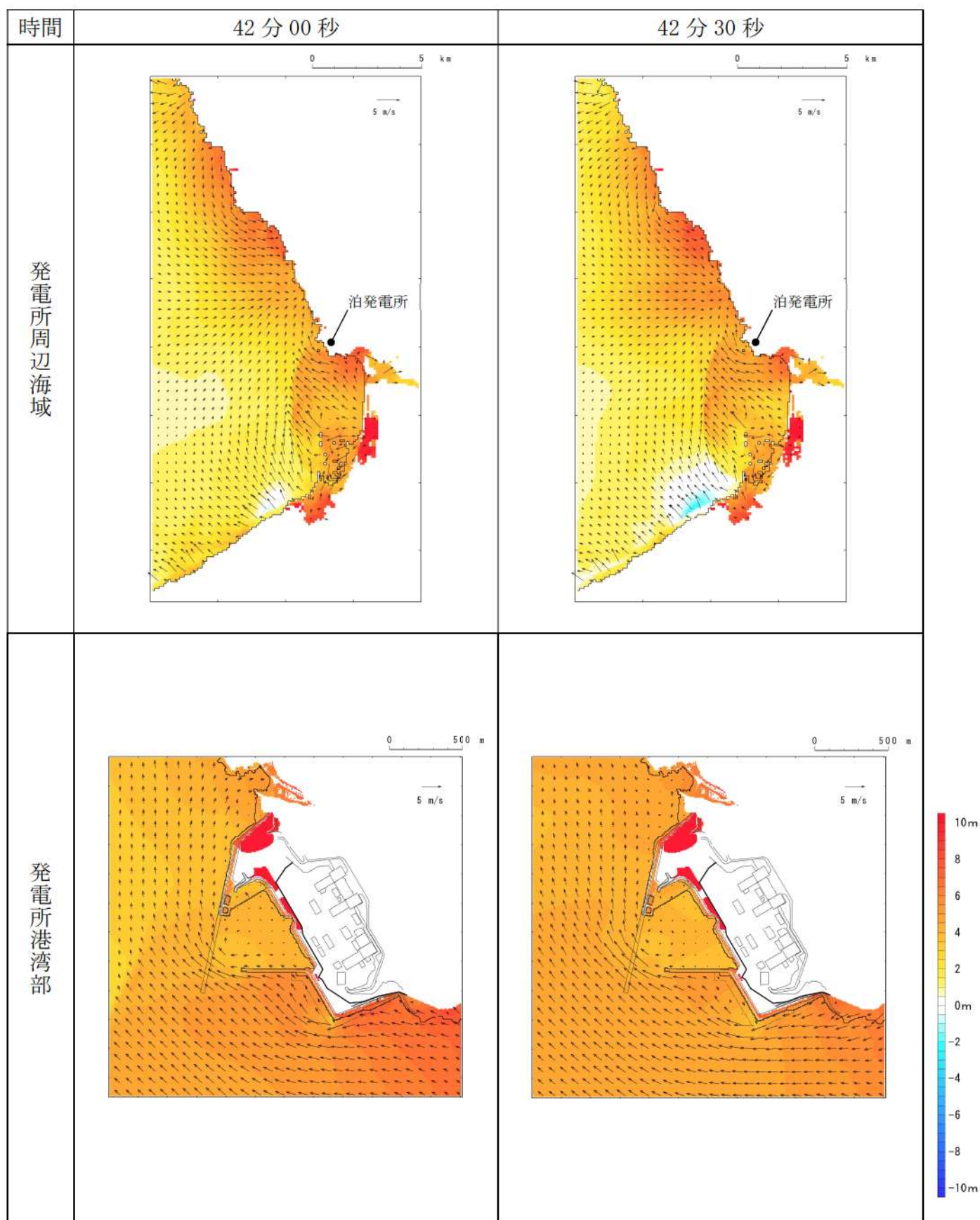
第 18 図-35 基準津波 L（北防波堤損傷）の水位変動・流向ベクトル(35/53)
