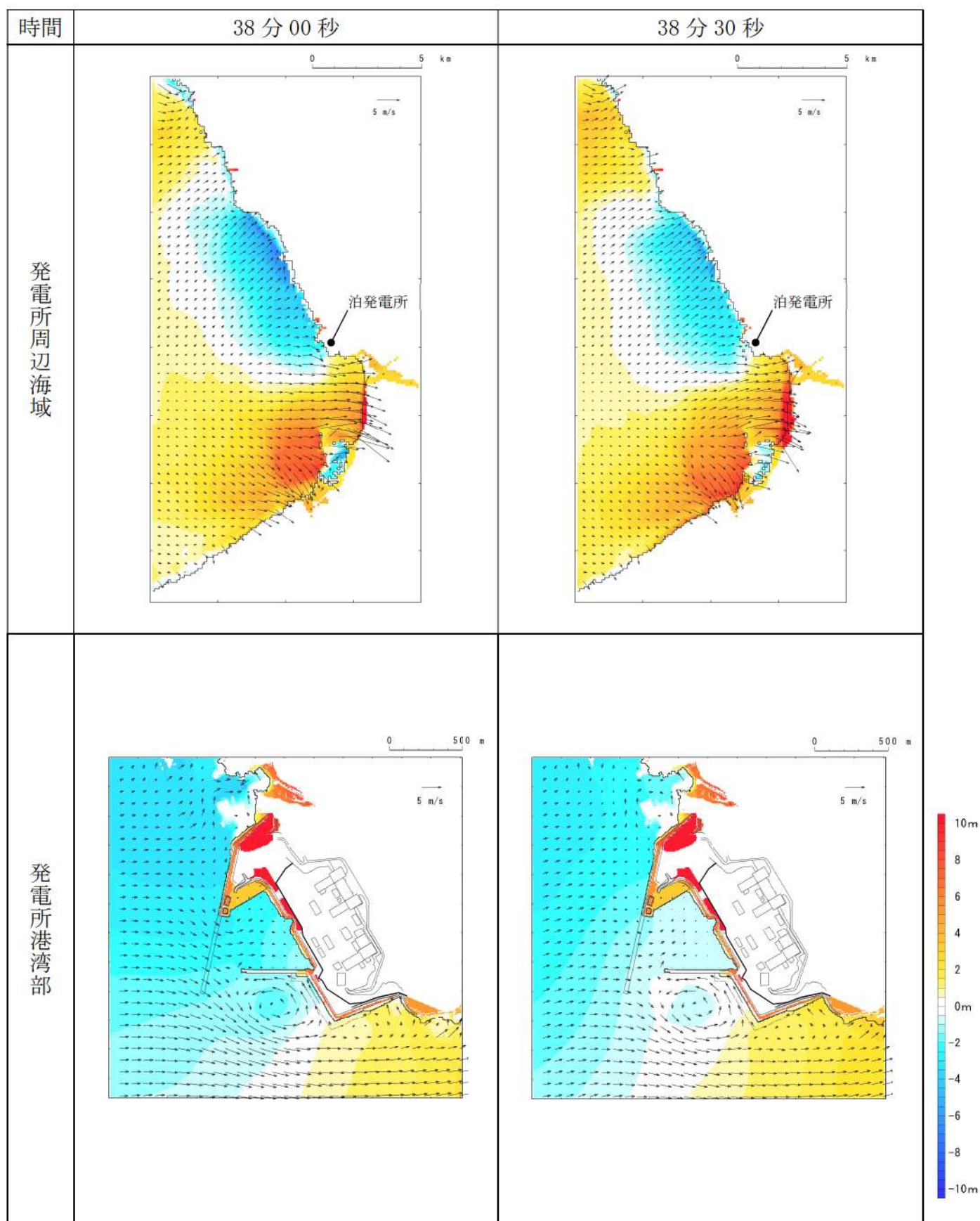
第 18 図-31 基準津波 L（北防波堤損傷）の水位変動・流向ベクトル(31/53)
