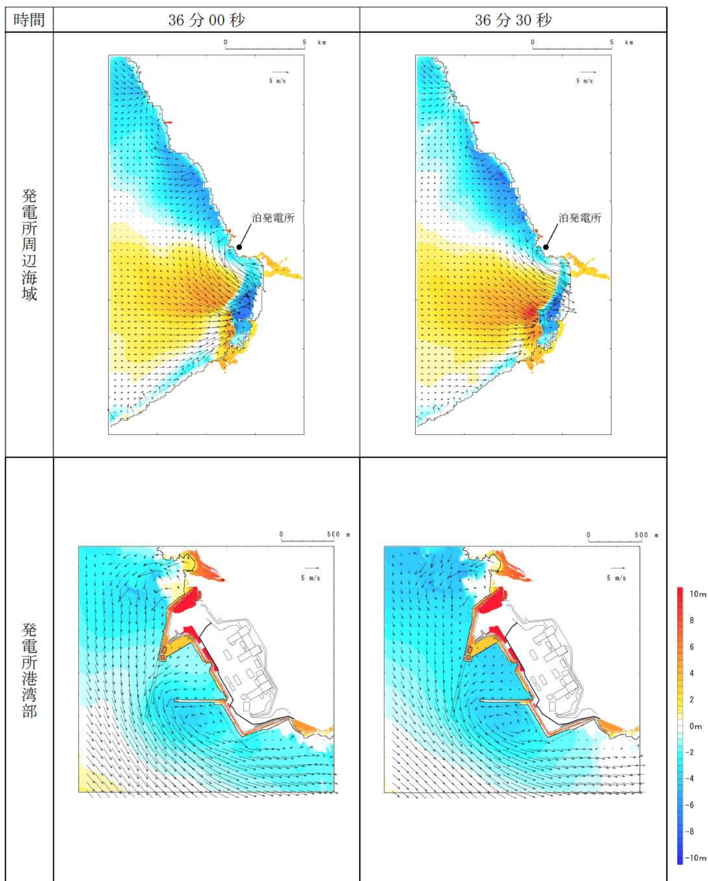
第 18 図-29 基準津波 L（北防波堤損傷）の水位変動・流向ベクトル (29/53)
