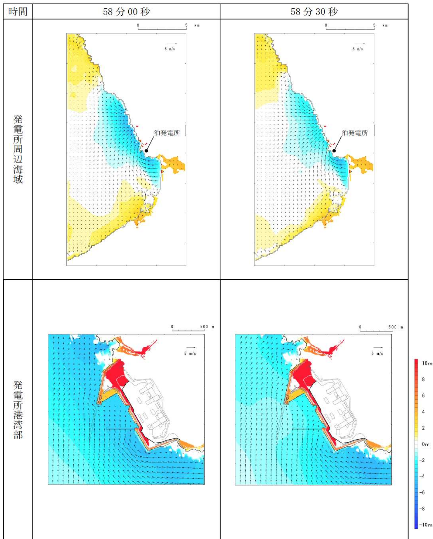
第 16 図-47 基準津波 J（北及び南防波堤損傷）の水位変動・流向ベクトル(47/49)
