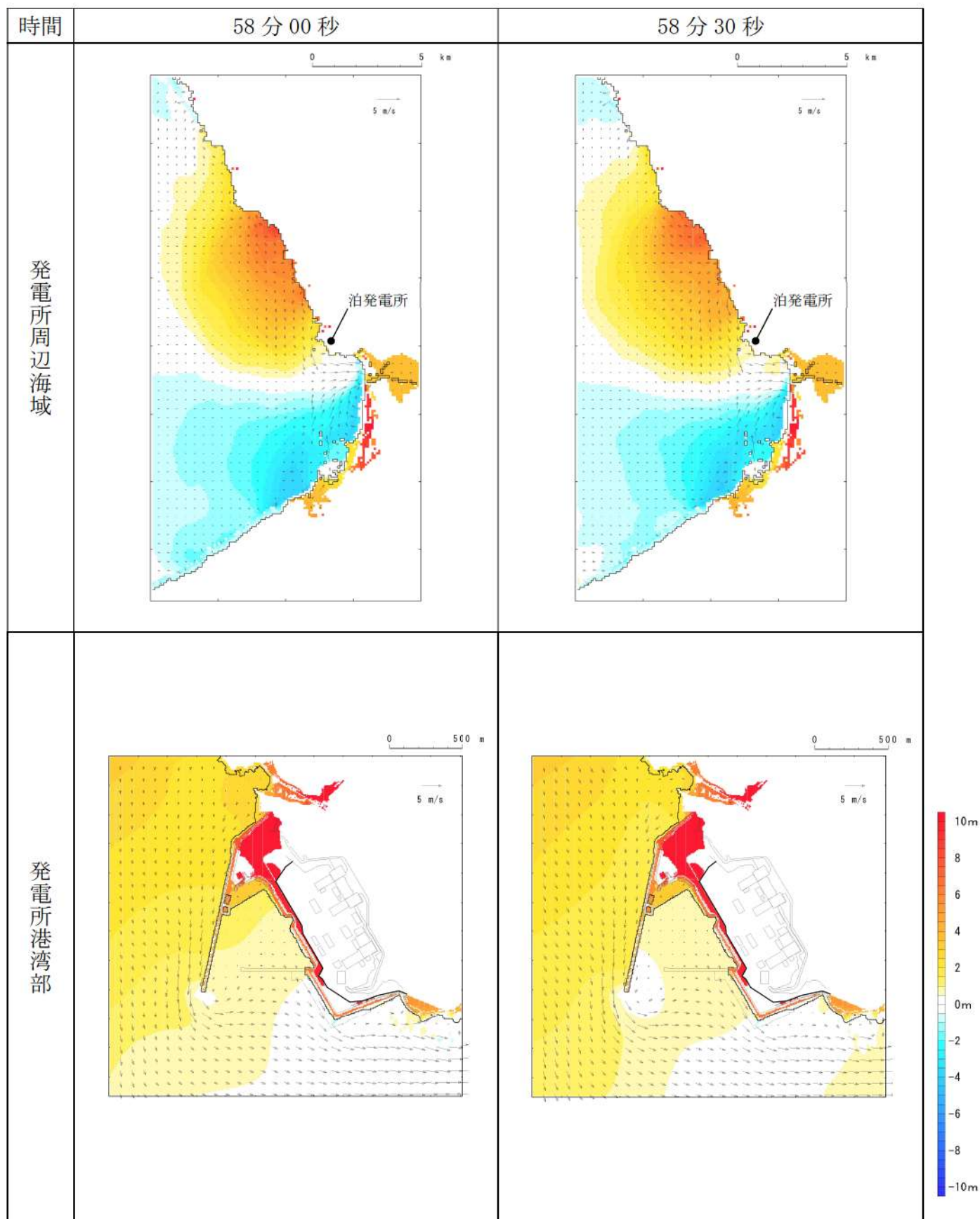
第 17 図-51 基準津波K（南防波堤損傷）の水位変動・流向ベクトル(51/53)
