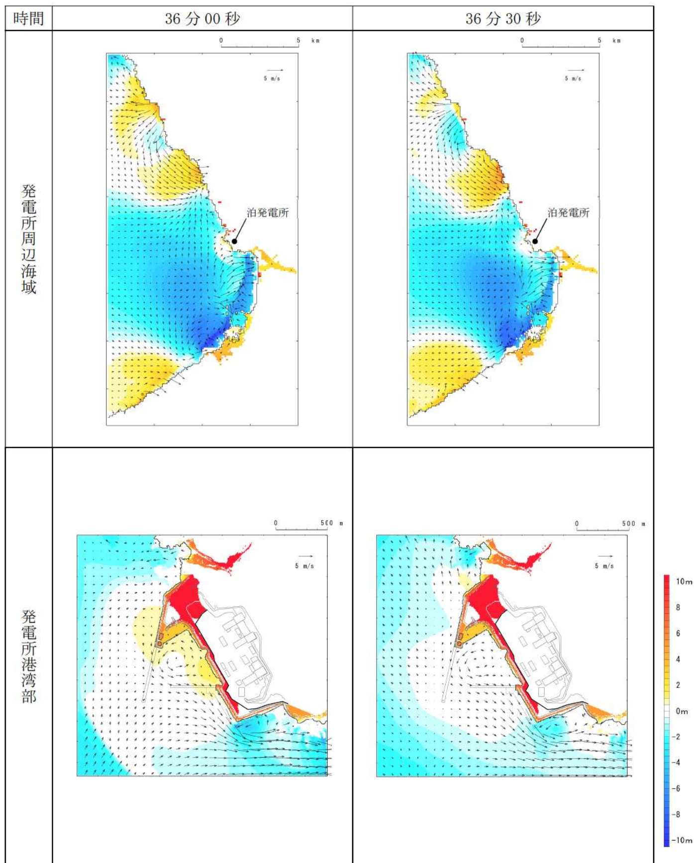
第 16 図-25 基準津波 J（北及び南防波堤損傷）の水位変動・流向ベクトル(25/49)
