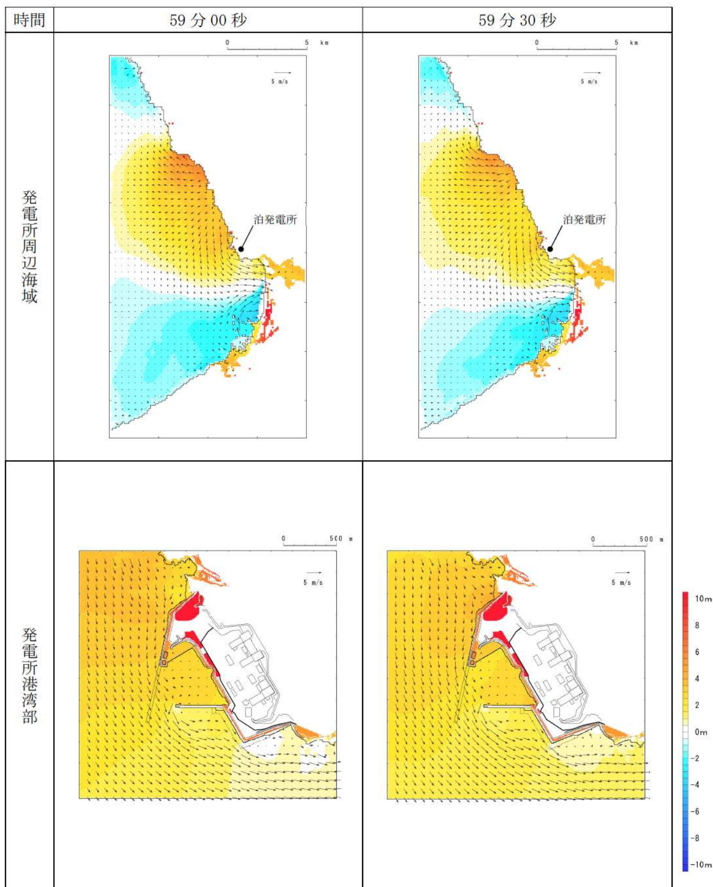
第 18 図-52 基準津波 L（北防波堤損傷）の水位変動・流向ベクトル(52/53)
