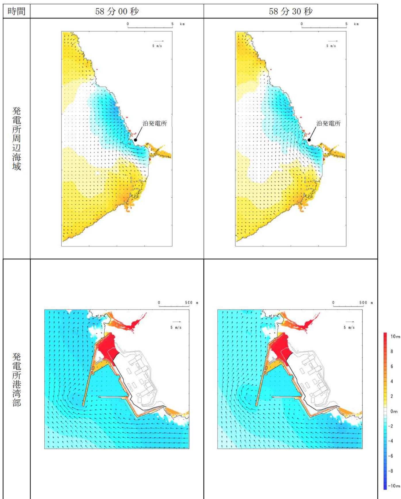
第 15 図-48 基準津波 I（防波堤損傷なし）の水位変動・流向ベクトル(48/50)
