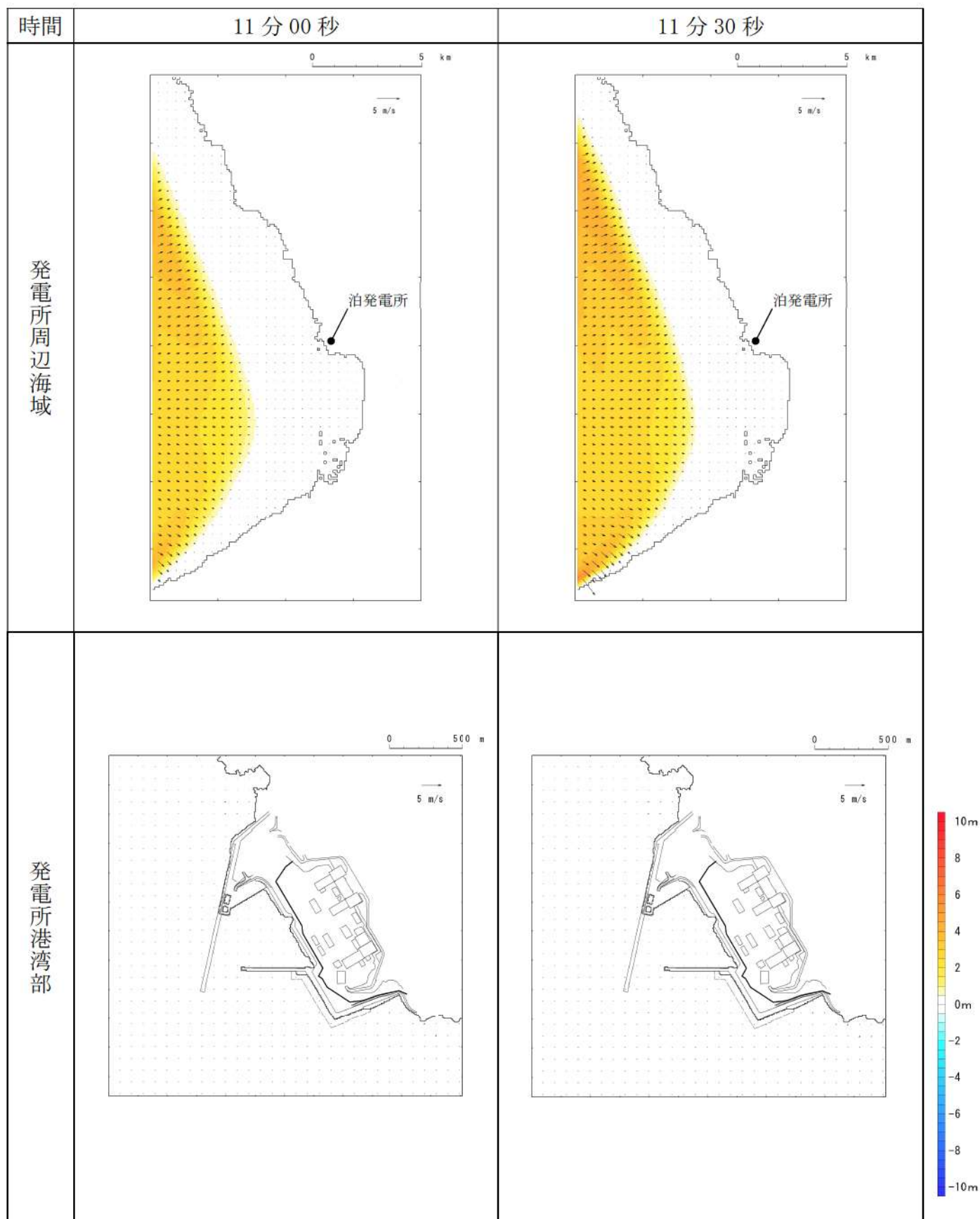
第 18 図-4 基準津波 L（北防波堤損傷）の水位変動・流向ベクトル (4/53)
