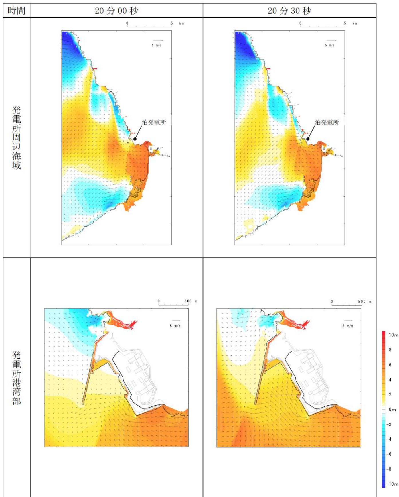
第 17 図-13 基準津波K（南防波堤損傷）の水位変動・流向ベクトル(13/53)
