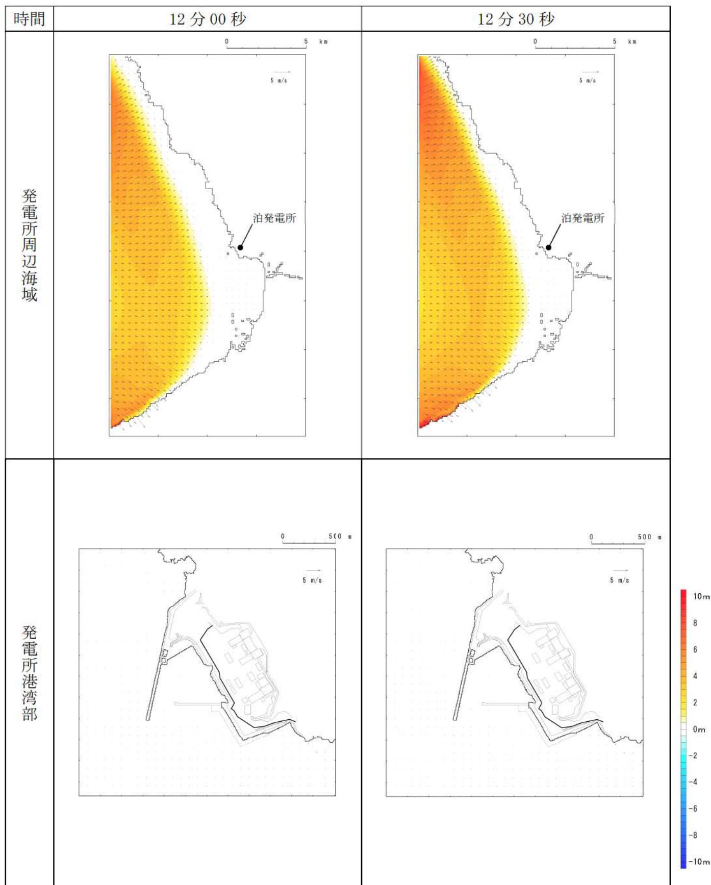
第 17 図-5 基準津波K（南防波堤損傷）の水位変動・流向ベクトル(5/53)
