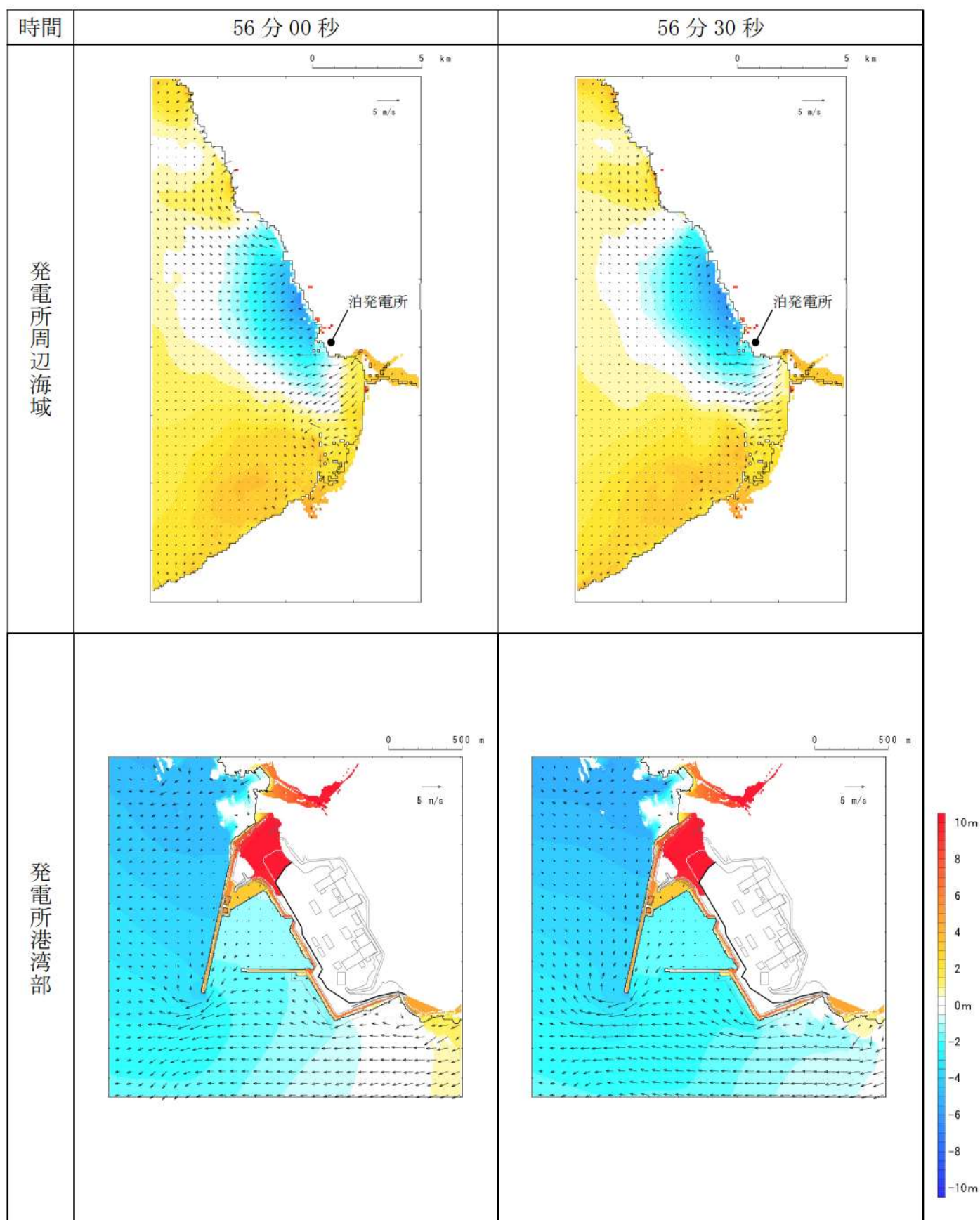
第 15 図-46 基準津波 I（防波堤損傷なし）の水位変動・流向ベクトル(46/50)
