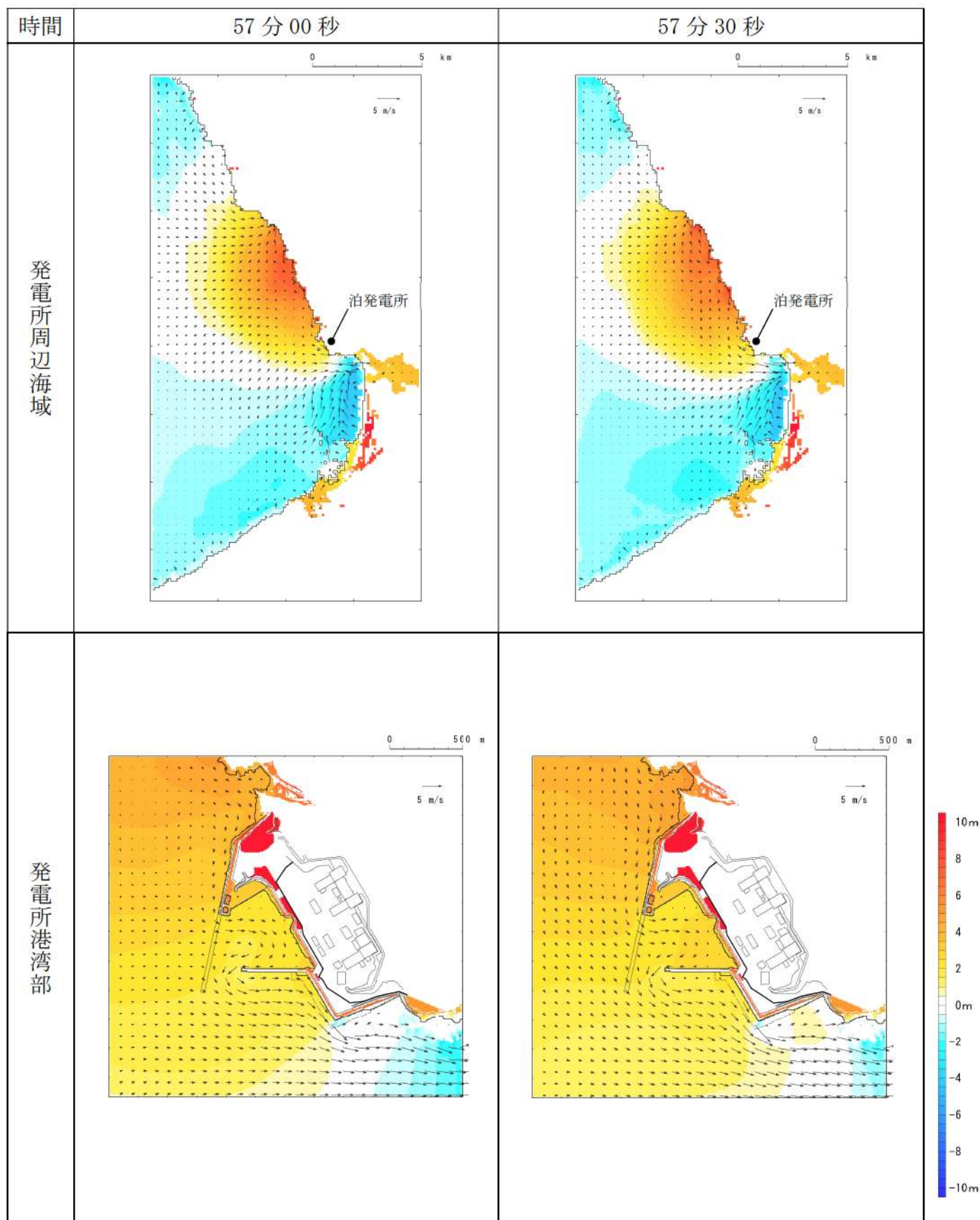
第 18 図-50 基準津波 L（北防波堤損傷）の水位変動・流向ベクトル(50/53)
