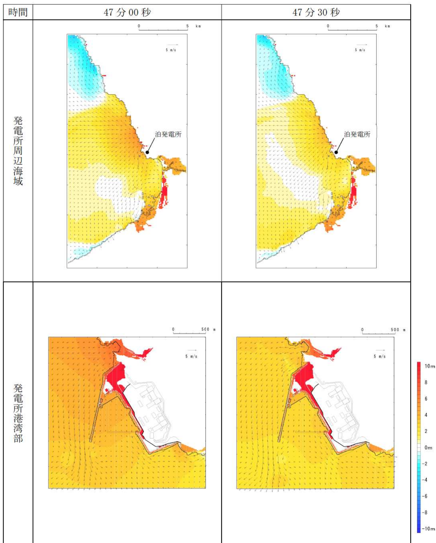
第 17 図-40 基準津波K（南防波堤損傷）の水位変動・流向ベクトル(40/53)
