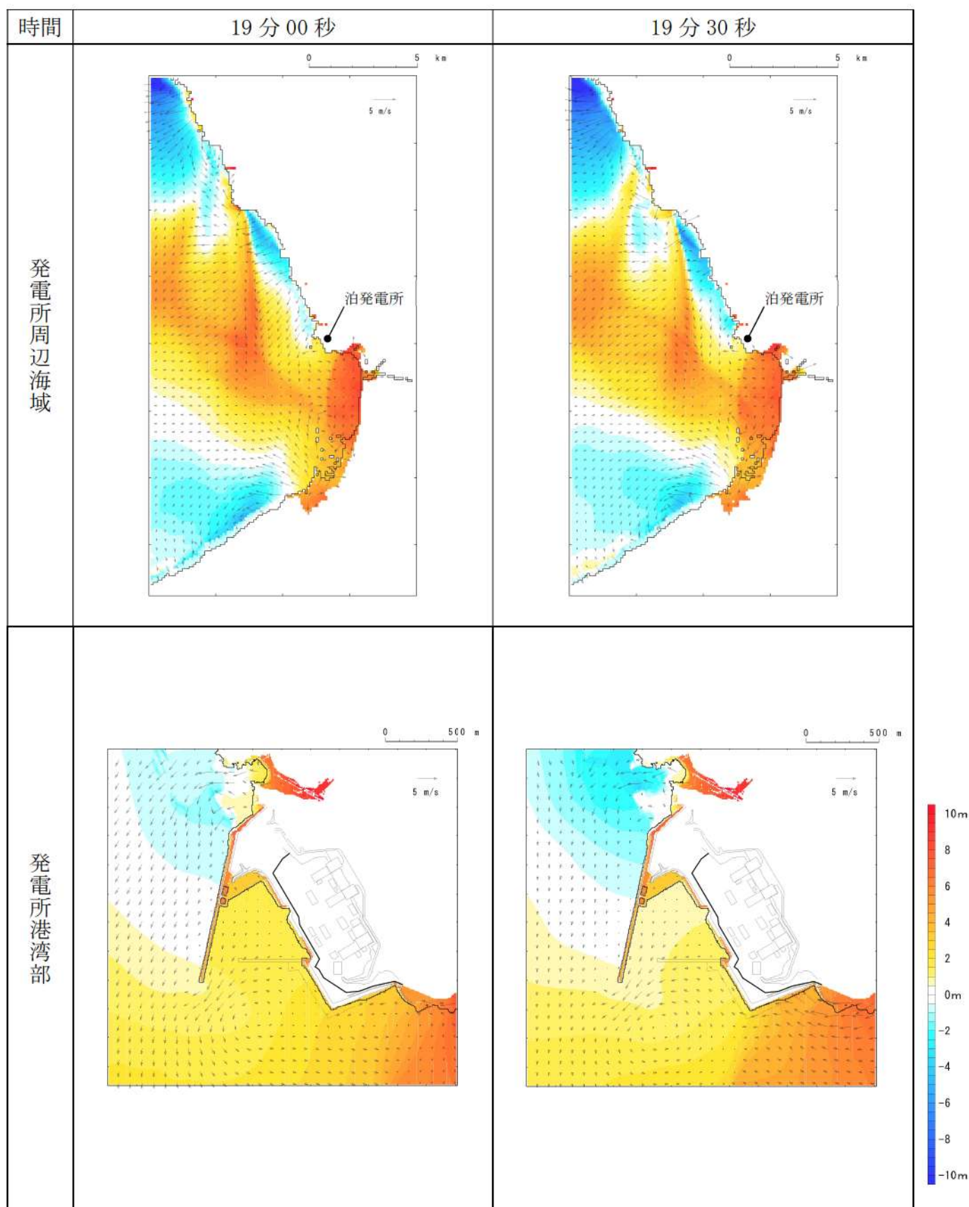
第 17 図-12 基準津波K（南防波堤損傷）の水位変動・流向ベクトル(12/53)
