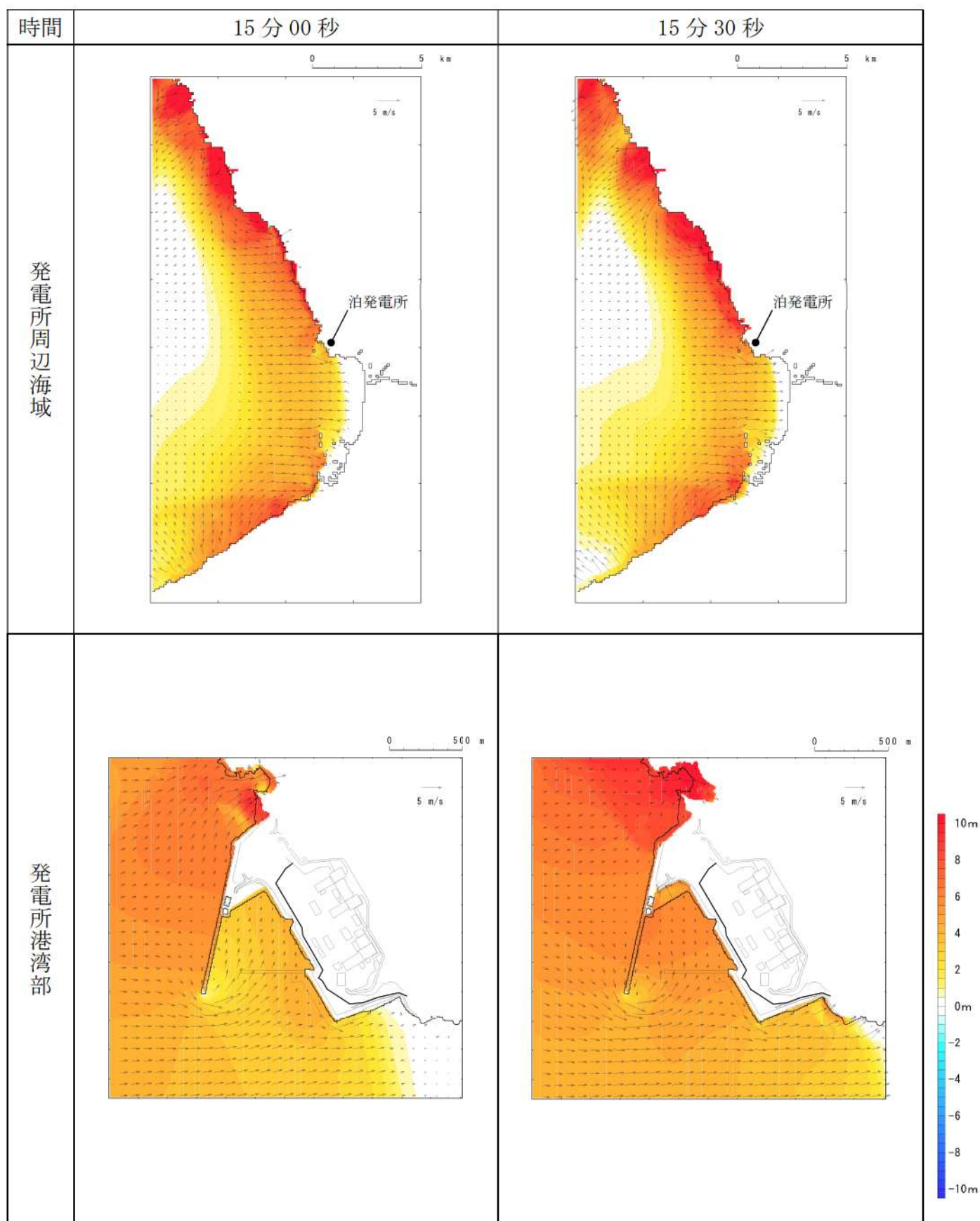
第 17 図-8 基準津波 K（南防波堤損傷）の水位変動・流向ベクトル (8/53)
