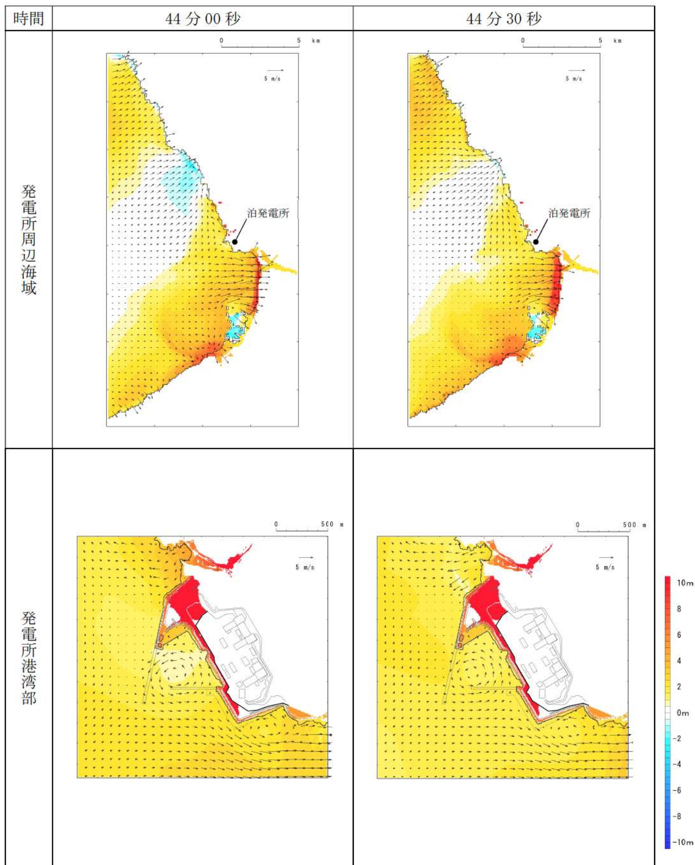
第 16 図-33 基準津波 J（北及び南防波堤損傷）の水位変動・流向ベクトル(33/49)
