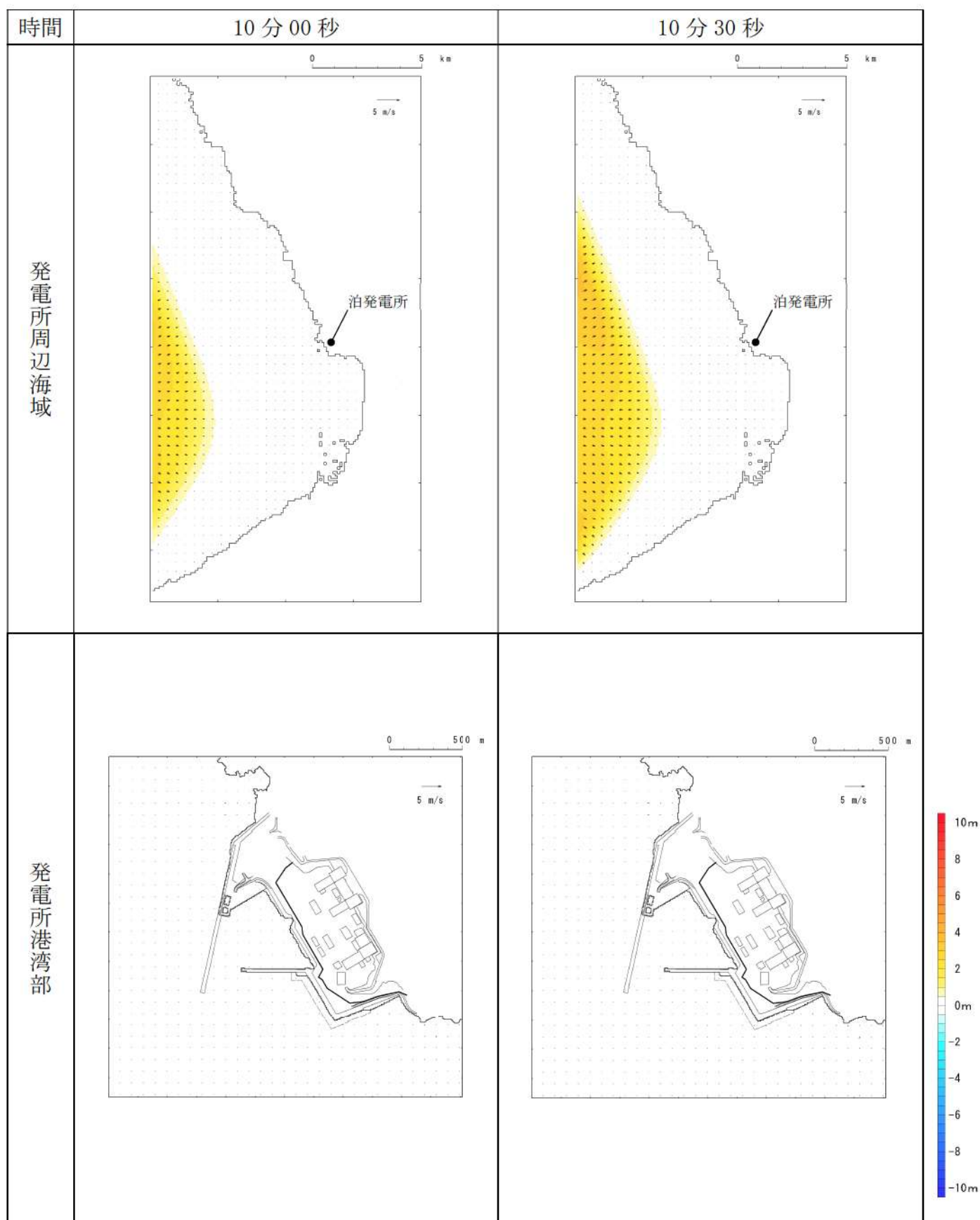
第 18 図-3 基準津波 L（北防波堤損傷）の水位変動・流向ベクトル (3/53)
