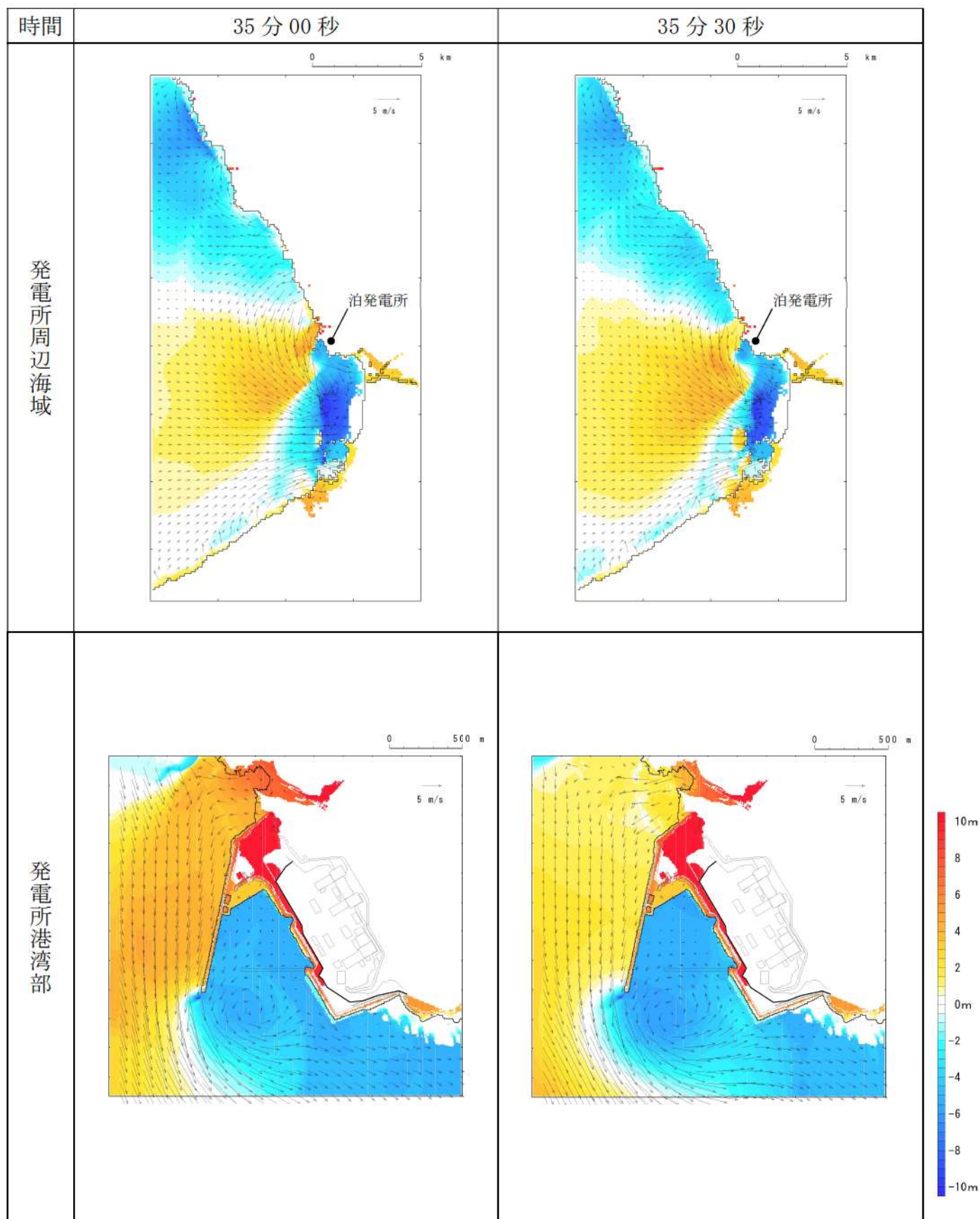
第 17 図-28 基準津波K（南防波堤損傷）の水位変動・流向ベクトル(28/53)
