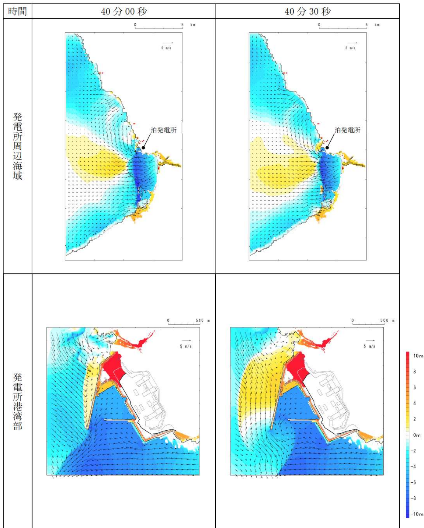
第 15 図-30 基準津波 I（防波堤損傷なし）の水位変動・流向ベクトル(30/50)
