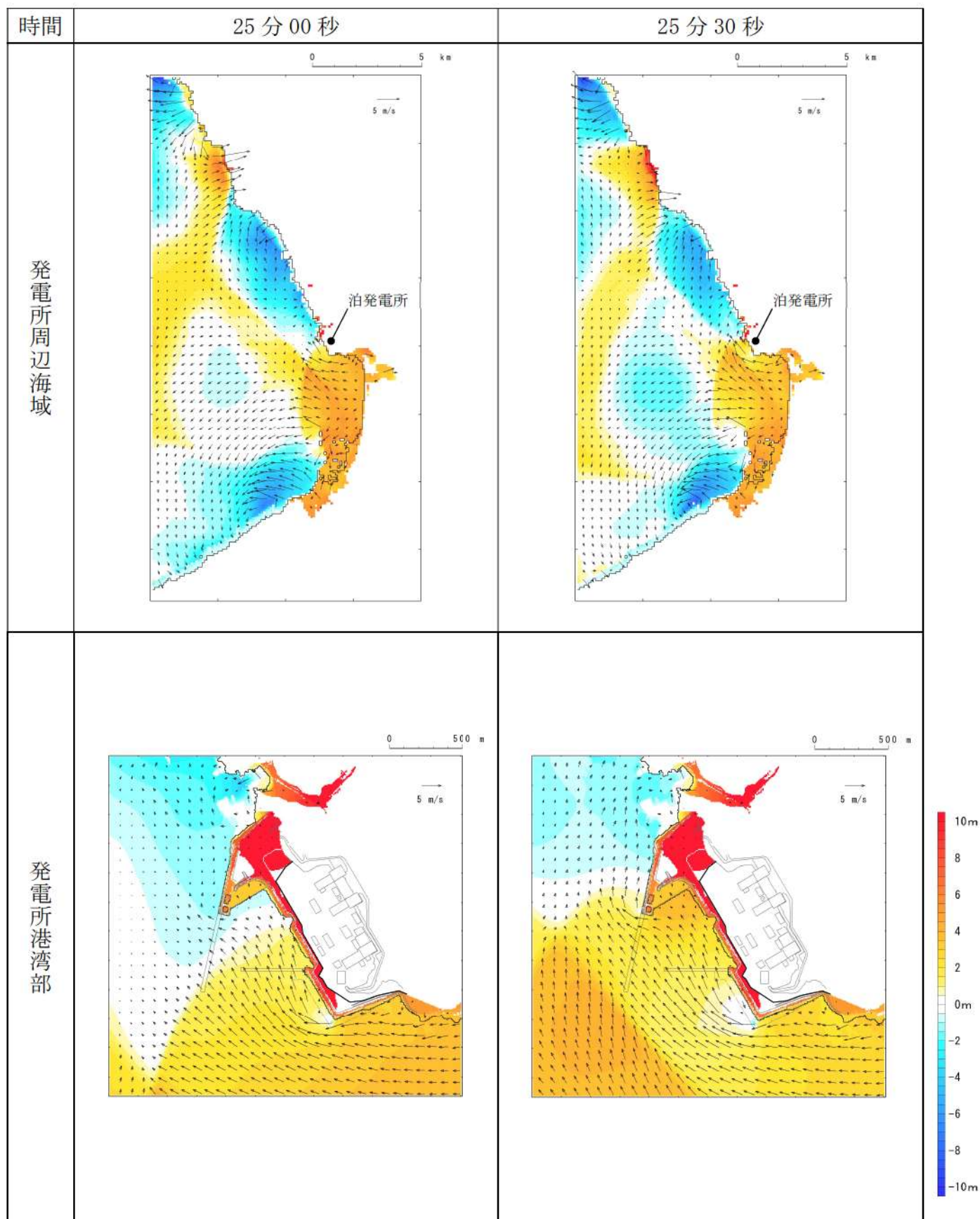
第 16 図-14 基準津波 J（北及び南防波堤損傷）の水位変動・流向ベクトル(14/49)
