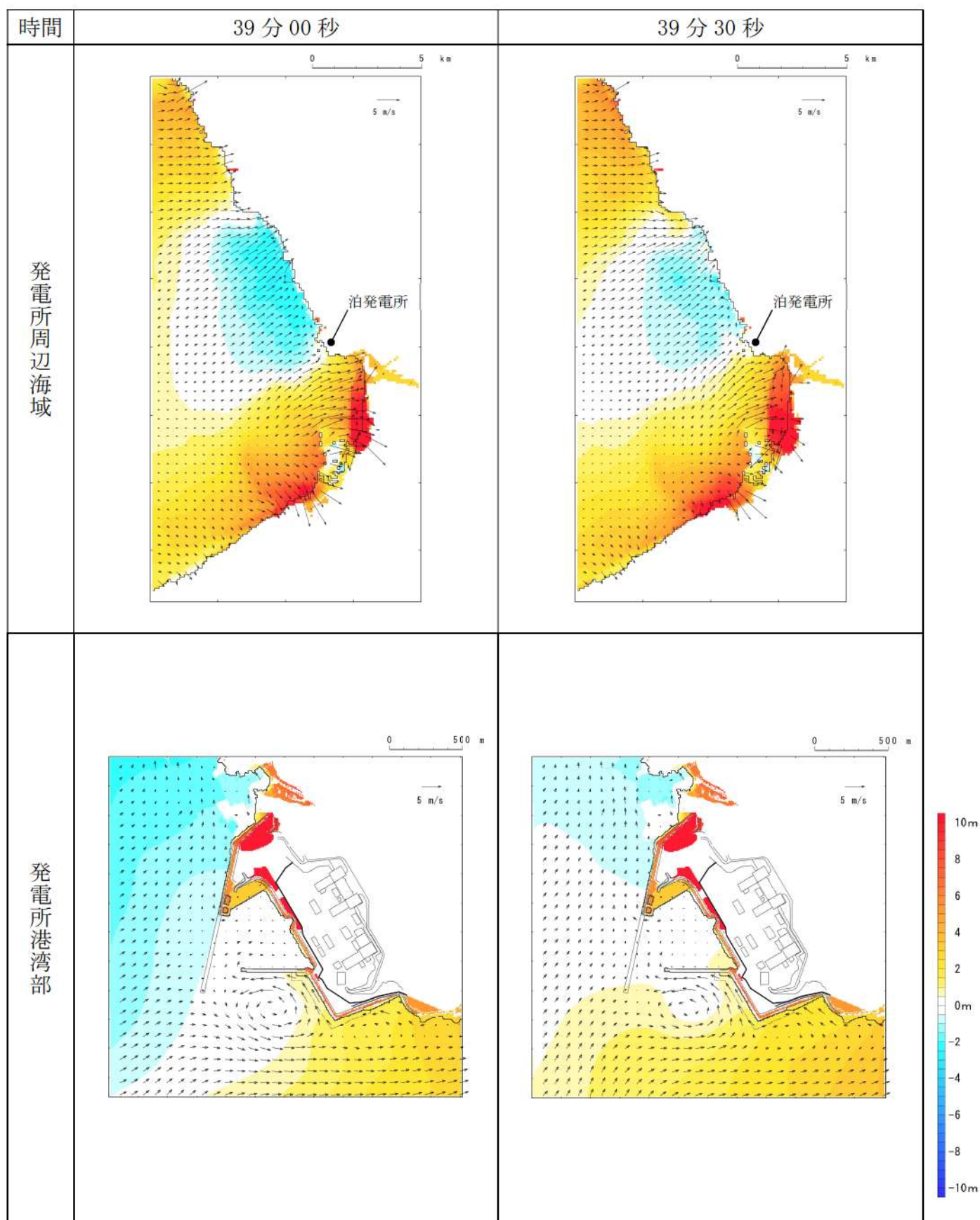
第 18 図-32 基準津波 L（北防波堤損傷）の水位変動・流向ベクトル(32/53)
