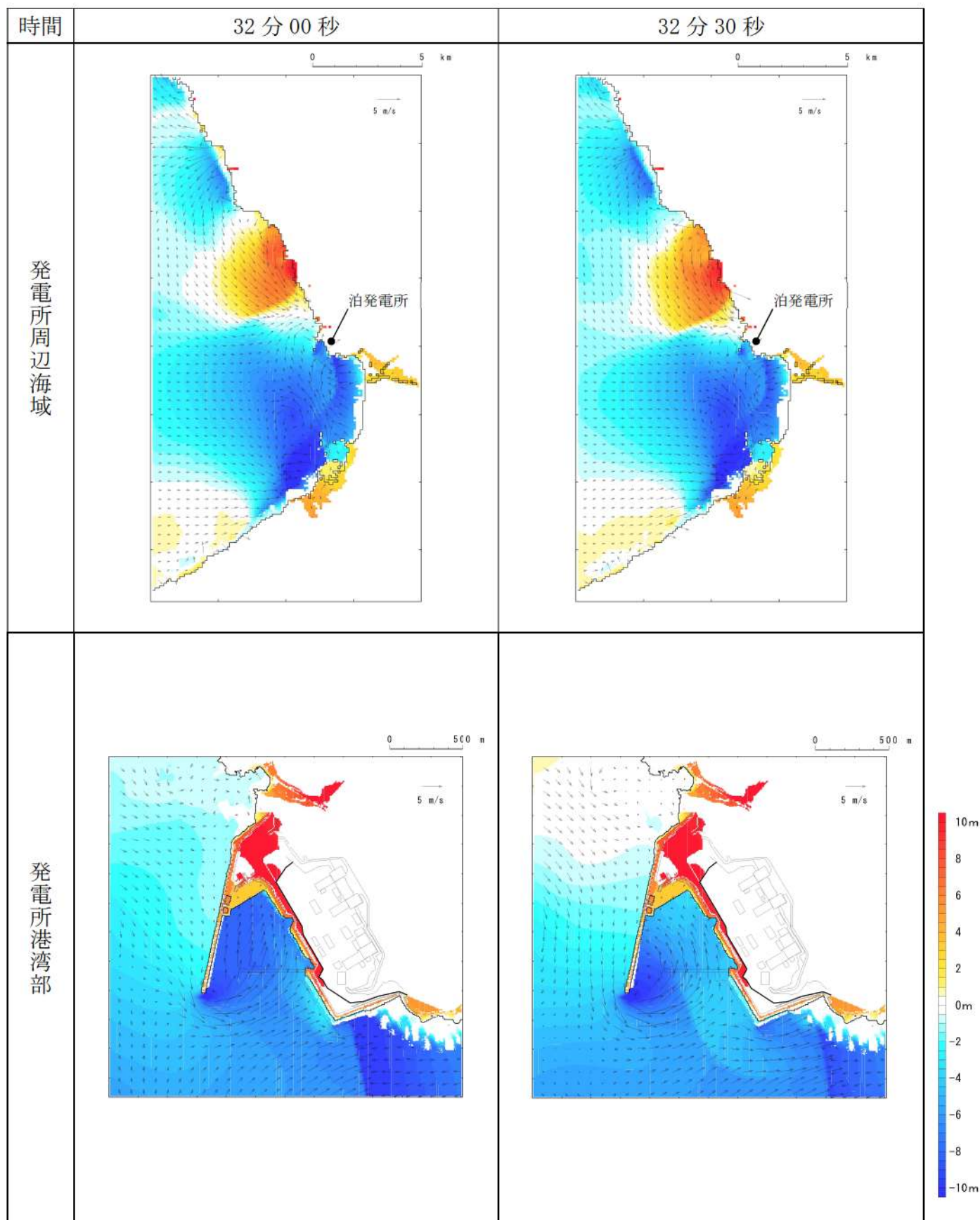
第 17 図-25 基準津波K（南防波堤損傷）の水位変動・流向ベクトル(25/53)
