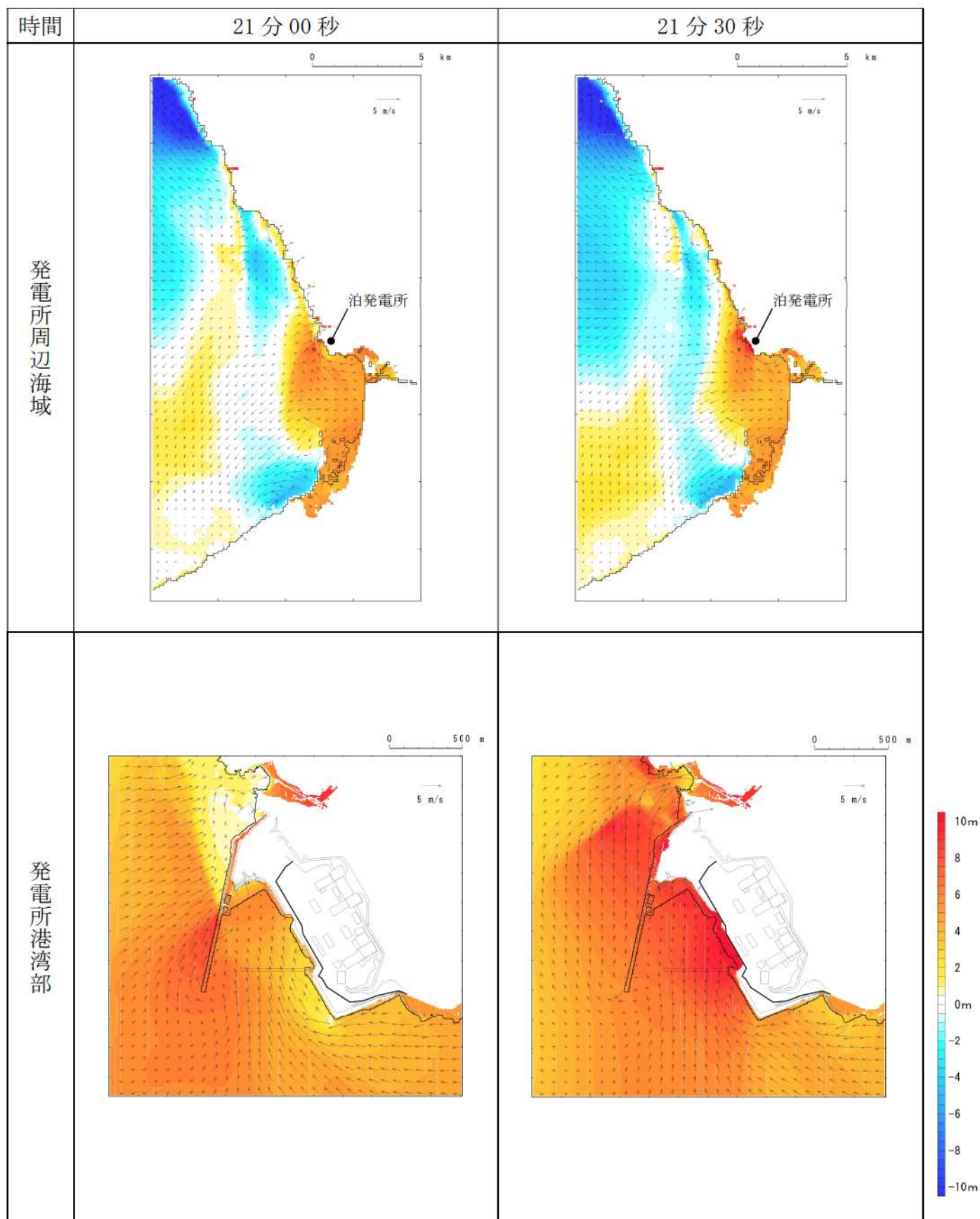
第 17 図-14 基準津波K（南防波堤損傷）の水位変動・流向ベクトル(14/53)
