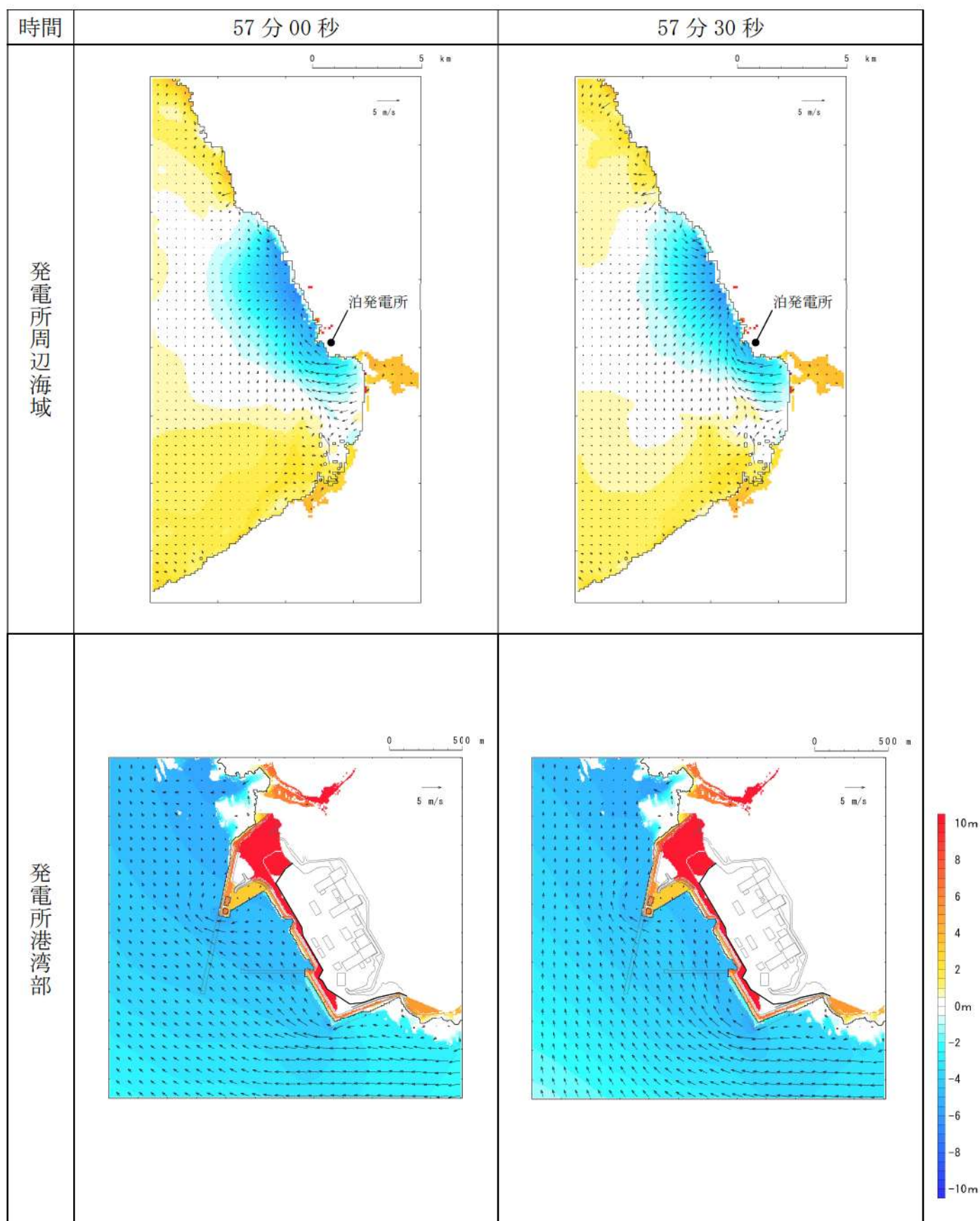
第 16 図-46 基準津波 J（北及び南防波堤損傷）の水位変動・流向ベクトル(46/49)
