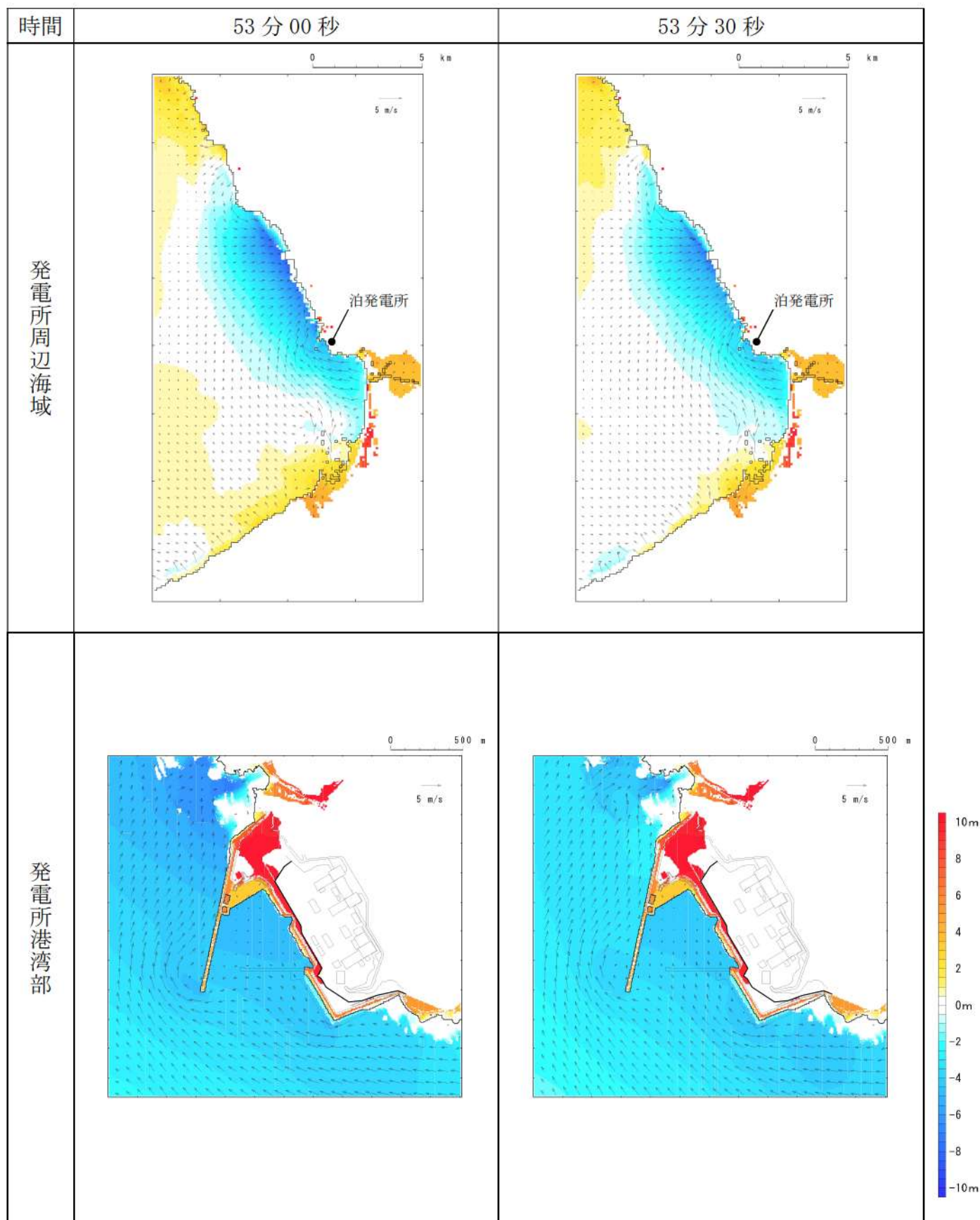
第 7 図-46 基準津波 D（南防波堤損傷）の水位変動・流向ベクトル(46/53)
