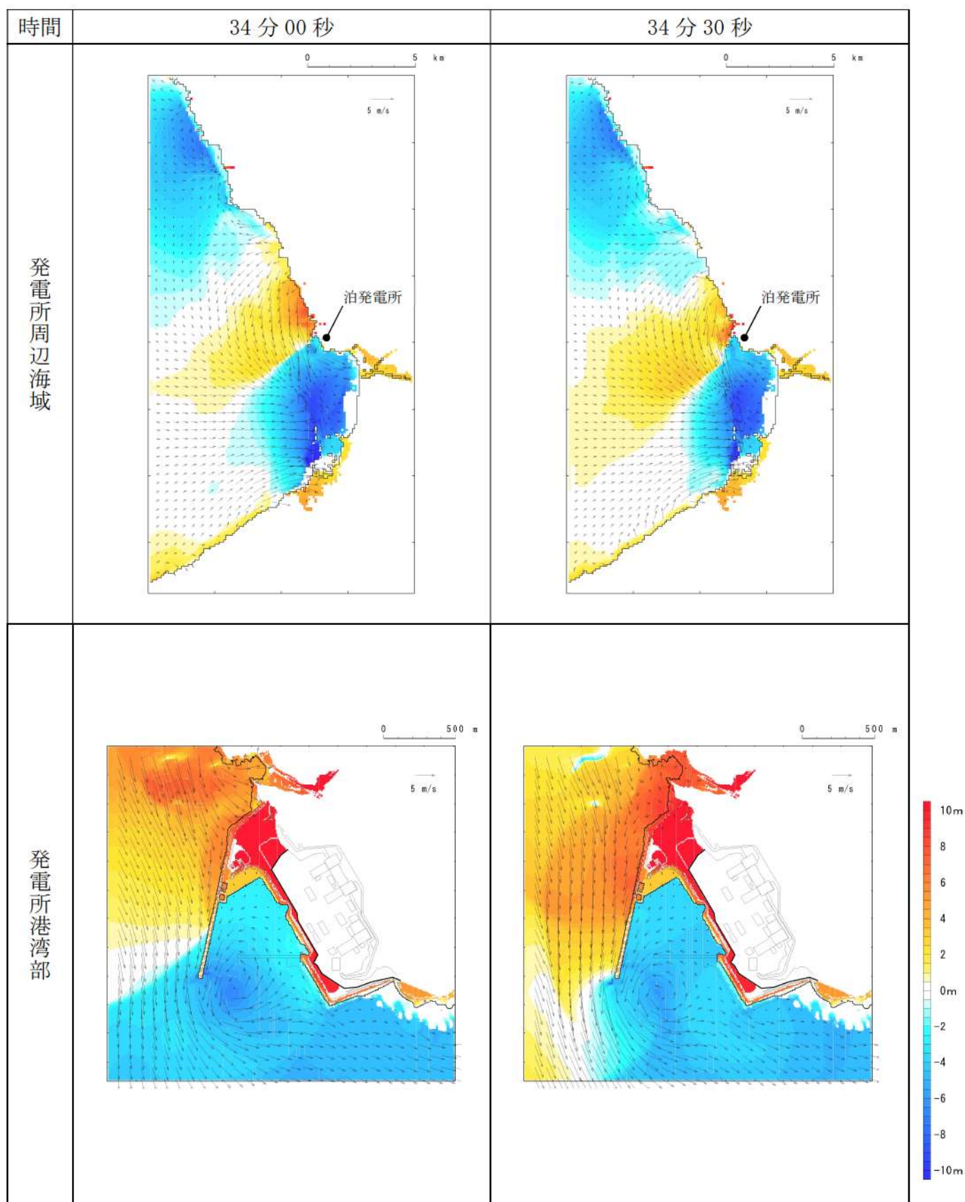
第 10 図-27 基準津波 E（南防波堤損傷）の水位変動・流向ベクトル (27/53)
