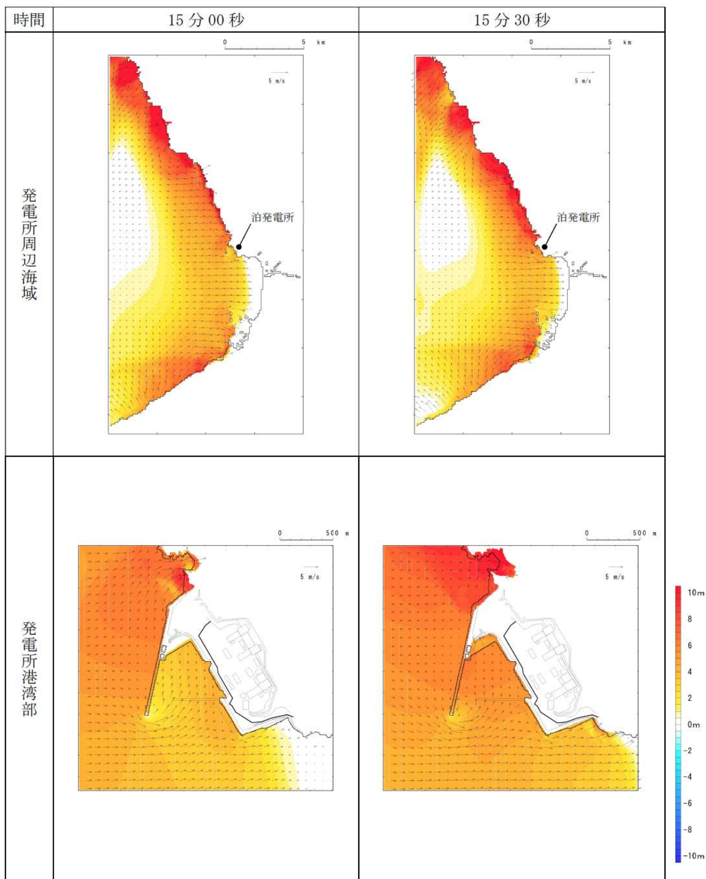
第 10 図-8 基準津波 E（南防波堤損傷）の水位変動・流向ベクトル (8/53)
