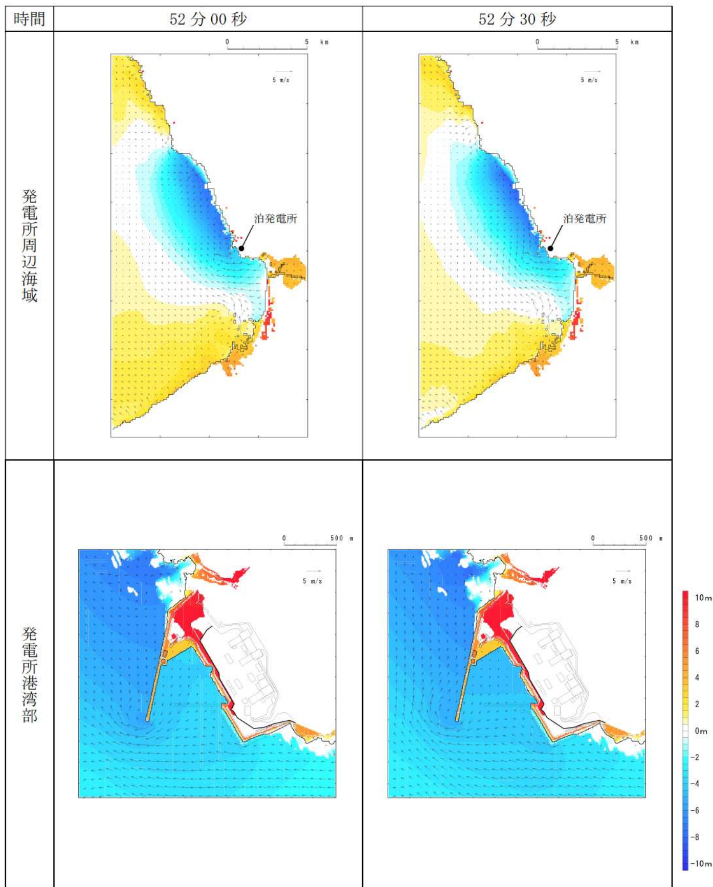
第 7 図-45 基準津波 D（南防波堤損傷）の水位変動・流向ベクトル (45/53)
