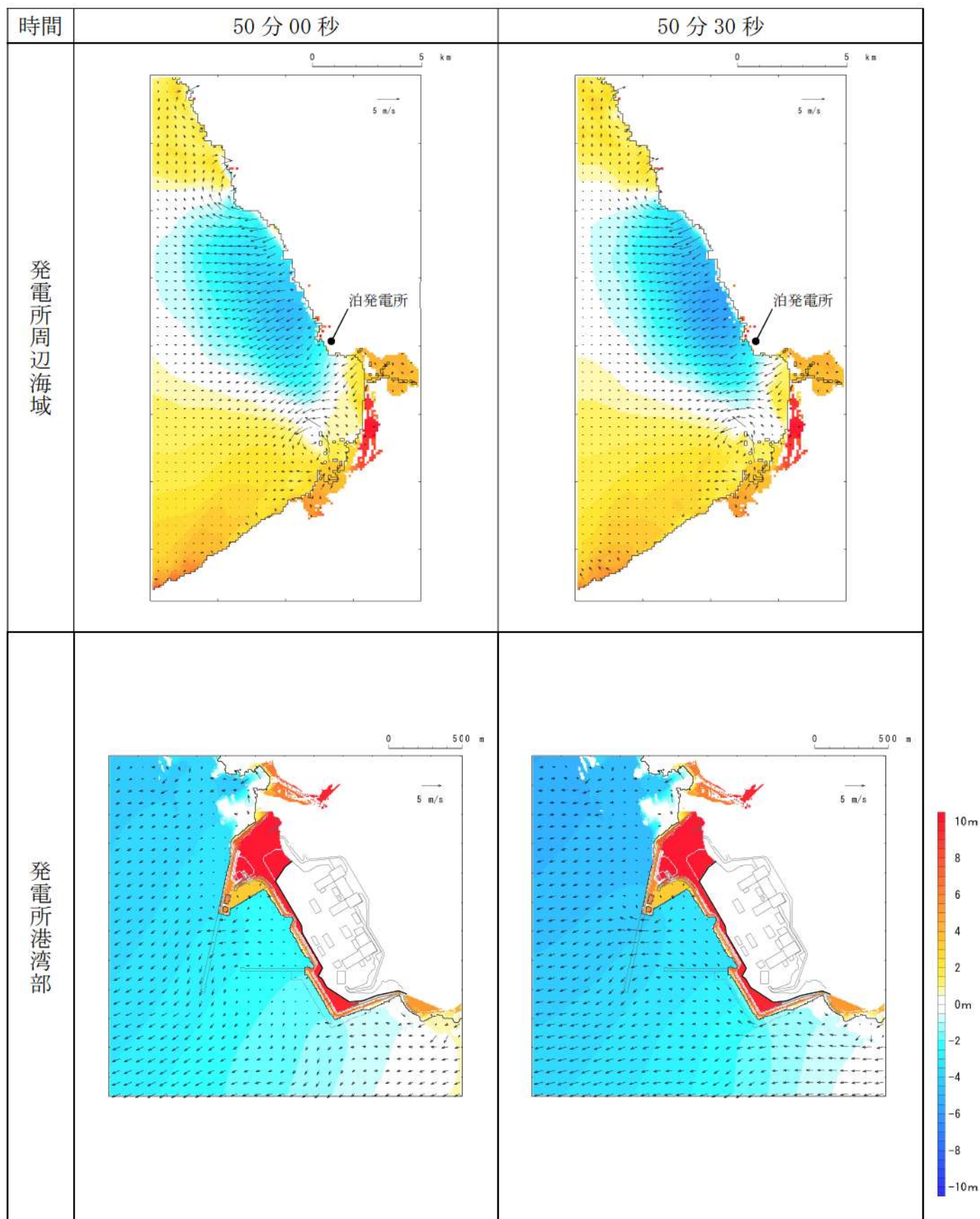
第9図-43 基準津波E（北及び南防波堤損傷）の水位変動・流向ベクトル(43/53)
