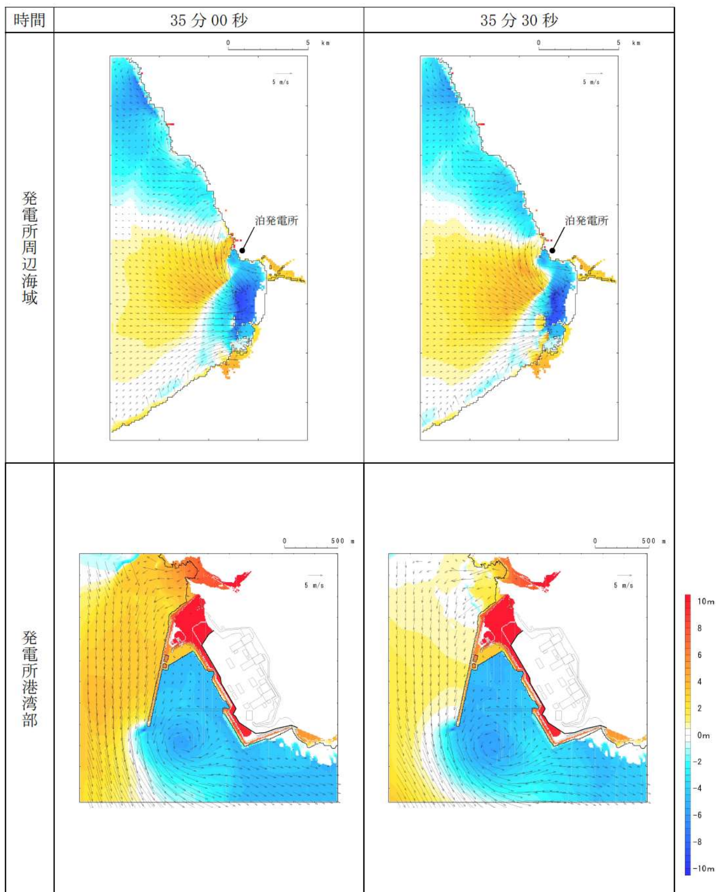
第 10 図-28 基準津波 E（南防波堤損傷）の水位変動・流向ベクトル (28/53)
