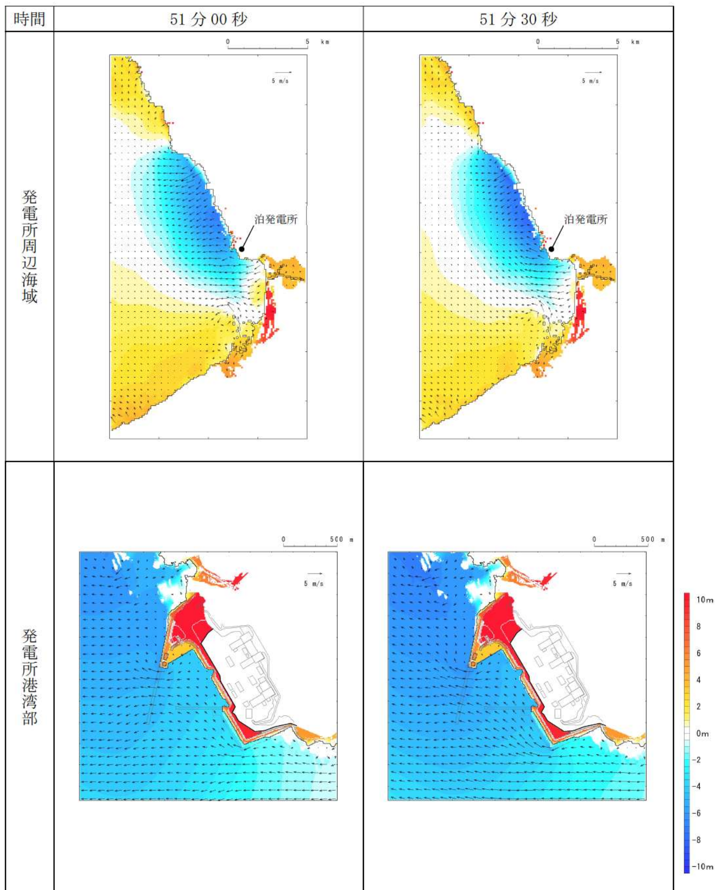
第 9 図-44 基準津波 E（北及び南防波堤損傷）の水位変動・流向ベクトル(44/53)
