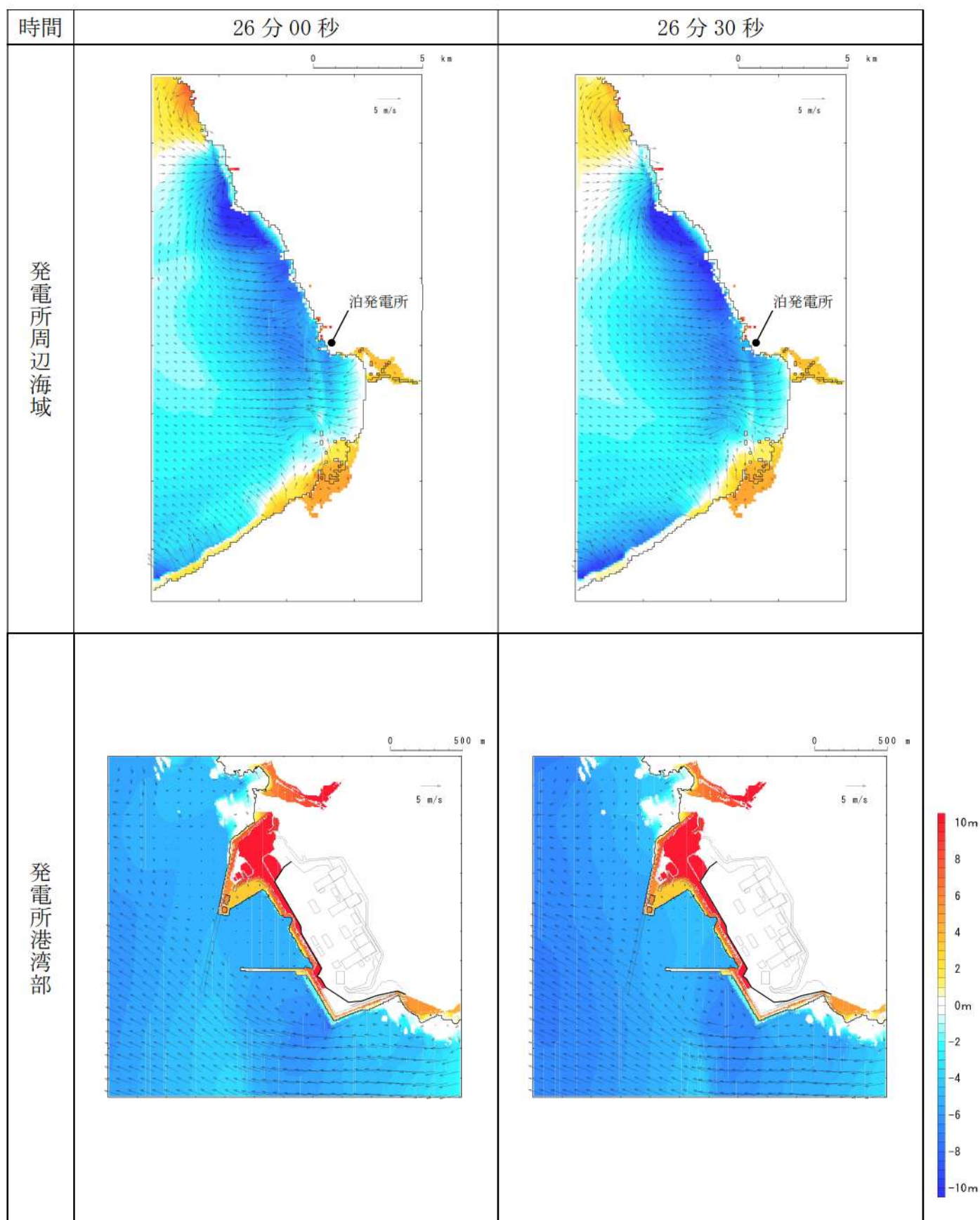
第8図-19 基準津波D（北防波堤損傷）の水位変動・流向ベクトル(19/53)
