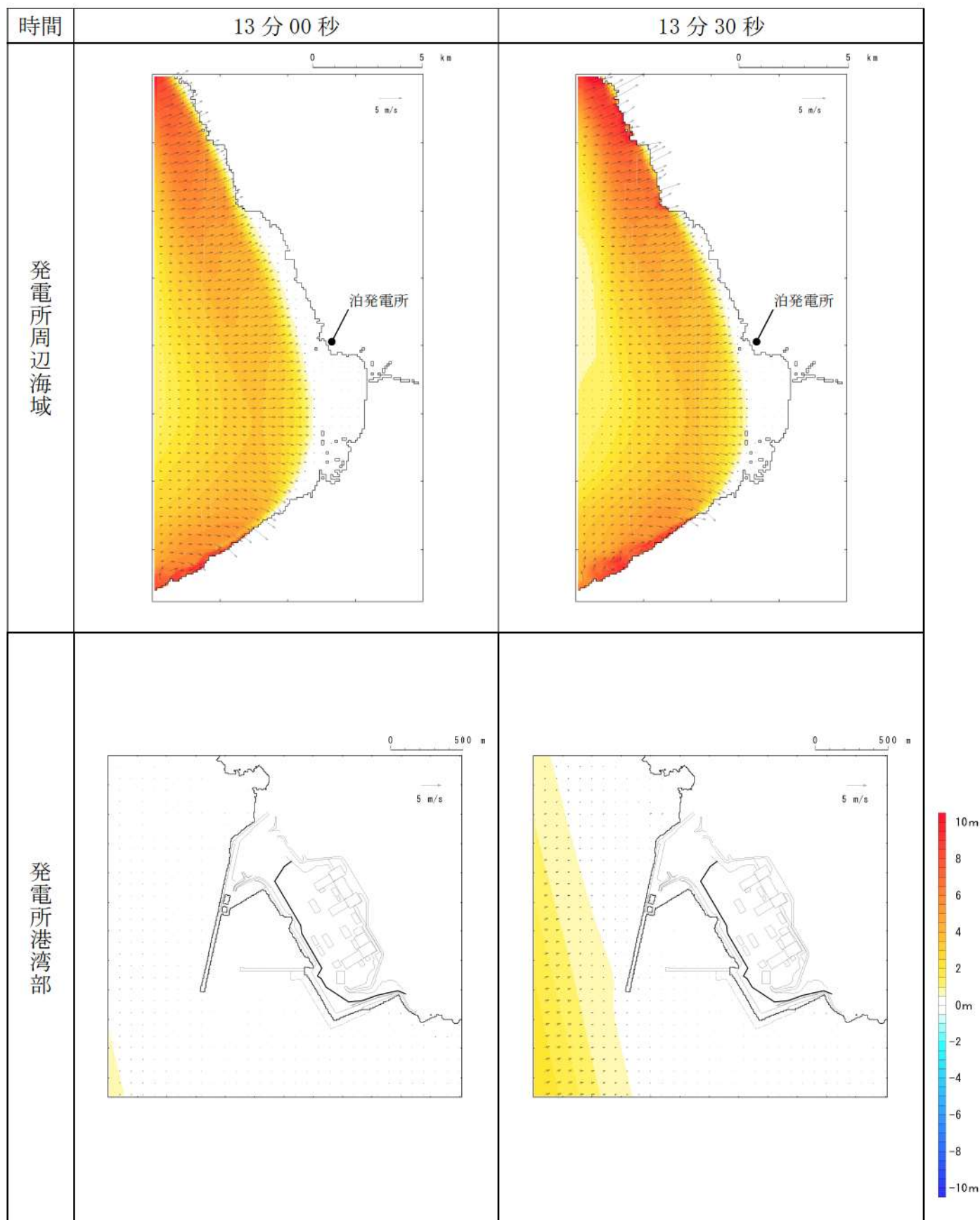
第 7 図-6 基準津波 D（南防波堤損傷）の水位変動・流向ベクトル (6/53)
