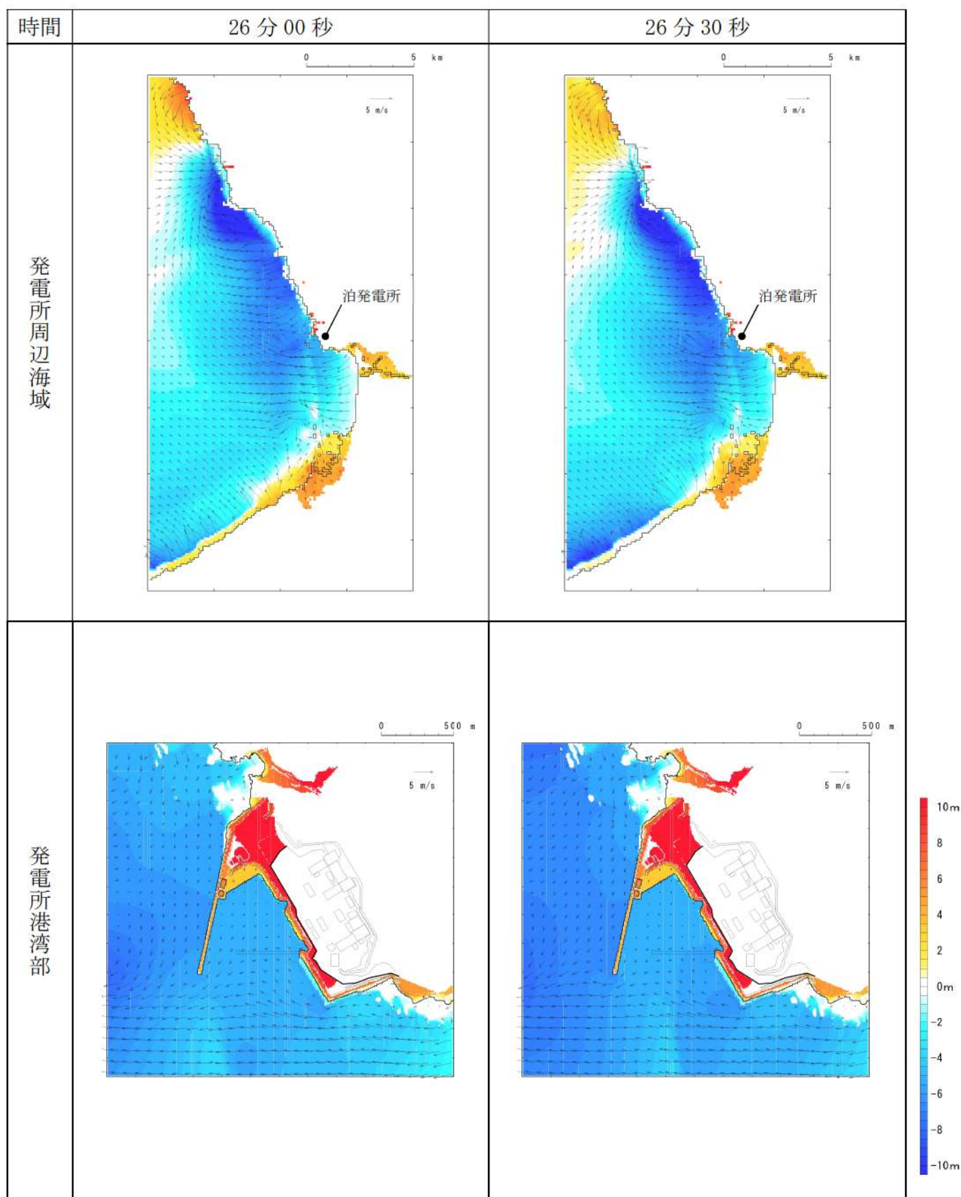
第 10 図-19 基準津波 E（南防波堤損傷）の水位変動・流向ベクトル(19/53)
