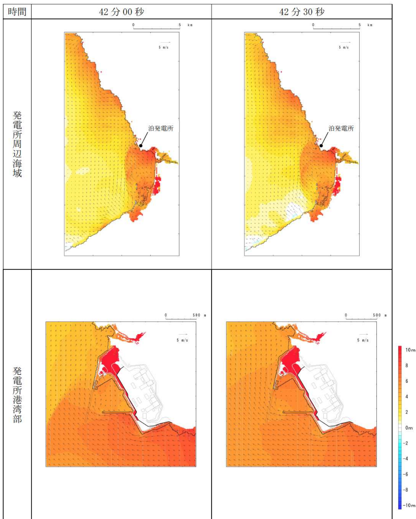
第 8 図-35 基準津波 D（北防波堤損傷）の水位変動・流向ベクトル(35/53)
