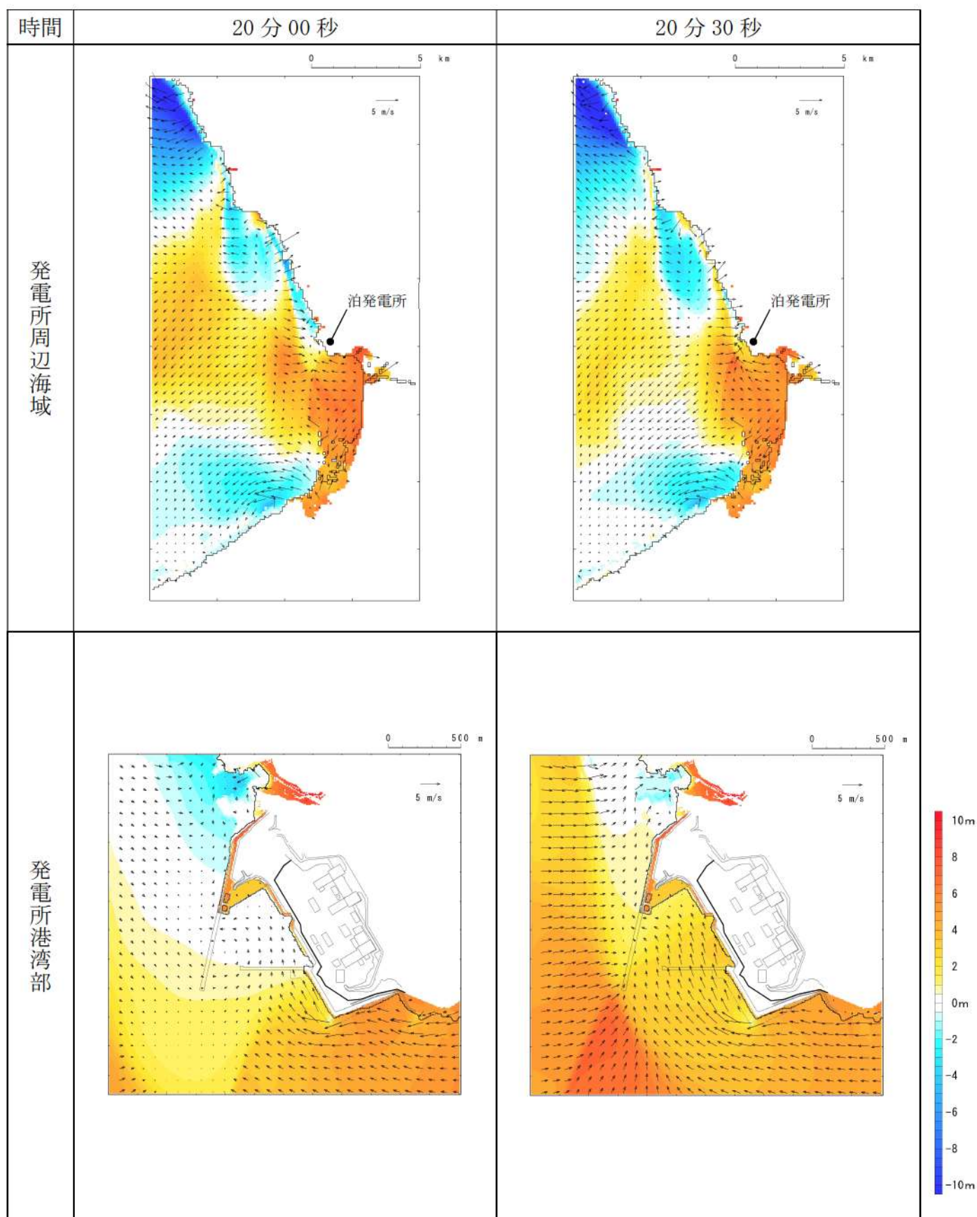
第 9 図-13 基準津波 E（北及び南防波堤損傷）の水位変動・流向ベクトル(13/53)
