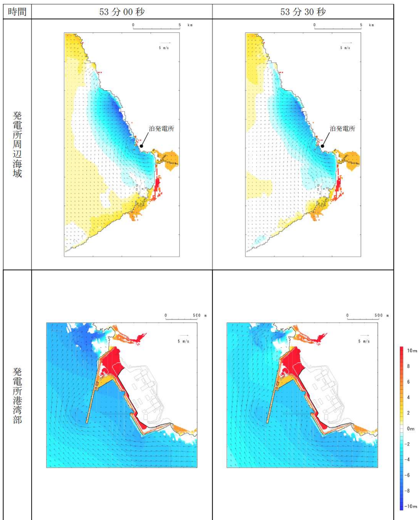
第 10 図-46 基準津波 E（南防波堤損傷）の水位変動・流向ベクトル(46/53)
