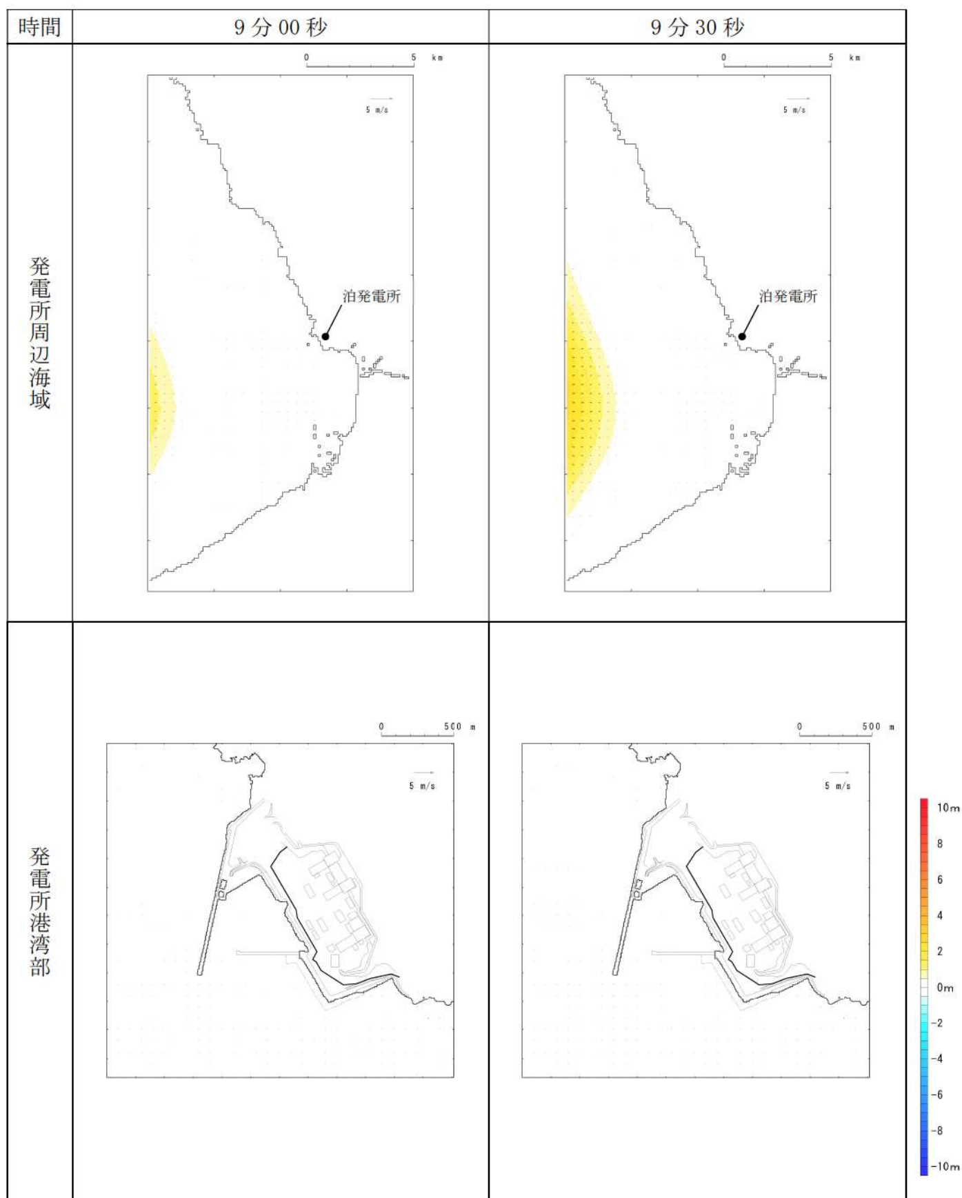
第 10 図-2 基準津波 E（南防波堤損傷）の水位変動・流向ベクトル (2/53)
