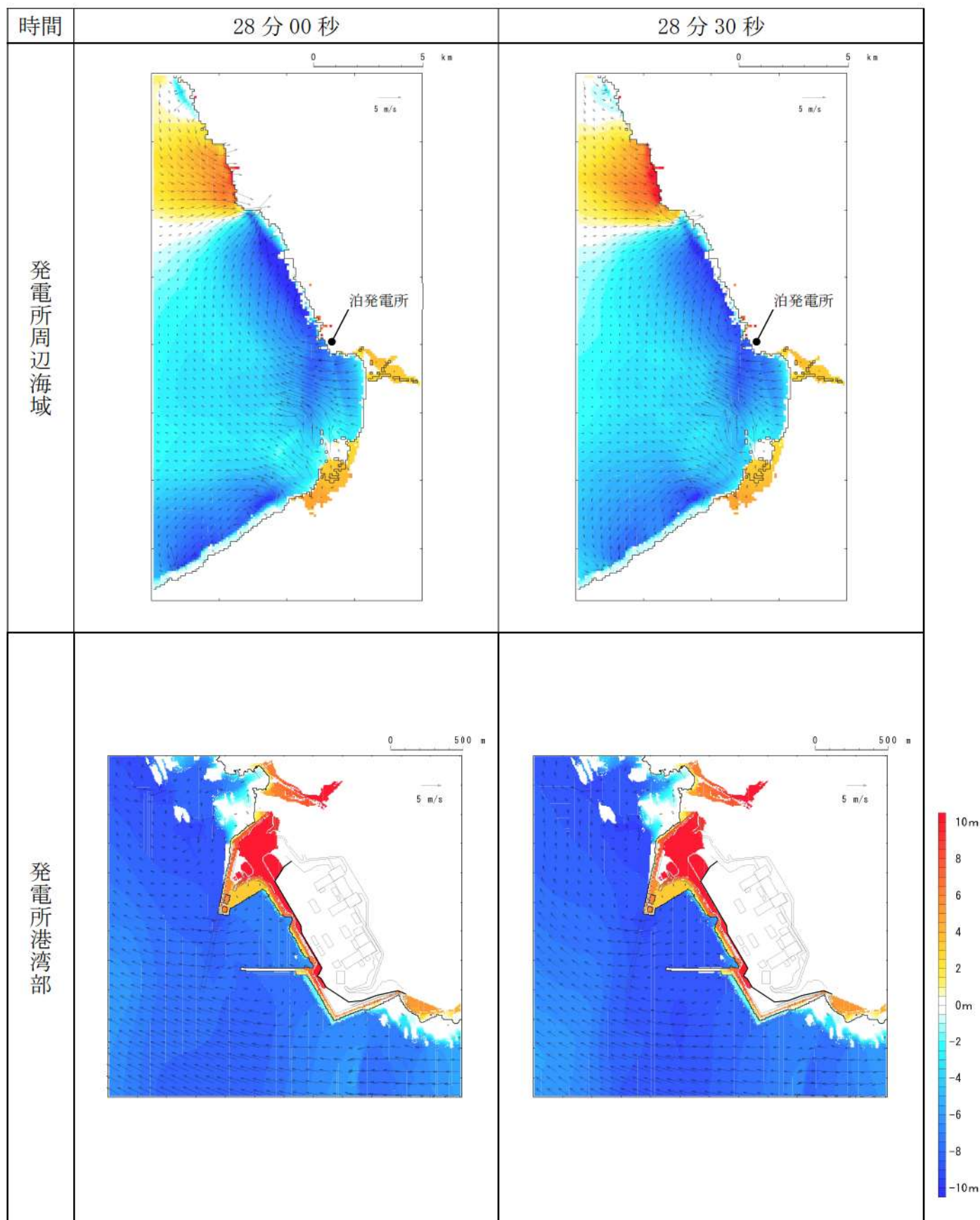
第8図-21 基準津波D（北防波堤損傷）の水位変動・流向ベクトル(21/53)
