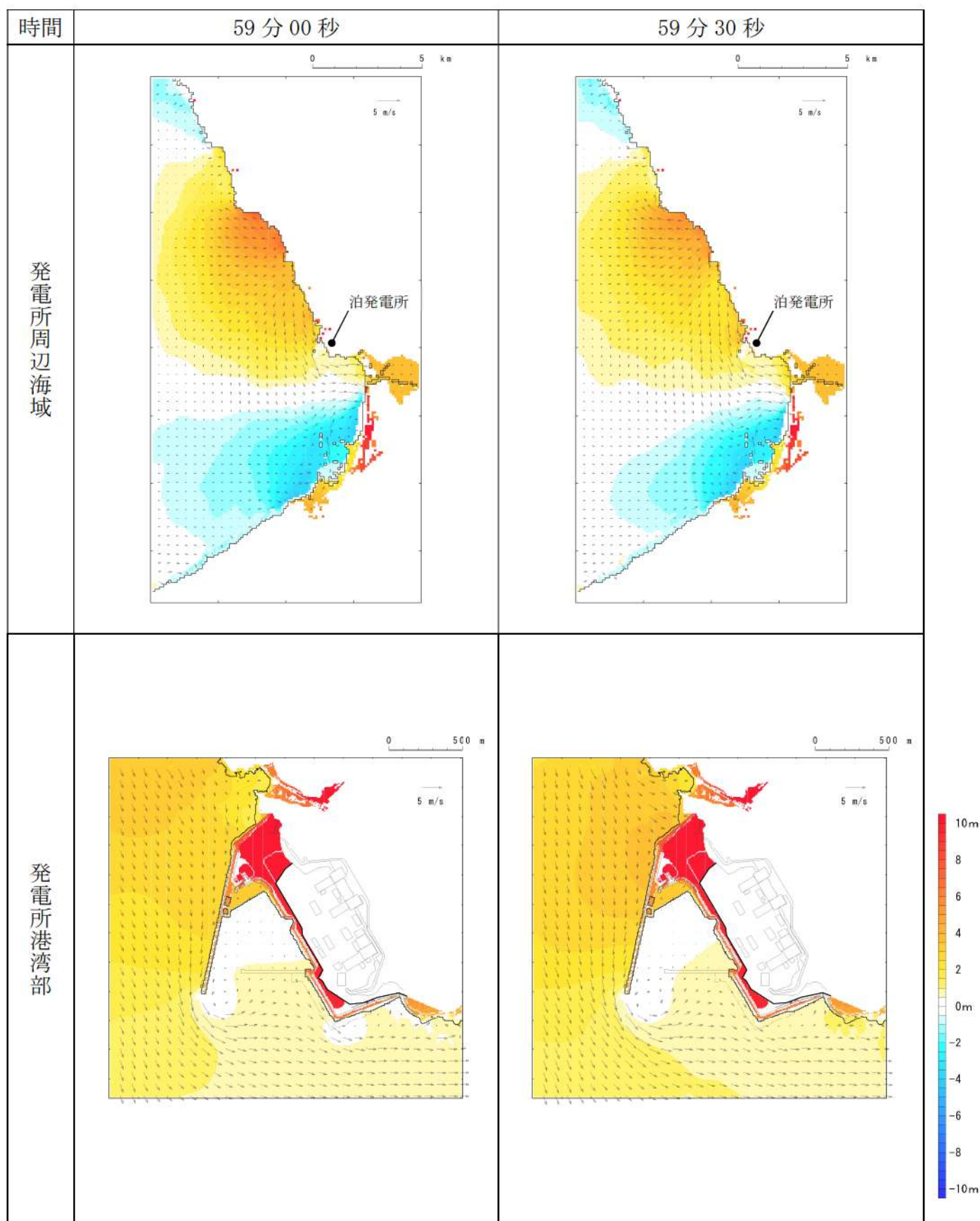
第 10 図-52 基準津波 E（南防波堤損傷）の水位変動・流向ベクトル(52/53)
