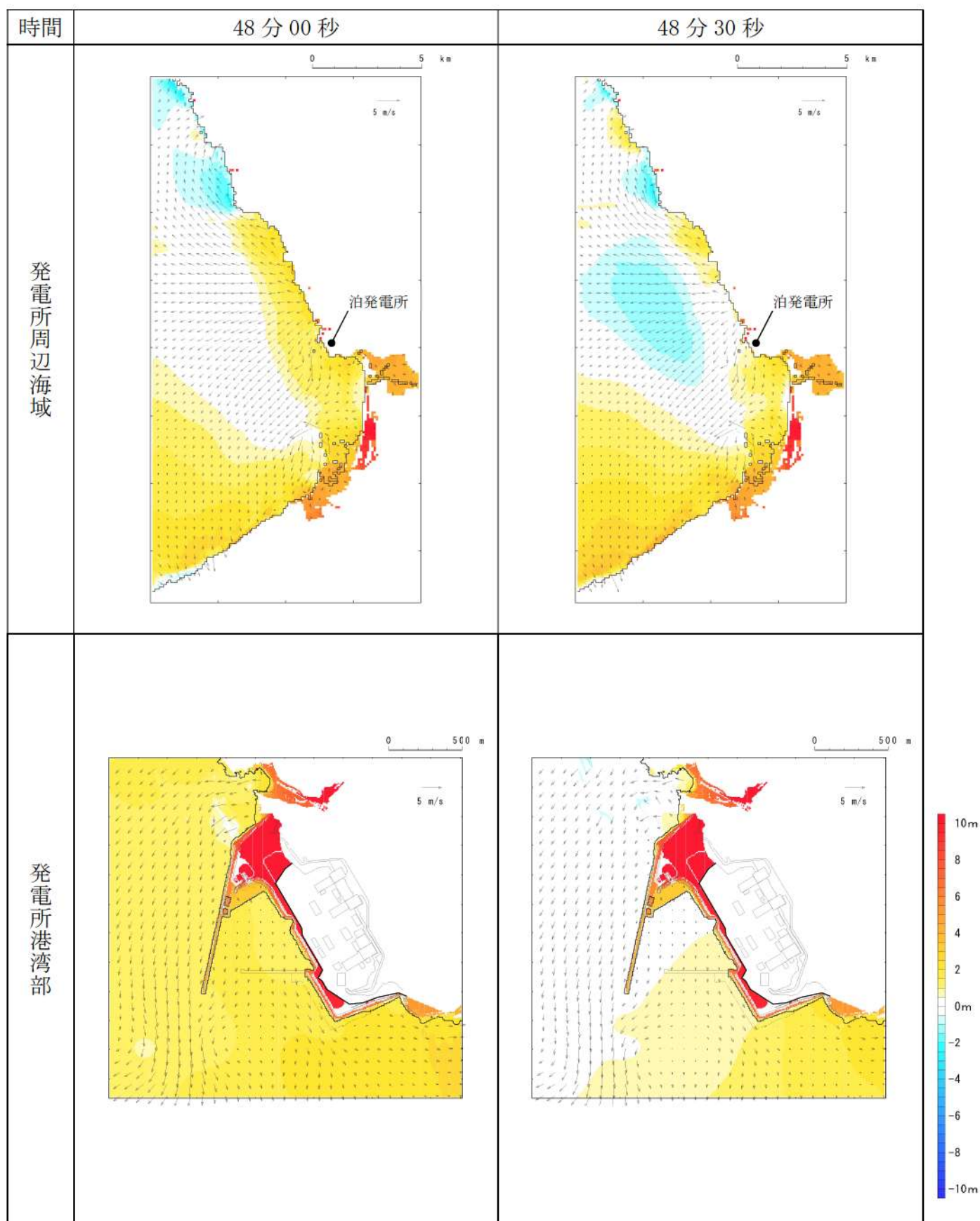
第 10 図-41 基準津波 E（南防波堤損傷）の水位変動・流向ベクトル (41/53)
