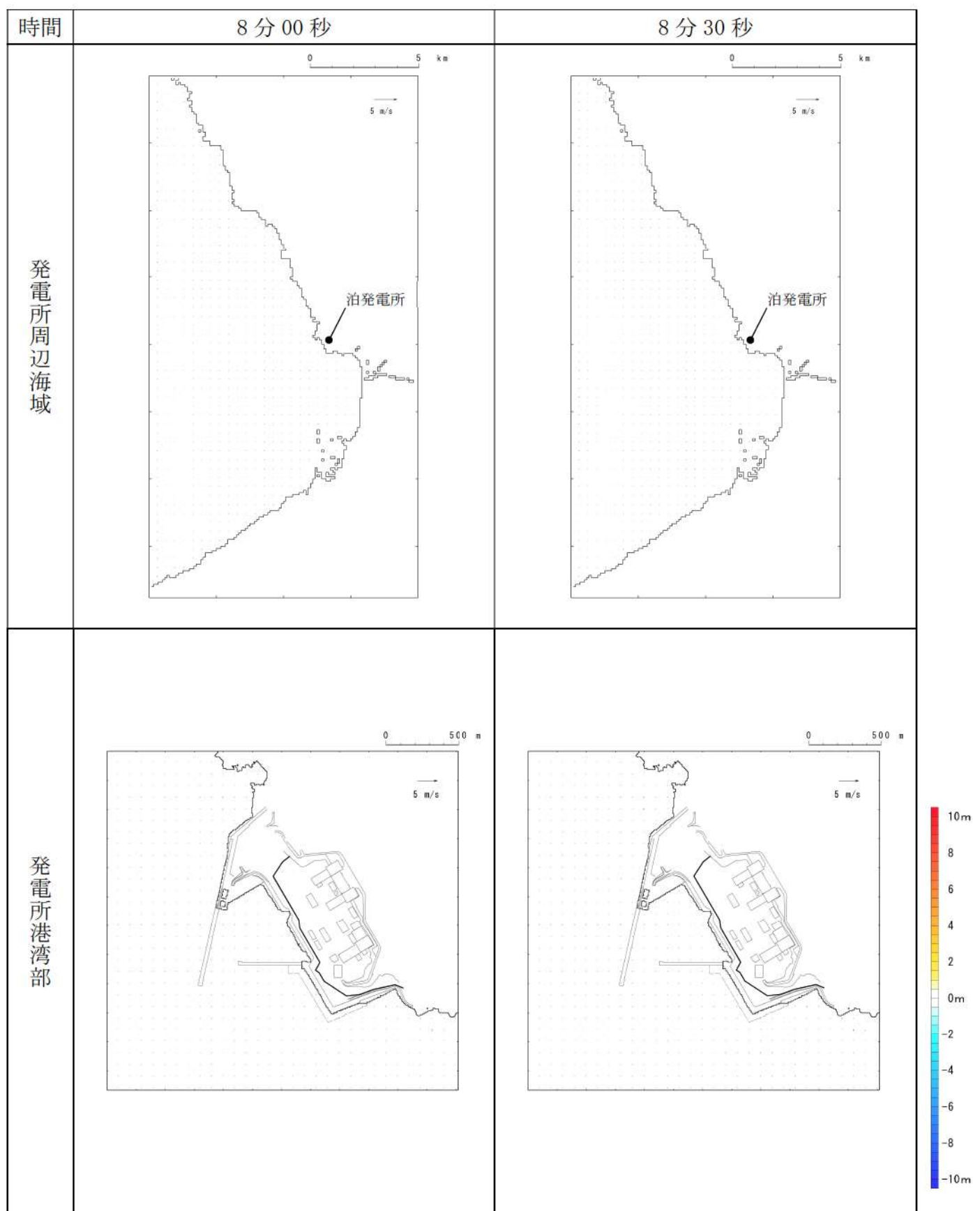
第9図-1 基準津波E（北及び南防波堤損傷）の水位変動・流向ベクトル(1/53)
