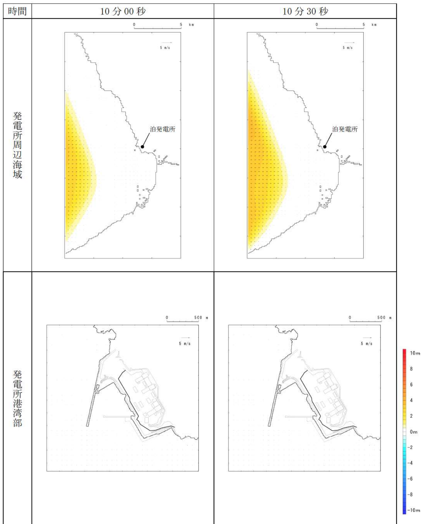
第 10 図-3 基準津波 E（南防波堤損傷）の水位変動・流向ベクトル (3/53)
