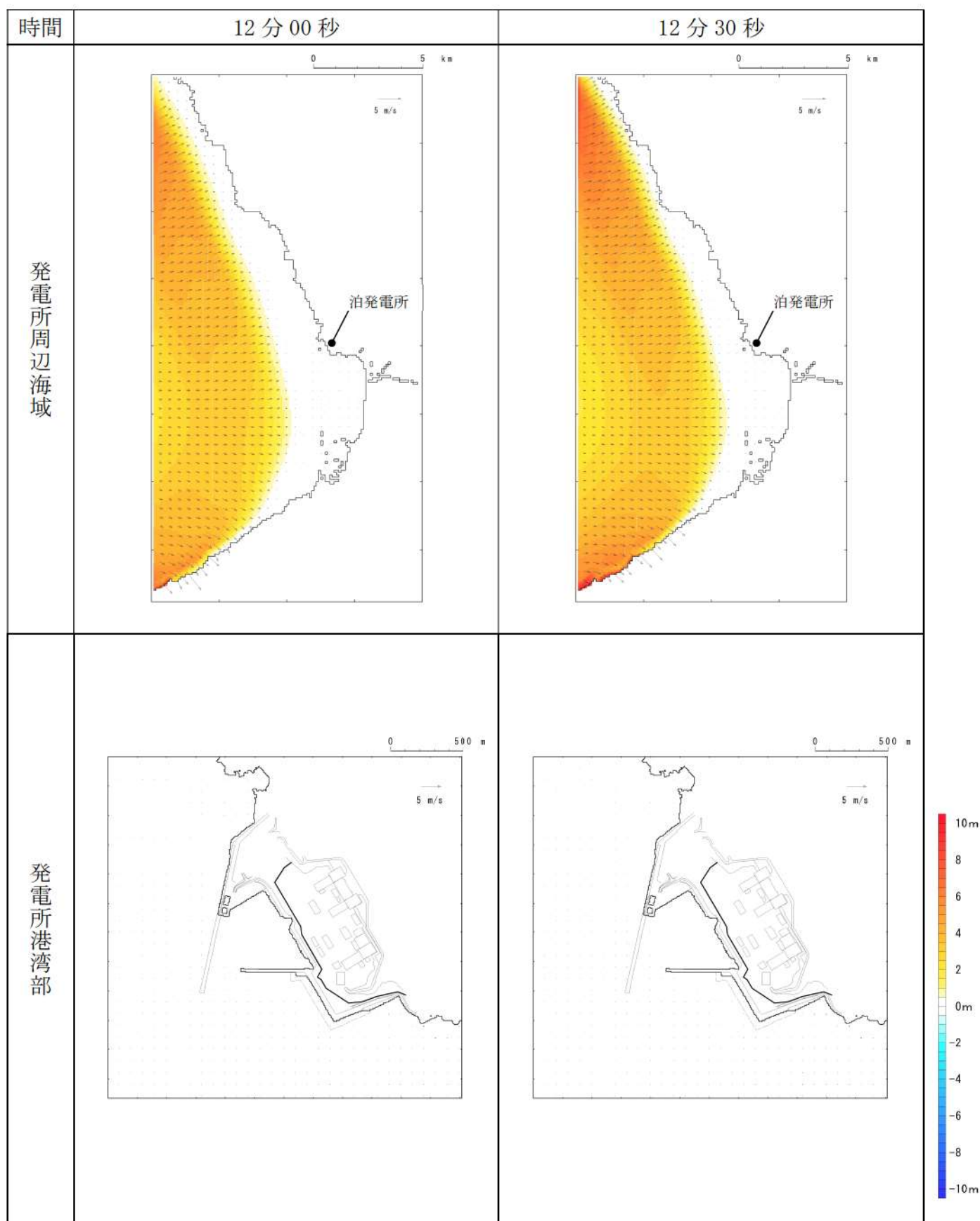
第8図-5 基準津波D（北防波堤損傷）の水位変動・流向ベクトル(5/53)
