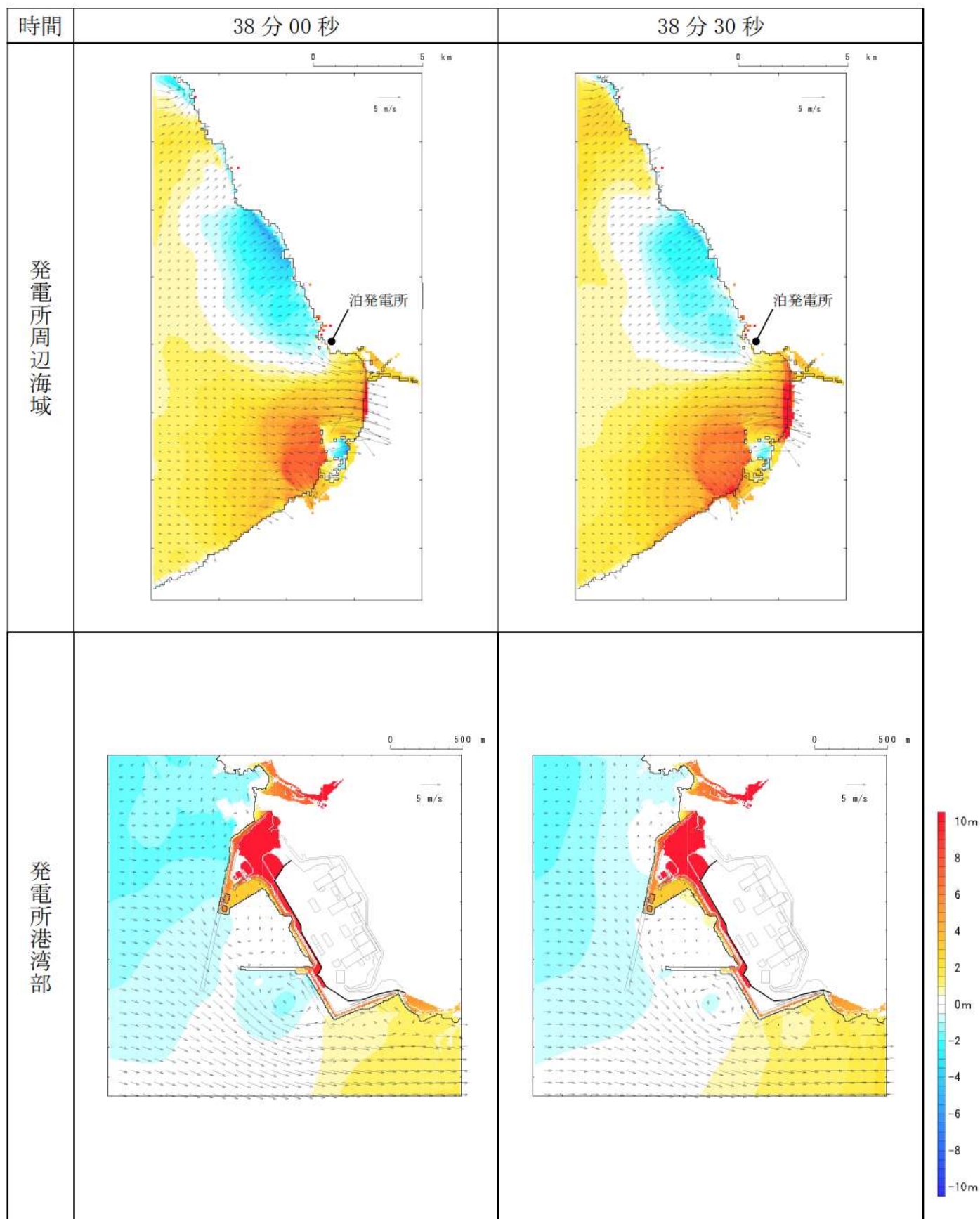
第 8 図-31 基準津波 D（北防波堤損傷）の水位変動・流向ベクトル(31/53)
