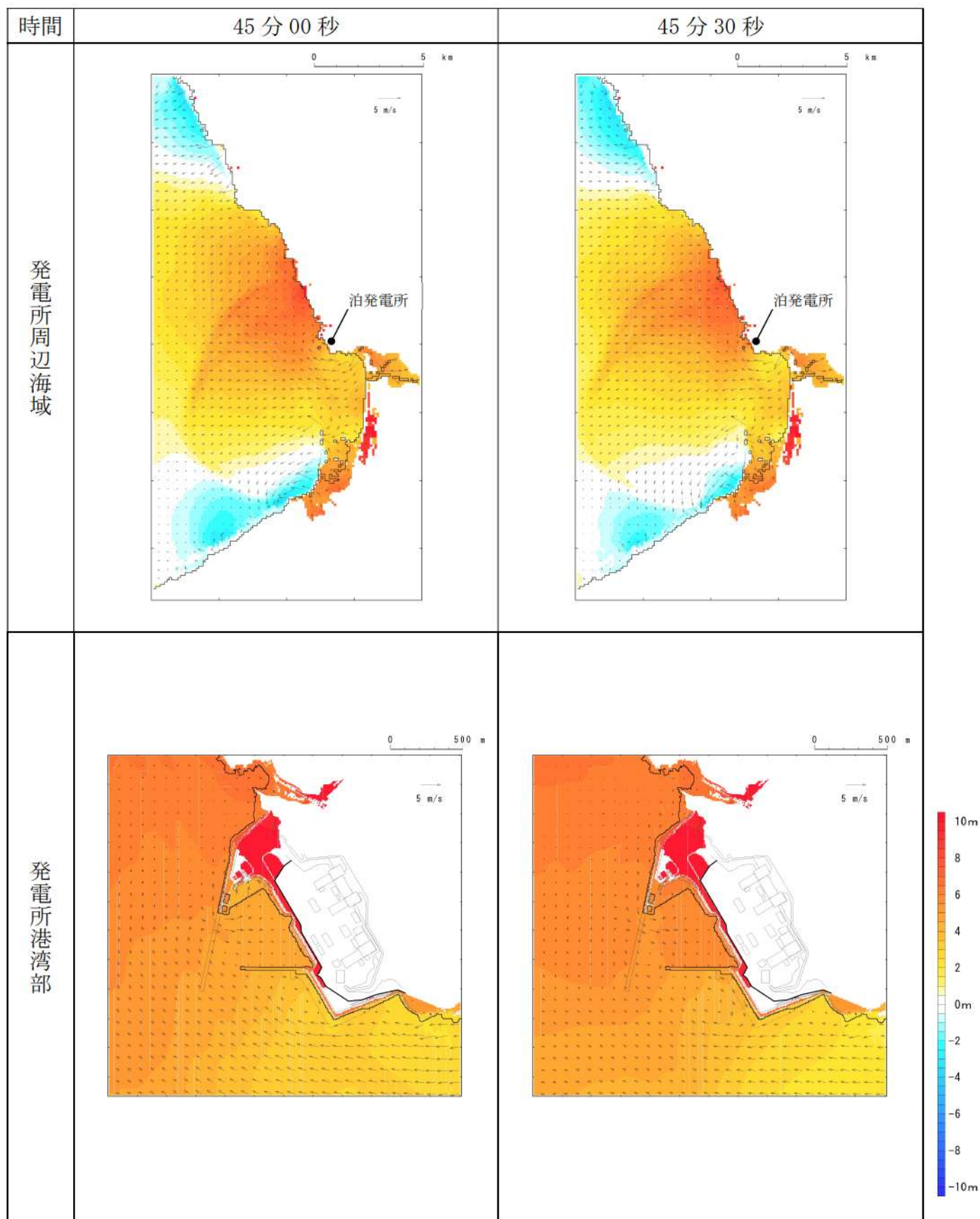
第 8 図-38 基準津波 D（北防波堤損傷）の水位変動・流向ベクトル (38/53)
