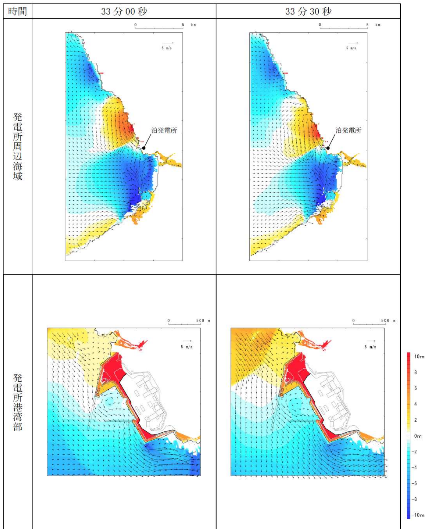
第 9 図-26 基準津波 E（北及び南防波堤損傷）の水位変動・流向ベクトル(26/53)
