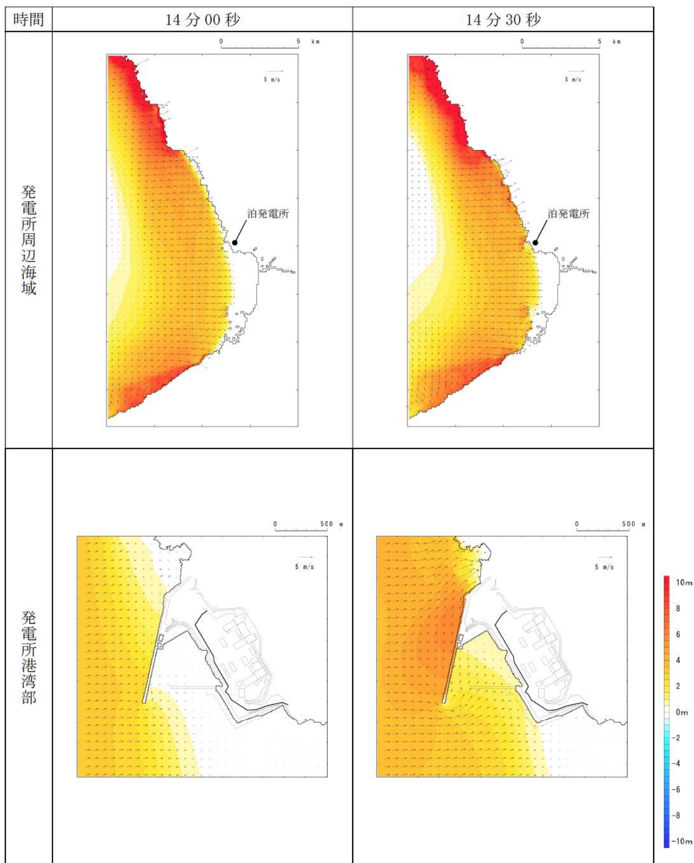
第 10 図-7 基準津波 E（南防波堤損傷）の水位変動・流向ベクトル (7/53)
