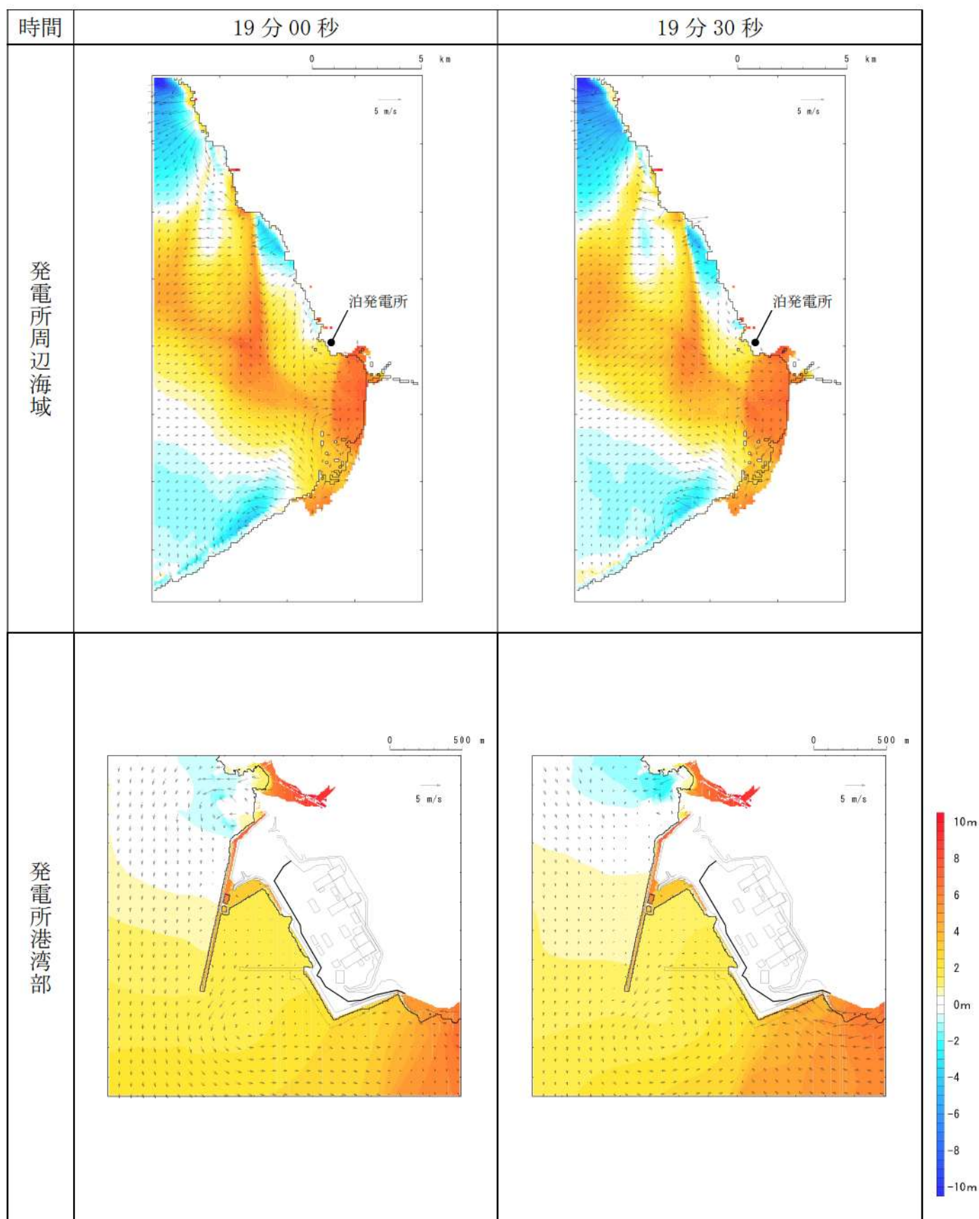
第 7 図-12 基準津波 D（南防波堤損傷）の水位変動・流向ベクトル(12/53)
