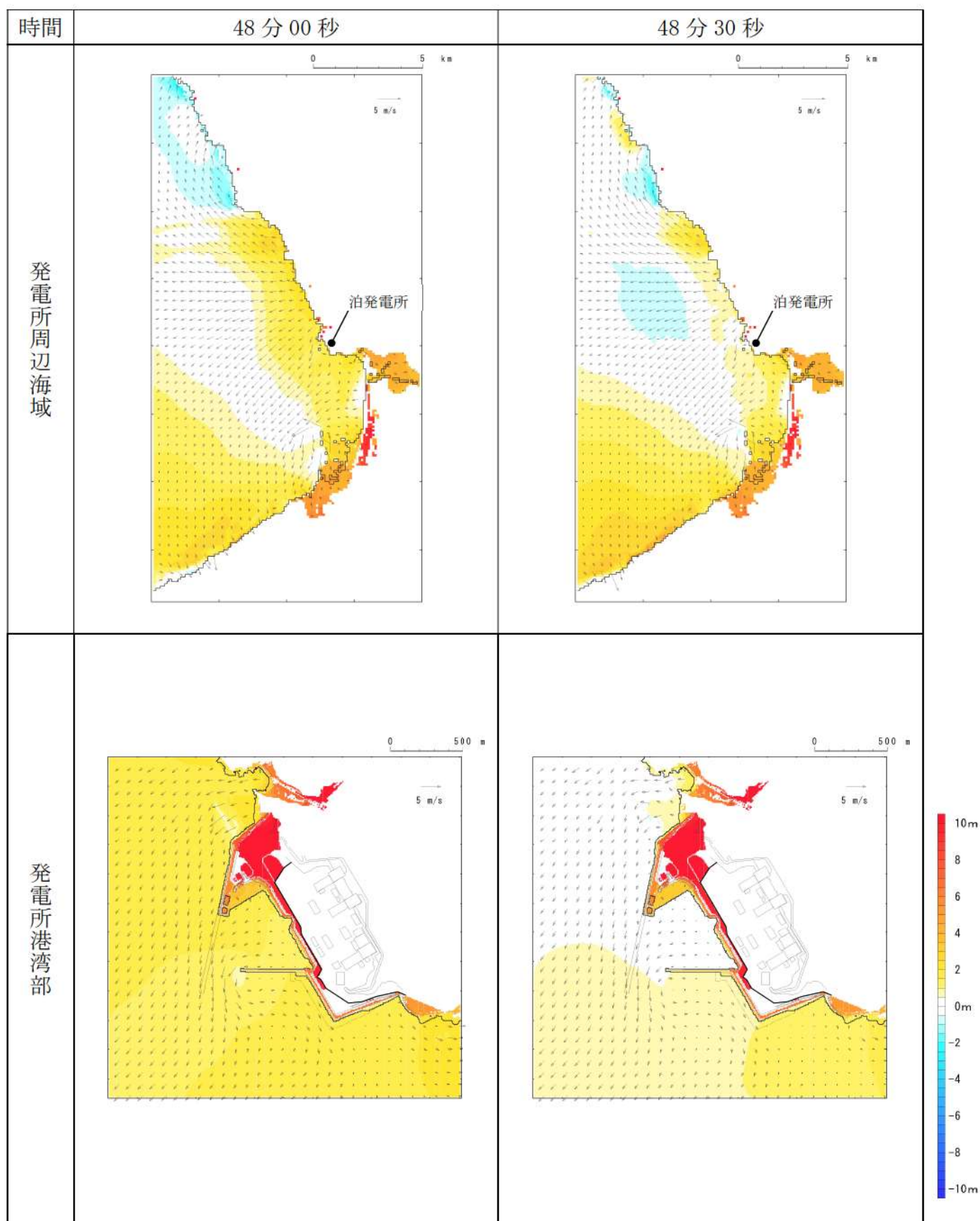
第 8 図-41 基準津波 D（北防波堤損傷）の水位変動・流向ベクトル(41/53)
