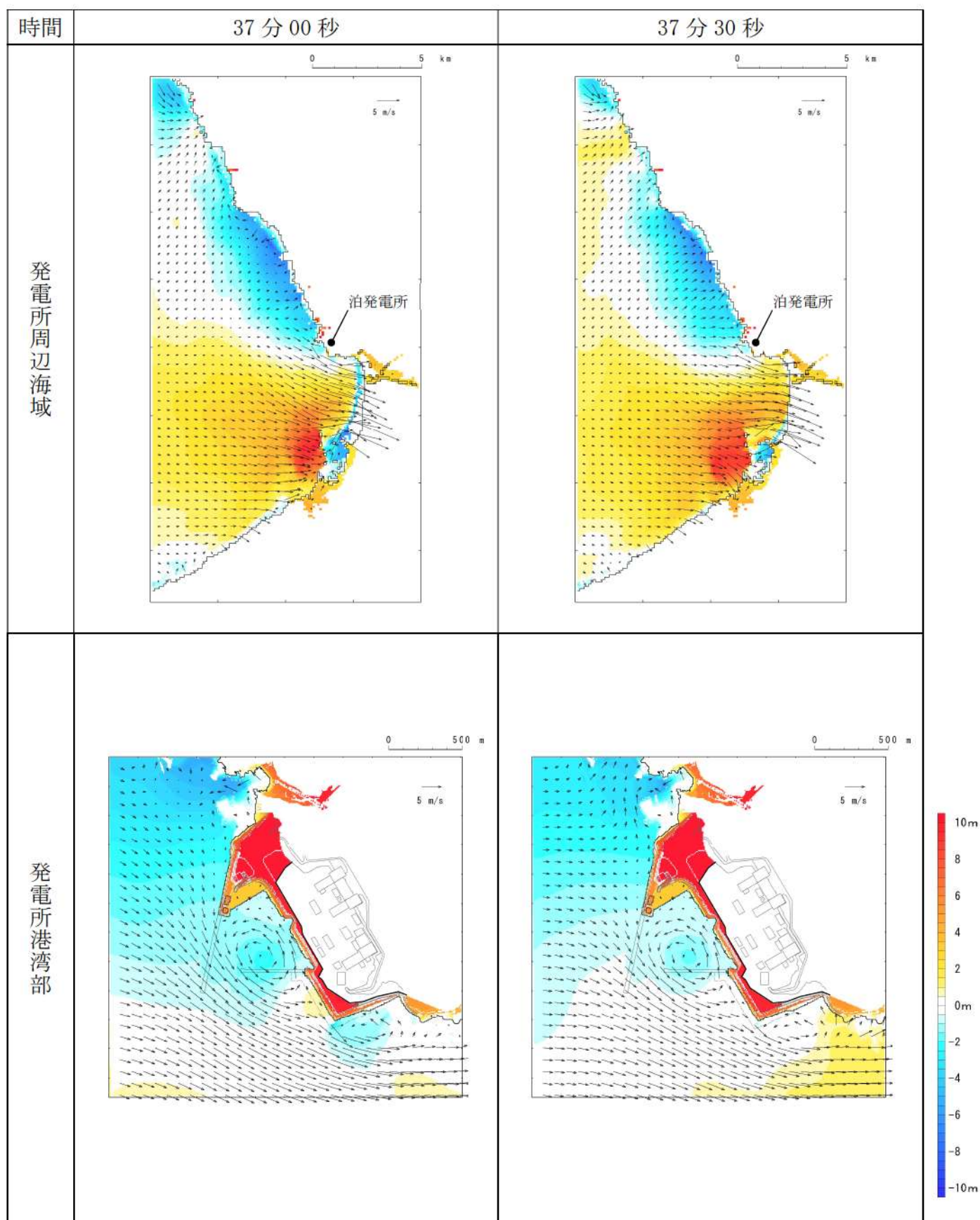
第 9 図-30 基準津波 E（北及び南防波堤損傷）の水位変動・流向ベクトル(30/53)
