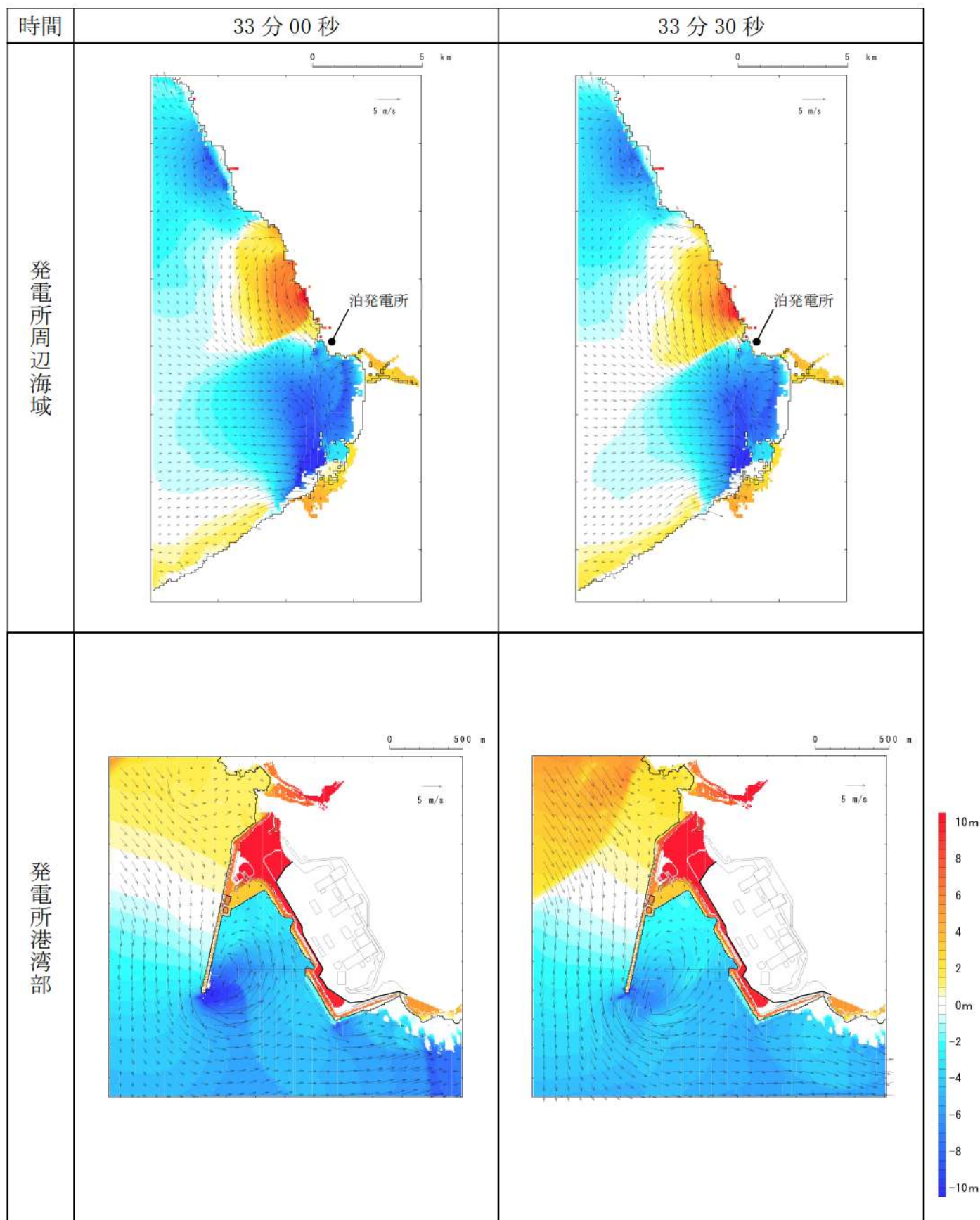
第 10 図-26 基準津波 E（南防波堤損傷）の水位変動・流向ベクトル (26/53)
