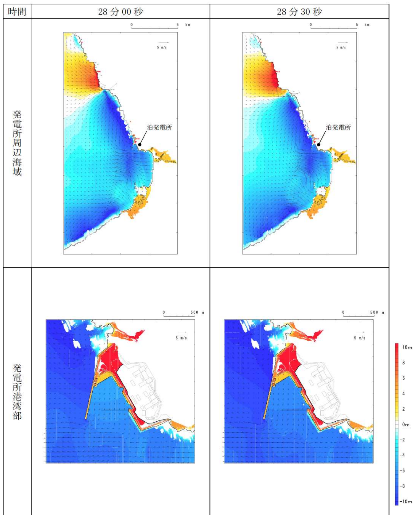
第 10 図-21 基準津波 E（南防波堤損傷）の水位変動・流向ベクトル (21/53)
