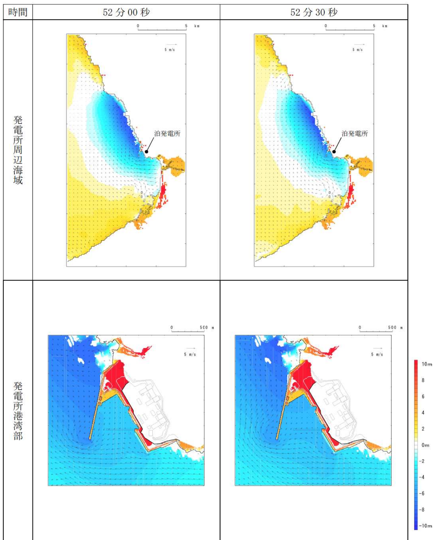
第 10 図-45 基準津波 E（南防波堤損傷）の水位変動・流向ベクトル(45/53)
