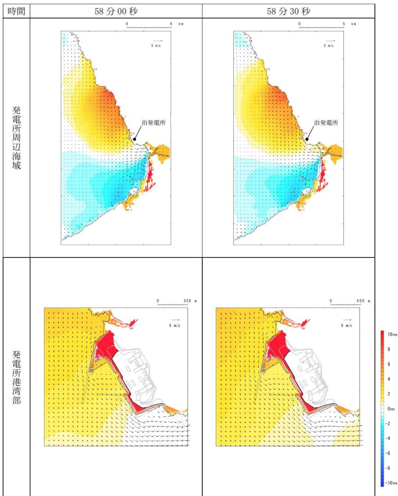
第9図-51 基準津波E（北及び南防波堤損傷）の水位変動・流向ベクトル(51/53)
