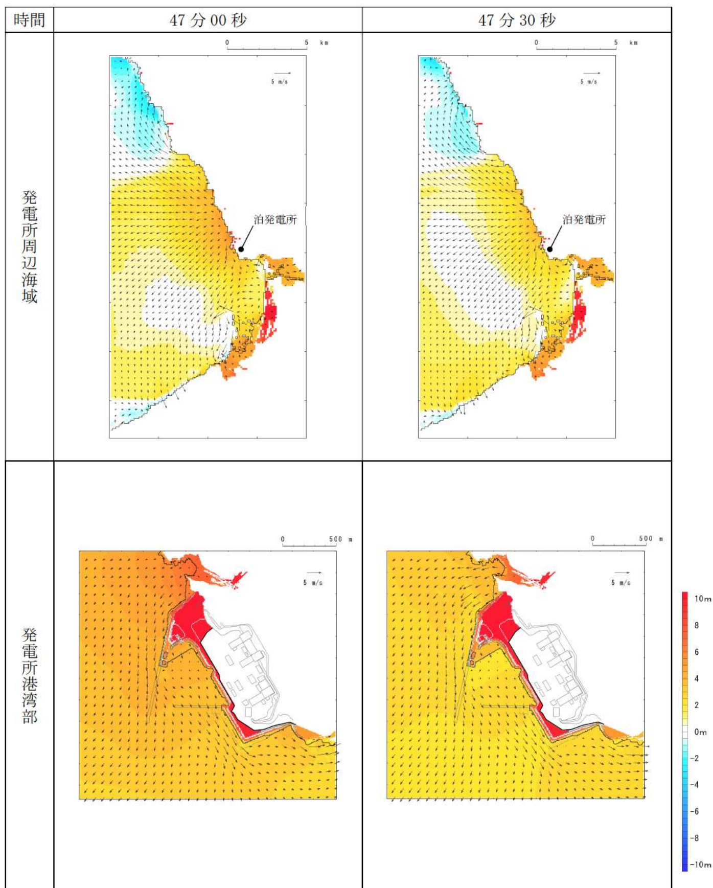
第 9 図-40 基準津波 E（北及び南防波堤損傷）の水位変動・流向ベクトル(40/53)
