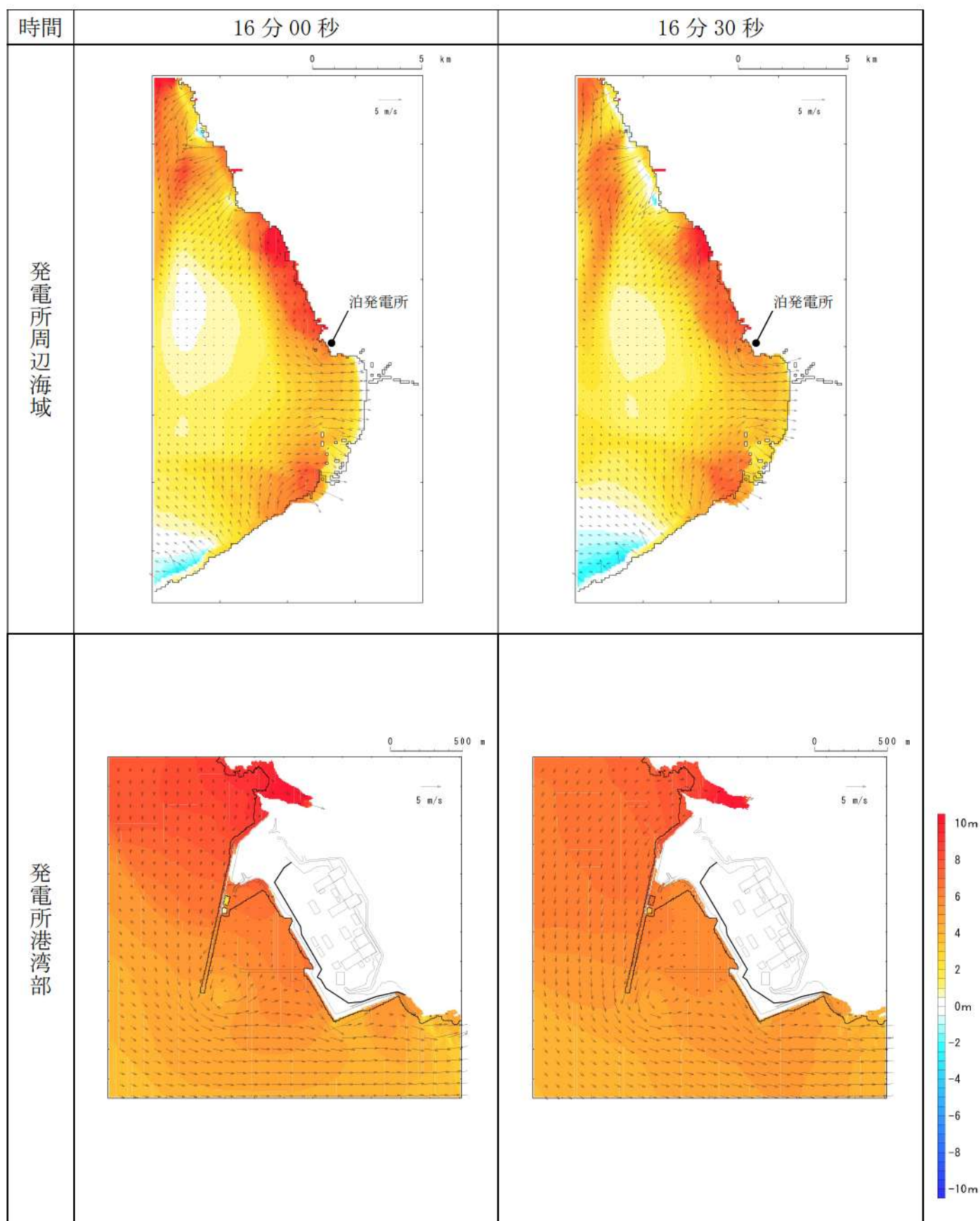
第 7 図-9 基準津波 D（南防波堤損傷）の水位変動・流向ベクトル (9/53)
