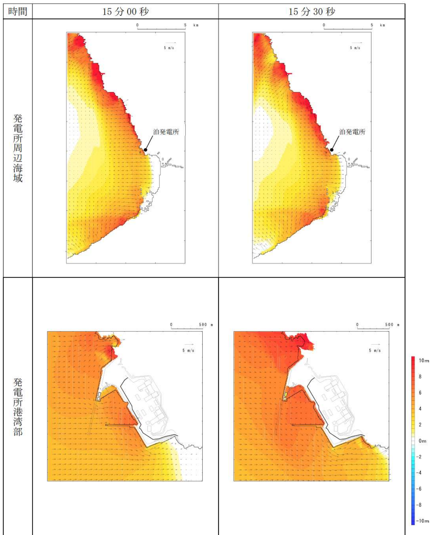
第8図-8 基準津波D（北防波堤損傷）の水位変動・流向ベクトル(8/53)
