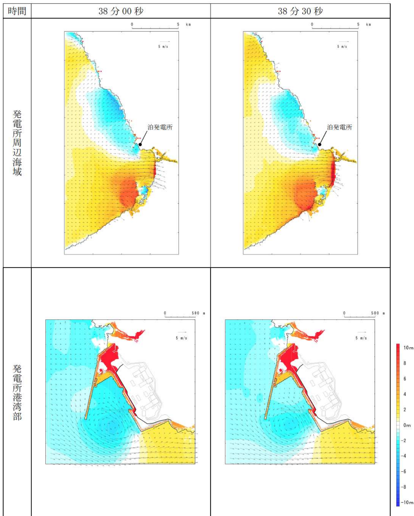
第7図-31 基準津波D（南防波堤損傷）の水位変動・流向ベクトル(31/53)
