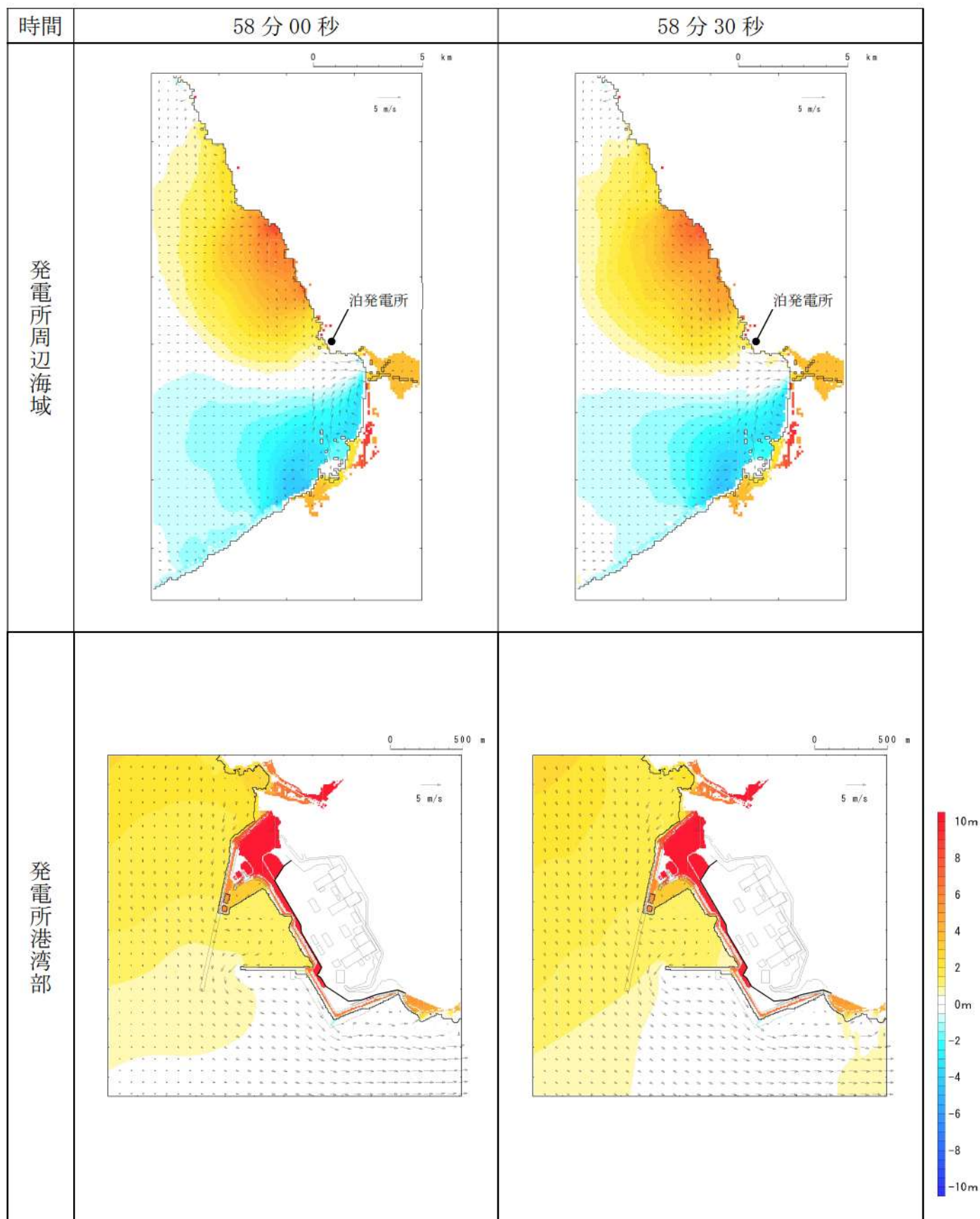
第 8 図-51 基準津波 D（北防波堤損傷）の水位変動・流向ベクトル (51/53)
