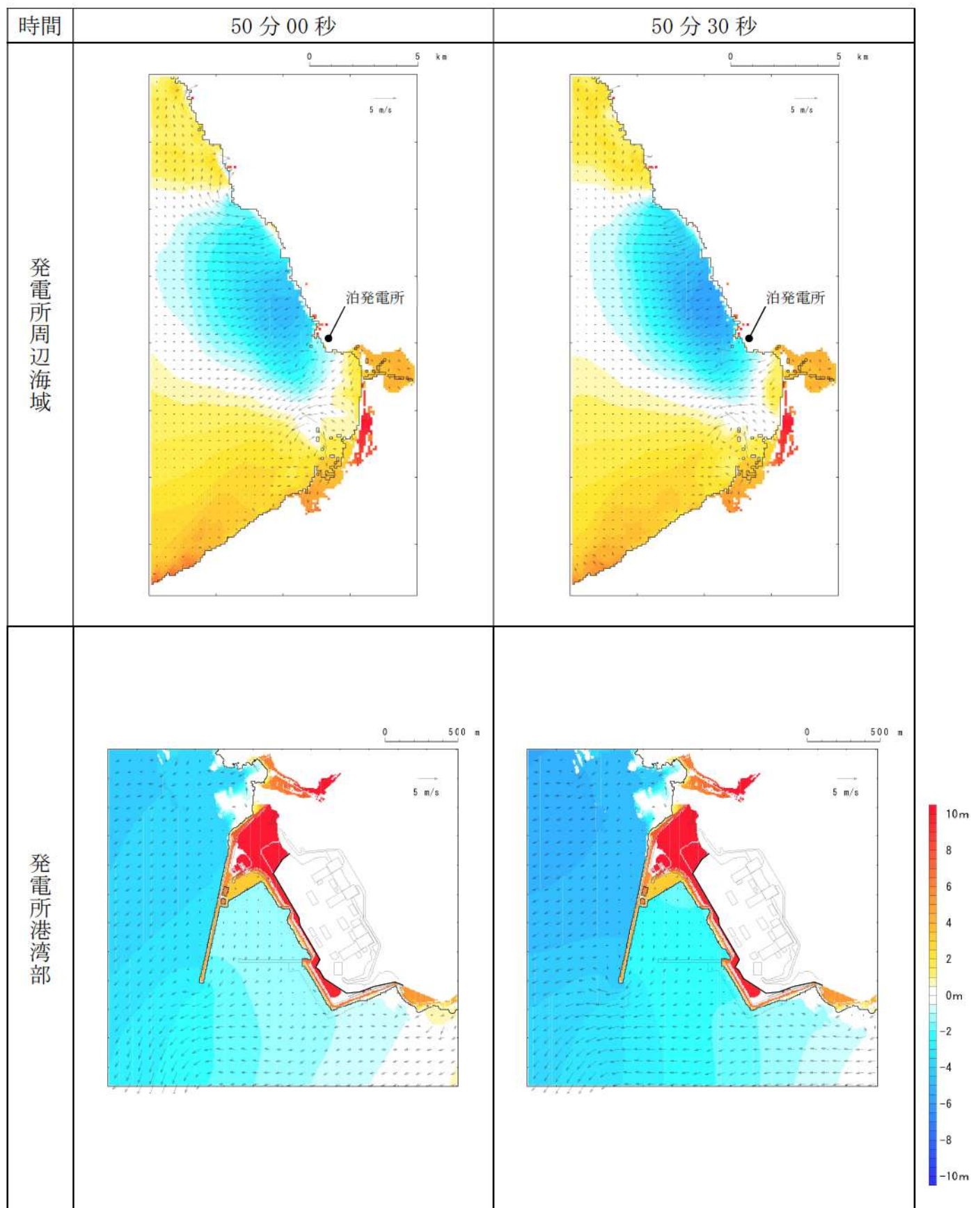
第 10 図-43 基準津波 E（南防波堤損傷）の水位変動・流向ベクトル(43/53)
