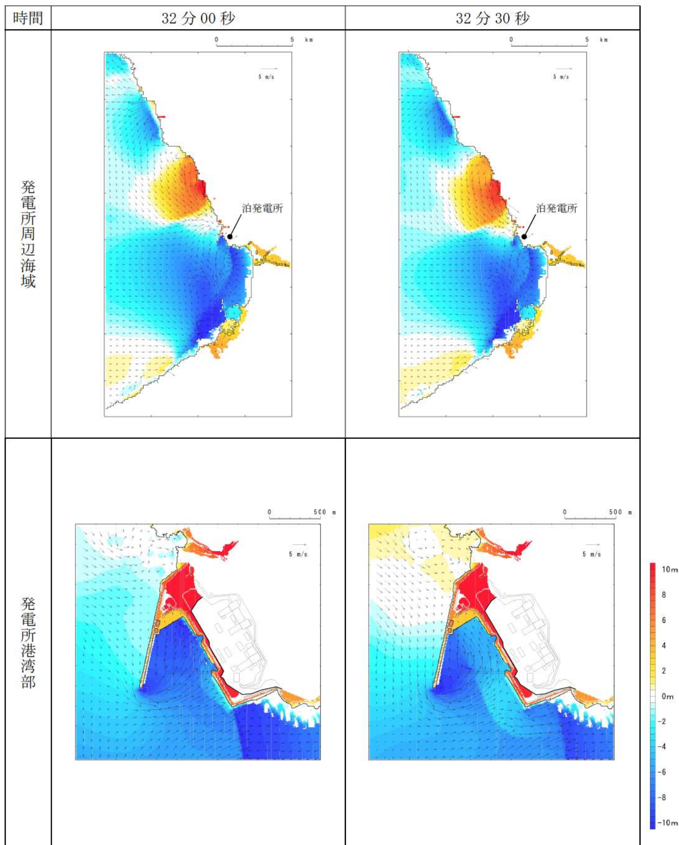
第 10 図-25 基準津波 E（南防波堤損傷）の水位変動・流向ベクトル (25/53)
