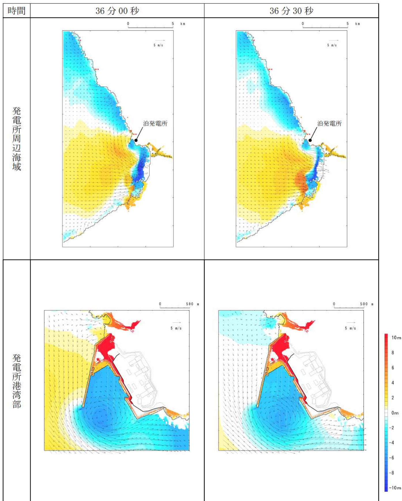
第7図-29 基準津波D（南防波堤損傷）の水位変動・流向ベクトル(29/53)
