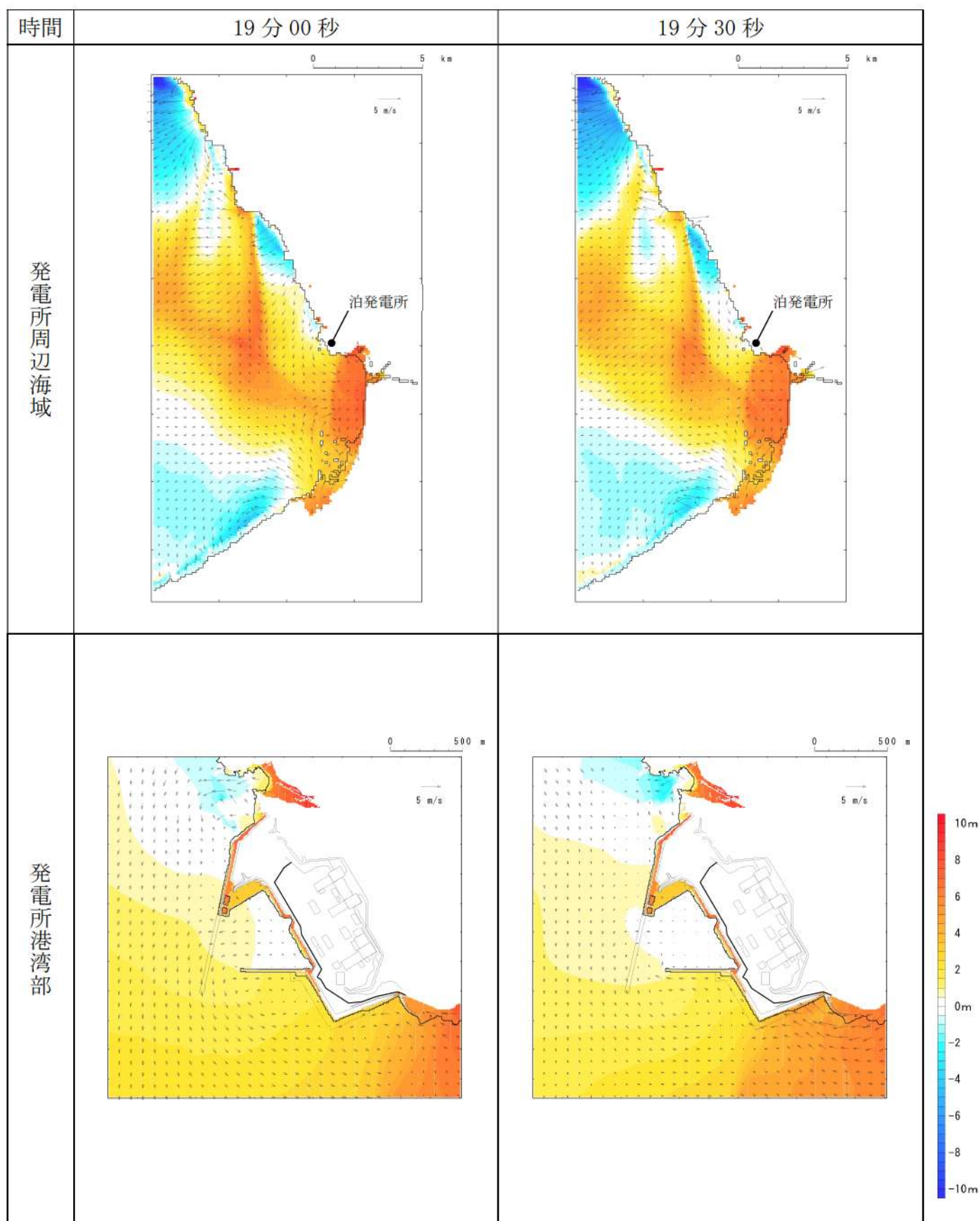
第 8 図-12 基準津波 D（北防波堤損傷）の水位変動・流向ベクトル(12/53)
