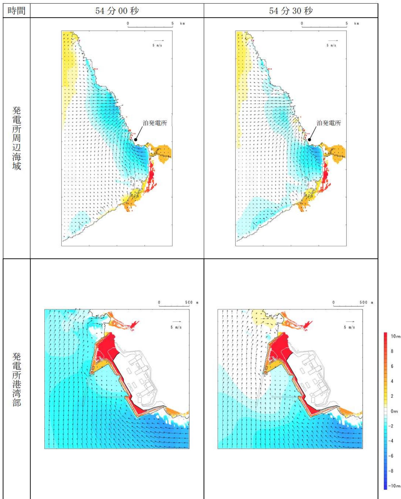
第 9 図-47 基準津波 E（北及び南防波堤損傷）の水位変動・流向ベクトル(47/53)
