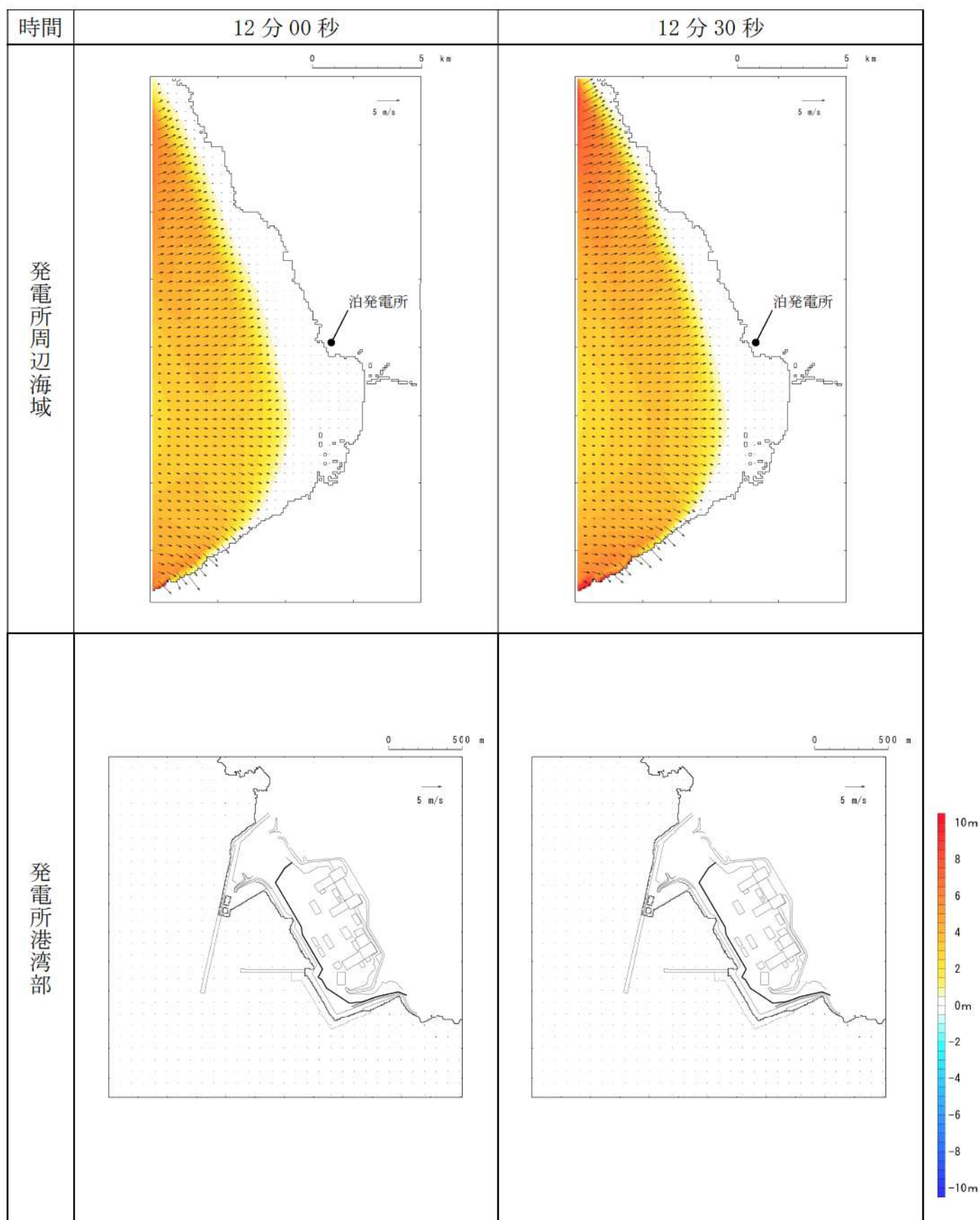
第9図-5 基準津波E（北及び南防波堤損傷）の水位変動・流向ベクトル(5/53)
