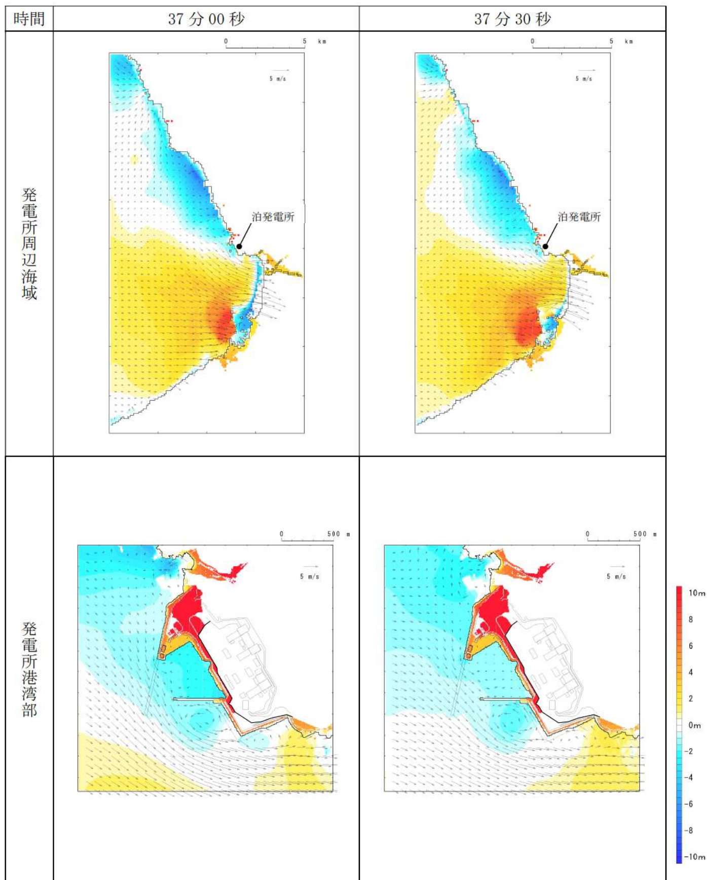
第 8 図-30 基準津波 D（北防波堤損傷）の水位変動・流向ベクトル(30/53)
