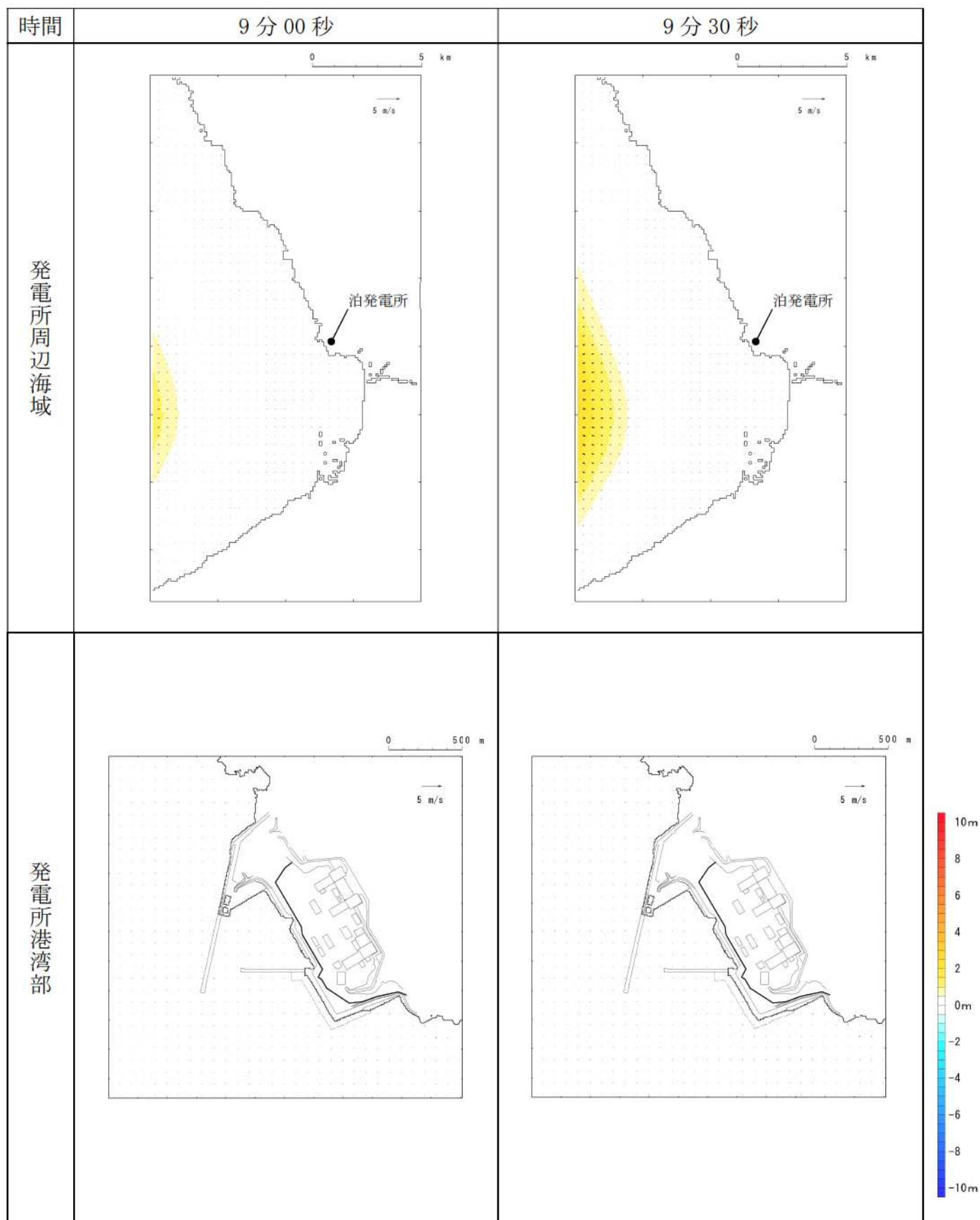
第9図-2 基準津波E（北及び南防波堤損傷）の水位変動・流向ベクトル(2/53)
