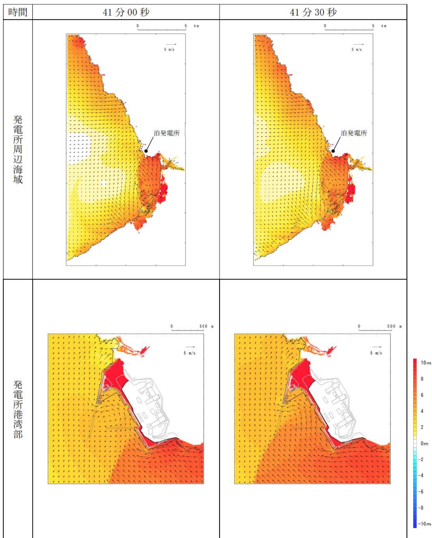
第 9 図-34 基準津波 E（北及び南防波堤損傷）の水位変動・流向ベクトル(34/53)
