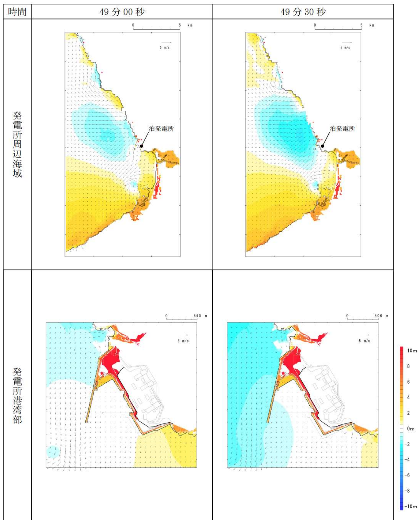
第 7 図-42 基準津波 D（南防波堤損傷）の水位変動・流向ベクトル(42/53)
