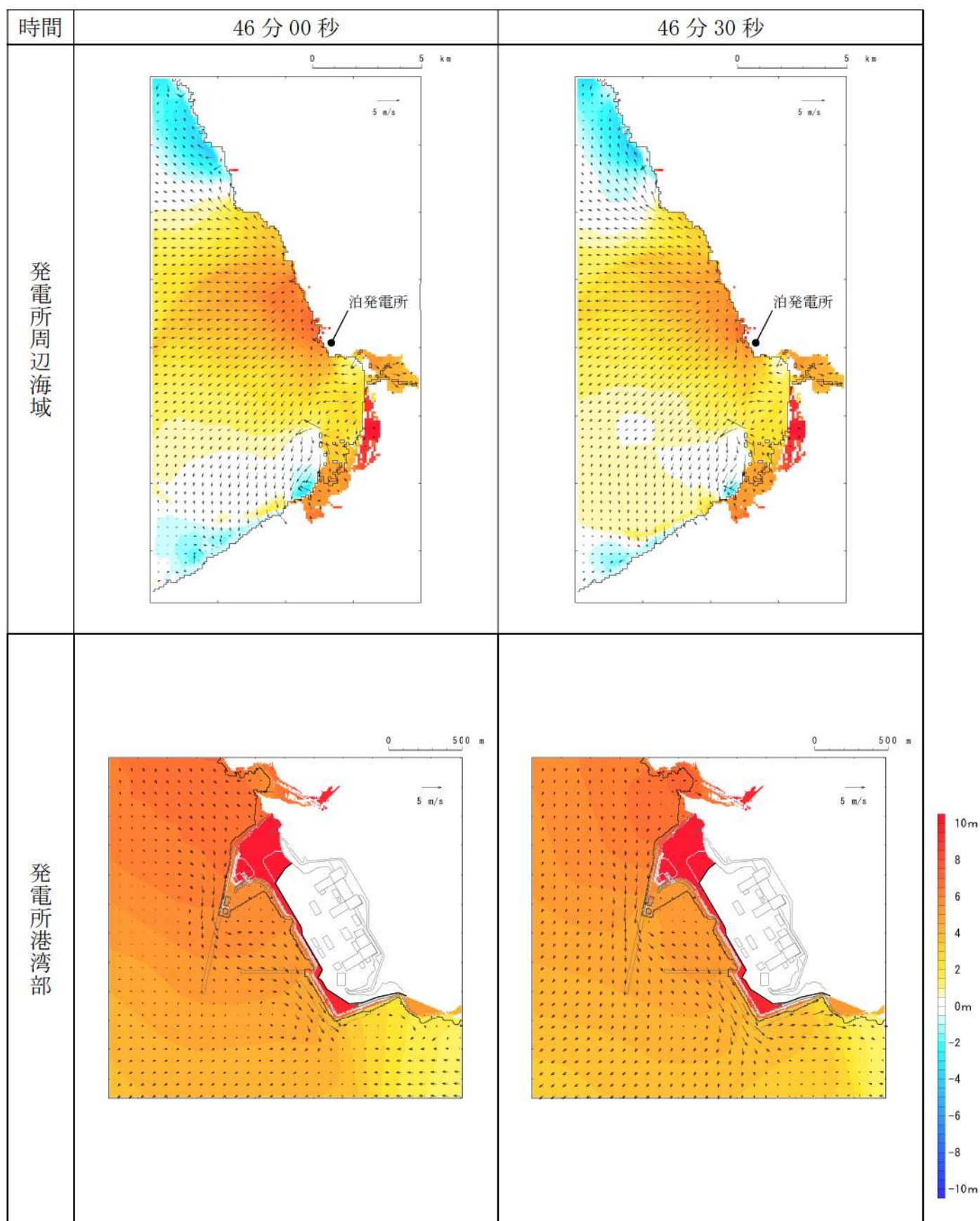
第 9 図-39 基準津波 E（北及び南防波堤損傷）の水位変動・流向ベクトル(39/53)
