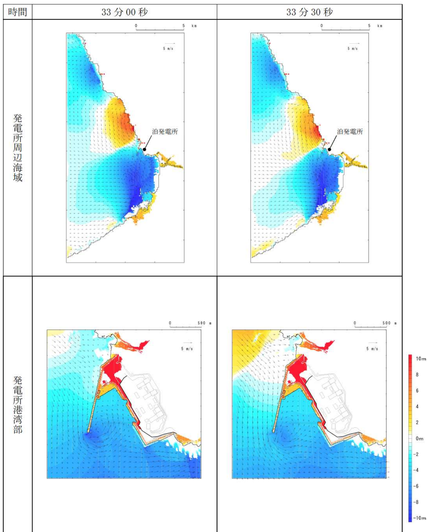
第7図-26 基準津波D（南防波堤損傷）の水位変動・流向ベクトル(26/53)
