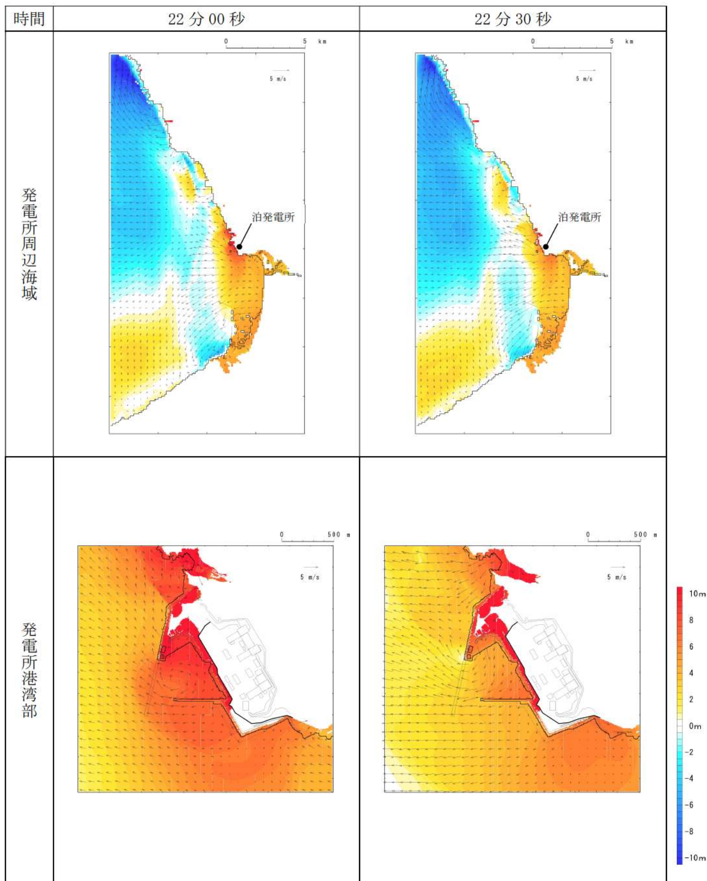
第8図-15 基準津波D（北防波堤損傷）の水位変動・流向ベクトル(15/53)
