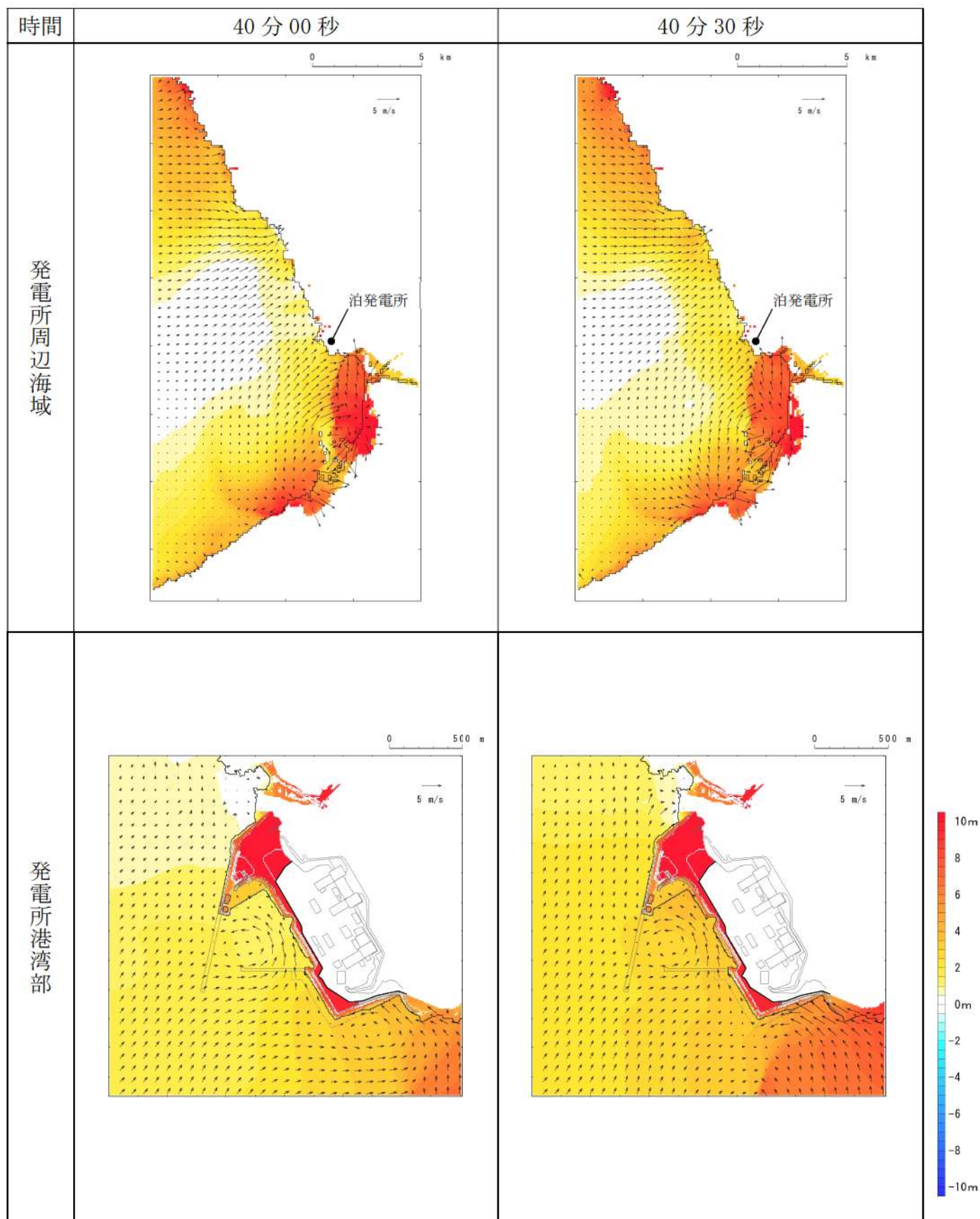
第 9 図-33 基準津波 E（北及び南防波堤損傷）の水位変動・流向ベクトル(33/53)
