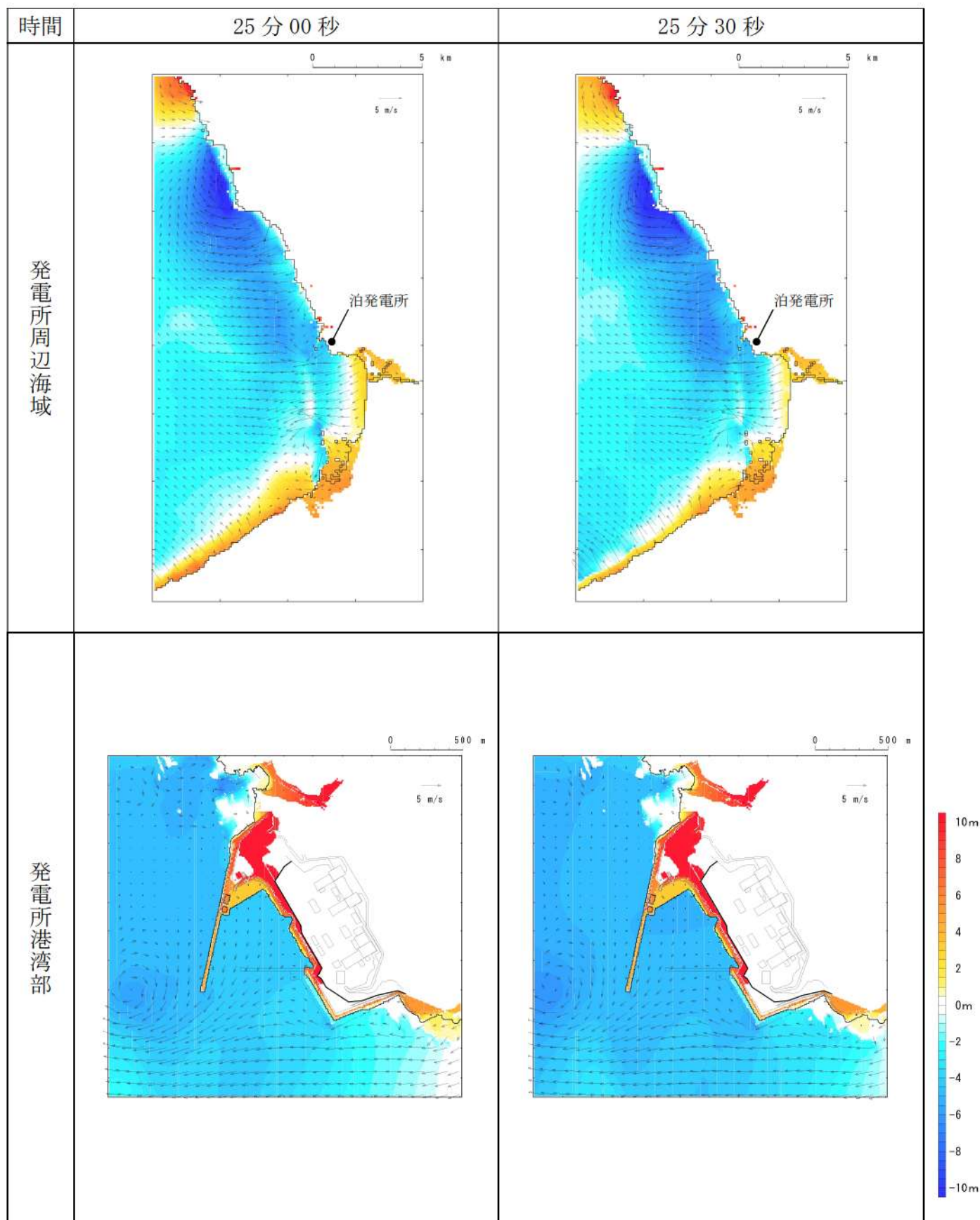
第7図-18 基準津波D（南防波堤損傷）の水位変動・流向ベクトル(18/53)
