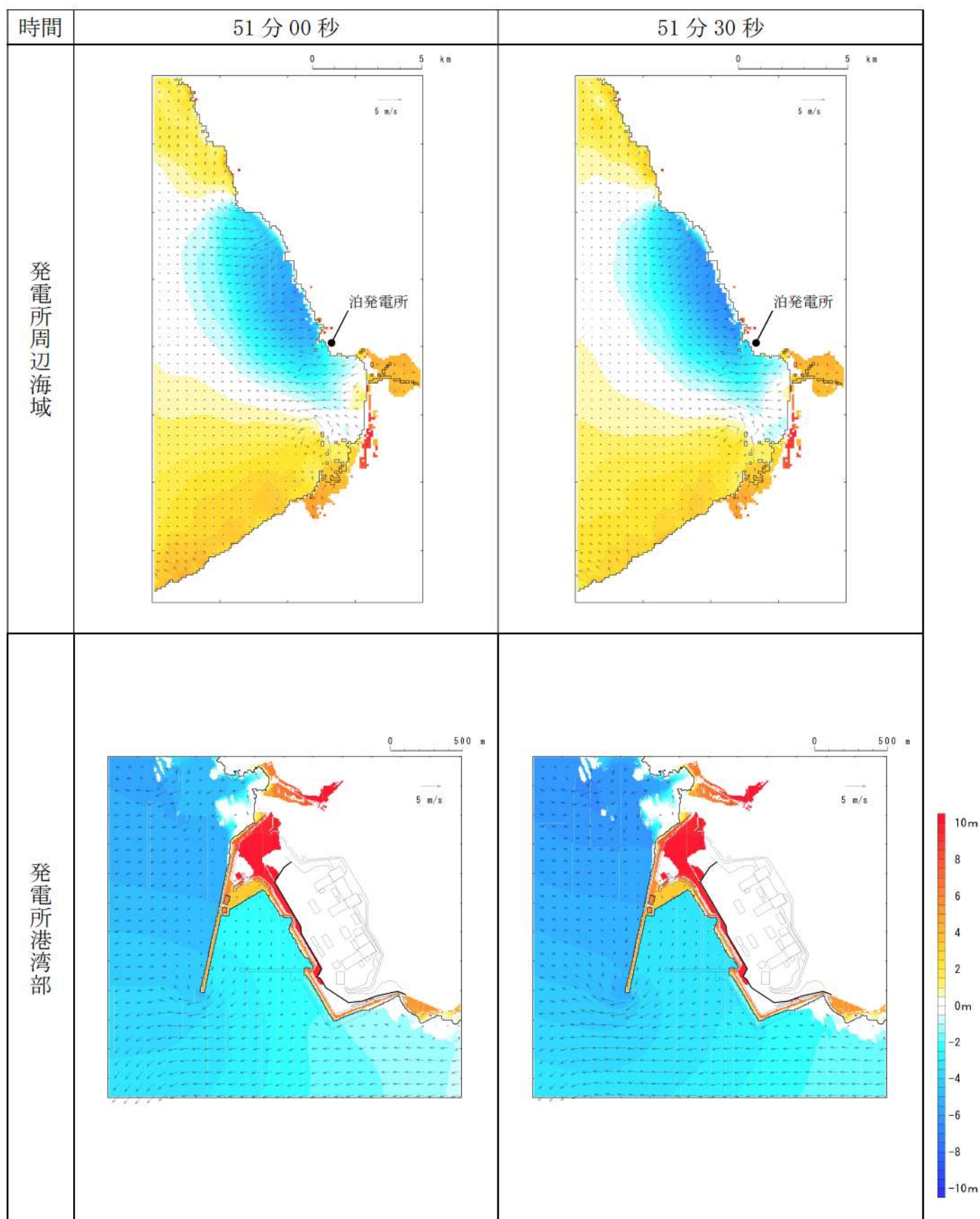
第 7 図-44 基準津波 D（南防波堤損傷）の水位変動・流向ベクトル(44/53)
