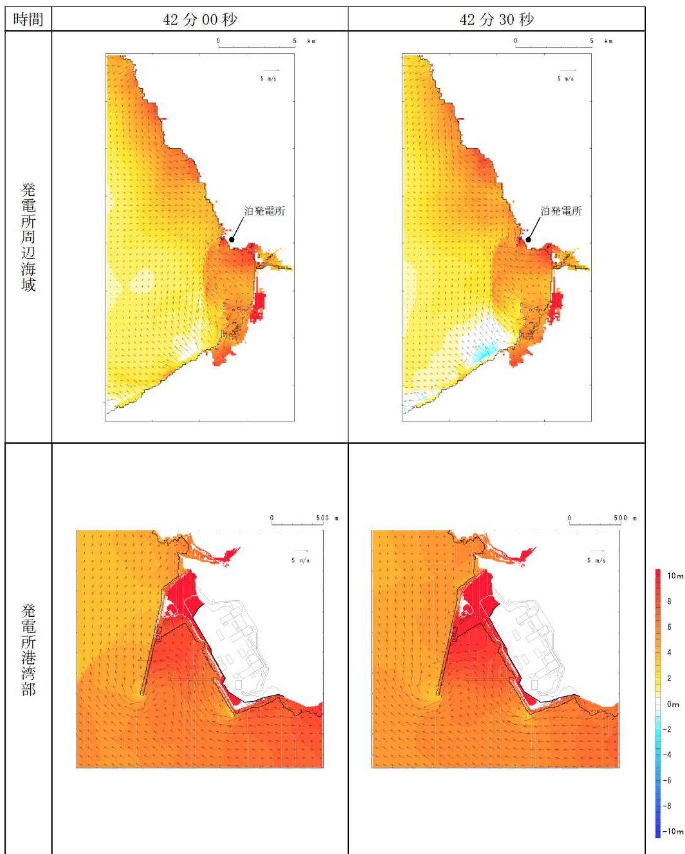
第 10 図-35 基準津波 E（南防波堤損傷）の水位変動・流向ベクトル(35/53)
