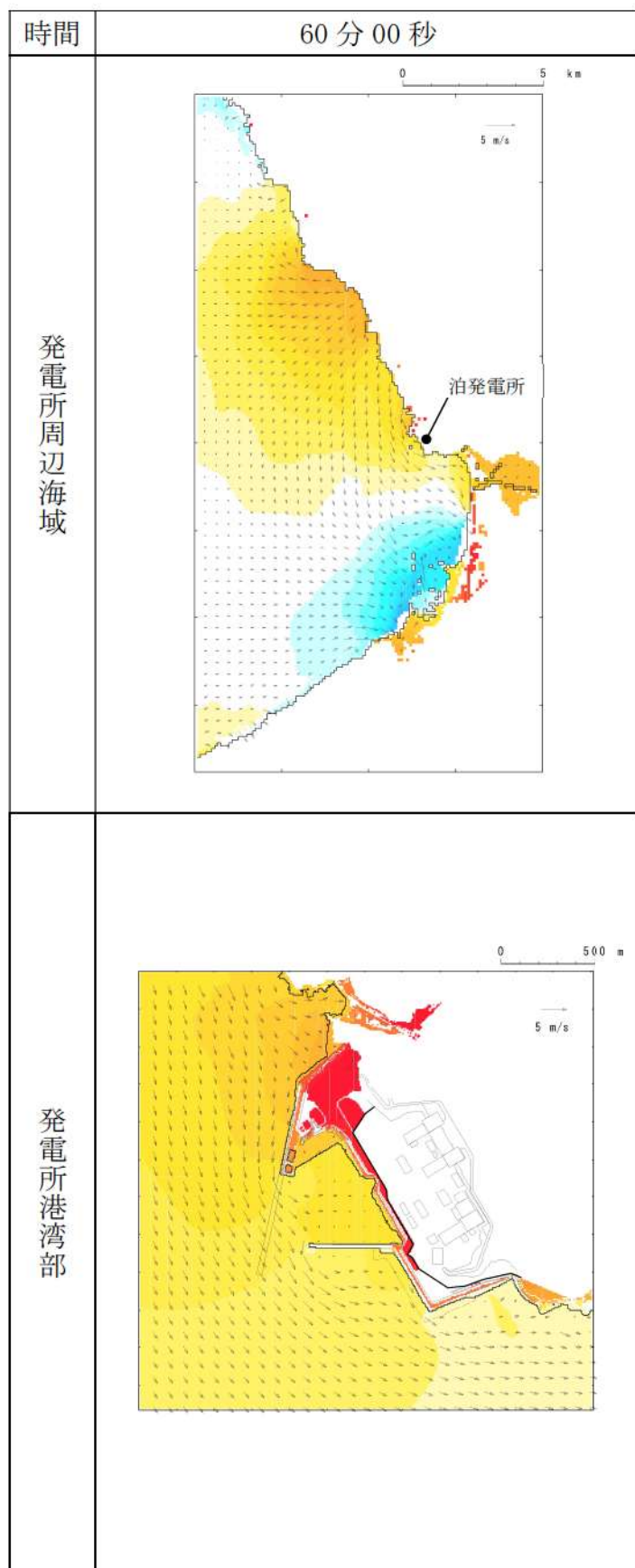
第 8 図-53 基準津波 D（北防波堤損傷）の水位変動・流向ベクトル (53/53)
