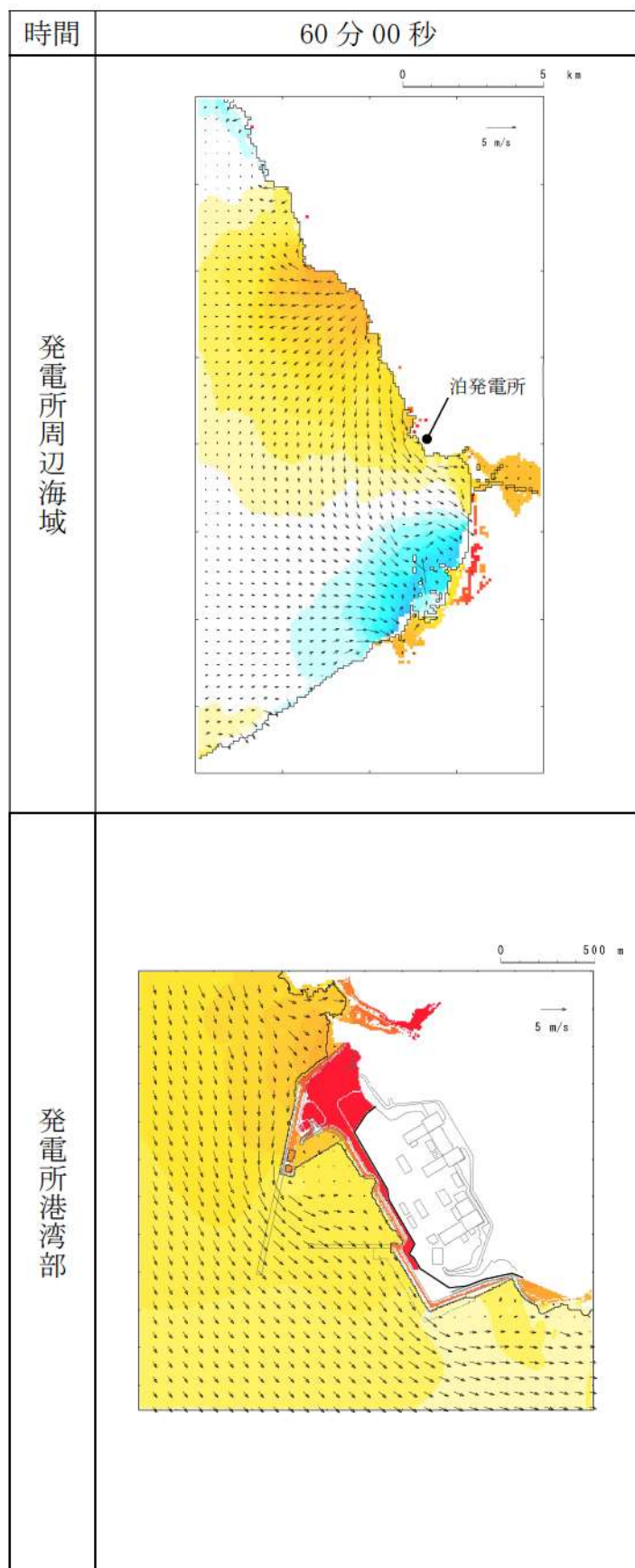
第 6 図-53 基準津波 D（北及び南防波堤損傷）の水位変動・流向ベクトル(53/53)
