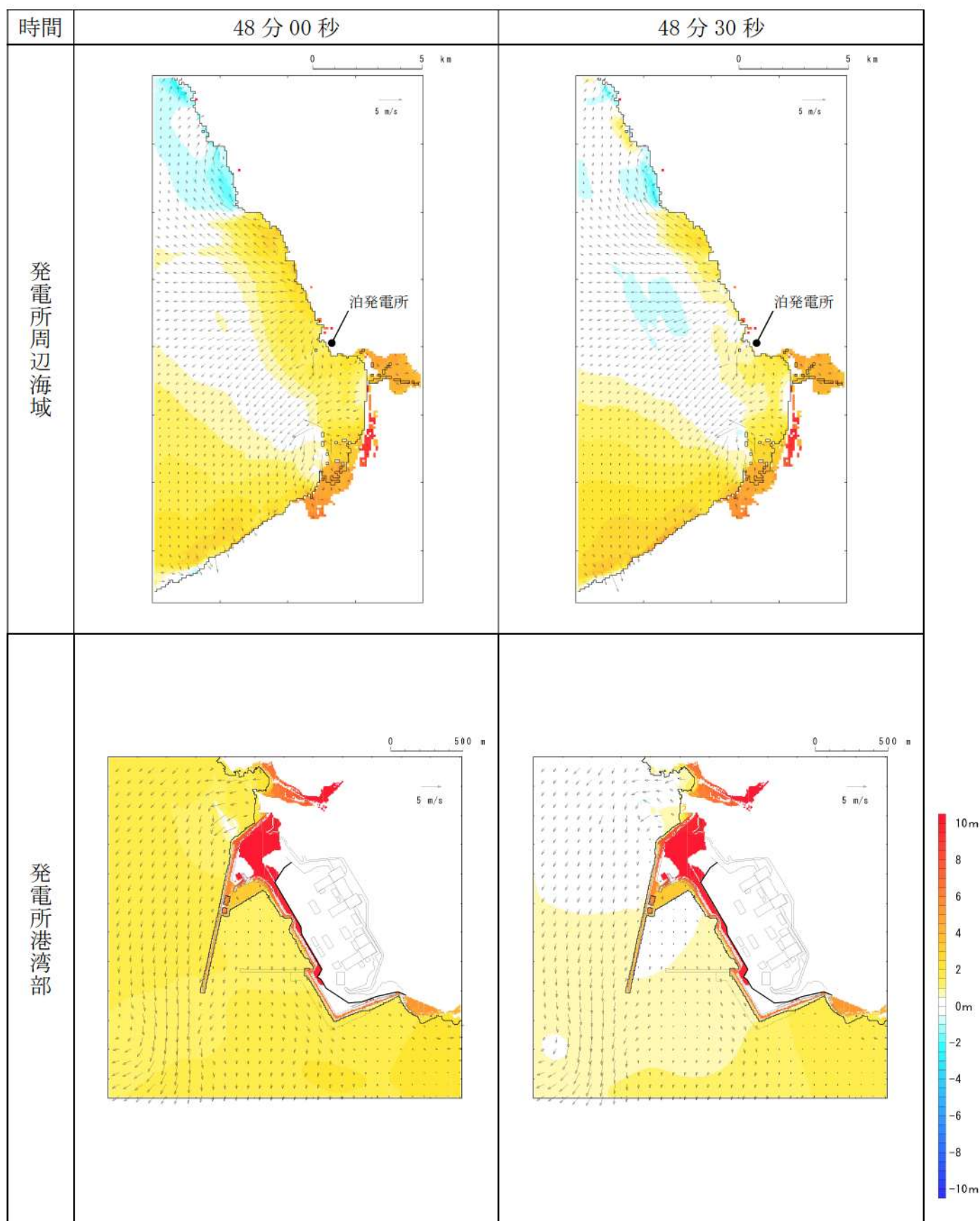
第 7 図-41 基準津波 D（南防波堤損傷）の水位変動・流向ベクトル(41/53)
