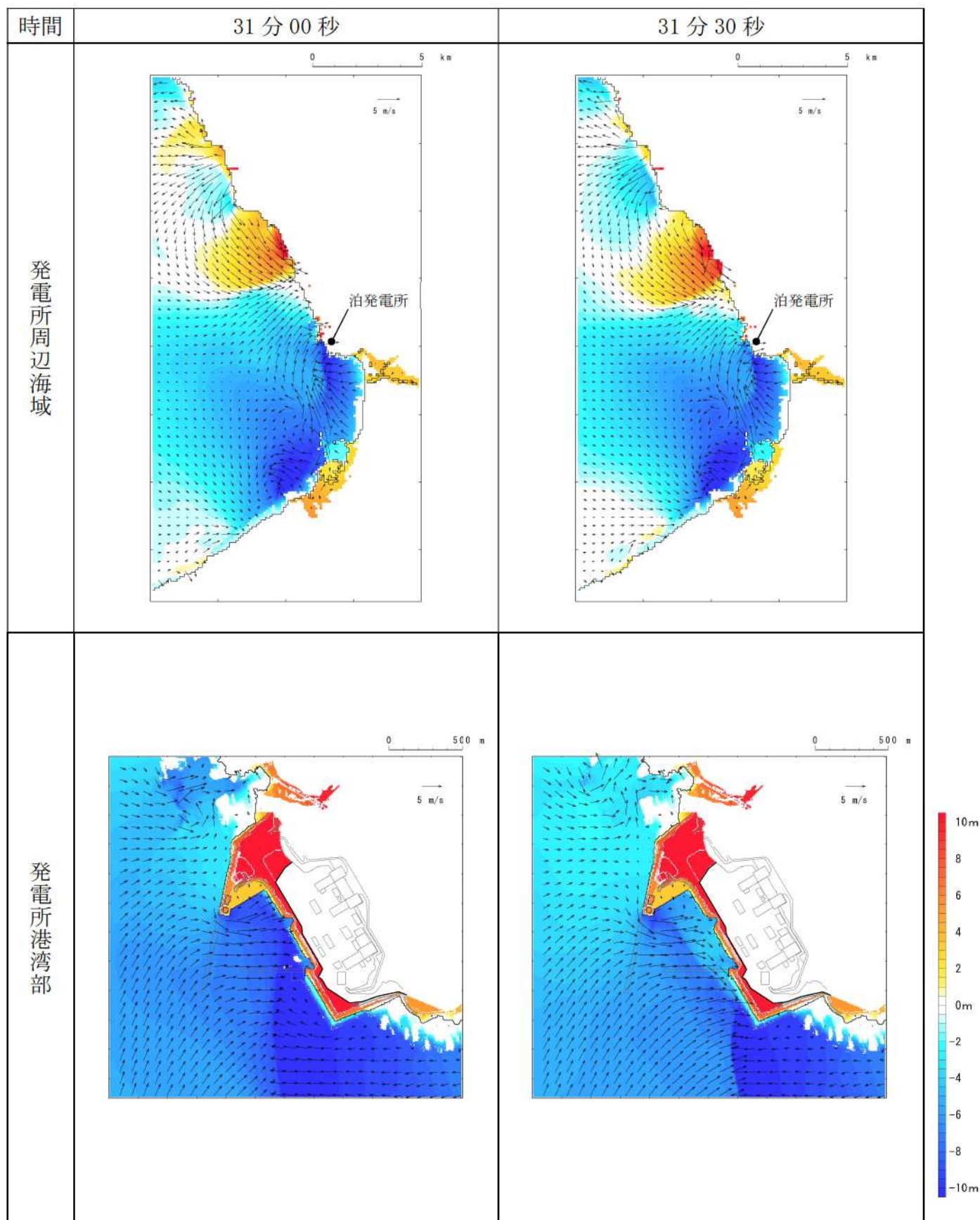
第9図-24 基準津波E（北及び南防波堤損傷）の水位変動・流向ベクトル(24/53)
