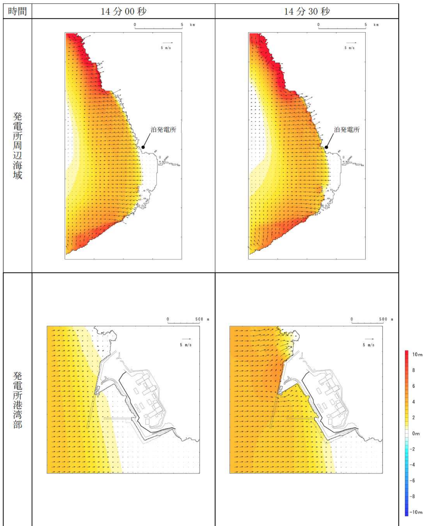
第9図-7 基準津波E（北及び南防波堤損傷）の水位変動・流向ベクトル(7/53)
