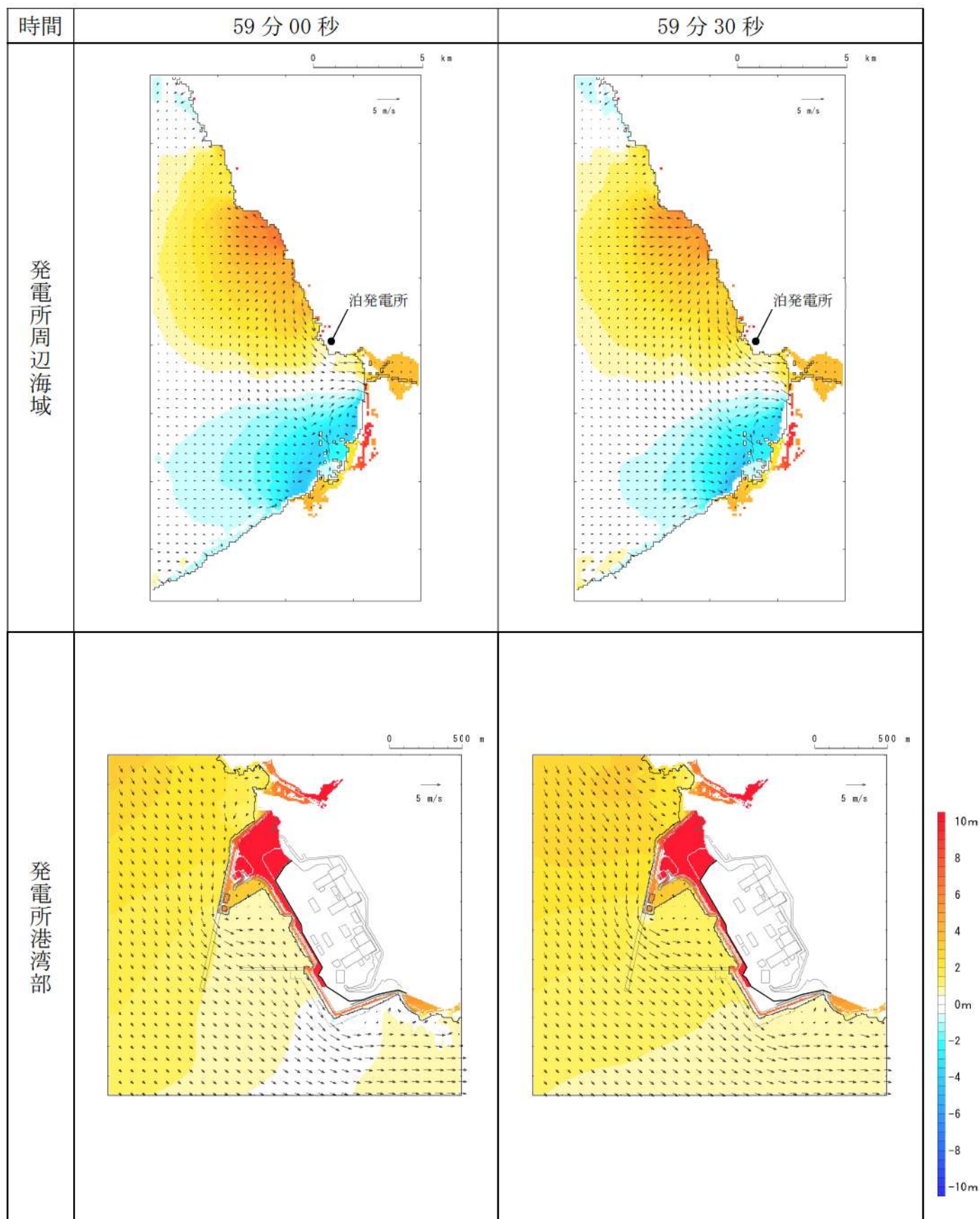
第 6 図-52 基準津波 D（北及び南防波堤損傷）の水位変動・流向ベクトル(52/53)
