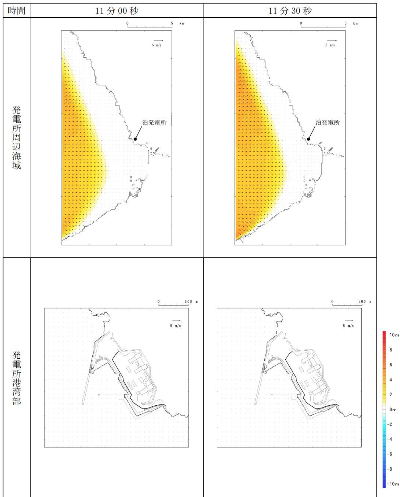
第9図-4 基準津波E（北及び南防波堤損傷）の水位変動・流向ベクトル(4/53)
