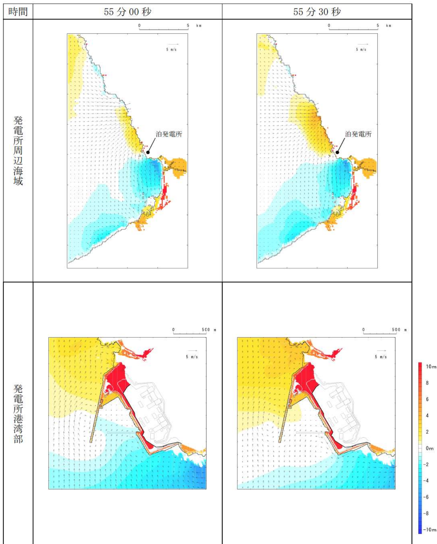
第 10 図-48 基準津波 E（南防波堤損傷）の水位変動・流向ベクトル(48/53)
