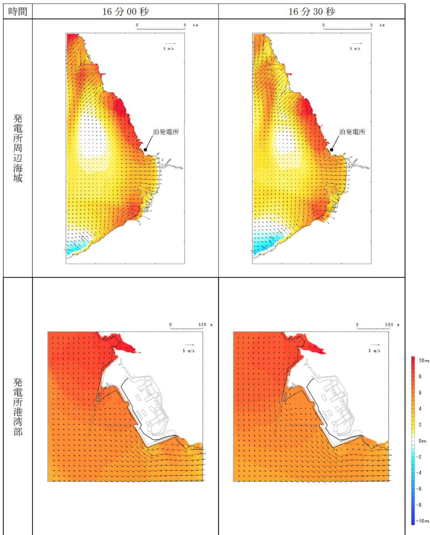
第9図-9 基準津波E（北及び南防波堤損傷）の水位変動・流向ベクトル(9/53)
