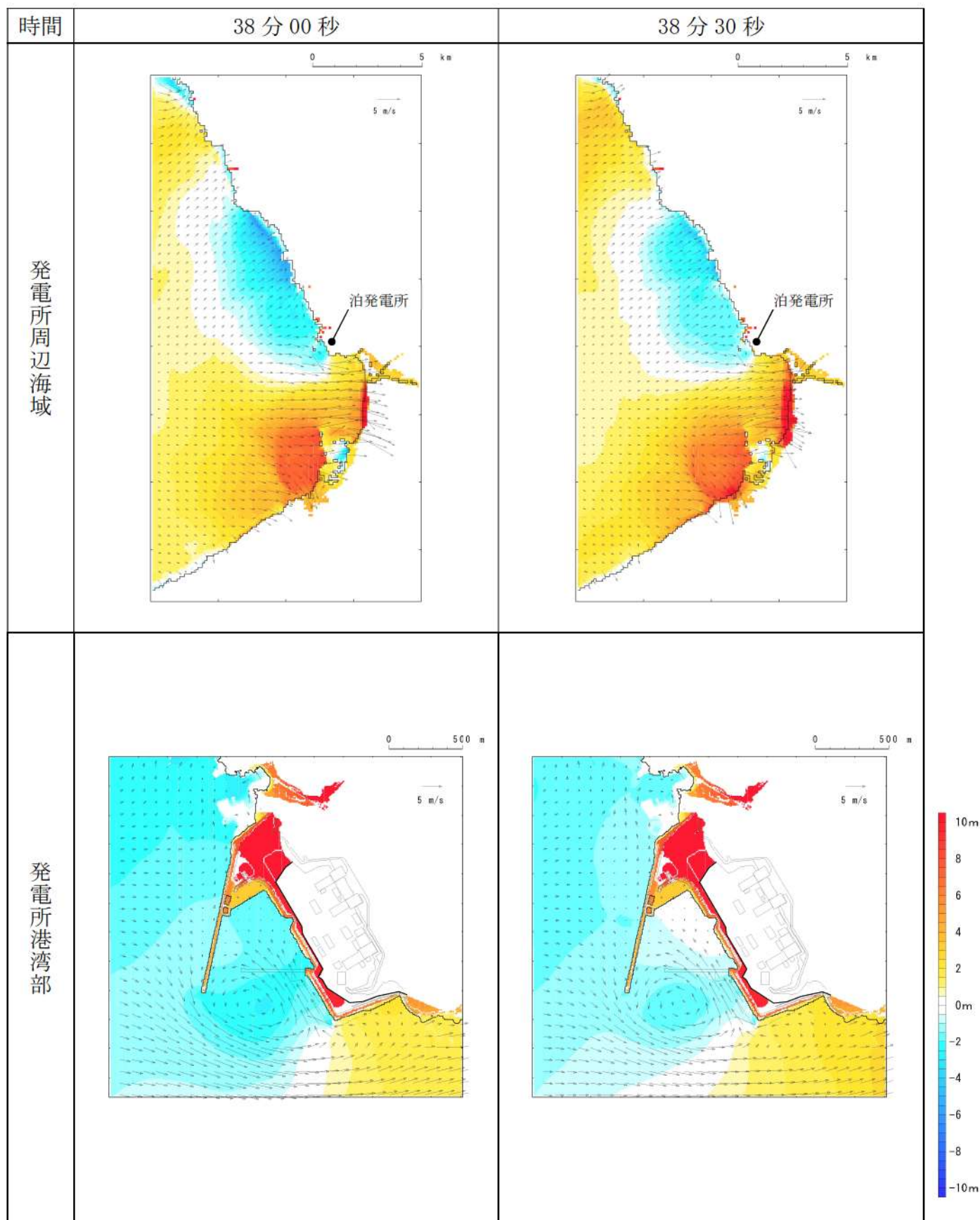
第 10 図-31 基準津波 E（南防波堤損傷）の水位変動・流向ベクトル(31/53)
