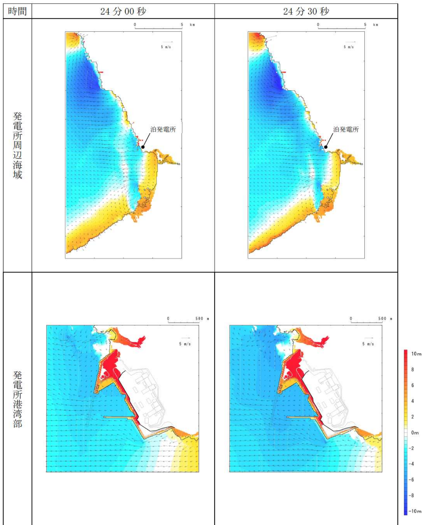
第8図-17 基準津波D（北防波堤損傷）の水位変動・流向ベクトル(17/53)
