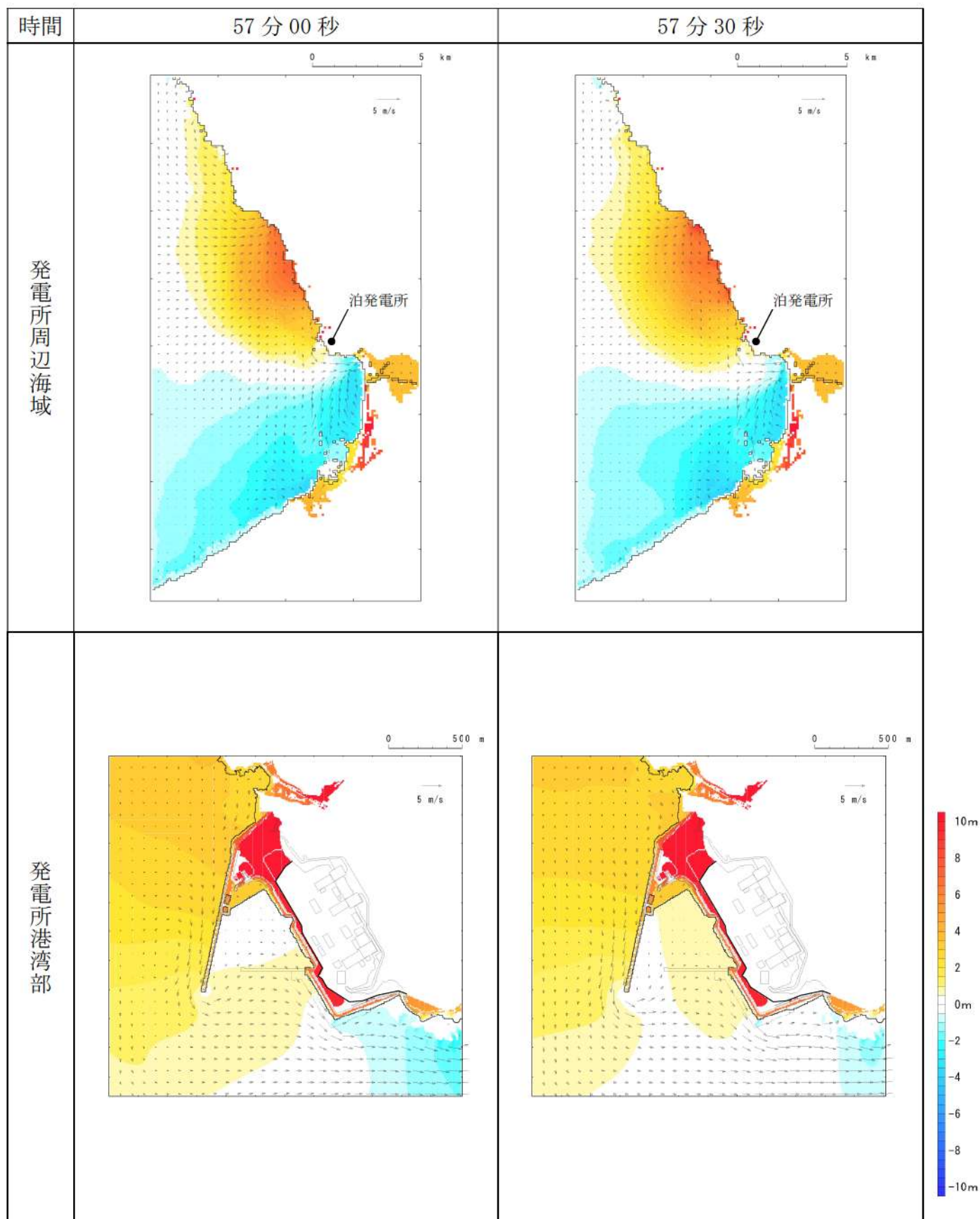
第 10 図-50 基準津波 E（南防波堤損傷）の水位変動・流向ベクトル (50/53)
