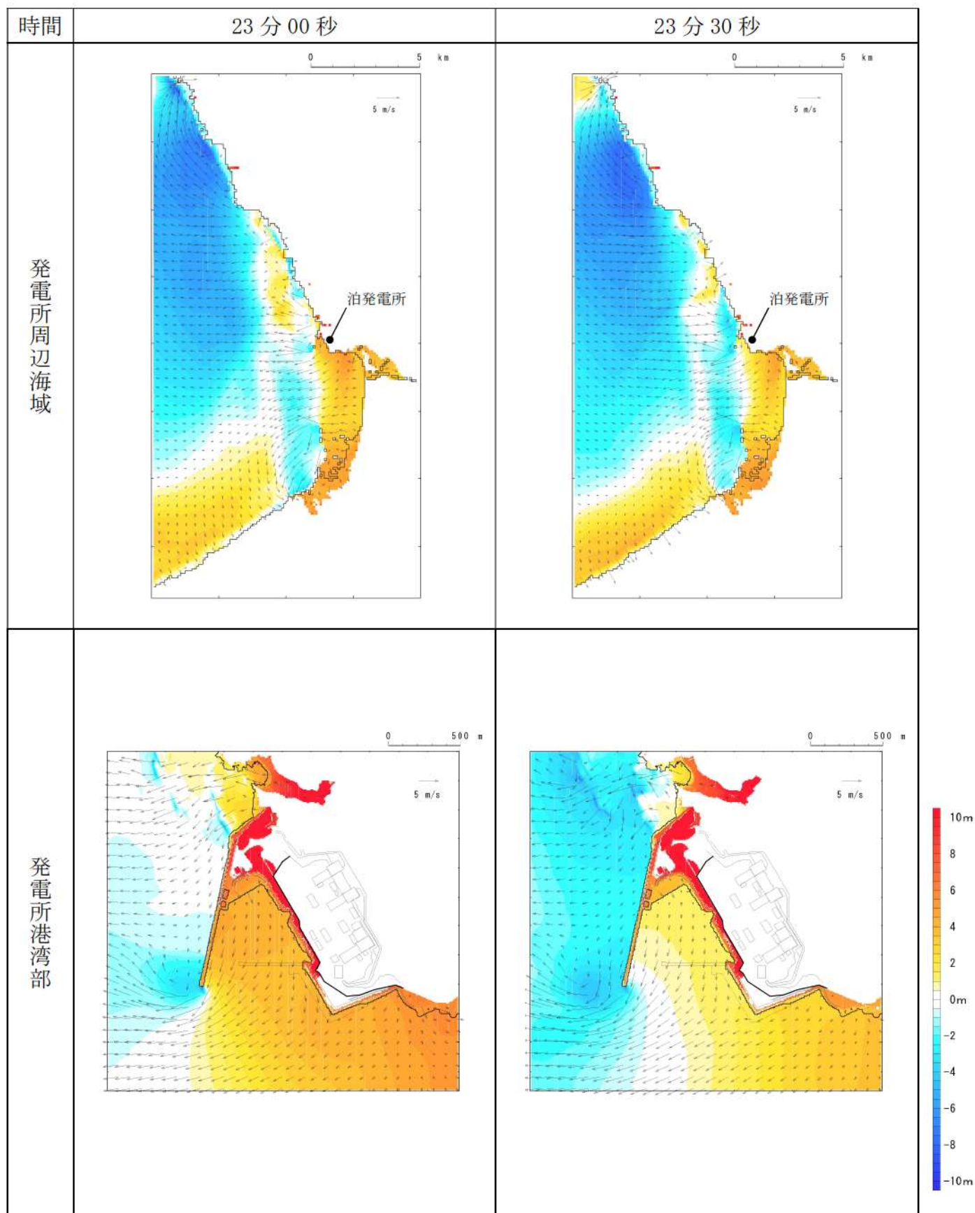
第 7 図-16 基準津波 D（南防波堤損傷）の水位変動・流向ベクトル(16/53)
