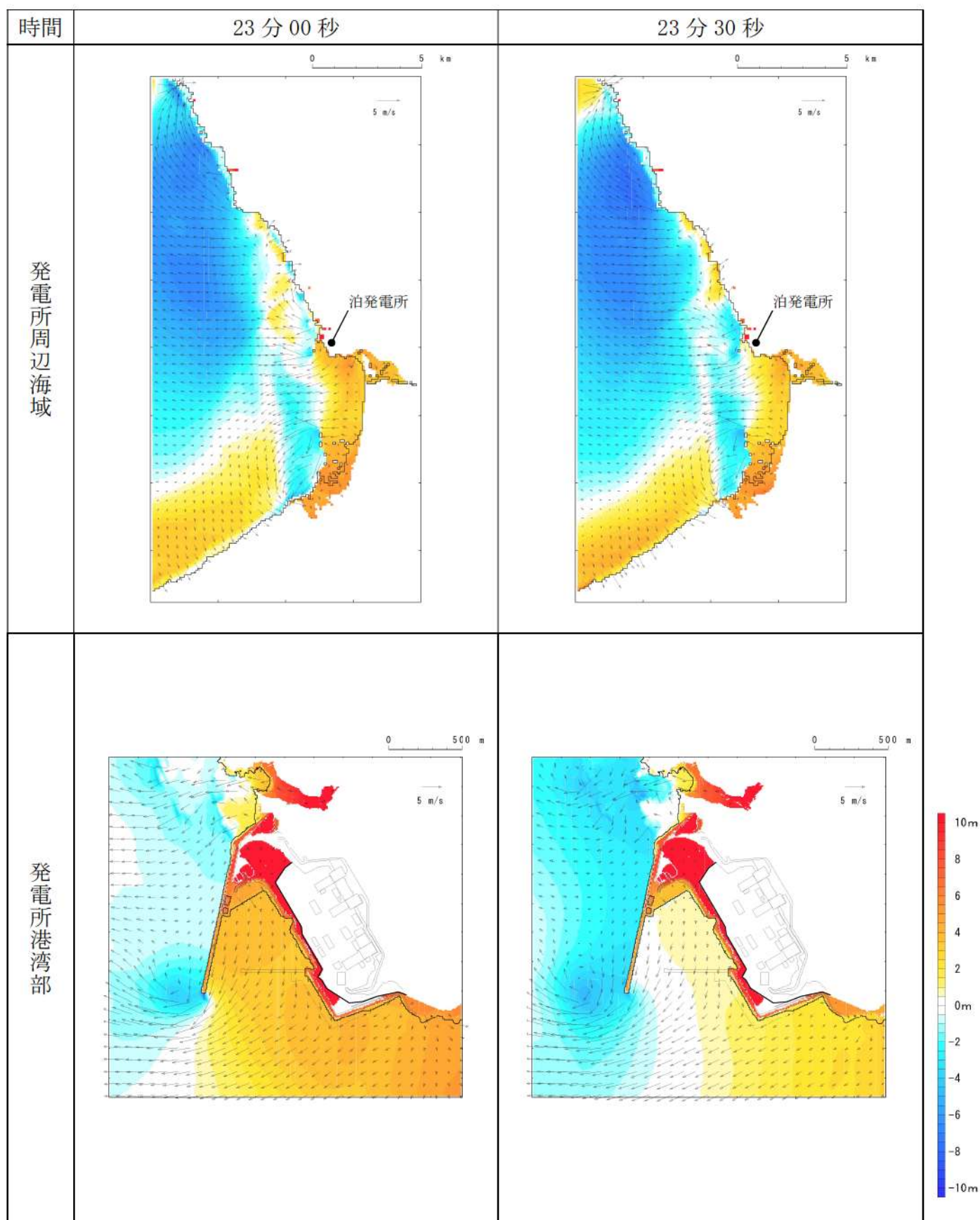
第 10 図-16 基準津波 E（南防波堤損傷）の水位変動・流向ベクトル(16/53)
