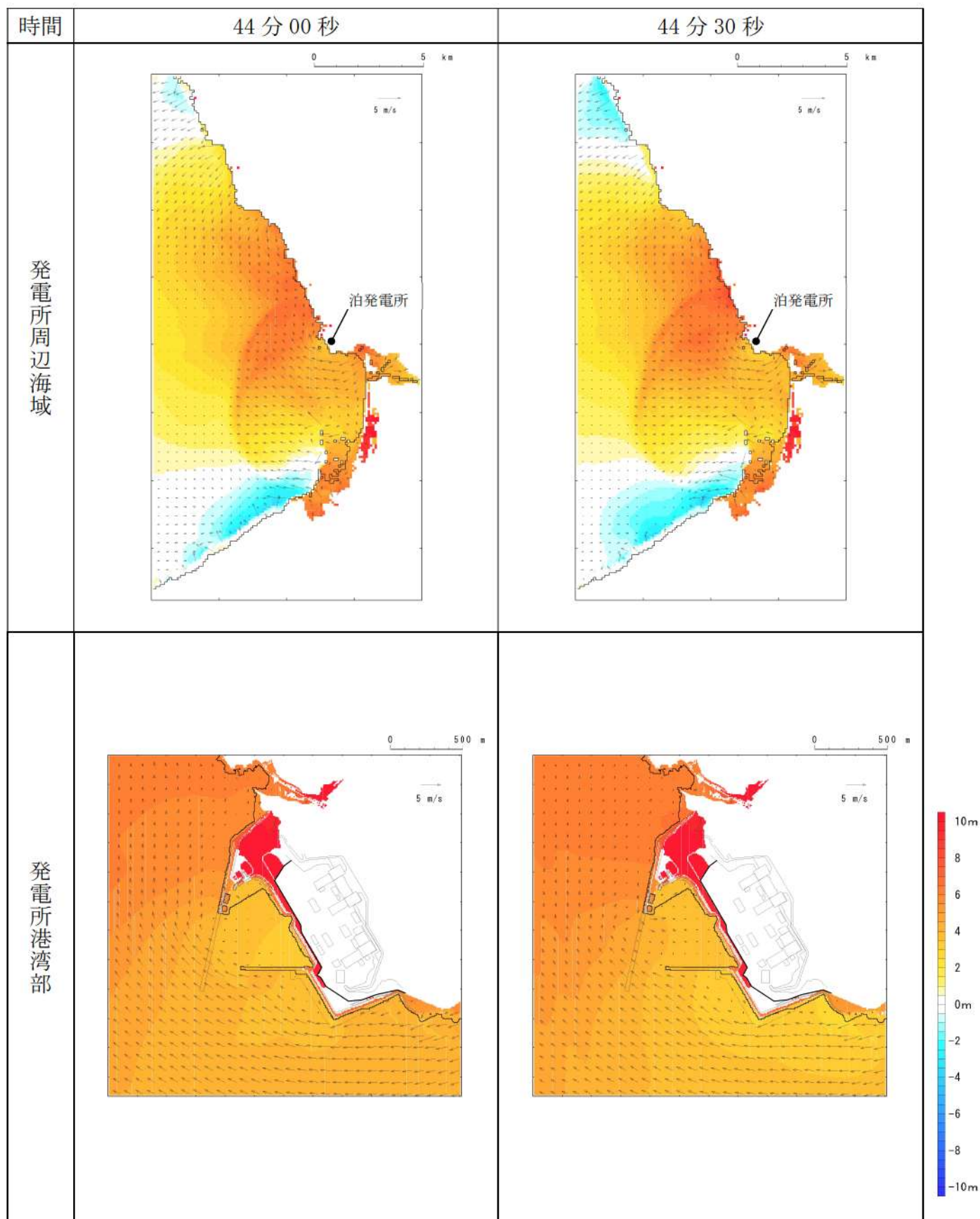
第8図-37 基準津波D（北防波堤損傷）の水位変動・流向ベクトル(37/53)
