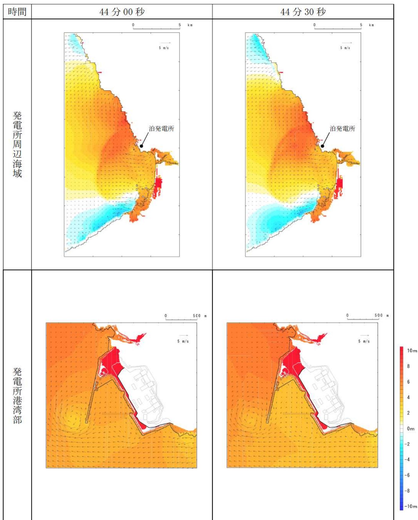
第 10 図-37 基準津波 E（南防波堤損傷）の水位変動・流向ベクトル(37/53)
