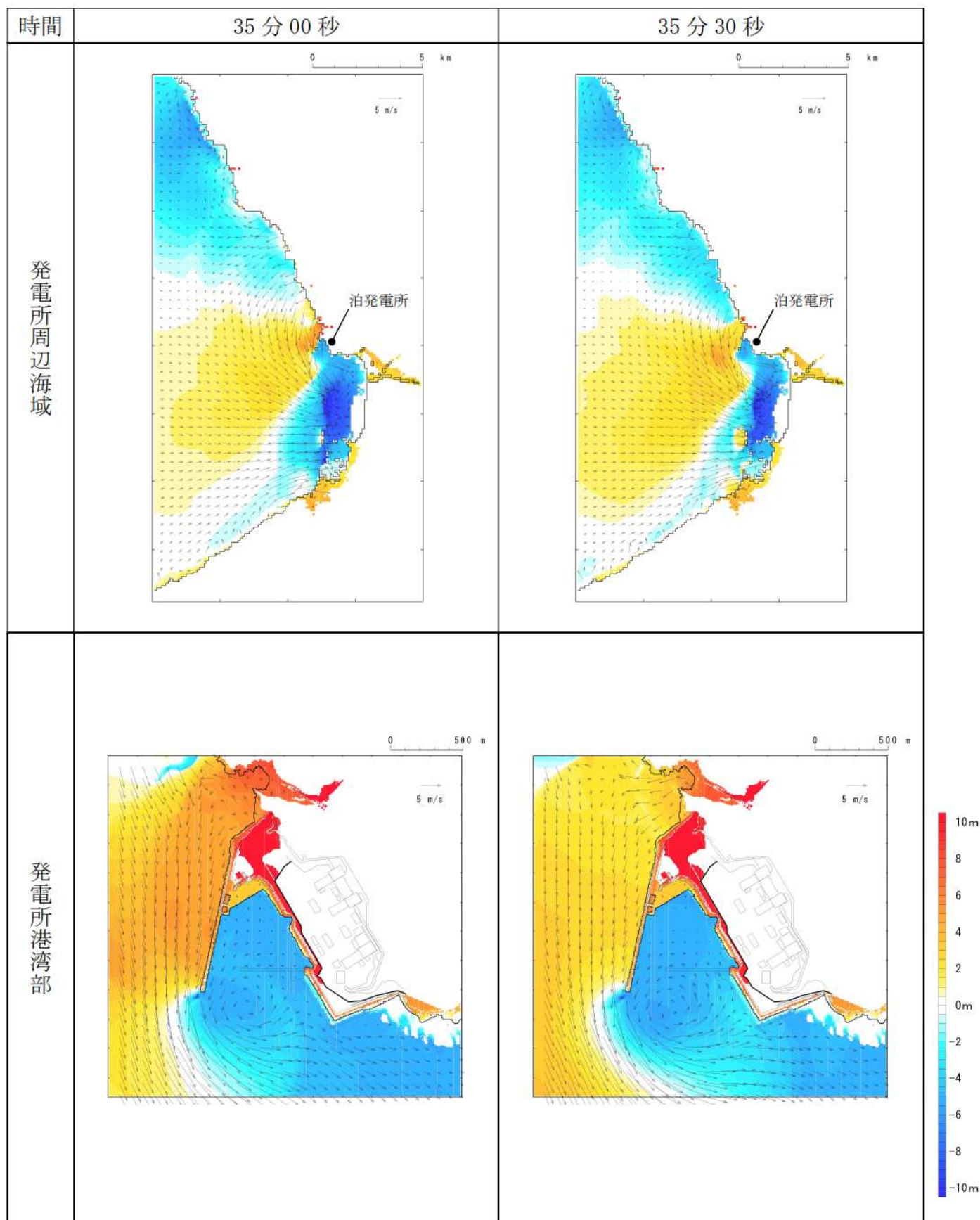
第7図-28 基準津波D（南防波堤損傷）の水位変動・流向ベクトル(28/53)
