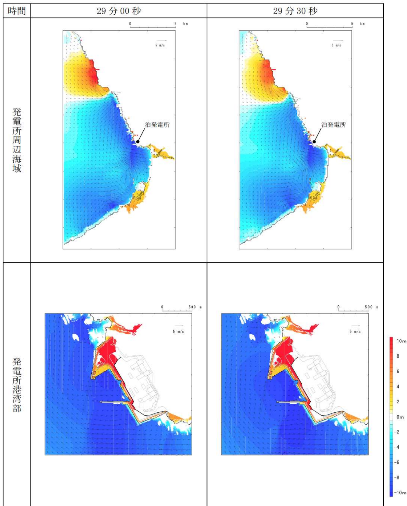
第8図-22 基準津波D（北防波堤損傷）の水位変動・流向ベクトル(22/53)
