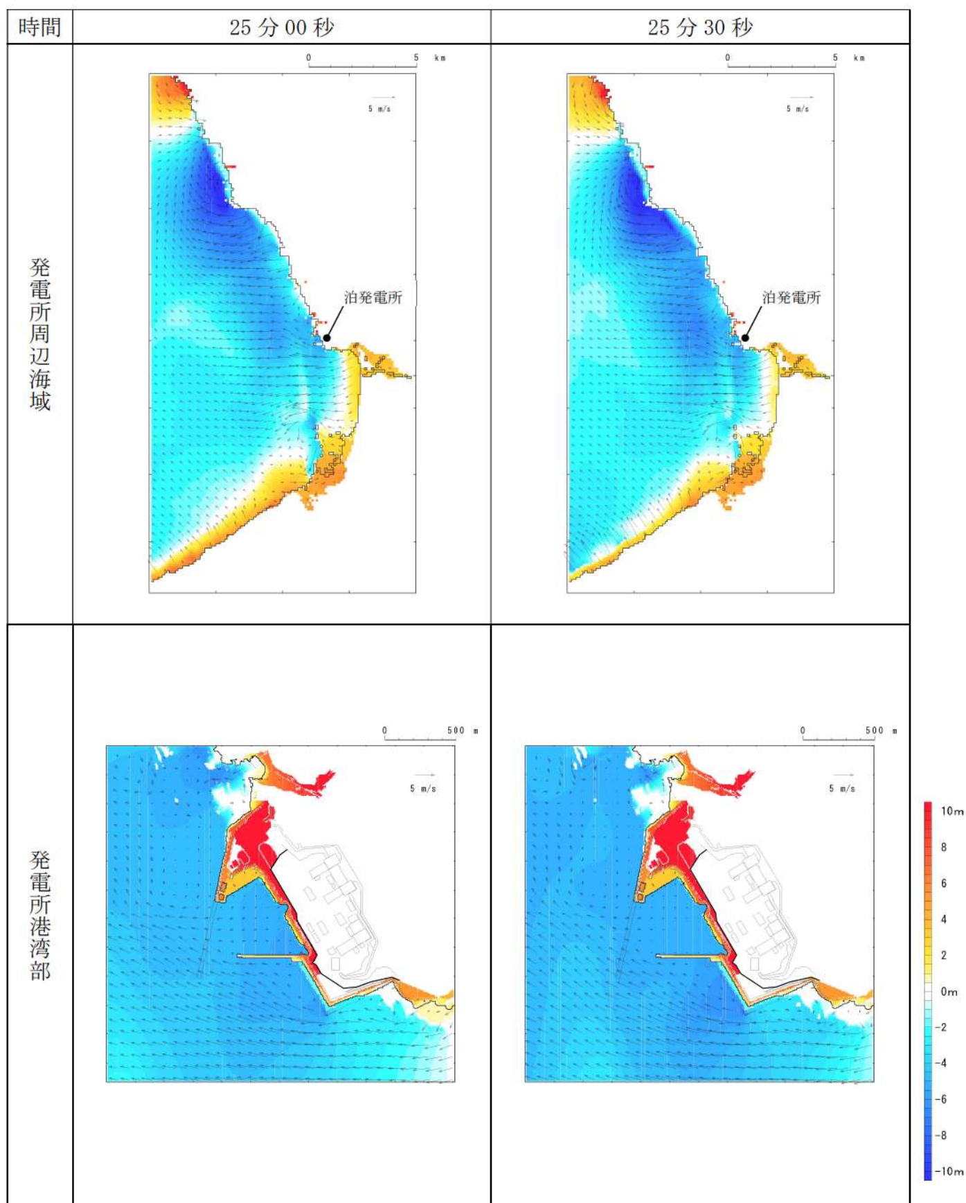
第8図-18 基準津波D（北防波堤損傷）の水位変動・流向ベクトル(18/53)
