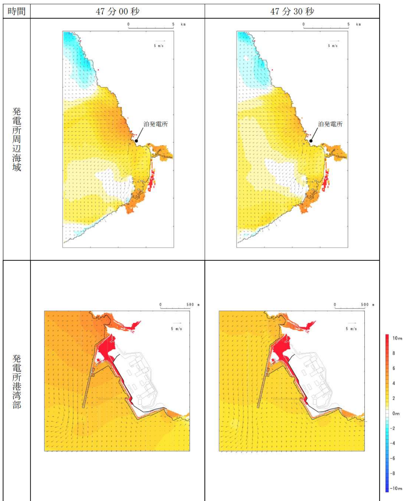
第7図-40 基準津波D（南防波堤損傷）の水位変動・流向ベクトル(40/53)
