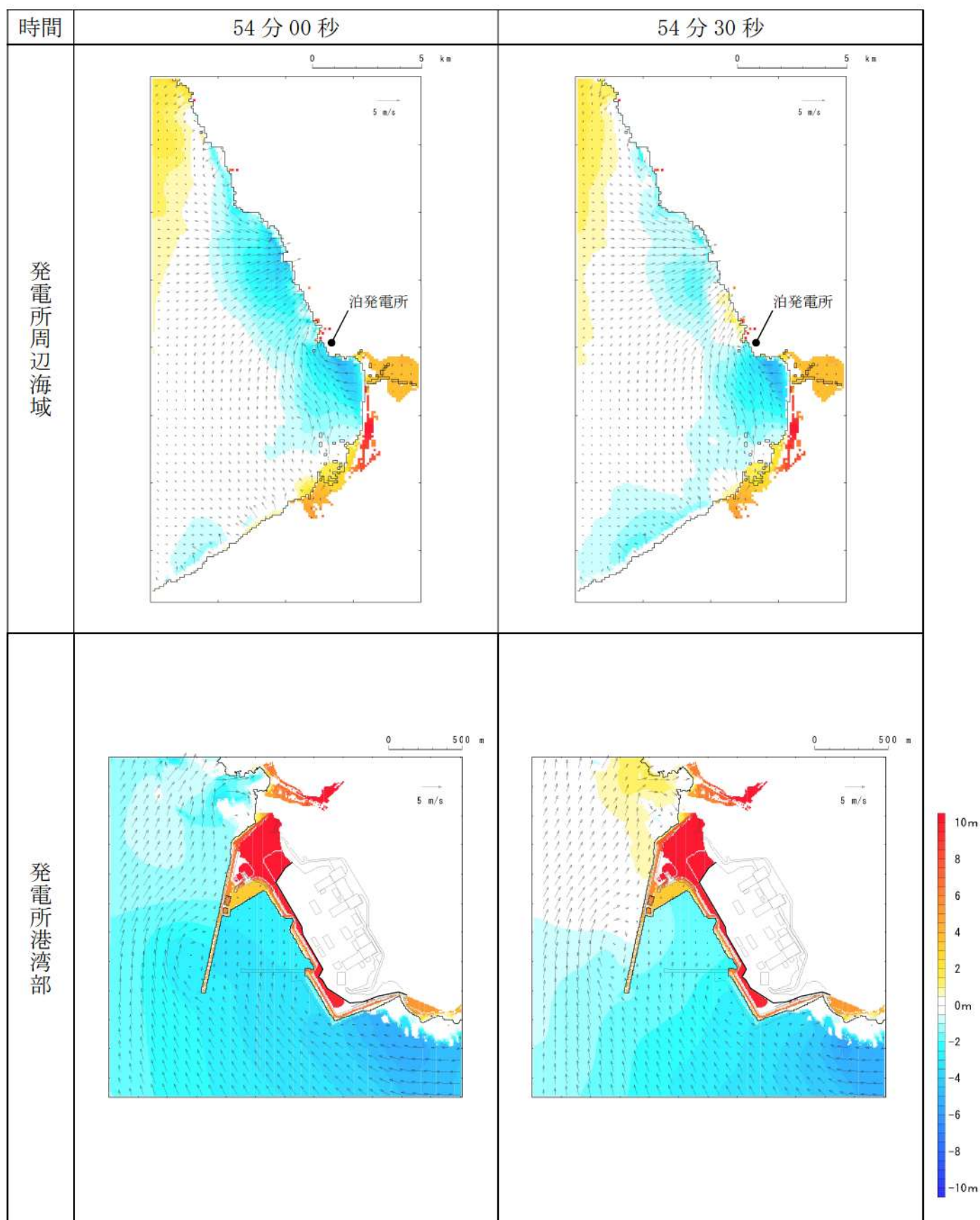
第 10 図-47 基準津波 E（南防波堤損傷）の水位変動・流向ベクトル(47/53)
