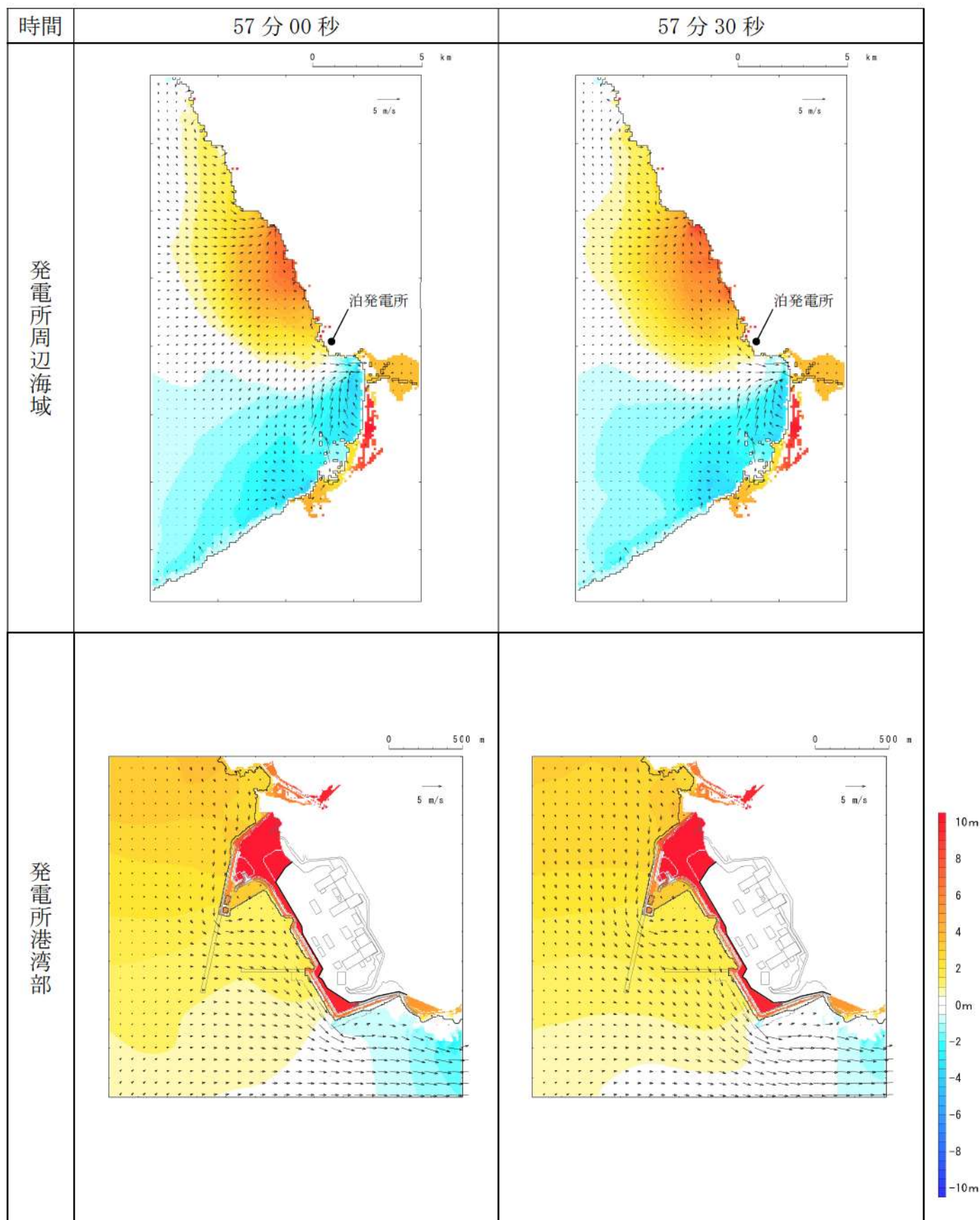
第 9 図-50 基準津波 E（北及び南防波堤損傷）の水位変動・流向ベクトル(50/53)
