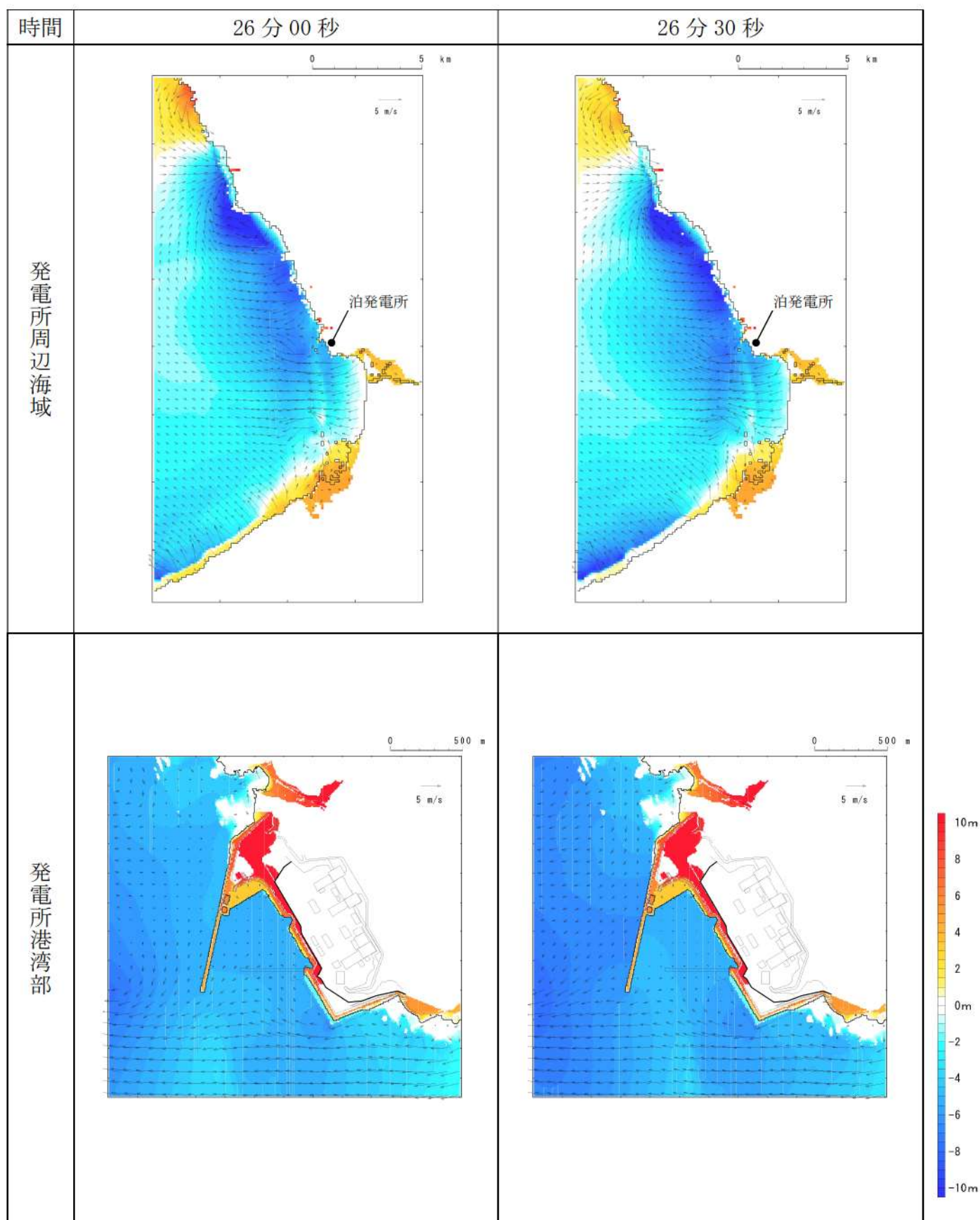
第7図-19 基準津波D（南防波堤損傷）の水位変動・流向ベクトル(19/53)
