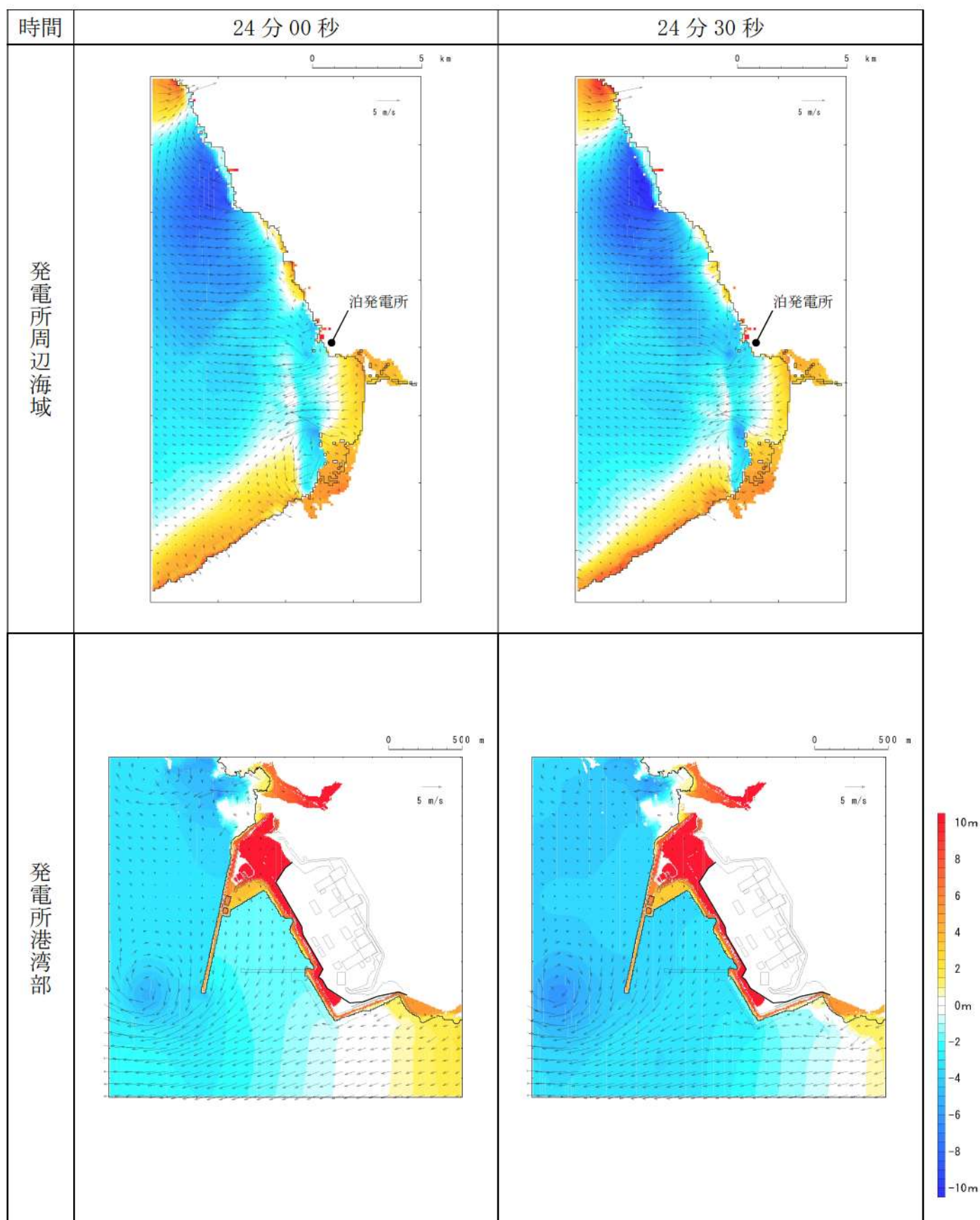
第 10 図-17 基準津波 E（南防波堤損傷）の水位変動・流向ベクトル(17/53)
