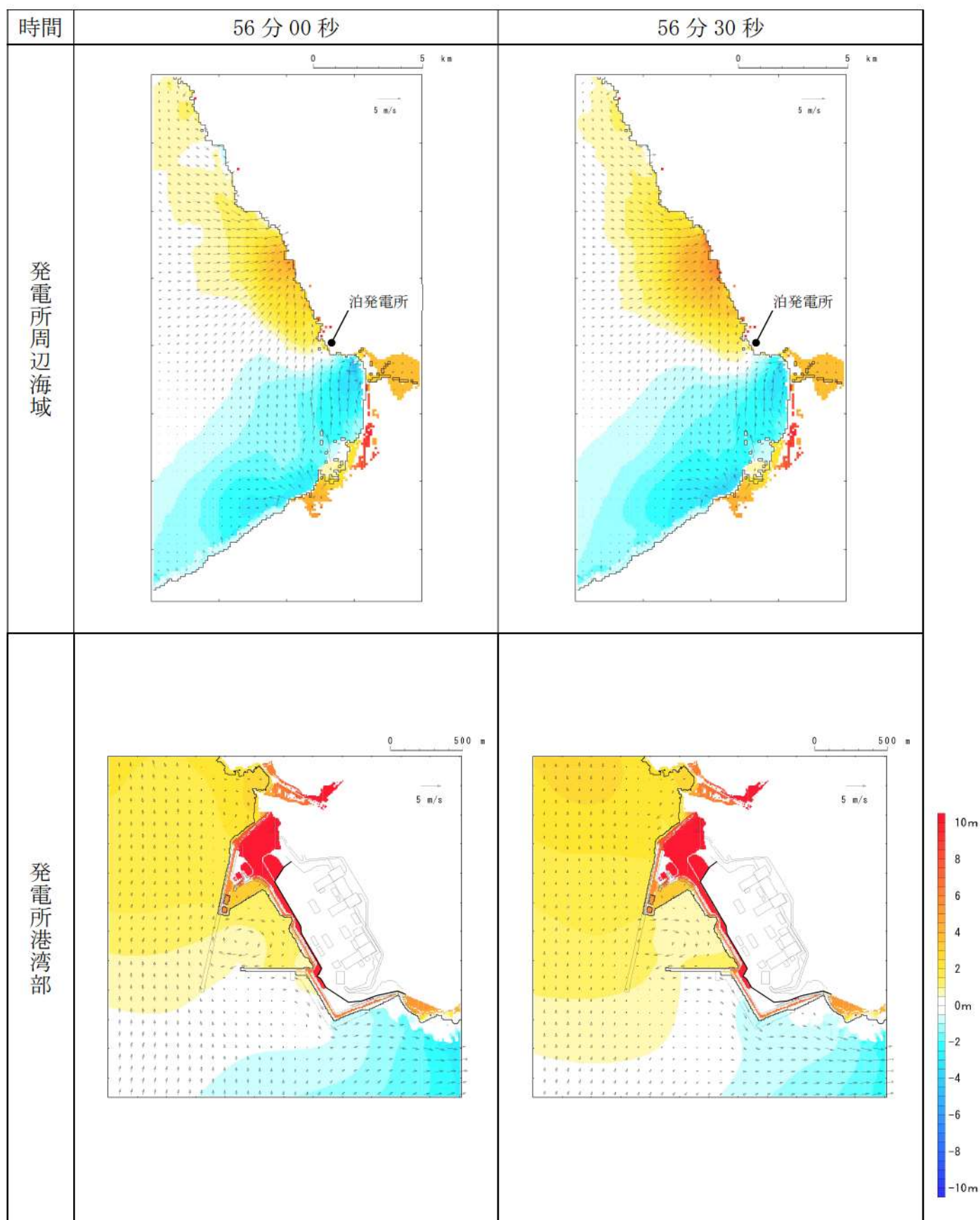
第 8 図-49 基準津波 D（北防波堤損傷）の水位変動・流向ベクトル(49/53)
