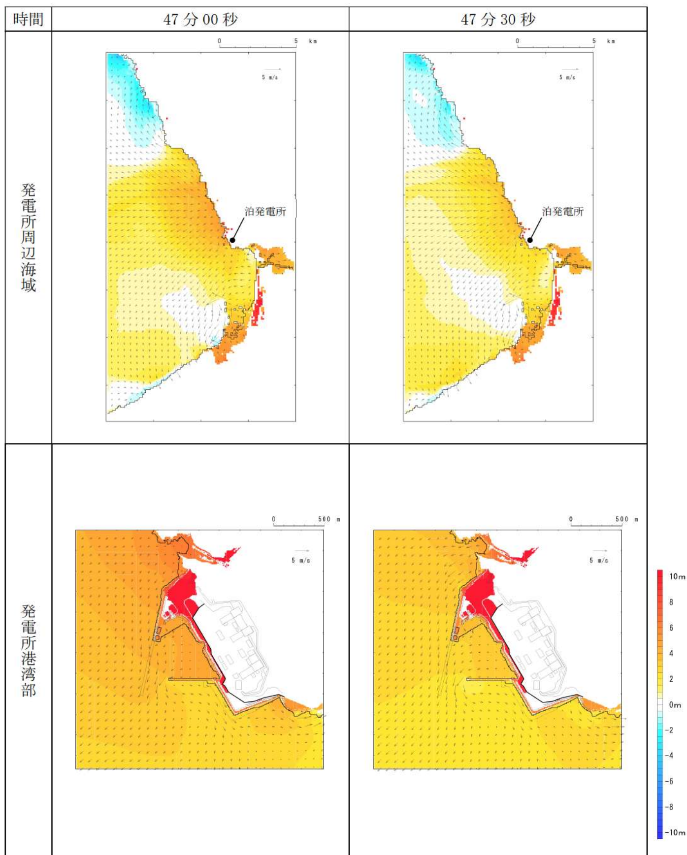
第 8 図-40 基準津波 D（北防波堤損傷）の水位変動・流向ベクトル(40/53)
