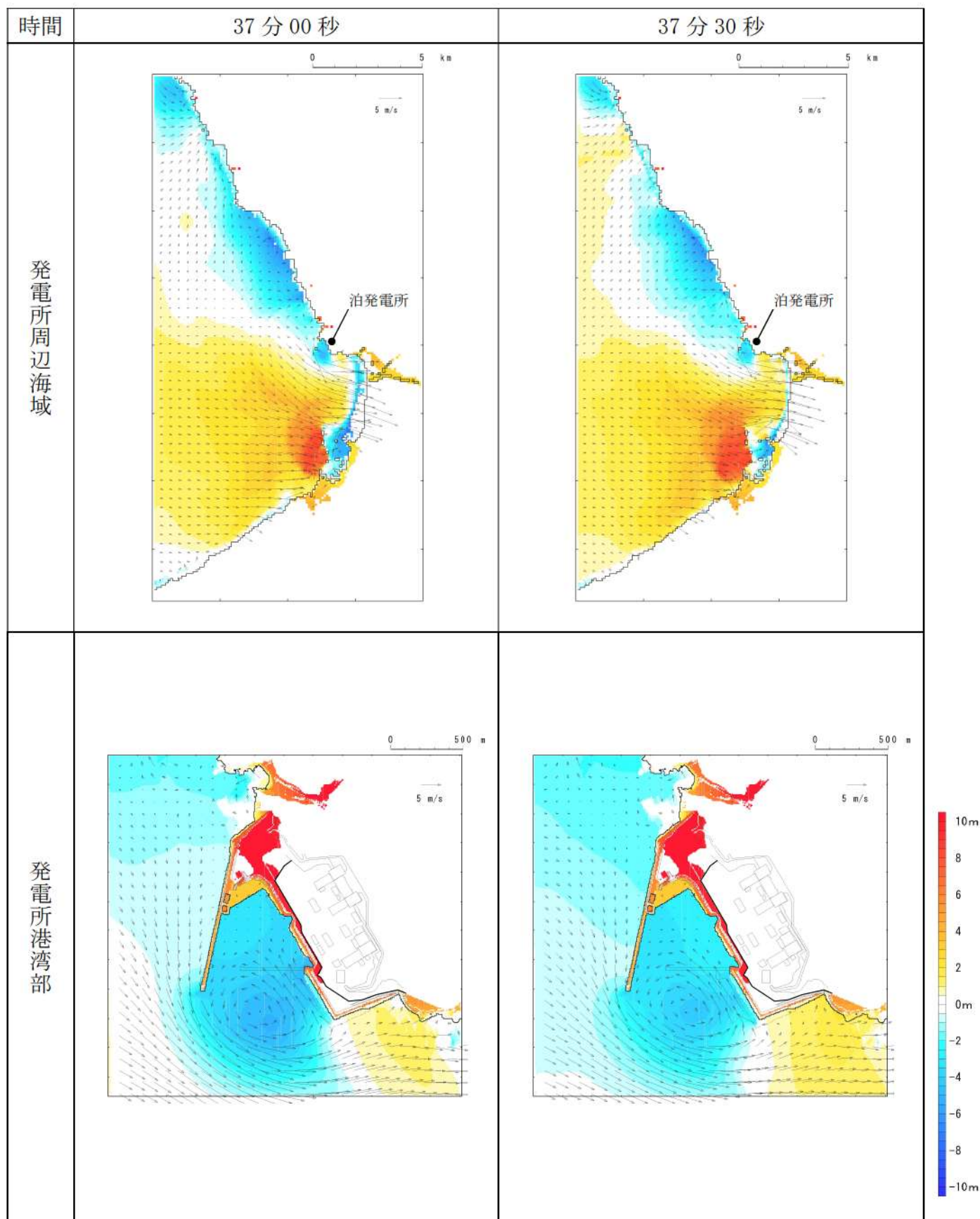
第 7 図-30 基準津波 D (南防波堤損傷) の水位変動・流向ベクトル (30/53)
