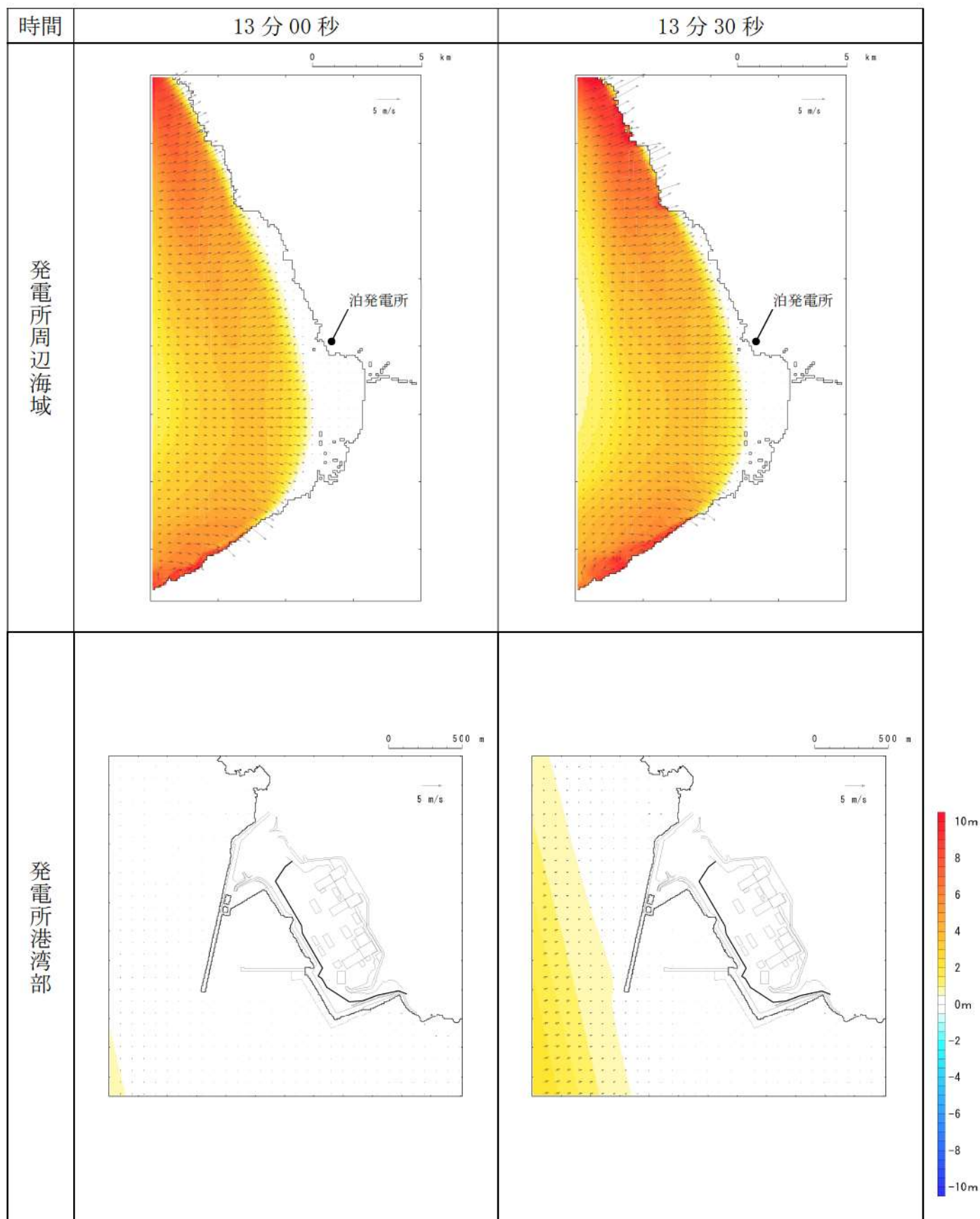
第 10 図-6 基準津波 E（南防波堤損傷）の水位変動・流向ベクトル (6/53)
