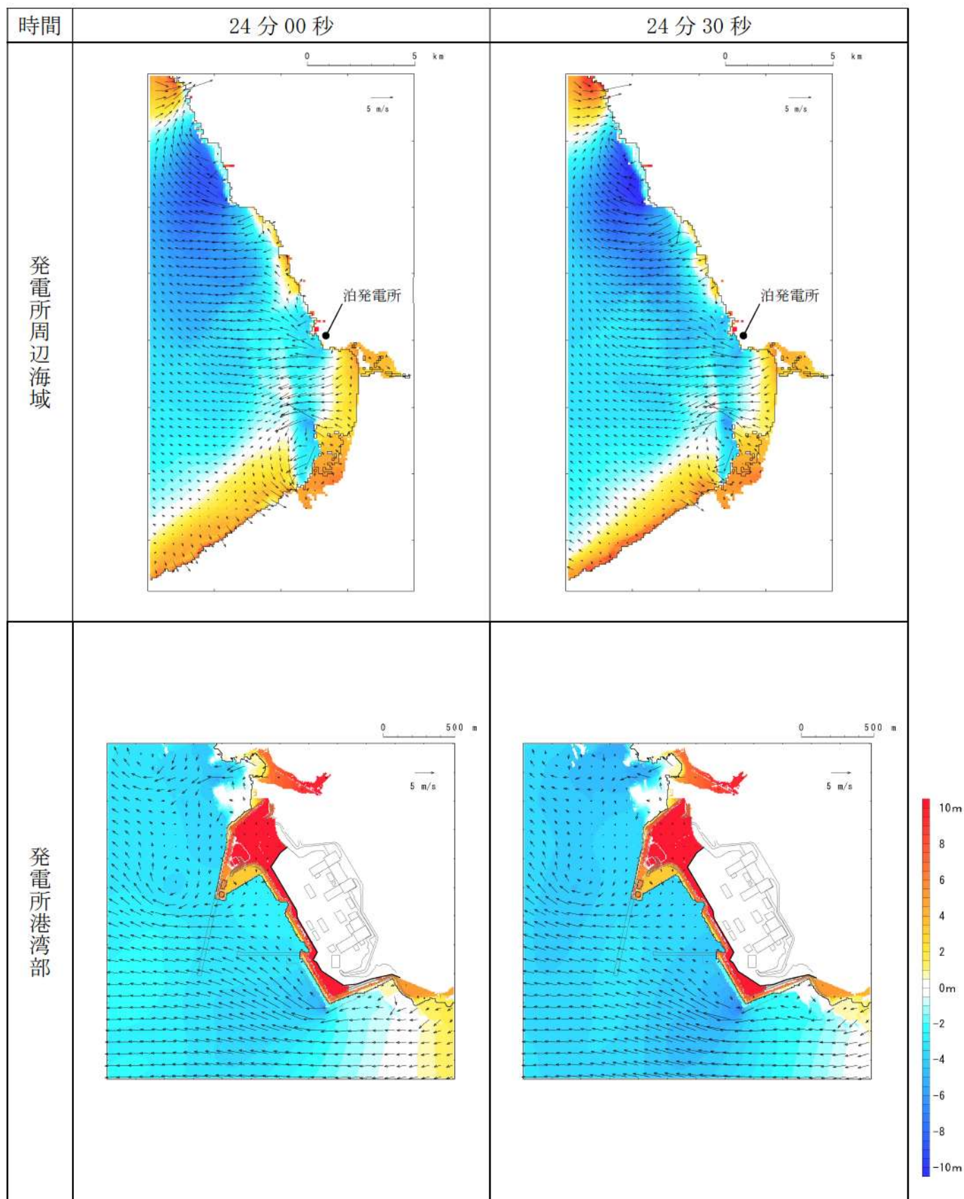
第 9 図-17 基準津波 E（北及び南防波堤損傷）の水位変動・流向ベクトル(17/53)
