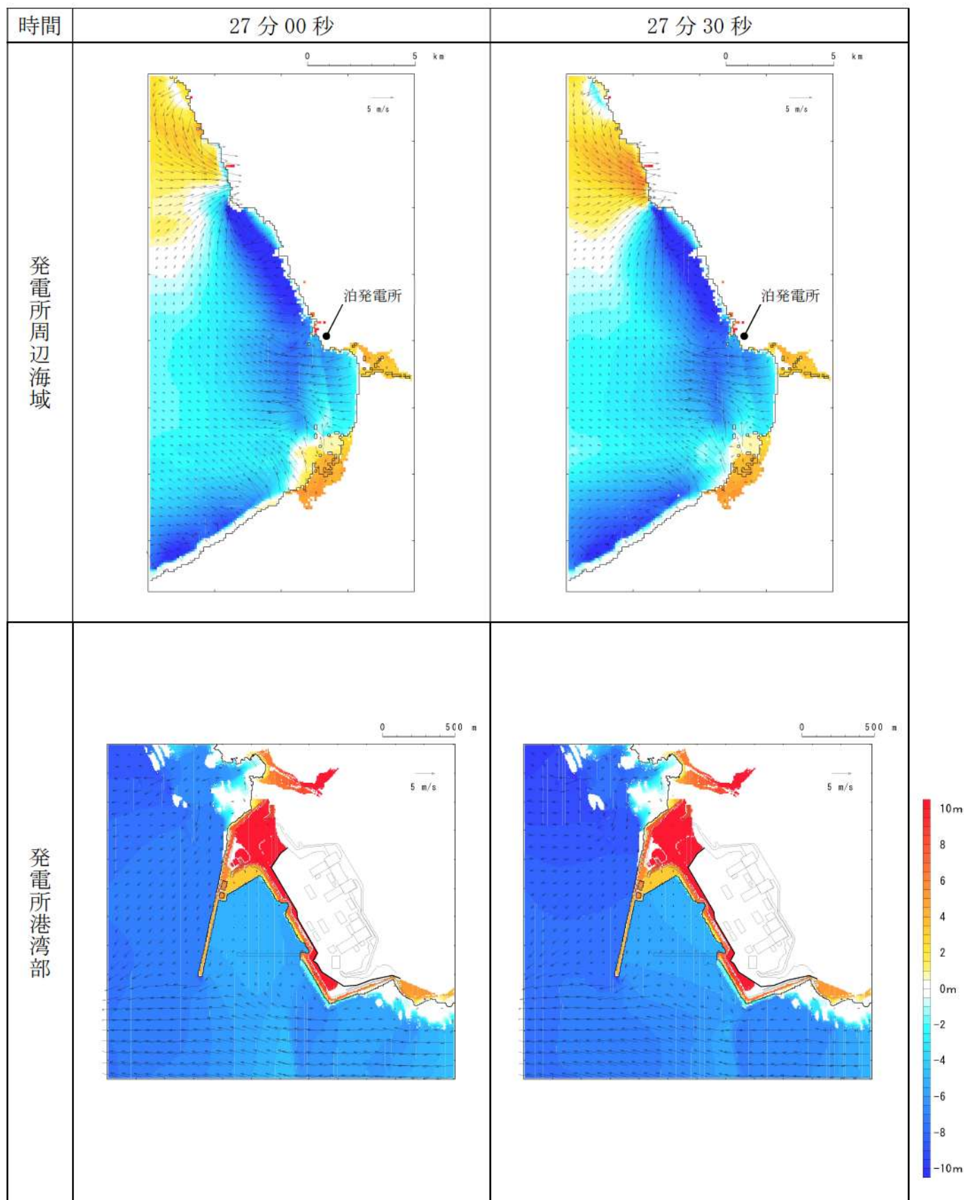
第 10 図-20 基準津波 E（南防波堤損傷）の水位変動・流向ベクトル (20/53)
