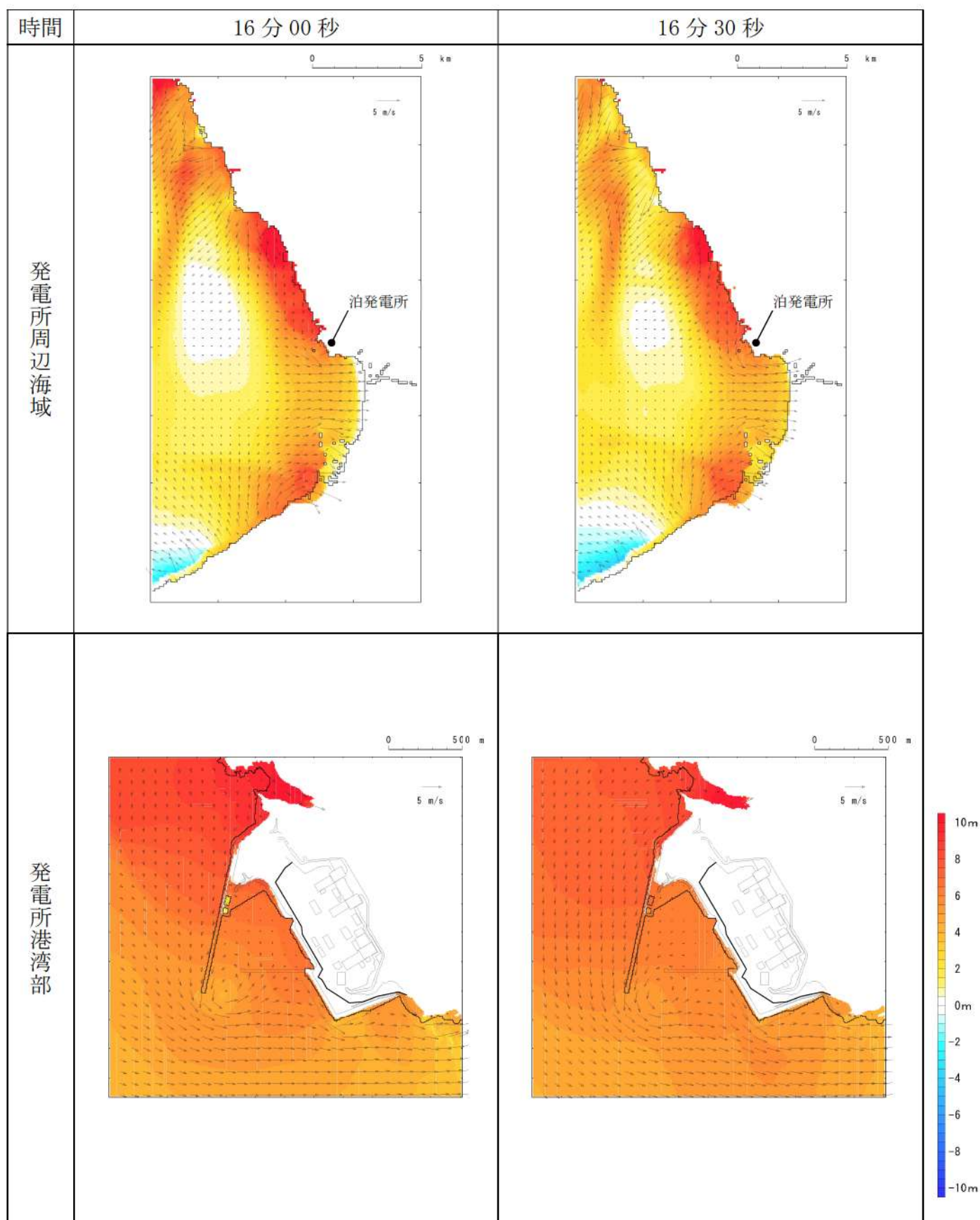
第 10 図-9 基準津波 E（南防波堤損傷）の水位変動・流向ベクトル (9/53)
