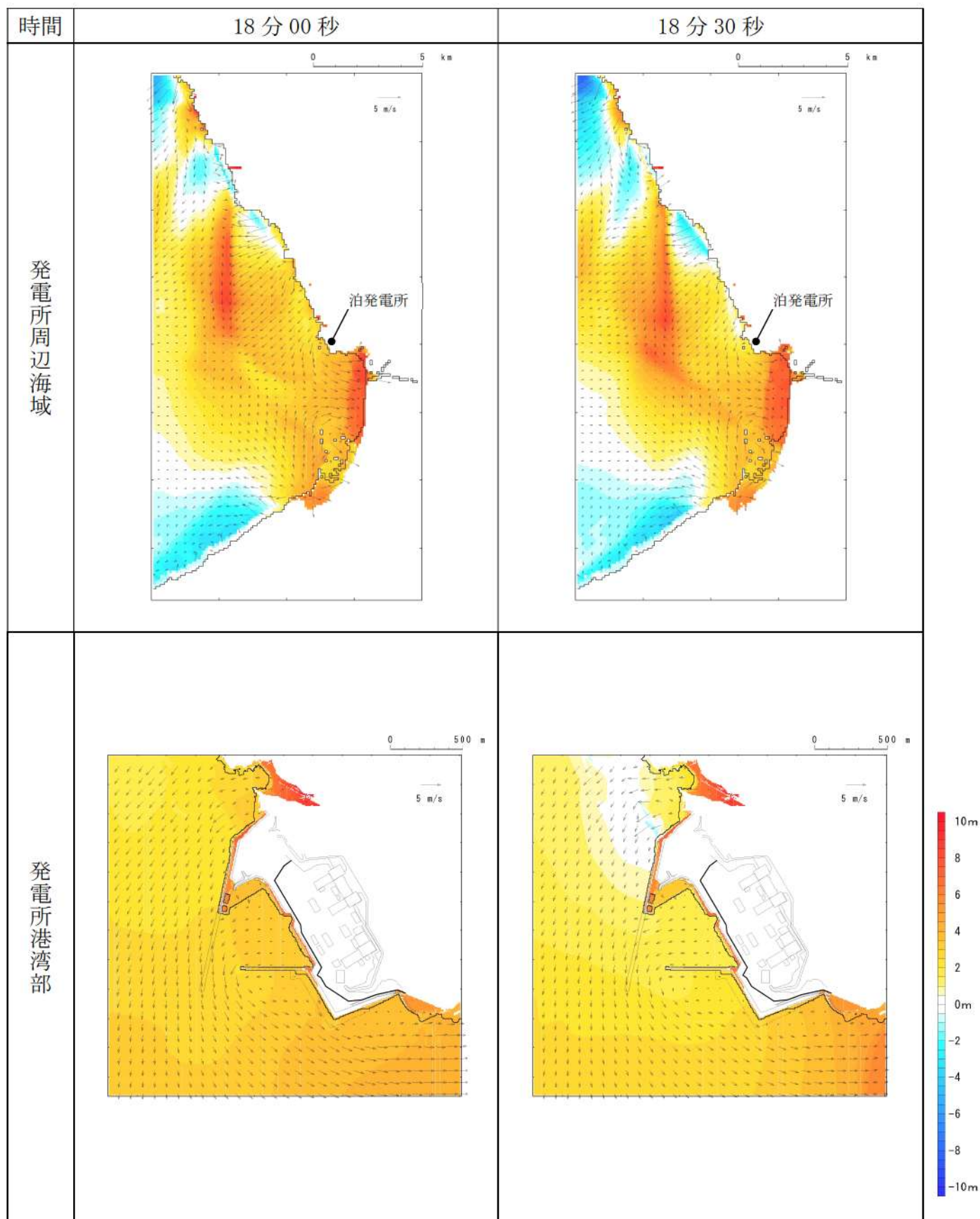
第 8 図-11 基準津波 D（北防波堤損傷）の水位変動・流向ベクトル(11/53)
