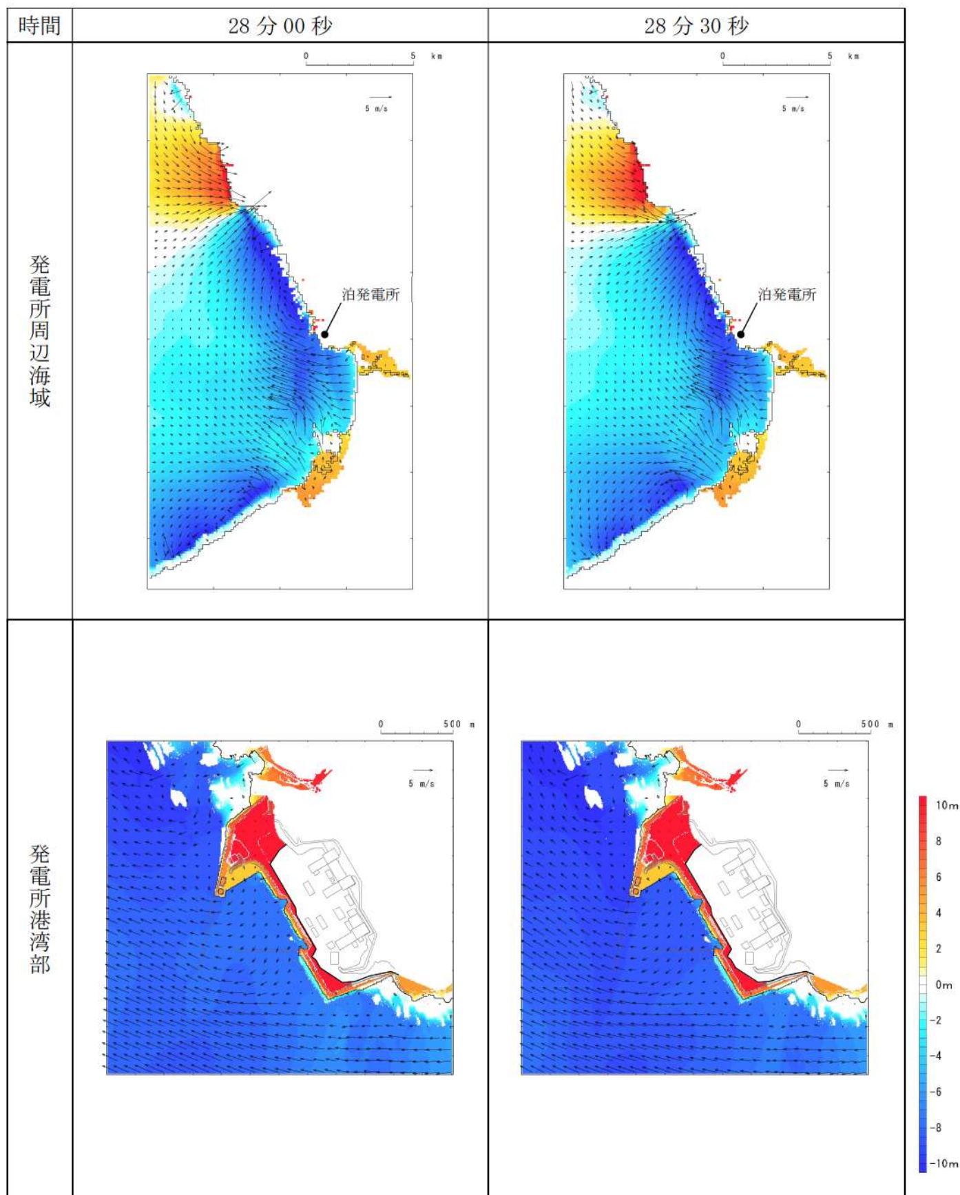
第9図-21 基準津波E（北及び南防波堤損傷）の水位変動・流向ベクトル(21/53)
