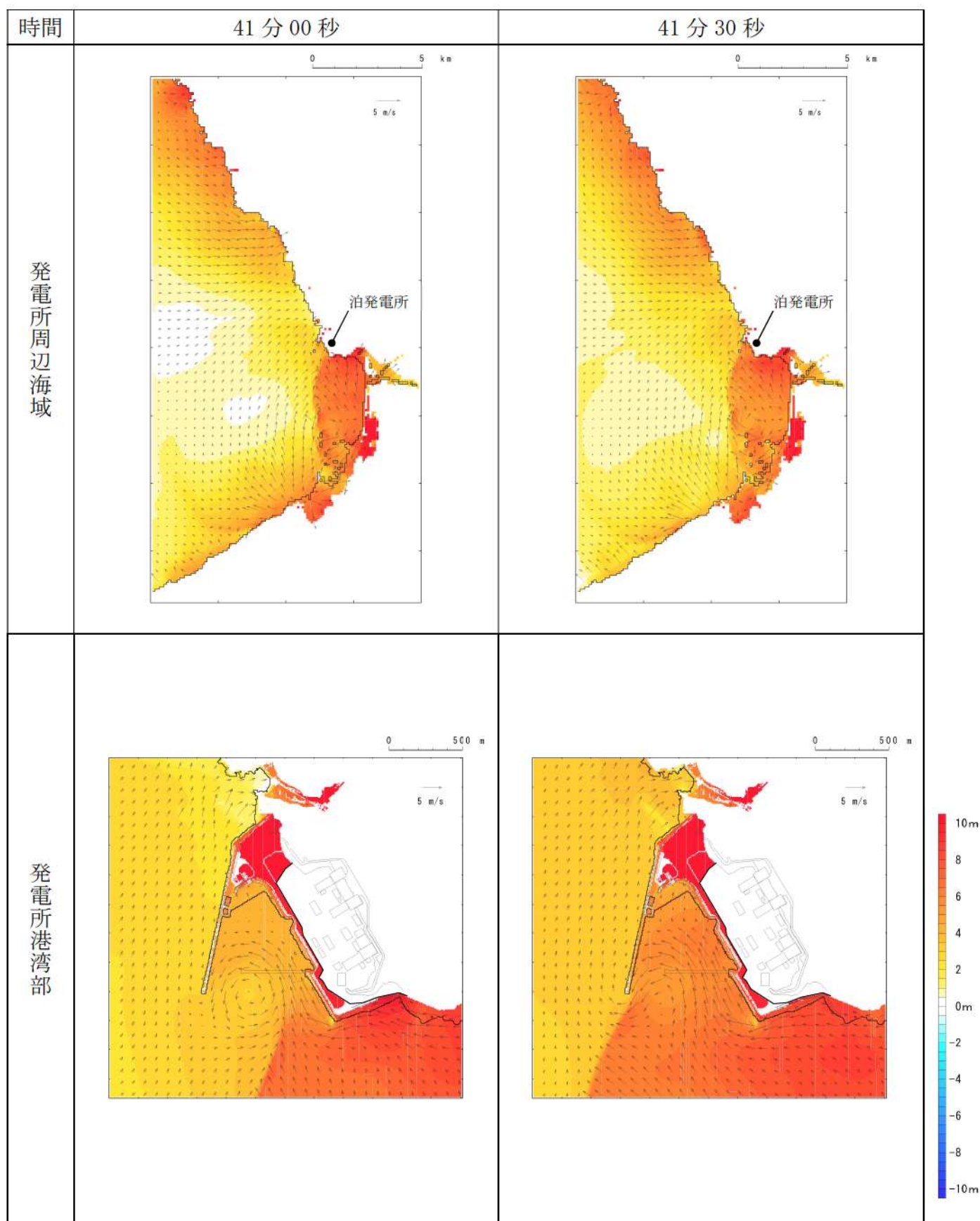
第 10 図-34 基準津波 E（南防波堤損傷）の水位変動・流向ベクトル(34/53)
