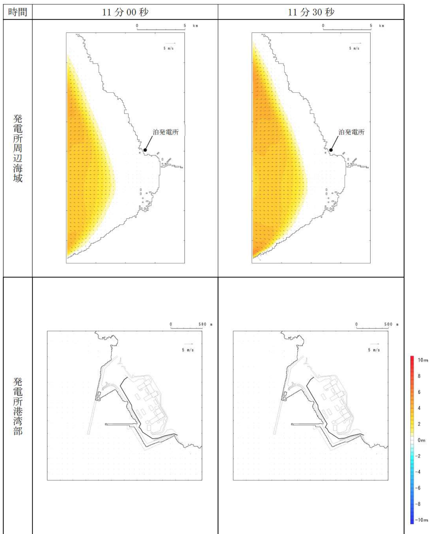
第8図-4 基準津波D（北防波堤損傷）の水位変動・流向ベクトル(4/53)
