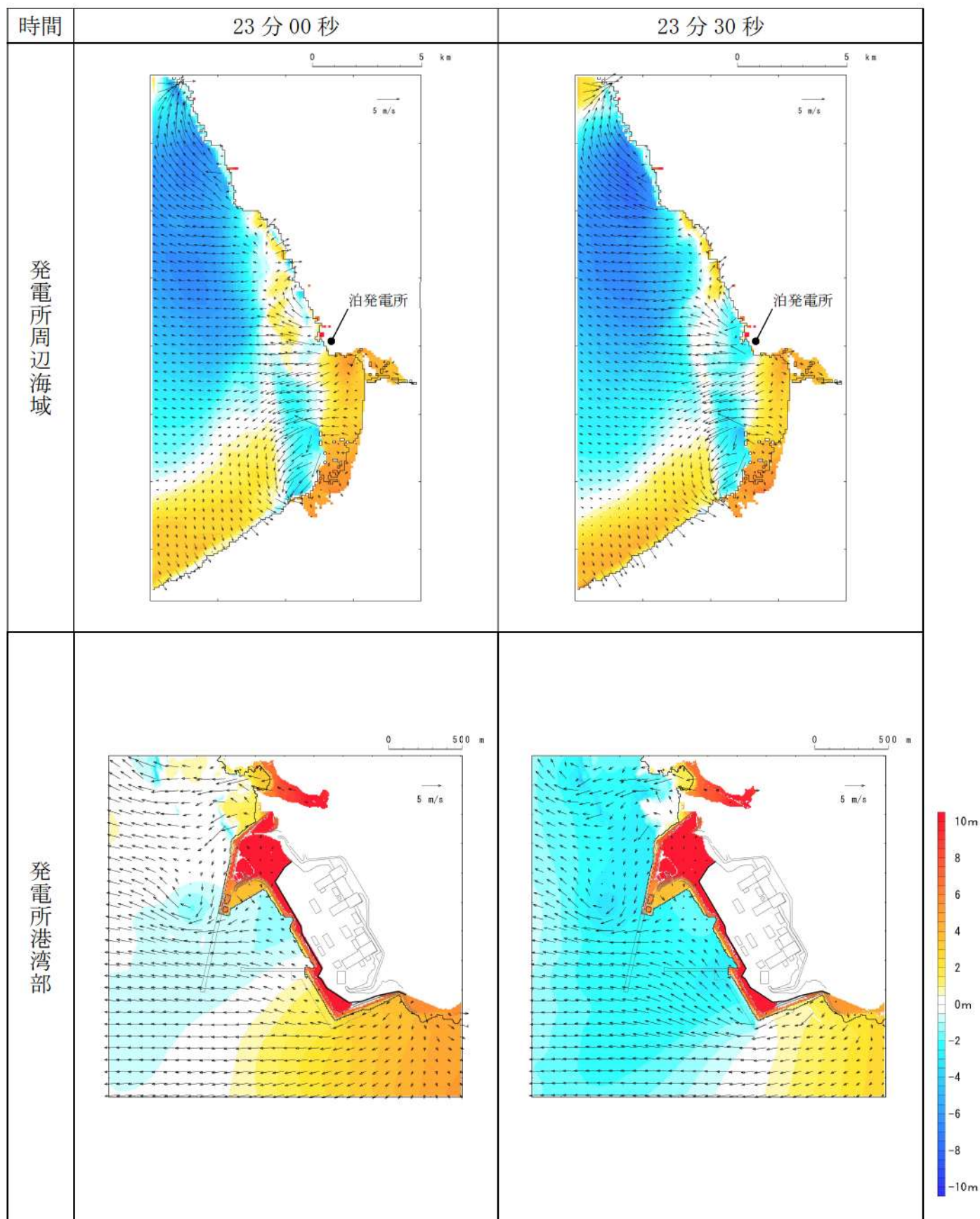
第 9 図-16 基準津波 E（北及び南防波堤損傷）の水位変動・流向ベクトル(16/53)
