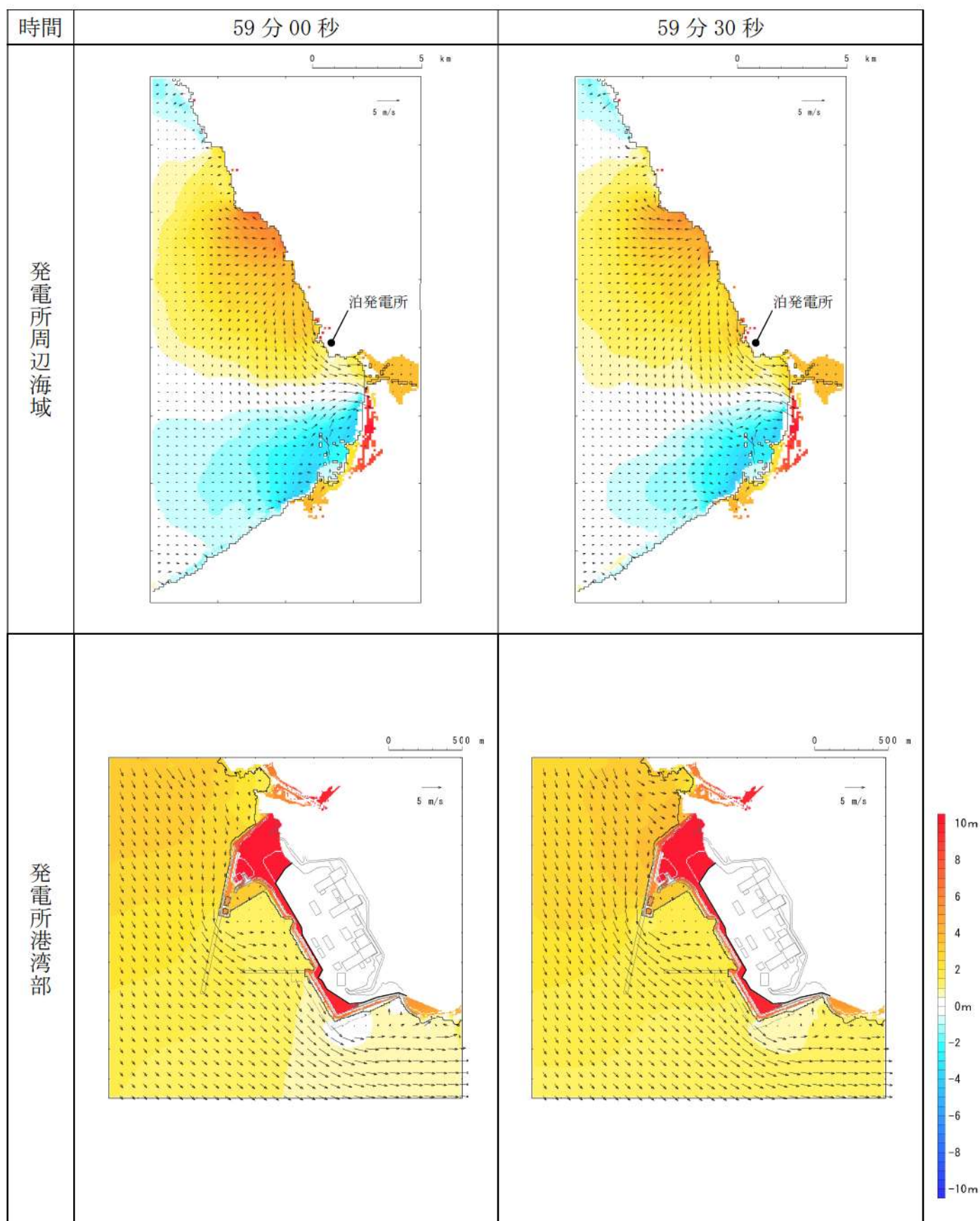
第 9 図-52 基準津波 E（北及び南防波堤損傷）の水位変動・流向ベクトル(52/53)
