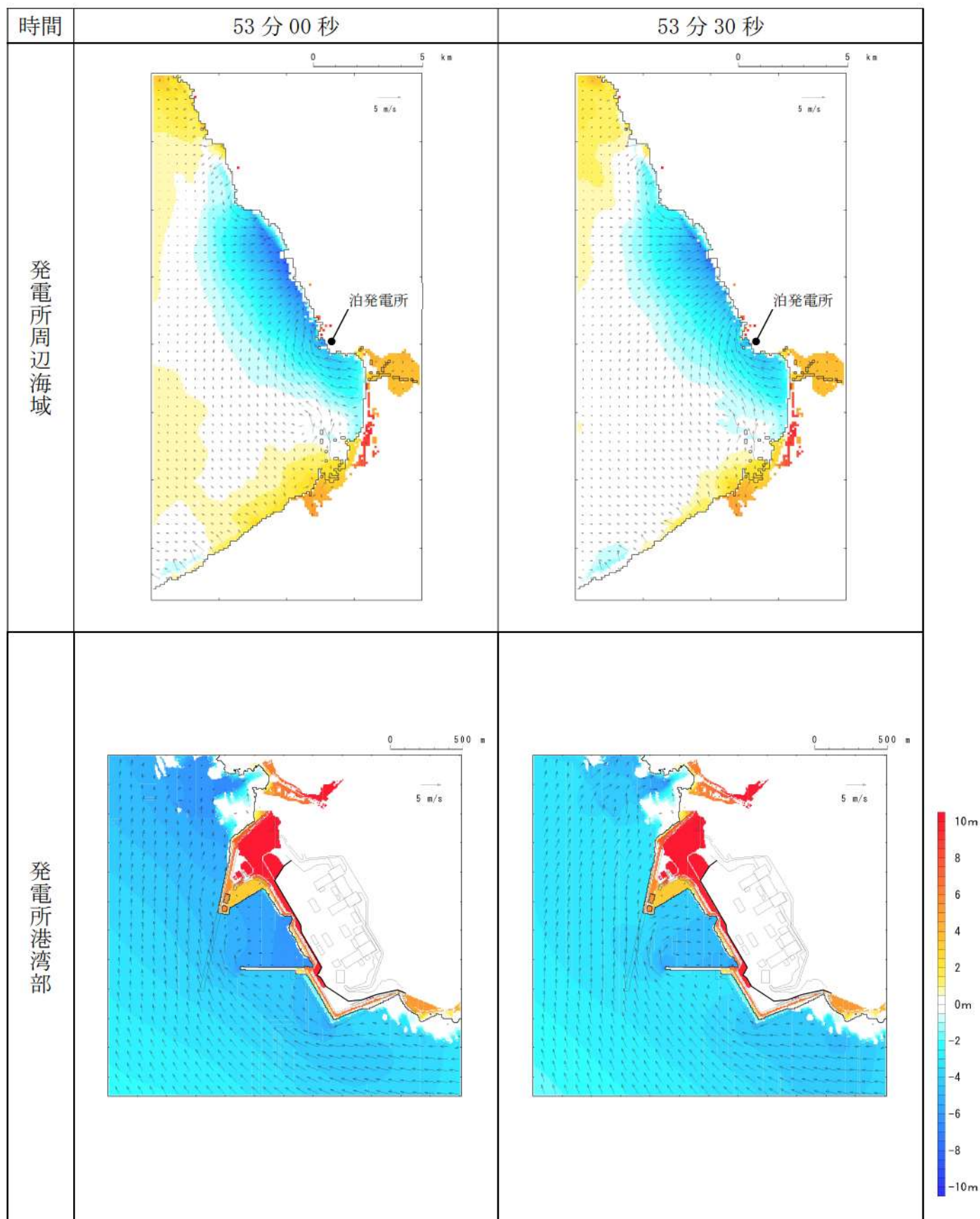
第 8 図-46 基準津波 D（北防波堤損傷）の水位変動・流向ベクトル(46/53)
