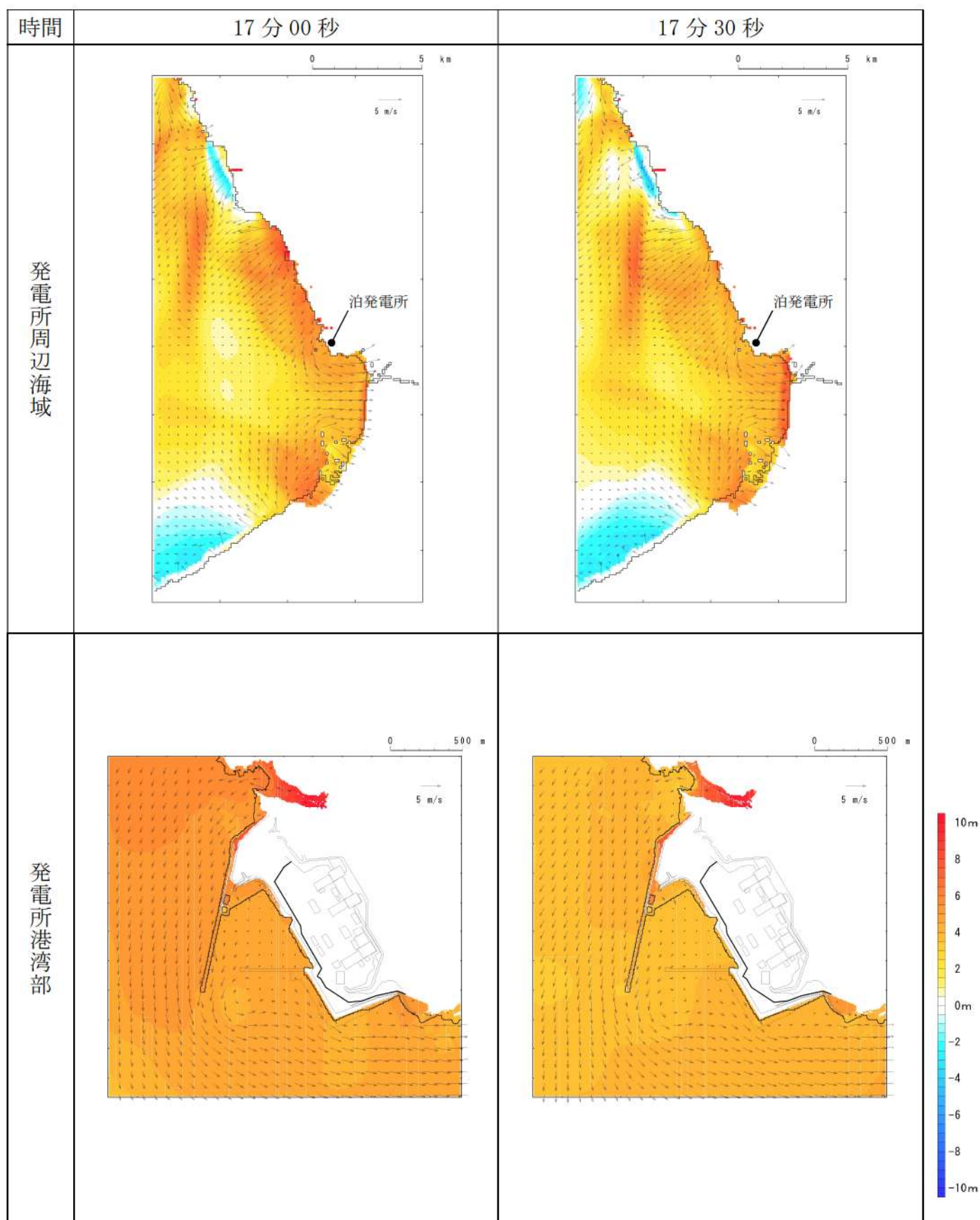
第 7 図-10 基準津波 D（南防波堤損傷）の水位変動・流向ベクトル(10/53)
