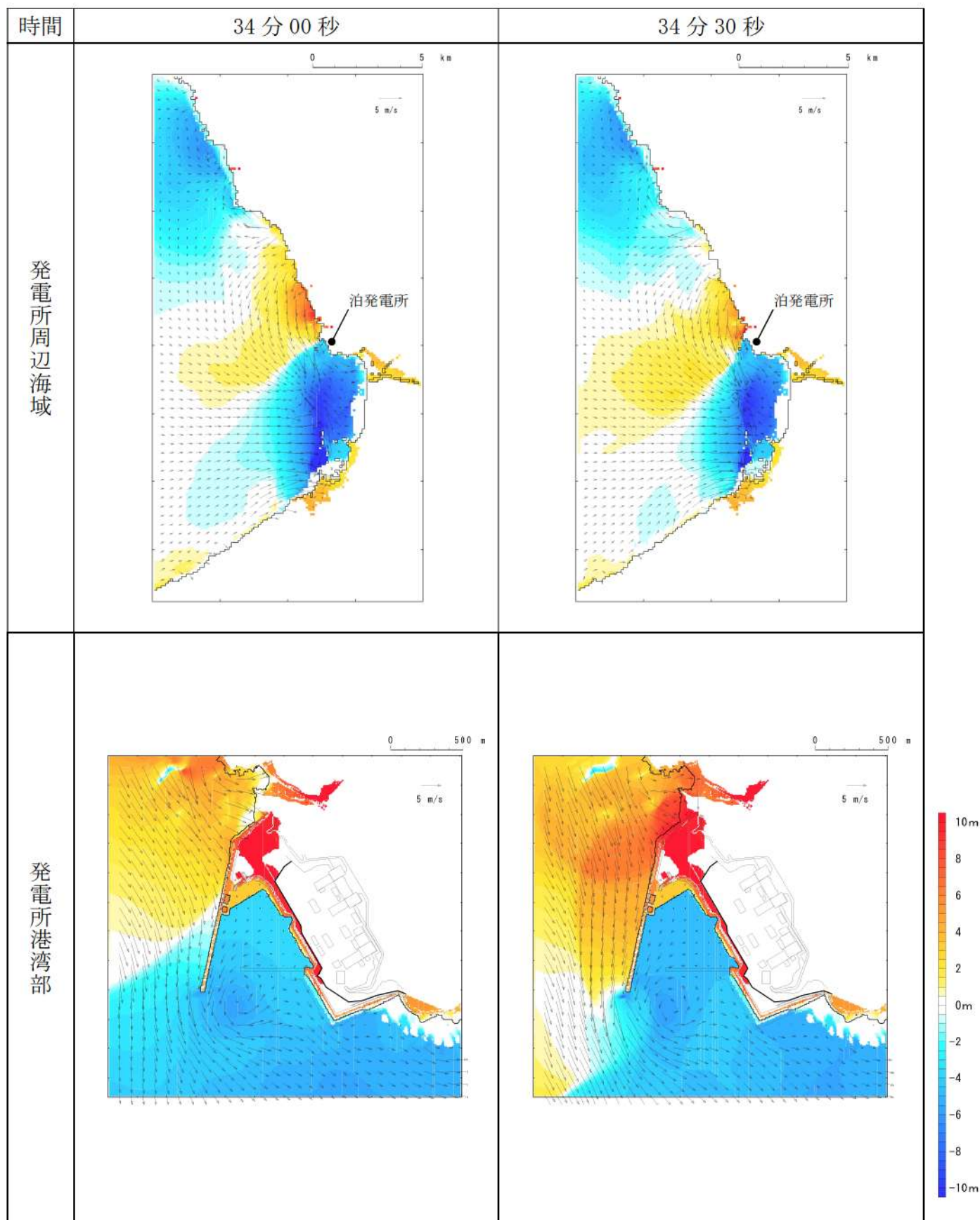
第7図-27 基準津波D（南防波堤損傷）の水位変動・流向ベクトル(27/53)
