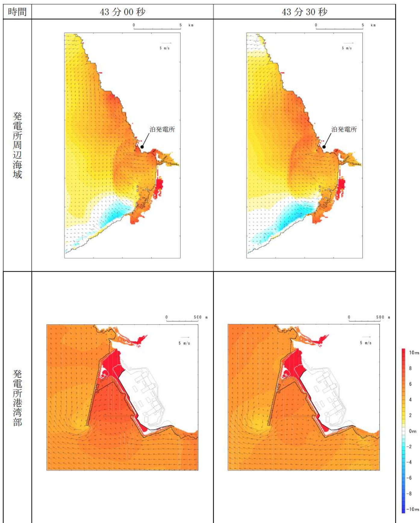
第 10 図-36 基準津波 E（南防波堤損傷）の水位変動・流向ベクトル(36/53)
