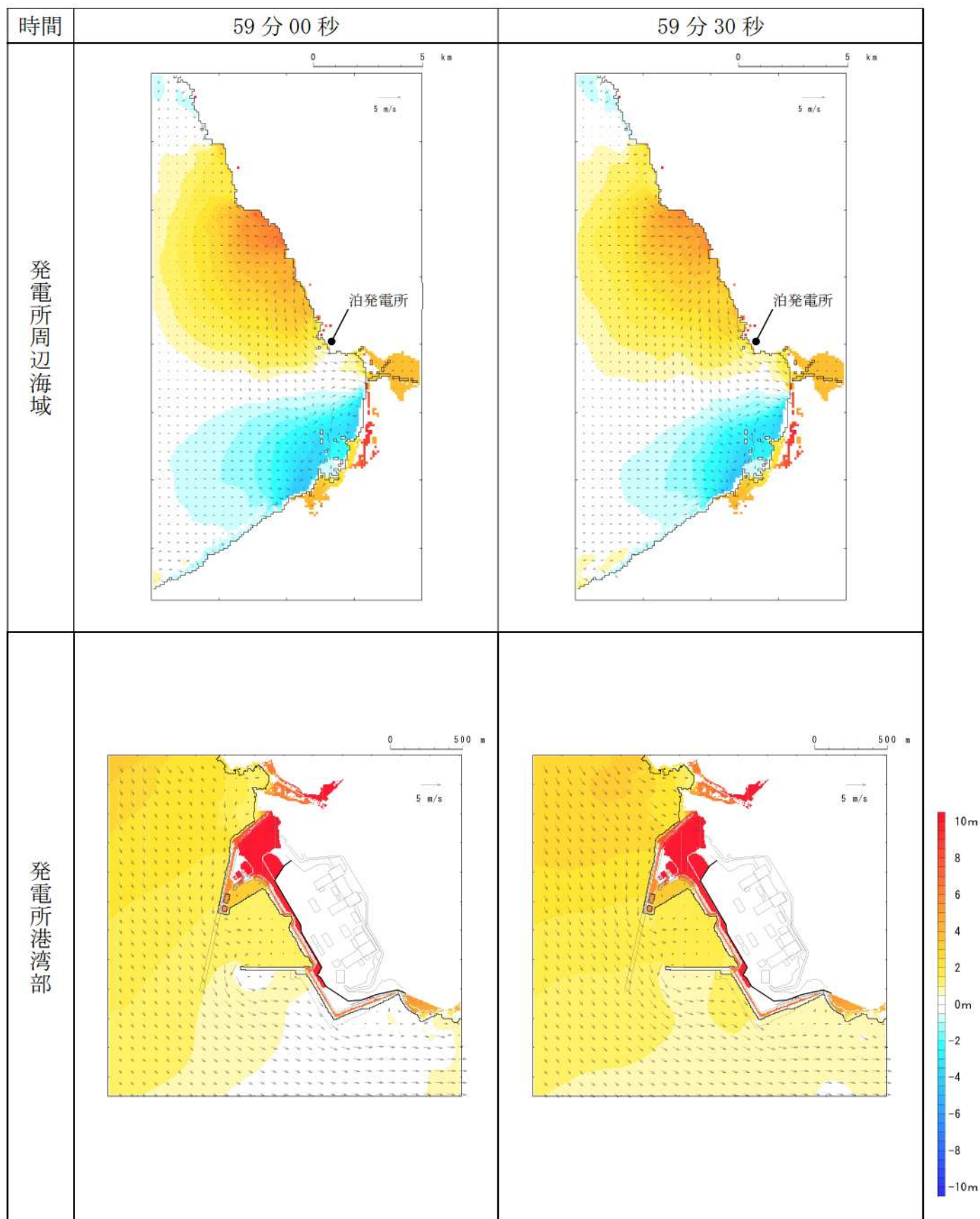
第 8 図-52 基準津波 D（北防波堤損傷）の水位変動・流向ベクトル (52/53)
