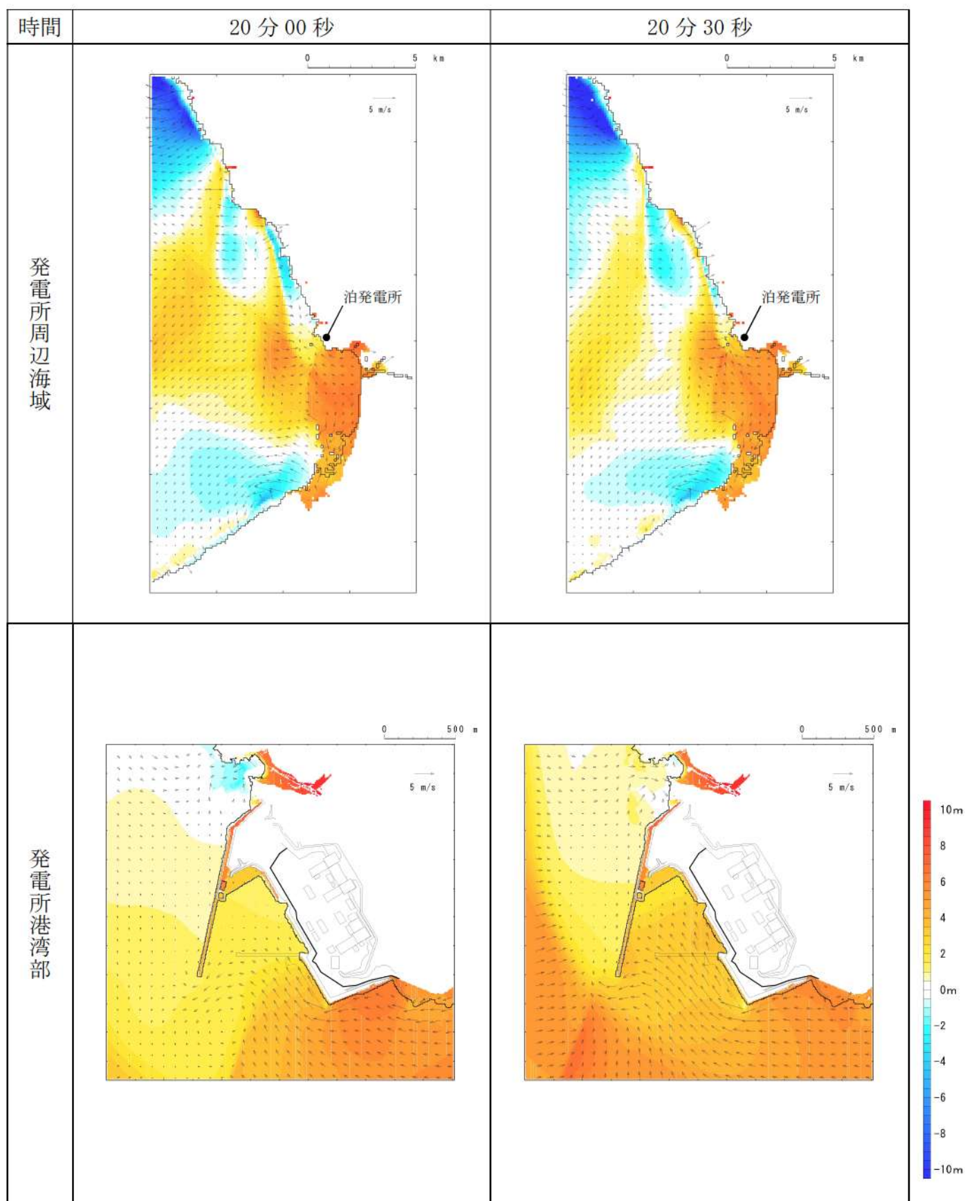
第 7 図-13 基準津波 D（南防波堤損傷）の水位変動・流向ベクトル(13/53)
