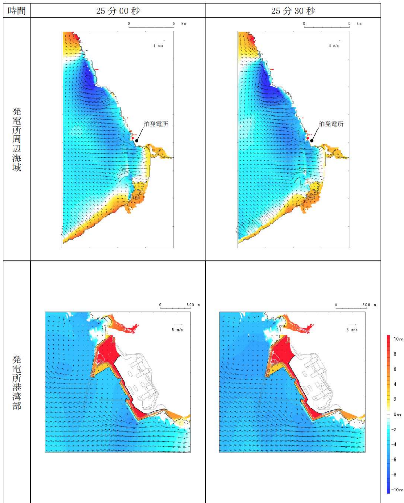
第 9 図-18 基準津波 E（北及び南防波堤損傷）の水位変動・流向ベクトル(18/53)
