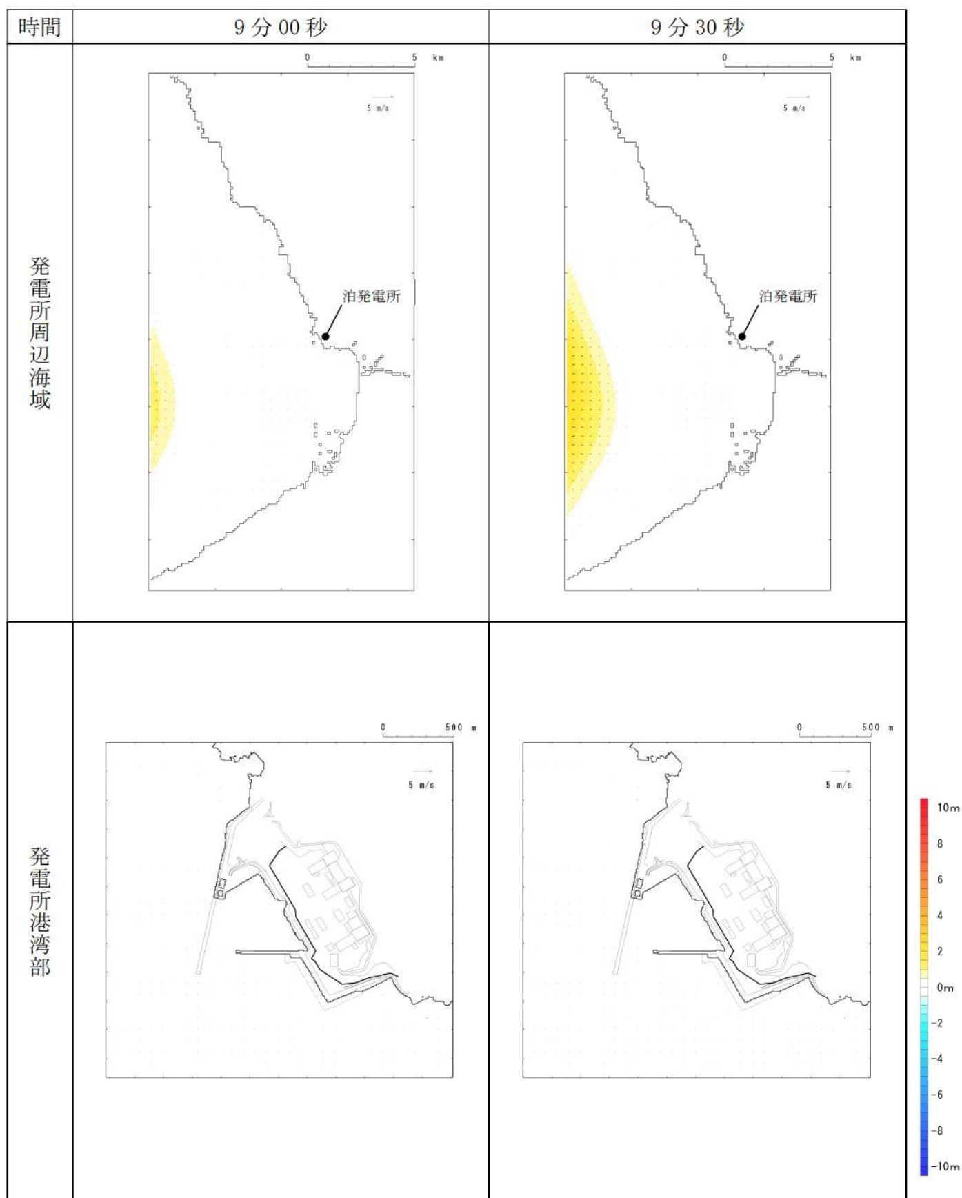
第 8 図- 2 基準津波 D（北防波堤損傷）の水位変動・流向ベクトル (2/53)
