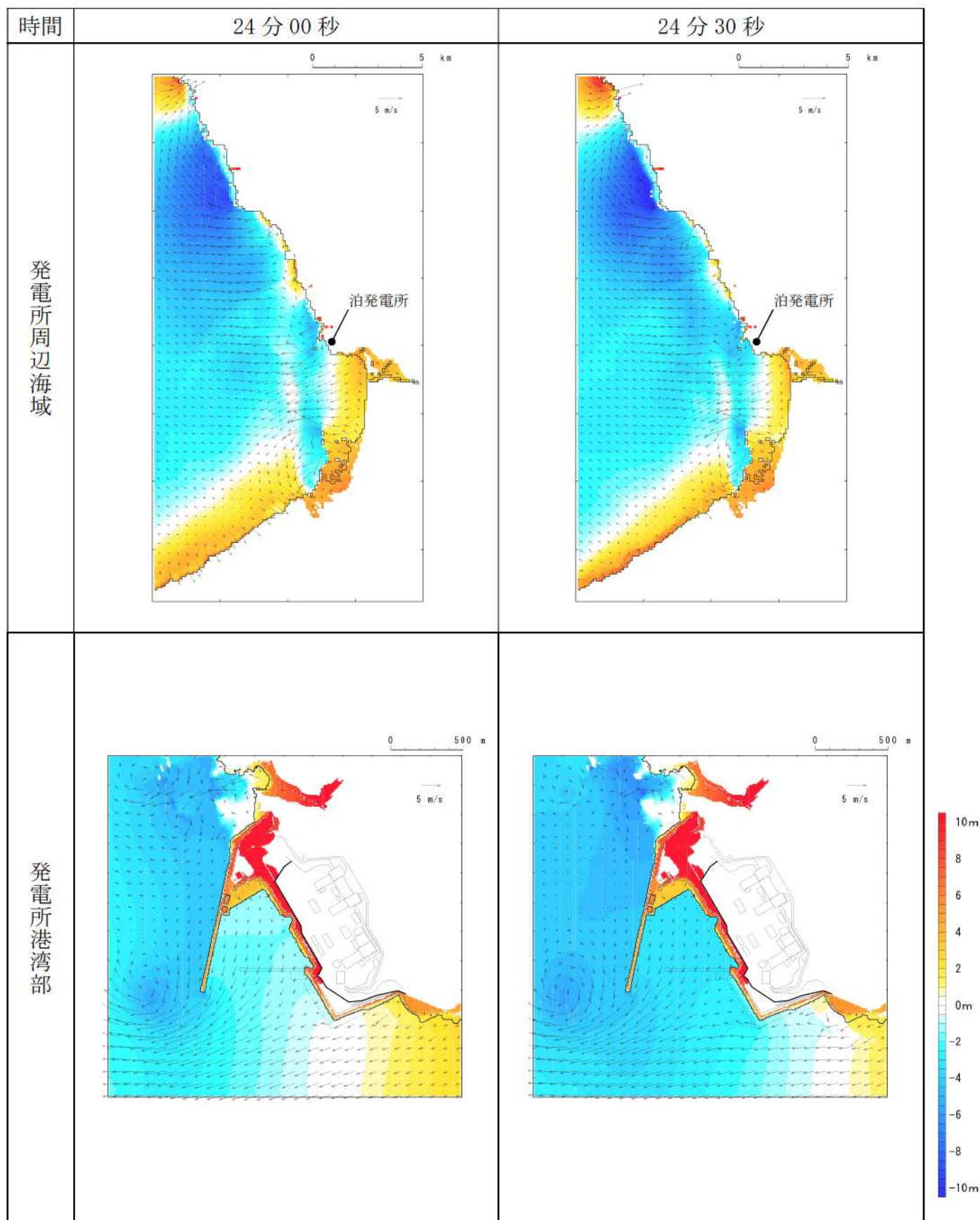
第7図-17 基準津波D（南防波堤損傷）の水位変動・流向ベクトル(17/53)
