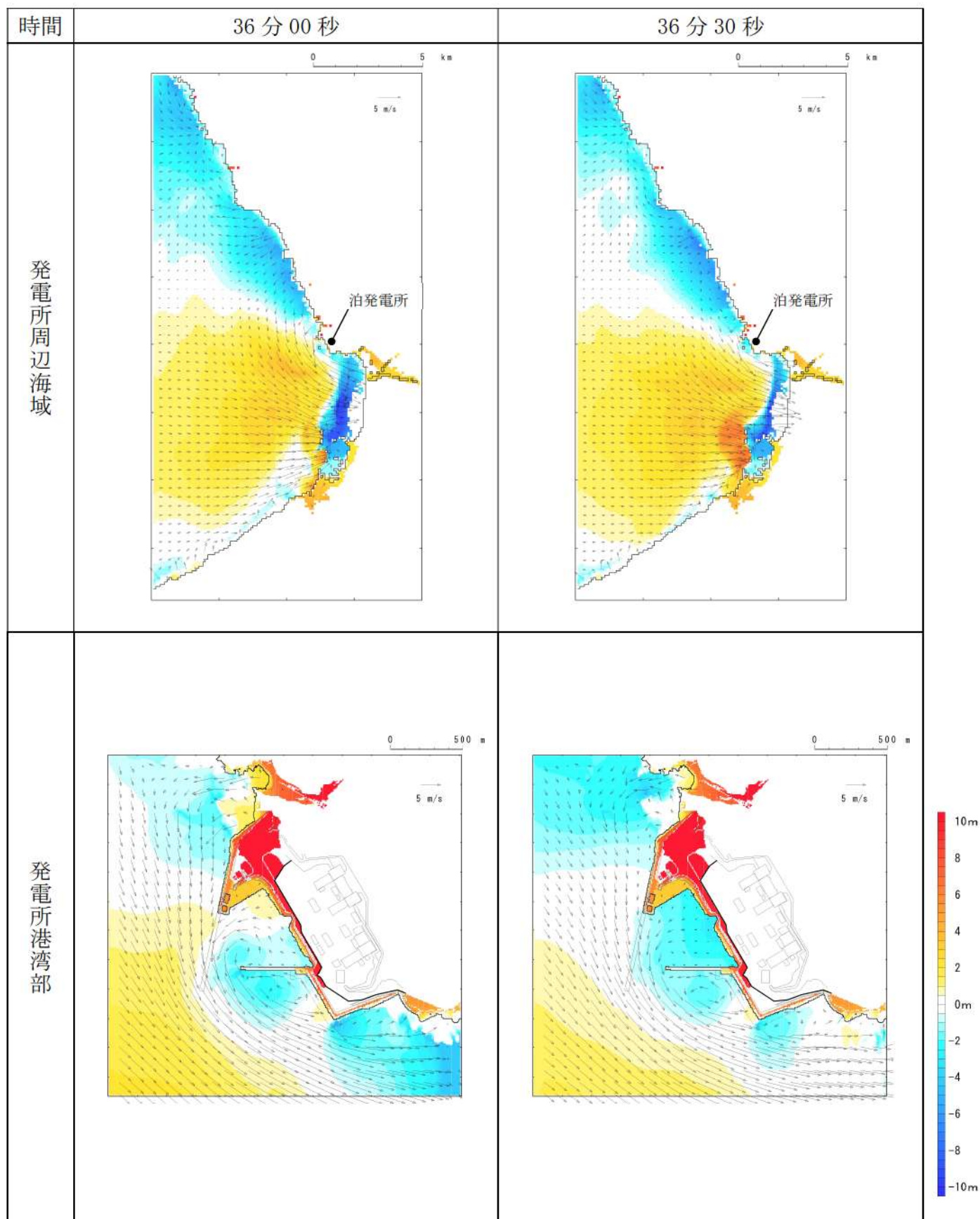
第 8 図-29 基準津波 D（北防波堤損傷）の水位変動・流向ベクトル (29/53)
