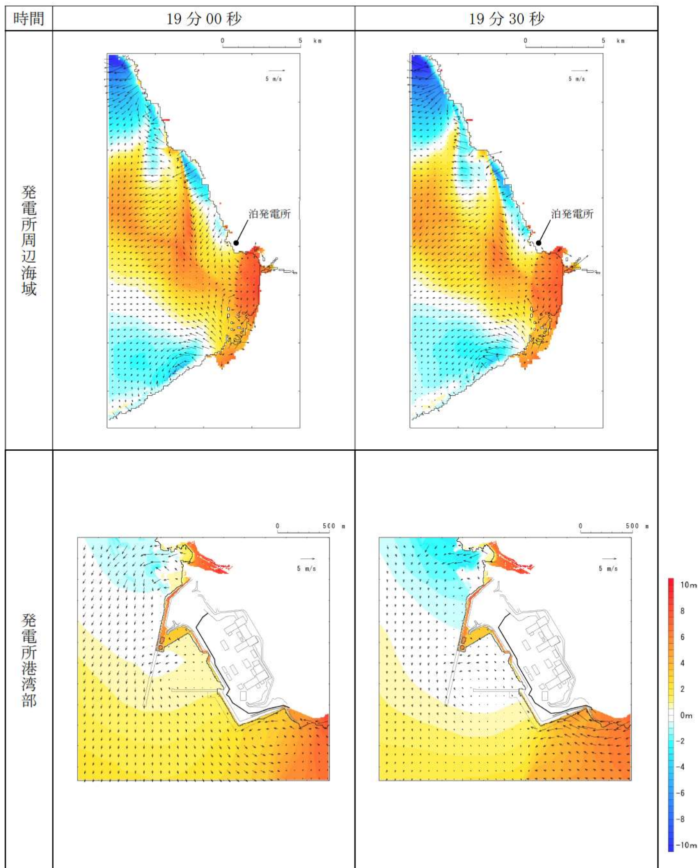
第 9 図-12 基準津波 E（北及び南防波堤損傷）の水位変動・流向ベクトル(12/53)
