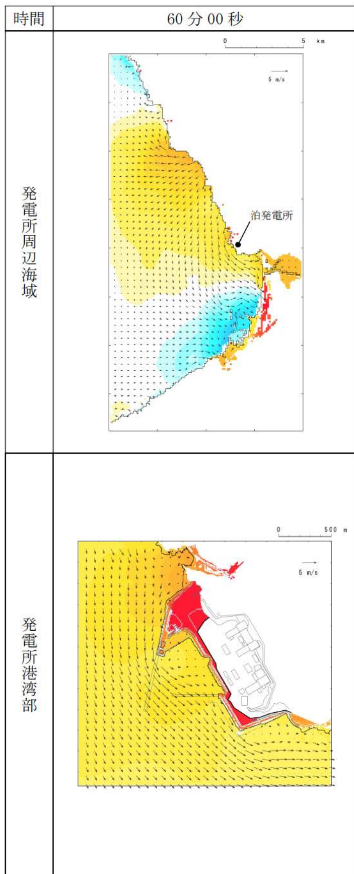
第9図-53 基準津波E（北及び南防波堤損傷）の水位変動・流向ベクトル(53/53)
