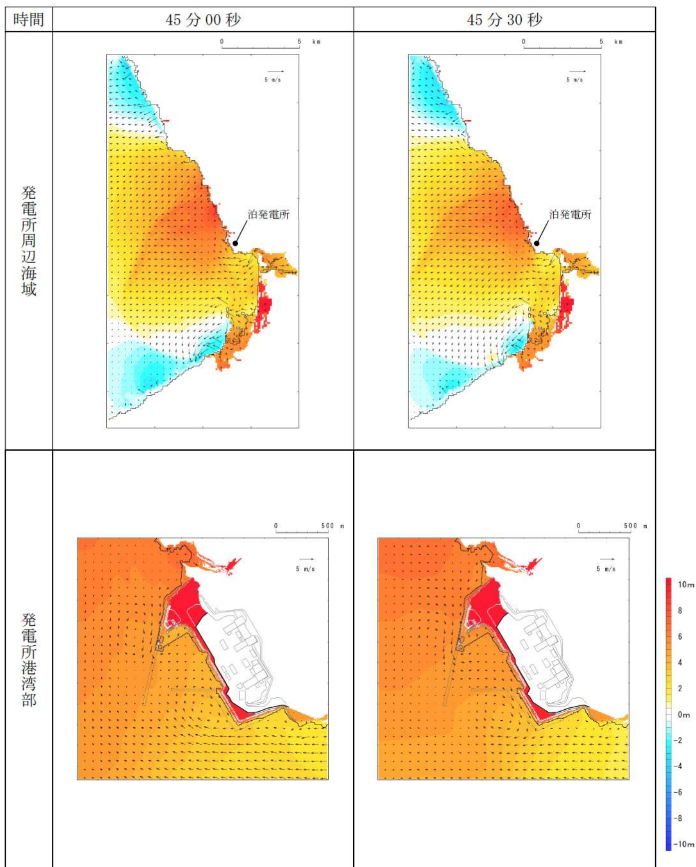
第 9 図-38 基準津波 E（北及び南防波堤損傷）の水位変動・流向ベクトル(38/53)
