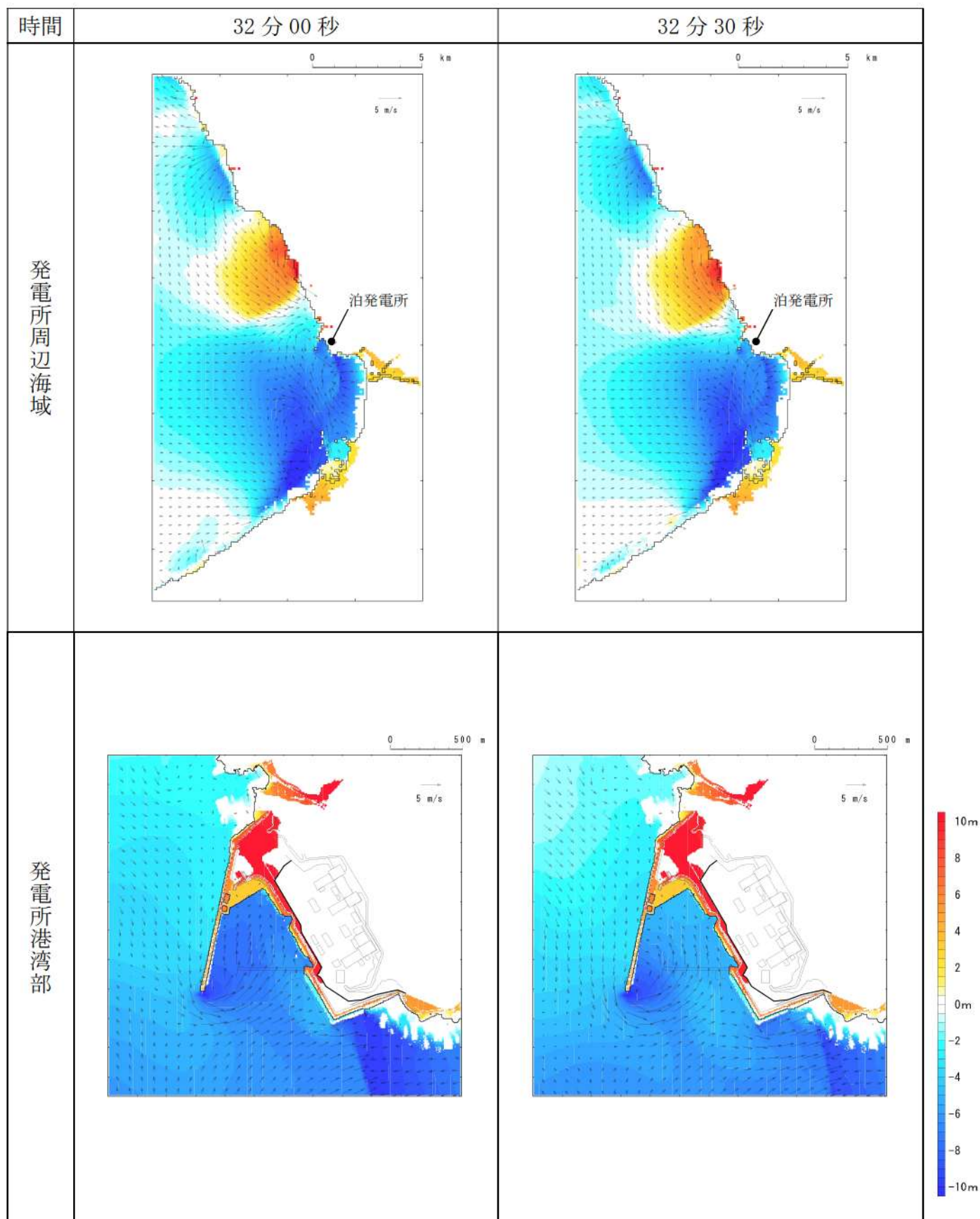
第 7 図-25 基準津波 D（南防波堤損傷）の水位変動・流向ベクトル (25/53)
