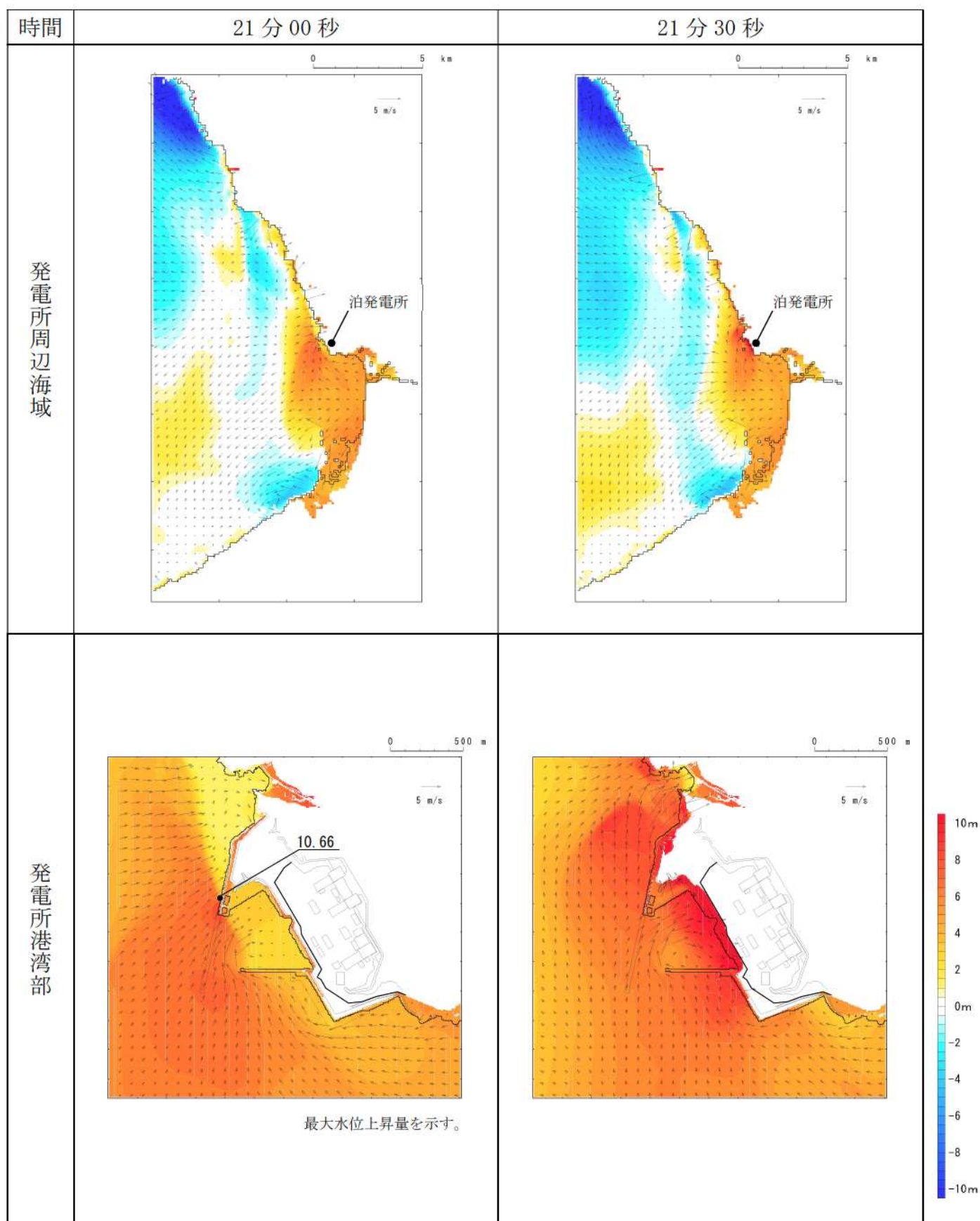
第 8 図-14 基準津波 D（北防波堤損傷）の水位変動・流向ベクトル(14/53)
