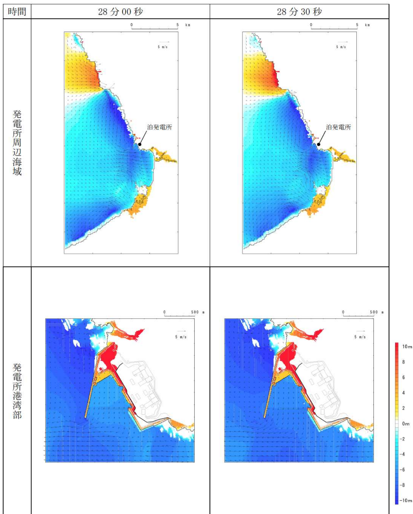
第7図-21 基準津波D（南防波堤損傷）の水位変動・流向ベクトル(21/53)
