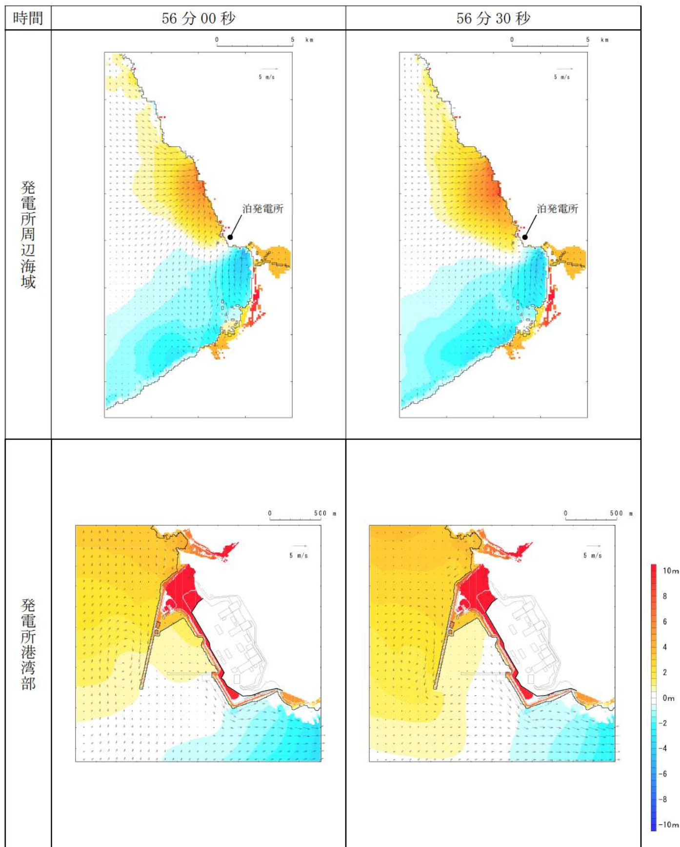
第 10 図-49 基準津波 E（南防波堤損傷）の水位変動・流向ベクトル(49/53)
