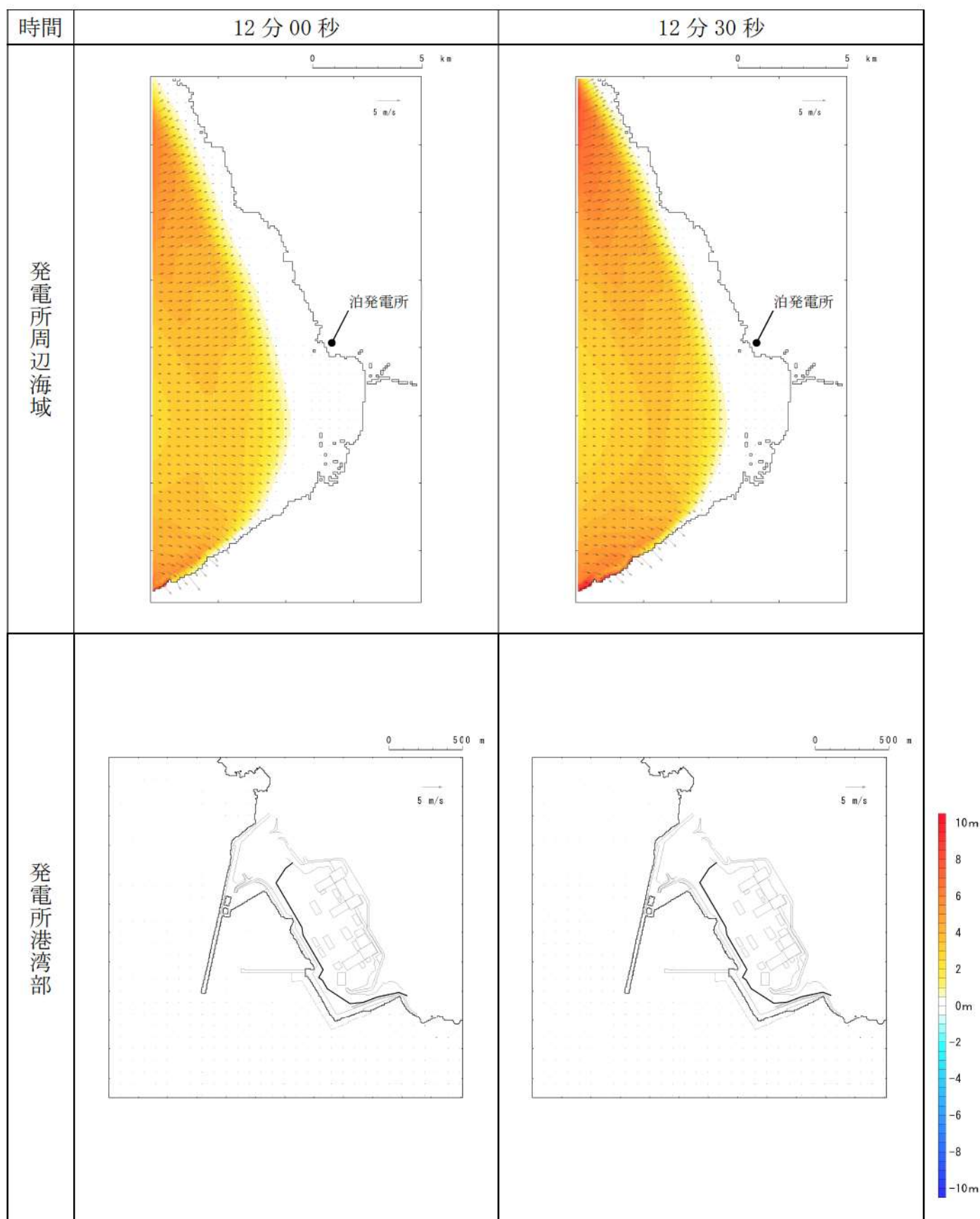
第 10 図-5 基準津波 E（南防波堤損傷）の水位変動・流向ベクトル (5/53)
