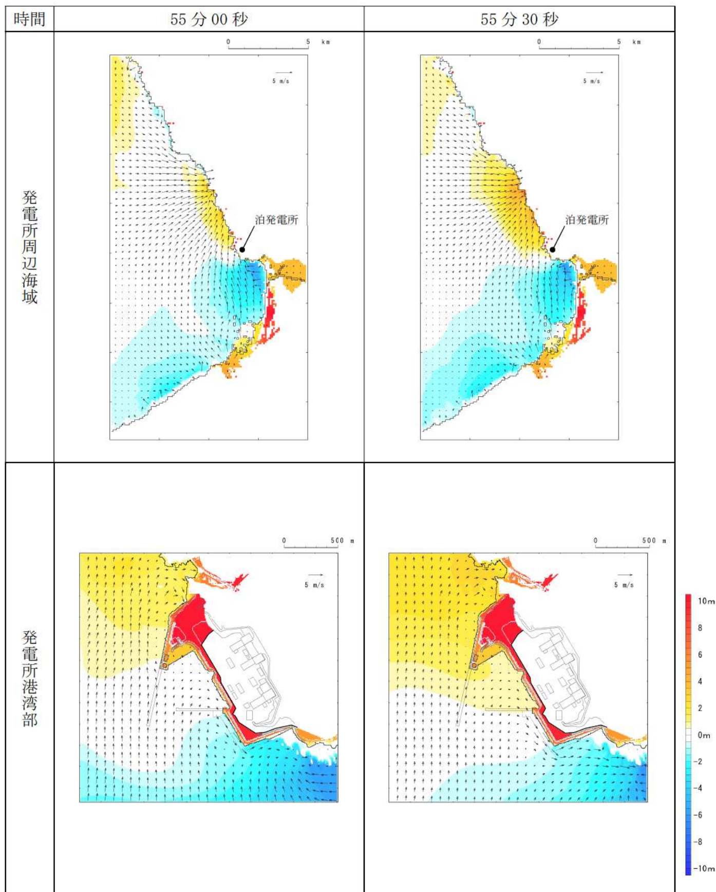
第 9 図-48 基準津波 E（北及び南防波堤損傷）の水位変動・流向ベクトル(48/53)
