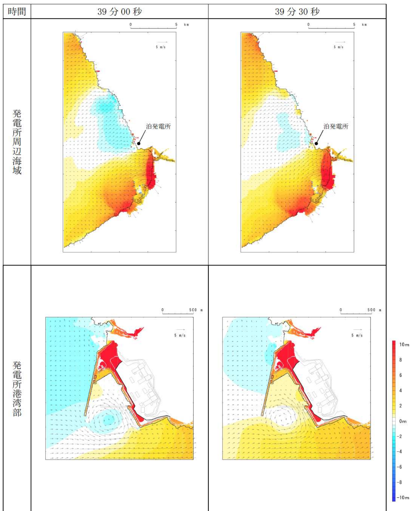
第 10 図-32 基準津波 E（南防波堤損傷）の水位変動・流向ベクトル(32/53)
