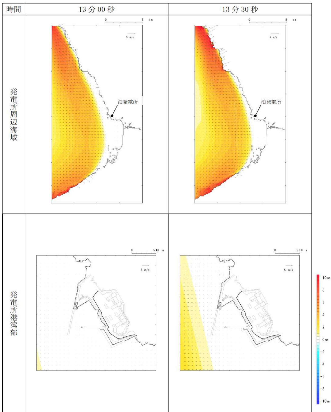
第8図-6 基準津波D（北防波堤損傷）の水位変動・流向ベクトル(6/53)
