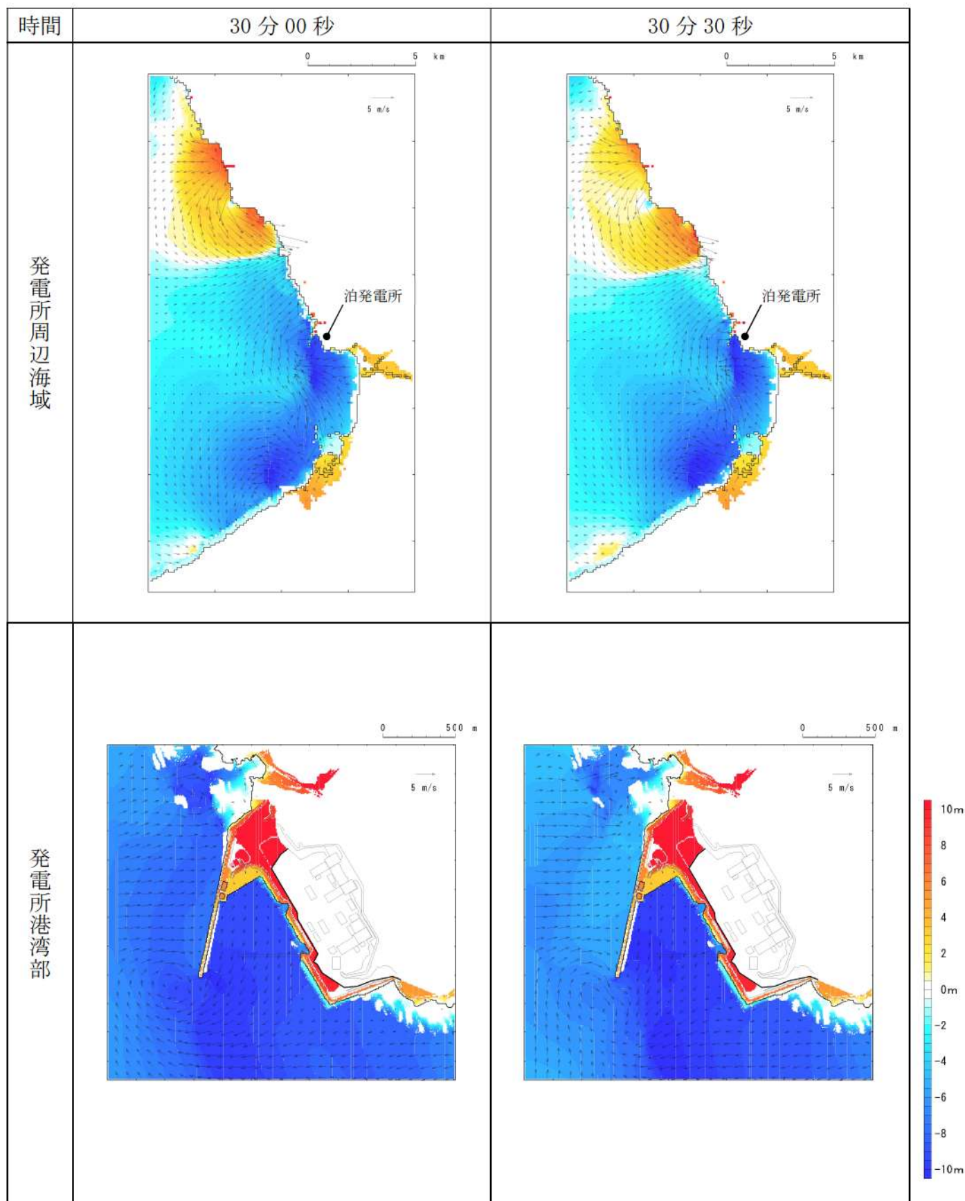
第 10 図-23 基準津波 E（南防波堤損傷）の水位変動・流向ベクトル (23/53)
