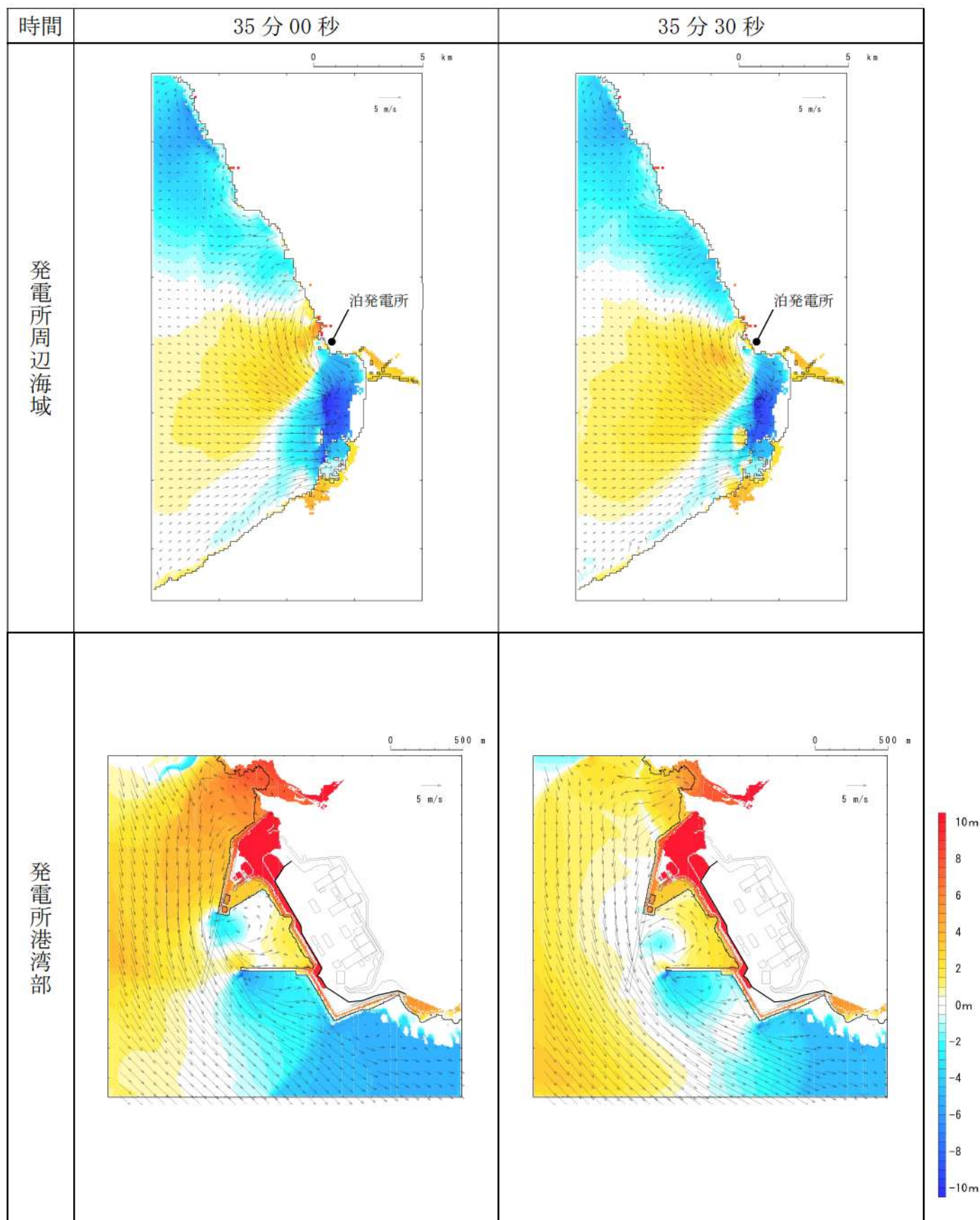
第 8 図-28 基準津波 D（北防波堤損傷）の水位変動・流向ベクトル (28/53)
