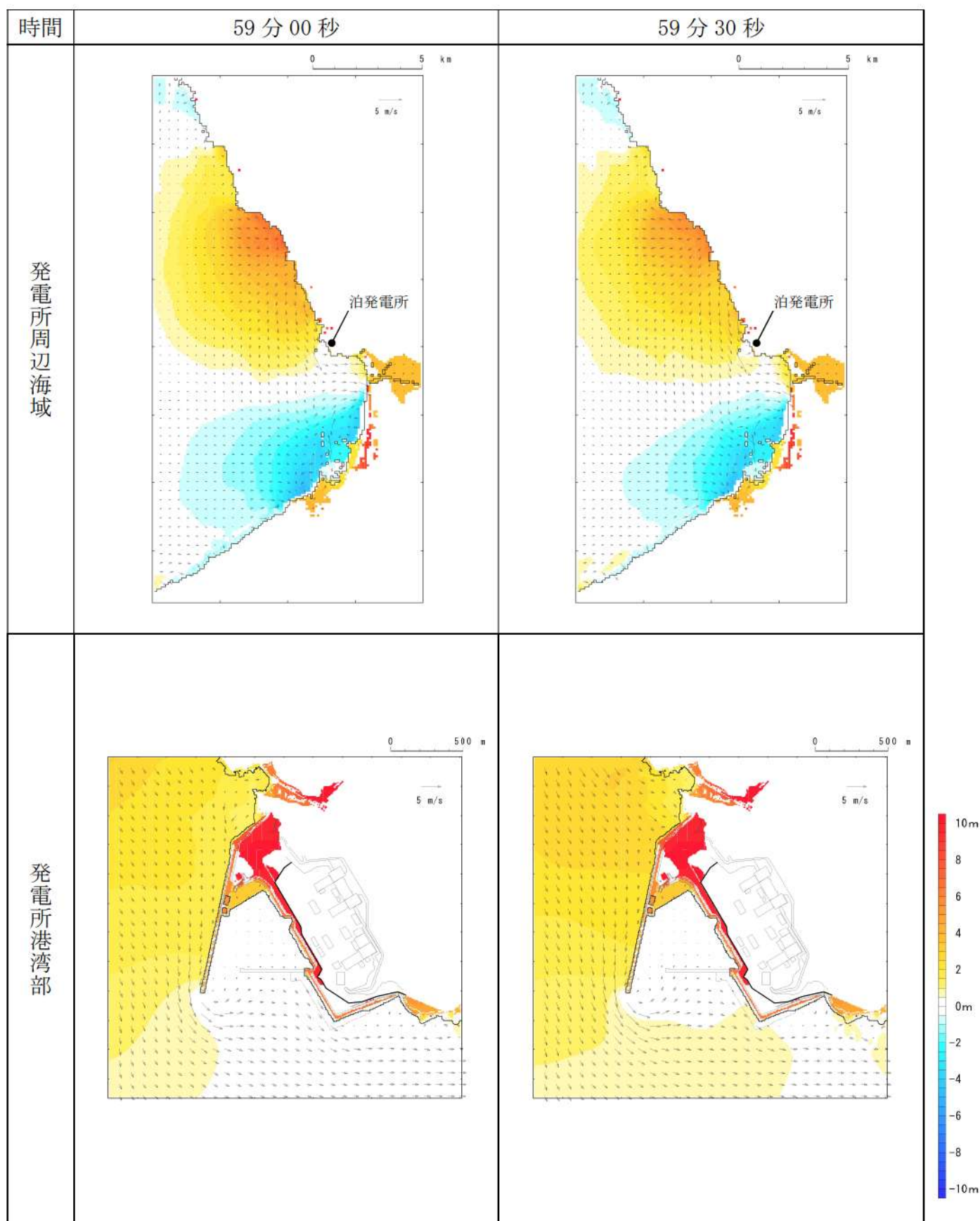
第 7 図-52 基準津波 D（南防波堤損傷）の水位変動・流向ベクトル (52/53)
