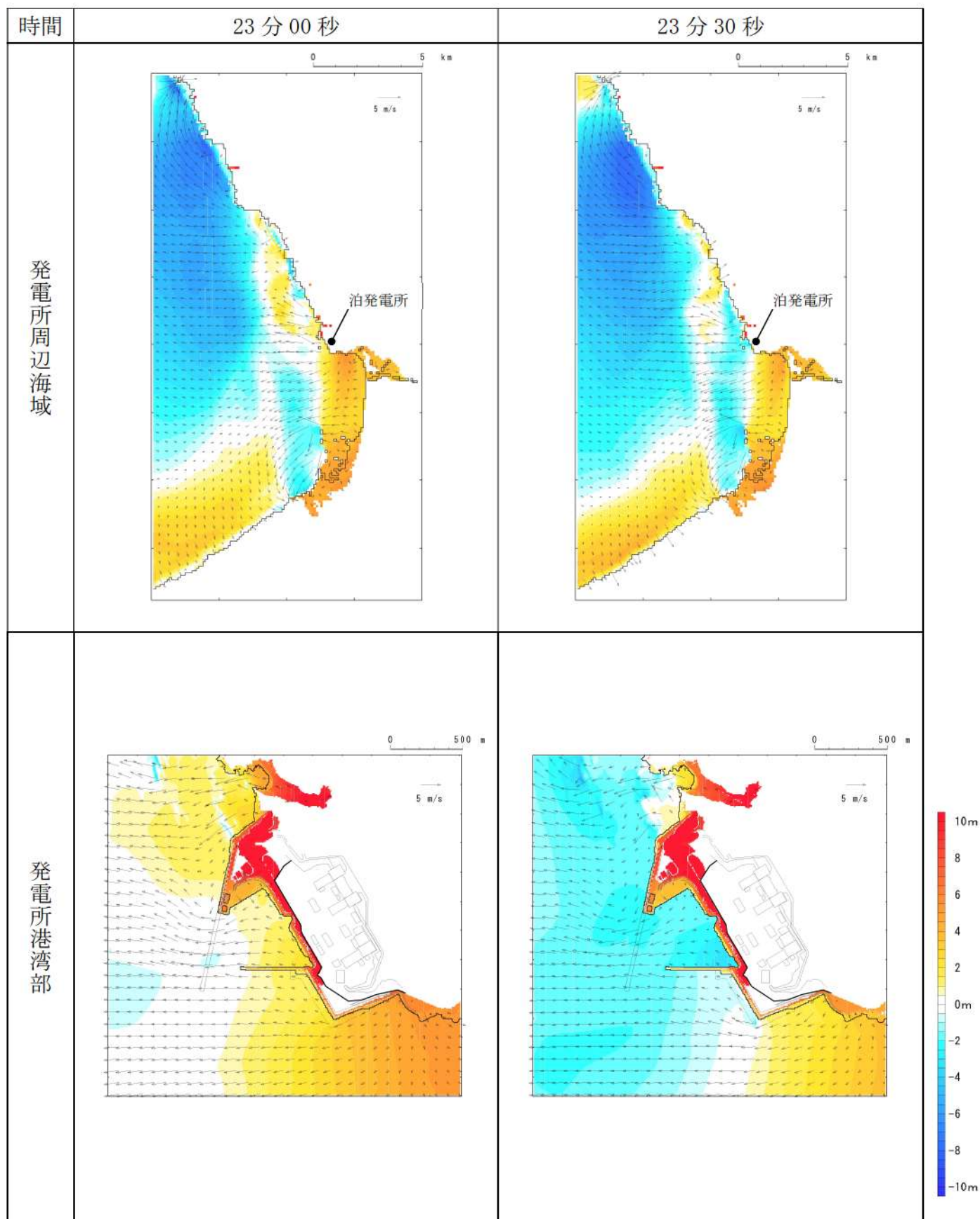
第 8 図-16 基準津波 D（北防波堤損傷）の水位変動・流向ベクトル(16/53)
