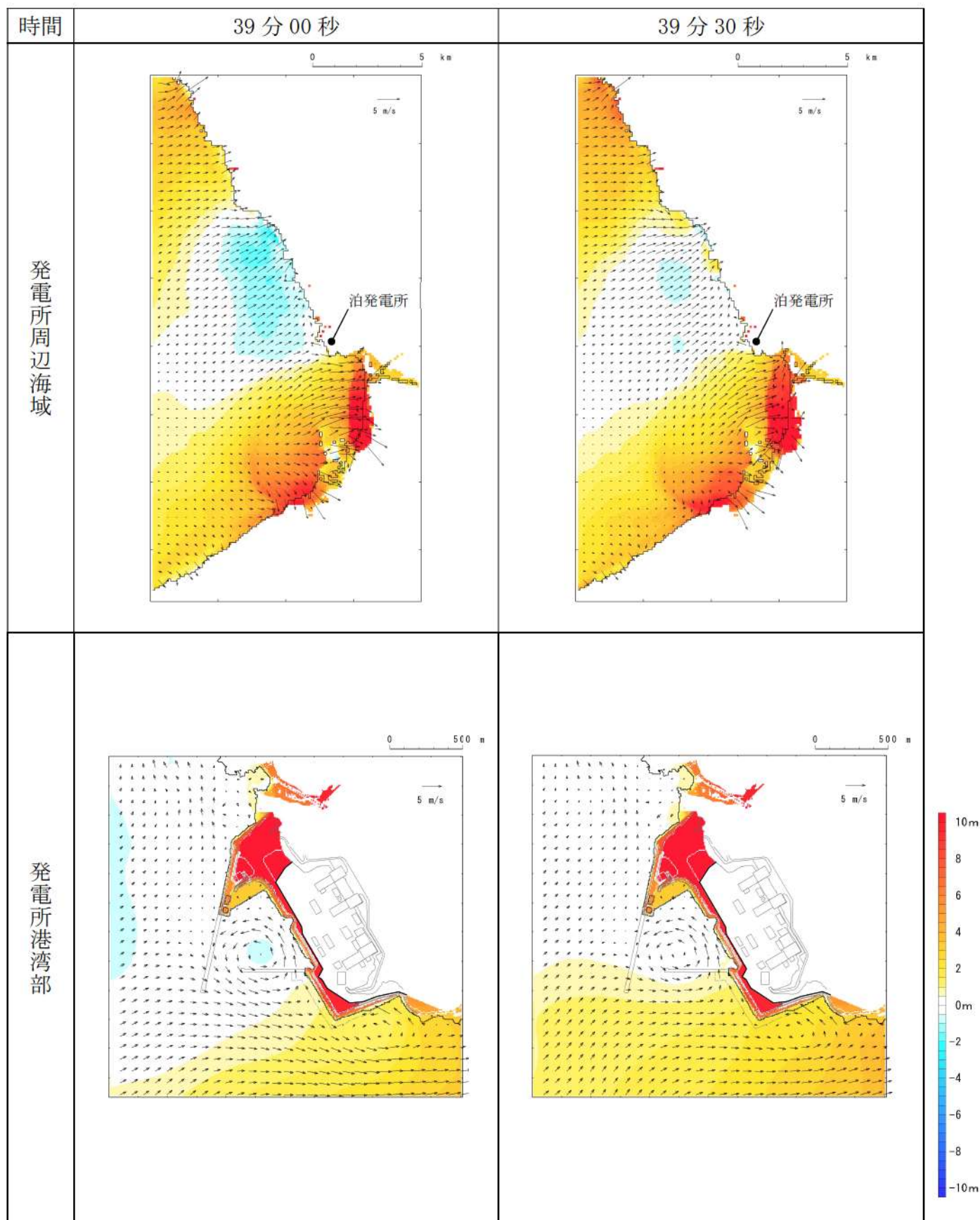
第 9 図-32 基準津波 E（北及び南防波堤損傷）の水位変動・流向ベクトル(32/53)
