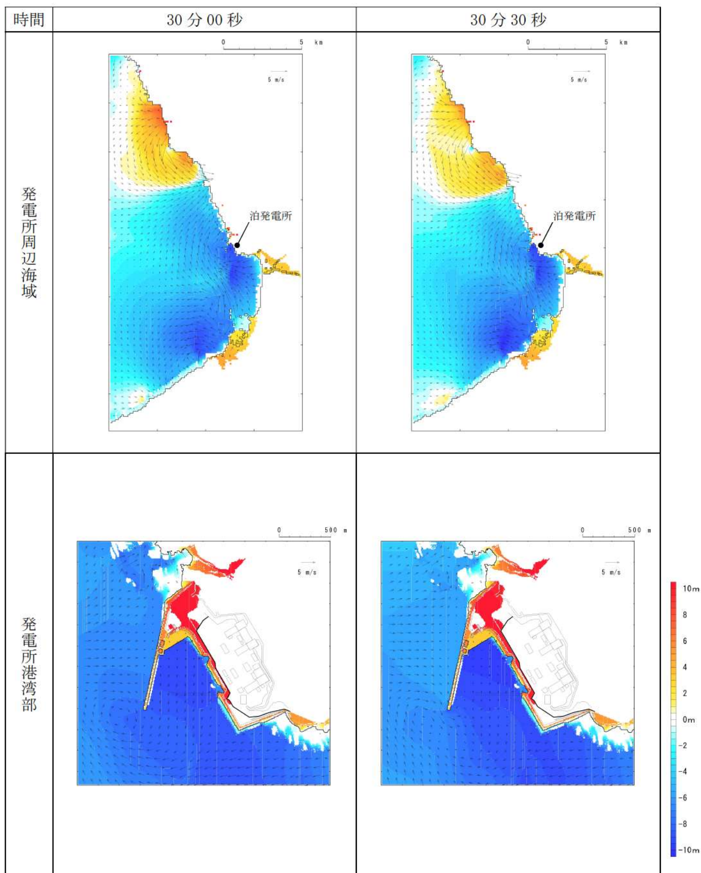
第7図-23 基準津波D（南防波堤損傷）の水位変動・流向ベクトル(23/53)
