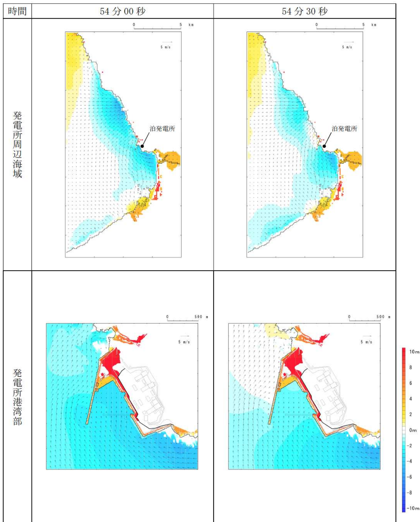
第7図-47 基準津波D（南防波堤損傷）の水位変動・流向ベクトル(47/53)
