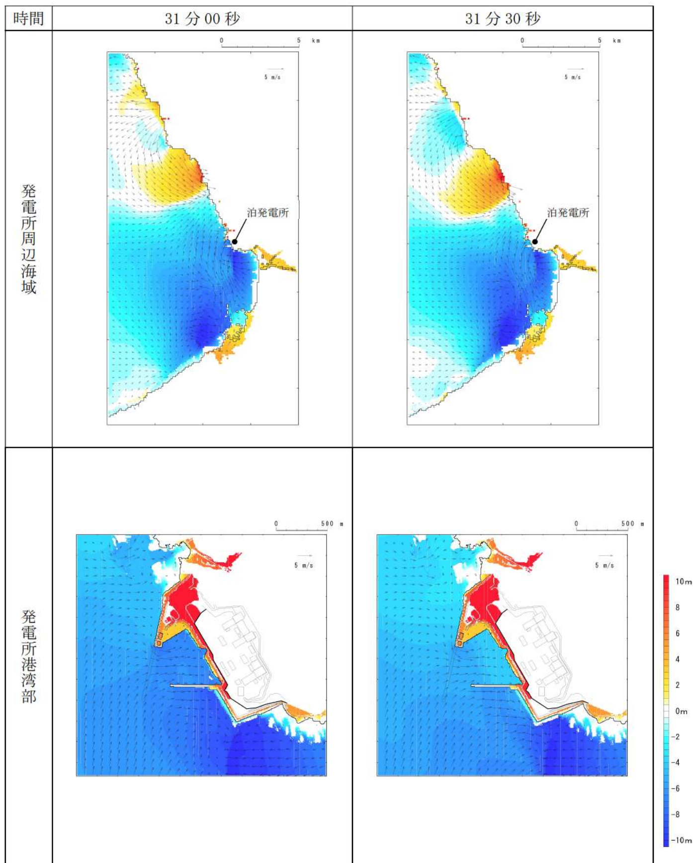
第8図-24 基準津波D（北防波堤損傷）の水位変動・流向ベクトル(24/53)
