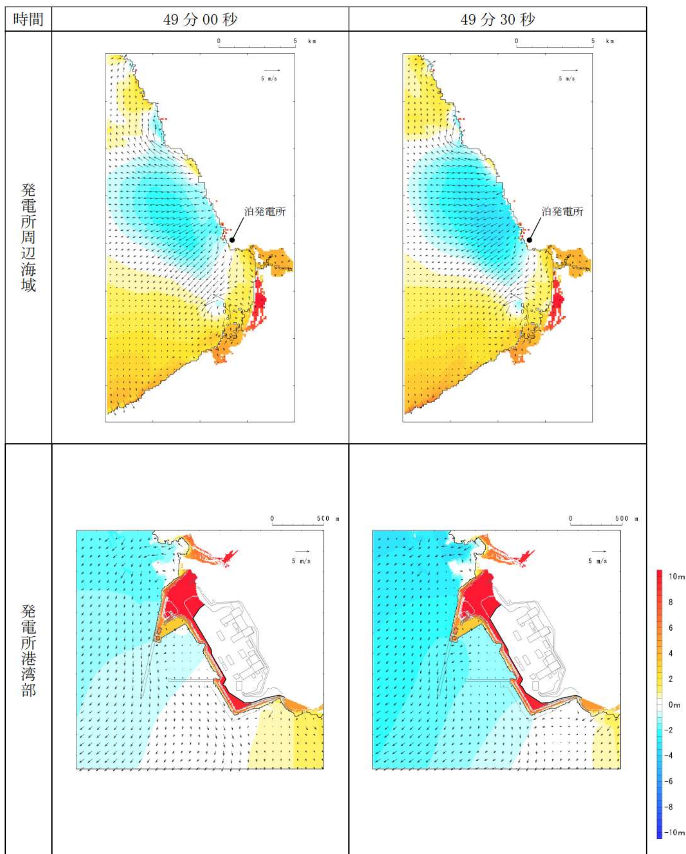
第 9 図-42 基準津波 E（北及び南防波堤損傷）の水位変動・流向ベクトル(42/53)
