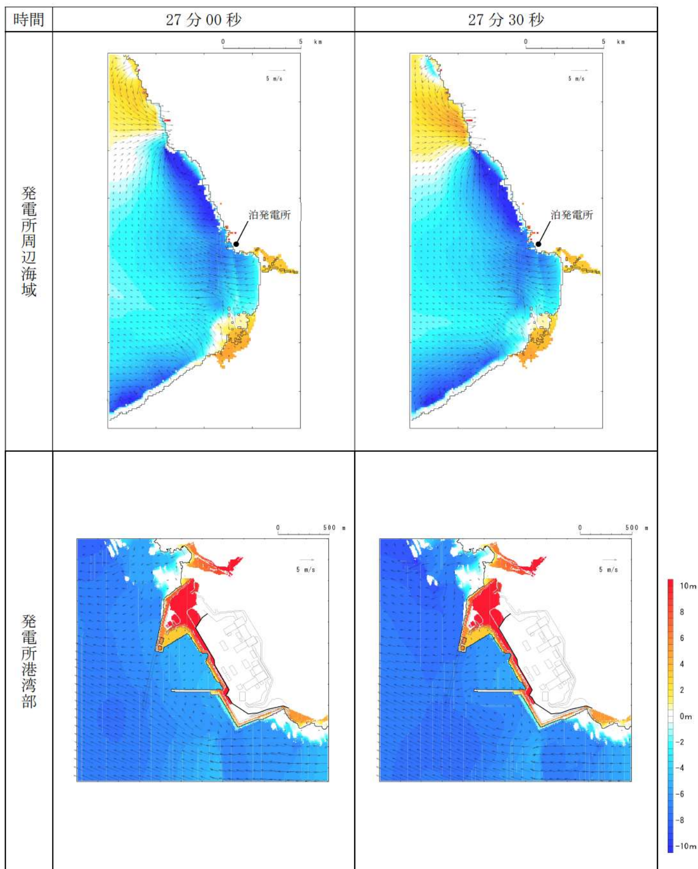
第 8 図-20 基準津波 D（北防波堤損傷）の水位変動・流向ベクトル (20/53)
