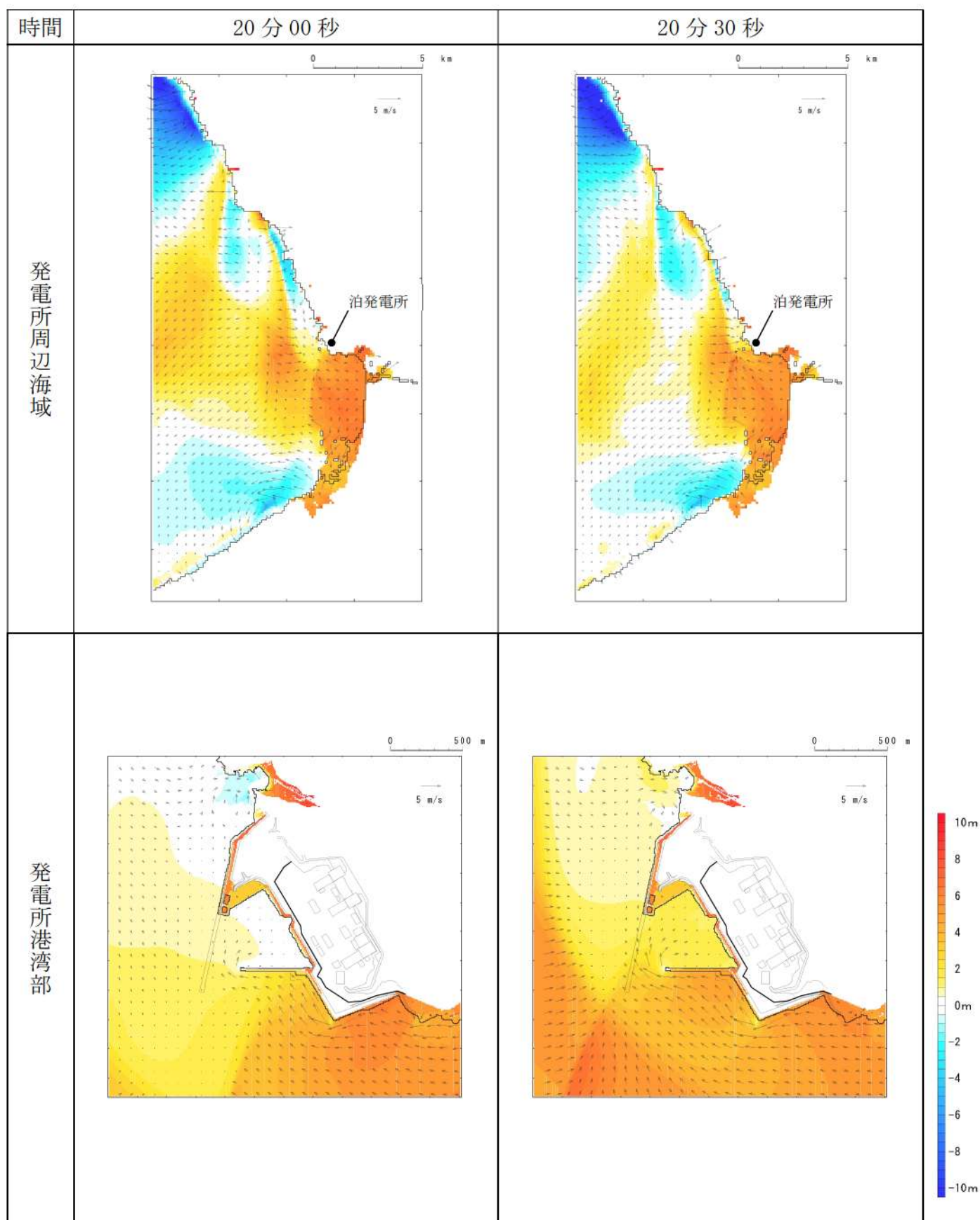
第 8 図-13 基準津波 D（北防波堤損傷）の水位変動・流向ベクトル(13/53)
