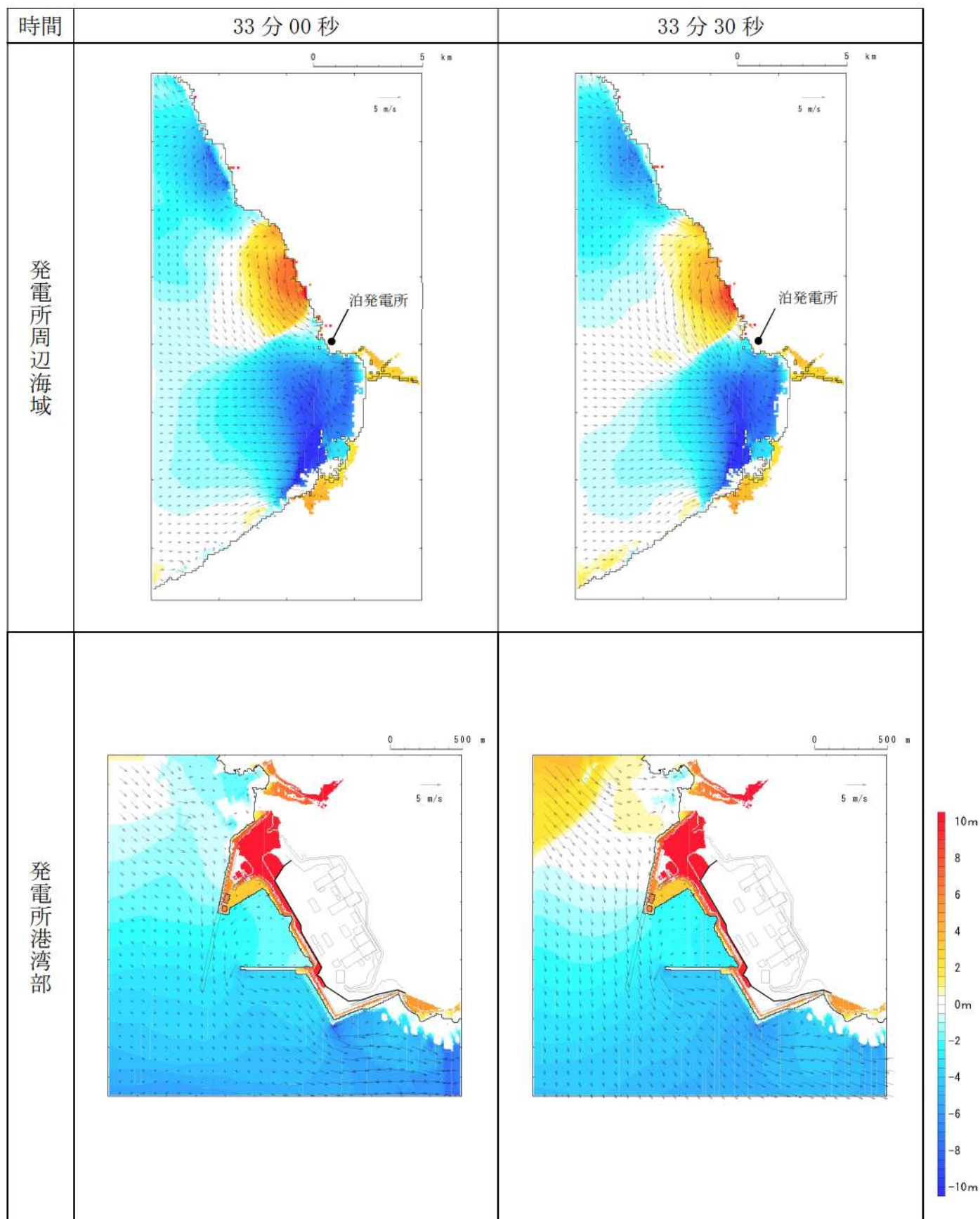
第 8 図-26 基準津波 D（北防波堤損傷）の水位変動・流向ベクトル (26/53)
