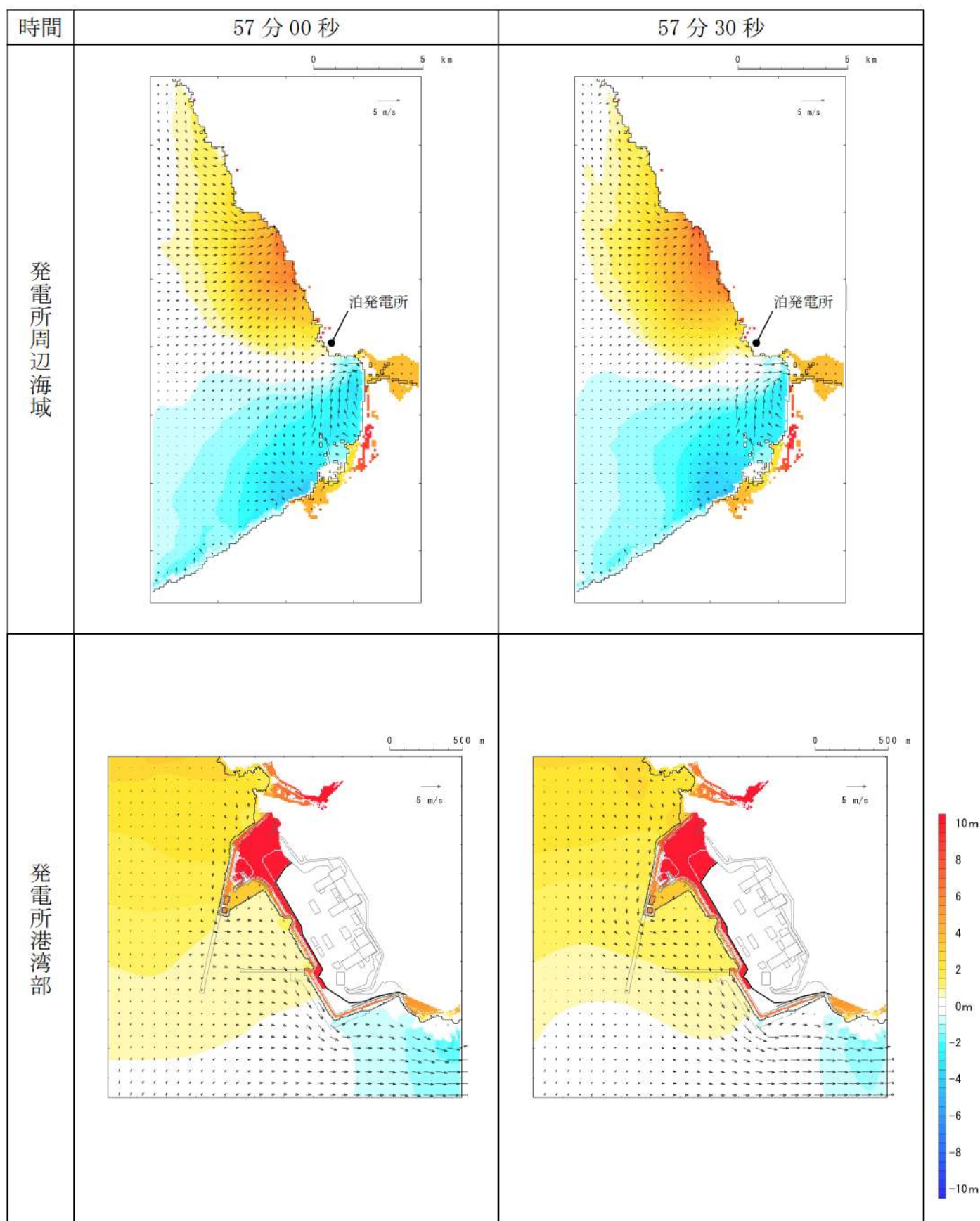
第 6 図-50 基準津波 D（北及び南防波堤損傷）の水位変動・流向ベクトル(50/53)
