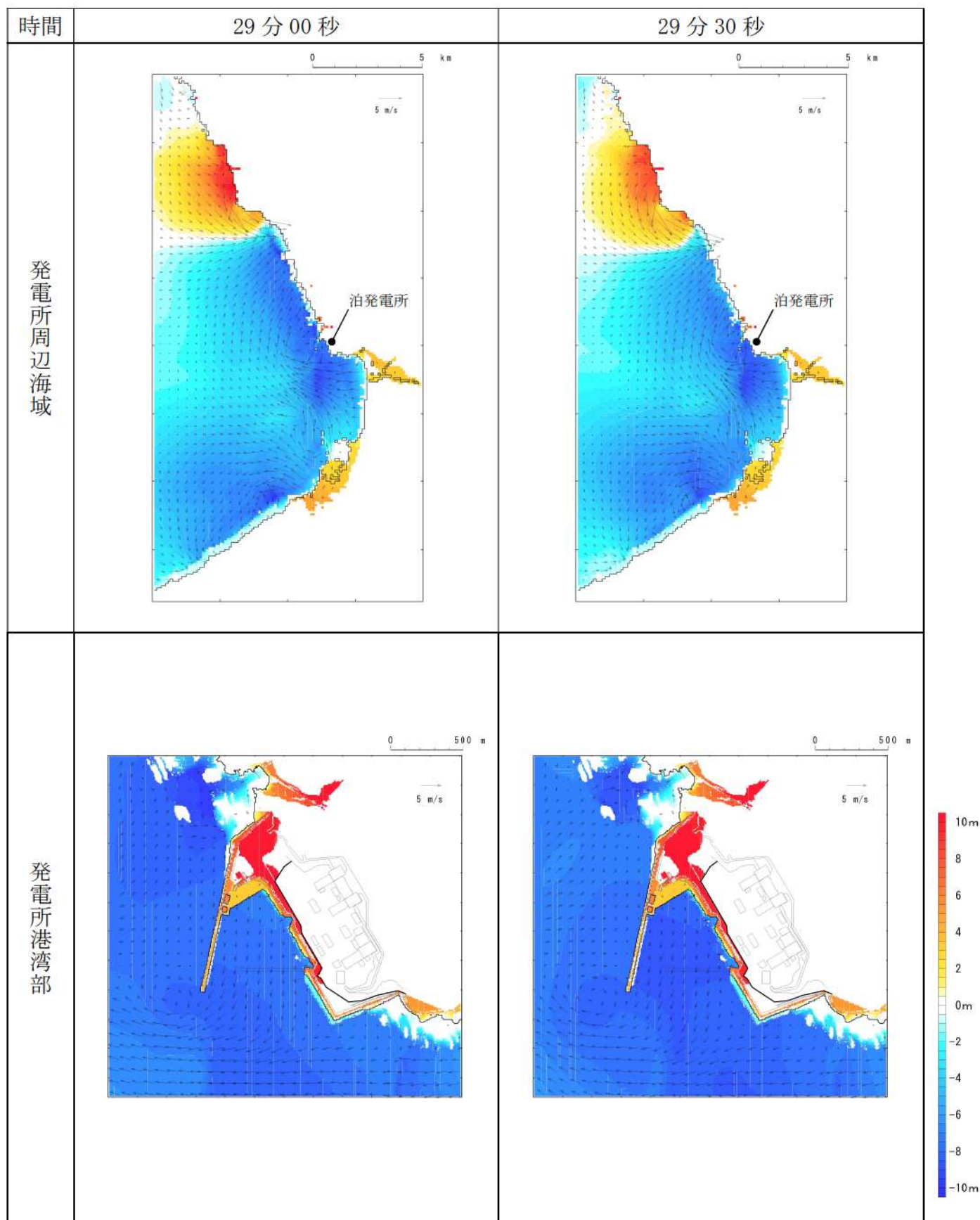
第 7 図-22 基準津波 D（南防波堤損傷）の水位変動・流向ベクトル (22/53)
