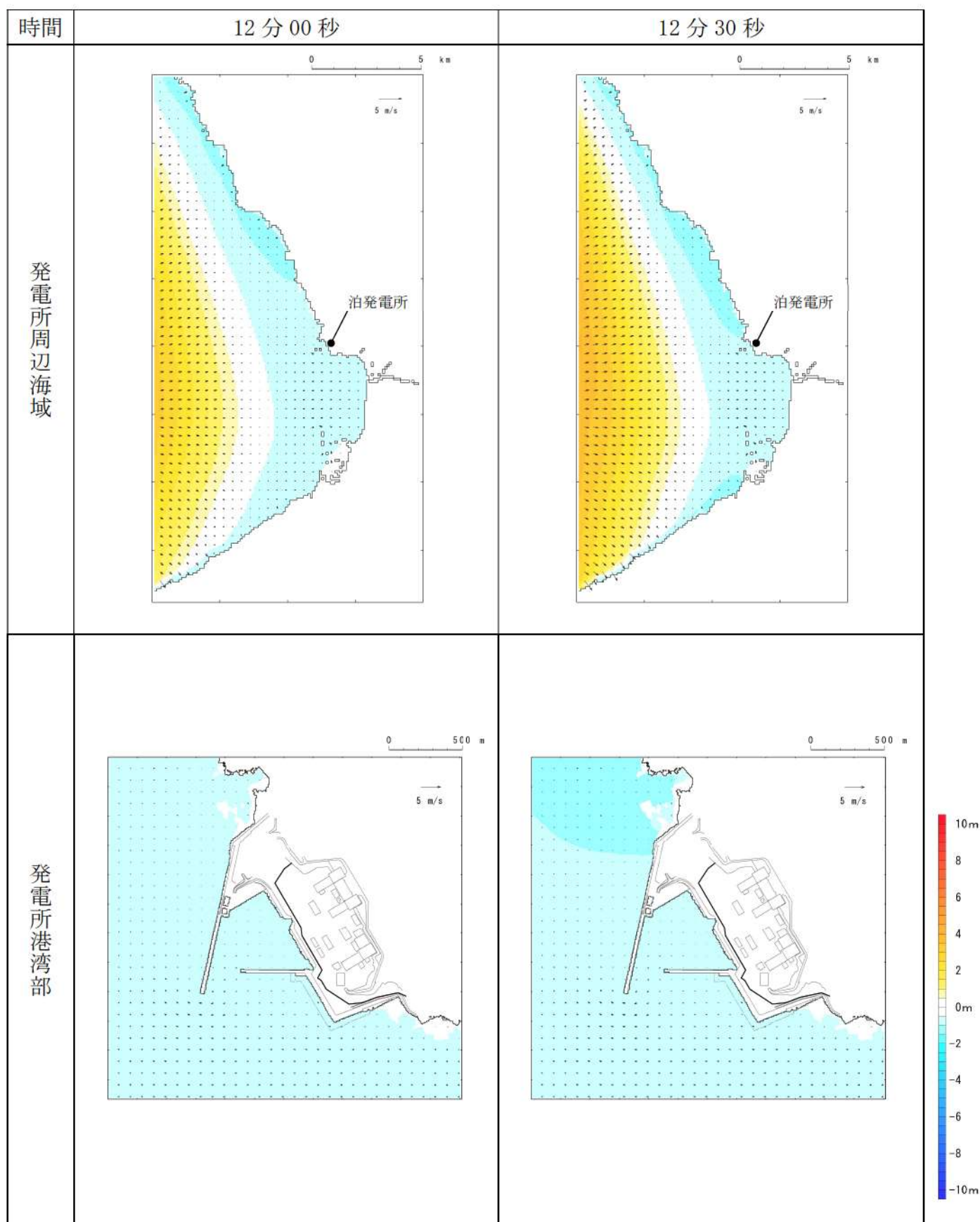
第4図-6 基準津波C（防波堤損傷なし）の水位変動・流向ベクトル(6/54)
