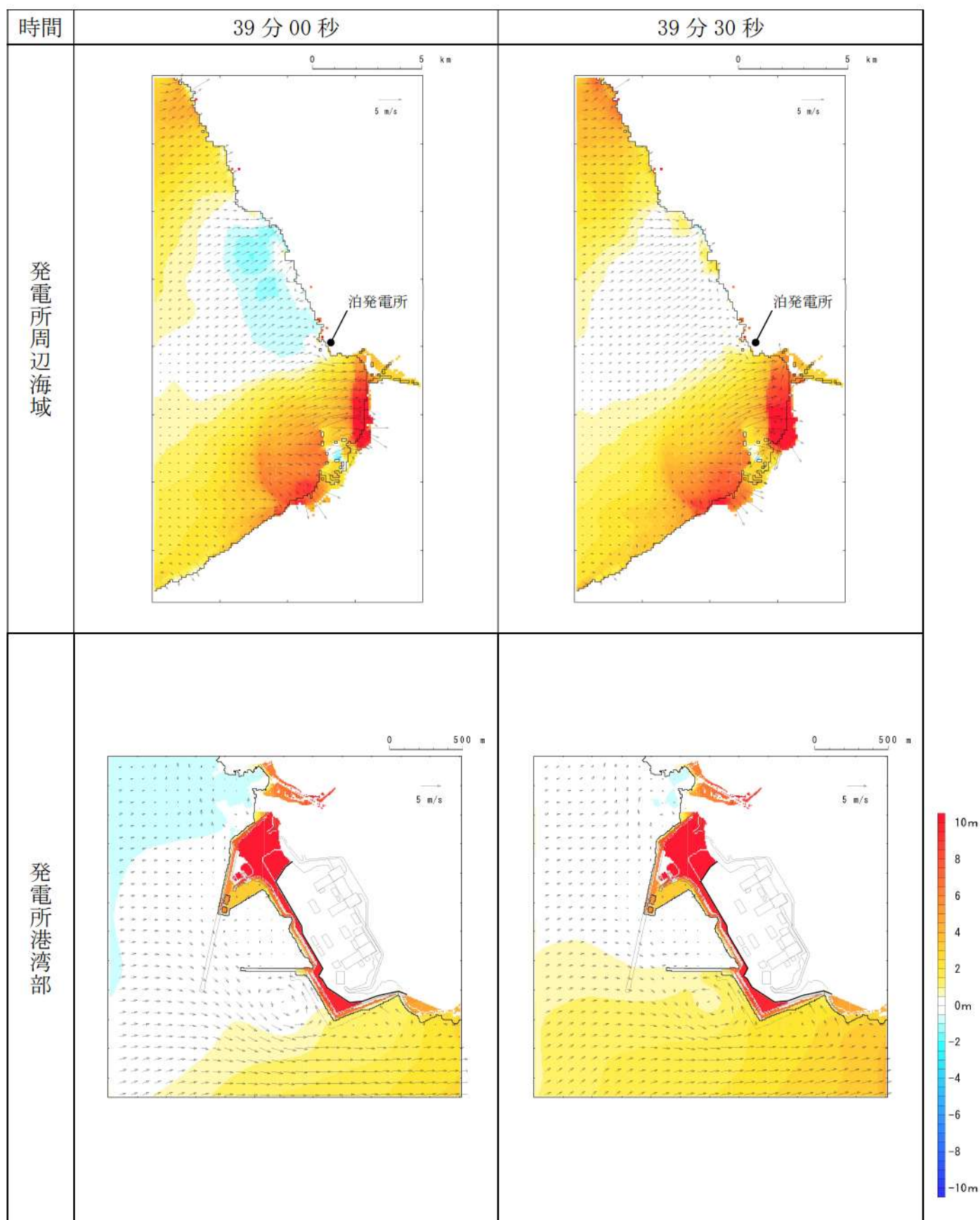
第3図-32 基準津波B（北防波堤損傷）の水位変動・流向ベクトル(32/53)
