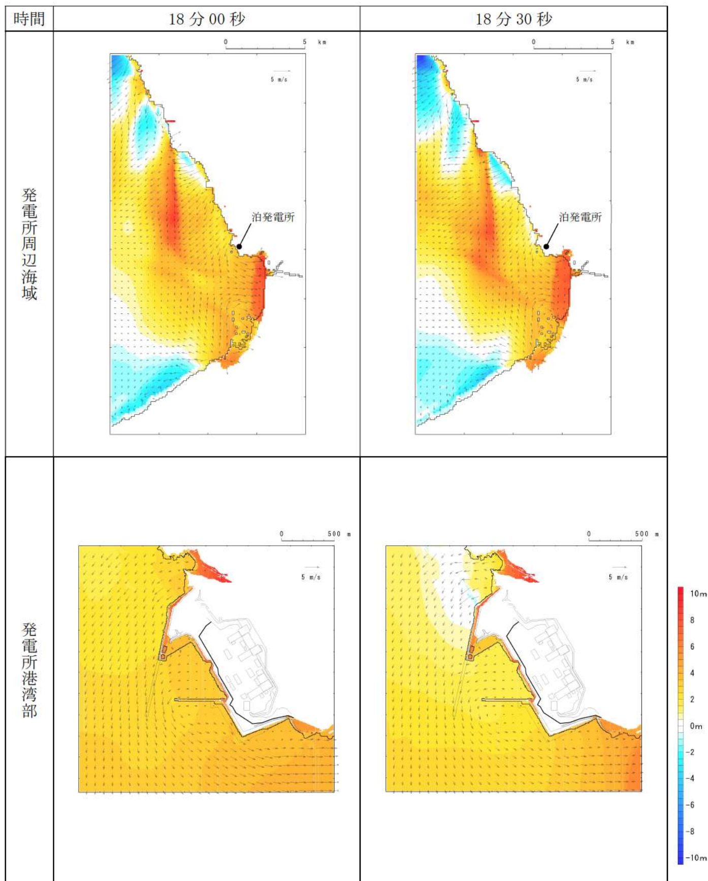
第3図-11 基準津波B（北防波堤損傷）の水位変動・流向ベクトル(11/53)
