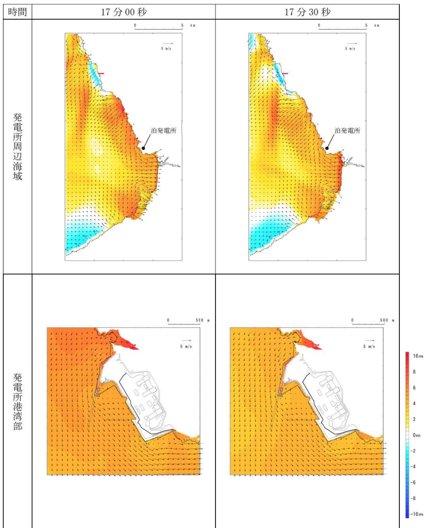
第 6 図-10 基準津波 D（北及び南防波堤損傷）の水位変動・流向ベクトル(10/53)
