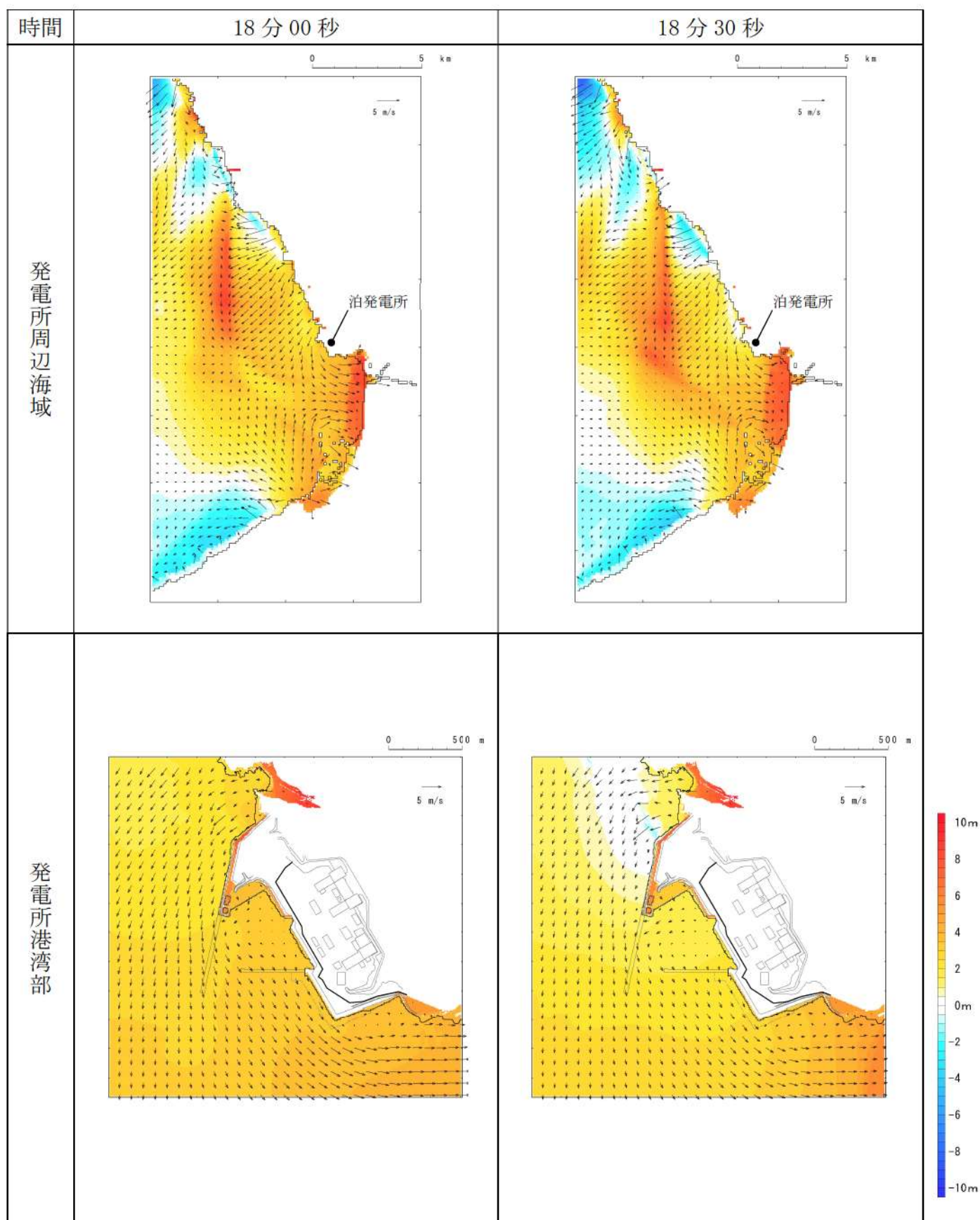
第 6 図-11 基準津波 D（北及び南防波堤損傷）の水位変動・流向ベクトル(11/53)
