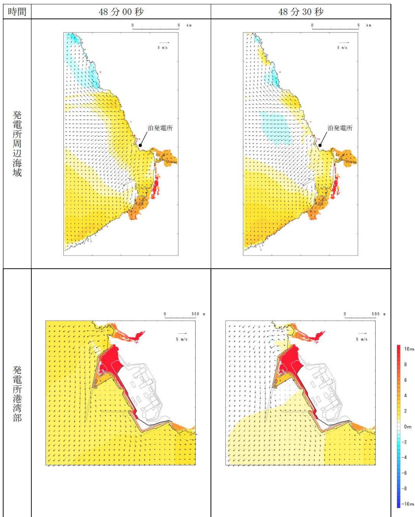
第 6 図-41 基準津波 D（北及び南防波堤損傷）の水位変動・流向ベクトル(41/53)
