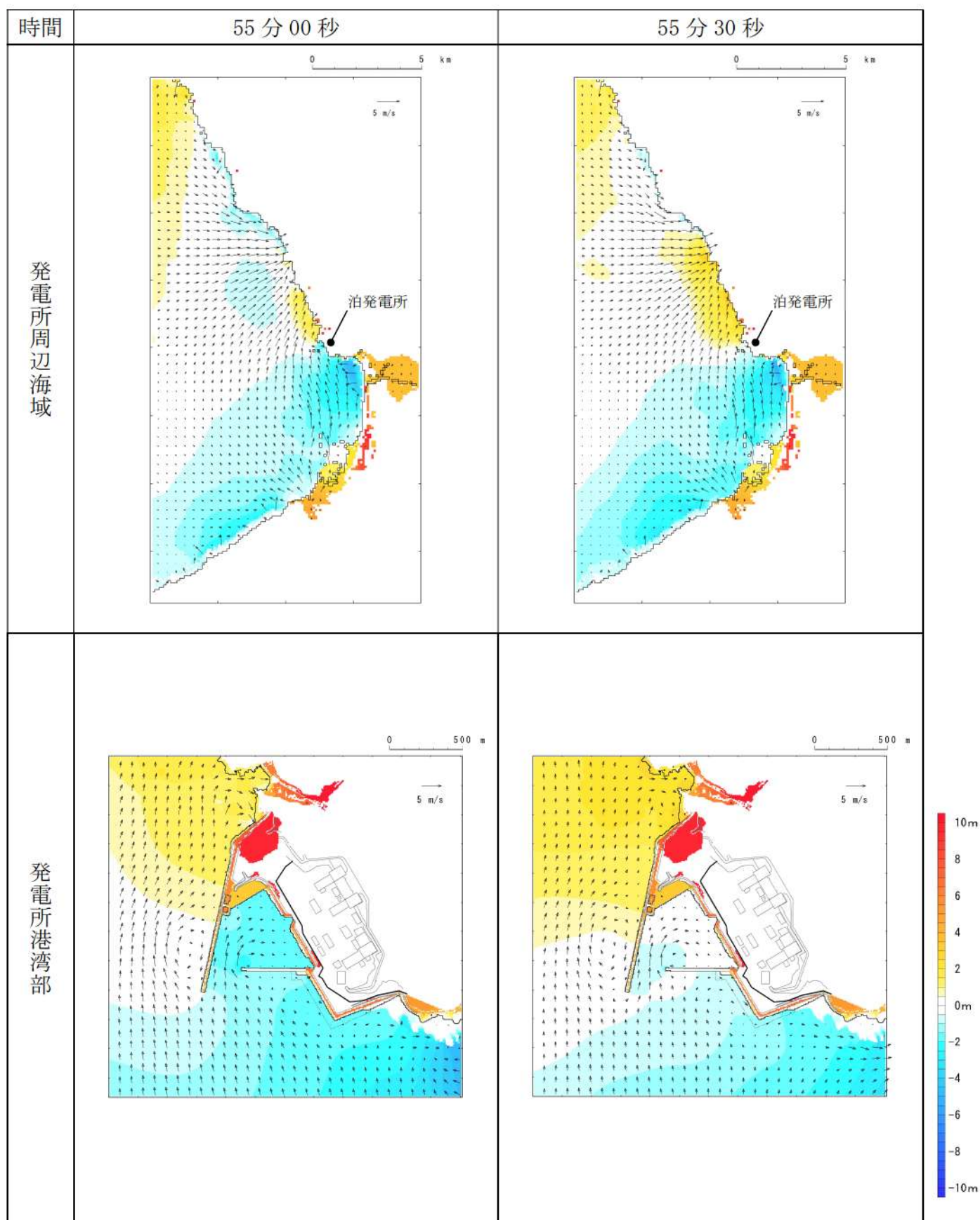
第 5 図-48 基準津波 D（防波堤損傷なし）の水位変動・流向ベクトル(48/53)
