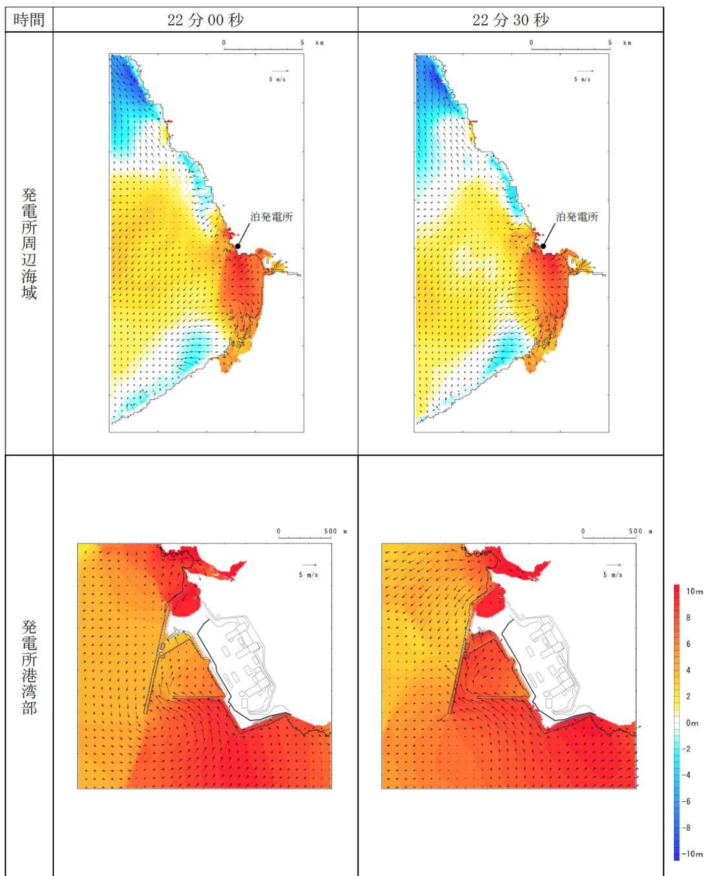
第 4 図-16 基準津波 C（防波堤損傷なし）の水位変動・流向ベクトル(16/54)
