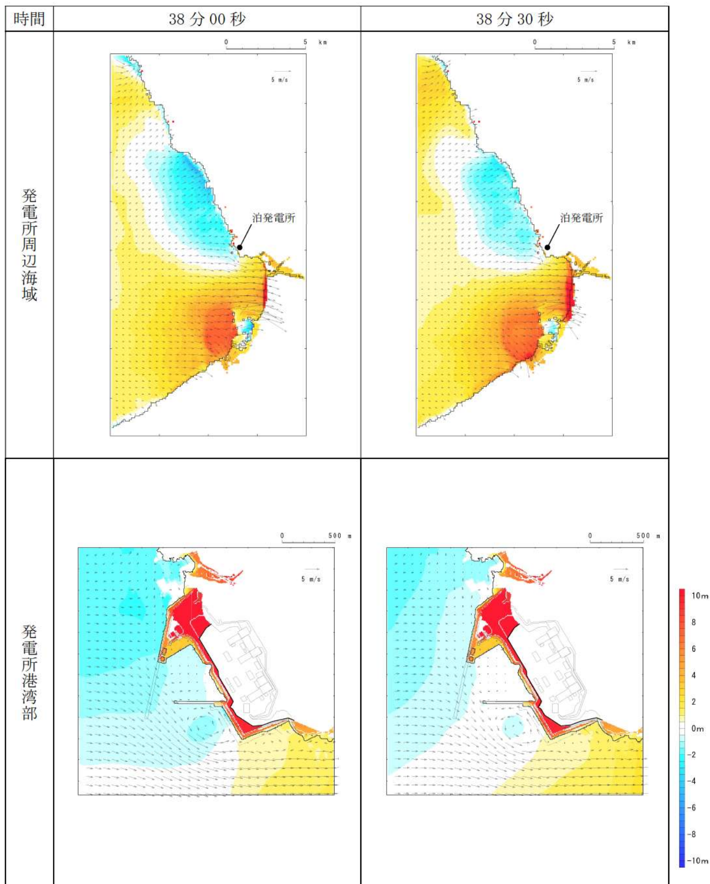
第3図-31 基準津波B（北防波堤損傷）の水位変動・流向ベクトル(31/53)
