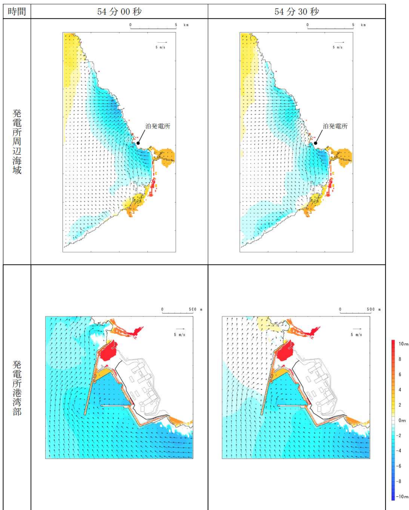
第 5 図-47 基準津波 D（防波堤損傷なし）の水位変動・流向ベクトル(47/53)
