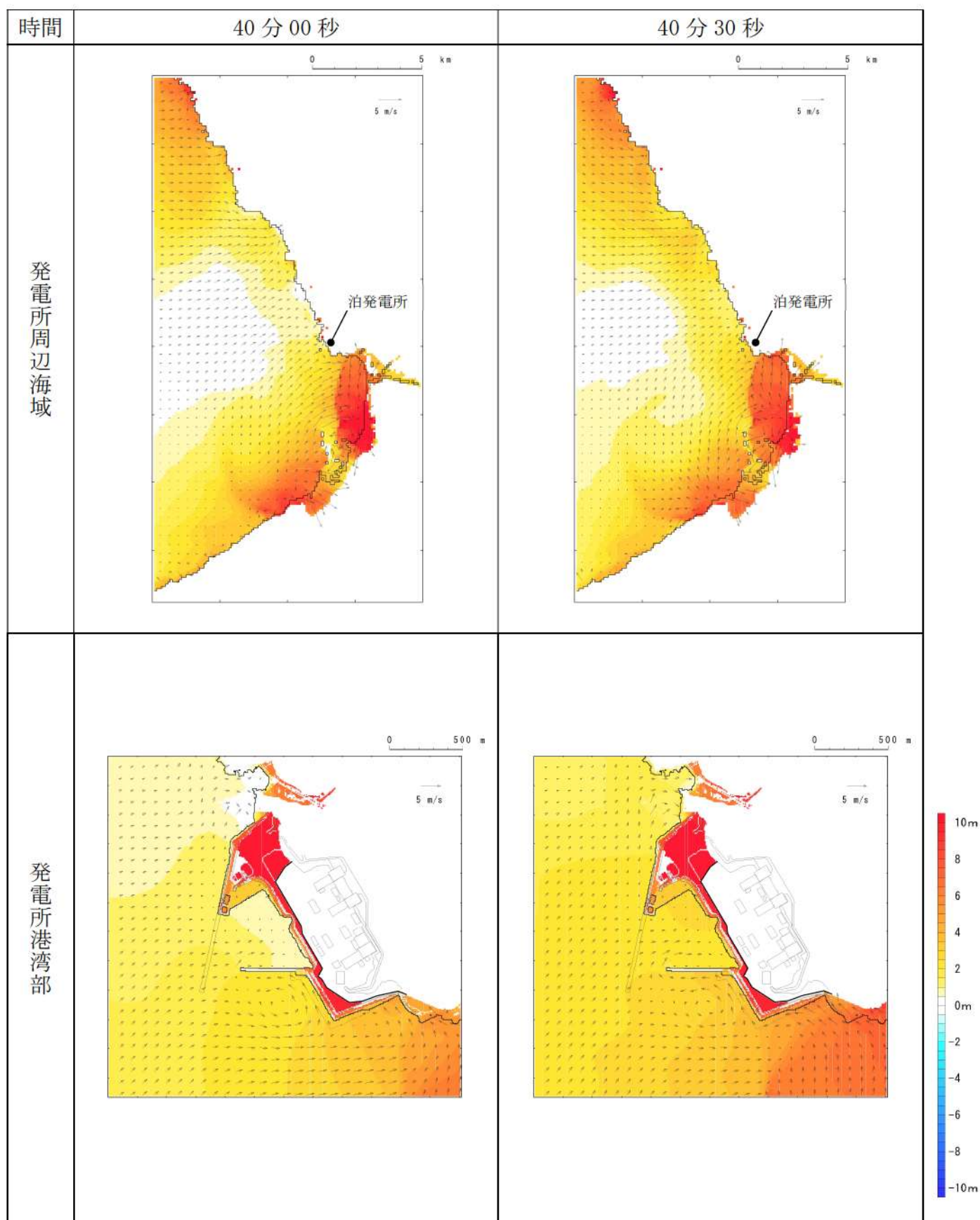
第3図-33 基準津波B（北防波堤損傷）の水位変動・流向ベクトル(33/53)
