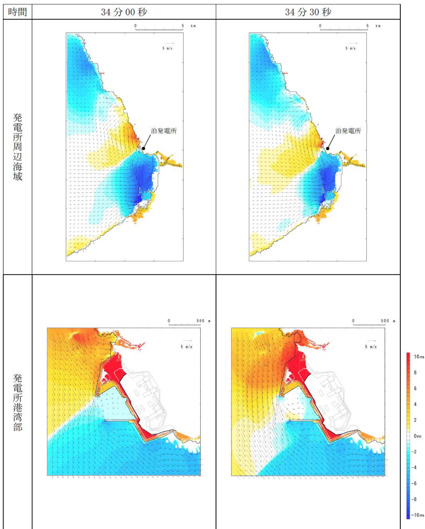
第3図-27 基準津波B（北防波堤損傷）の水位変動・流向ベクトル(27/53)
