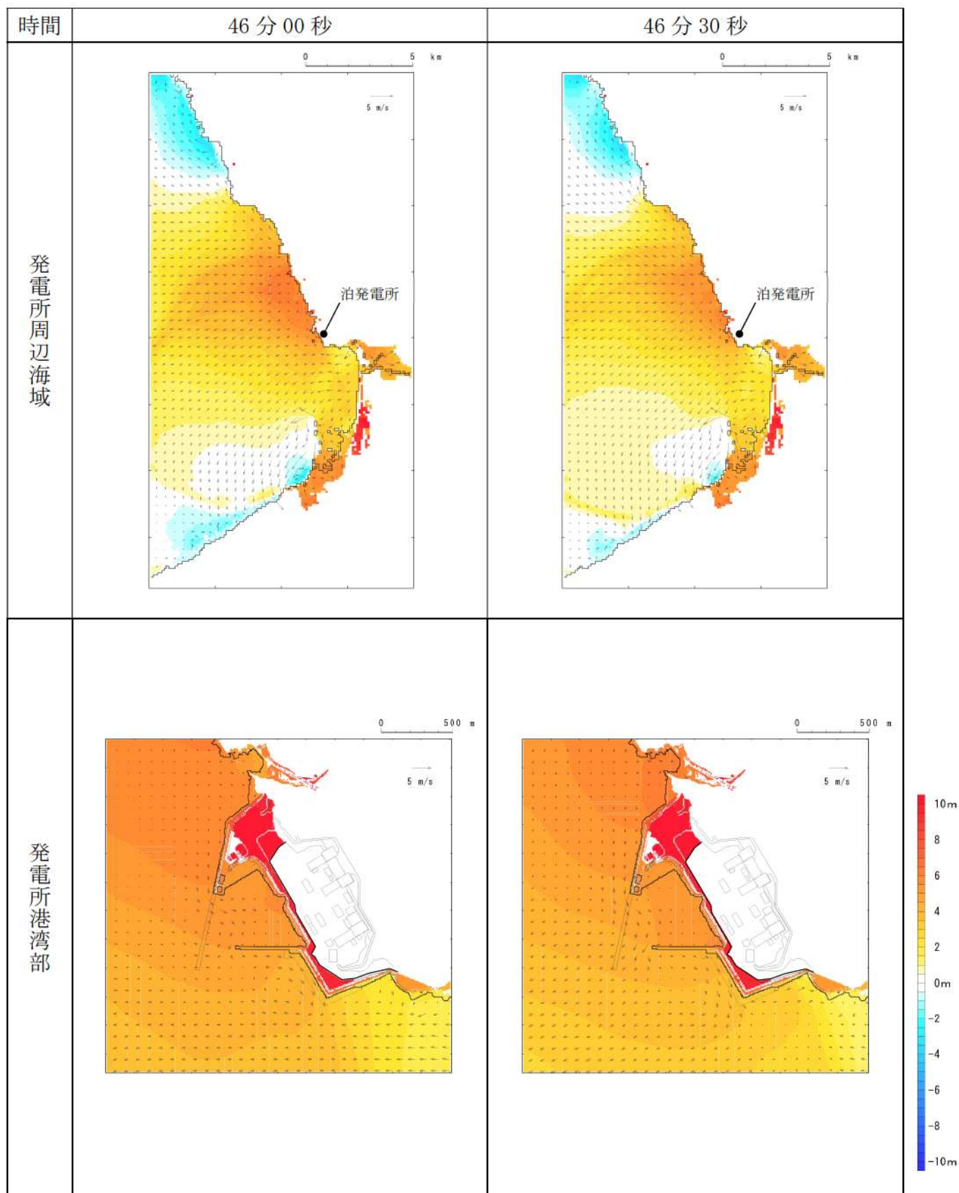
第 3 図-39 基準津波 B（北防波堤損傷）の水位変動・流向ベクトル(39/53)
