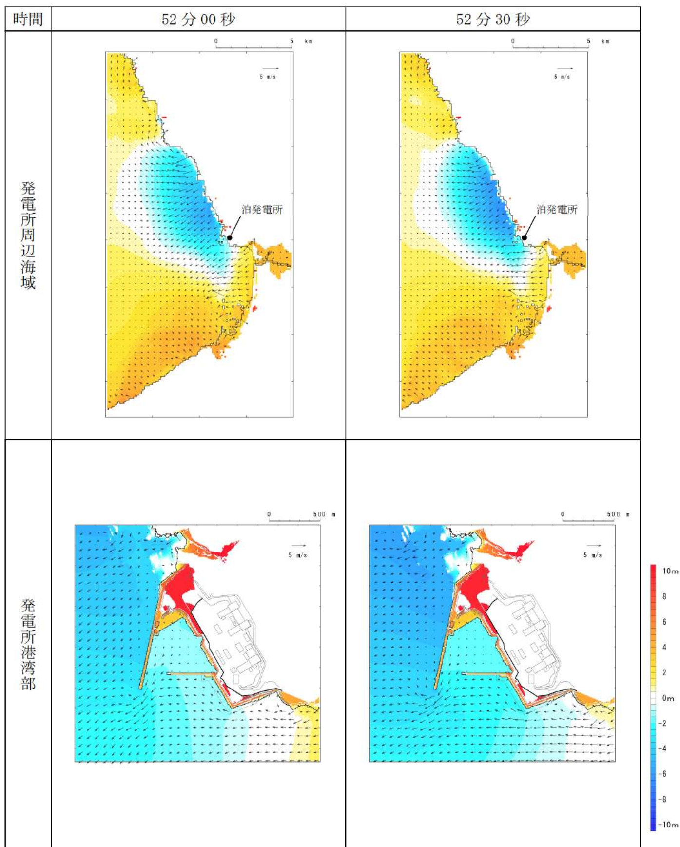
第 4 図-46 基準津波 C（防波堤損傷なし）の水位変動・流向ベクトル(46/54)
