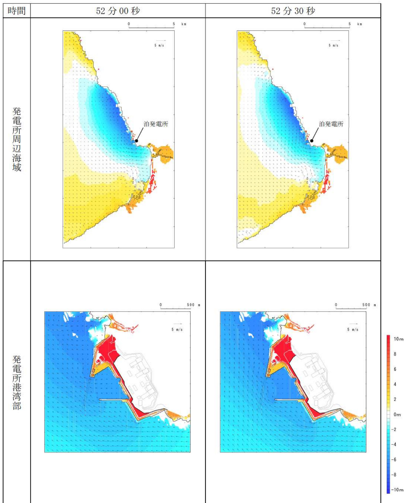
第3図-45 基準津波B（北防波堤損傷）の水位変動・流向ベクトル(45/53)
