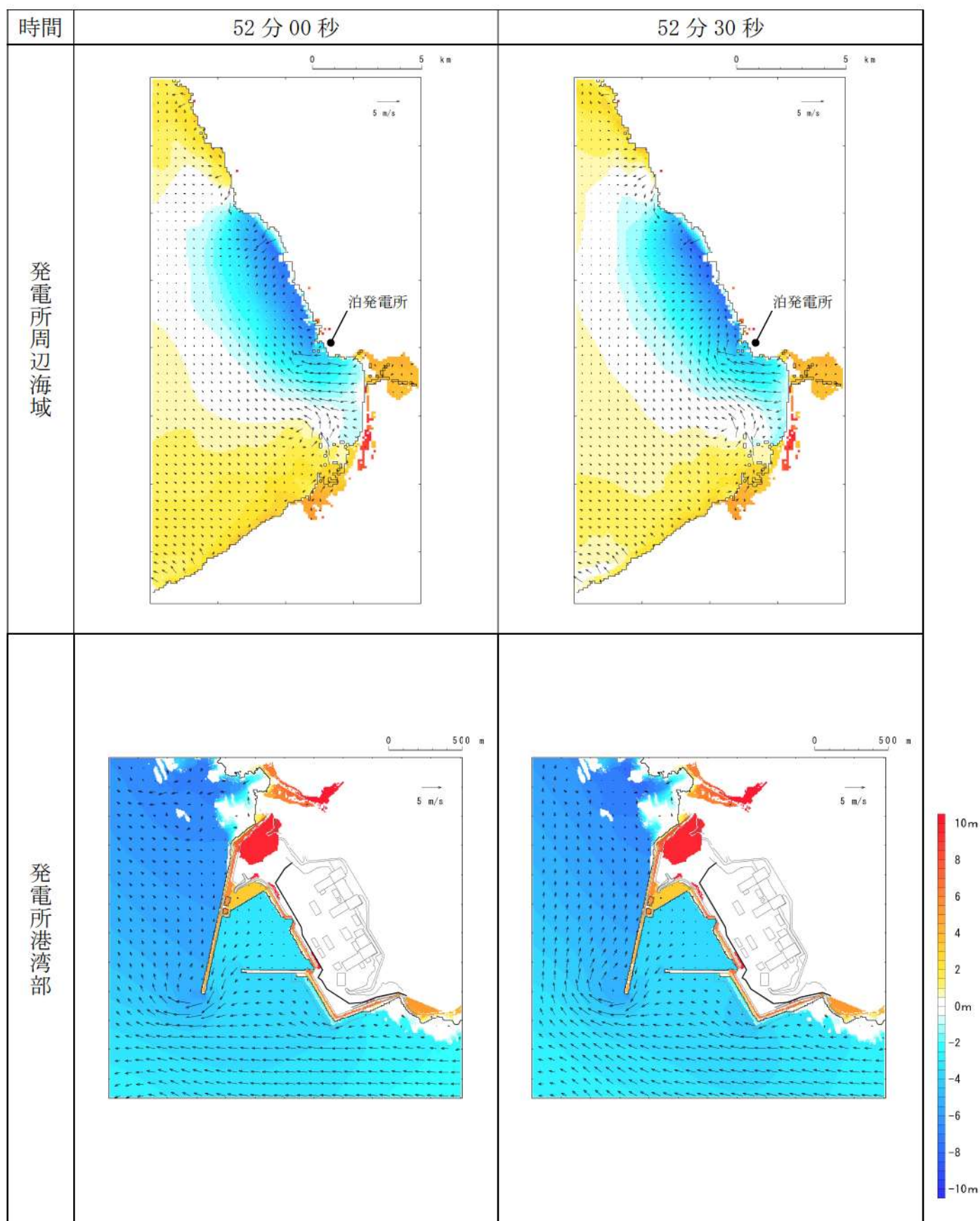
第 5 図-45 基準津波 D（防波堤損傷なし）の水位変動・流向ベクトル(45/53)
