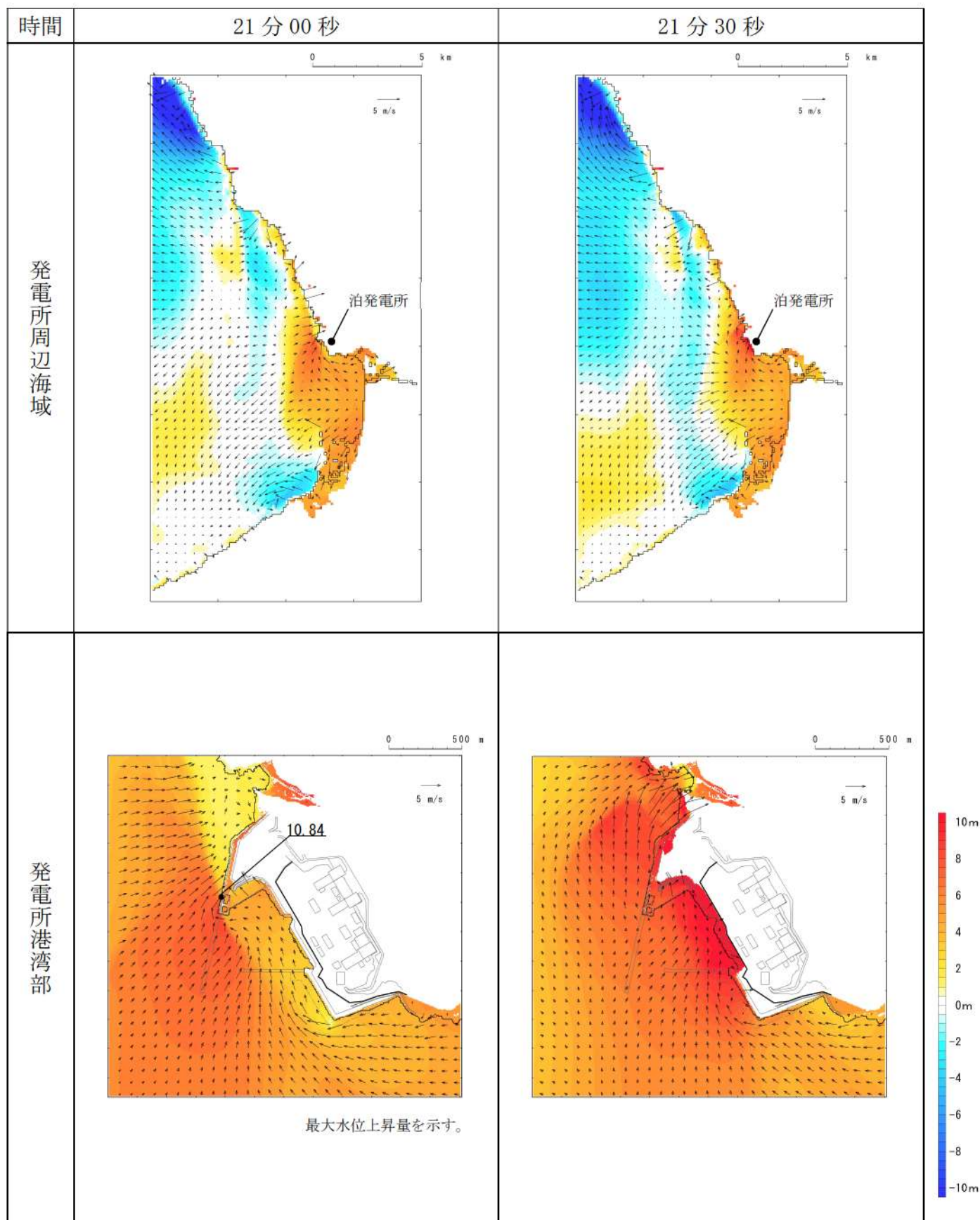
第 6 図-14 基準津波 D（北及び南防波堤損傷）の水位変動・流向ベクトル(14/53)
