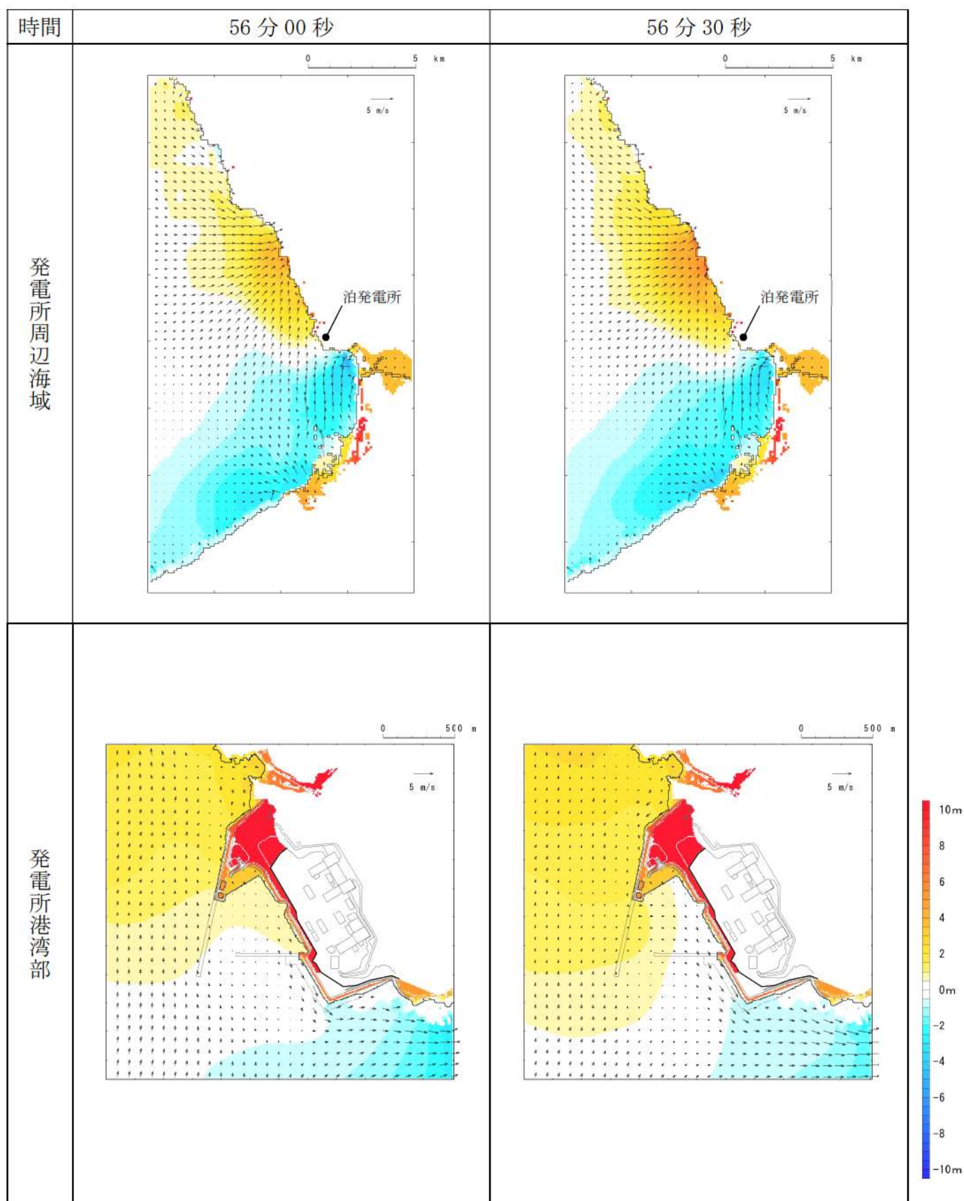
第 6 図-49 基準津波 D（北及び南防波堤損傷）の水位変動・流向ベクトル(49/53)
