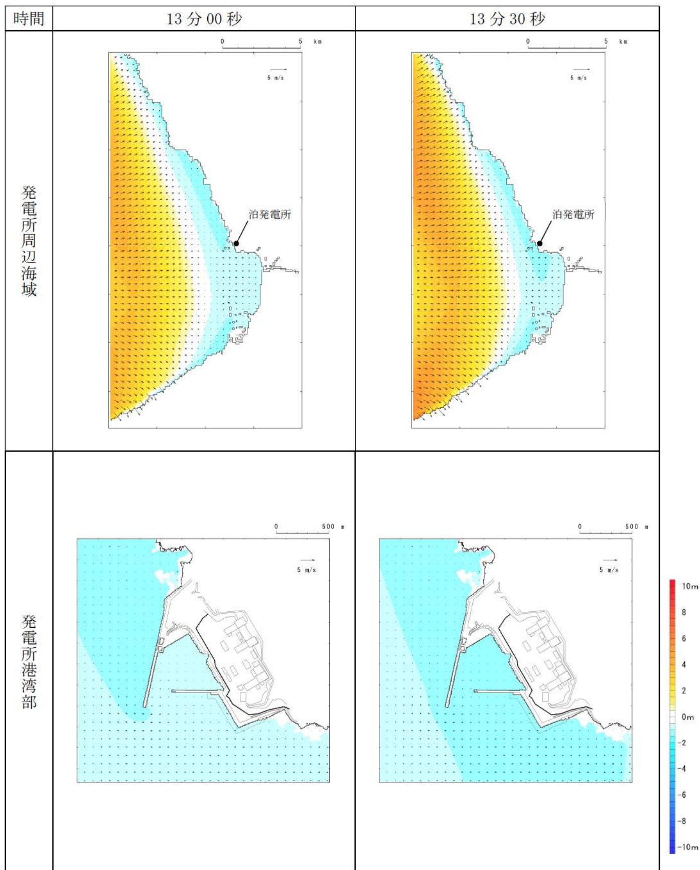
第4図-7 基準津波C（防波堤損傷なし）の水位変動・流向ベクトル(7/54)
