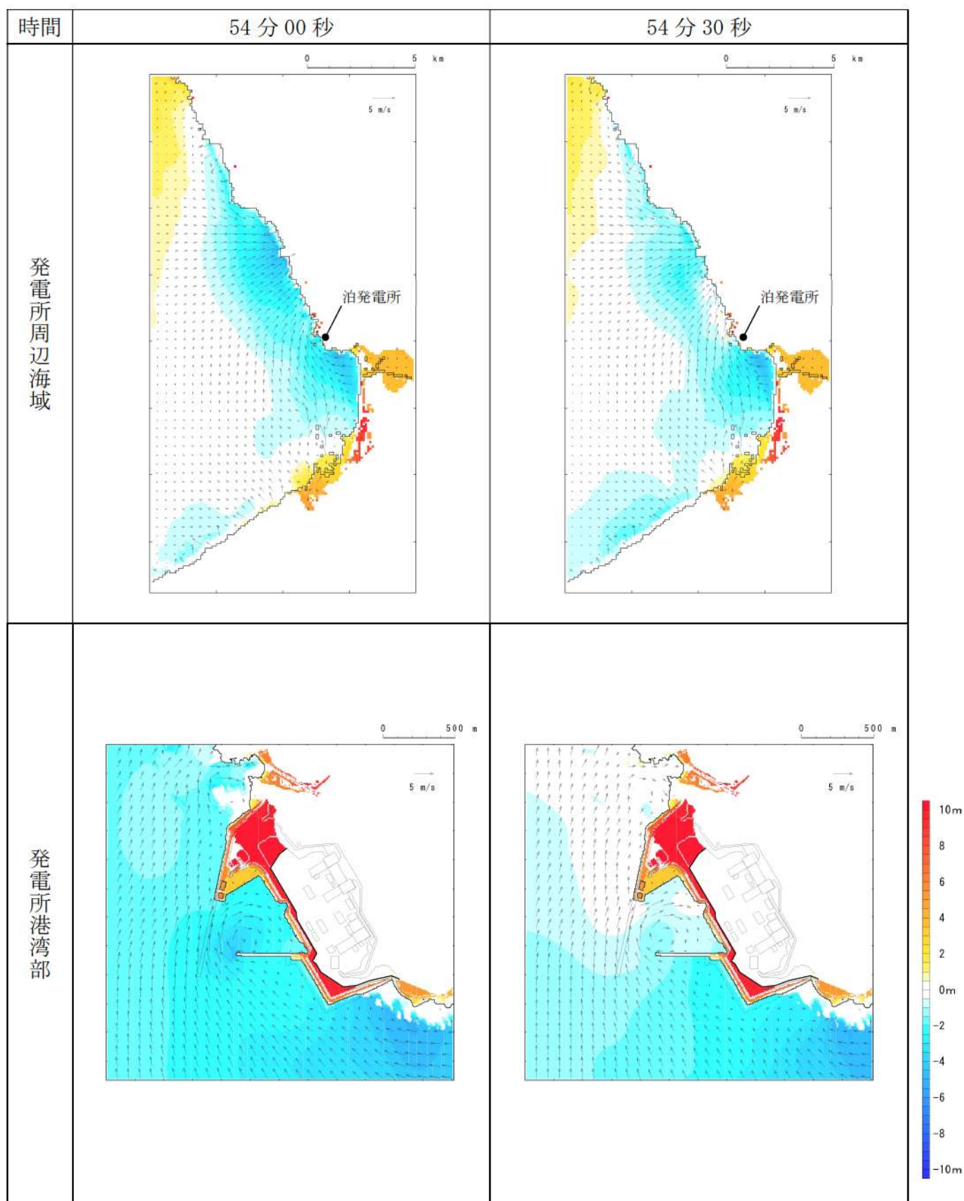
第3図-47 基準津波B（北防波堤損傷）の水位変動・流向ベクトル(47/53)
