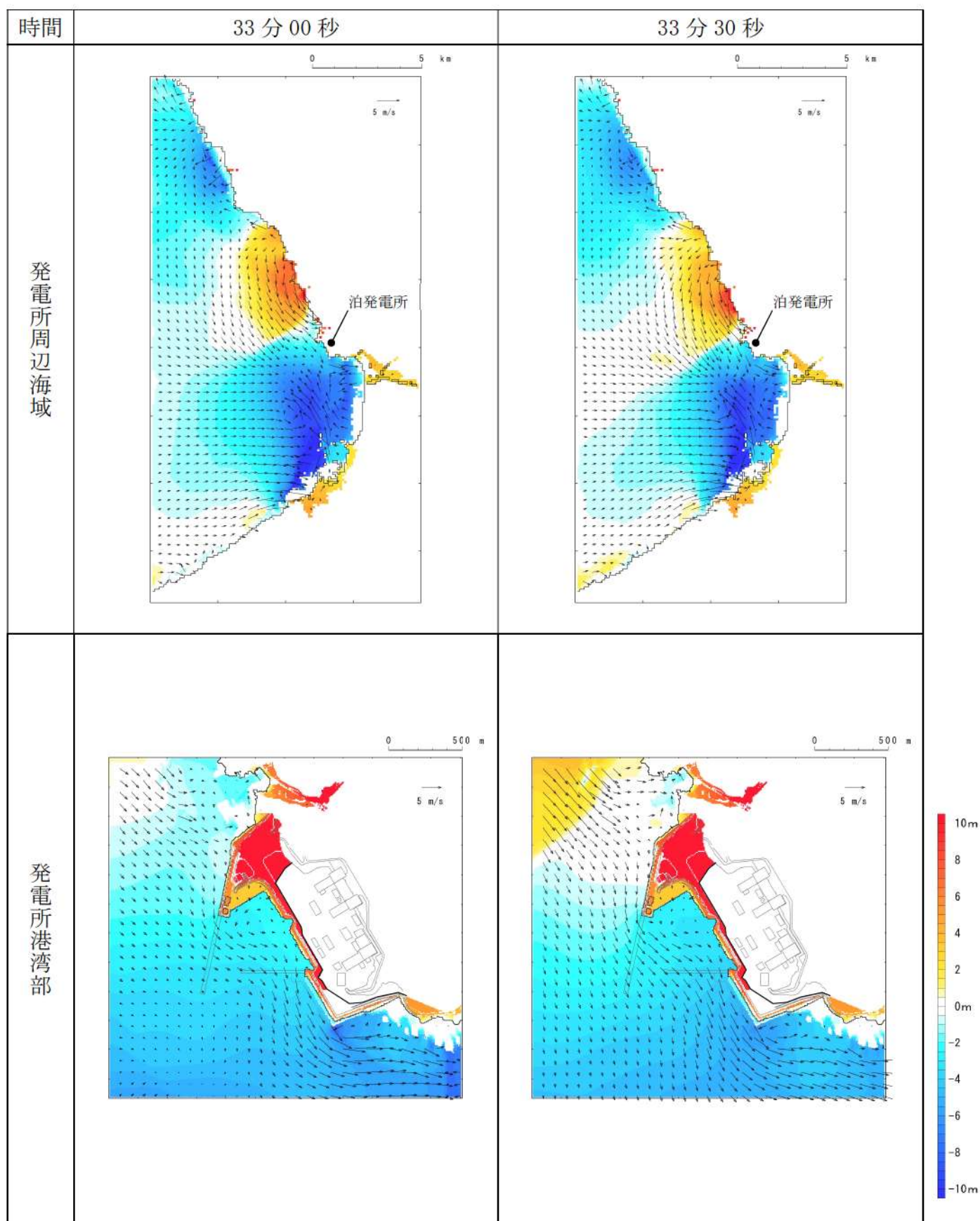
第 6 図-26 基準津波 D（北及び南防波堤損傷）の水位変動・流向ベクトル (26/53)
