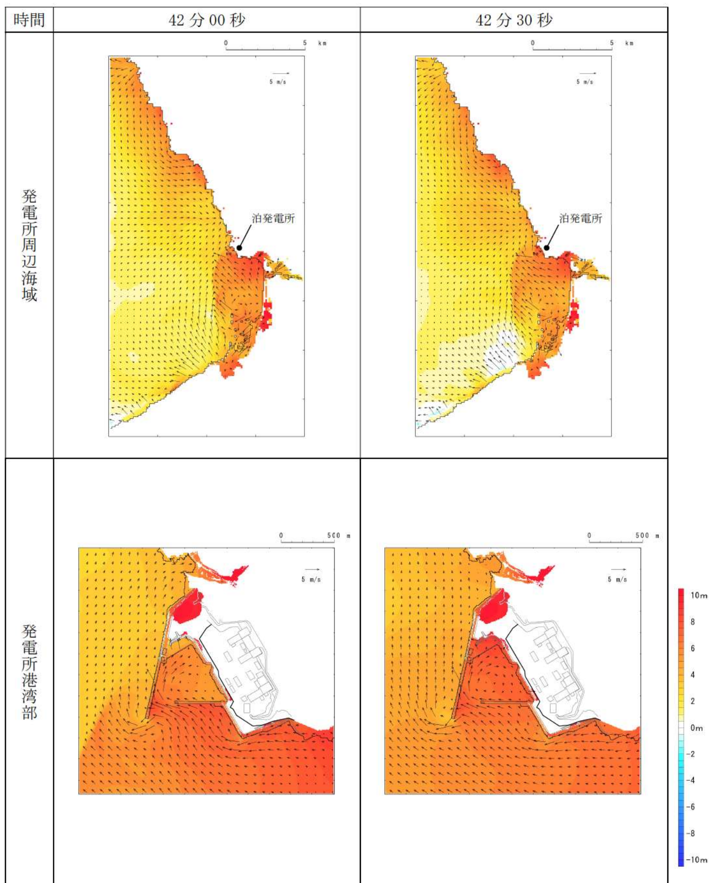
第 5 図-35 基準津波 D（防波堤損傷なし）の水位変動・流向ベクトル (35/53)
