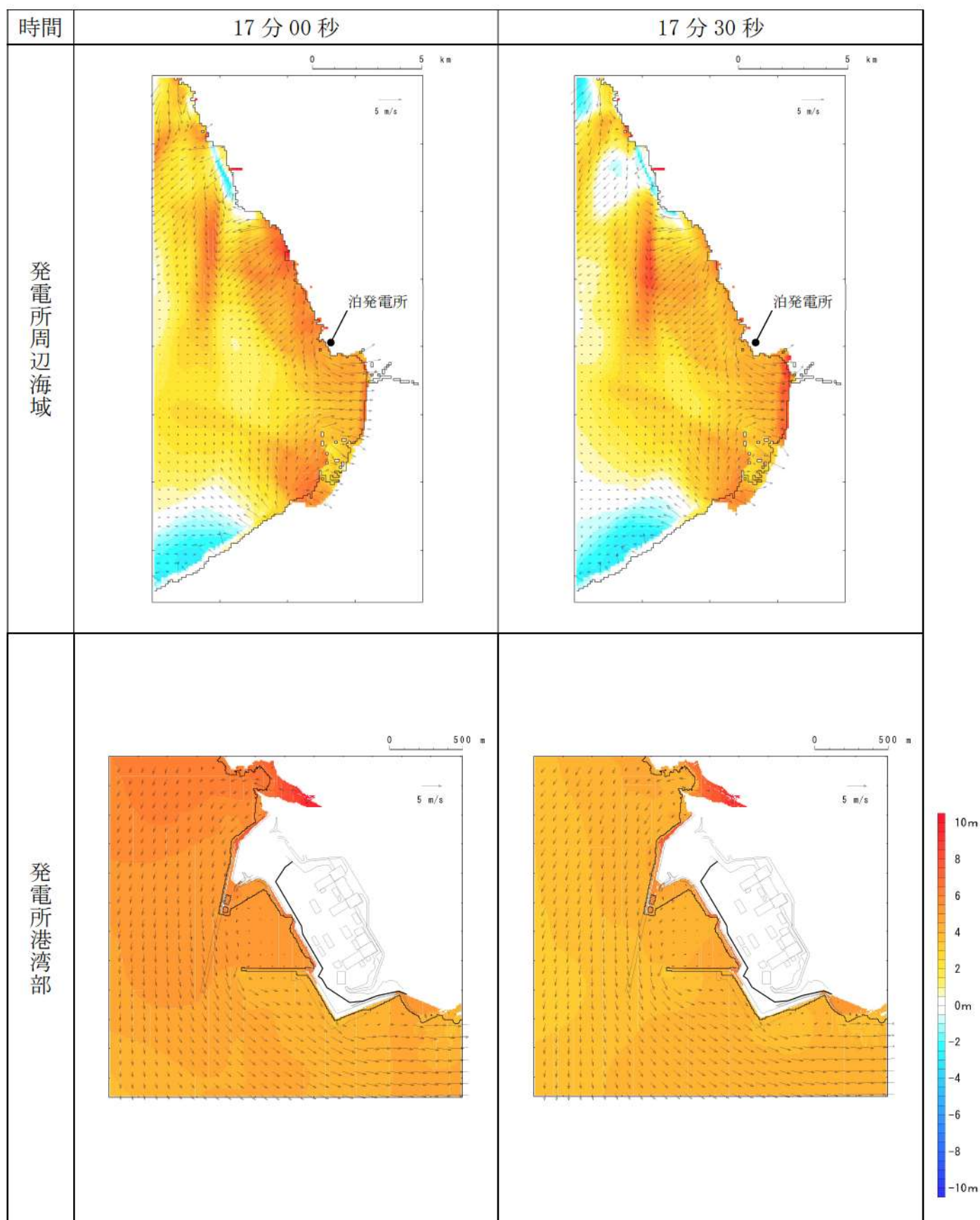
第3図-10 基準津波B（北防波堤損傷）の水位変動・流向ベクトル(10/53)
