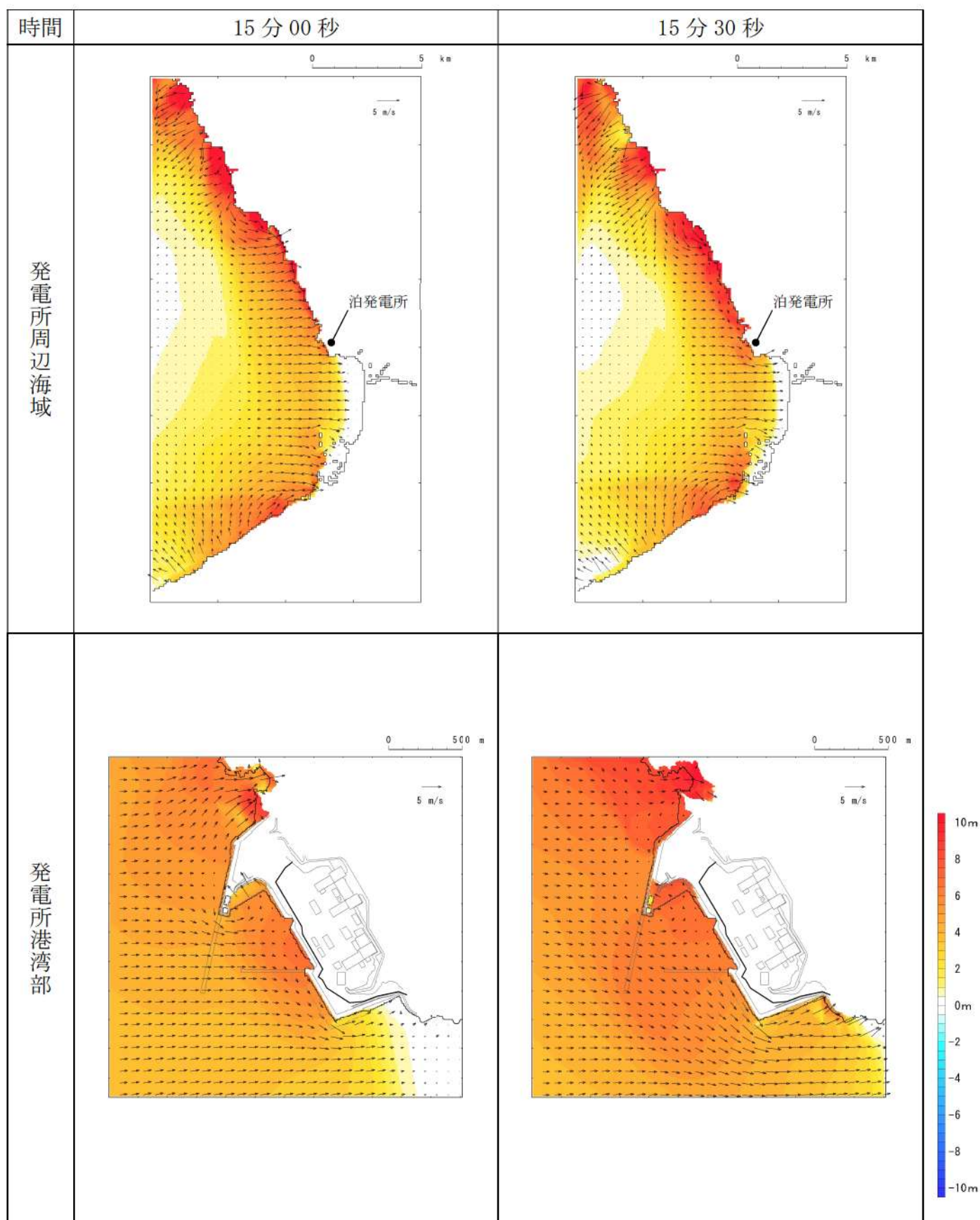
第 6 図- 8 基準津波 D（北及び南防波堤損傷）の水位変動・流向ベクトル (8/53)
