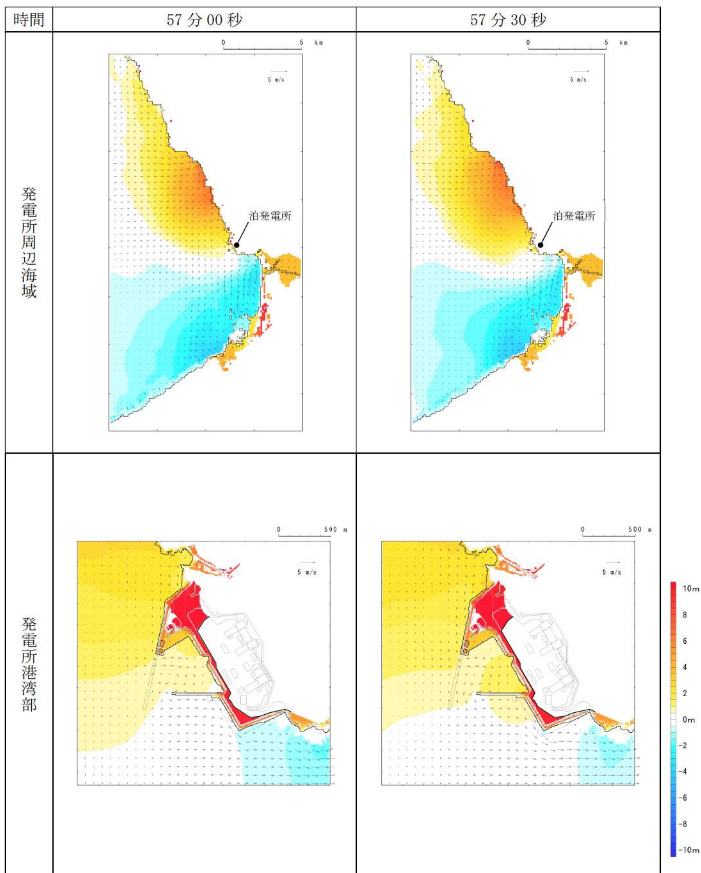
第3図-50 基準津波B（北防波堤損傷）の水位変動・流向ベクトル(50/53)
