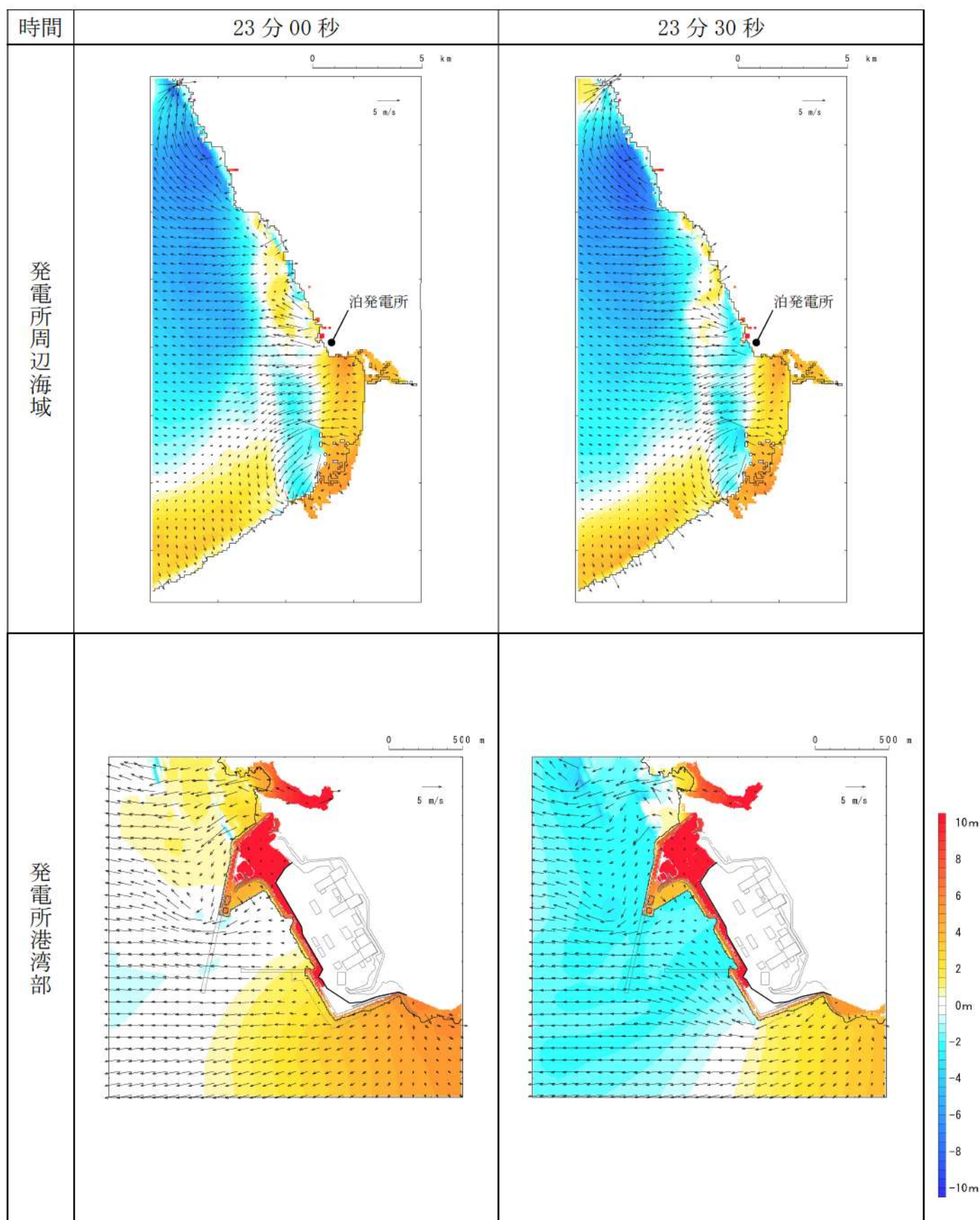
第 6 図-16 基準津波 D（北及び南防波堤損傷）の水位変動・流向ベクトル(16/53)
