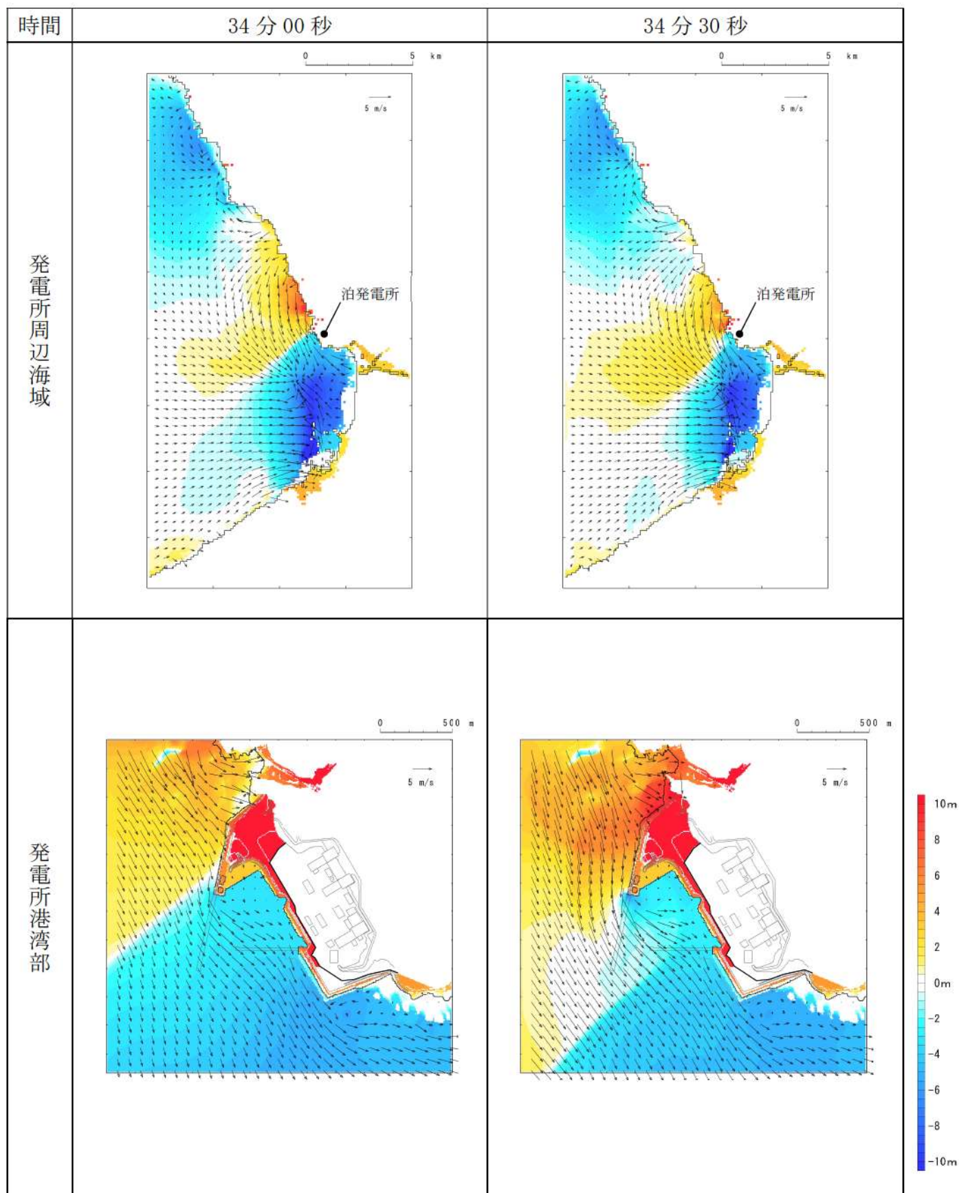
第 6 図-27 基準津波 D（北及び南防波堤損傷）の水位変動・流向ベクトル (27/53)
