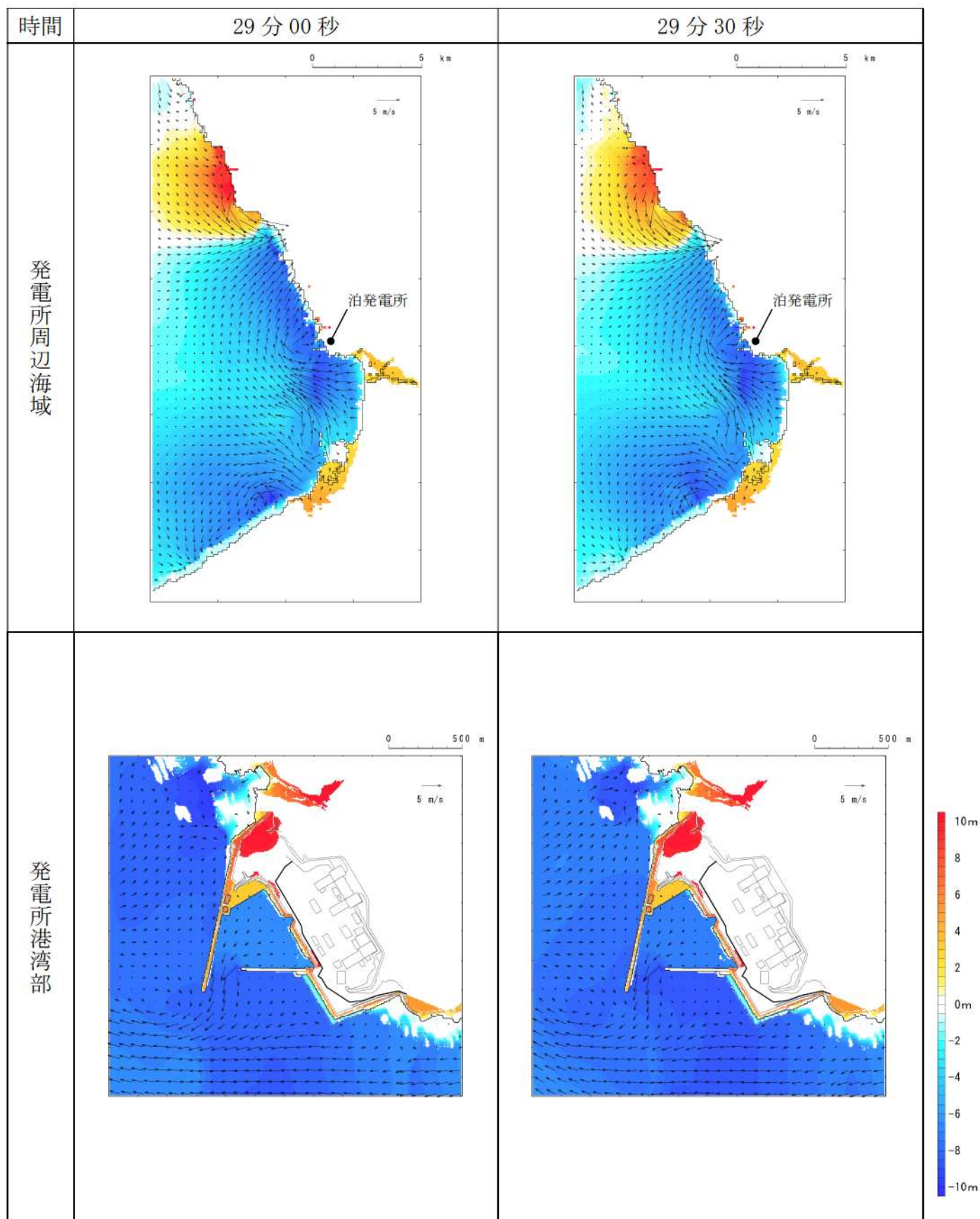
第 5 図-22 基準津波 D（防波堤損傷なし）の水位変動・流向ベクトル (22/53)
