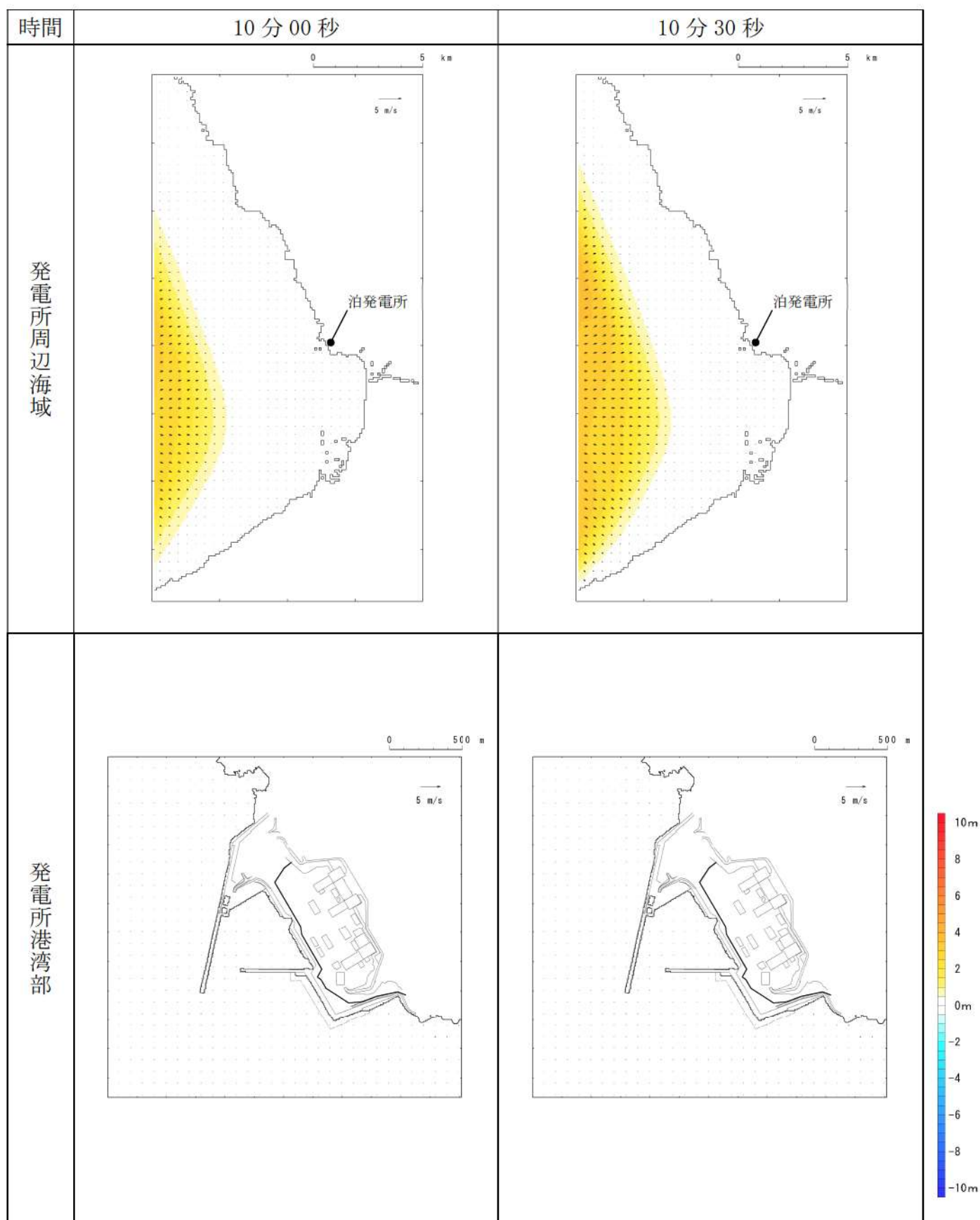
第5図-3 基準津波D（防波堤損傷なし）の水位変動・流向ベクトル(3/53)
