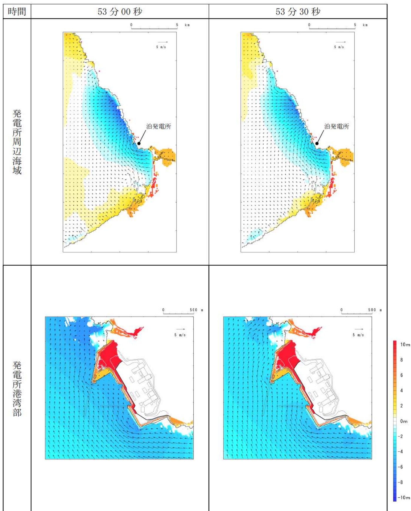
第 6 図-46 基準津波 D（北及び南防波堤損傷）の水位変動・流向ベクトル(46/53)
