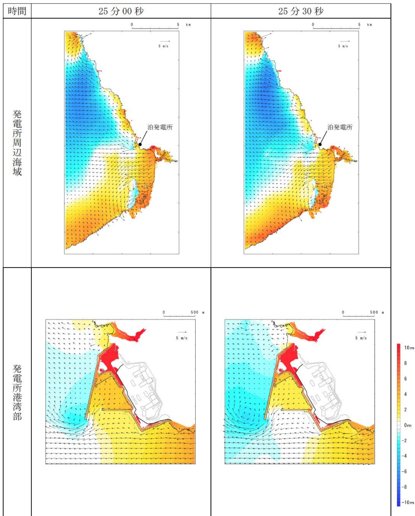
第4図-19 基準津波C（防波堤損傷なし）の水位変動・流向ベクトル(19/54)
