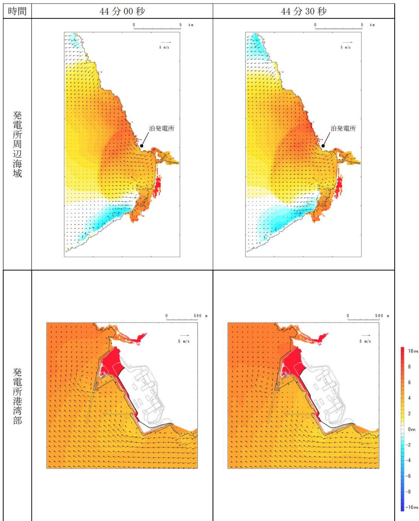
第 6 図-37 基準津波 D（北及び南防波堤損傷）の水位変動・流向ベクトル(37/53)
