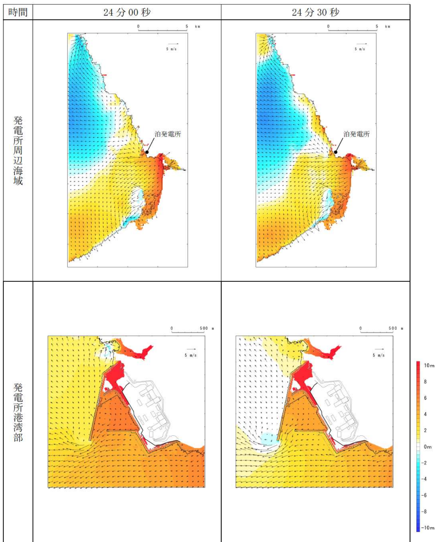
第 4 図-18 基準津波 C（防波堤損傷なし）の水位変動・流向ベクトル(18/54)
