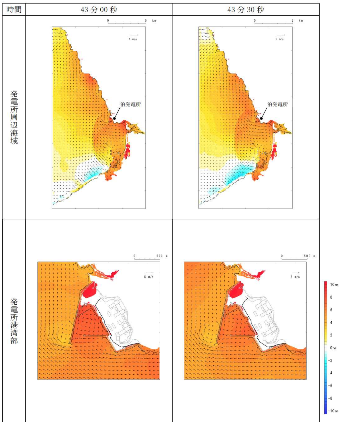
第 5 図-36 基準津波 D（防波堤損傷なし）の水位変動・流向ベクトル (36/53)
