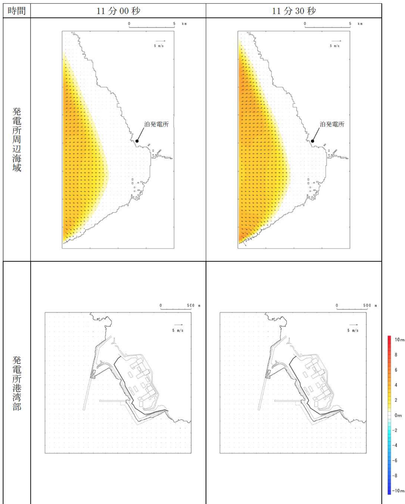
第 6 図-4 基準津波 D（北及び南防波堤損傷）の水位変動・流向ベクトル(4/53)
