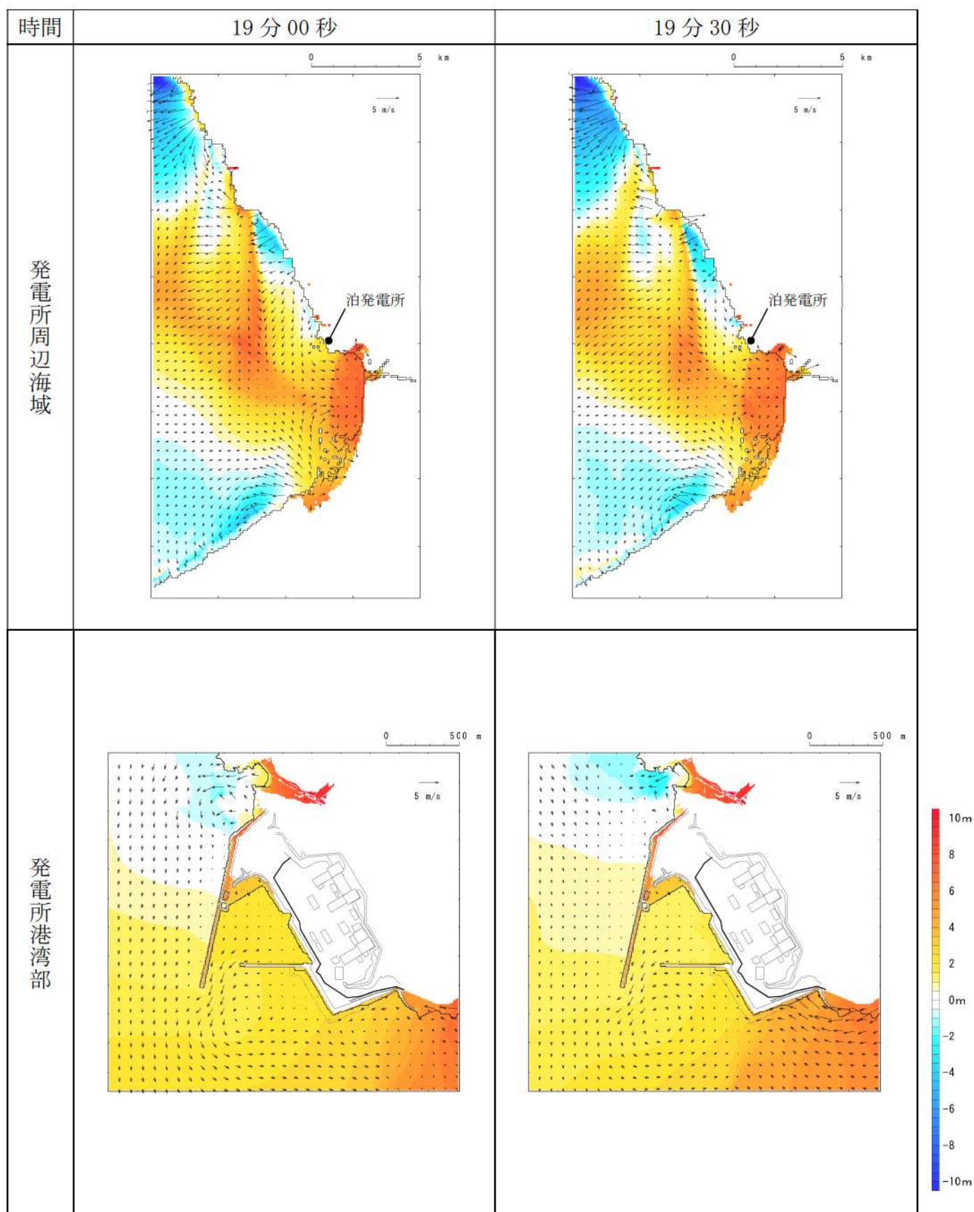
第 5 図-12 基準津波 D（防波堤損傷なし）の水位変動・流向ベクトル(12/53)
