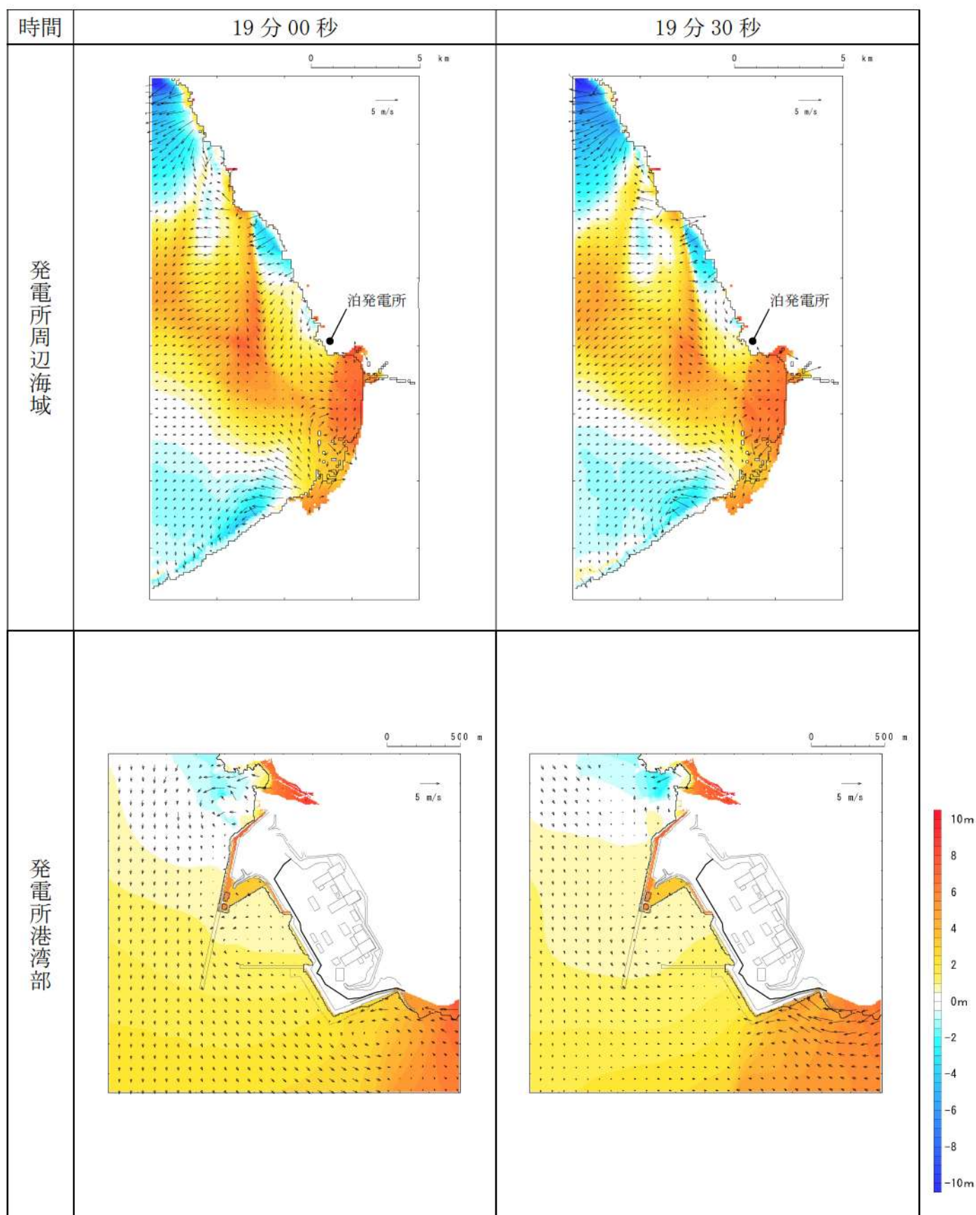
第 6 図-12 基準津波 D（北及び南防波堤損傷）の水位変動・流向ベクトル(12/53)
