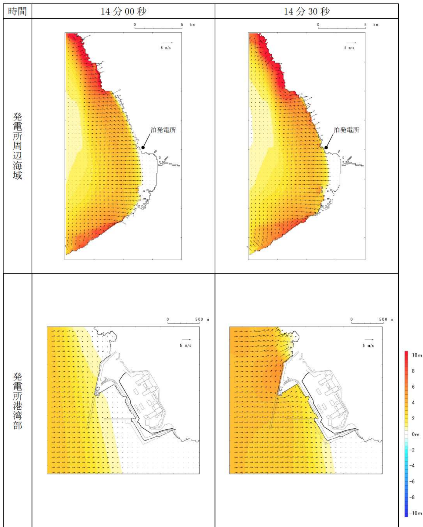
第 6 図- 7 基準津波 D（北及び南防波堤損傷）の水位変動・流向ベクトル (7/53)
