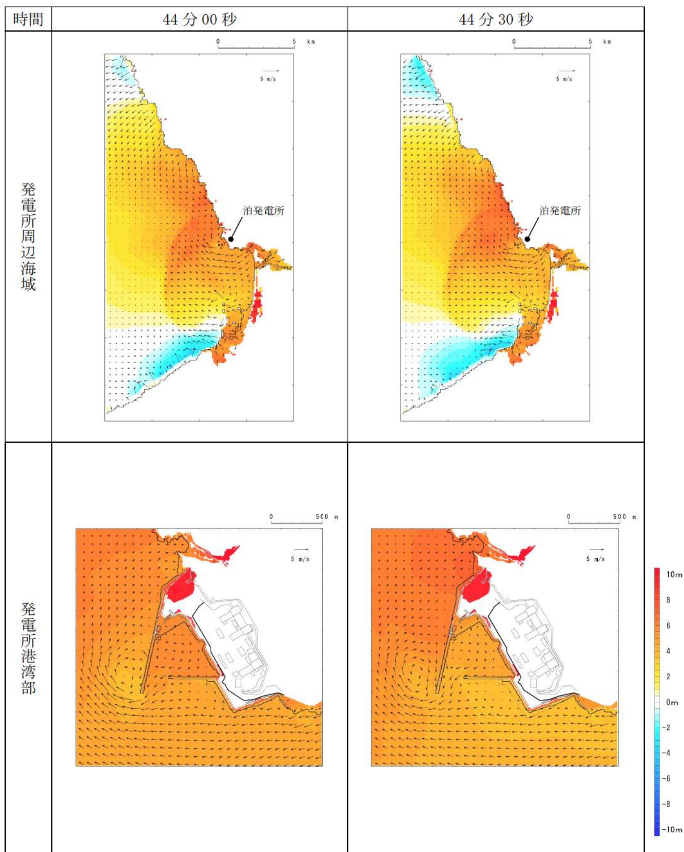
第 5 図-37 基準津波 D (防波堤損傷なし) の水位変動・流向ベクトル (37/53)
