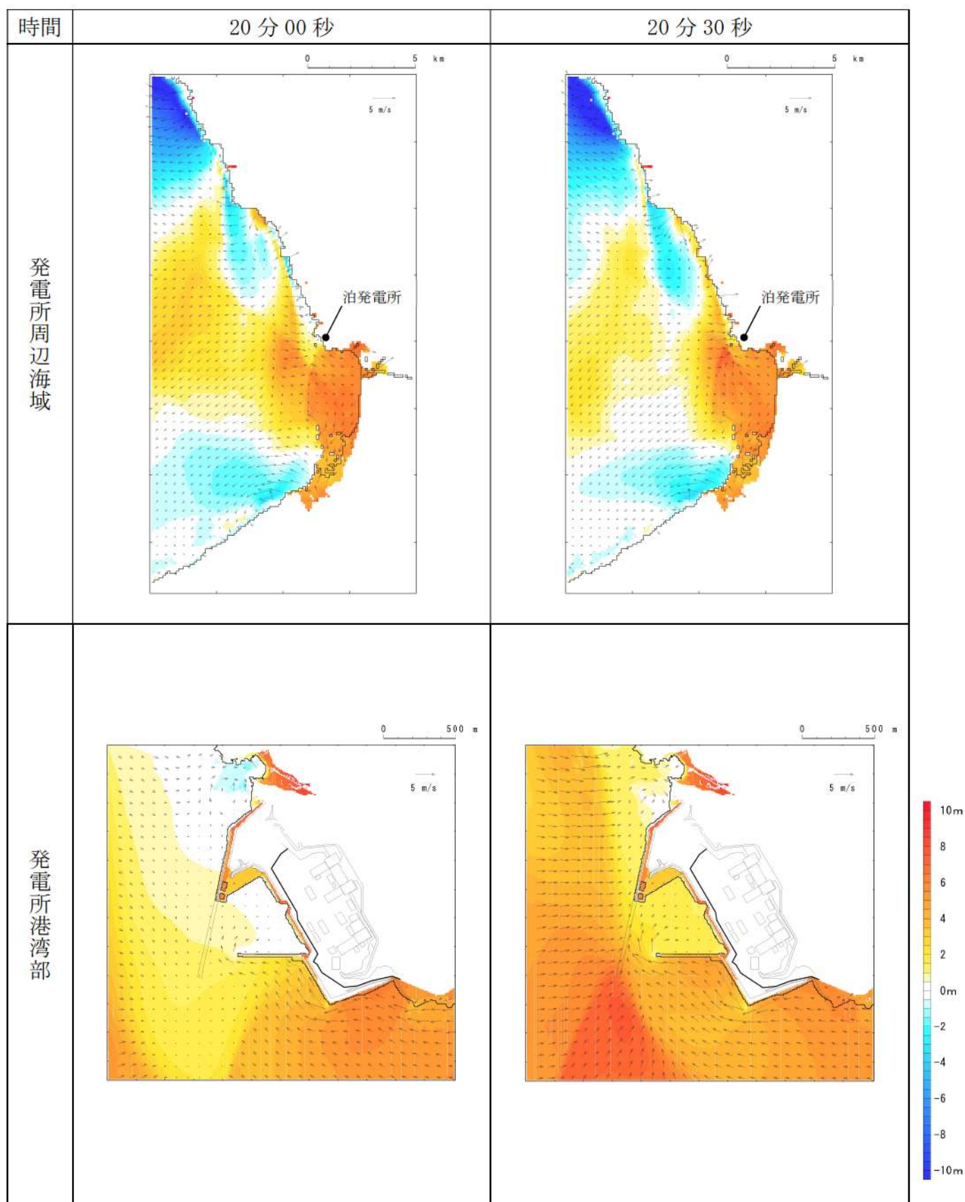
第3図-13 基準津波B（北防波堤損傷）の水位変動・流向ベクトル(13/53)
