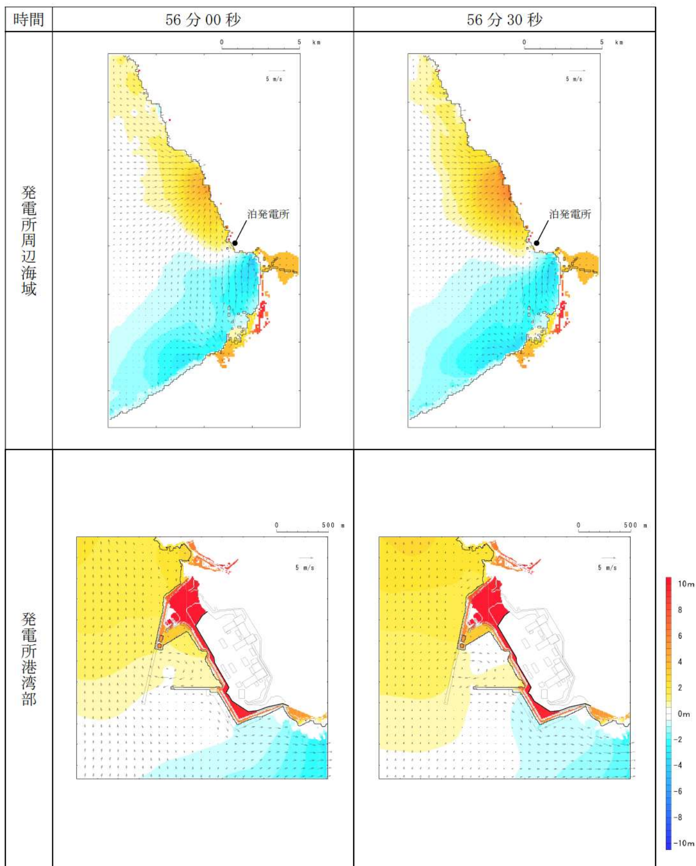
第3図-49 基準津波B（北防波堤損傷）の水位変動・流向ベクトル(49/53)
