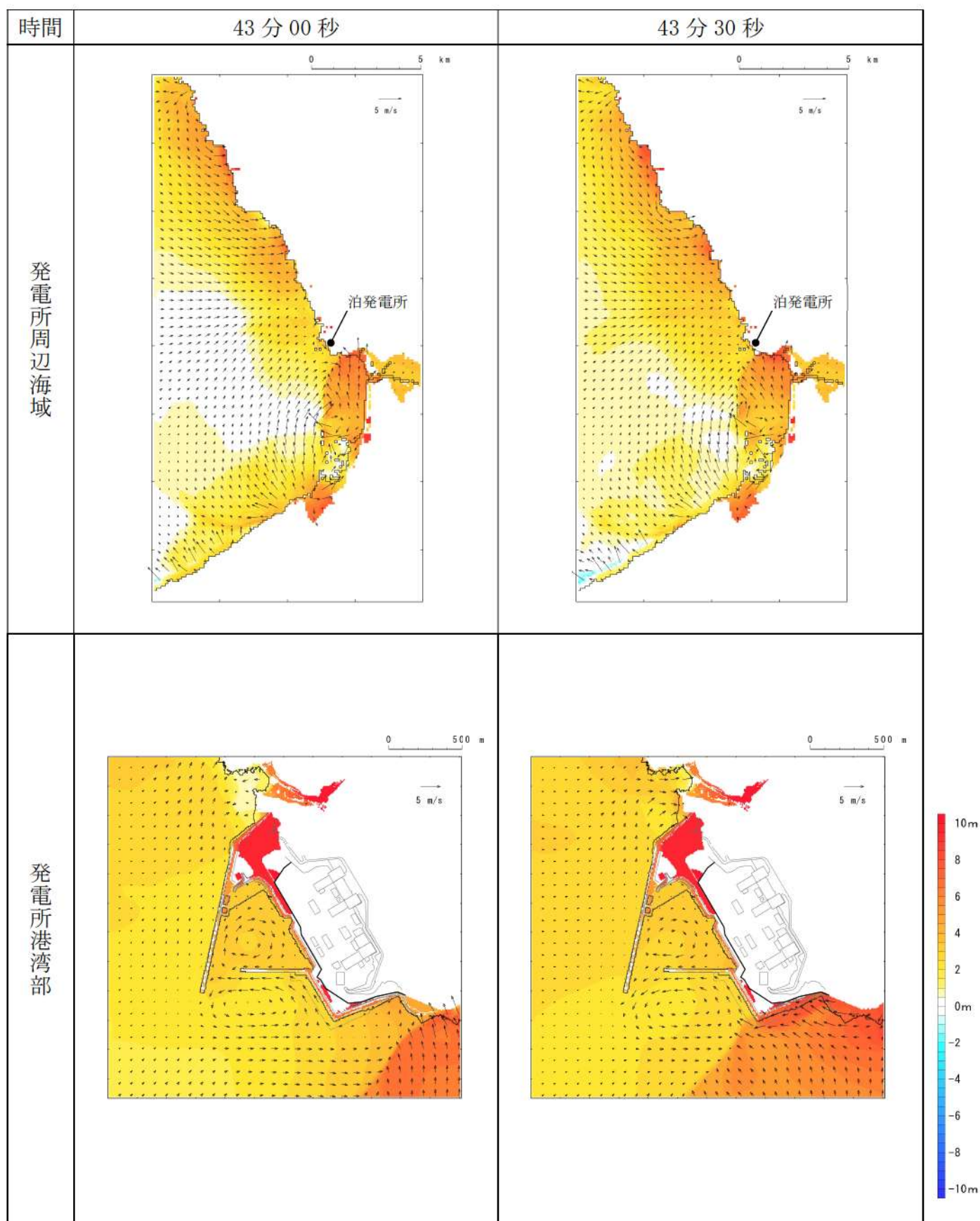
第4図-37 基準津波C（防波堤損傷なし）の水位変動・流向ベクトル(37/54)
