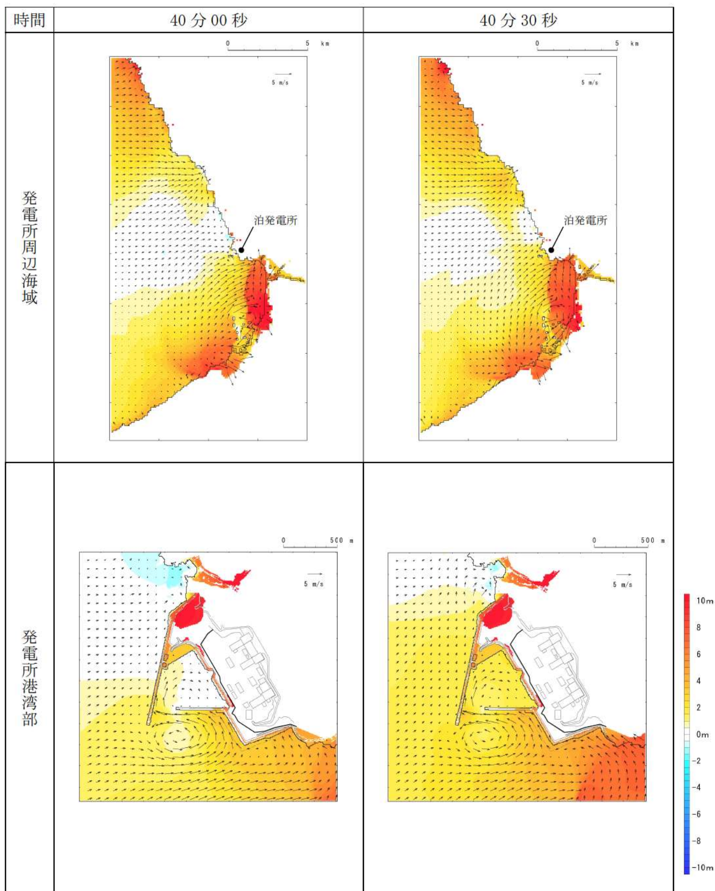
第 5 図-33 基準津波 D (防波堤損傷なし) の水位変動・流向ベクトル (33/53)
