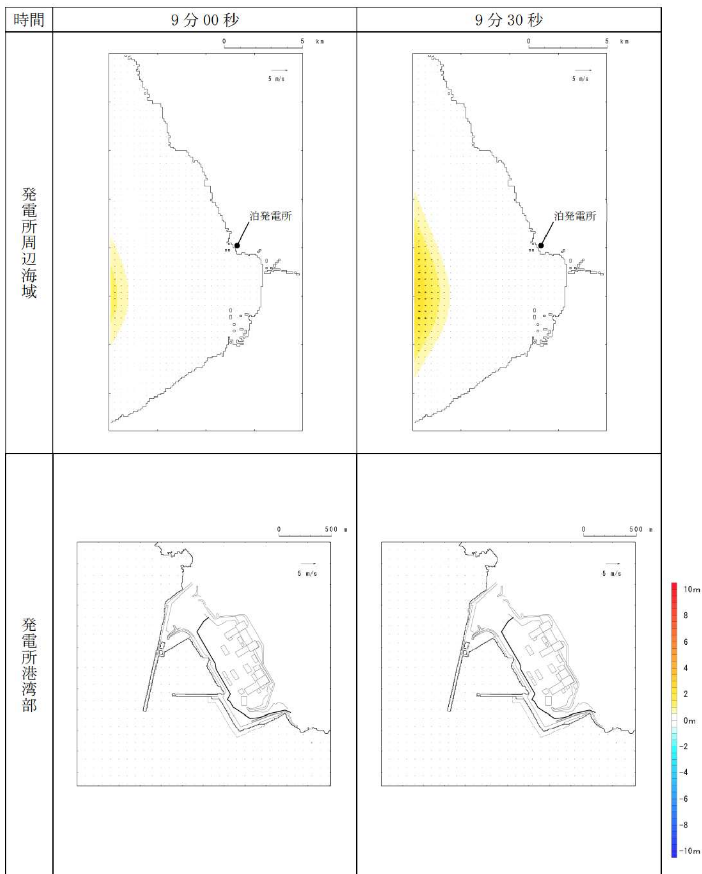
第5図-2 基準津波D（防波堤損傷なし）の水位変動・流向ベクトル(2/53)
