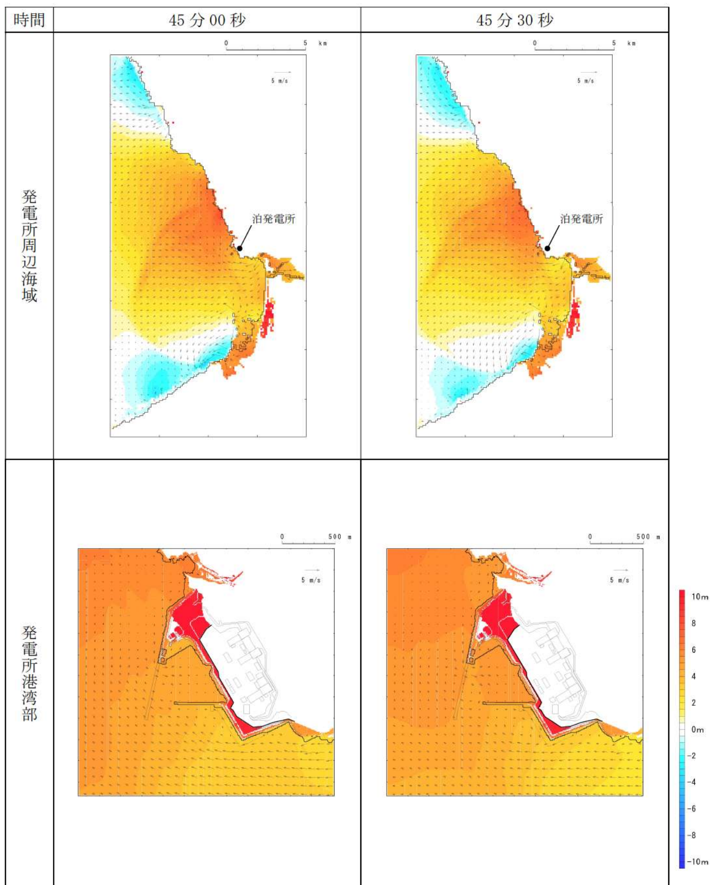
第3図-38 基準津波B（北防波堤損傷）の水位変動・流向ベクトル(38/53)
