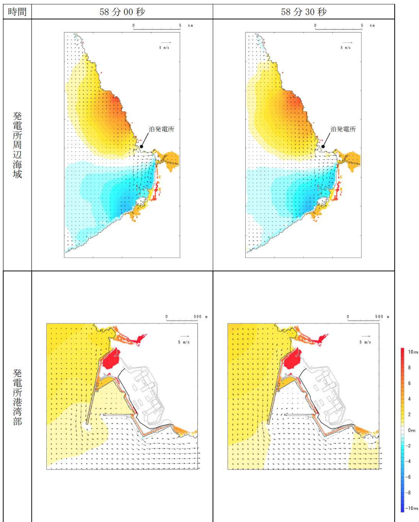
第 5 図-51 基準津波 D（防波堤損傷なし）の水位変動・流向ベクトル (51/53)
