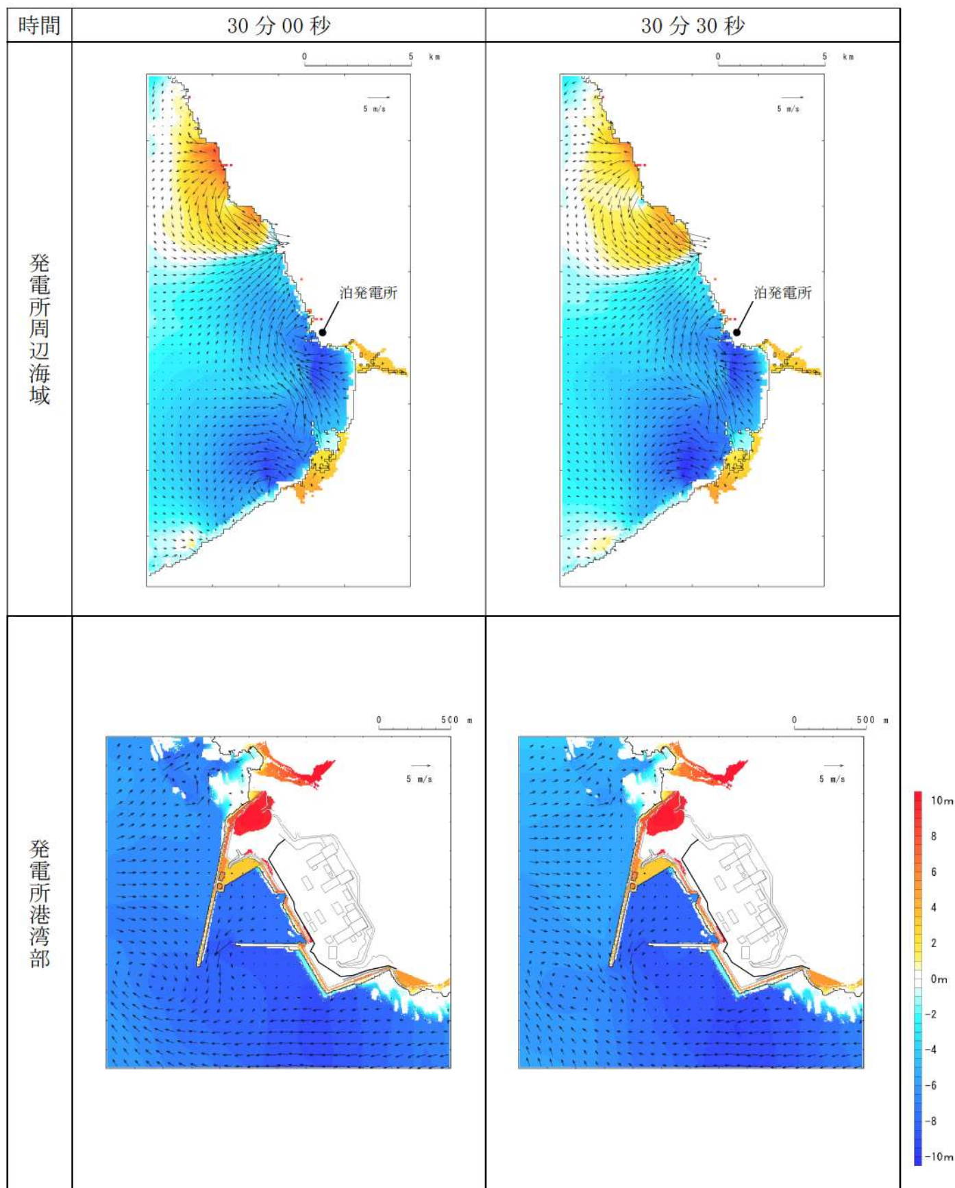
第 5 図-23 基準津波 D（防波堤損傷なし）の水位変動・流向ベクトル (23/53)
