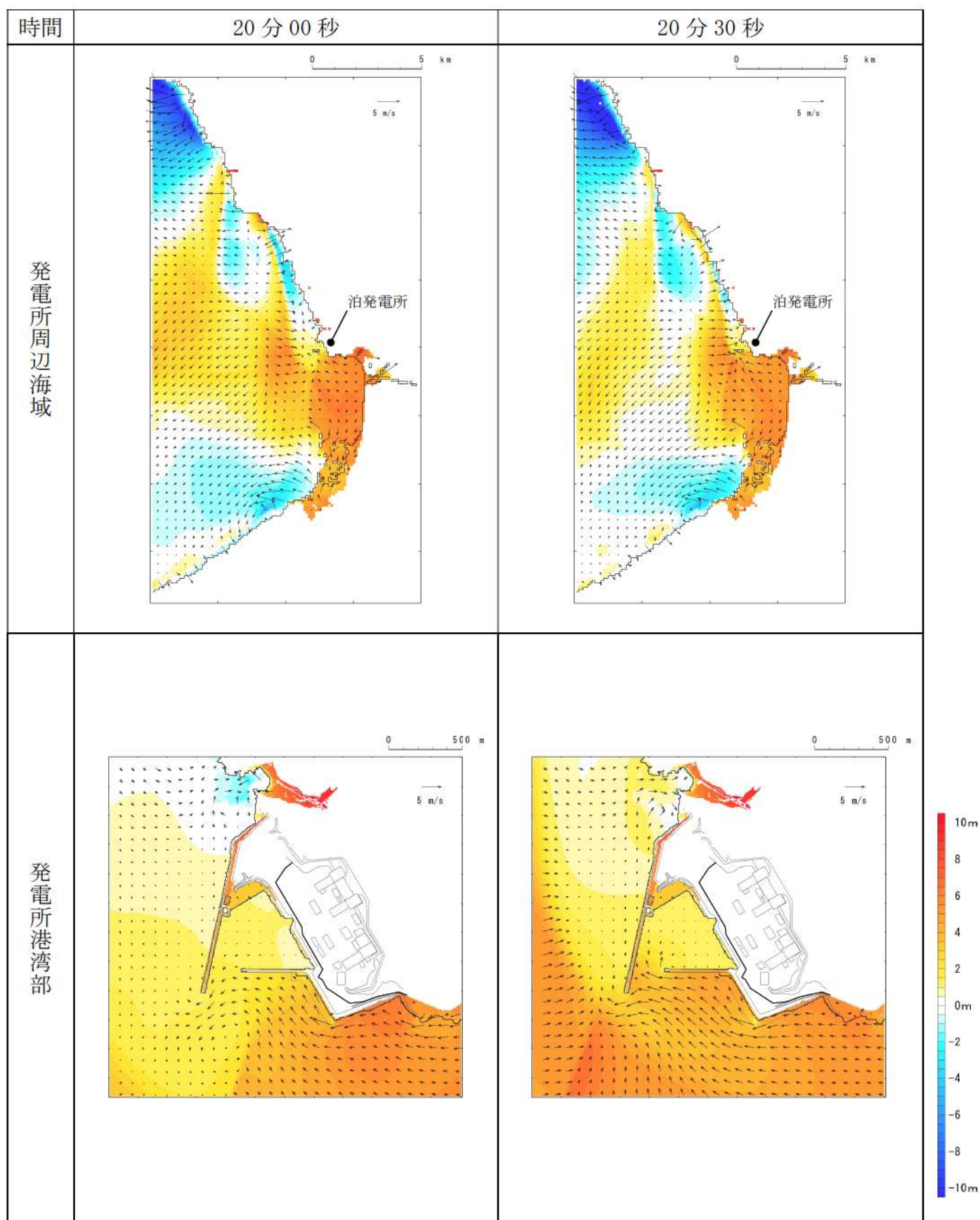
第 5 図-13 基準津波 D（防波堤損傷なし）の水位変動・流向ベクトル(13/53)
