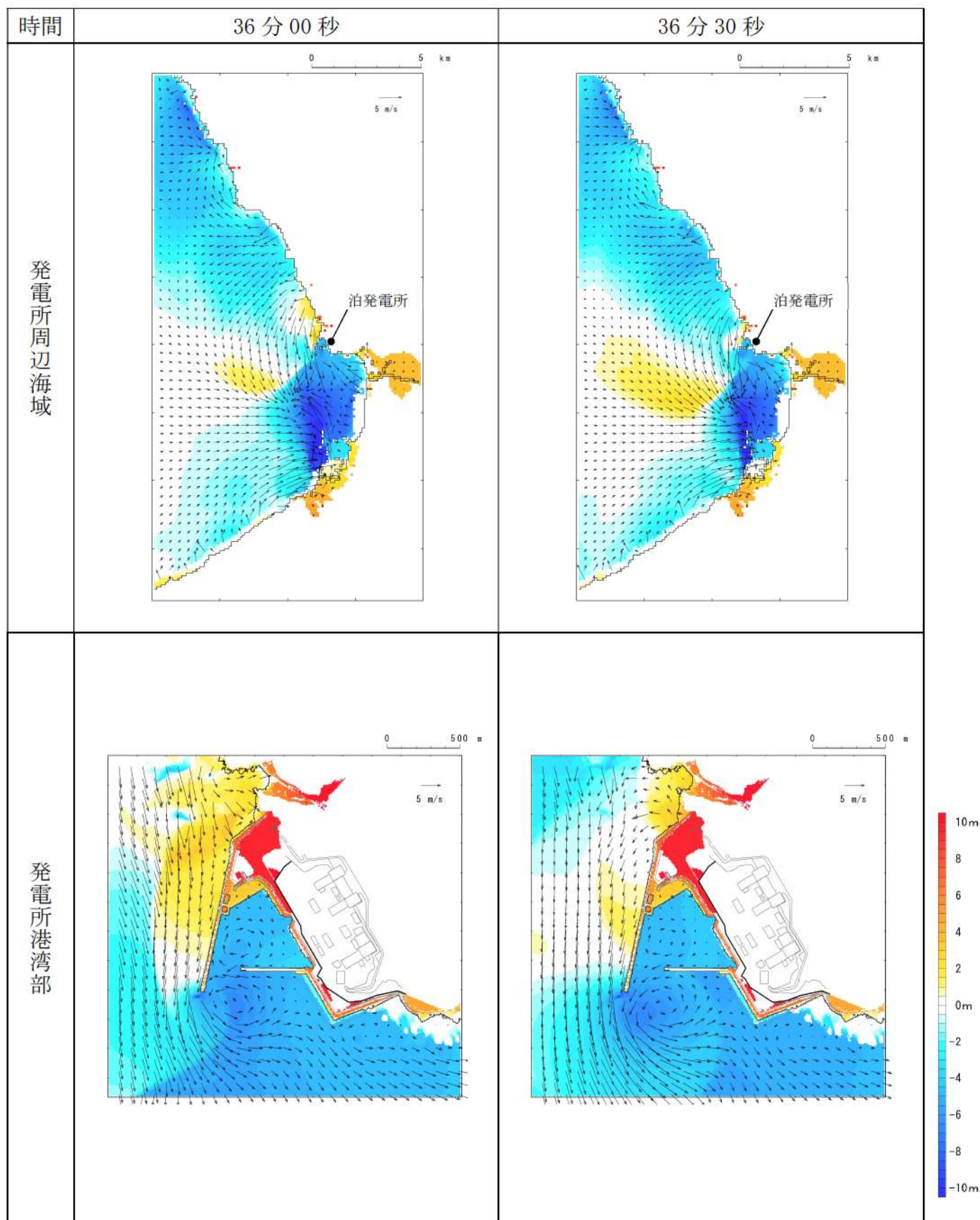
第 4 図-30 基準津波 C（防波堤損傷なし）の水位変動・流向ベクトル(30/54)
