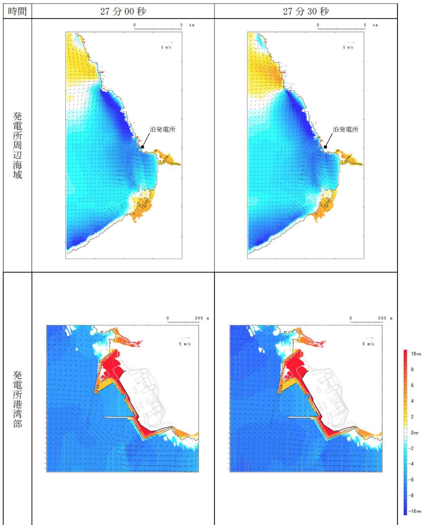
第3図-20 基準津波B（北防波堤損傷）の水位変動・流向ベクトル(20/53)
