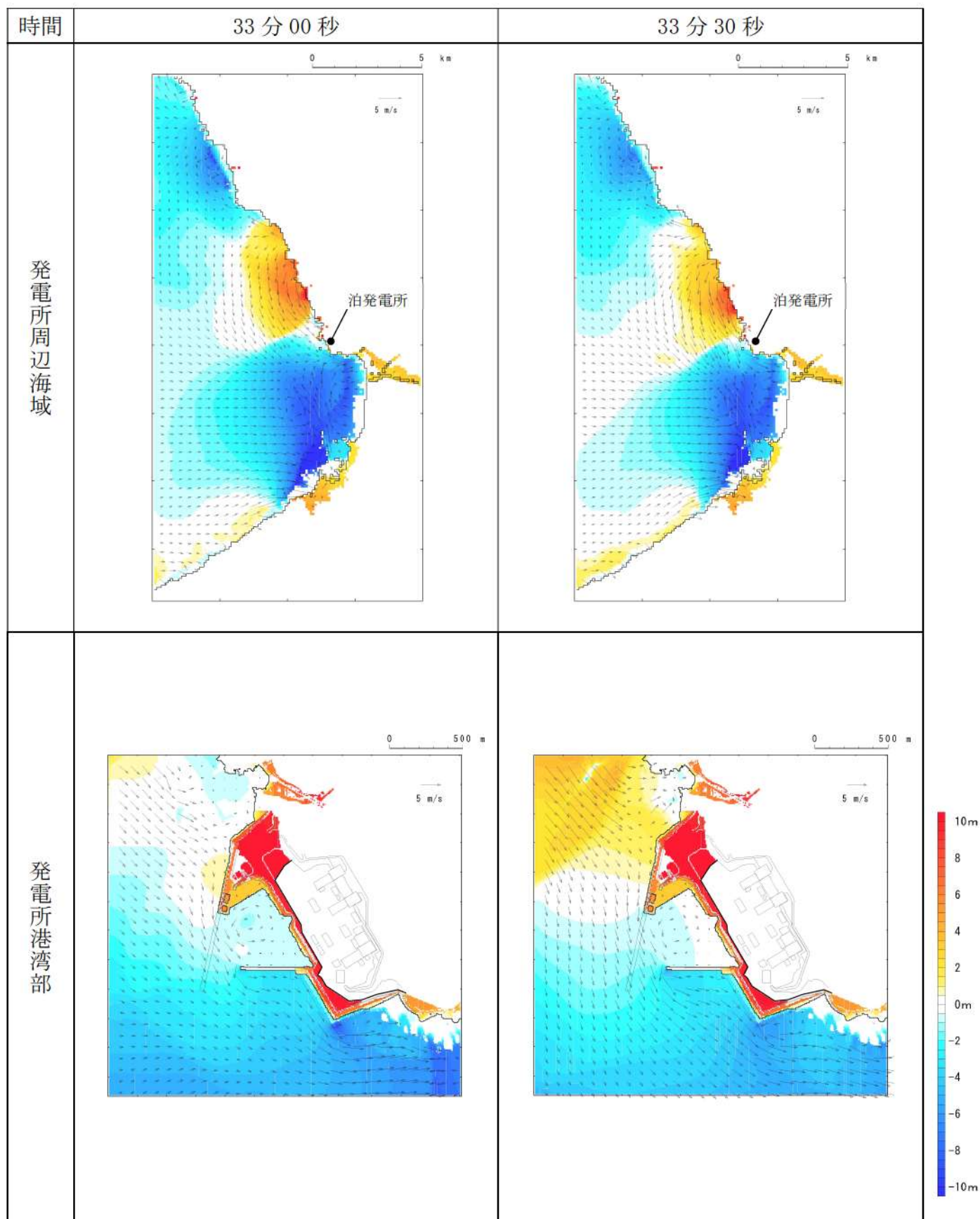
第3図-26 基準津波B（北防波堤損傷）の水位変動・流向ベクトル(26/53)
