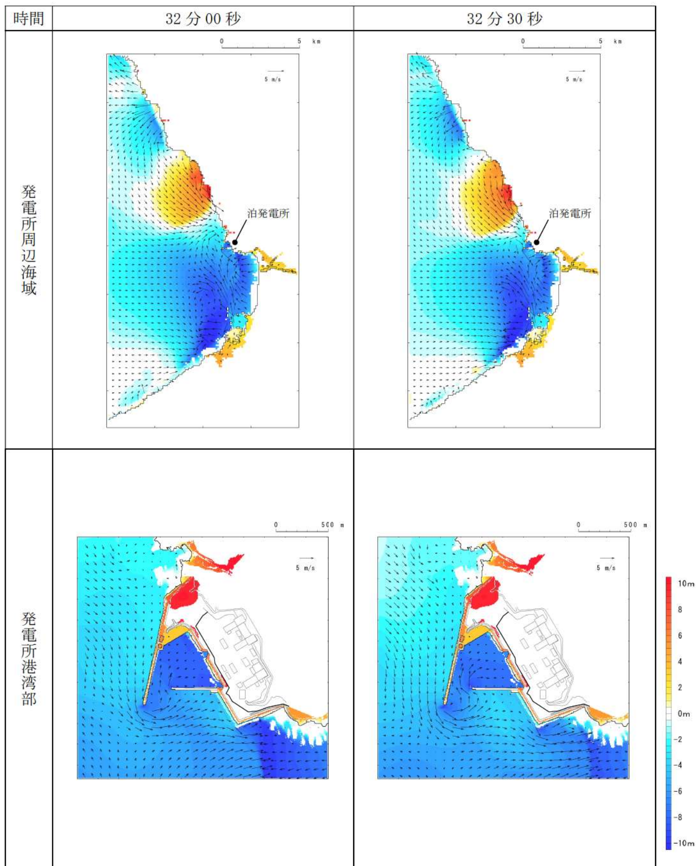
第 5 図-25 基準津波 D（防波堤損傷なし）の水位変動・流向ベクトル (25/53)
