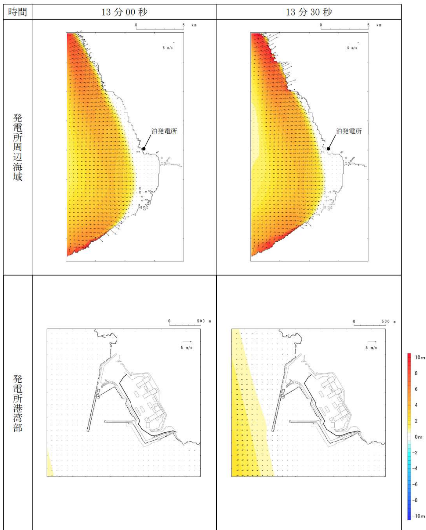
第5図-6 基準津波D（防波堤損傷なし）の水位変動・流向ベクトル(6/53)
