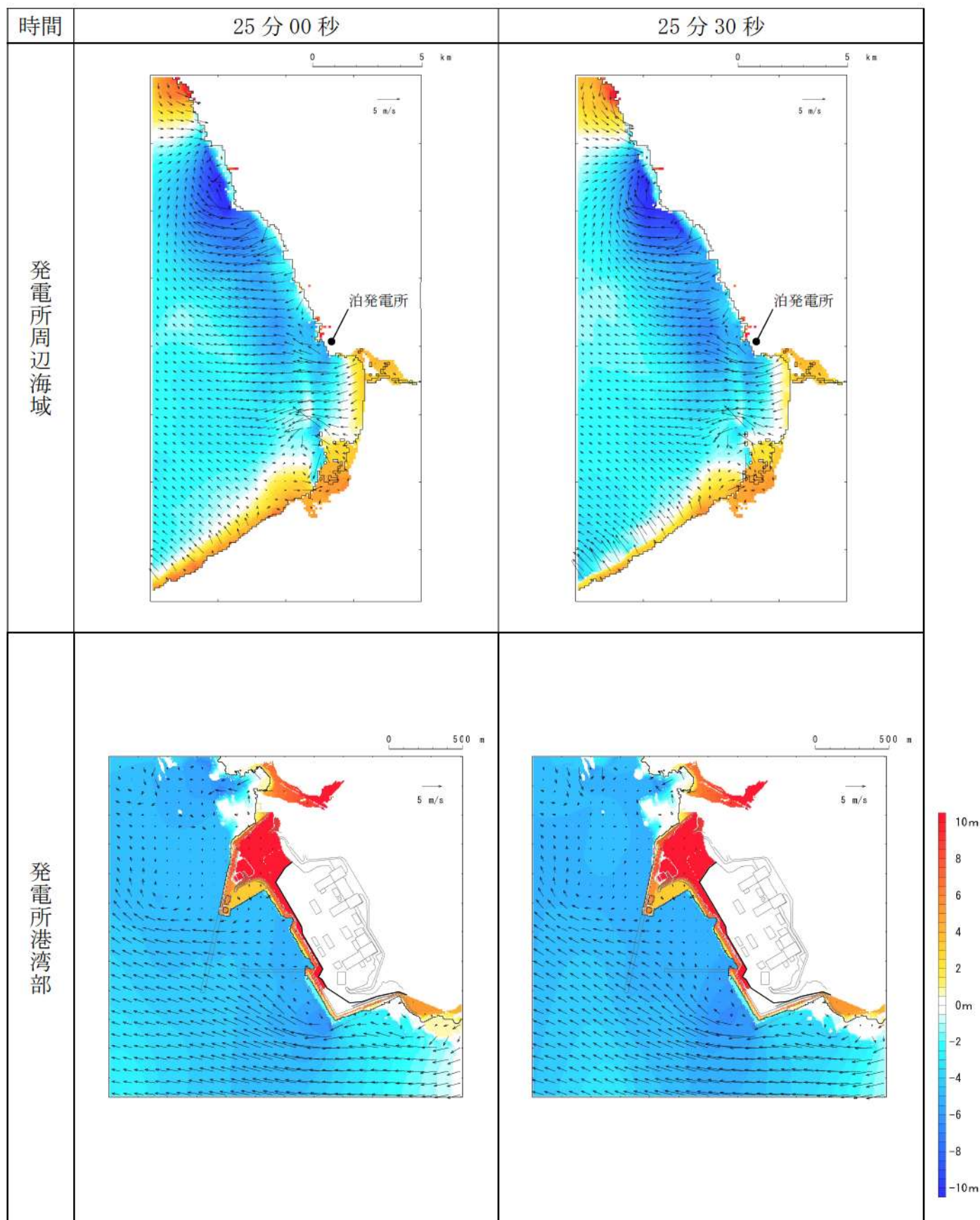
第 6 図-18 基準津波 D（北及び南防波堤損傷）の水位変動・流向ベクトル(18/53)
