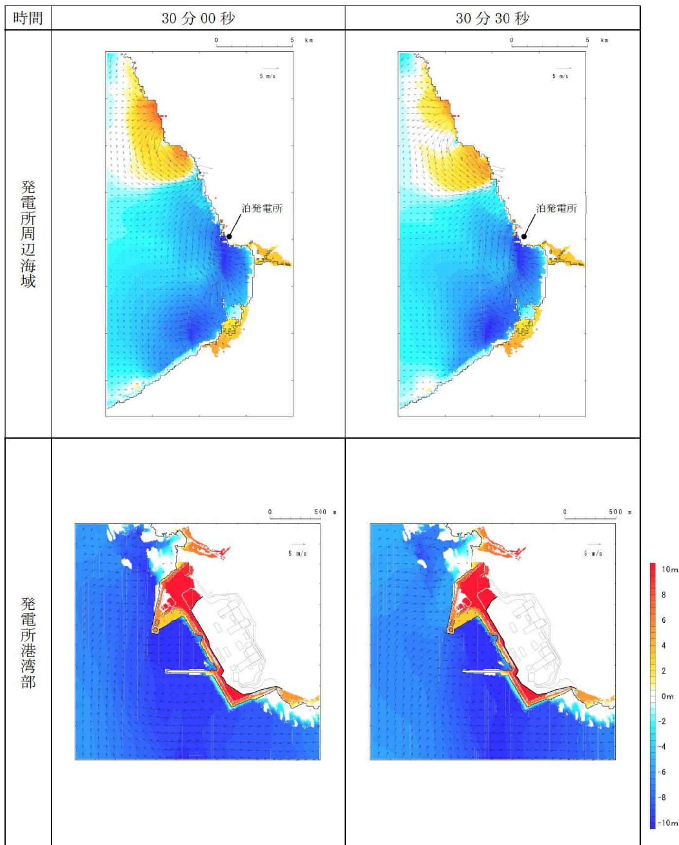
第3図-23 基準津波B（北防波堤損傷）の水位変動・流向ベクトル(23/53)
