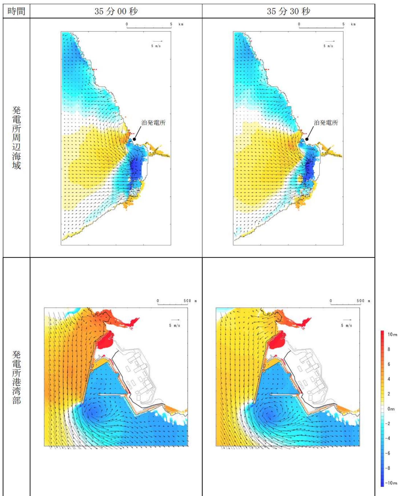
第 5 図-28 基準津波 D（防波堤損傷なし）の水位変動・流向ベクトル (28/53)
