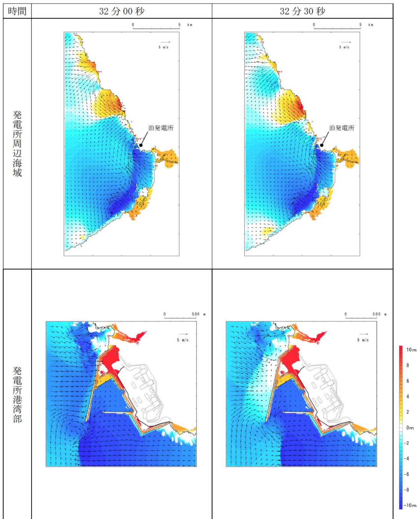
第4図-26 基準津波C（防波堤損傷なし）の水位変動・流向ベクトル(26/54)
