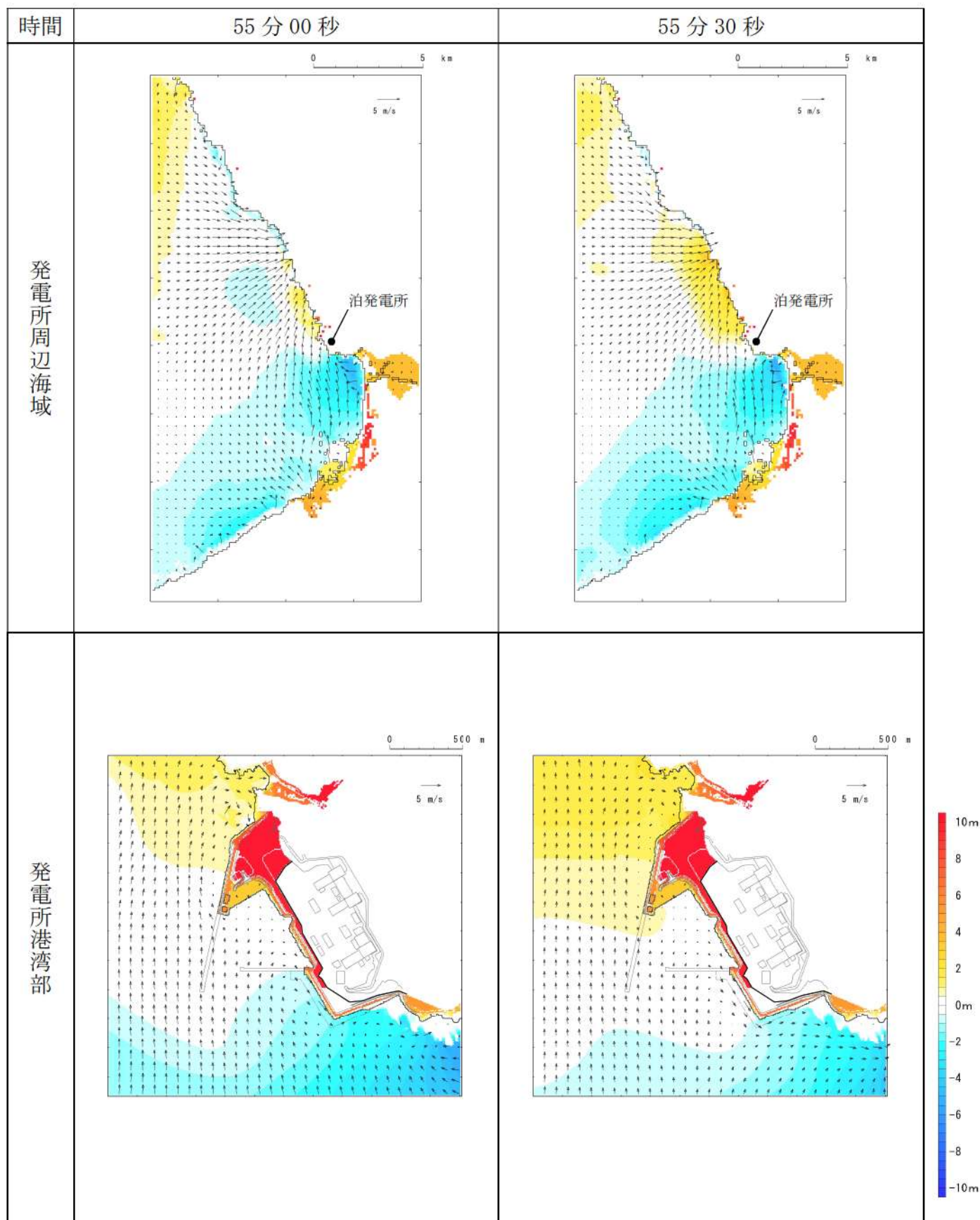
第 6 図-48 基準津波 D（北及び南防波堤損傷）の水位変動・流向ベクトル(48/53)
