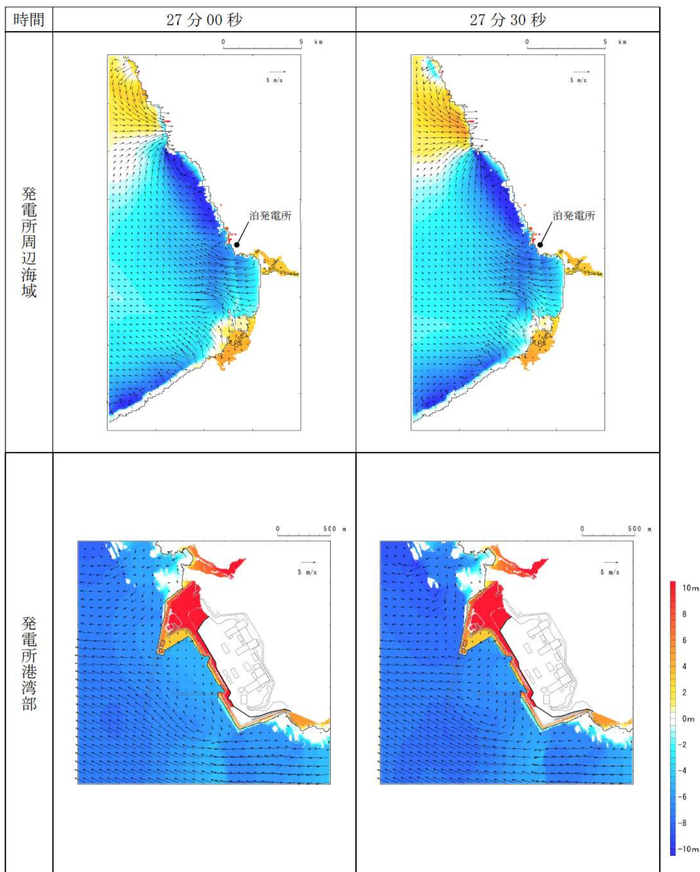
第 6 図-20 基準津波 D（北及び南防波堤損傷）の水位変動・流向ベクトル (20/53)
