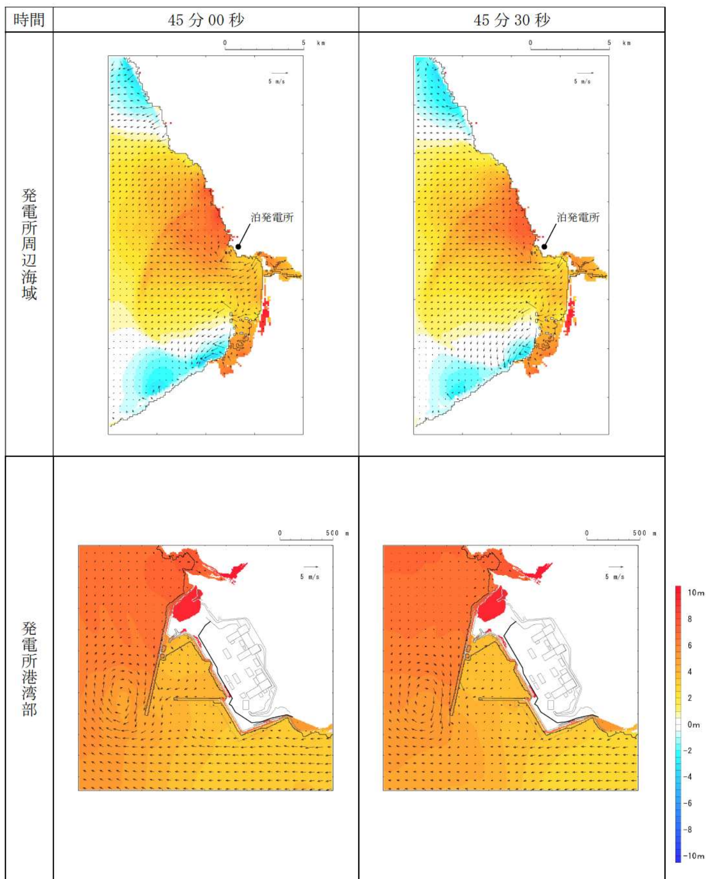
第 5 図-38 基準津波 D（防波堤損傷なし）の水位変動・流向ベクトル (38/53)
