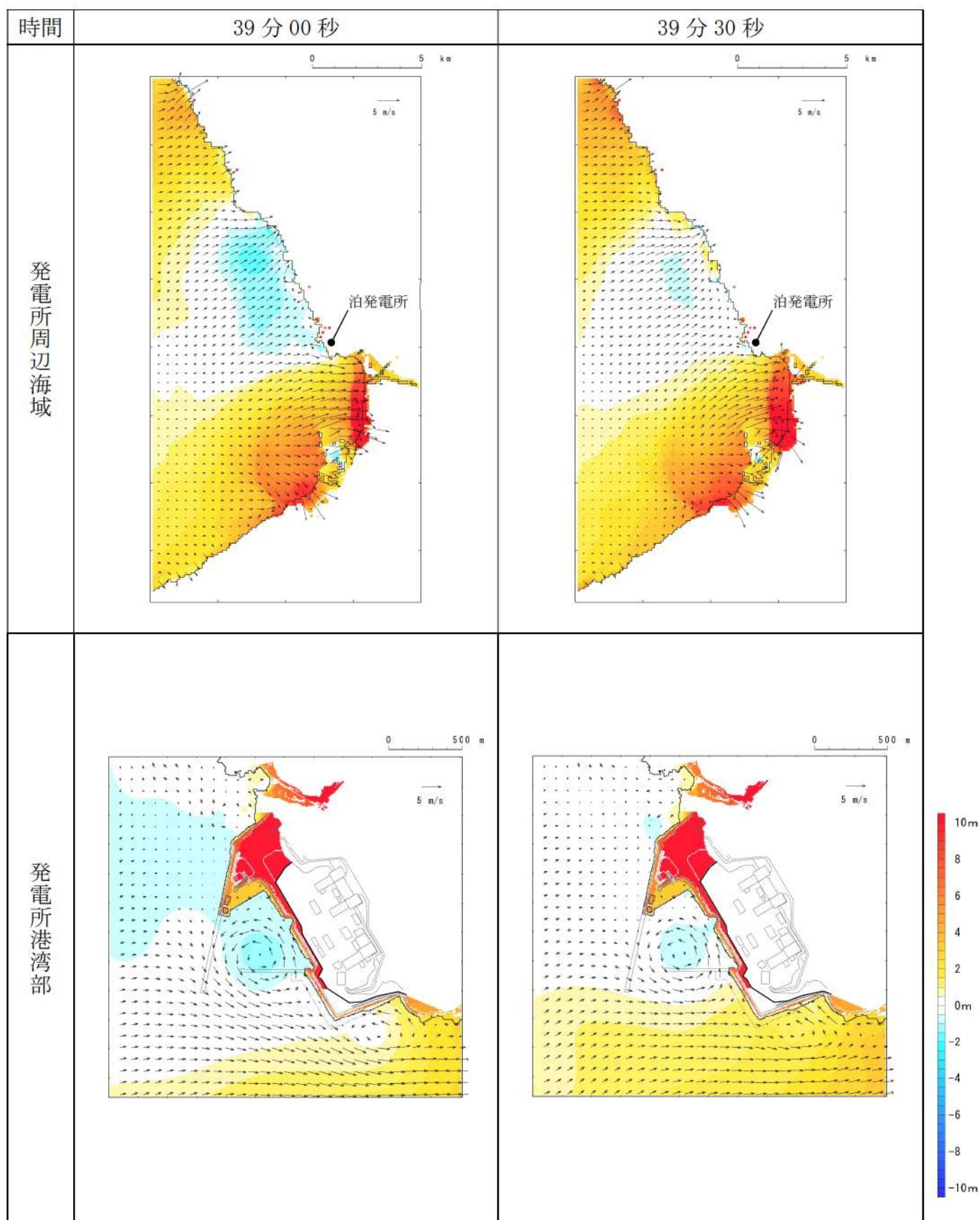
第 6 図-32 基準津波 D（北及び南防波堤損傷）の水位変動・流向ベクトル(32/53)
