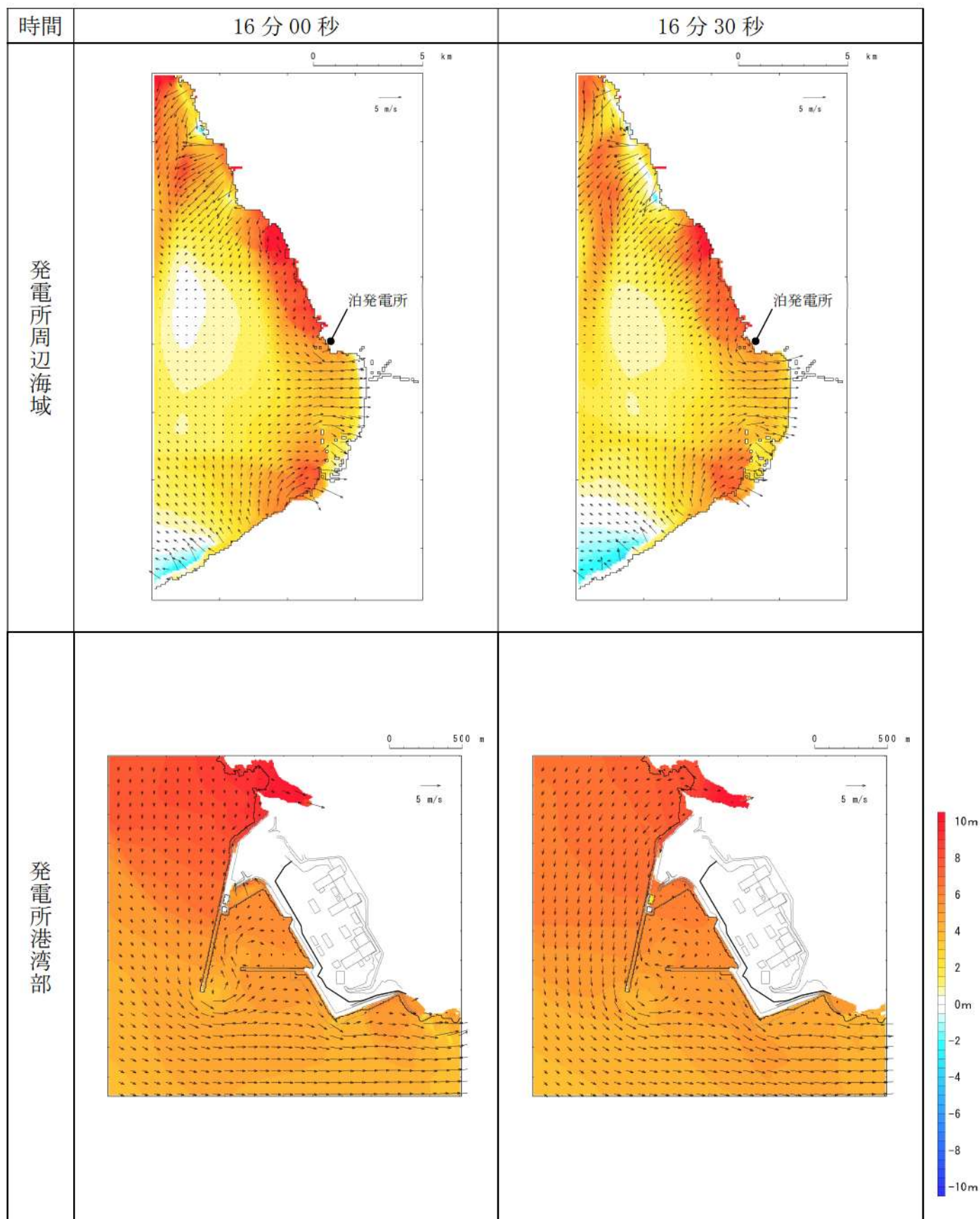
第5図-9 基準津波D（防波堤損傷なし）の水位変動・流向ベクトル(9/53)
