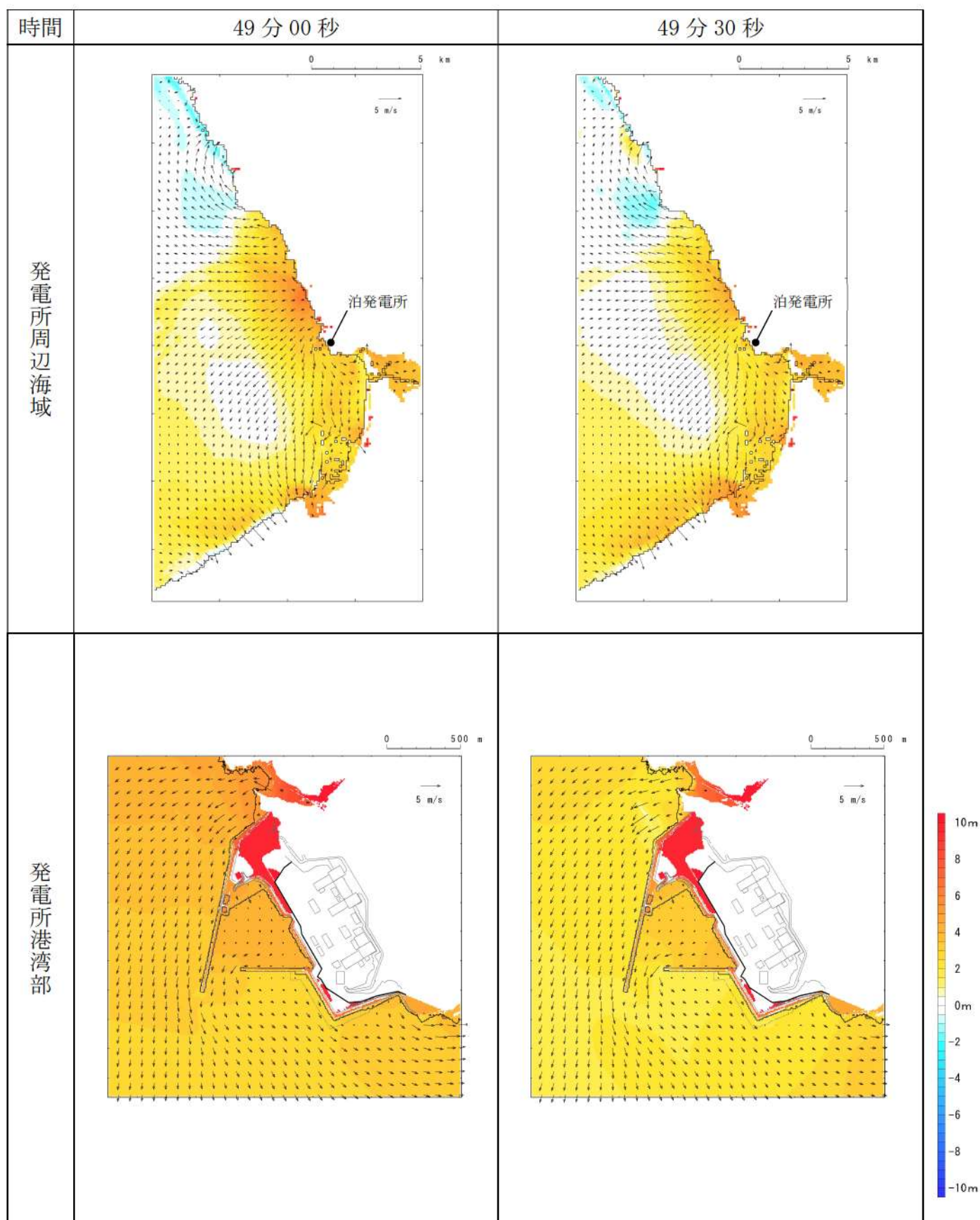
第4図-43 基準津波C（防波堤損傷なし）の水位変動・流向ベクトル(43/54)
