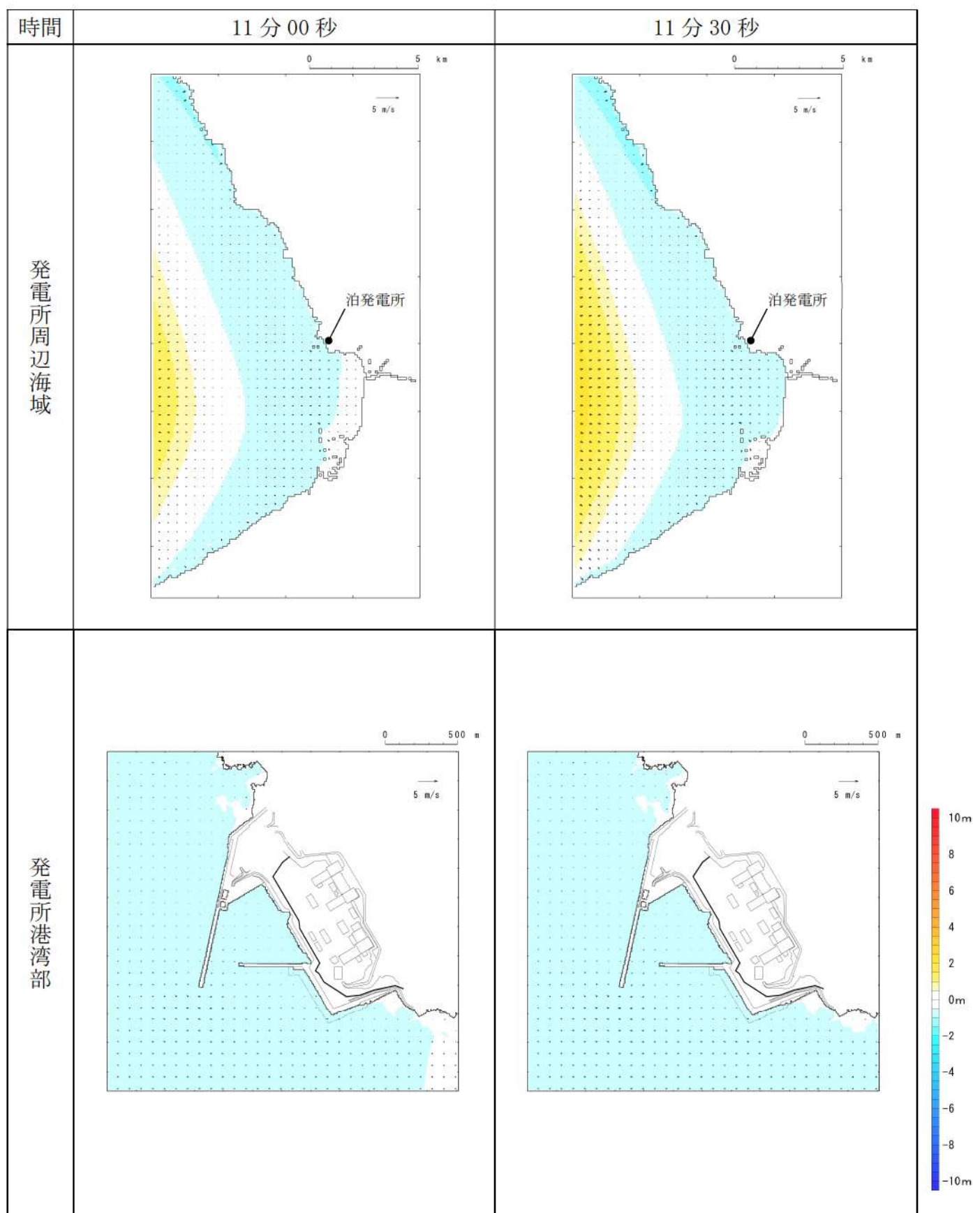
第4図-5 基準津波C（防波堤損傷なし）の水位変動・流向ベクトル(5/54)
