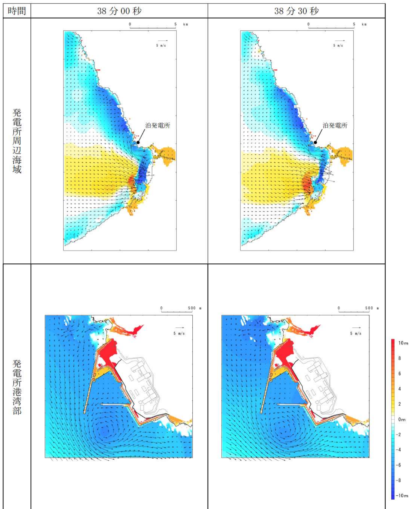
第 4 図-32 基準津波 C（防波堤損傷なし）の水位変動・流向ベクトル (32/54)
