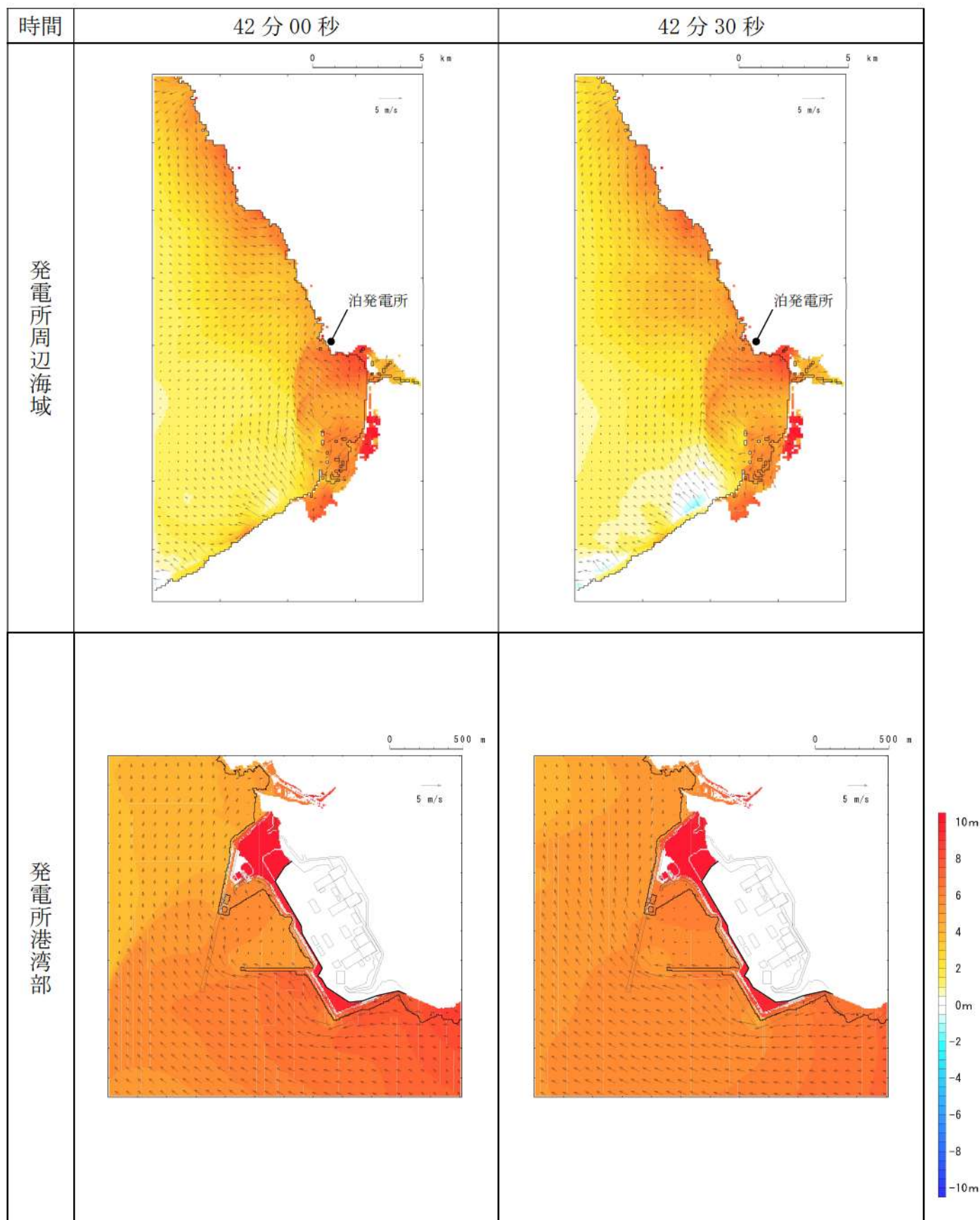
第 3 図-35 基準津波 B（北防波堤損傷）の水位変動・流向ベクトル(35/53)
