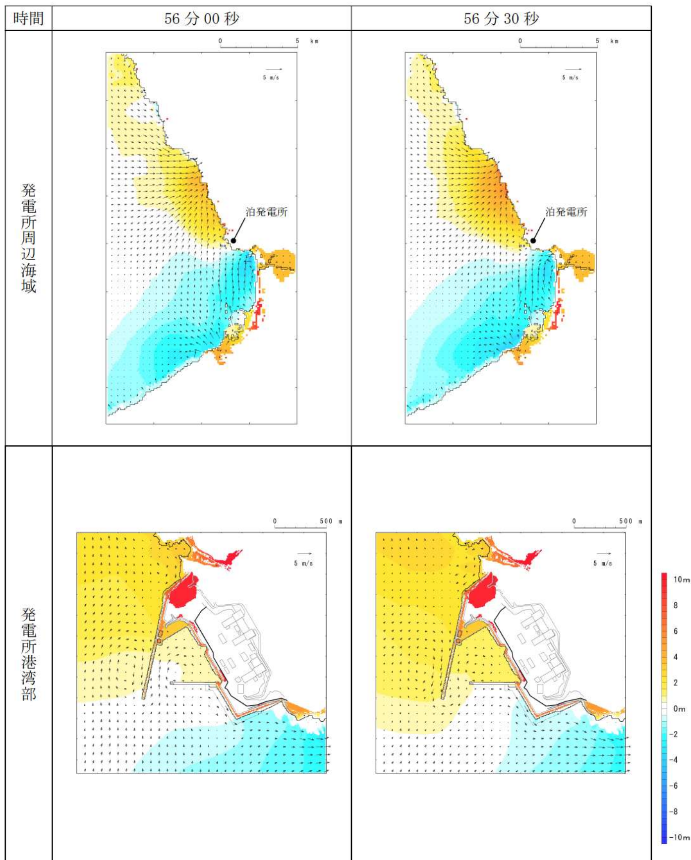
第 5 図-49 基準津波 D（防波堤損傷なし）の水位変動・流向ベクトル(49/53)
