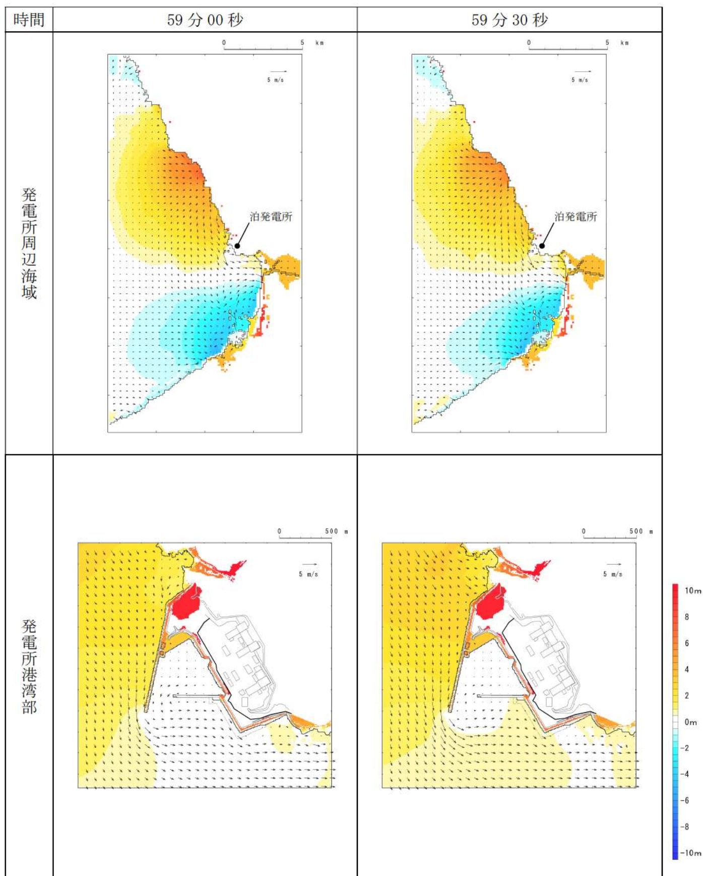
第 5 図-52 基準津波 D（防波堤損傷なし）の水位変動・流向ベクトル(52/53)
