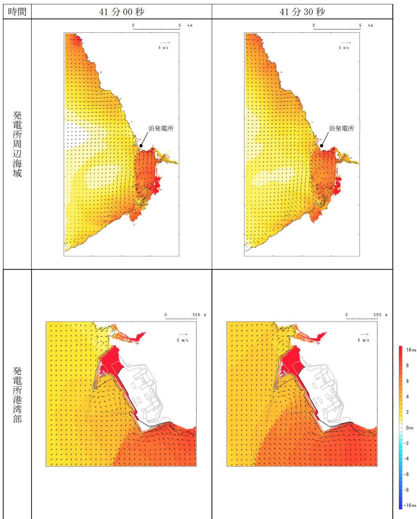
第 6 図-34 基準津波 D（北及び南防波堤損傷）の水位変動・流向ベクトル(34/53)
