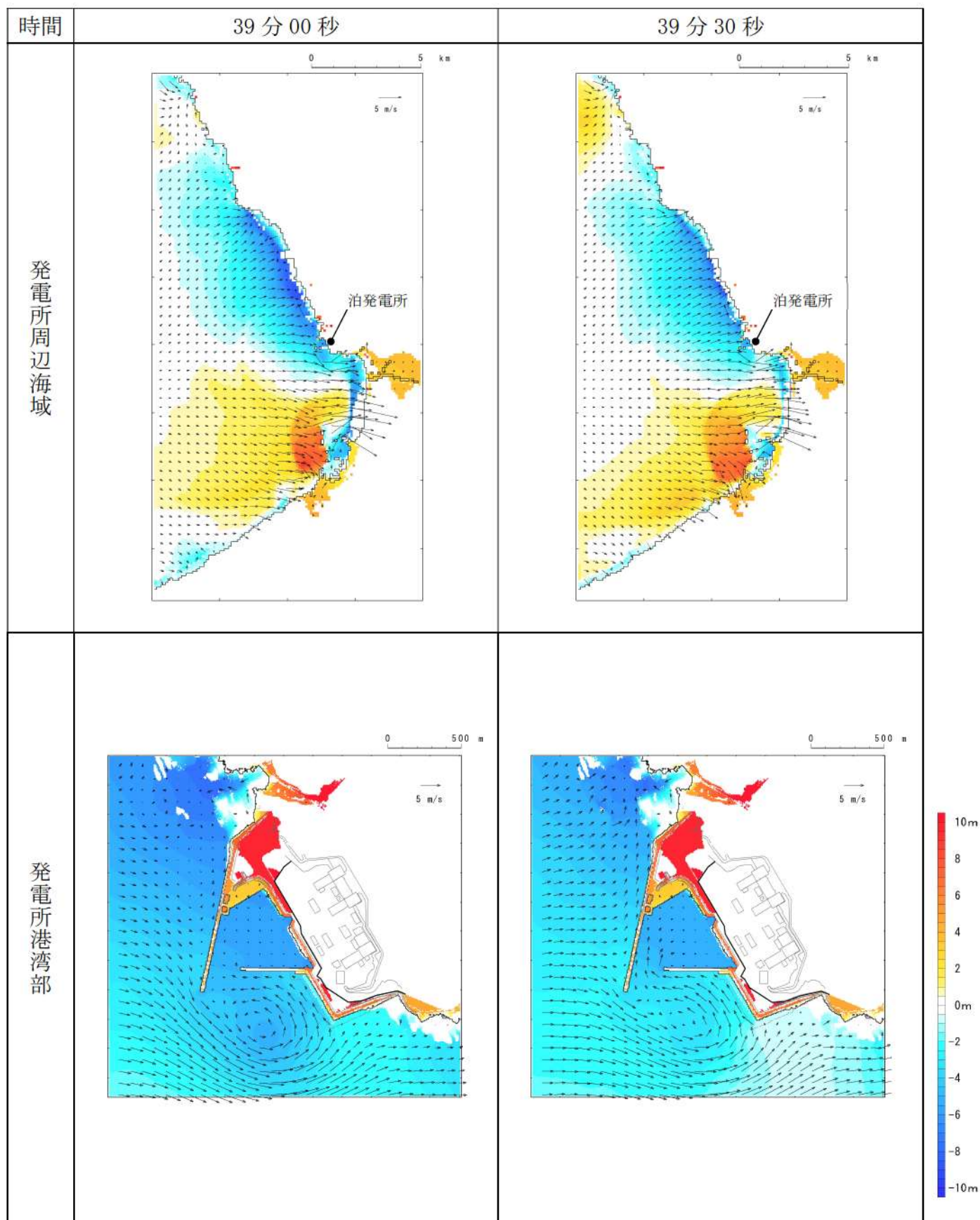
第4図-33 基準津波C（防波堤損傷なし）の水位変動・流向ベクトル(33/54)
