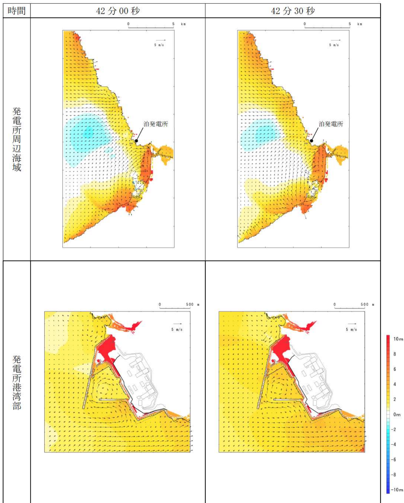
第4図-36 基準津波C（防波堤損傷なし）の水位変動・流向ベクトル(36/54)
