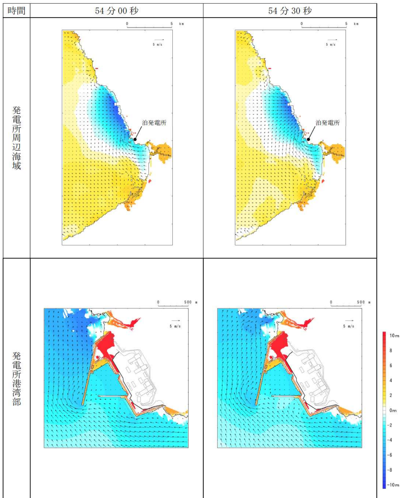
第4図-48 基準津波C（防波堤損傷なし）の水位変動・流向ベクトル(48/54)
