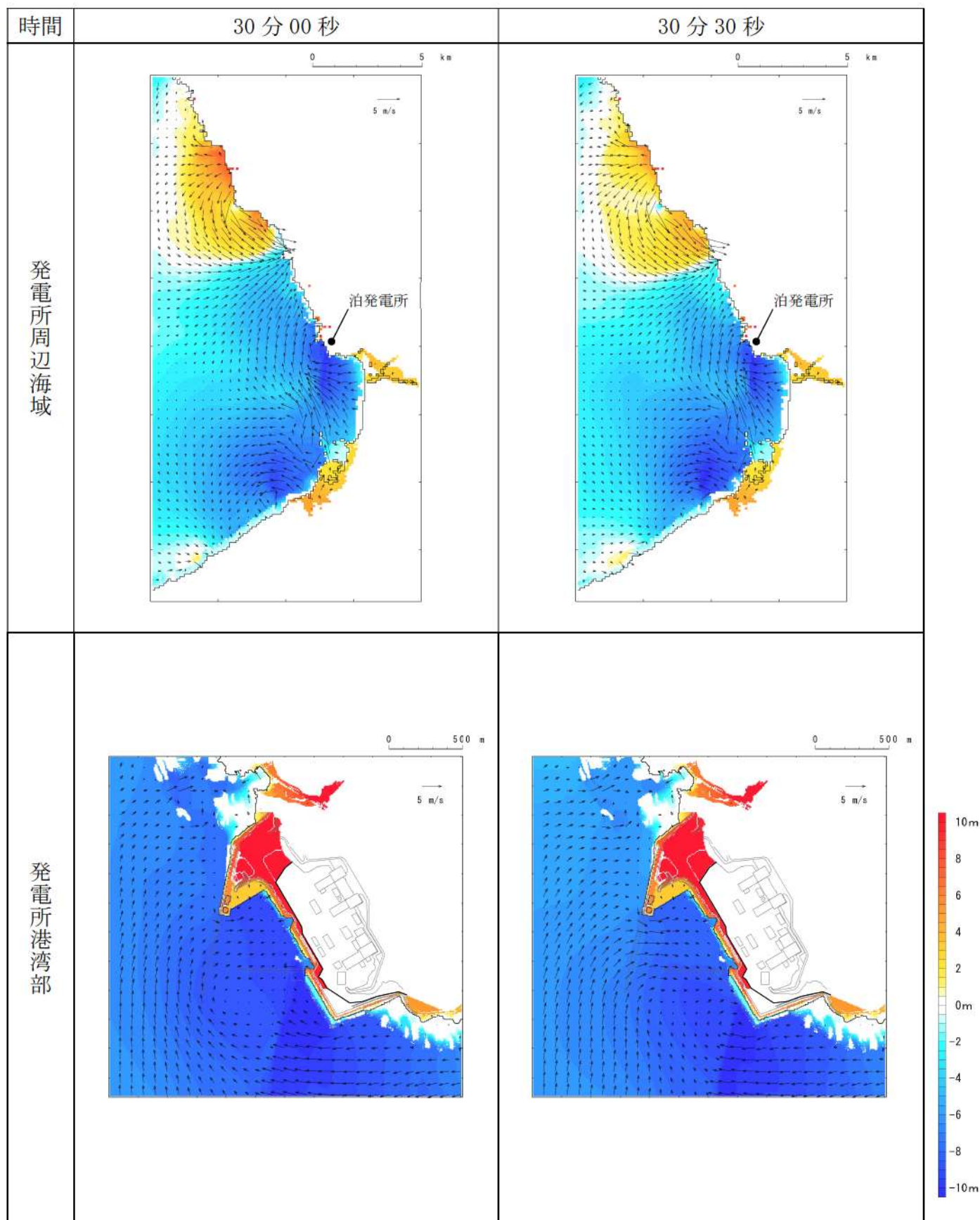
第 6 図-23 基準津波 D（北及び南防波堤損傷）の水位変動・流向ベクトル (23/53)
