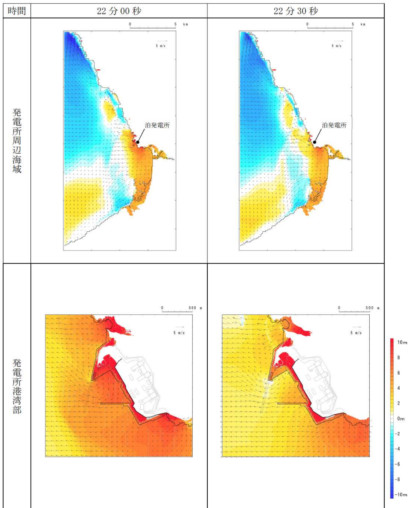
第3図-15 基準津波B（北防波堤損傷）の水位変動・流向ベクトル(15/53)
