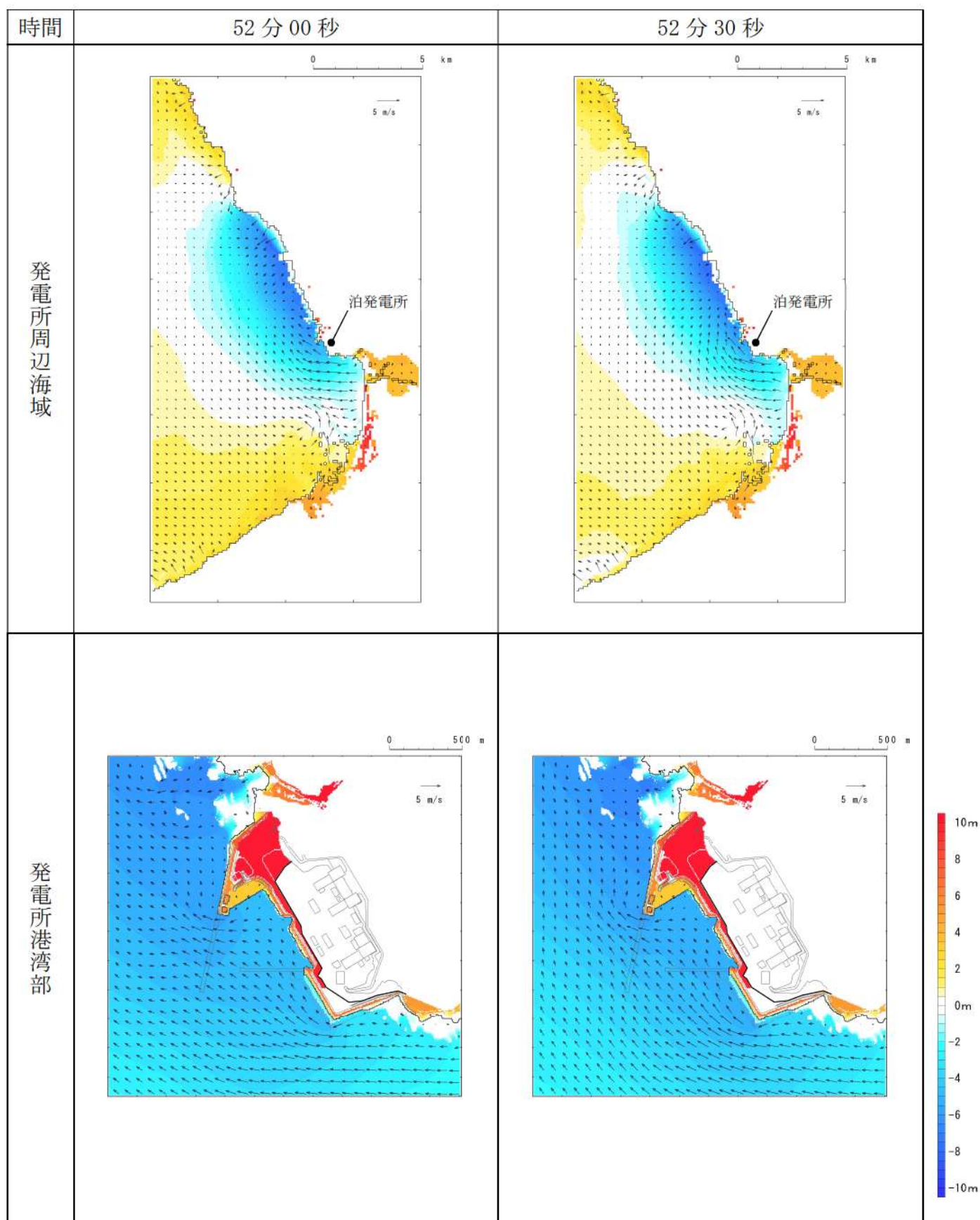
第 6 図-45 基準津波 D（北及び南防波堤損傷）の水位変動・流向ベクトル(45/53)
