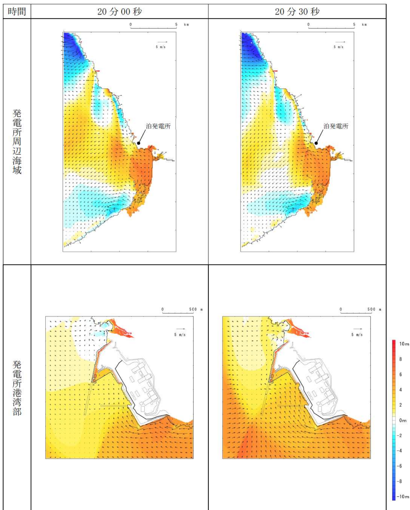
第 6 図-13 基準津波 D（北及び南防波堤損傷）の水位変動・流向ベクトル(13/53)
