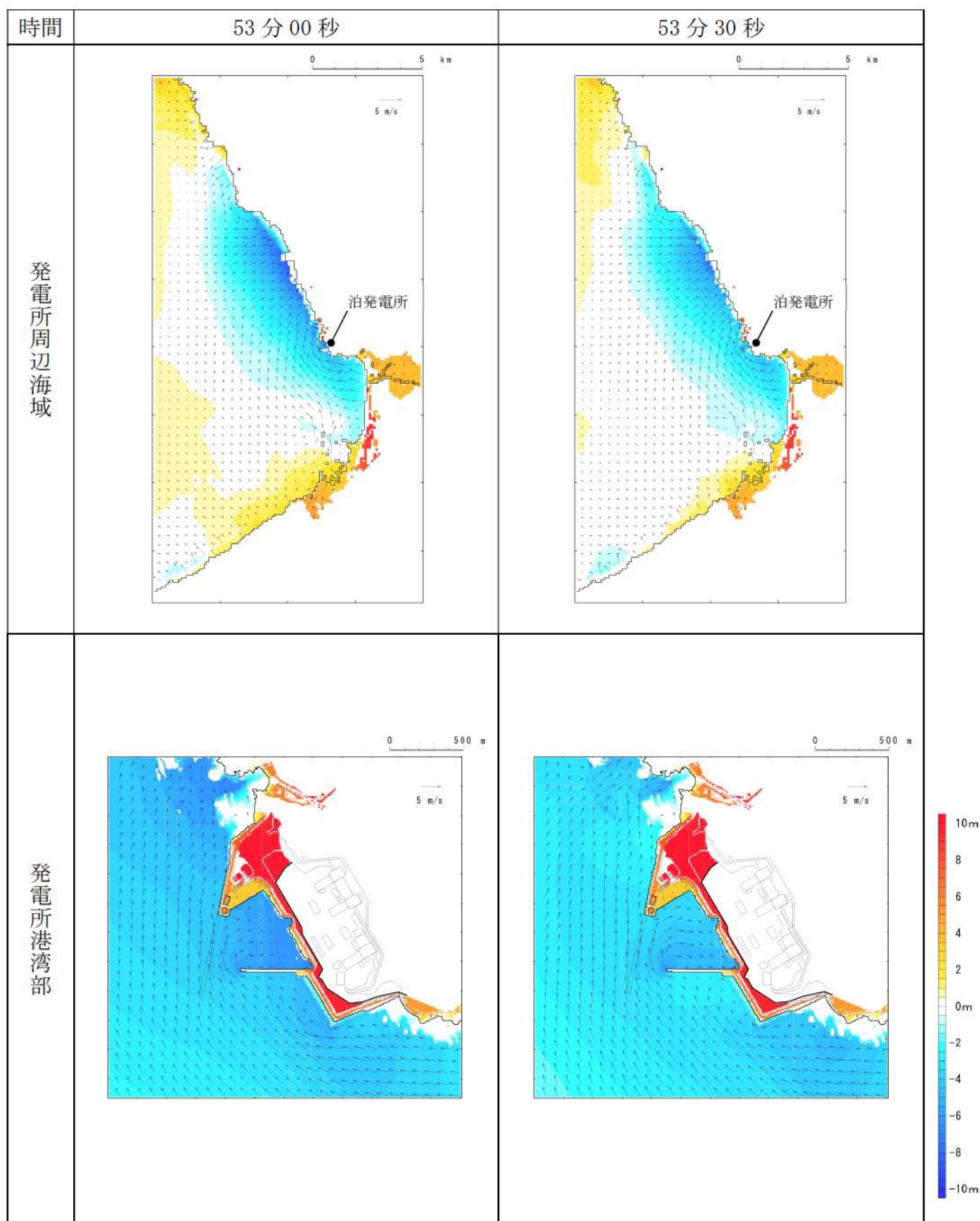
第3図-46 基準津波B（北防波堤損傷）の水位変動・流向ベクトル(46/53)
