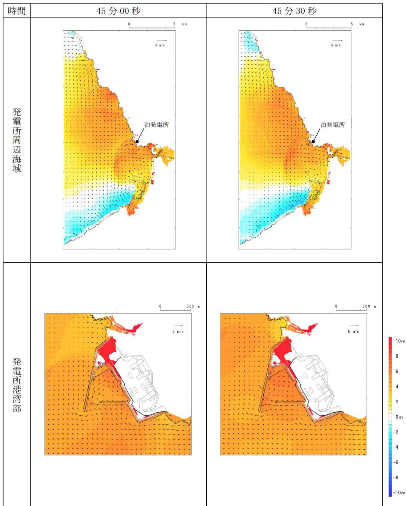
第4図-39 基準津波C（防波堤損傷なし）の水位変動・流向ベクトル(39/54)
