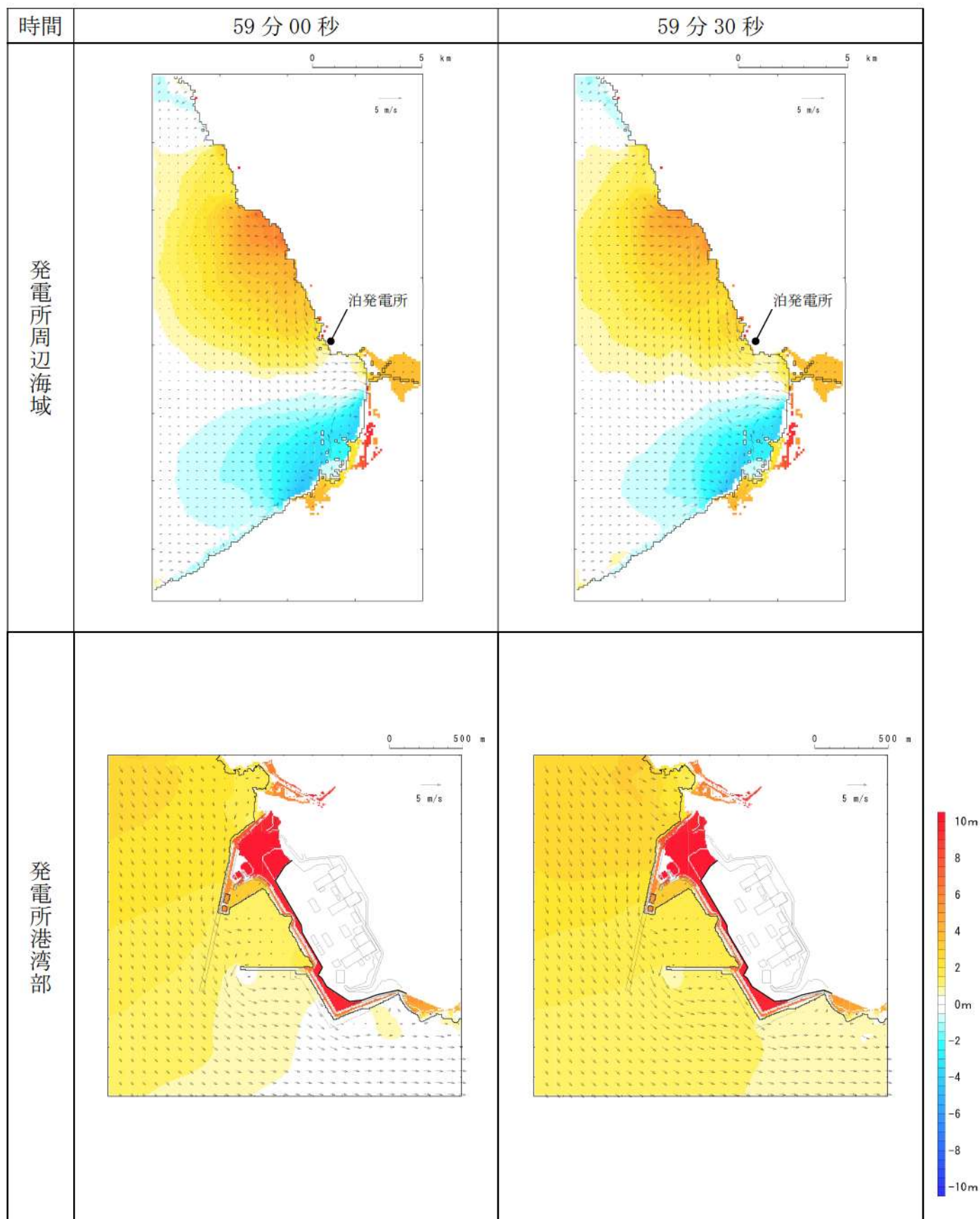
第3図-52 基準津波B（北防波堤損傷）の水位変動・流向ベクトル(52/53)
