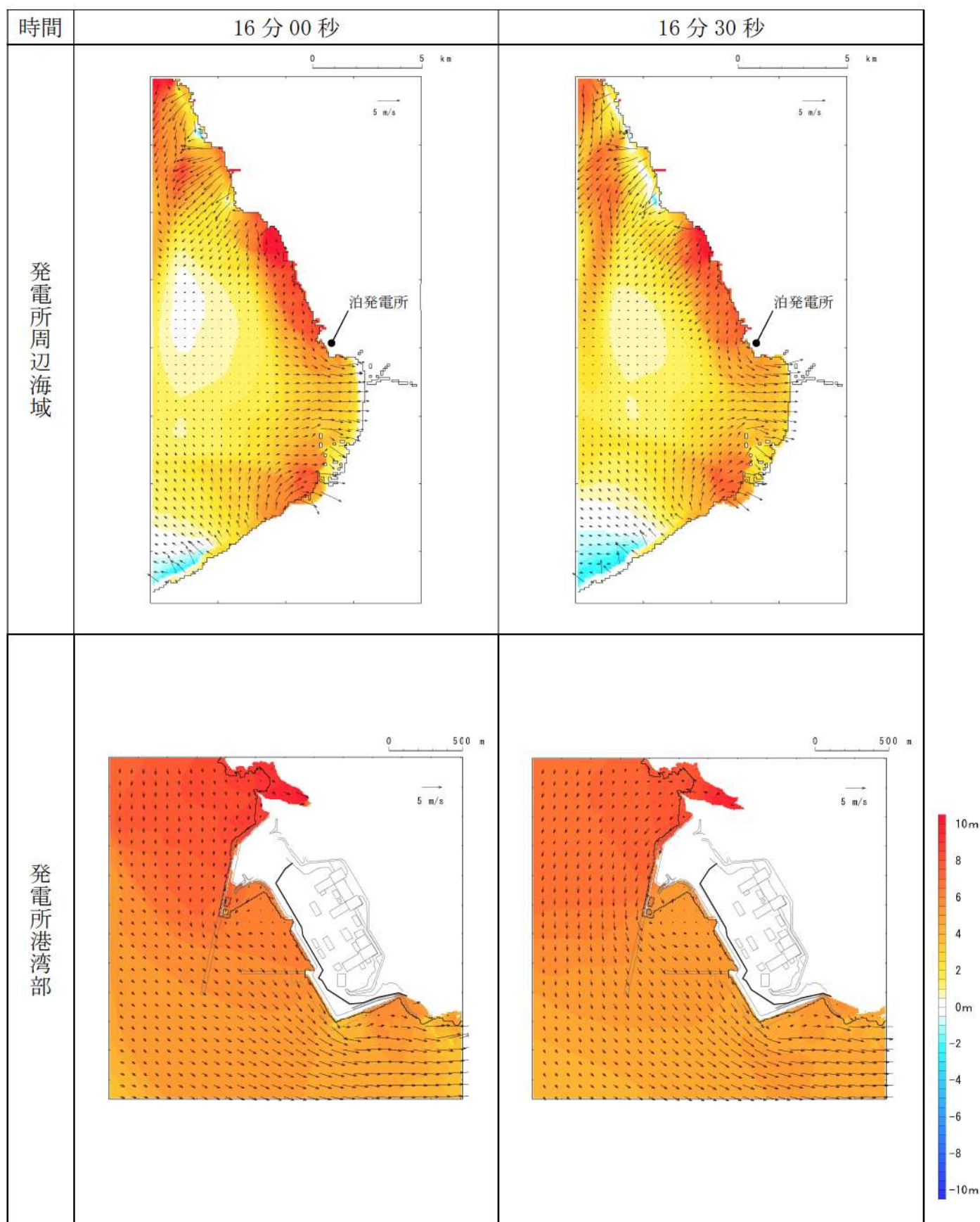
第 6 図- 9 基準津波 D（北及び南防波堤損傷）の水位変動・流向ベクトル (9/53)
