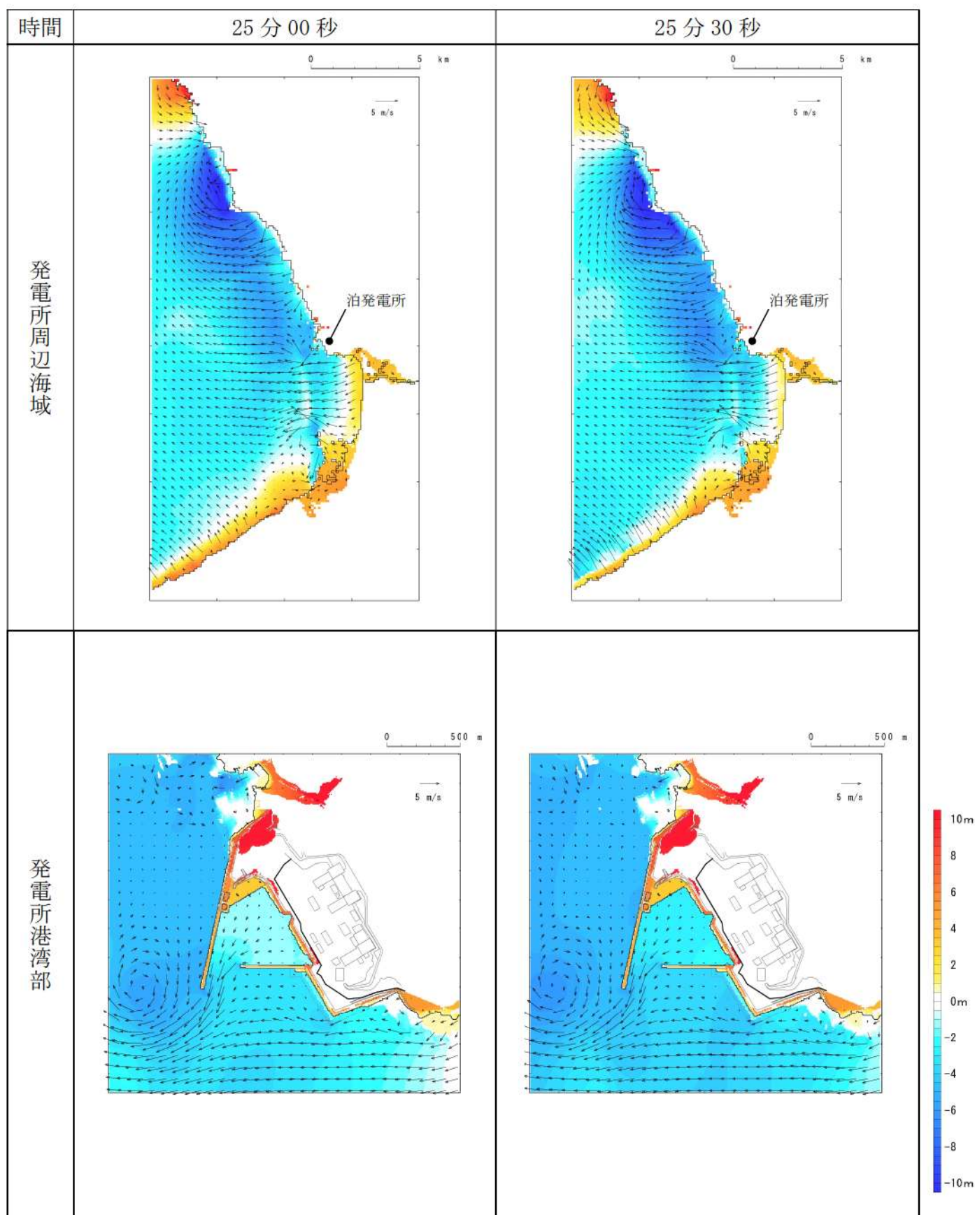
第 5 図-18 基準津波 D (防波堤損傷なし) の水位変動・流向ベクトル(18/53)
