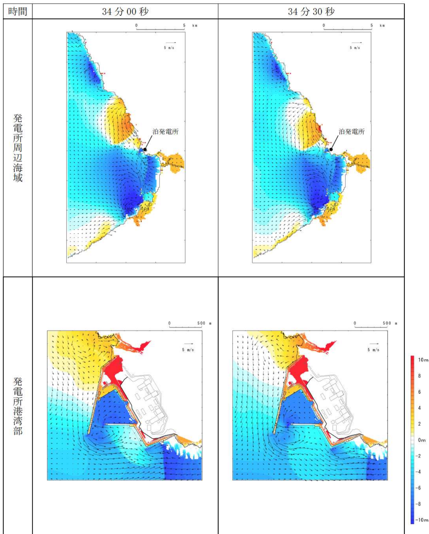
第4図-28 基準津波C（防波堤損傷なし）の水位変動・流向ベクトル(28/54)
