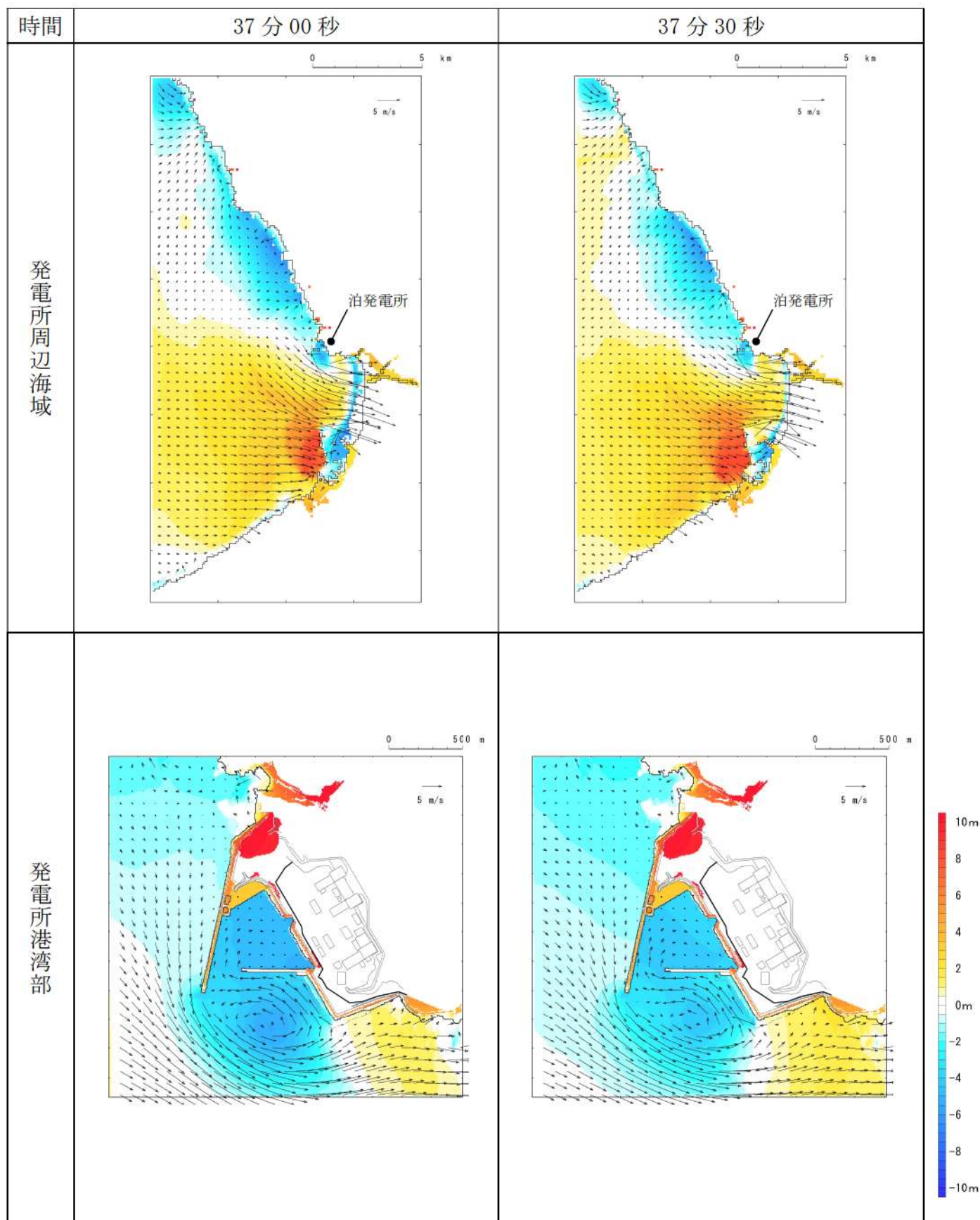
第 5 図-30 基準津波 D（防波堤損傷なし）の水位変動・流向ベクトル (30/53)
