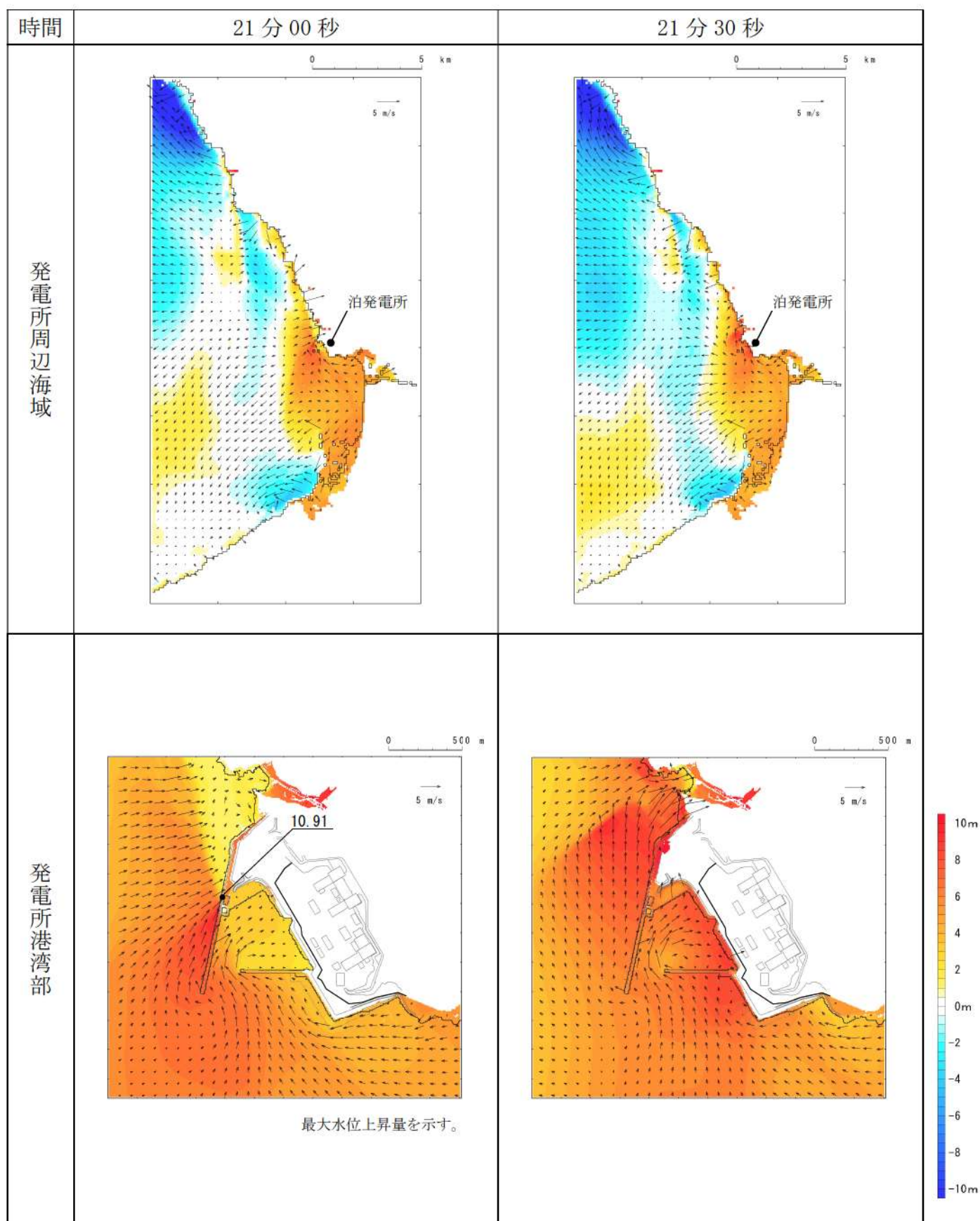
第5図-14 基準津波D（防波堤損傷なし）の水位変動・流向ベクトル(14/53)
