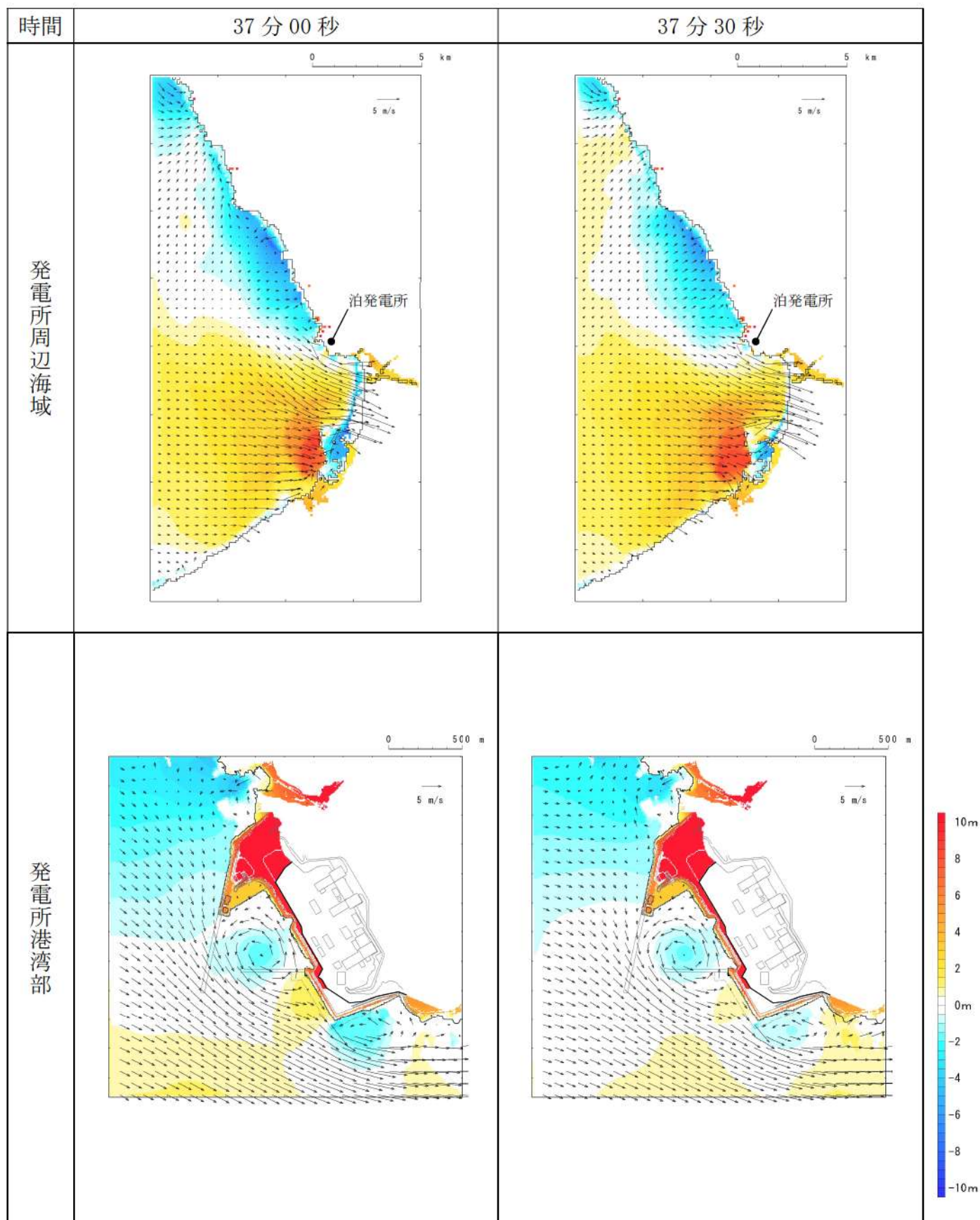
第 6 図-30 基準津波 D（北及び南防波堤損傷）の水位変動・流向ベクトル(30/53)
