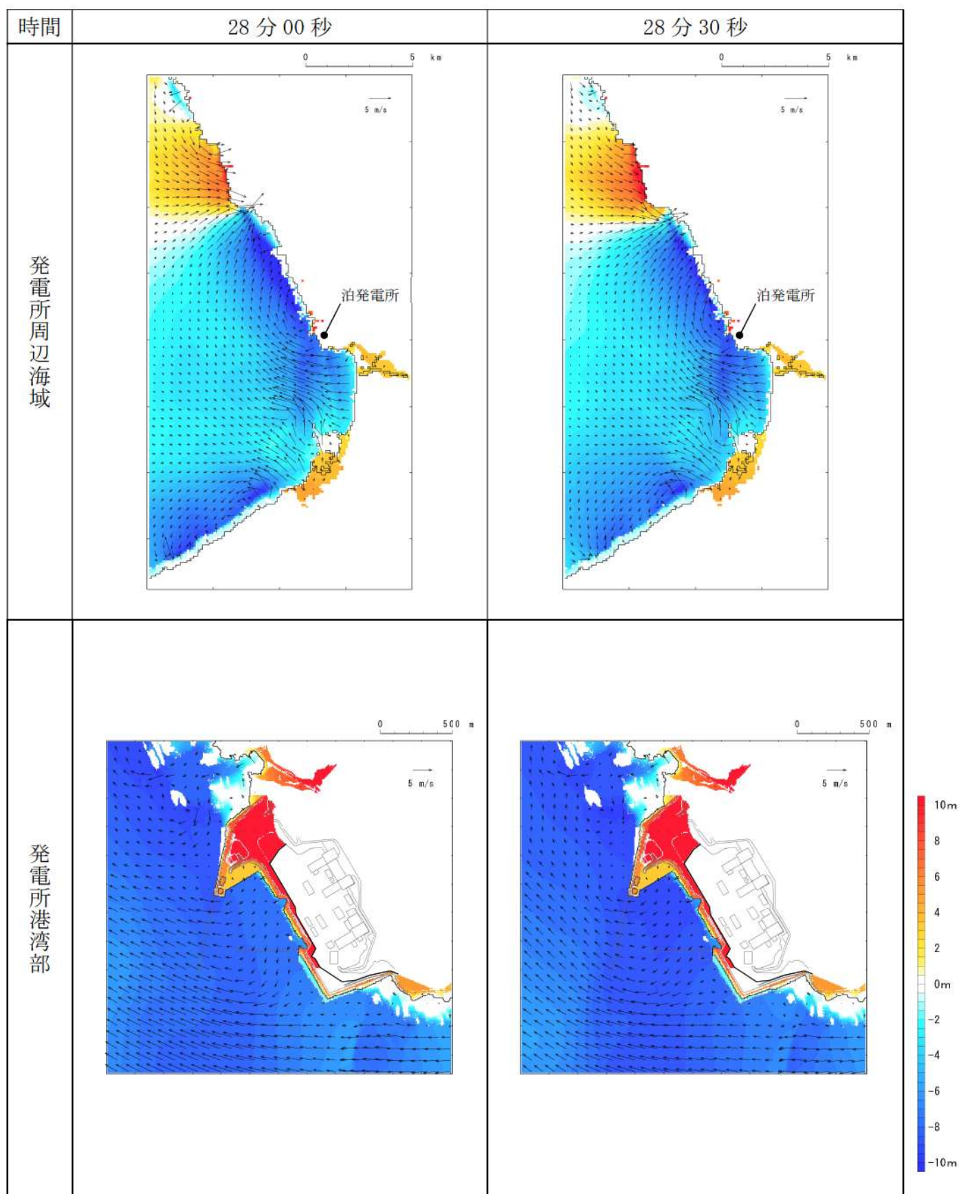
第 6 図-21 基準津波 D（北及び南防波堤損傷）の水位変動・流向ベクトル(21/53)
