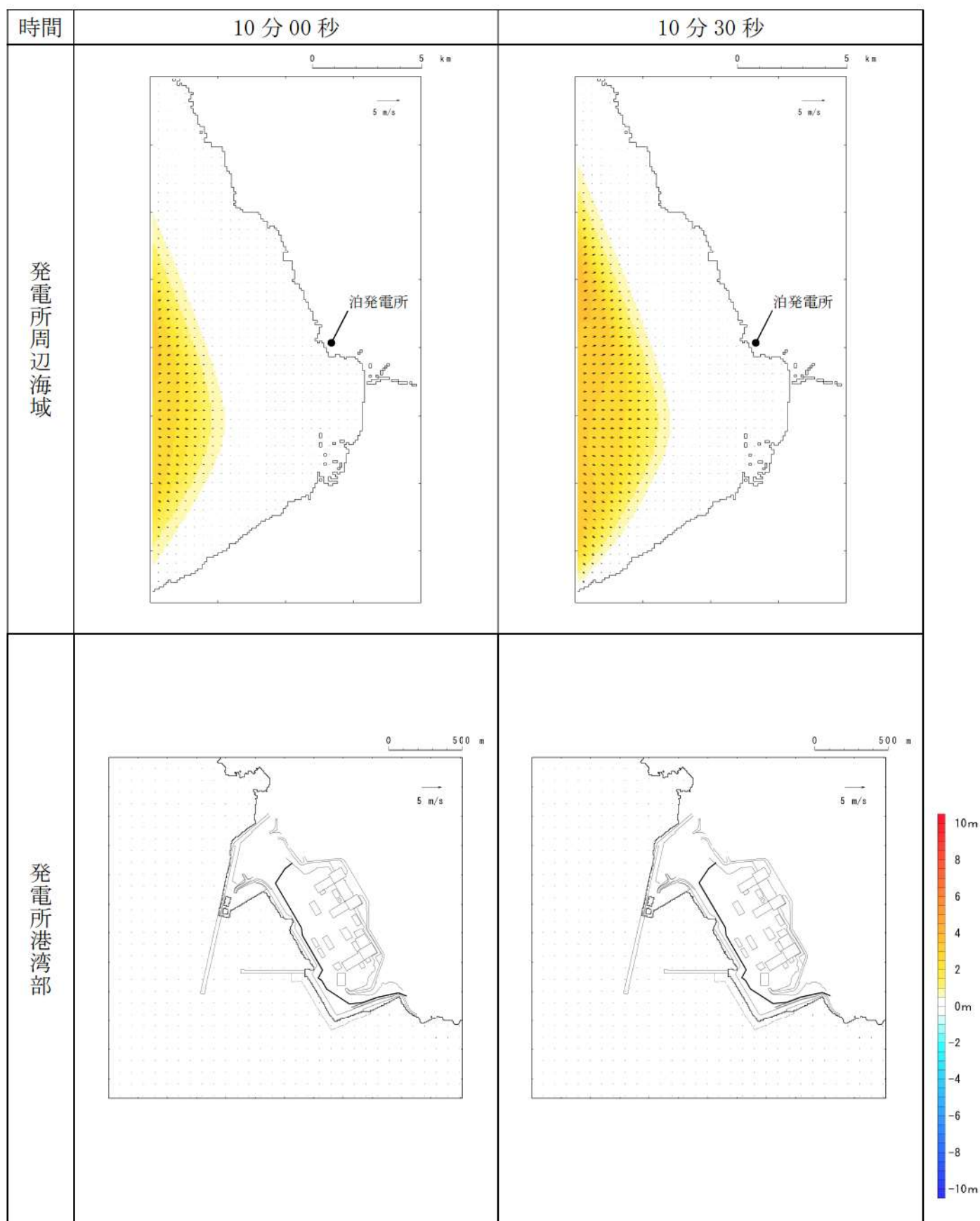
第 6 図- 3 基準津波 D（北及び南防波堤損傷）の水位変動・流向ベクトル (3/53)
