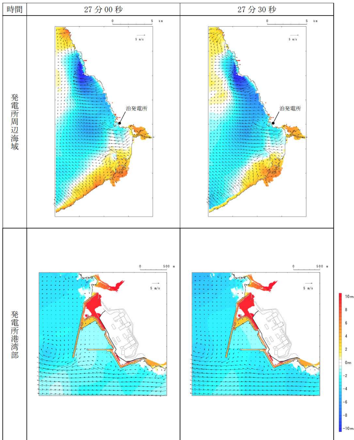
第4図-21 基準津波C（防波堤損傷なし）の水位変動・流向ベクトル(21/54)
