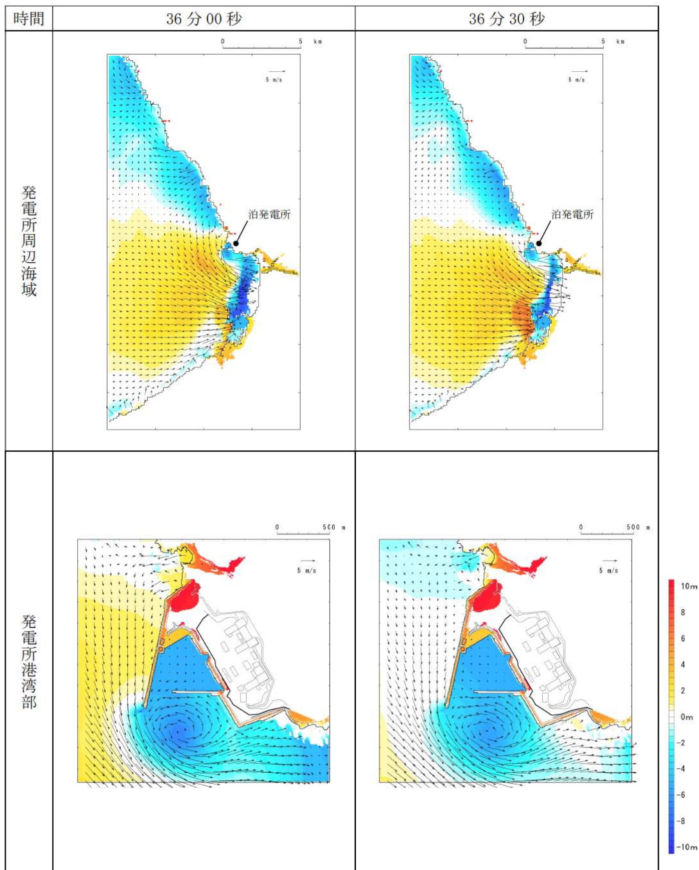
第 5 図-29 基準津波 D (防波堤損傷なし) の水位変動・流向ベクトル (29/53)
