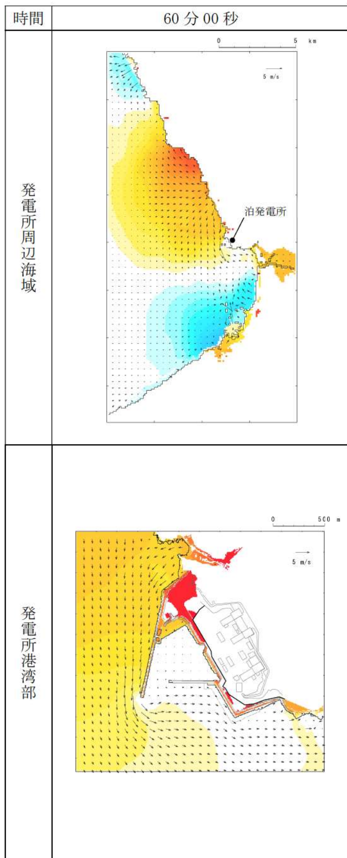
第4図-54 基準津波C（防波堤損傷なし）の水位変動・流向ベクトル(54/54)
