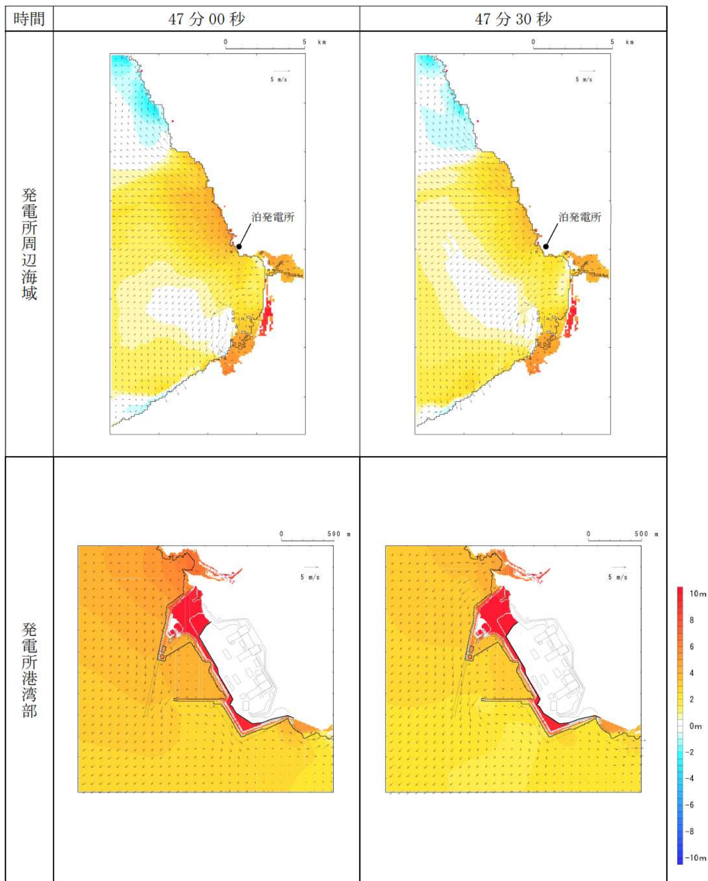
第3図-40 基準津波B（北防波堤損傷）の水位変動・流向ベクトル(40/53)
