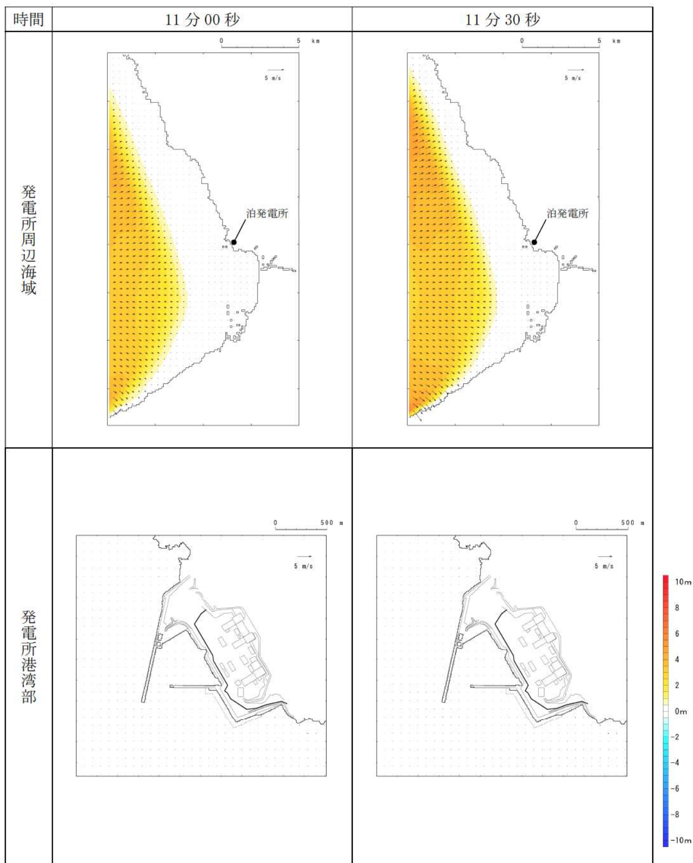
第5図-4 基準津波D（防波堤損傷なし）の水位変動・流向ベクトル(4/53)
