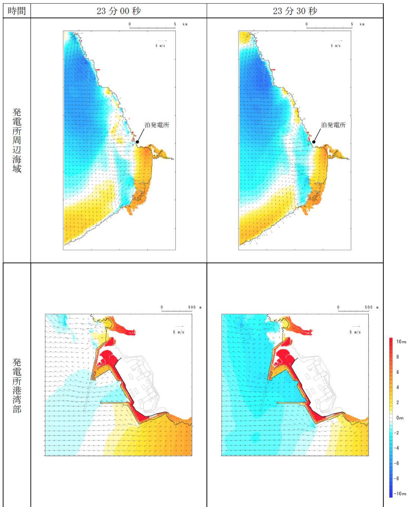
第3図-16 基準津波B（北防波堤損傷）の水位変動・流向ベクトル(16/53)
