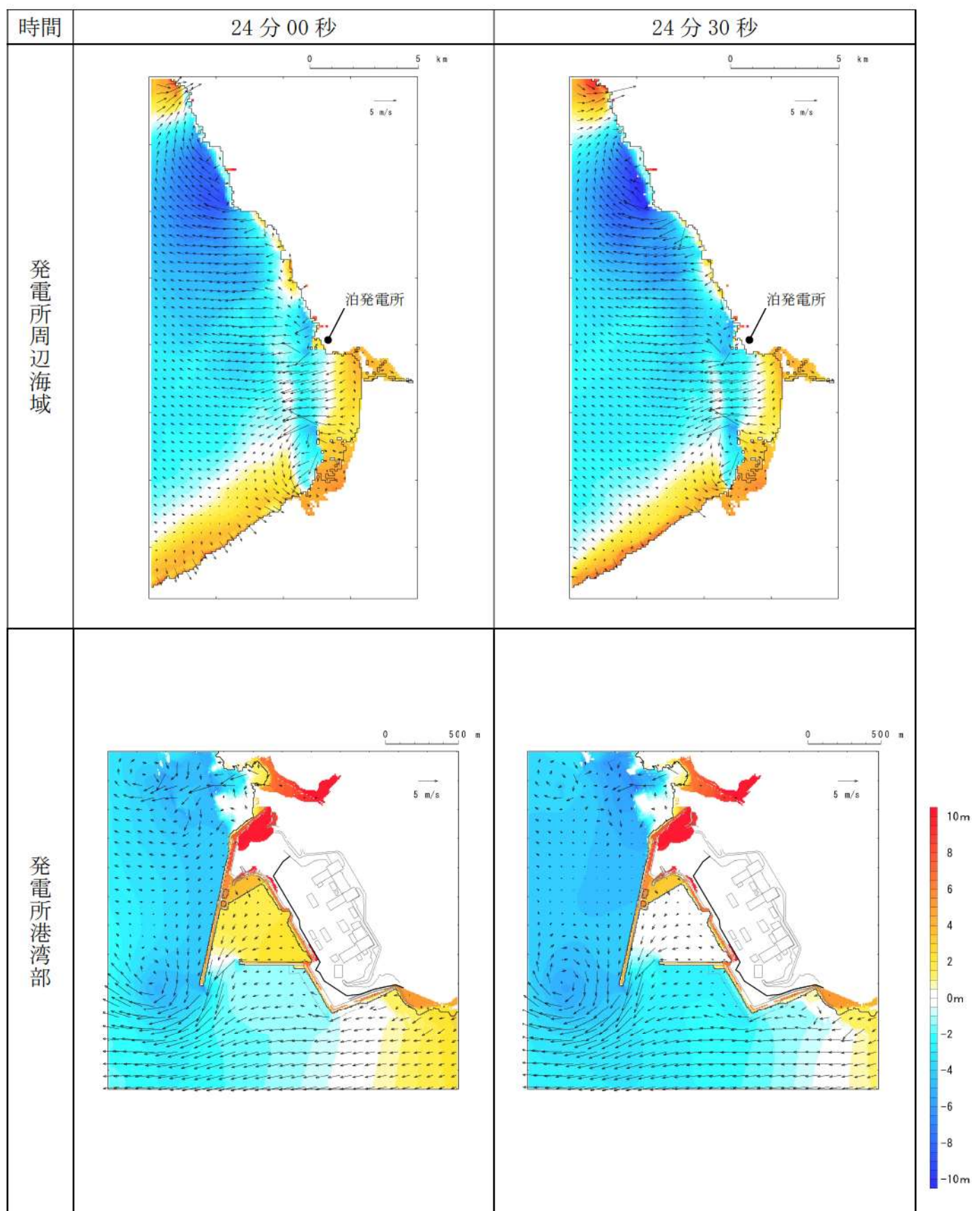
第 5 図-17 基準津波 D（防波堤損傷なし）の水位変動・流向ベクトル(17/53)
