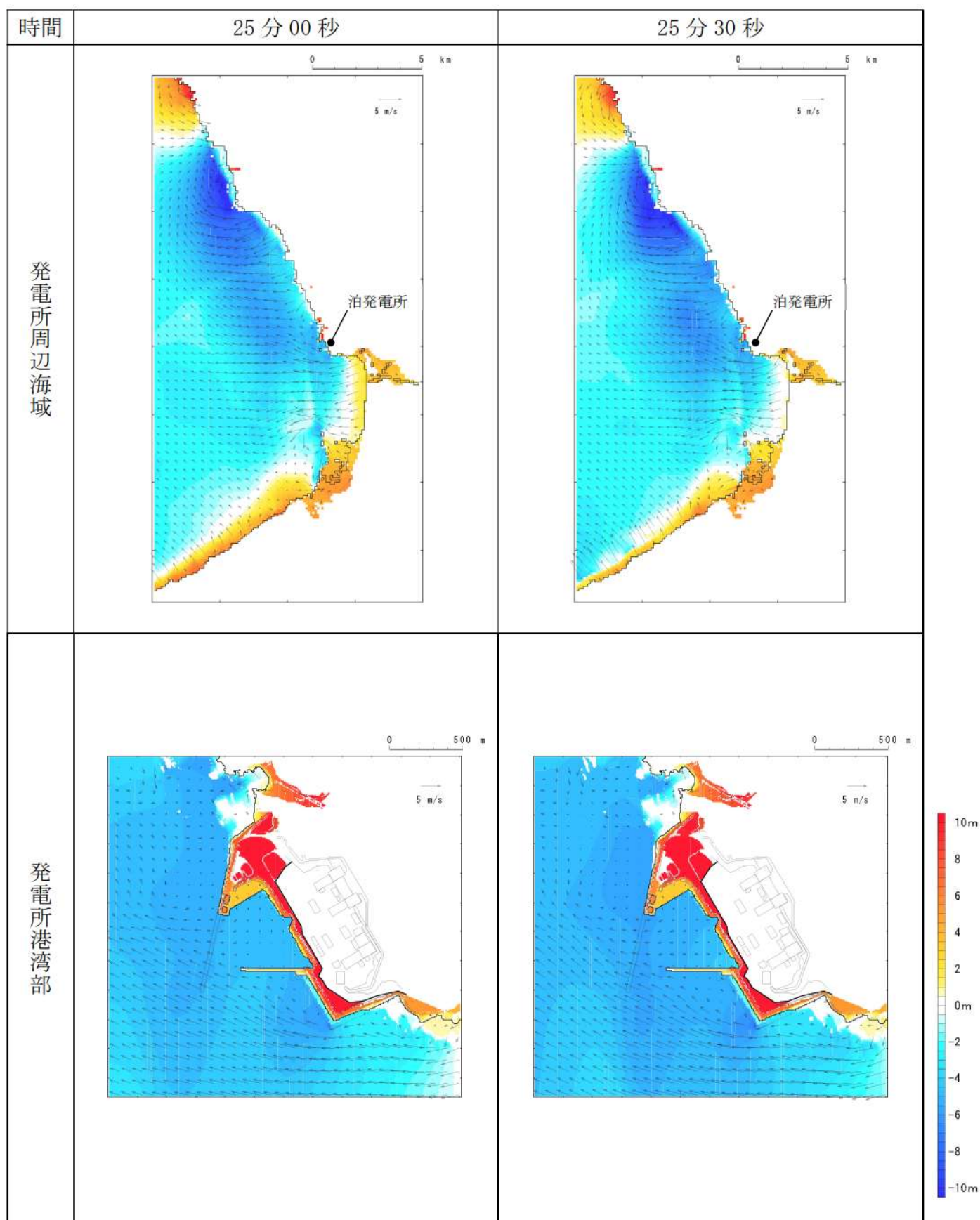
第3図-18 基準津波B（北防波堤損傷）の水位変動・流向ベクトル(18/53)
