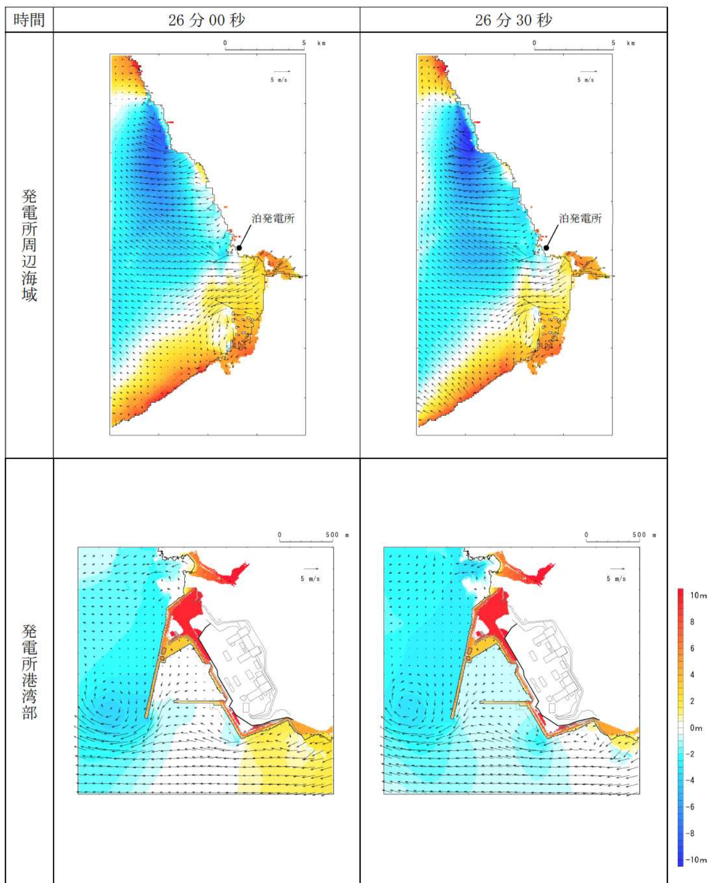
第 4 図-20 基準津波 C（防波堤損傷なし）の水位変動・流向ベクトル (20/54)
