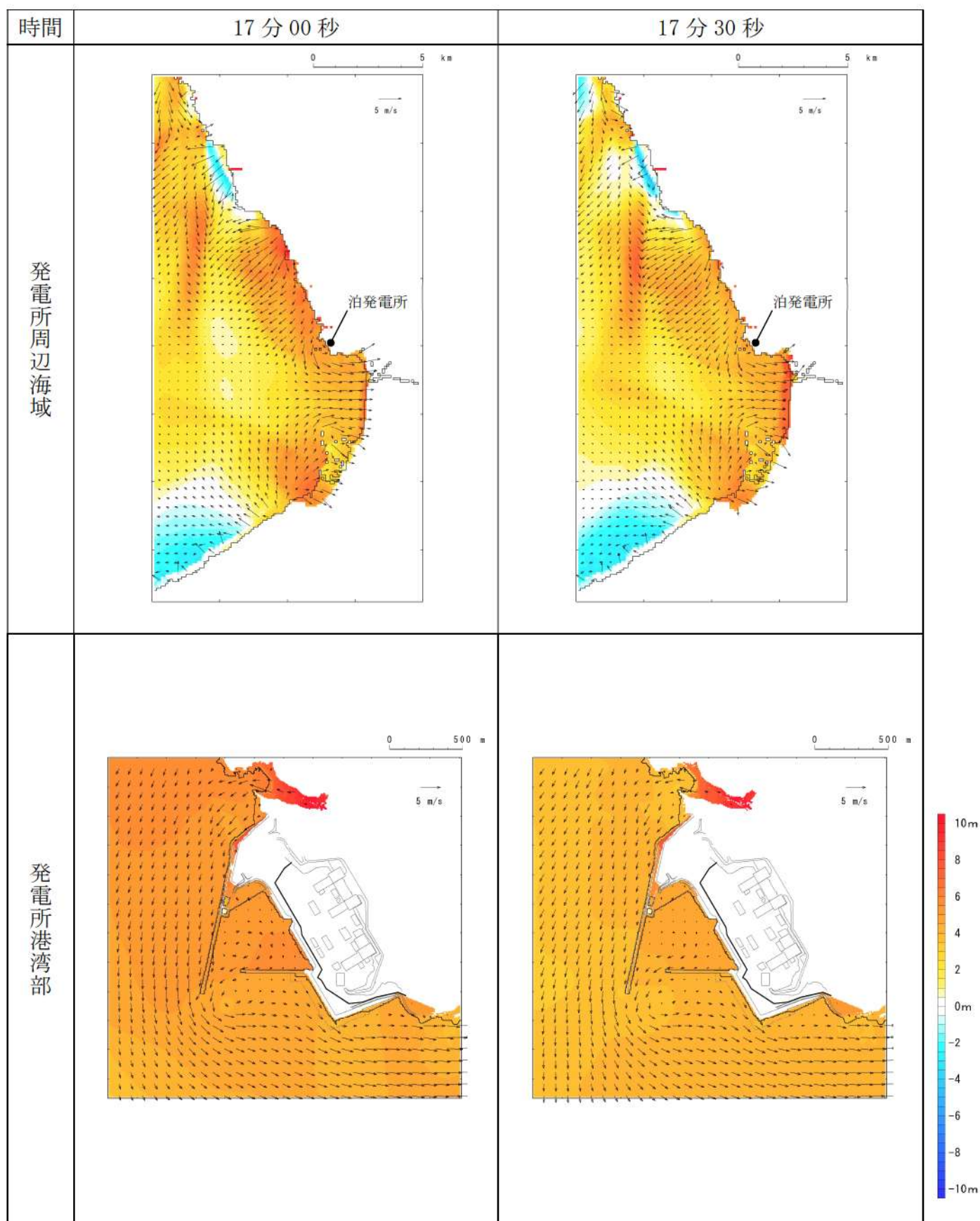
第 5 図-10 基準津波 D (防波堤損傷なし) の水位変動・流向ベクトル(10/53)
