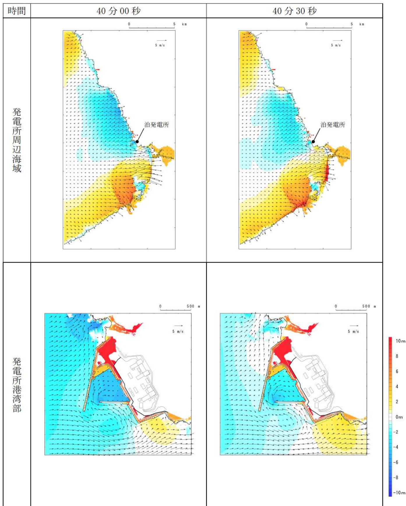
第4図-34 基準津波C（防波堤損傷なし）の水位変動・流向ベクトル(34/54)
