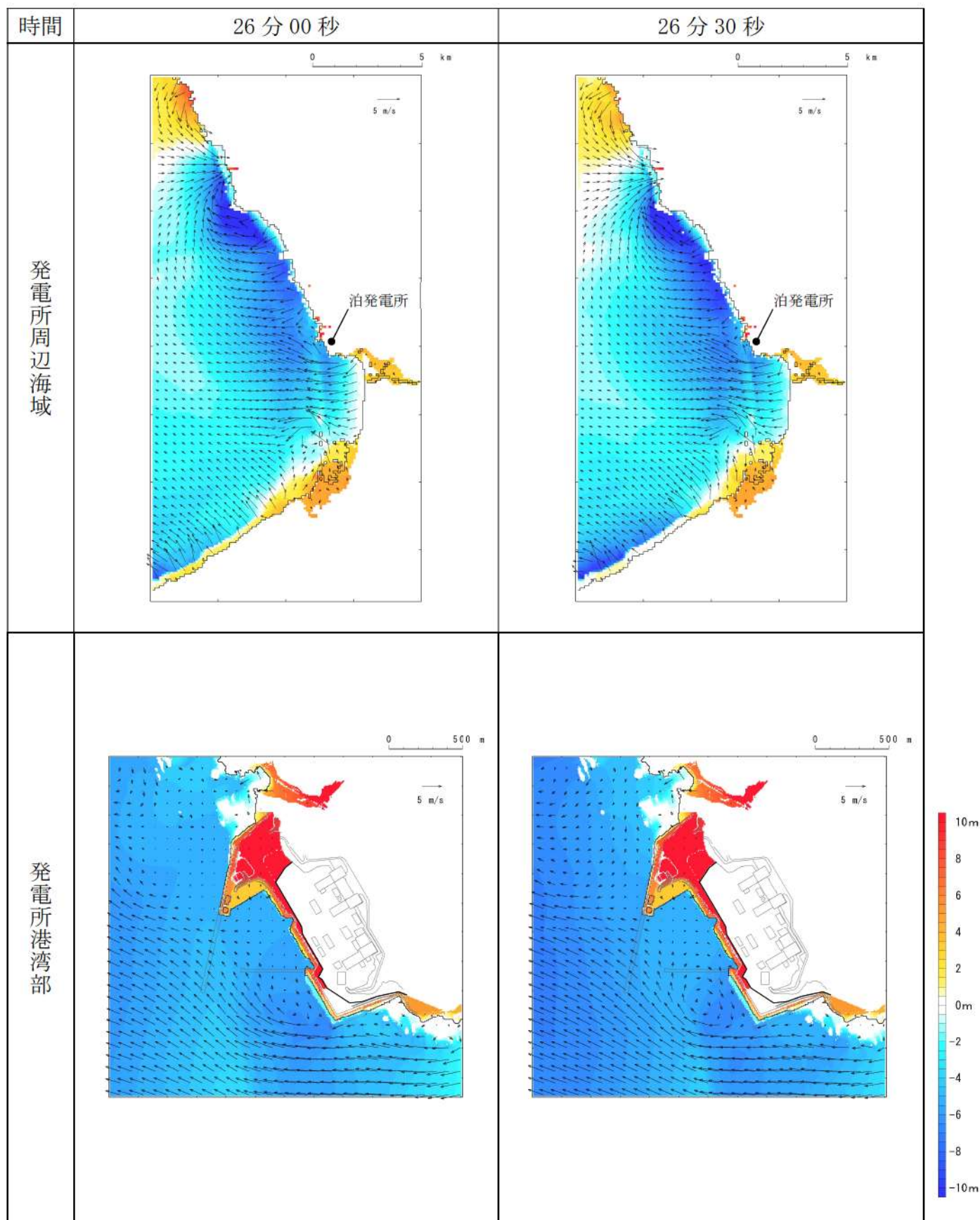
第 6 図-19 基準津波 D（北及び南防波堤損傷）の水位変動・流向ベクトル(19/53)
