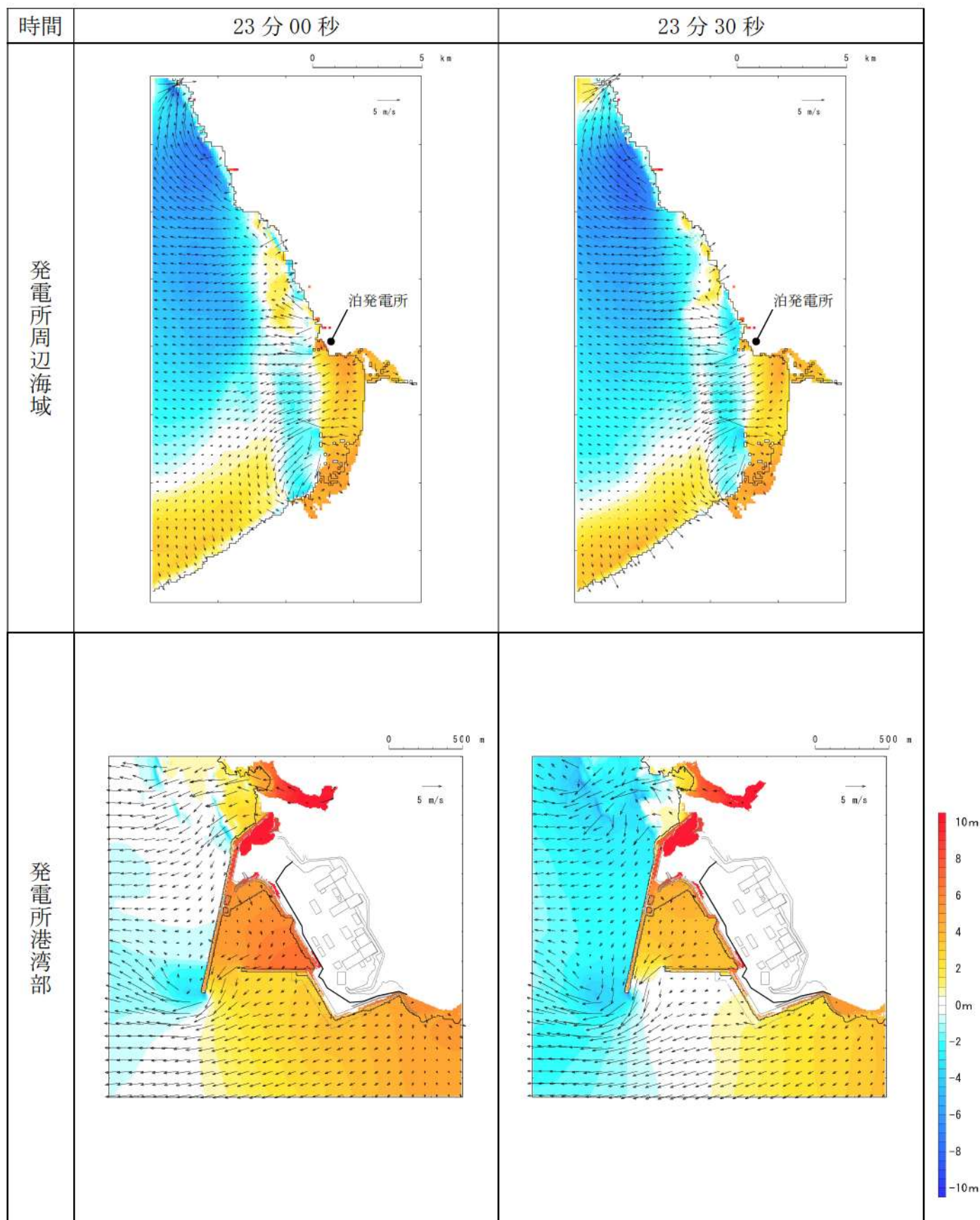
第 5 図-16 基準津波 D（防波堤損傷なし）の水位変動・流向ベクトル(16/53)
