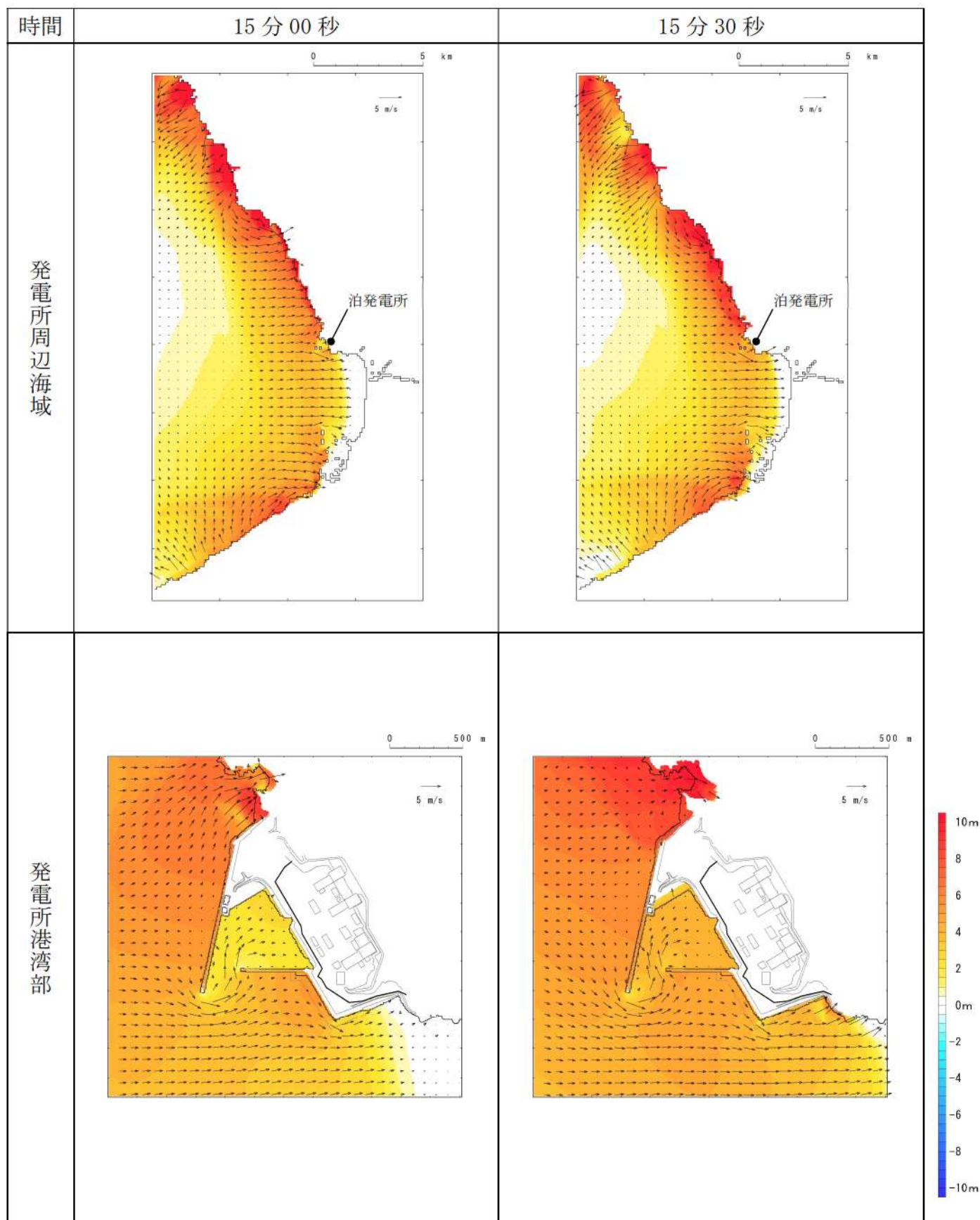
第5図-8 基準津波D（防波堤損傷なし）の水位変動・流向ベクトル(8/53)
