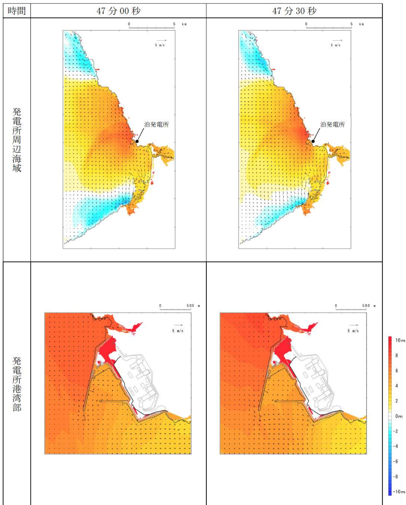
第4図-41 基準津波C（防波堤損傷なし）の水位変動・流向ベクトル(41/54)
