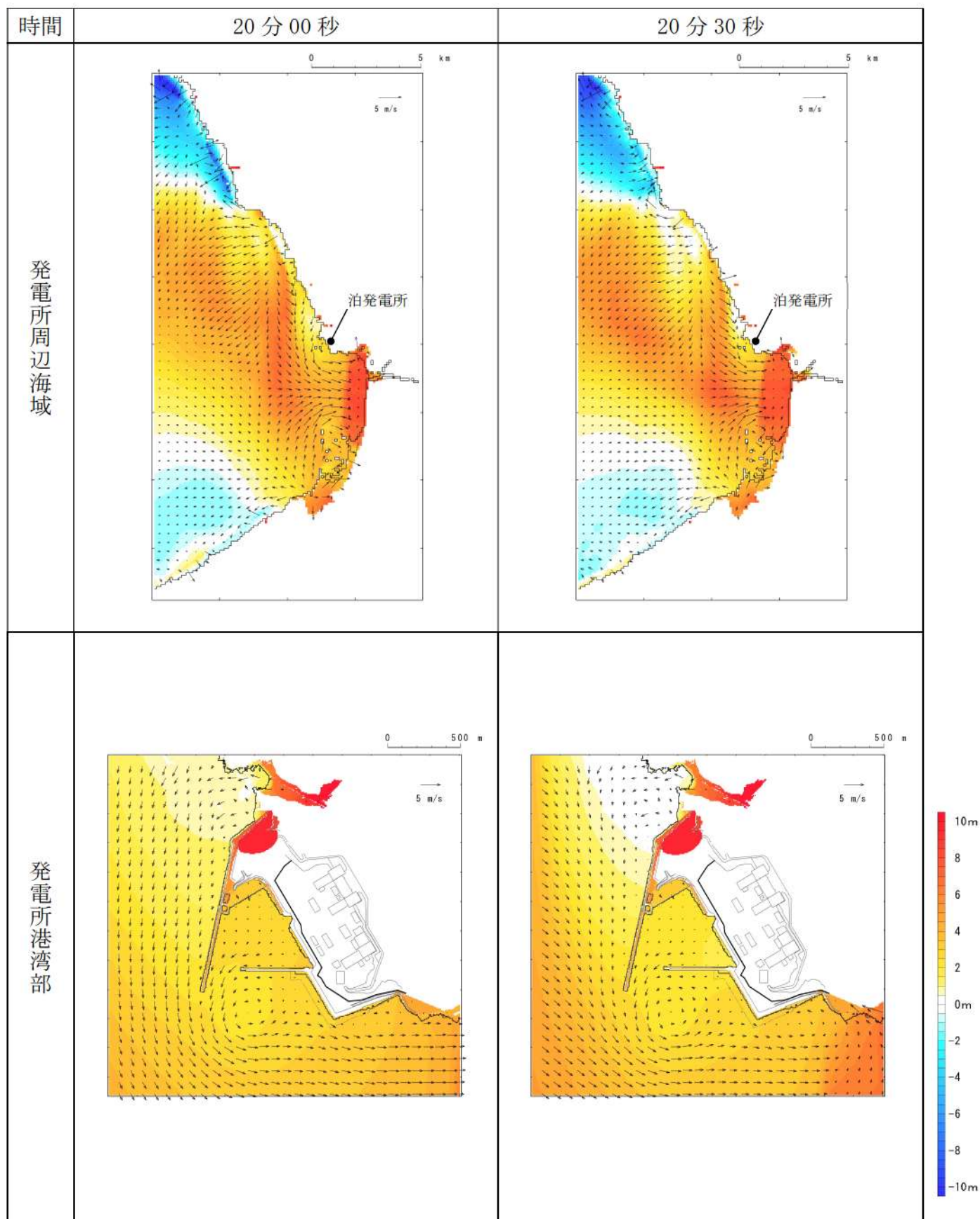
第4図-14 基準津波C（防波堤損傷なし）の水位変動・流向ベクトル(14/54)
