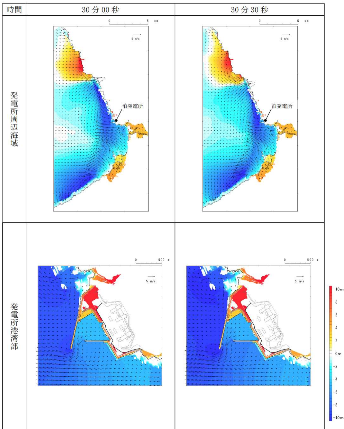
第4図-24 基準津波C（防波堤損傷なし）の水位変動・流向ベクトル(24/54)
