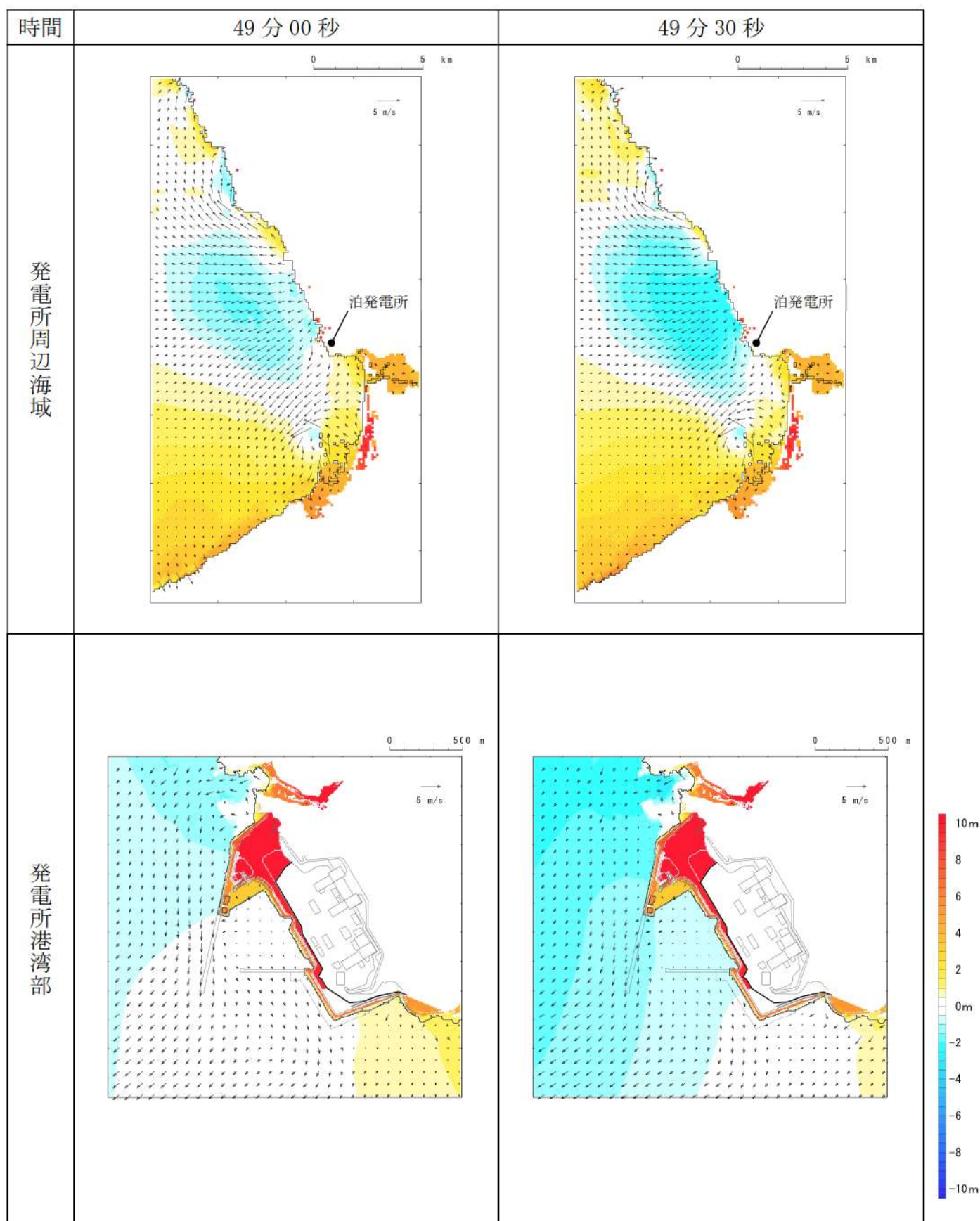
第 6 図-42 基準津波 D（北及び南防波堤損傷）の水位変動・流向ベクトル(42/53)
