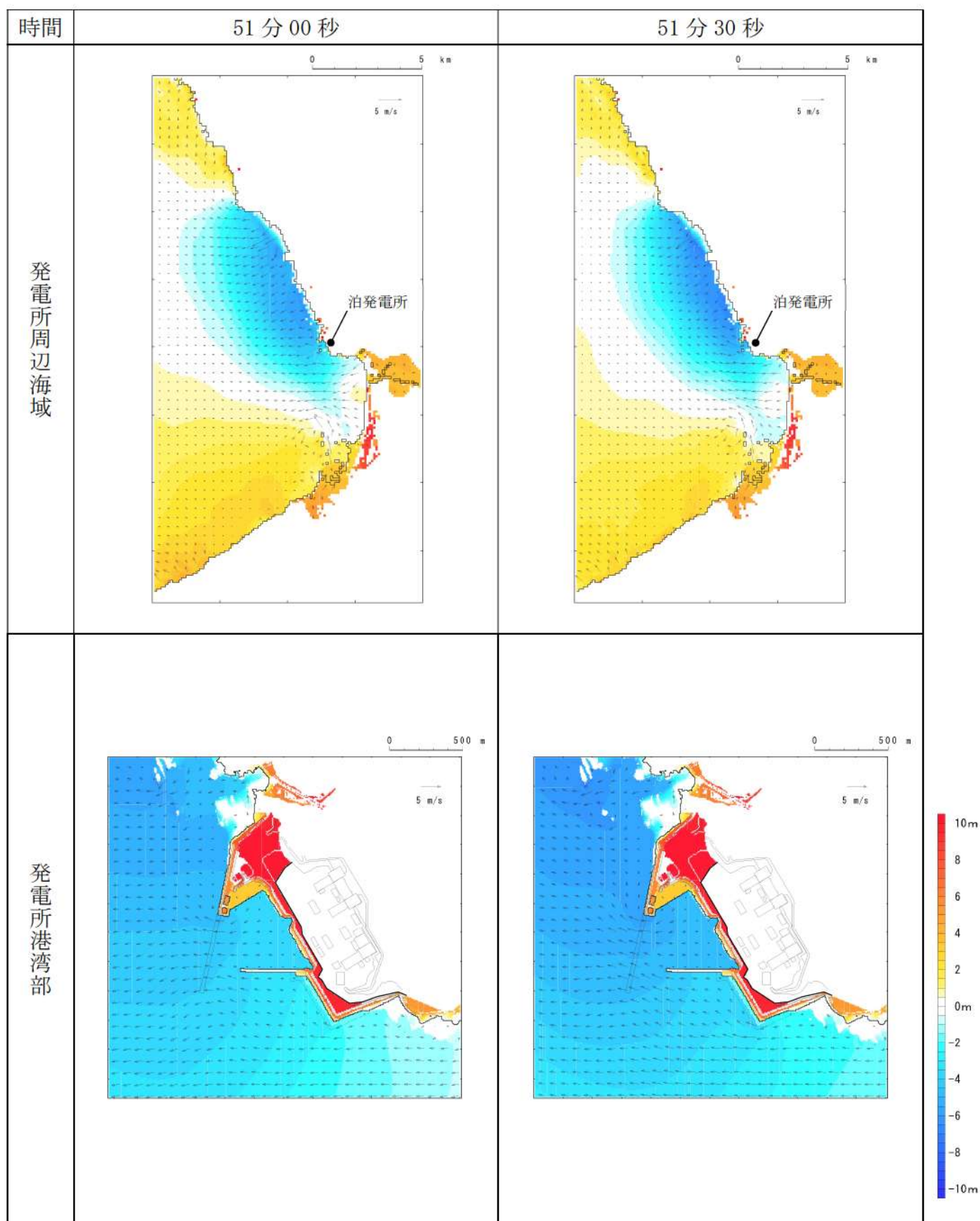
第3図-44 基準津波B（北防波堤損傷）の水位変動・流向ベクトル(44/53)
