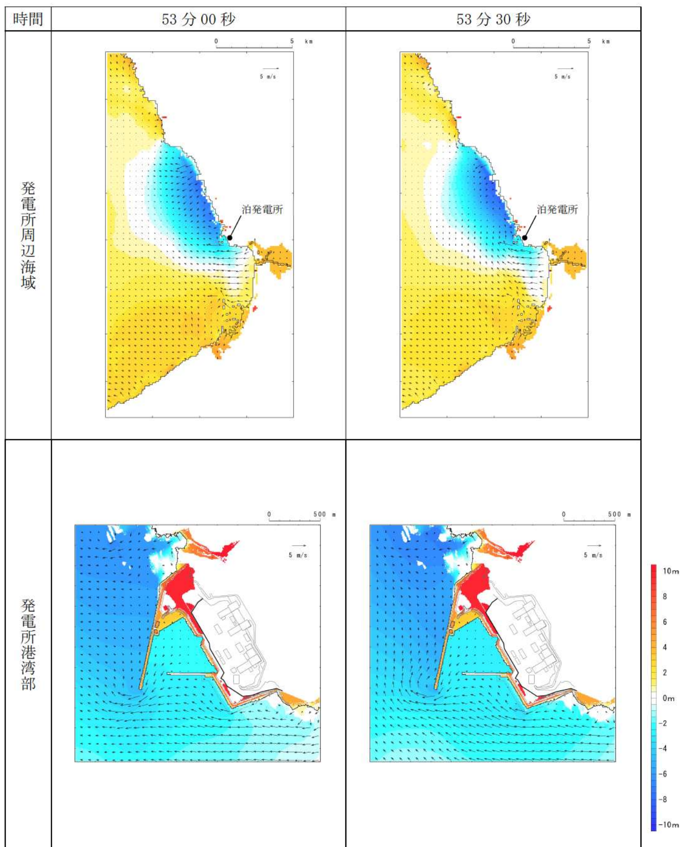
第 4 図-47 基準津波 C（防波堤損傷なし）の水位変動・流向ベクトル(47/54)
