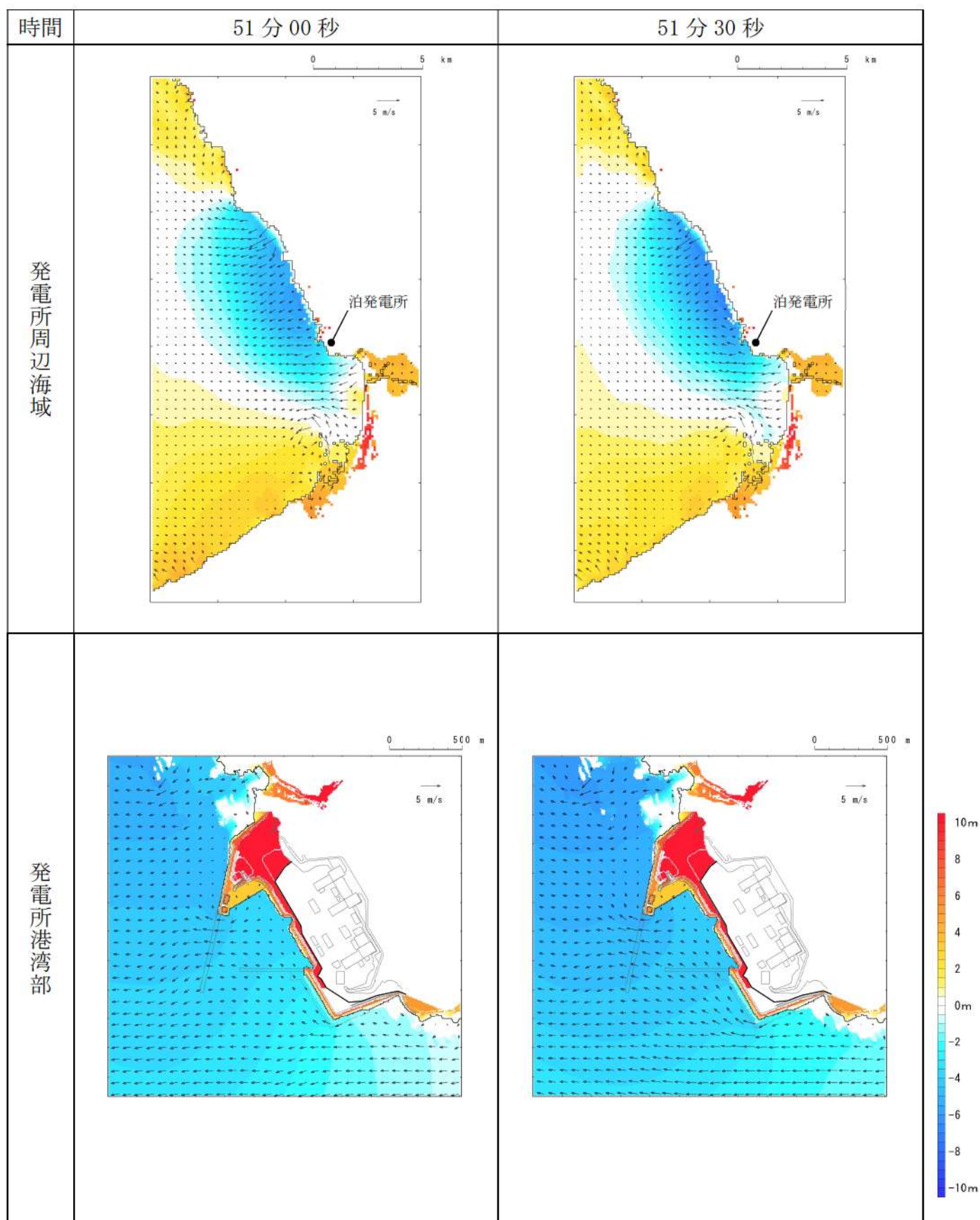
第 6 図-44 基準津波 D（北及び南防波堤損傷）の水位変動・流向ベクトル(44/53)
