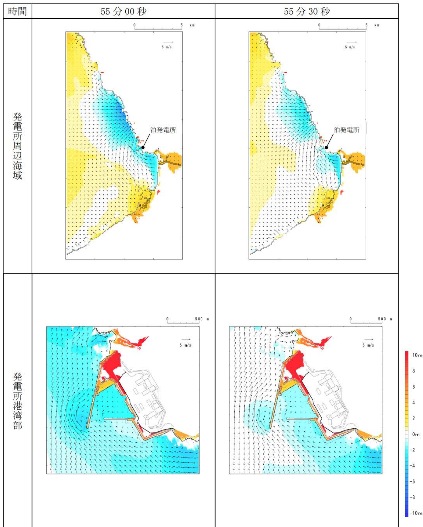
第 4 図-49 基準津波 C（防波堤損傷なし）の水位変動・流向ベクトル (49/54)
