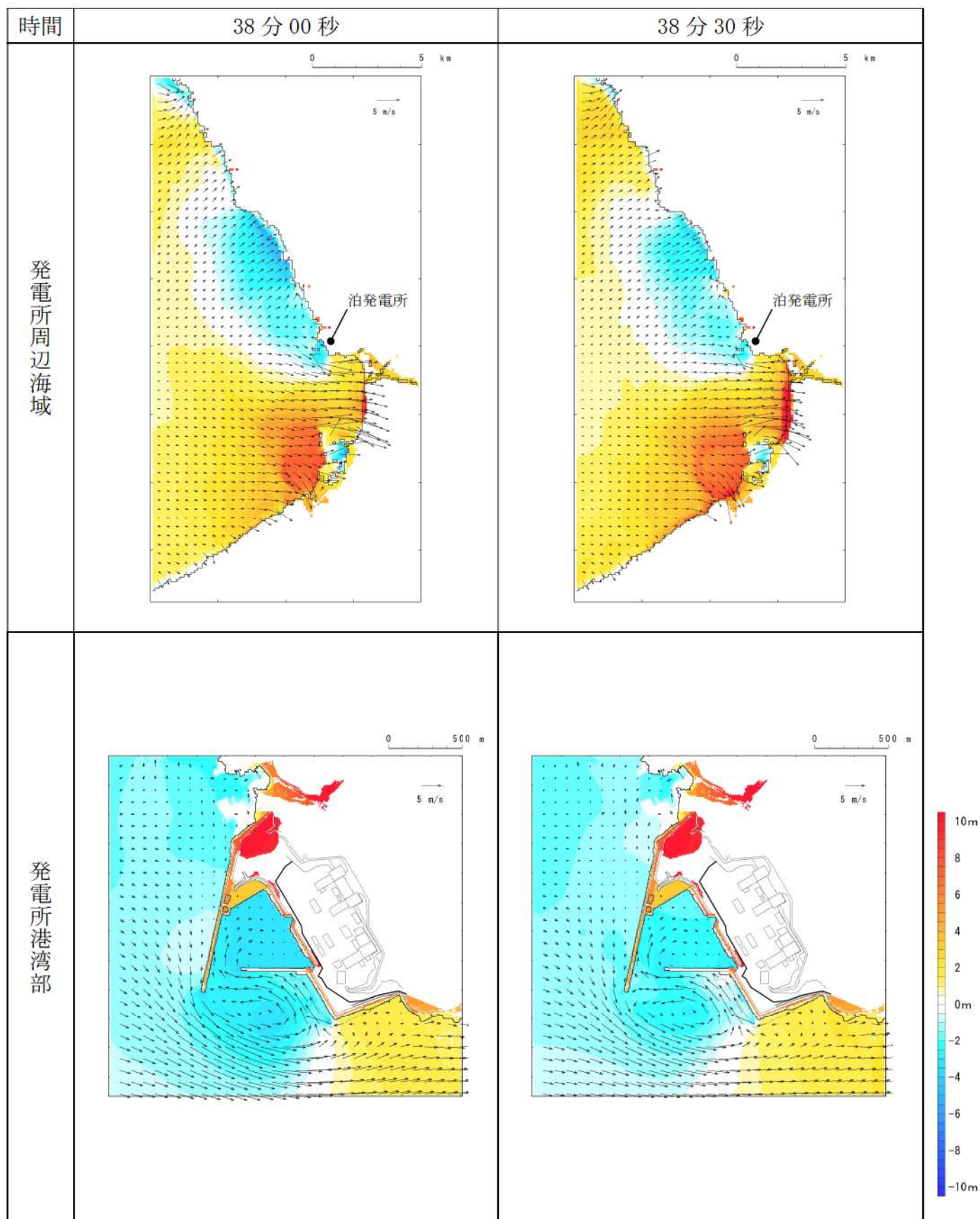
第 5 図-31 基準津波 D（防波堤損傷なし）の水位変動・流向ベクトル (31/53)
