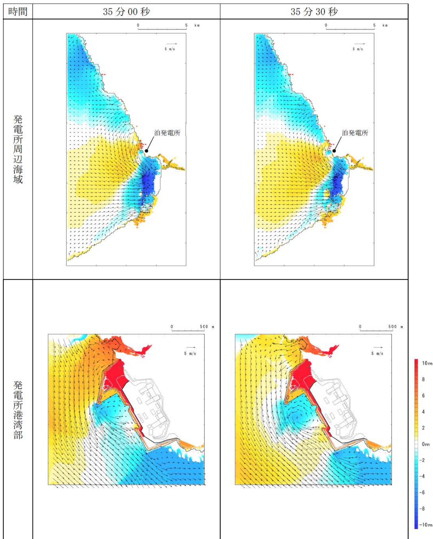
第 6 図-28 基準津波 D（北及び南防波堤損傷）の水位変動・流向ベクトル (28/53)
