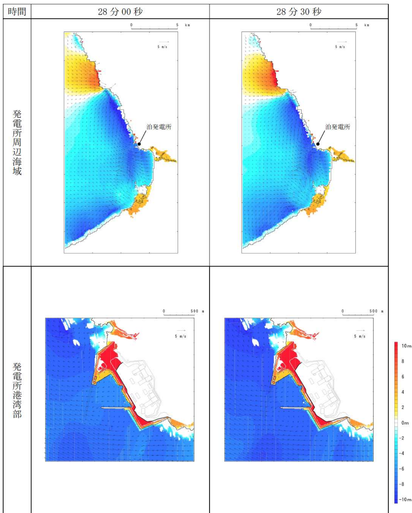
第3図-21 基準津波B（北防波堤損傷）の水位変動・流向ベクトル(21/53)
