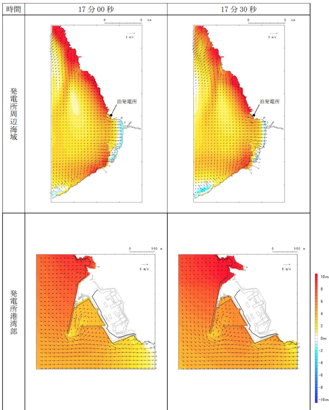
第4図-11 基準津波C（防波堤損傷なし）の水位変動・流向ベクトル(11/54)
