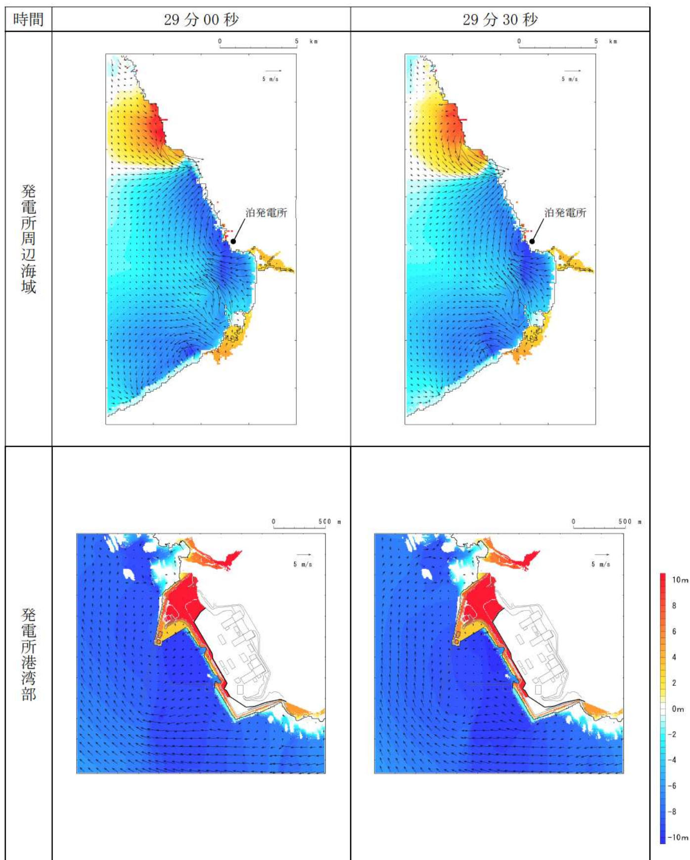
第 6 図-22 基準津波 D（北及び南防波堤損傷）の水位変動・流向ベクトル(22/53)
