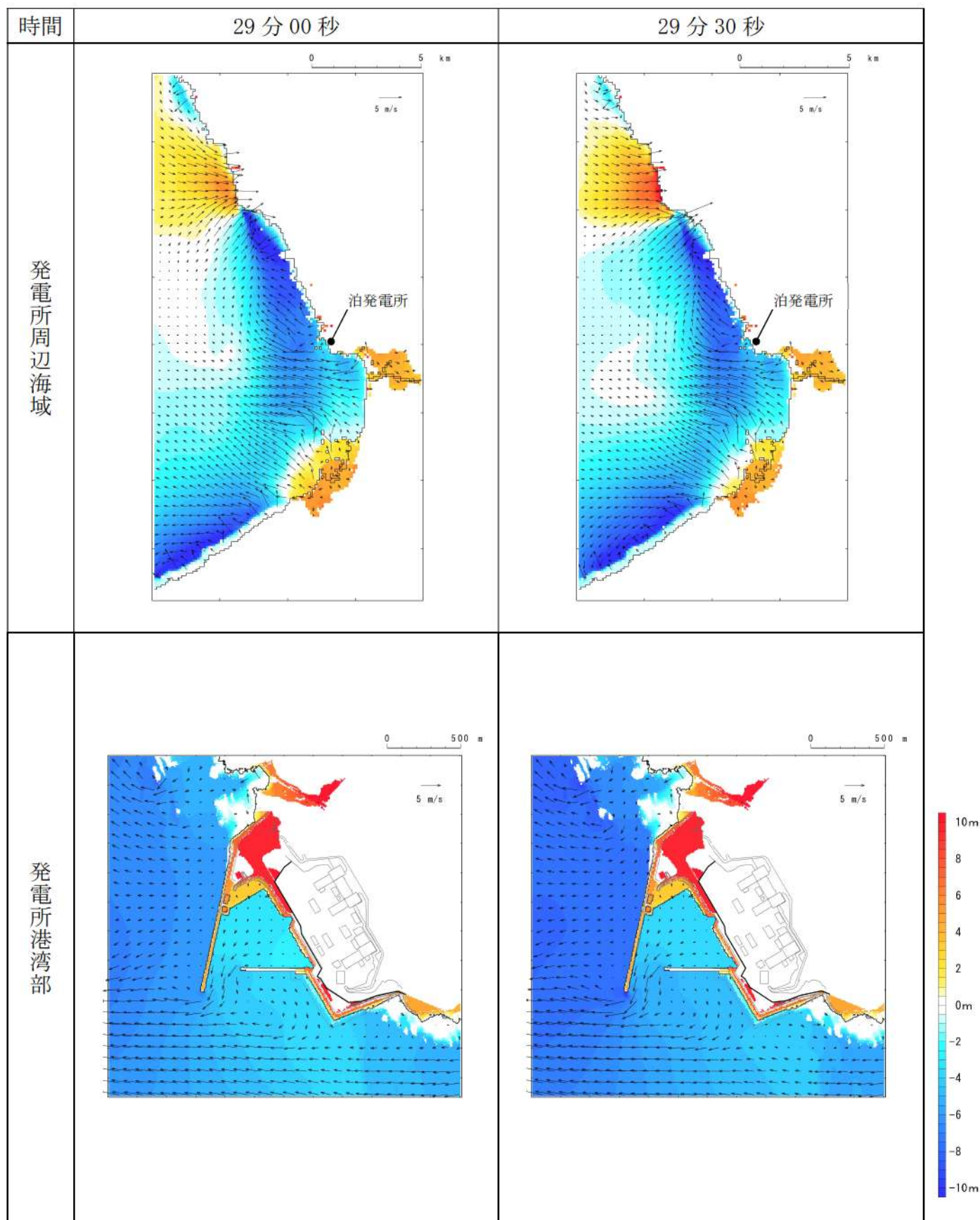
第 4 図-23 基準津波 C（防波堤損傷なし）の水位変動・流向ベクトル (23/54)
