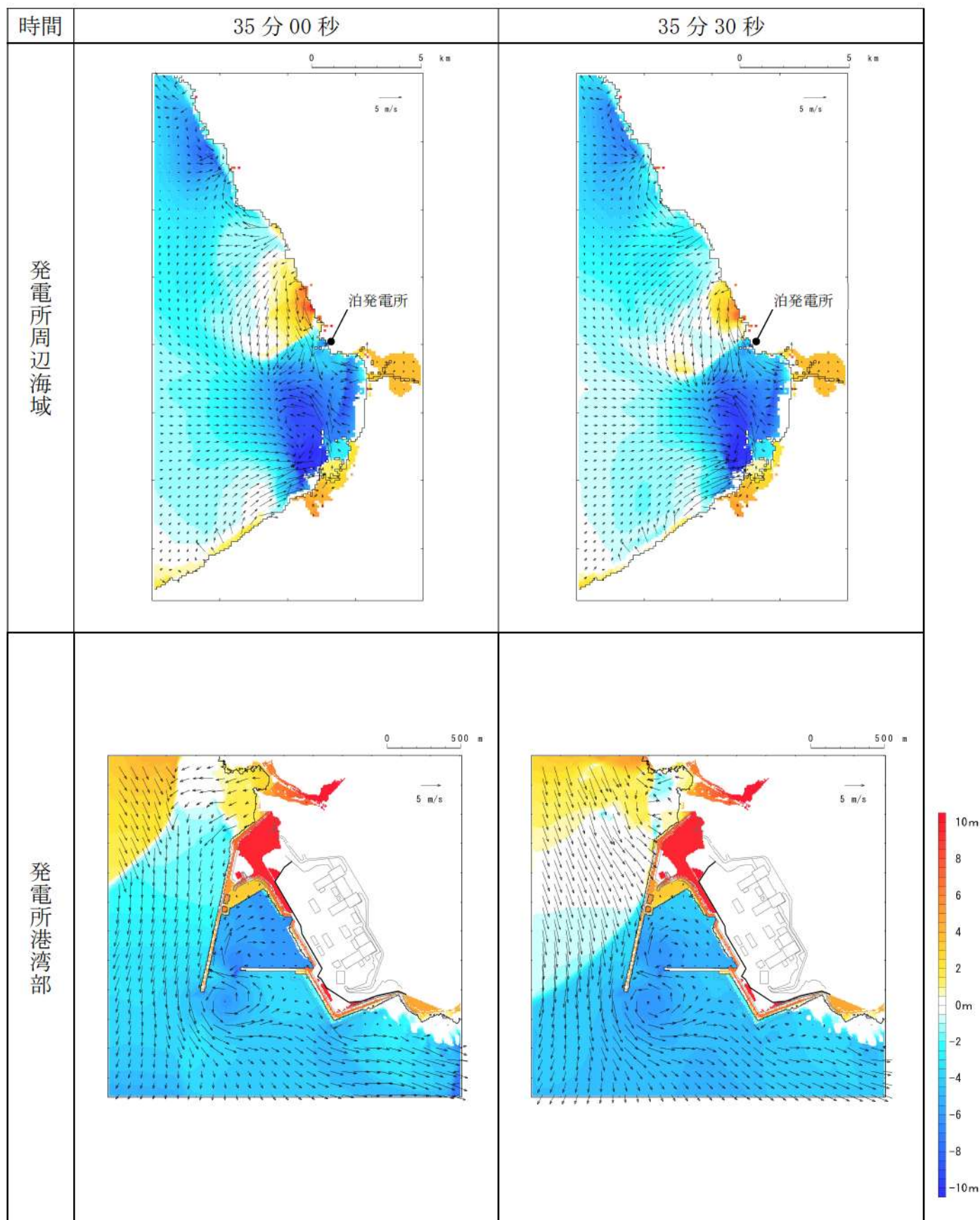
第4図-29 基準津波C（防波堤損傷なし）の水位変動・流向ベクトル(29/54)
