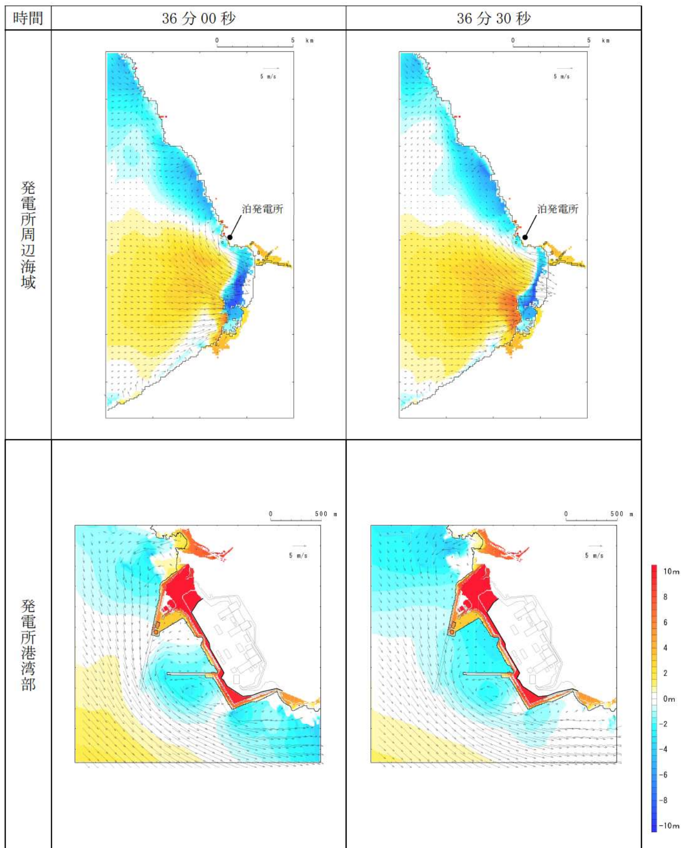
第3図-29 基準津波B（北防波堤損傷）の水位変動・流向ベクトル(29/53)
