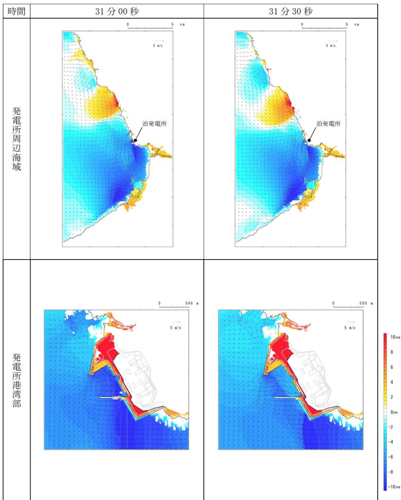
第3図-24 基準津波B（北防波堤損傷）の水位変動・流向ベクトル(24/53)
