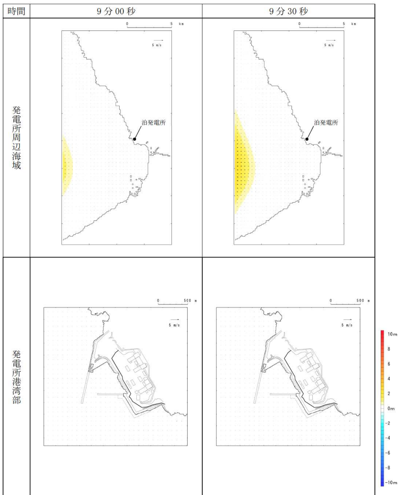
第 6 図- 2 基準津波 D（北及び南防波堤損傷）の水位変動・流向ベクトル (2/53)
