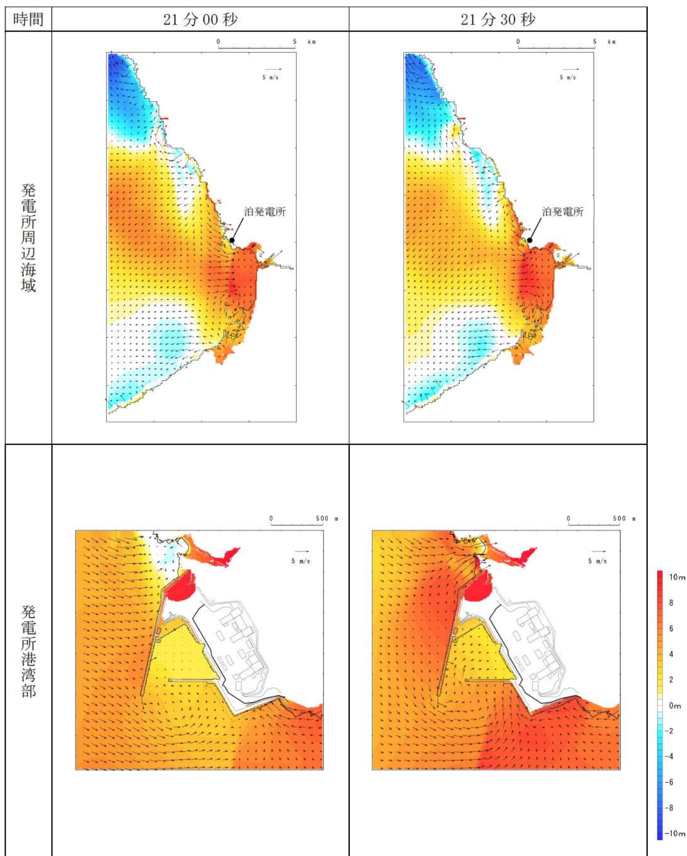
第4図-15 基準津波C（防波堤損傷なし）の水位変動・流向ベクトル(15/54)
