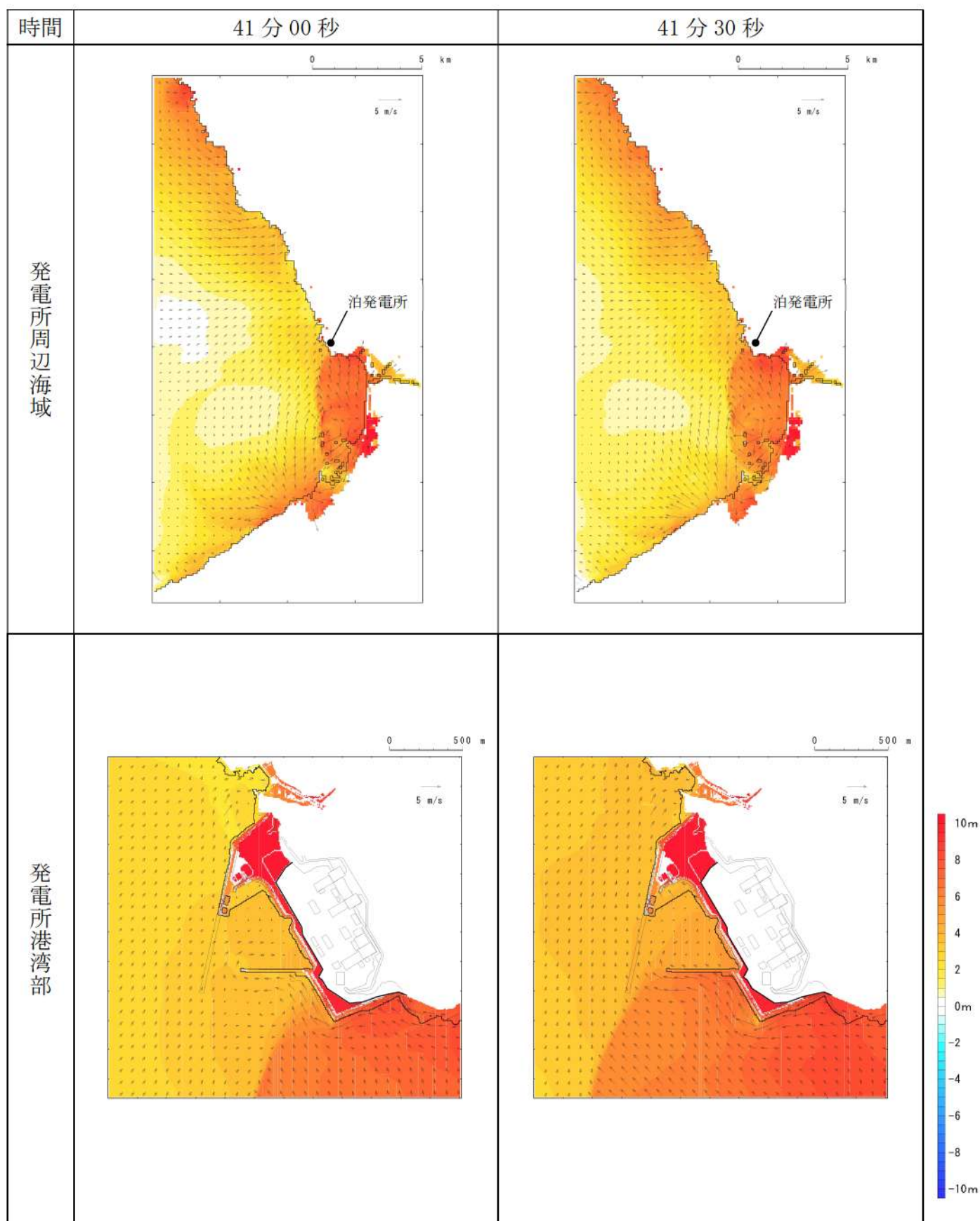
第 3 図-34 基準津波 B（北防波堤損傷）の水位変動・流向ベクトル(34/53)
