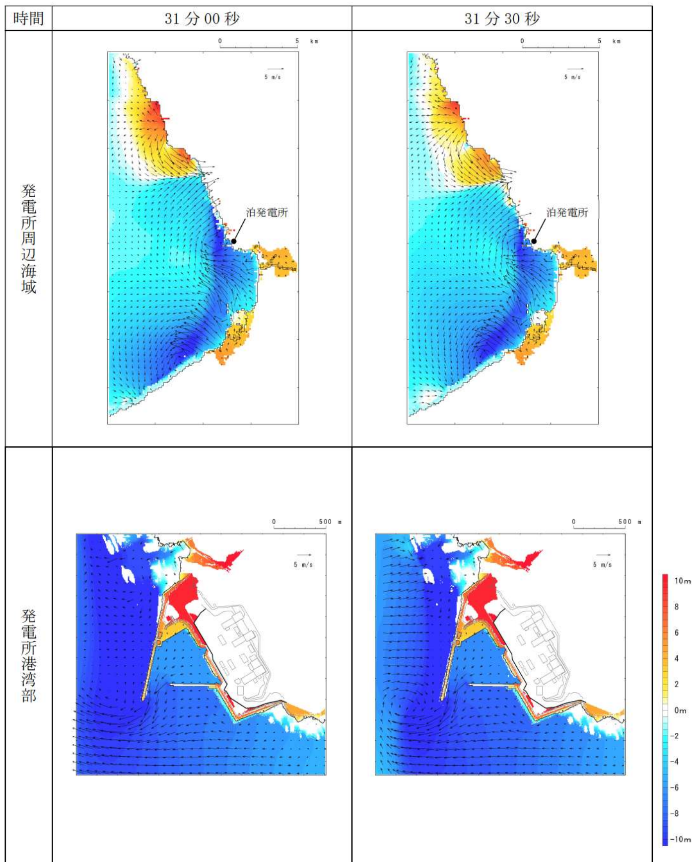
第 4 図-25 基準津波 C（防波堤損傷なし）の水位変動・流向ベクトル (25/54)
