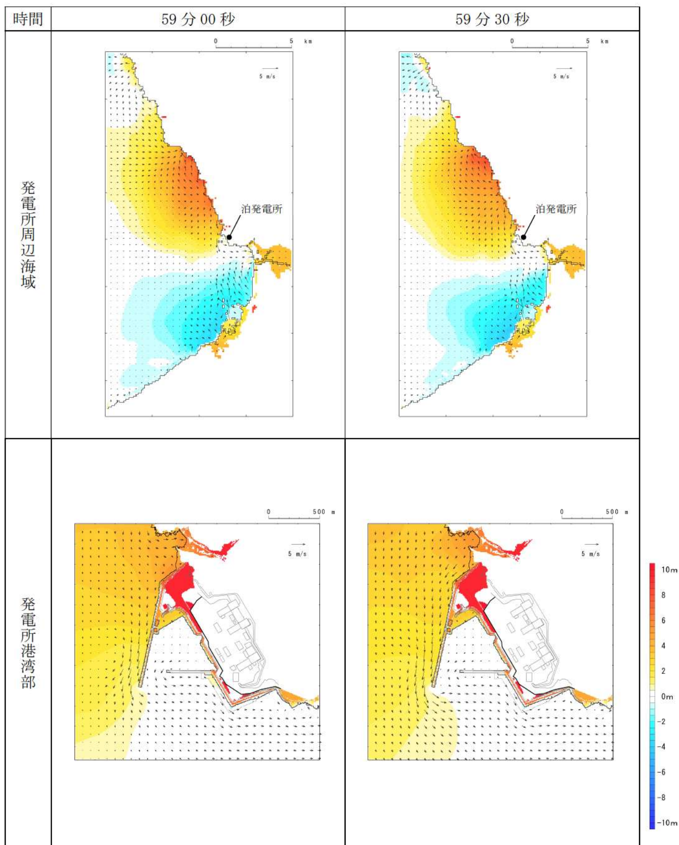
第 4 図-53 基準津波 C（防波堤損傷なし）の水位変動・流向ベクトル (53/54)
