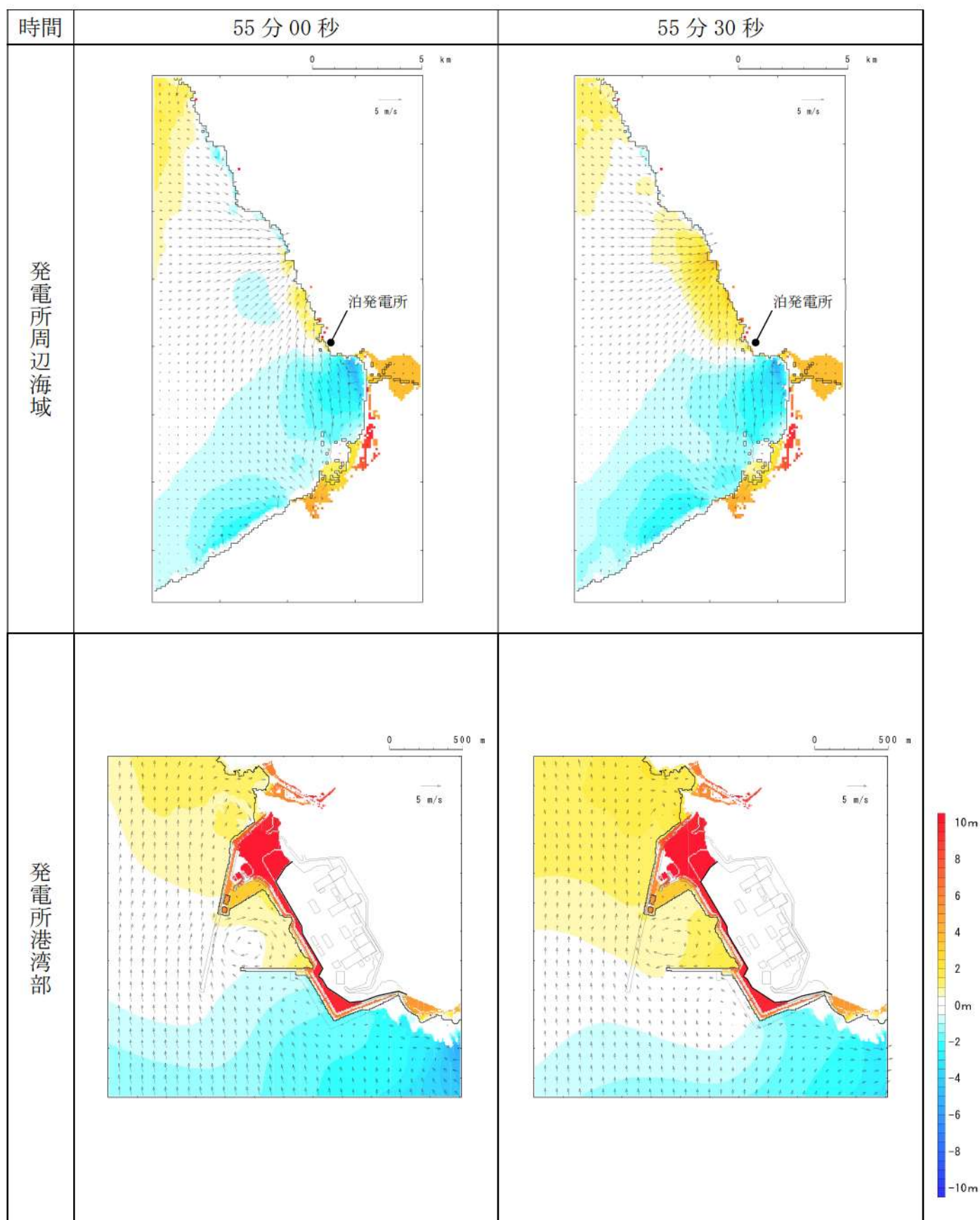
第3図-48 基準津波B（北防波堤損傷）の水位変動・流向ベクトル(48/53)
