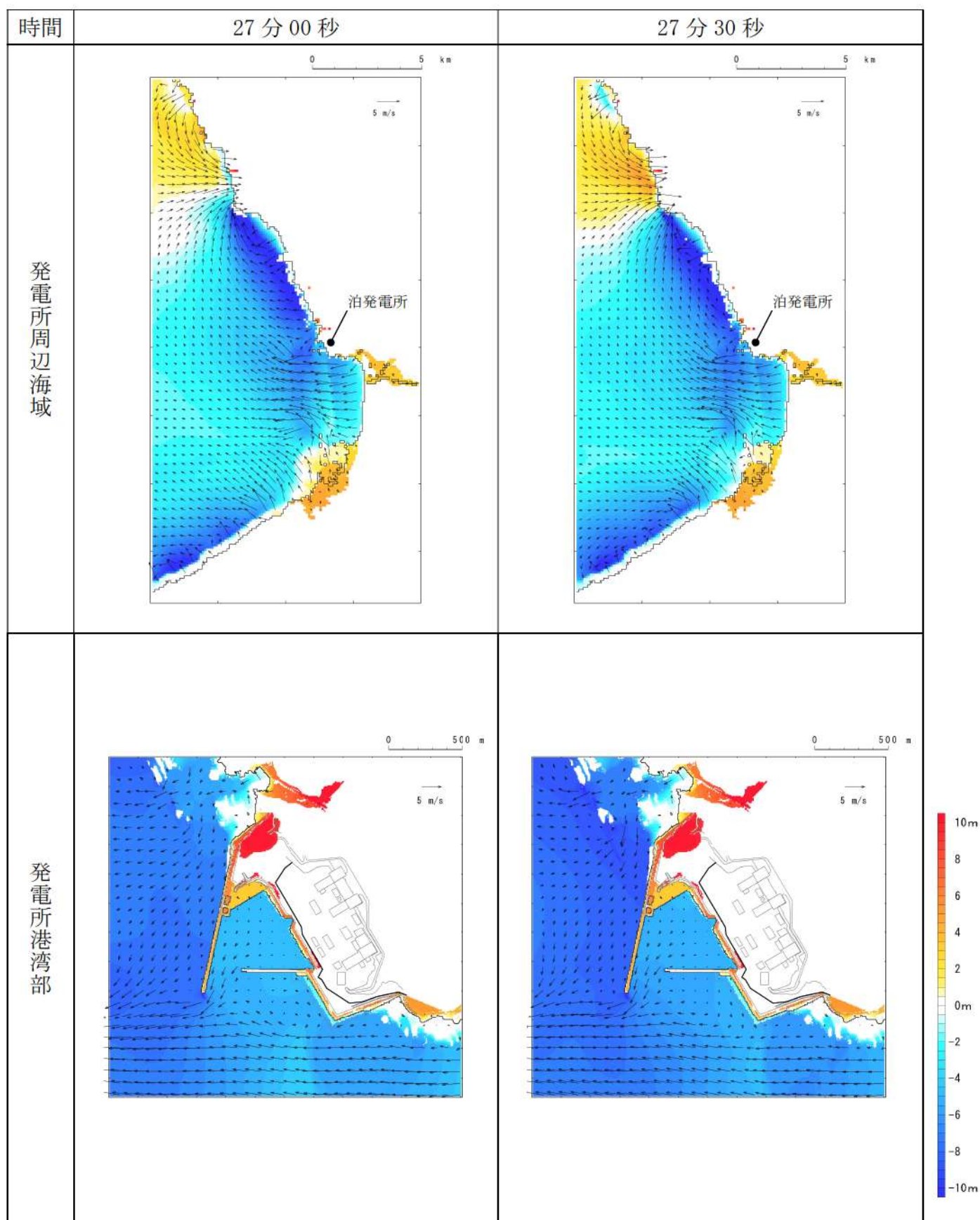
第 5 図-20 基準津波 D（防波堤損傷なし）の水位変動・流向ベクトル (20/53)
