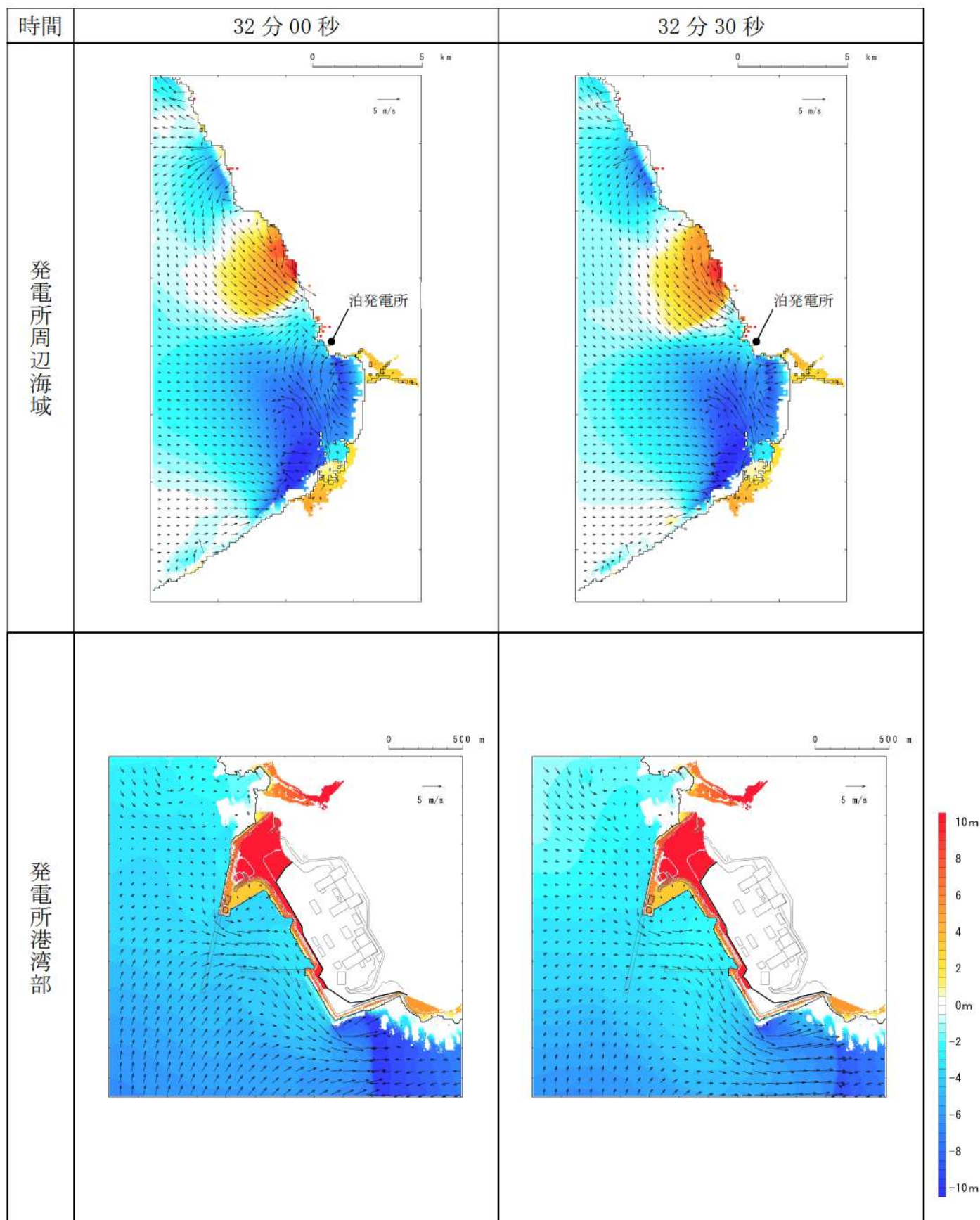
第 6 図-25 基準津波 D（北及び南防波堤損傷）の水位変動・流向ベクトル (25/53)
