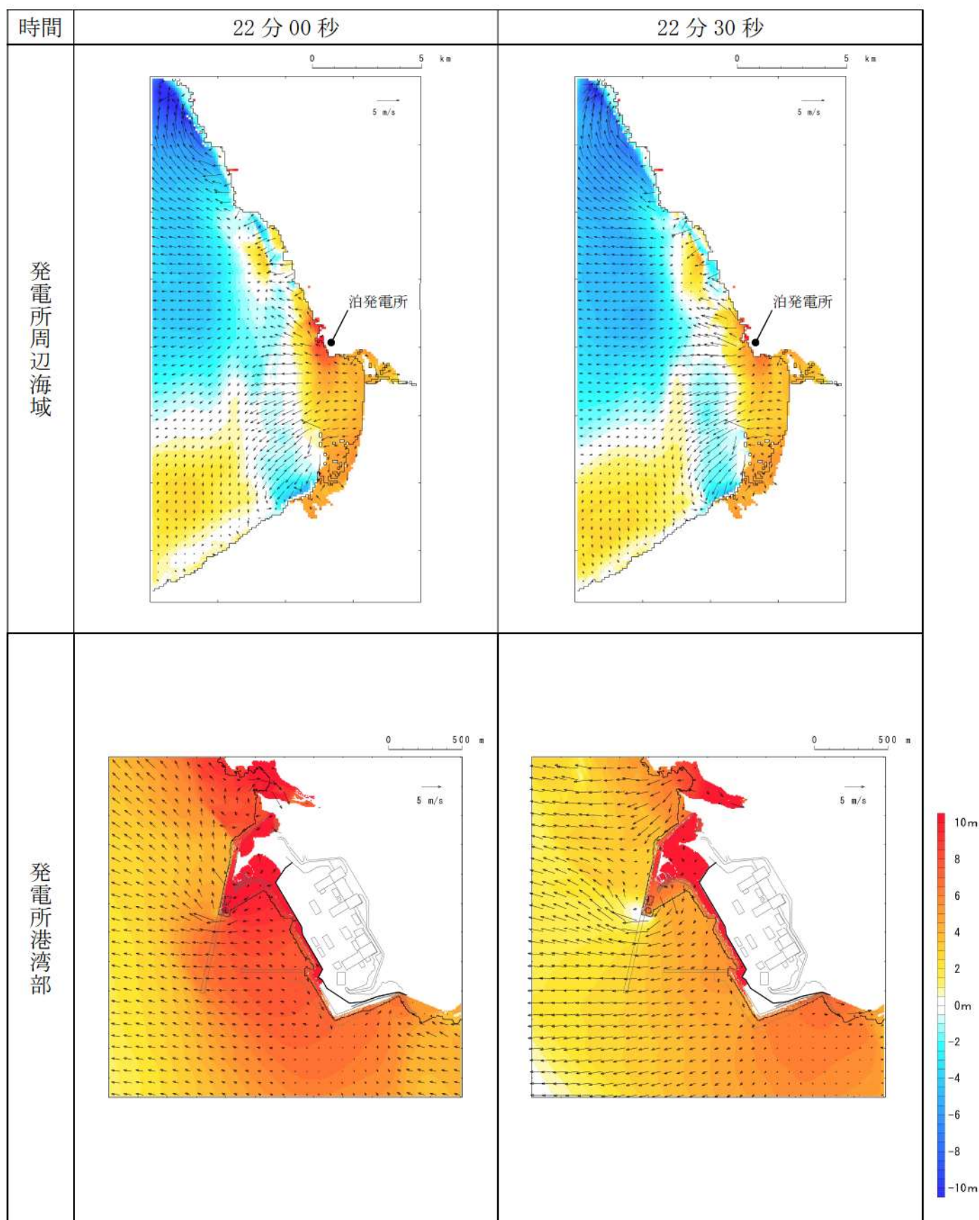
第 6 図-15 基準津波 D（北及び南防波堤損傷）の水位変動・流向ベクトル(15/53)
