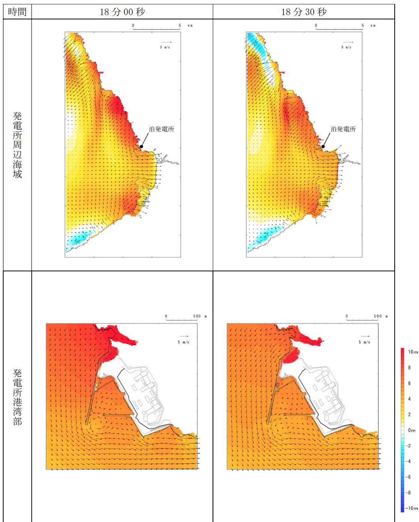
第4図-12 基準津波C（防波堤損傷なし）の水位変動・流向ベクトル(12/54)
