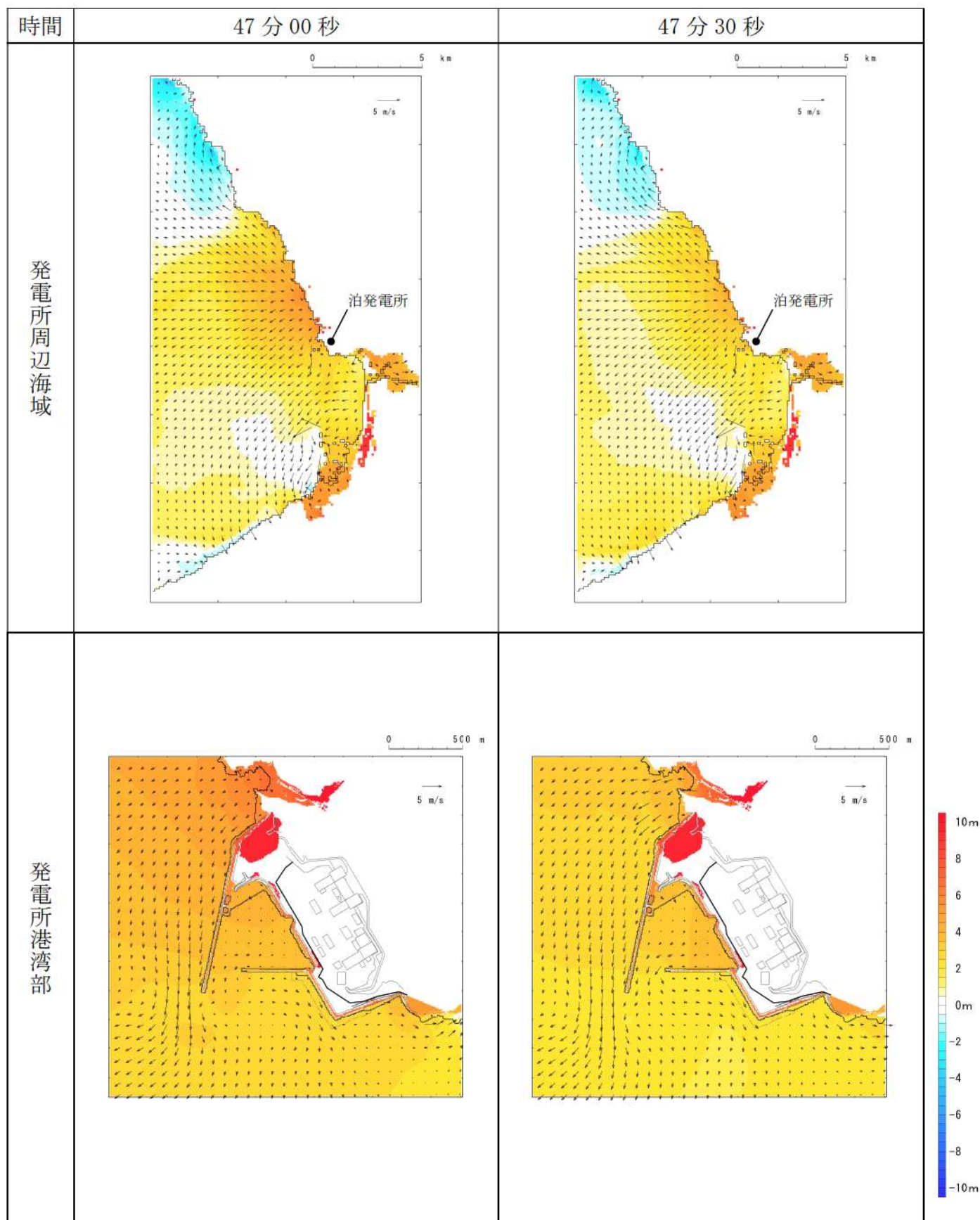
第 5 図-40 基準津波 D (防波堤損傷なし) の水位変動・流向ベクトル (40/53)
