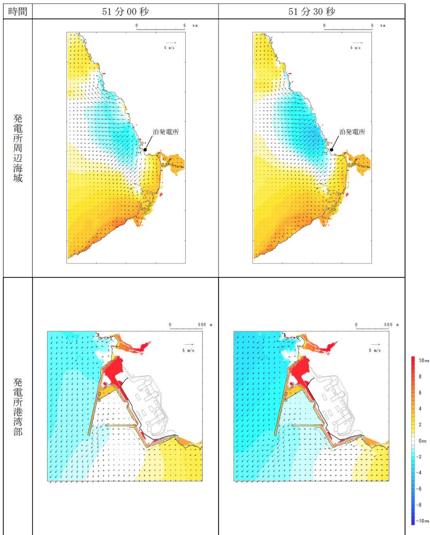
第 4 図-45 基準津波 C（防波堤損傷なし）の水位変動・流向ベクトル(45/54)
