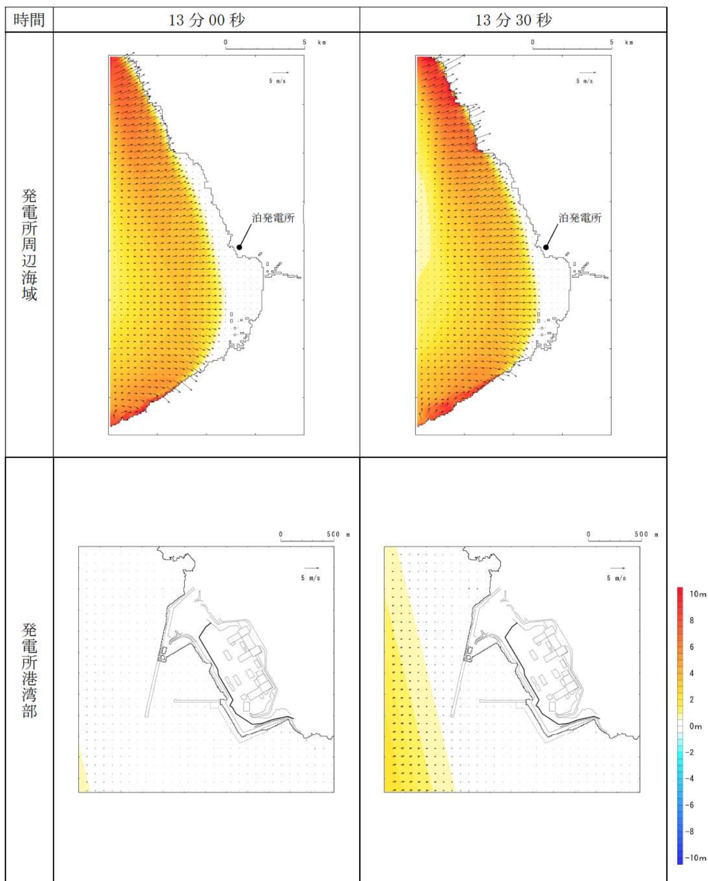
第 6 図-6 基準津波 D（北及び南防波堤損傷）の水位変動・流向ベクトル(6/53)
