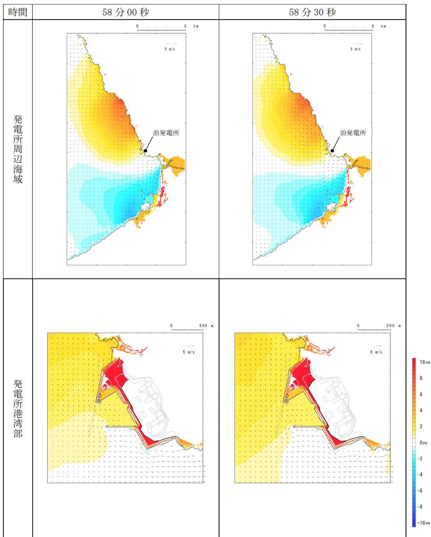
第3図-51 基準津波B（北防波堤損傷）の水位変動・流向ベクトル(51/53)
