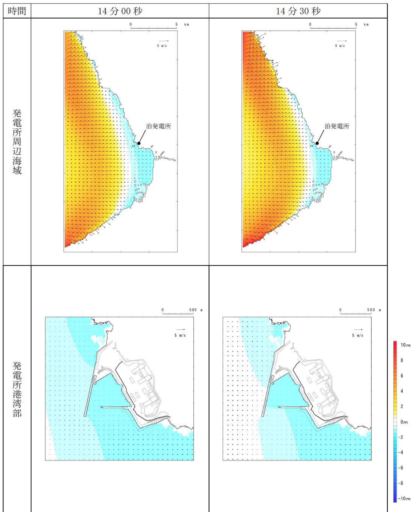
第4図-8 基準津波C（防波堤損傷なし）の水位変動・流向ベクトル(8/54)
