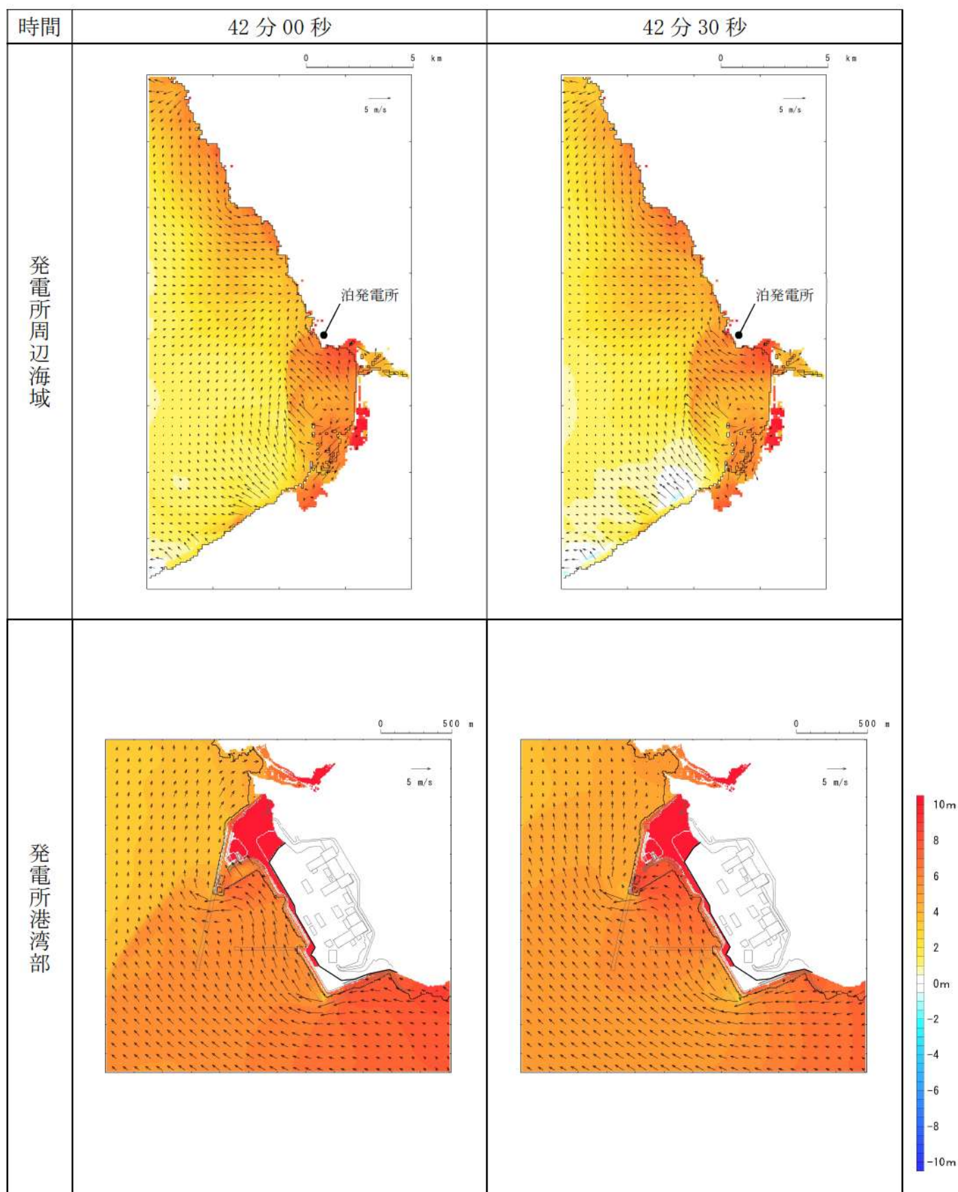
第 6 図-35 基準津波 D（北及び南防波堤損傷）の水位変動・流向ベクトル(35/53)
