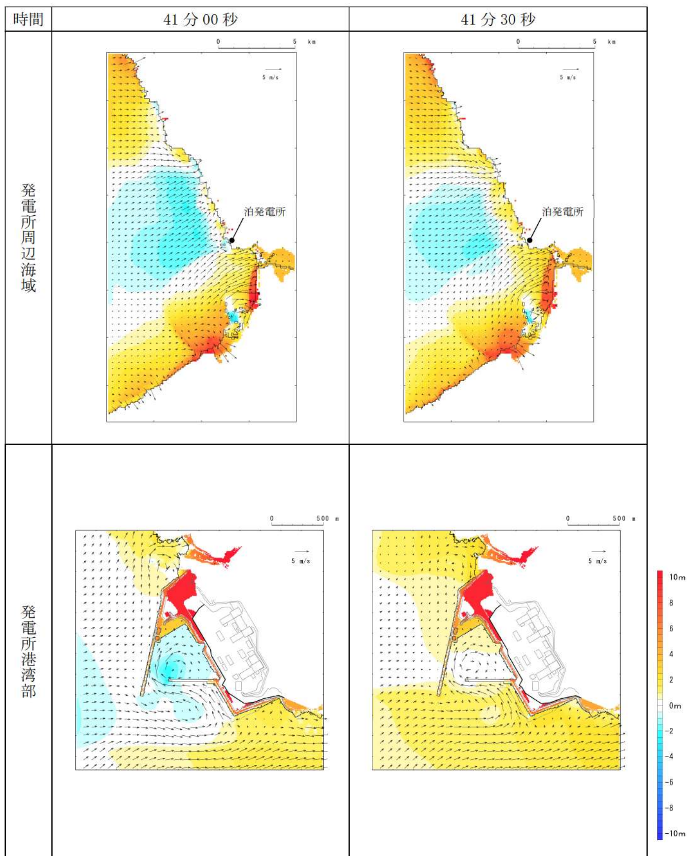
第4図-35 基準津波C（防波堤損傷なし）の水位変動・流向ベクトル(35/54)
