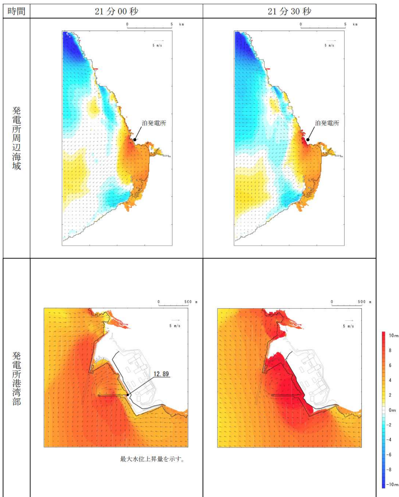
第3図-14 基準津波B（北防波堤損傷）の水位変動・流向ベクトル(14/53)
