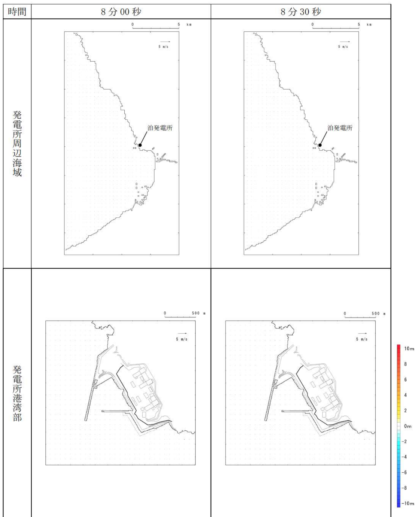
第5図-1 基準津波D（防波堤損傷なし）の水位変動・流向ベクトル(1/53)
