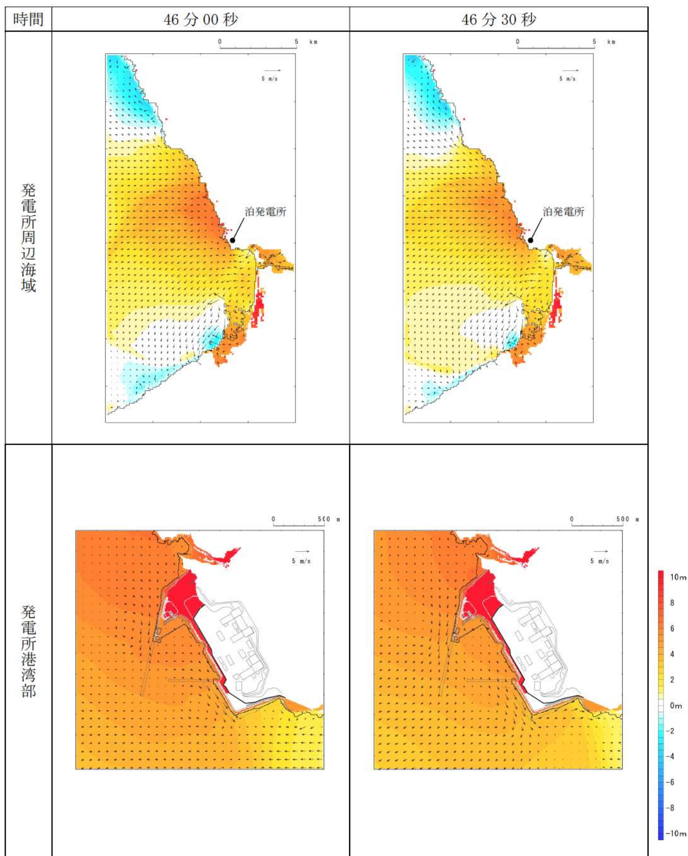
第 6 図-39 基準津波 D（北及び南防波堤損傷）の水位変動・流向ベクトル(39/53)
