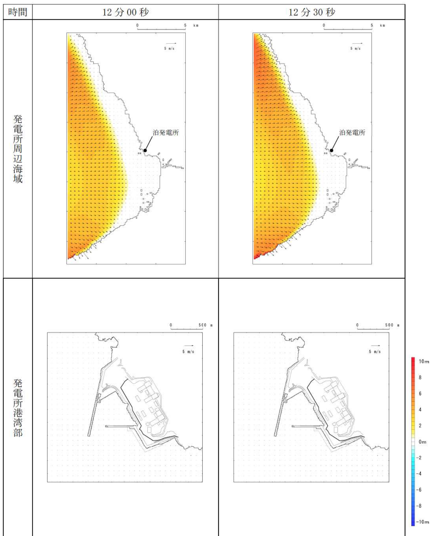
第5図-5 基準津波D（防波堤損傷なし）の水位変動・流向ベクトル(5/53)
