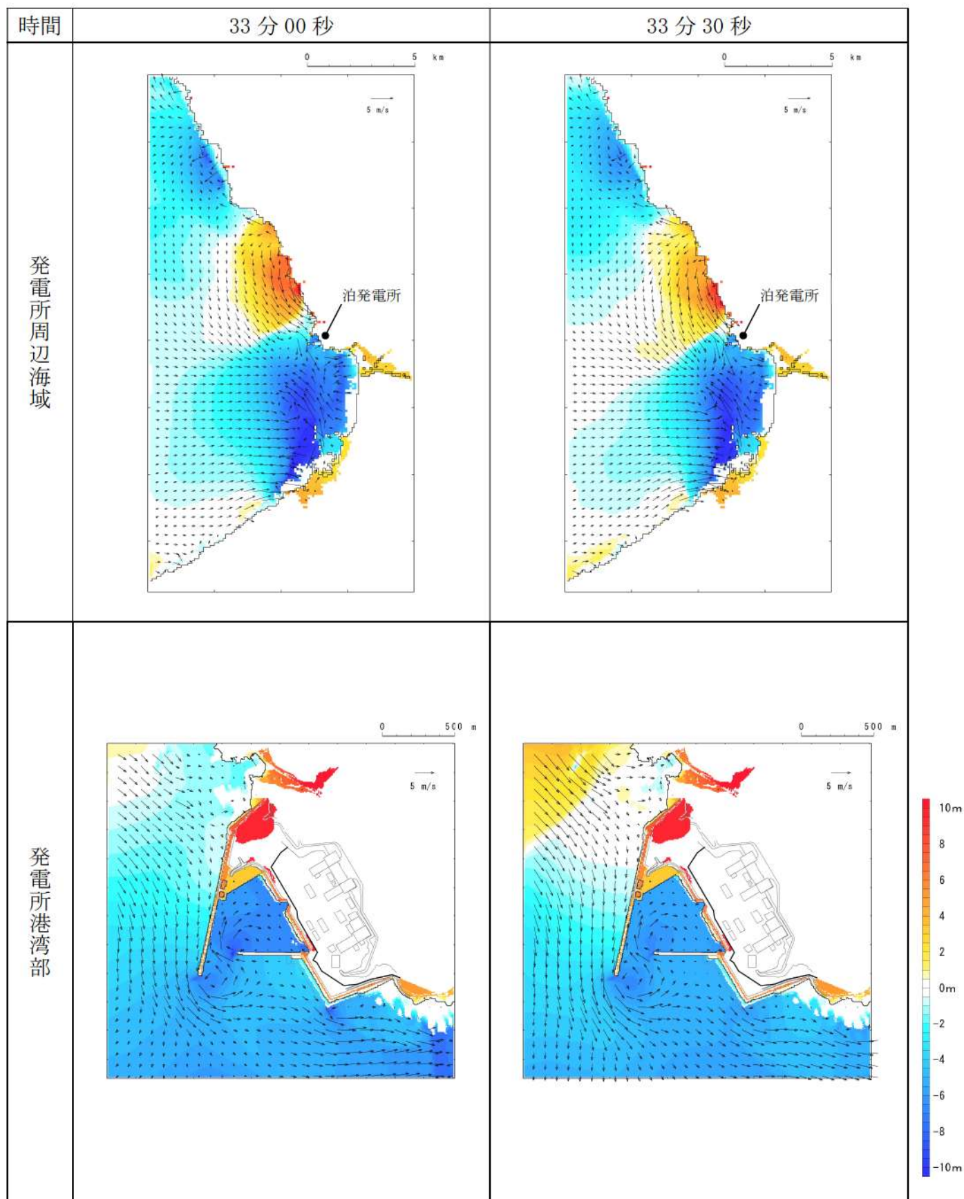
第 5 図-26 基準津波 D (防波堤損傷なし) の水位変動・流向ベクトル (26/53)
