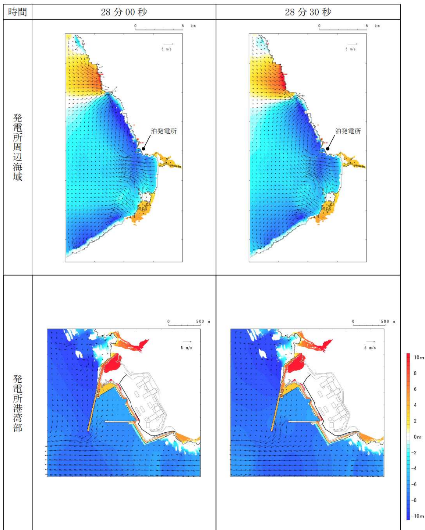
第 5 図-21 基準津波 D（防波堤損傷なし）の水位変動・流向ベクトル (21/53)
