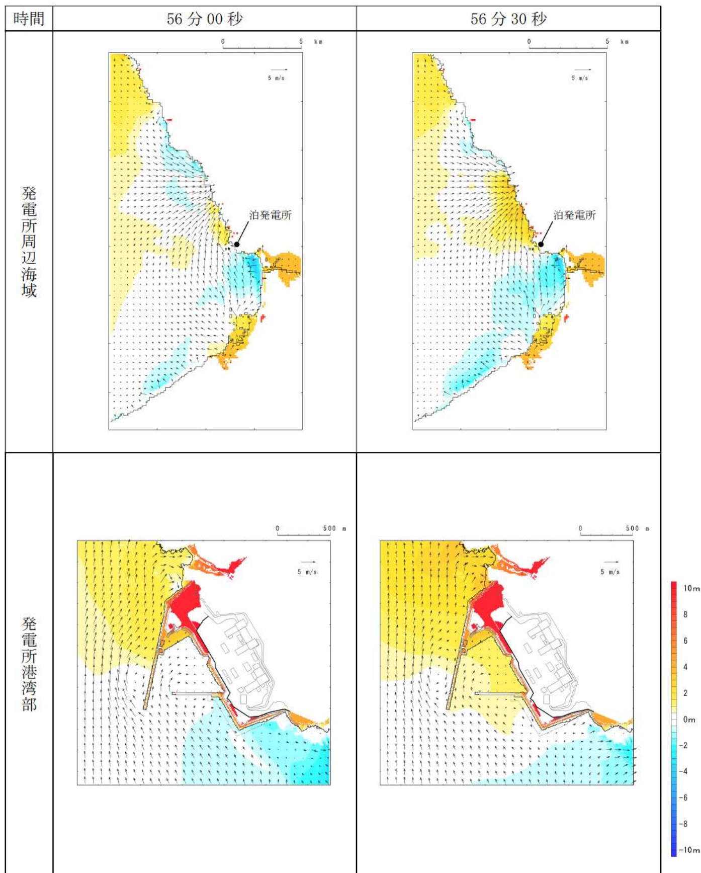
第4図-50 基準津波C（防波堤損傷なし）の水位変動・流向ベクトル(50/54)
