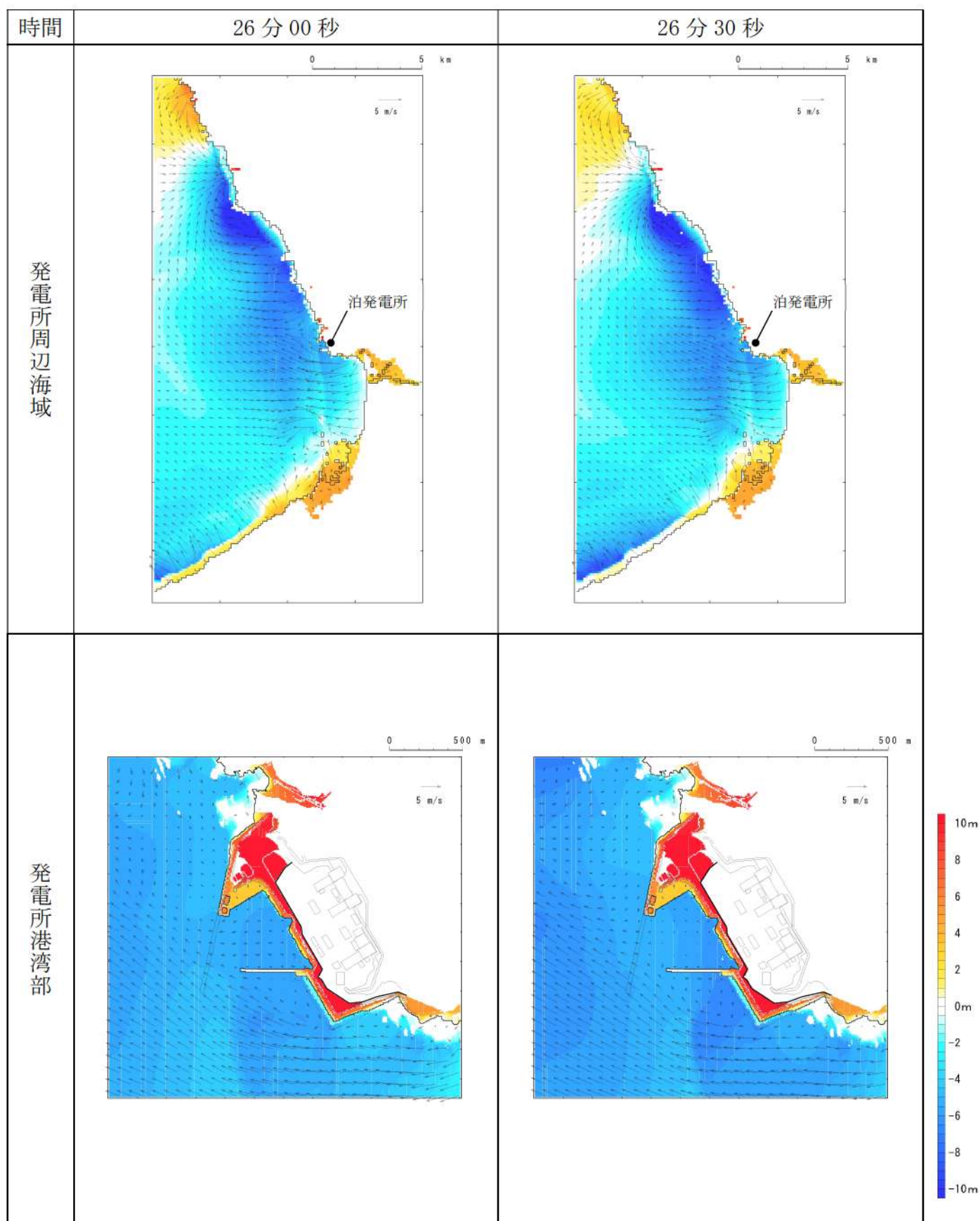
第3図-19 基準津波B（北防波堤損傷）の水位変動・流向ベクトル(19/53)
