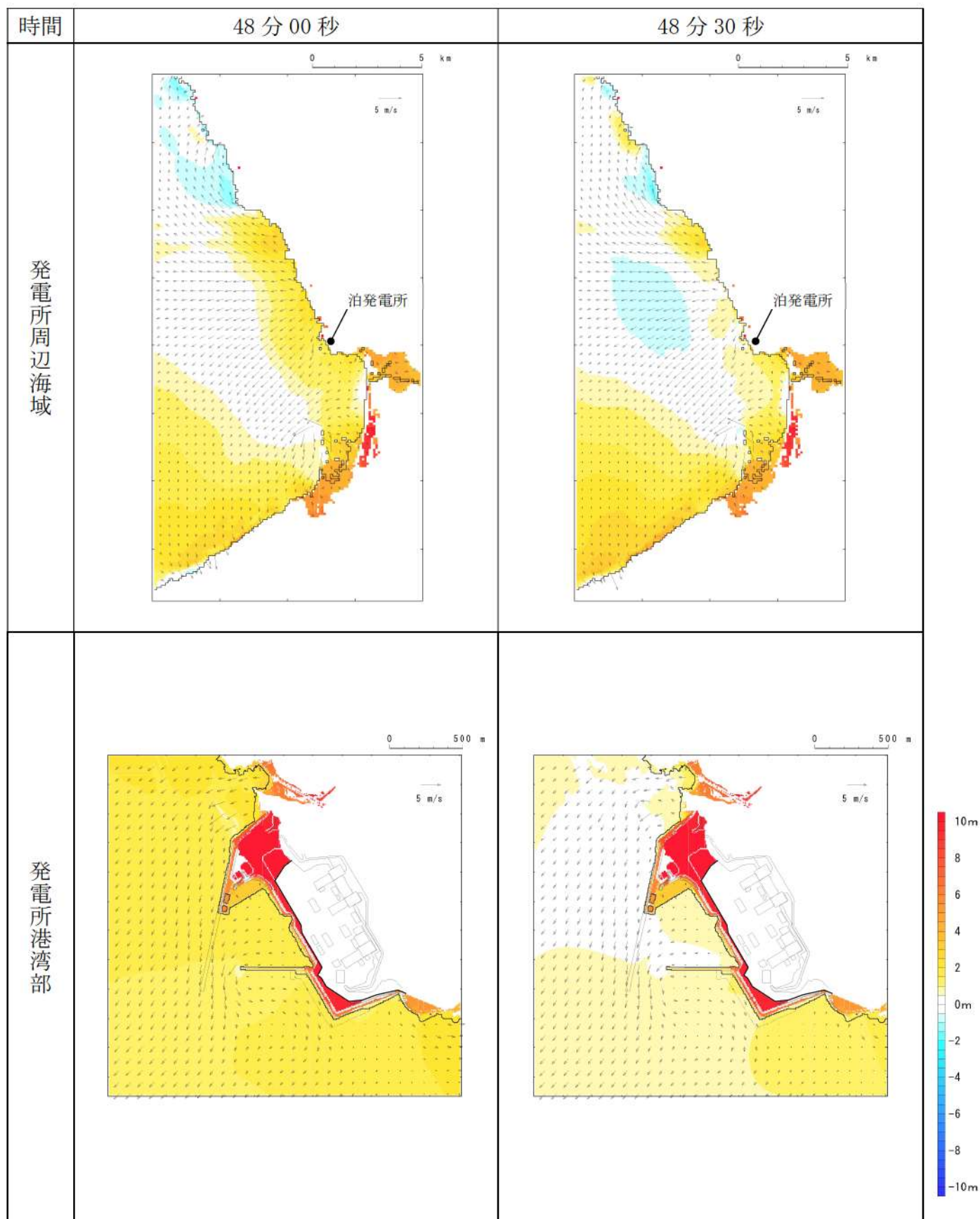
第3図-41 基準津波B（北防波堤損傷）の水位変動・流向ベクトル(41/53)
