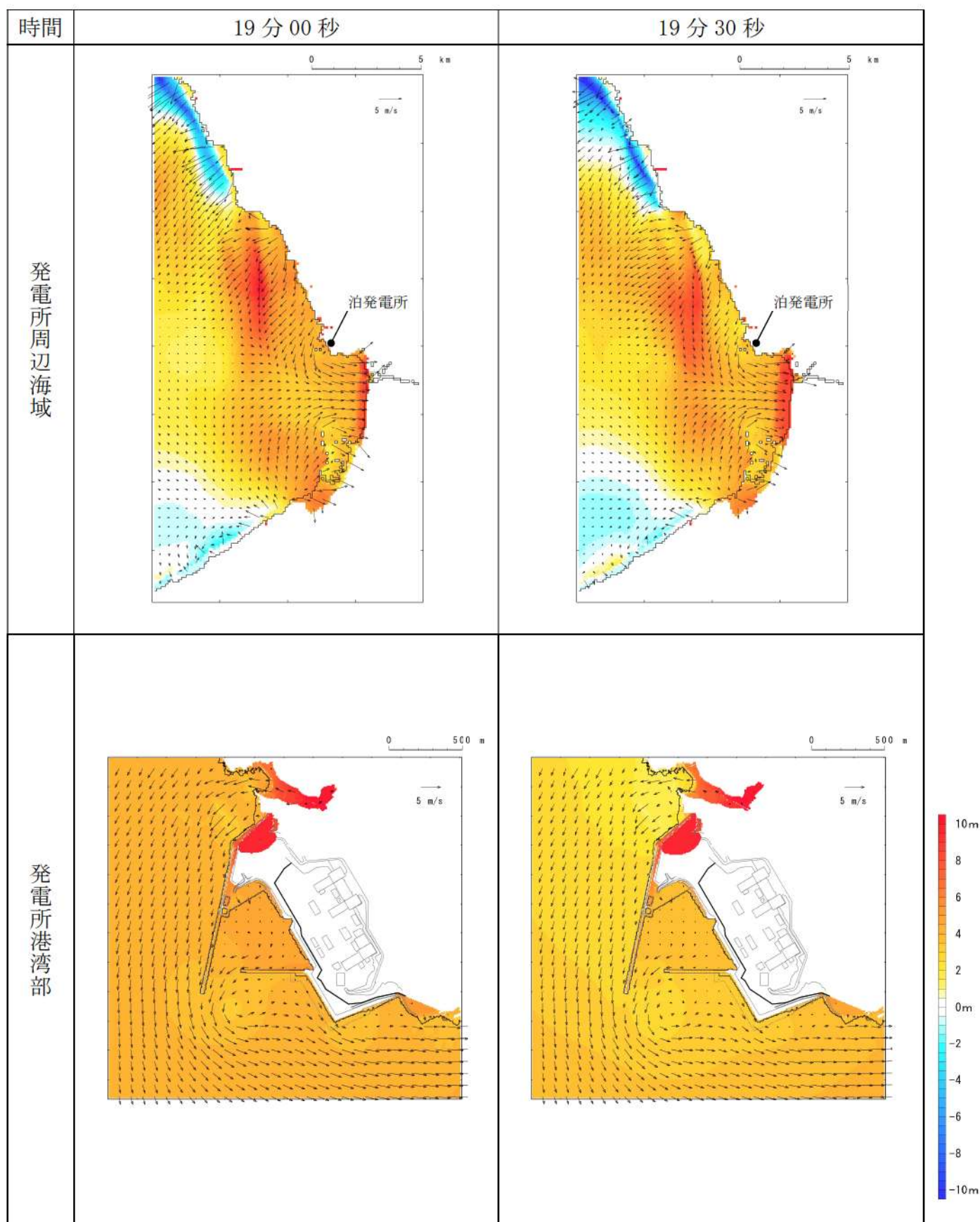
第4図-13 基準津波C（防波堤損傷なし）の水位変動・流向ベクトル(13/54)
