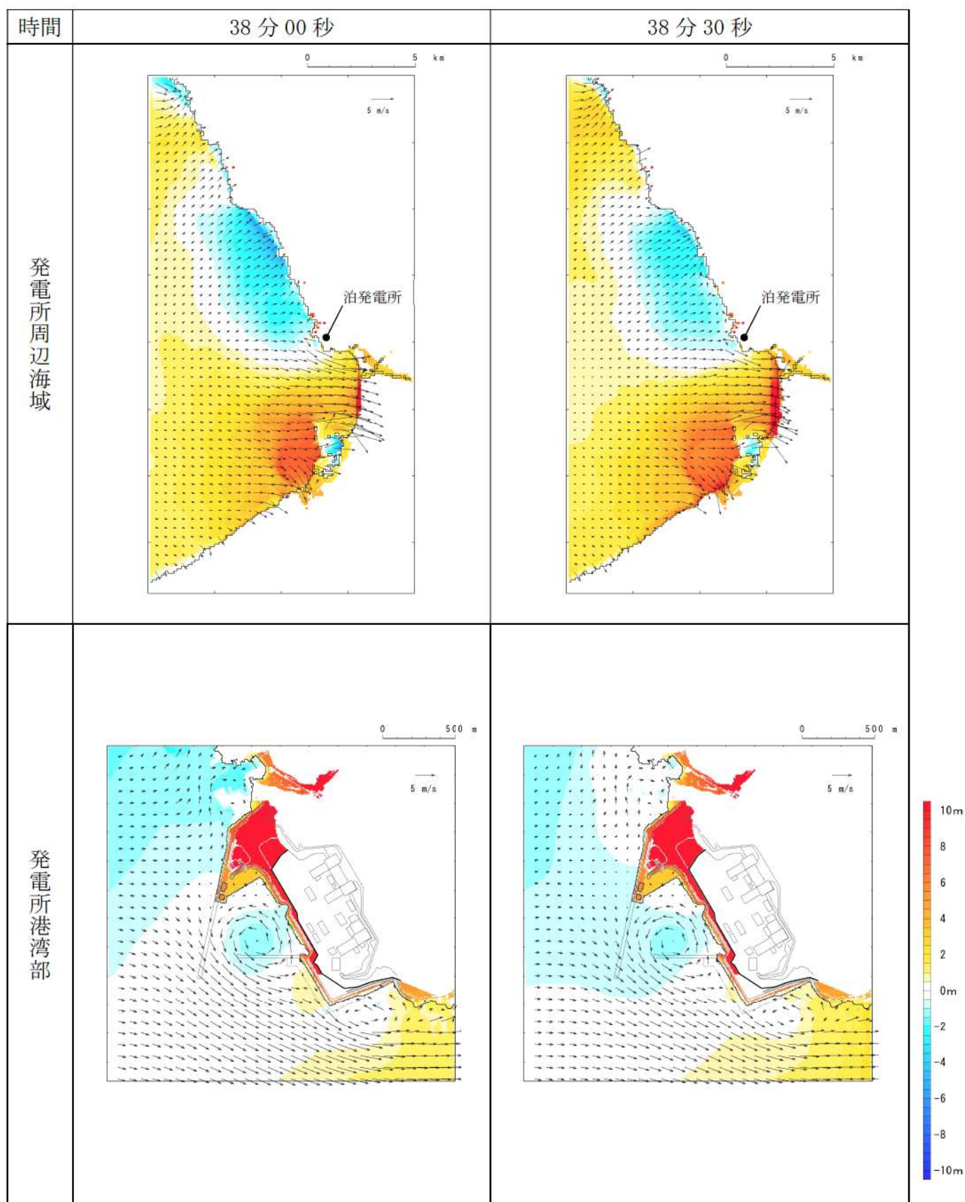
第 6 図-31 基準津波 D（北及び南防波堤損傷）の水位変動・流向ベクトル(31/53)
