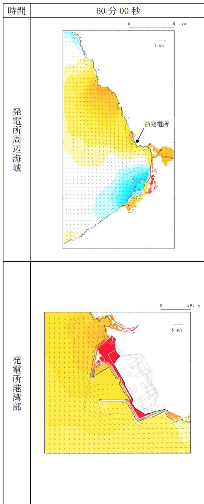
第 3 図-53 基準津波 B（北防波堤損傷）の水位変動・流向ベクトル(53/53)
