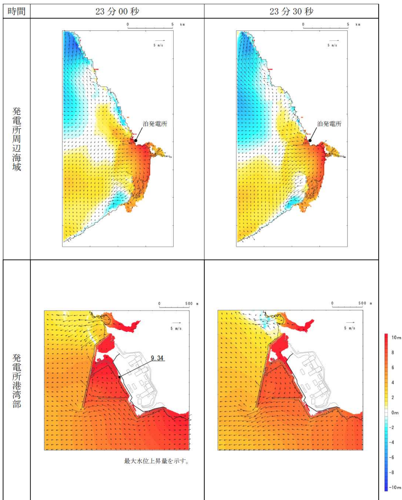
第4図-17 基準津波C（防波堤損傷なし）の水位変動・流向ベクトル(17/54)
