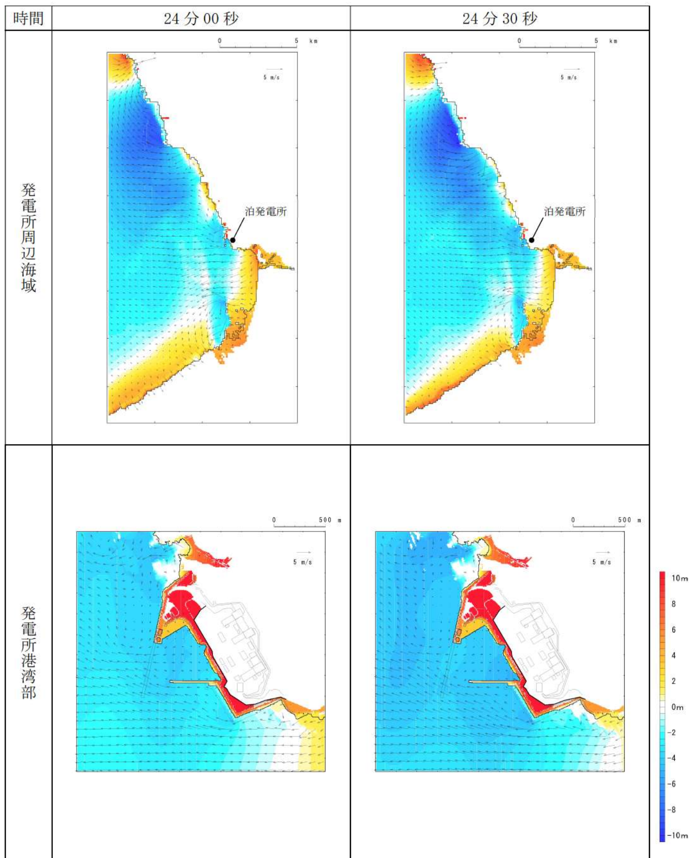
第3図-17 基準津波B（北防波堤損傷）の水位変動・流向ベクトル(17/53)
