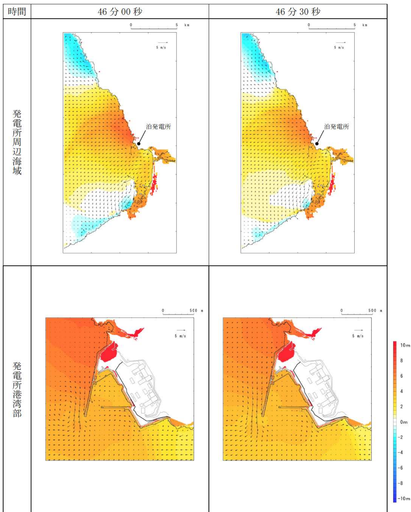
第 5 図-39 基準津波 D（防波堤損傷なし）の水位変動・流向ベクトル (39/53)
