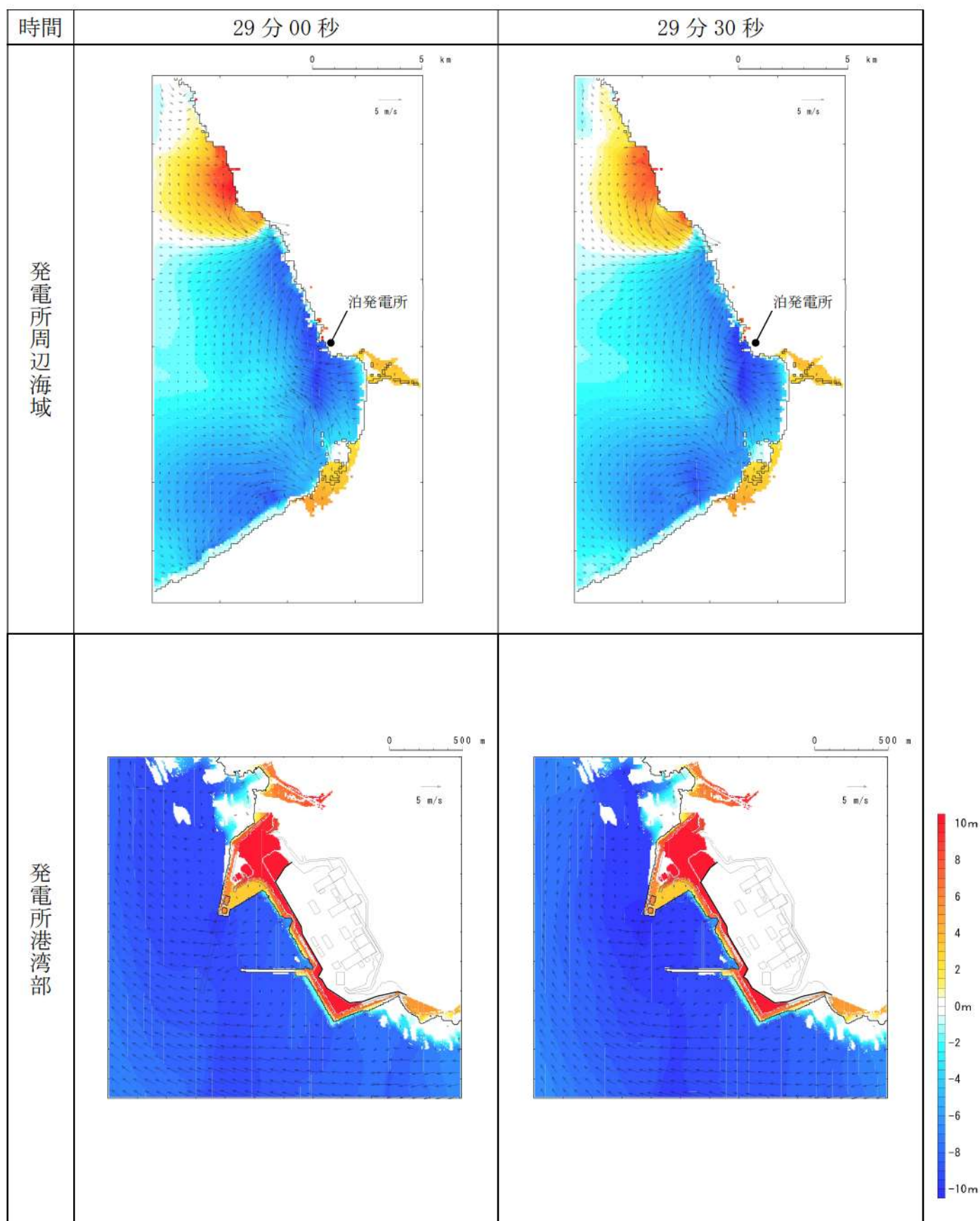
第3図-22 基準津波B（北防波堤損傷）の水位変動・流向ベクトル(22/53)
