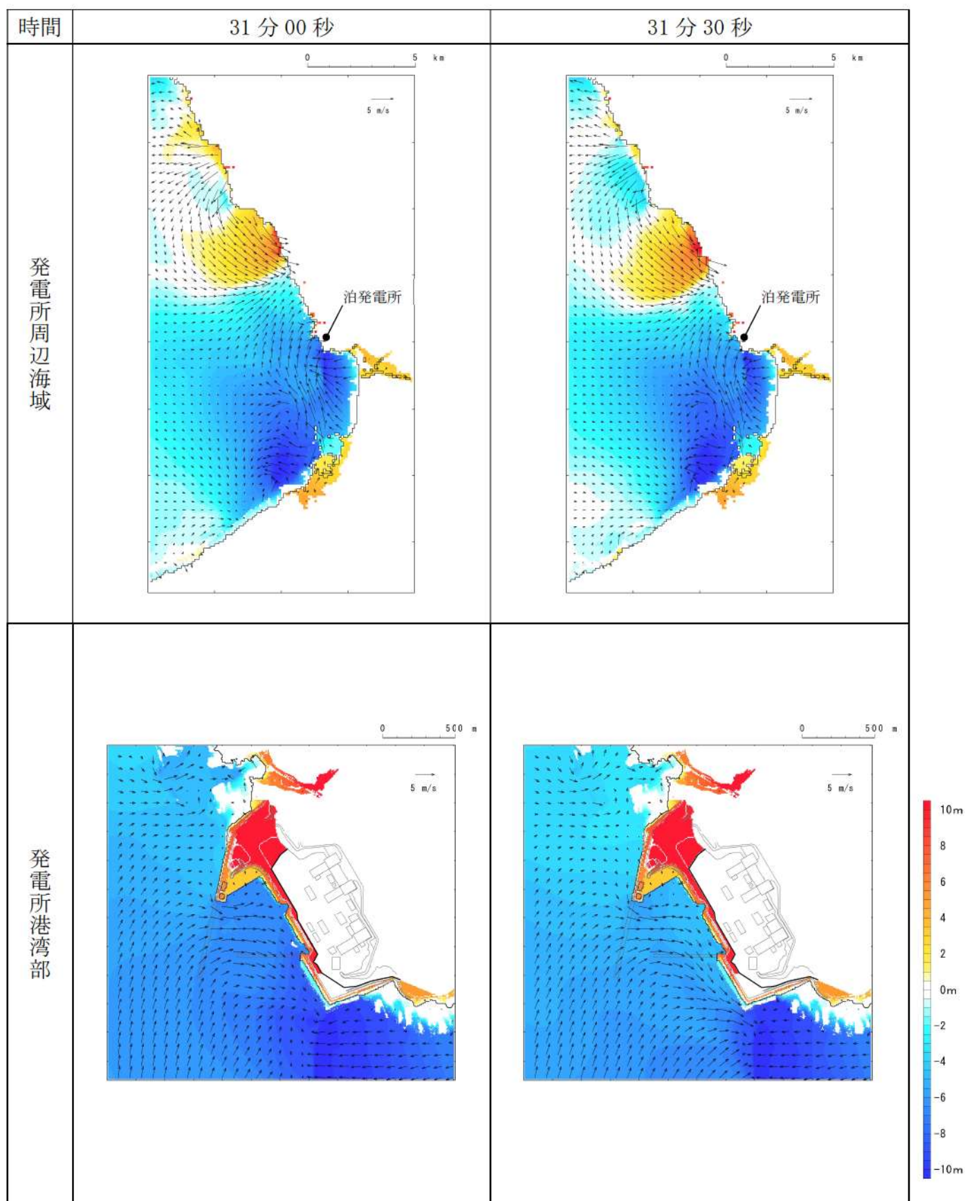
第 6 図-24 基準津波 D（北及び南防波堤損傷）の水位変動・流向ベクトル (24/53)
