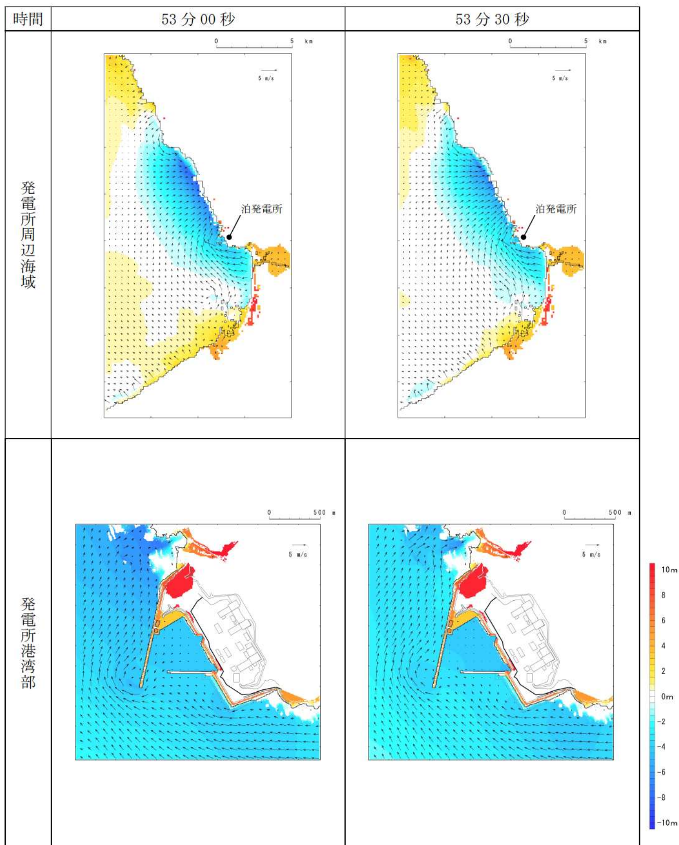
第 5 図-46 基準津波 D（防波堤損傷なし）の水位変動・流向ベクトル (46/53)
