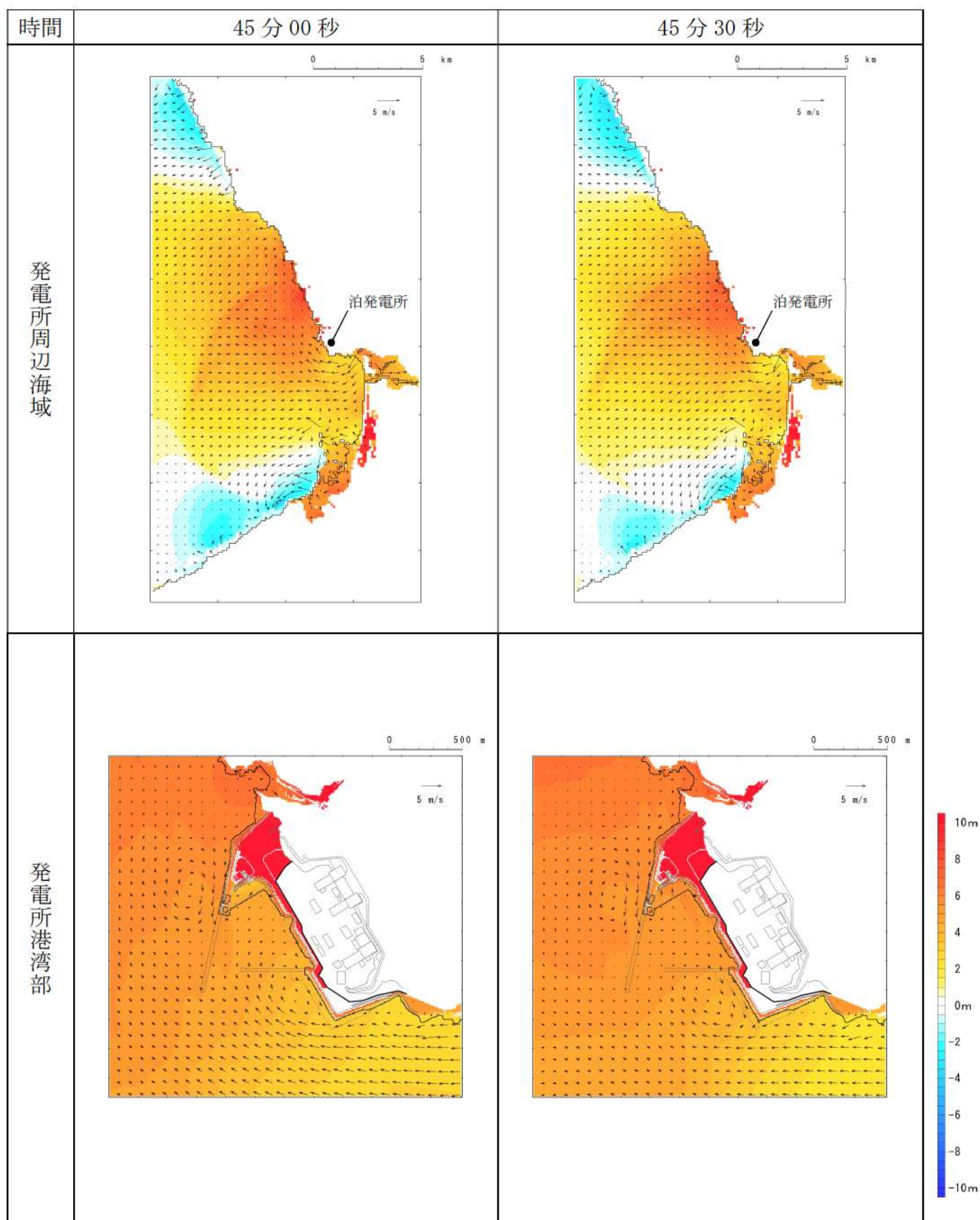
第 6 図-38 基準津波 D（北及び南防波堤損傷）の水位変動・流向ベクトル(38/53)
