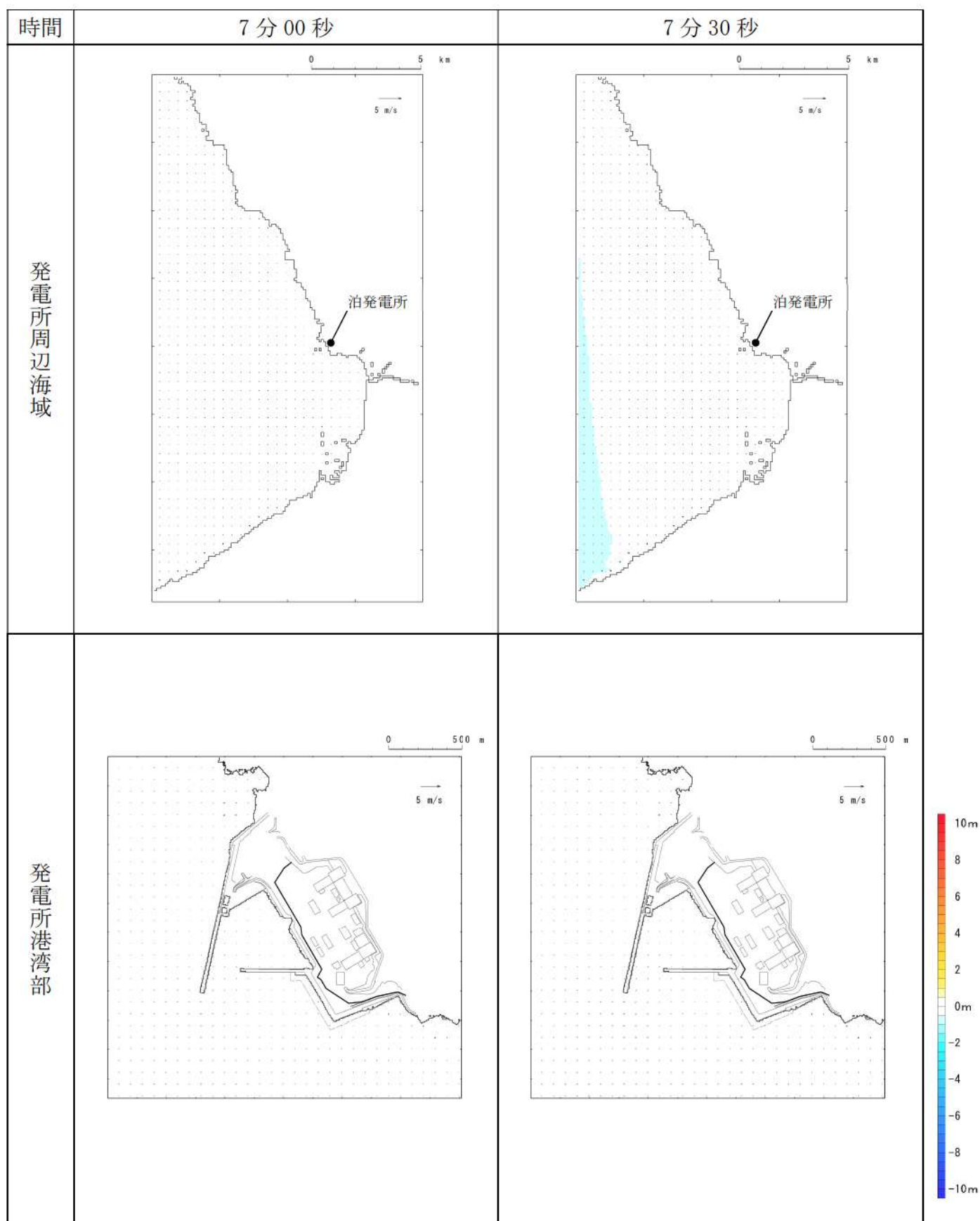
第 4 図- 1 基準津波 C（防波堤損傷なし）の水位変動・流向ベクトル (1/54)
