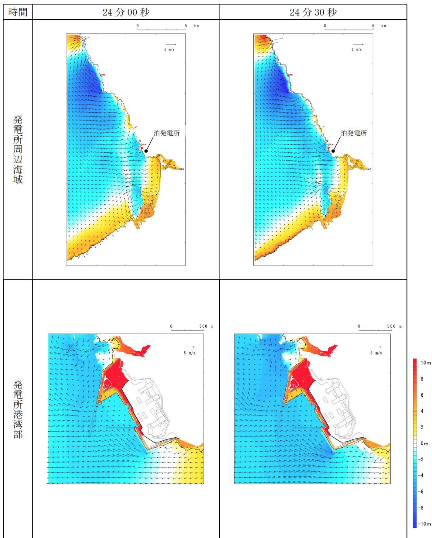
第 6 図-17 基準津波 D（北及び南防波堤損傷）の水位変動・流向ベクトル(17/53)
