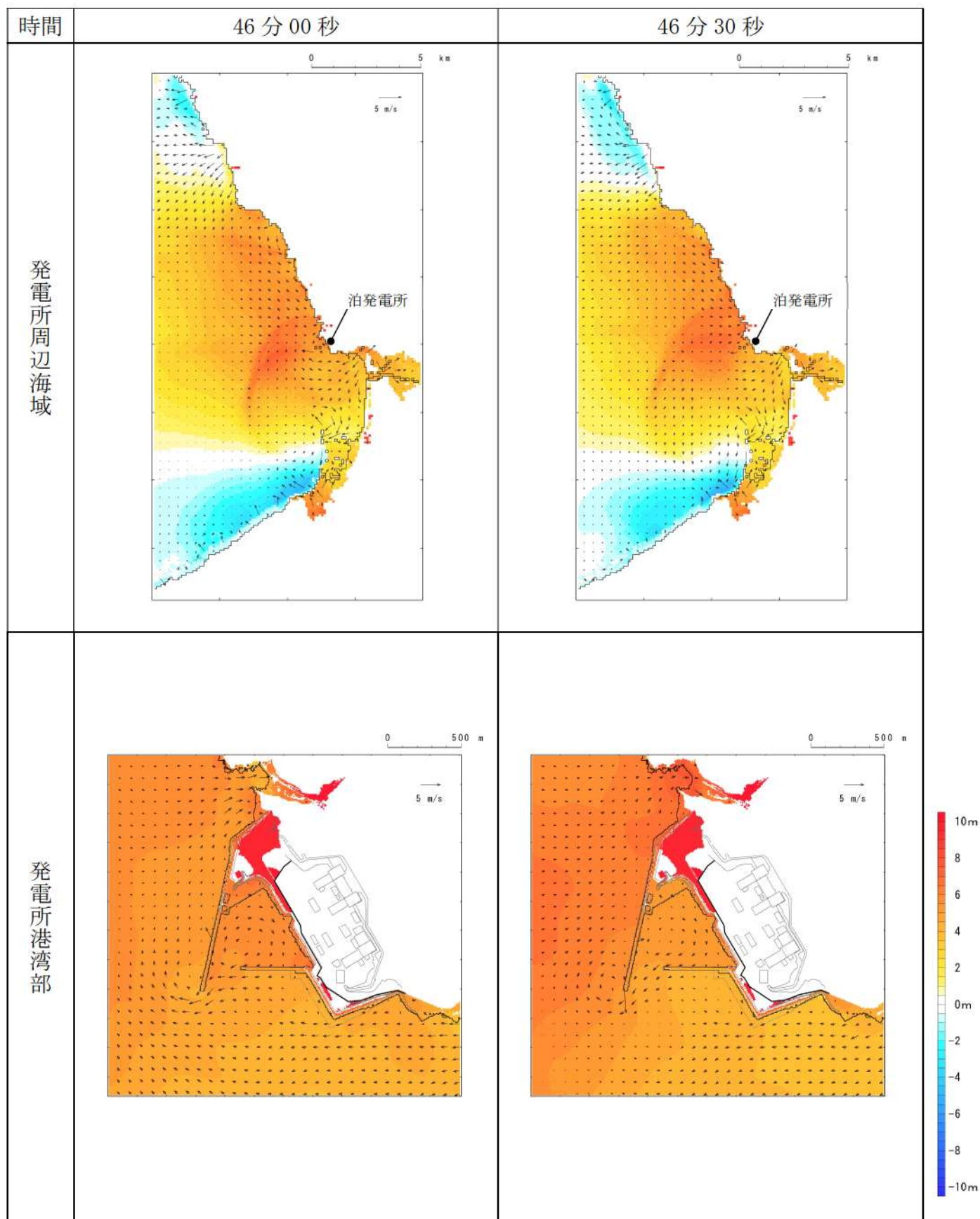
第4図-40 基準津波C（防波堤損傷なし）の水位変動・流向ベクトル(40/54)
