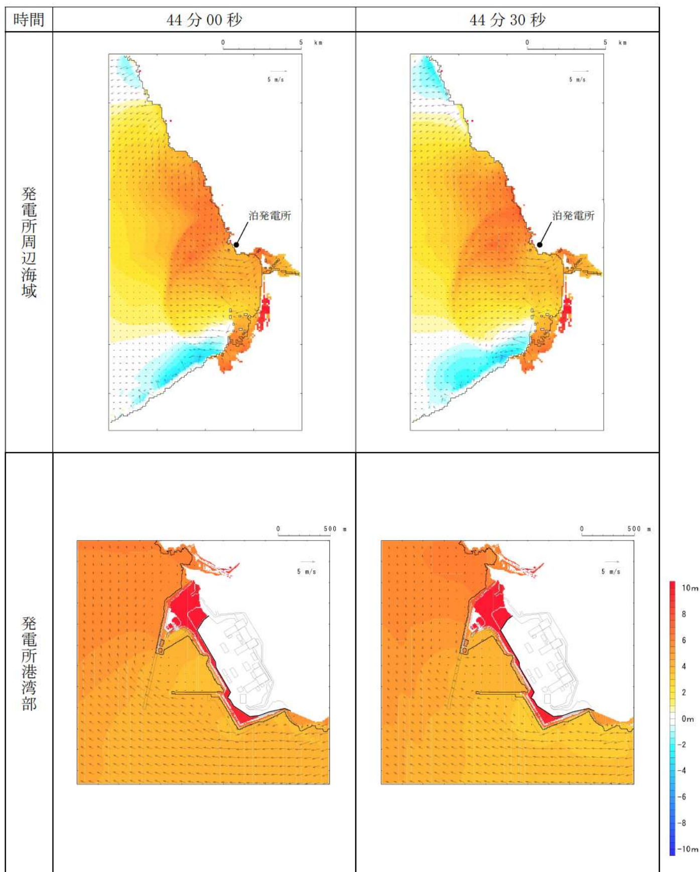
第3図-37 基準津波B（北防波堤損傷）の水位変動・流向ベクトル(37/53)
