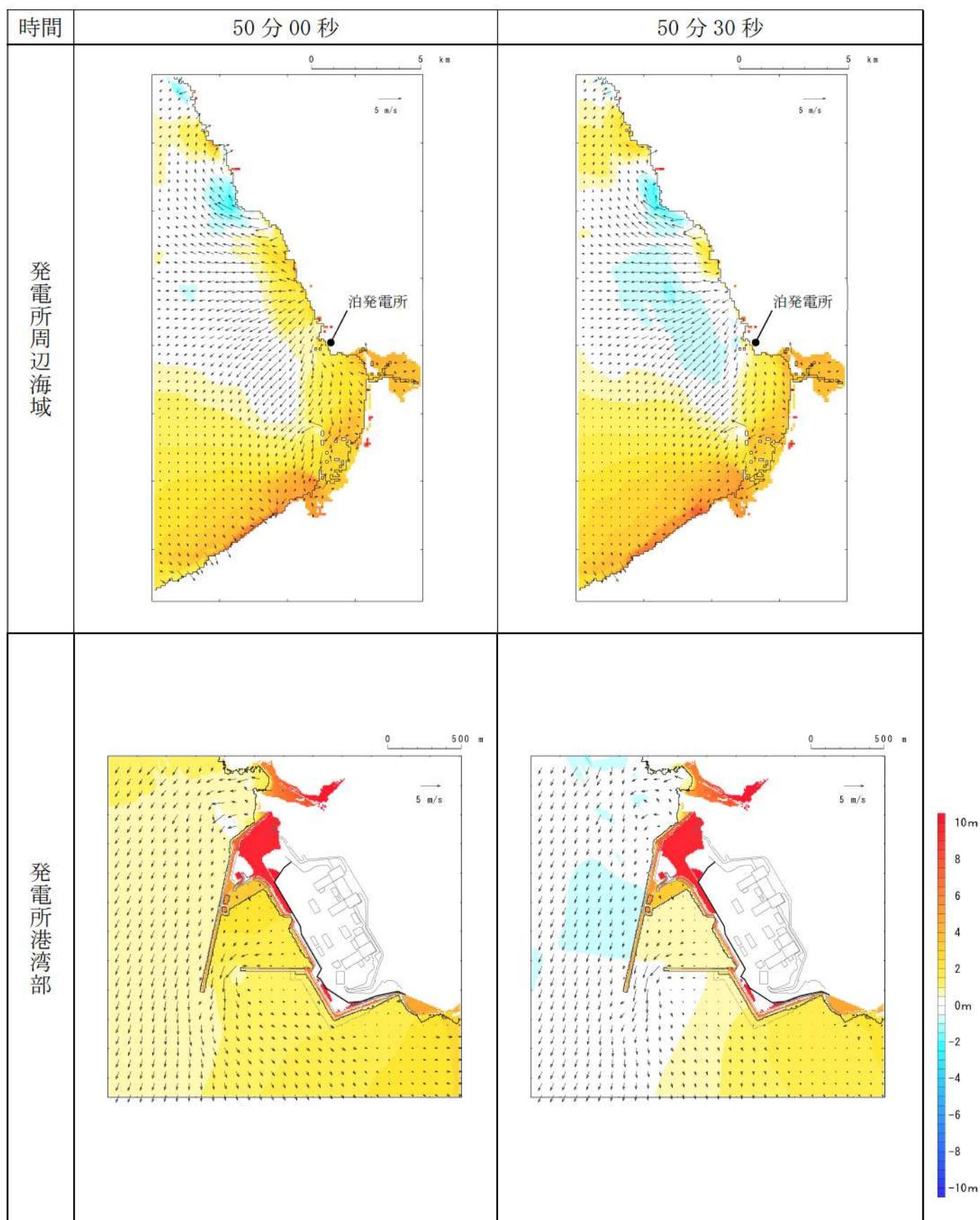
第4図-44 基準津波C（防波堤損傷なし）の水位変動・流向ベクトル(44/54)
