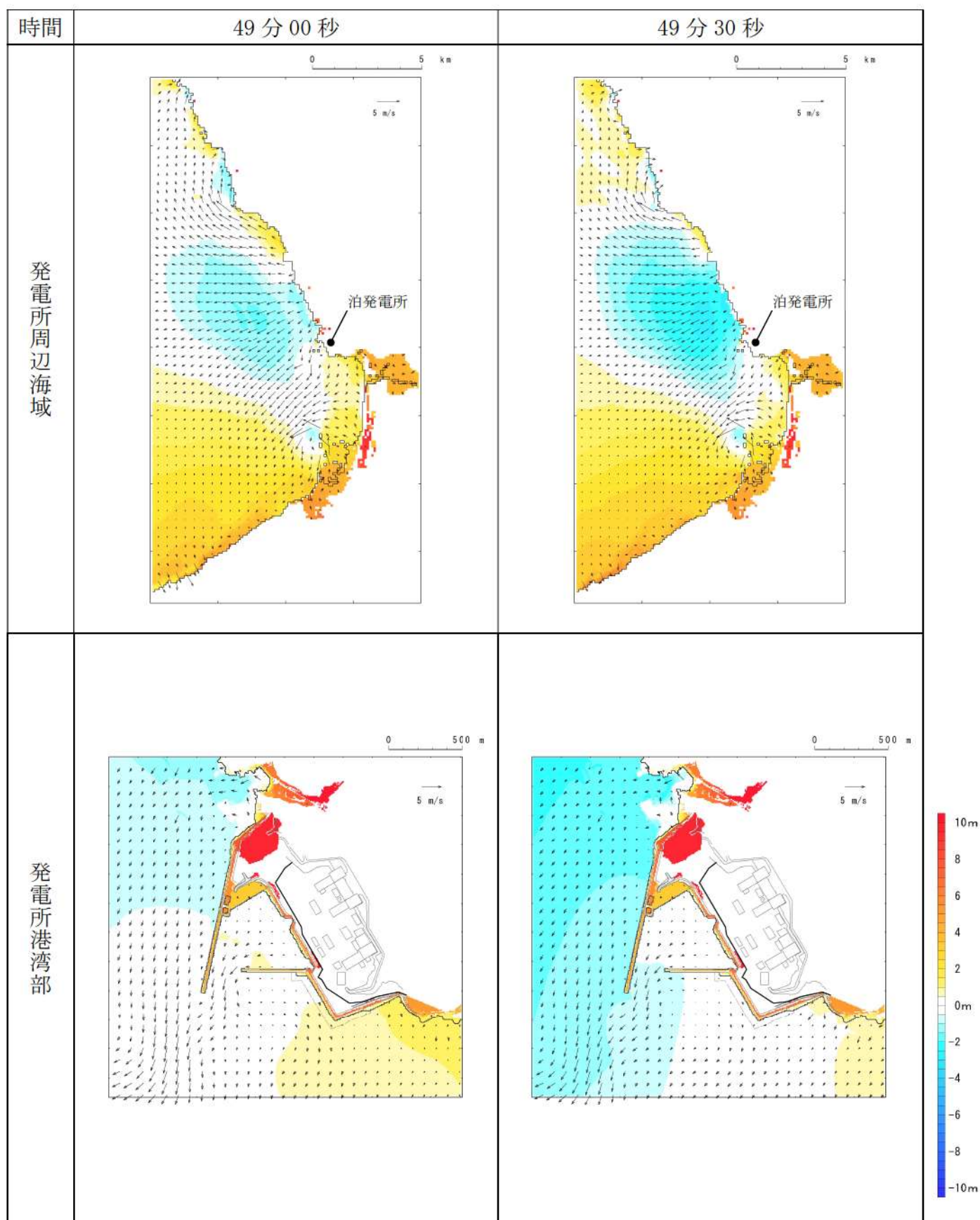
第 5 図-42 基準津波 D (防波堤損傷なし) の水位変動・流向ベクトル (42/53)
