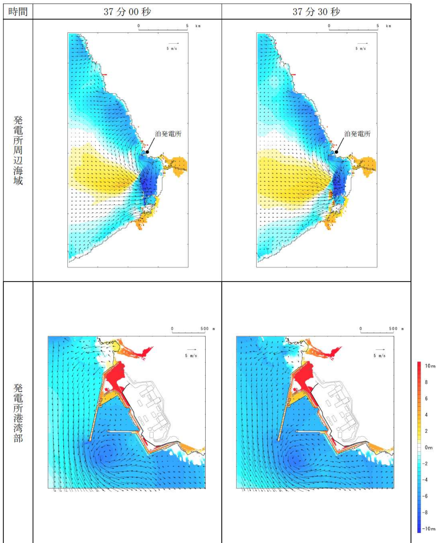
第4図-31 基準津波C（防波堤損傷なし）の水位変動・流向ベクトル(31/54)
