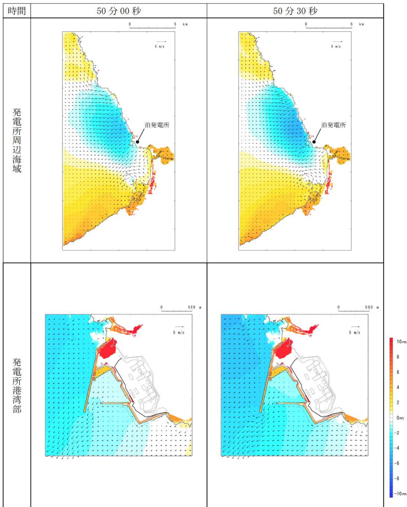
第 5 図-43 基準津波 D（防波堤損傷なし）の水位変動・流向ベクトル (43/53)
