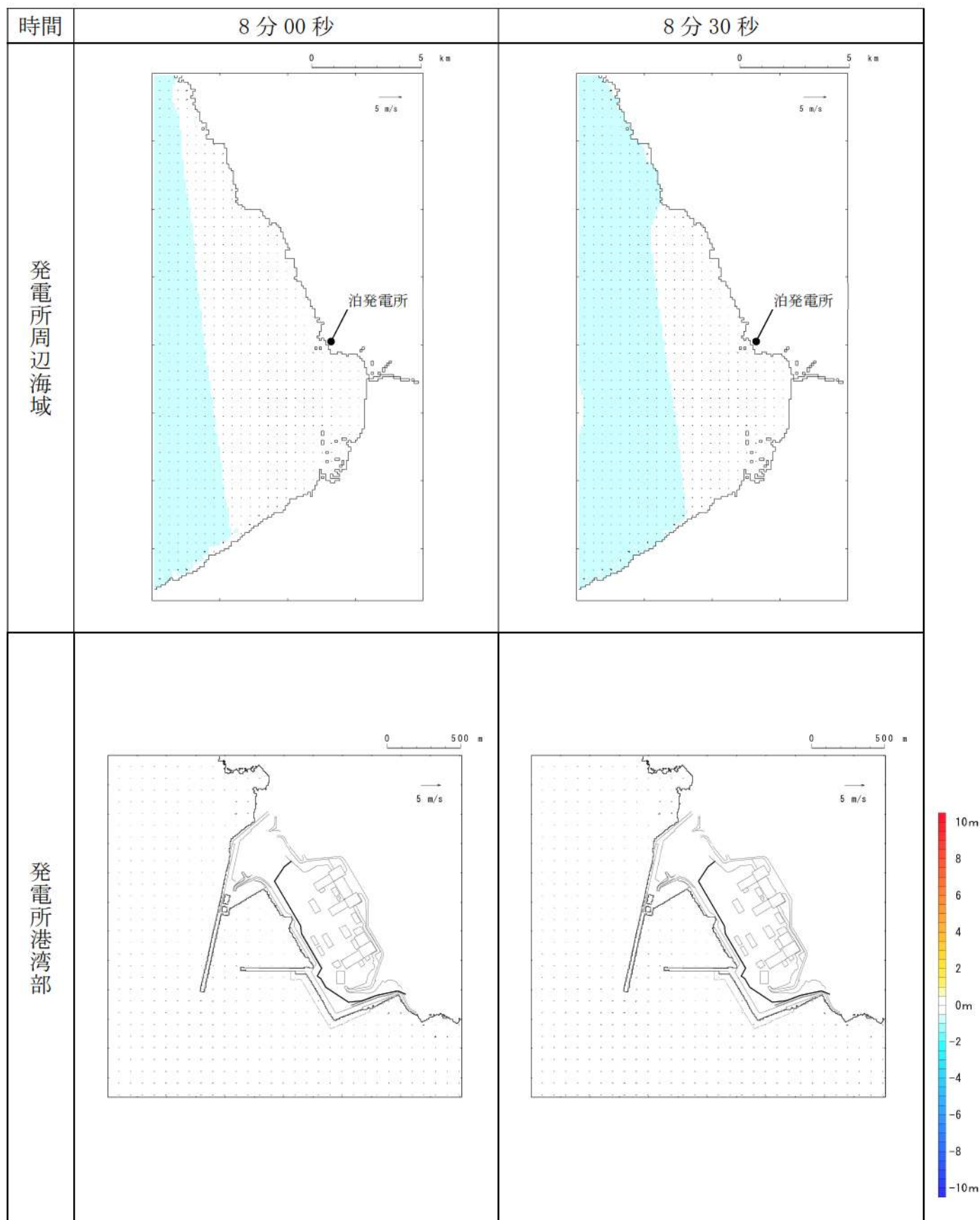
第 4 図- 2 基準津波 C（防波堤損傷なし）の水位変動・流向ベクトル (2/54)
