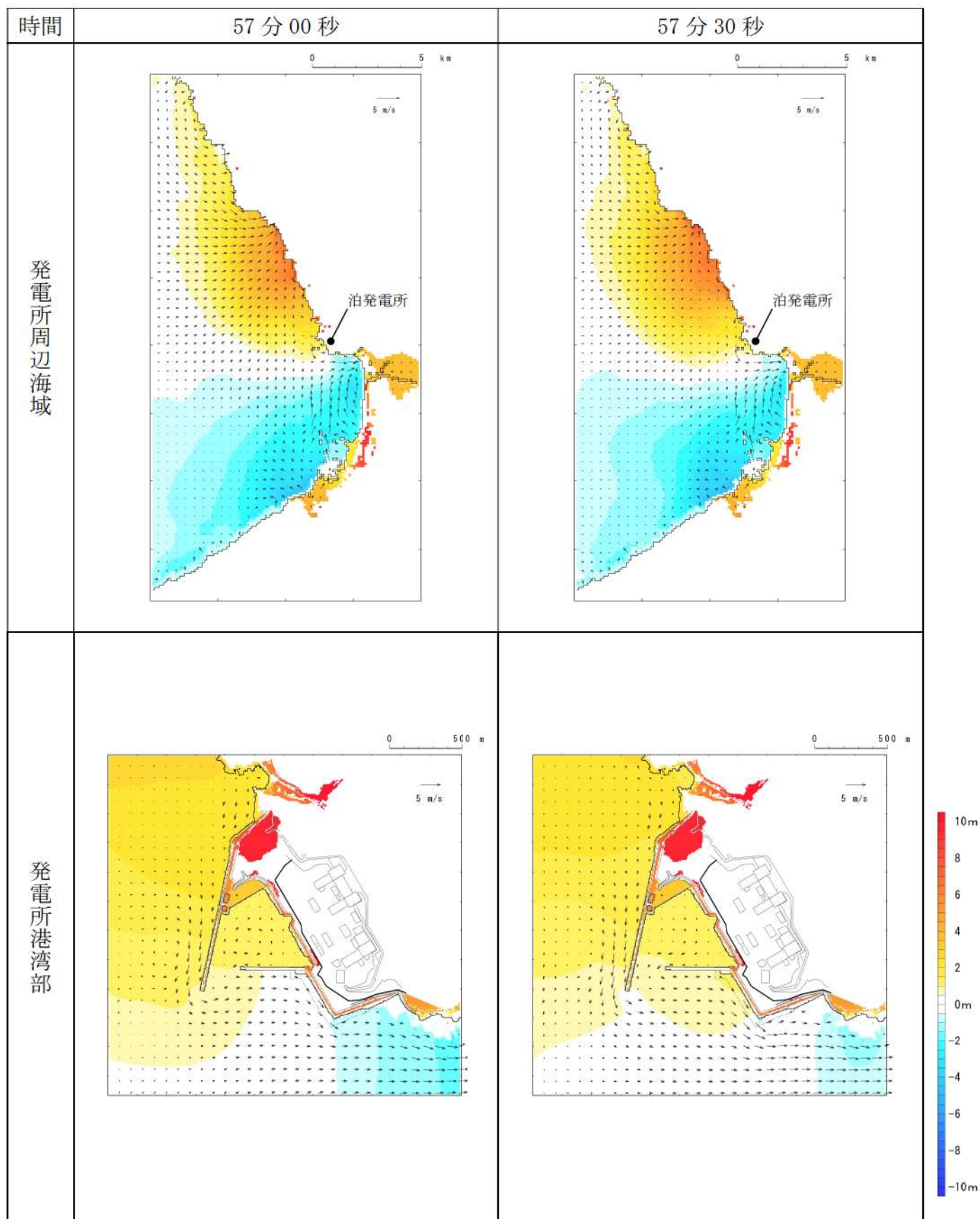
第 5 図-50 基準津波 D (防波堤損傷なし) の水位変動・流向ベクトル (50/53)
