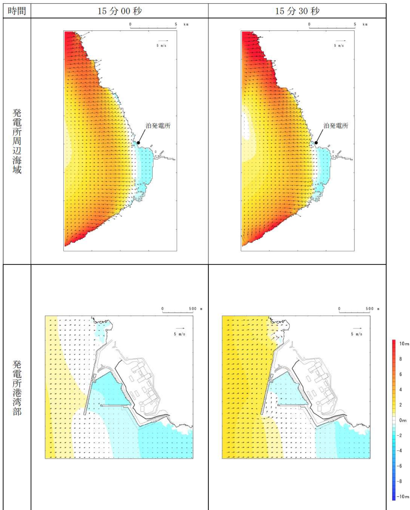
第4図-9 基準津波C（防波堤損傷なし）の水位変動・流向ベクトル(9/54)
