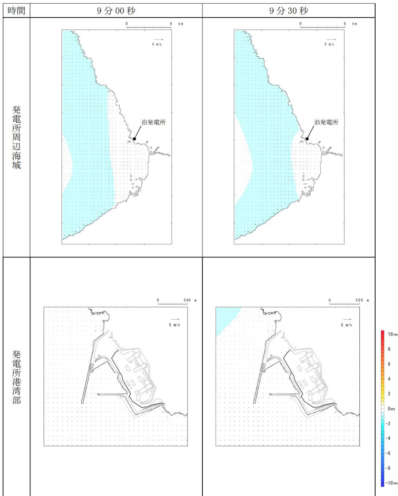
第 4 図- 3 基準津波 C (防波堤損傷なし) の水位変動・流向ベクトル (3/54)
