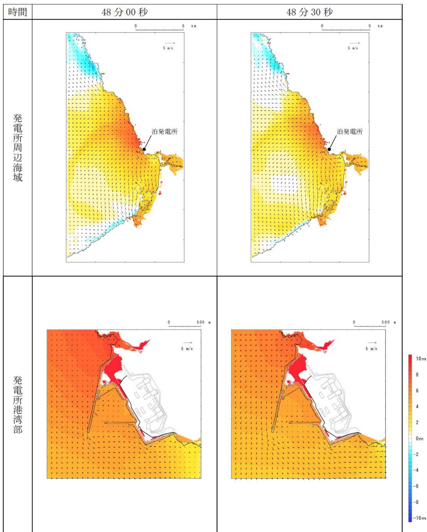
第4図-42 基準津波C（防波堤損傷なし）の水位変動・流向ベクトル(42/54)
