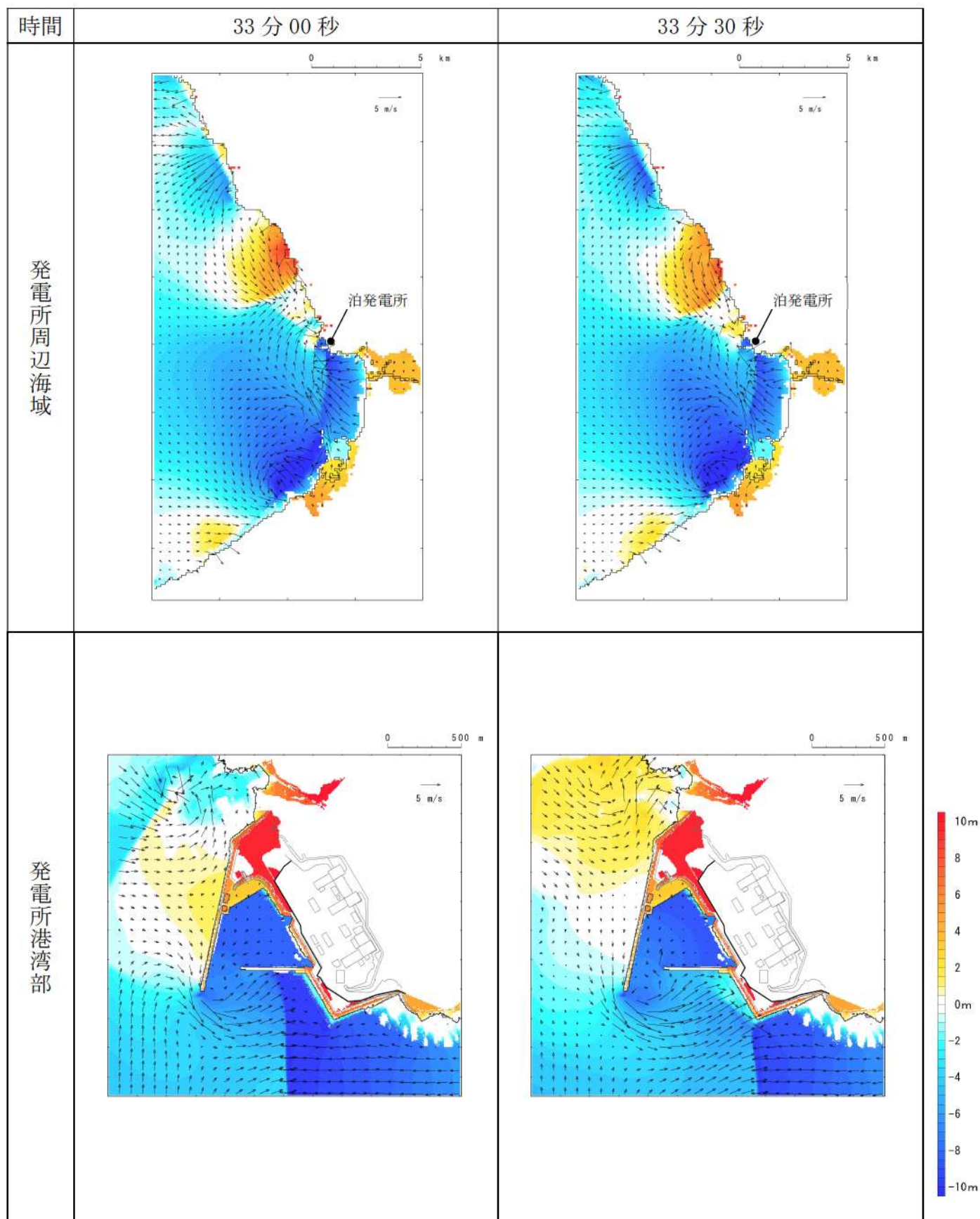
第4図-27 基準津波C（防波堤損傷なし）の水位変動・流向ベクトル(27/54)
