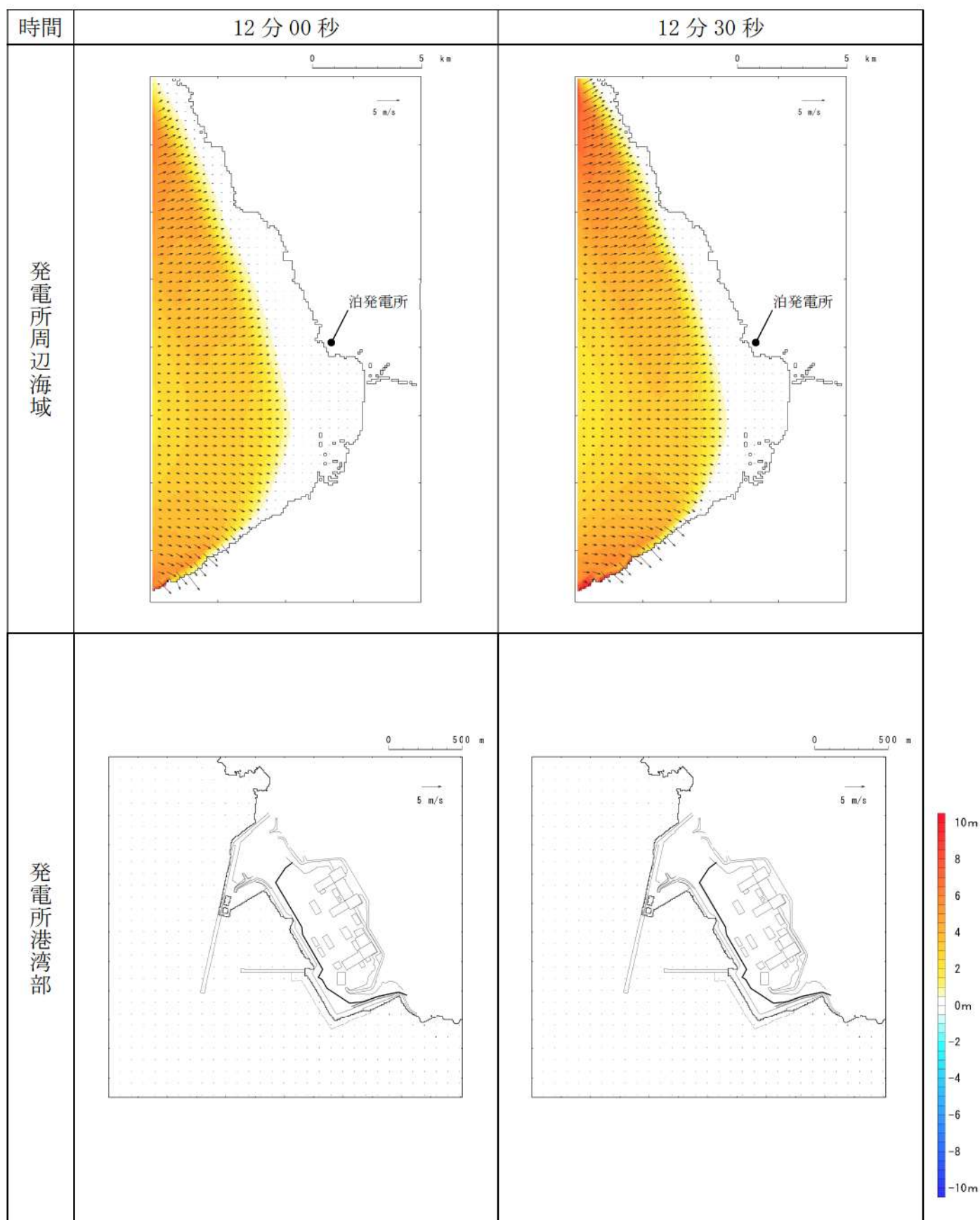
第 6 図- 5 基準津波 D（北及び南防波堤損傷）の水位変動・流向ベクトル (5/53)
