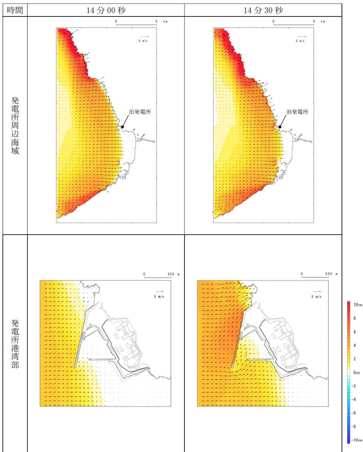
第5図-7 基準津波D（防波堤損傷なし）の水位変動・流向ベクトル(7/53)
