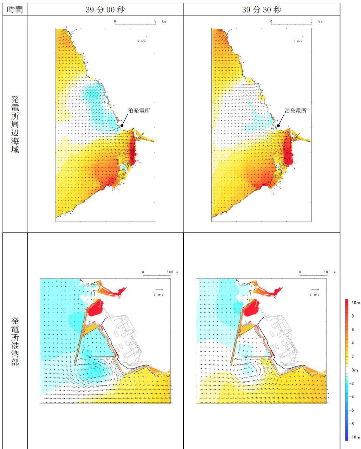
第 5 図-32 基準津波 D (防波堤損傷なし) の水位変動・流向ベクトル (32/53)
