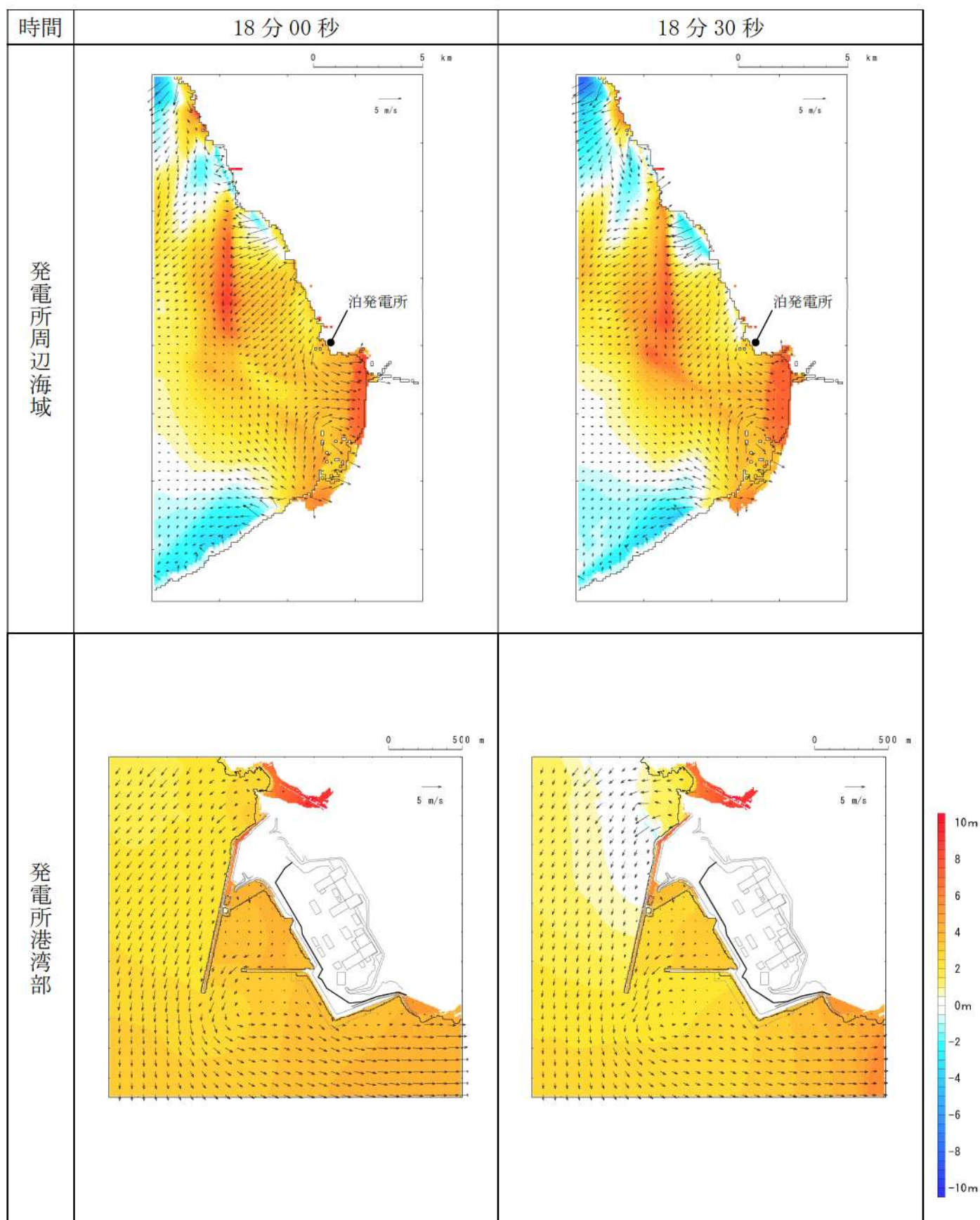
第 5 図-11 基準津波 D (防波堤損傷なし) の水位変動・流向ベクトル(11/53)
