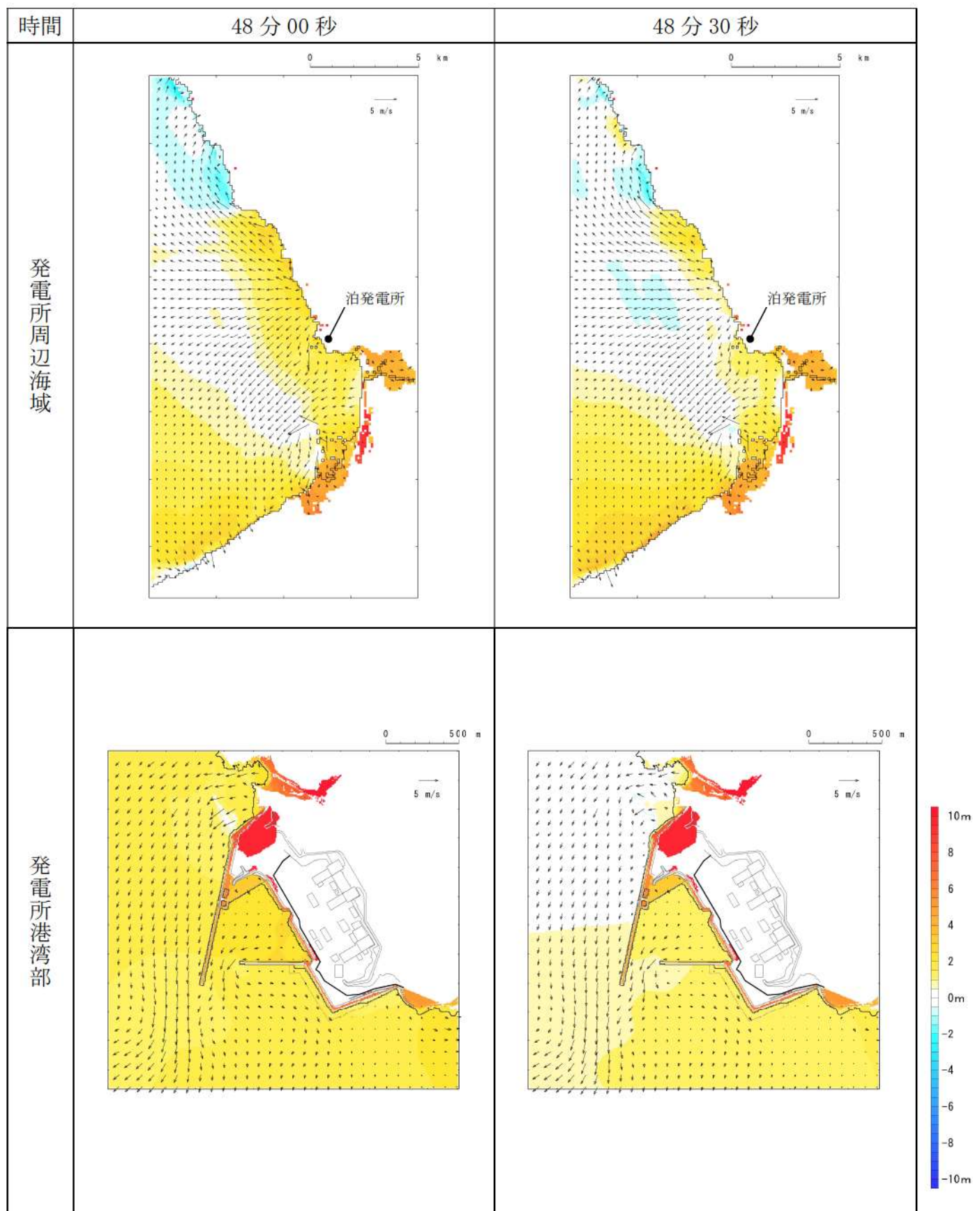
第 5 図-41 基準津波 D（防波堤損傷なし）の水位変動・流向ベクトル (41/53)
