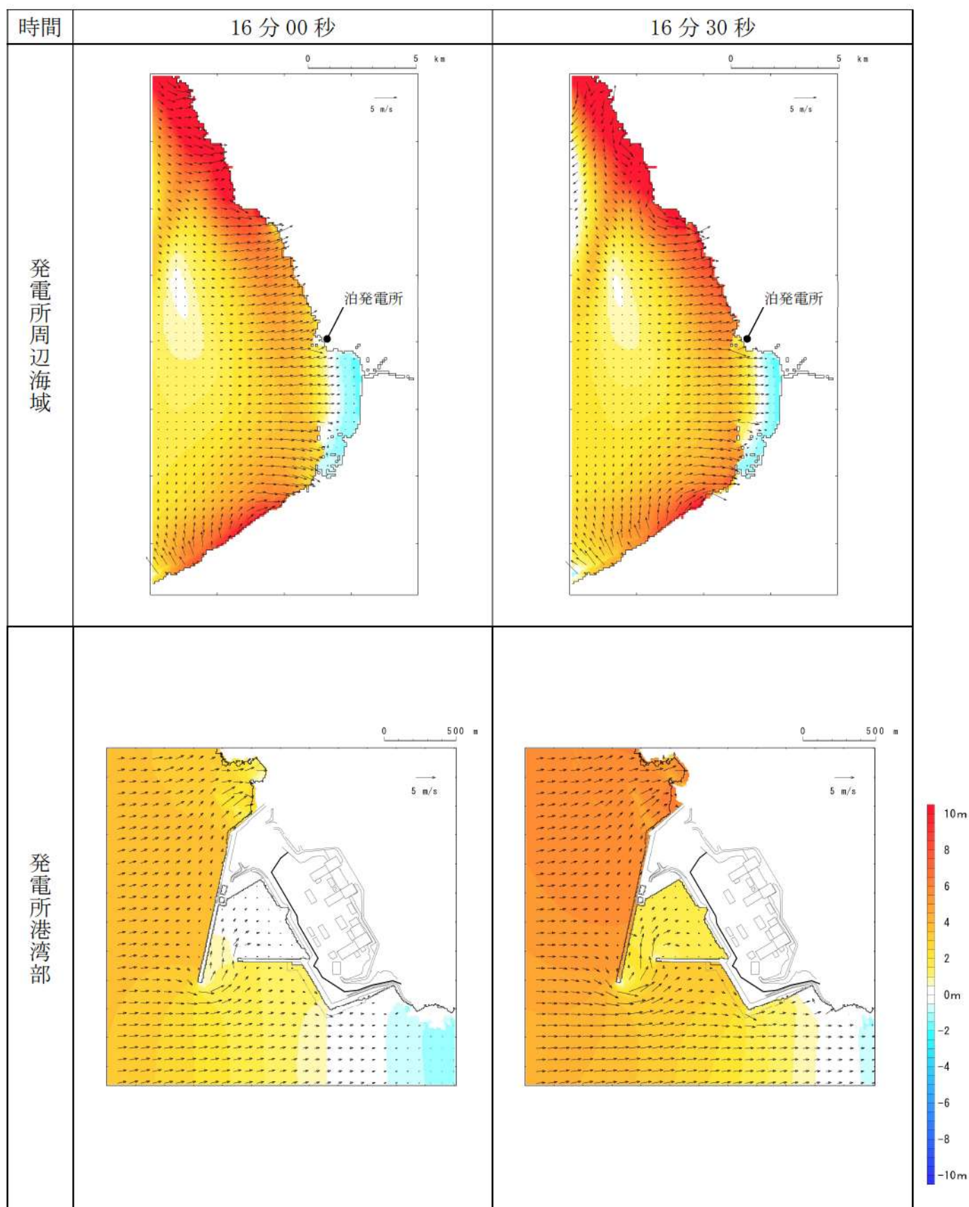
第4図-10 基準津波C（防波堤損傷なし）の水位変動・流向ベクトル(10/54)
