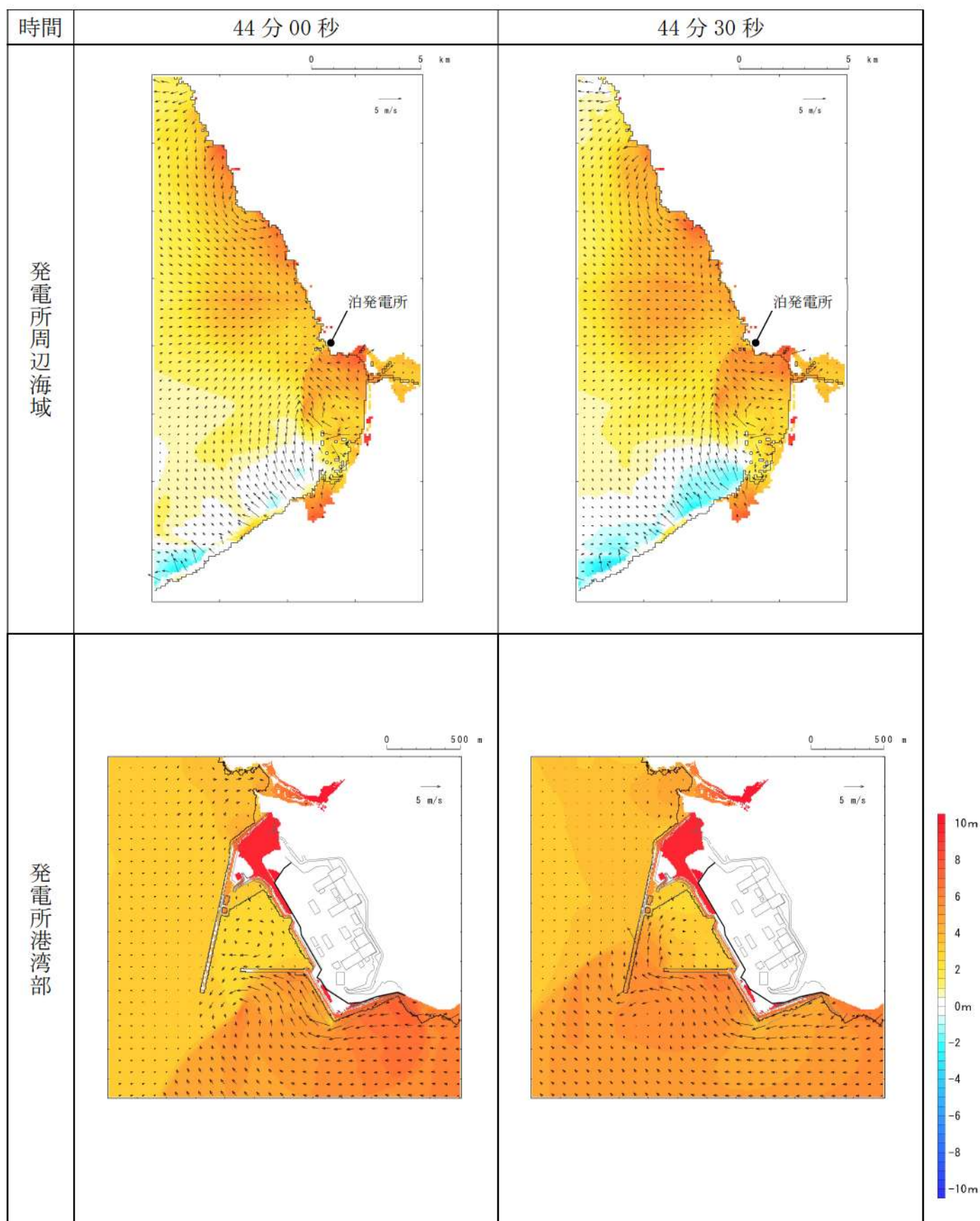
第 4 図-38 基準津波 C（防波堤損傷なし）の水位変動・流向ベクトル (38/54)
