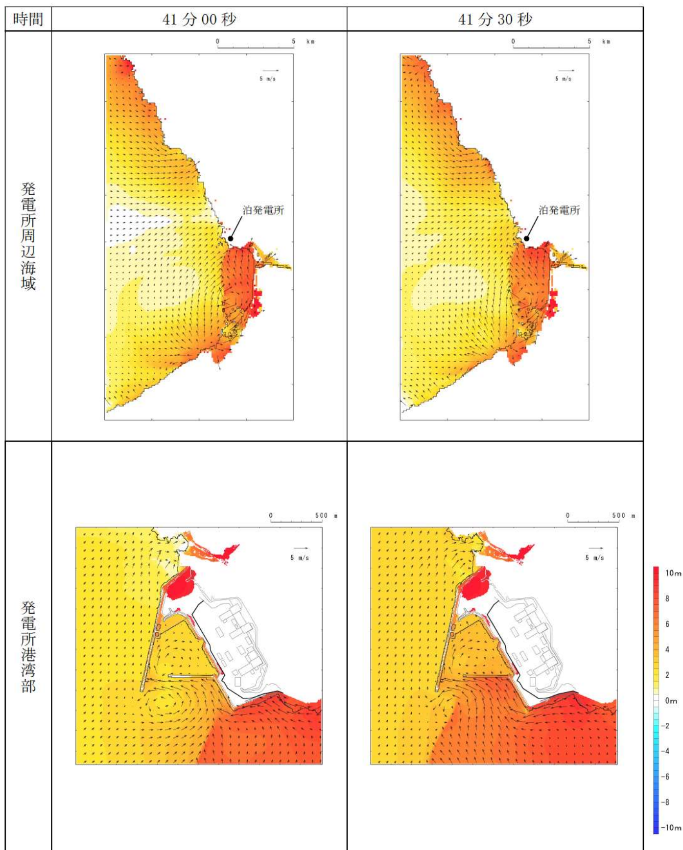
第 5 図-34 基準津波 D（防波堤損傷なし）の水位変動・流向ベクトル (34/53)
