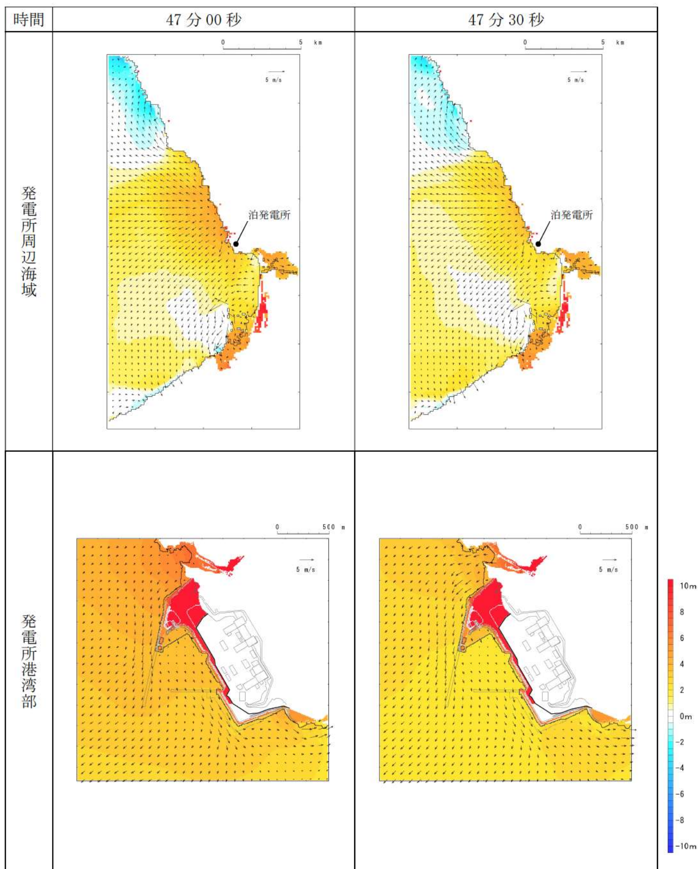
第 6 図-40 基準津波 D（北及び南防波堤損傷）の水位変動・流向ベクトル(40/53)
