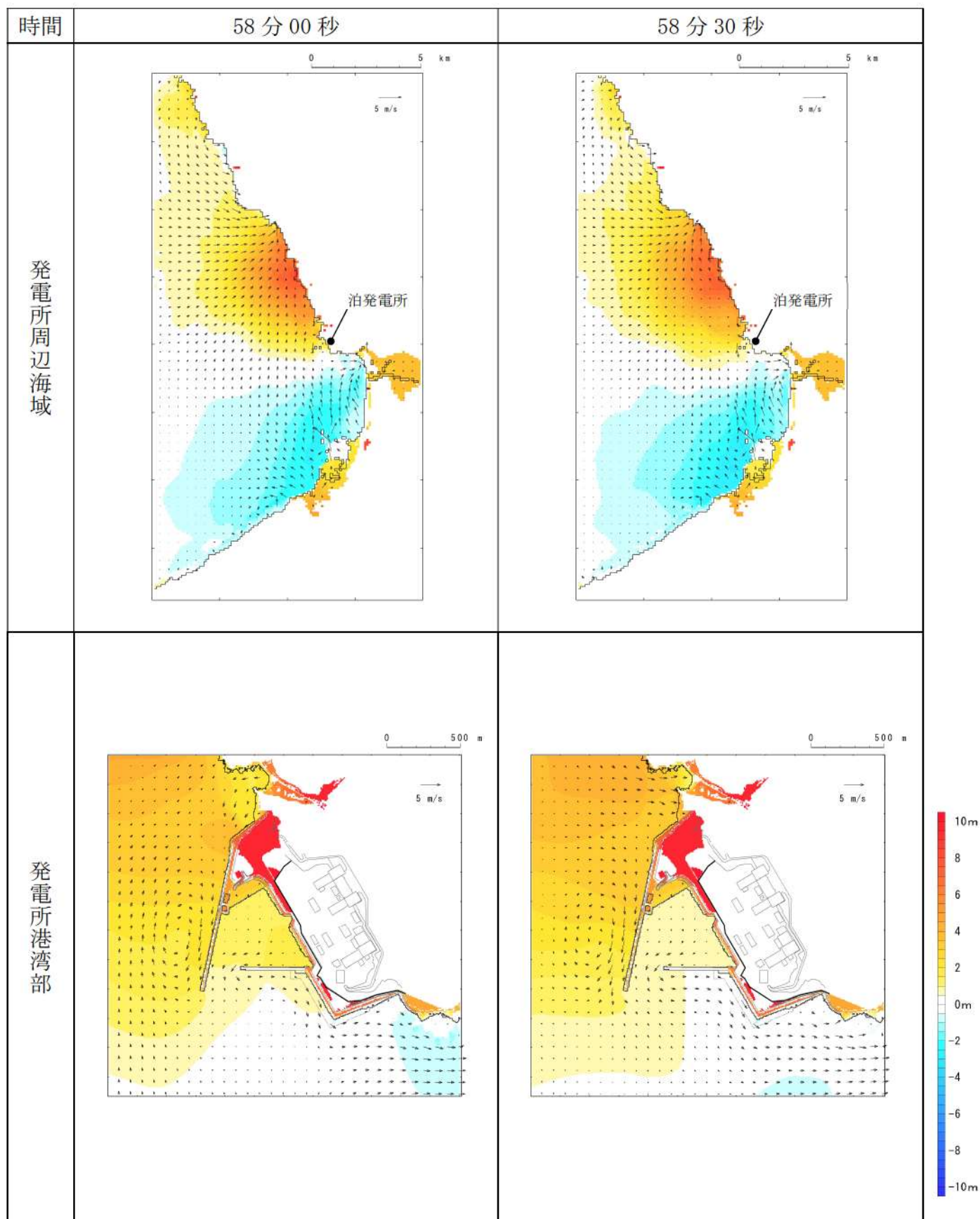
第4図-52 基準津波C（防波堤損傷なし）の水位変動・流向ベクトル(52/54)
