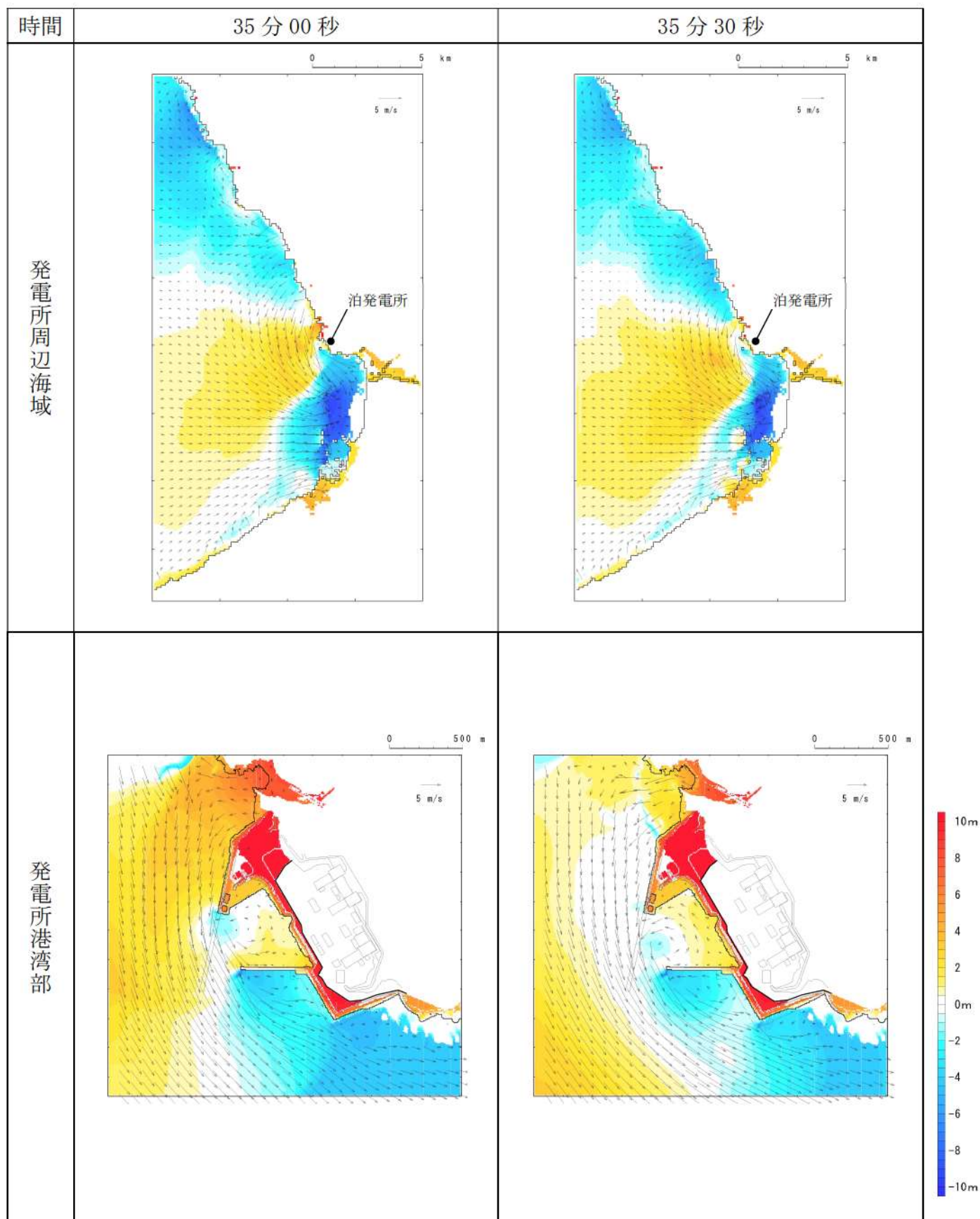
第3図-28 基準津波B（北防波堤損傷）の水位変動・流向ベクトル(28/53)
