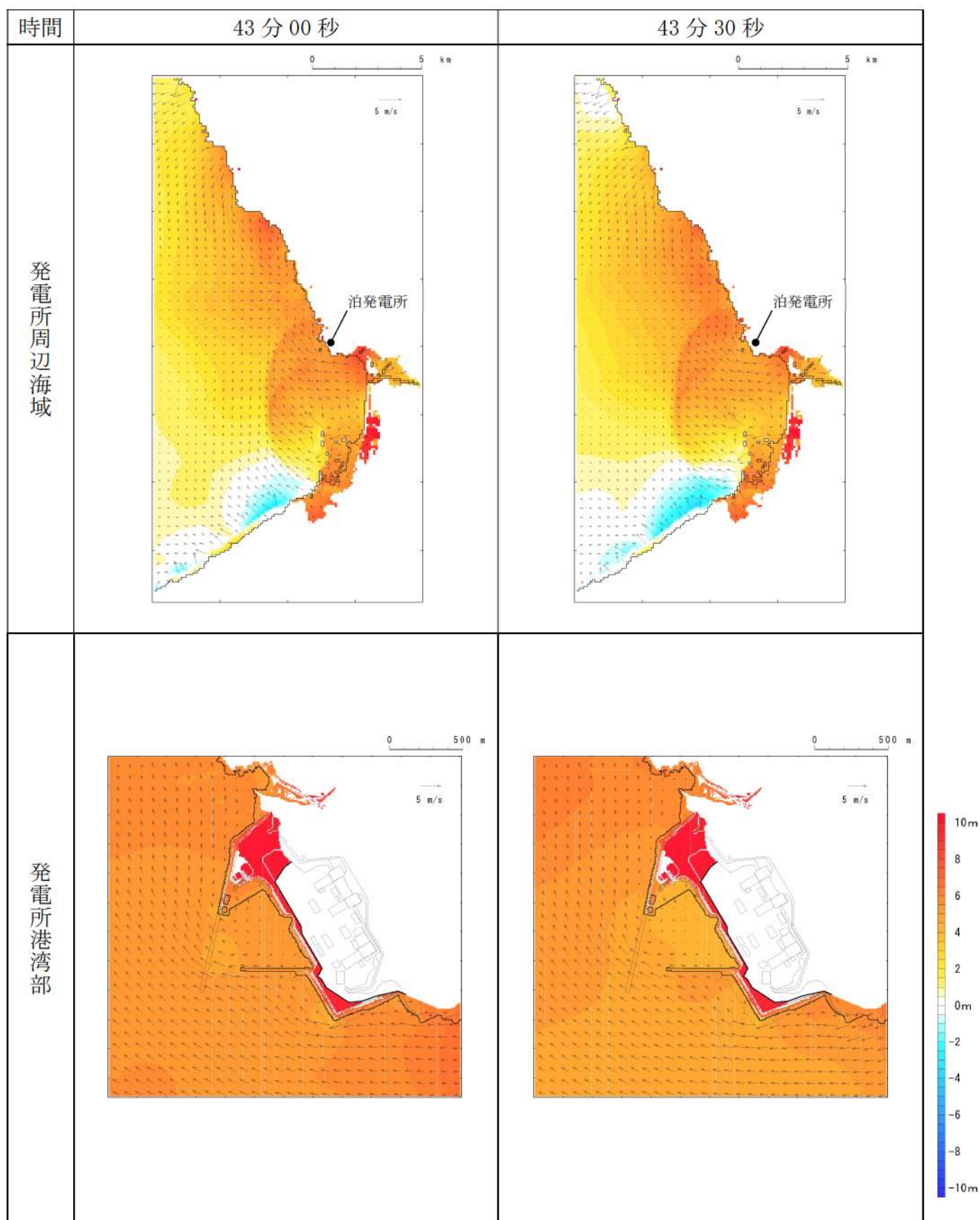
第3図-36 基準津波B（北防波堤損傷）の水位変動・流向ベクトル(36/53)
