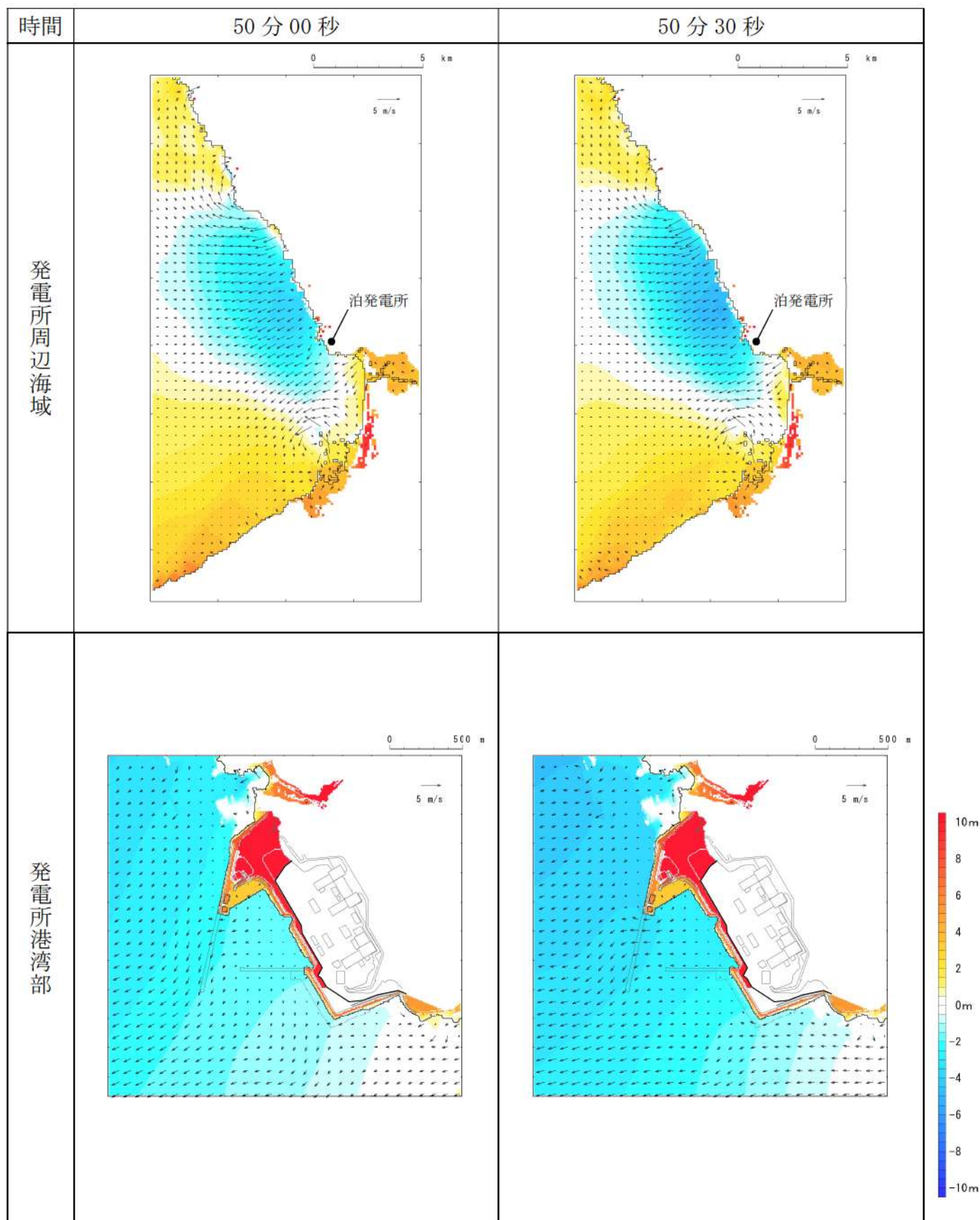
第 6 図-43 基準津波 D（北及び南防波堤損傷）の水位変動・流向ベクトル(43/53)
