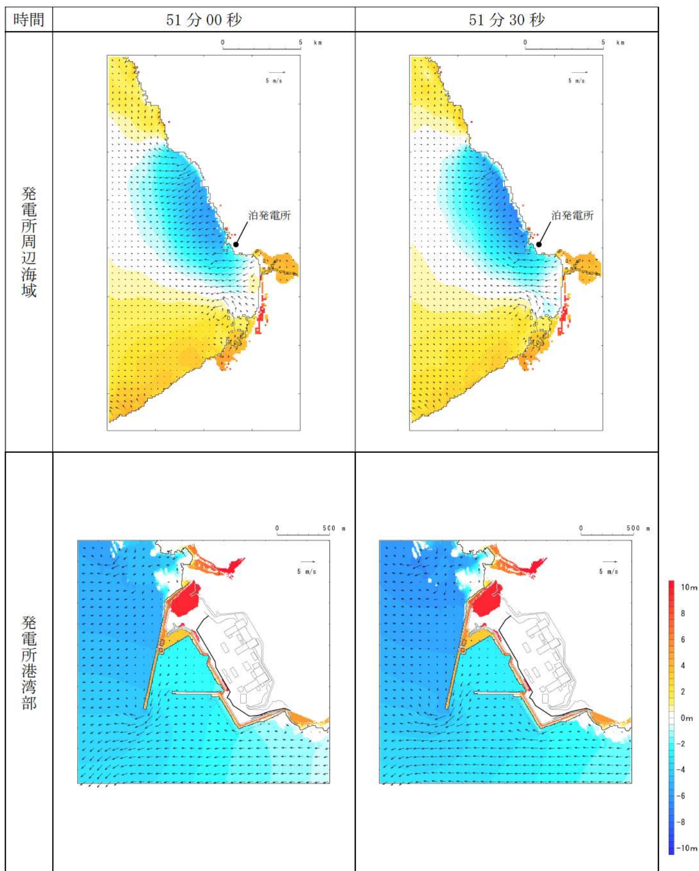
第 5 図-44 基準津波 D（防波堤損傷なし）の水位変動・流向ベクトル(44/53)
