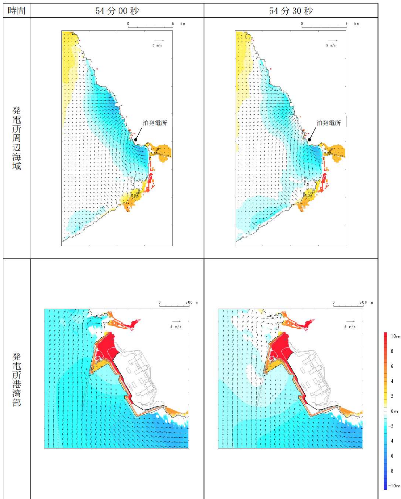
第 6 図-47 基準津波 D（北及び南防波堤損傷）の水位変動・流向ベクトル(47/53)
