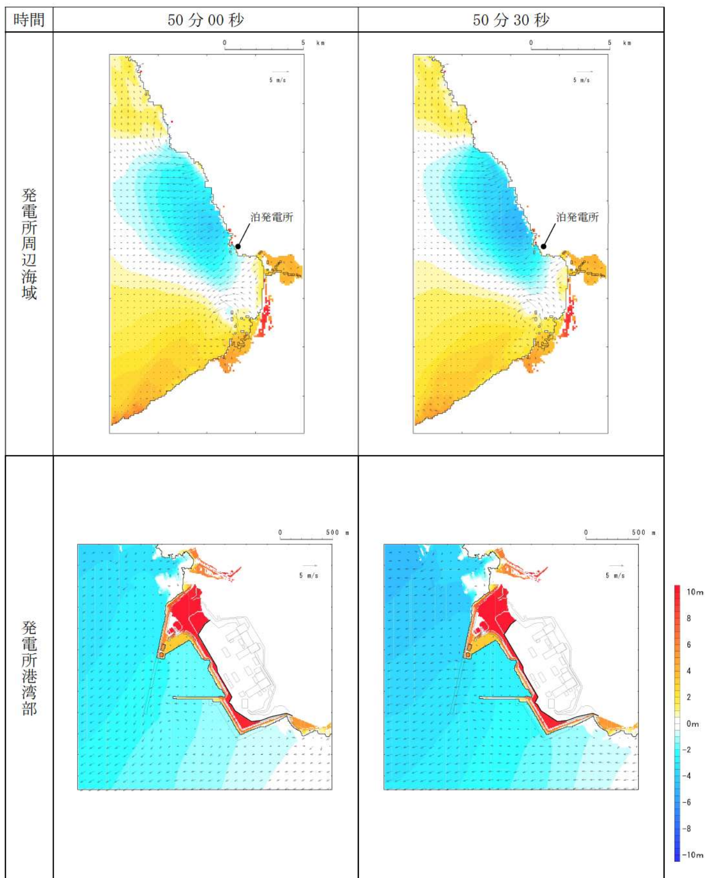
第3図-43 基準津波B（北防波堤損傷）の水位変動・流向ベクトル(43/53)
