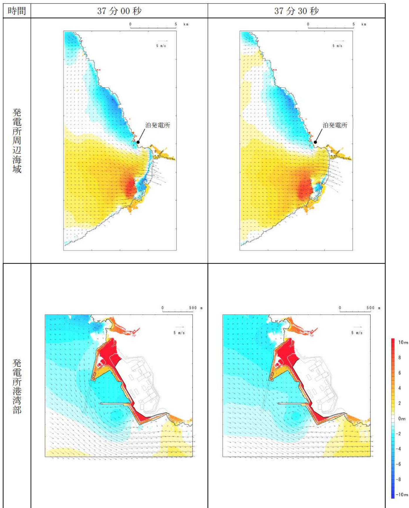
第3図-30 基準津波B（北防波堤損傷）の水位変動・流向ベクトル(30/53)
