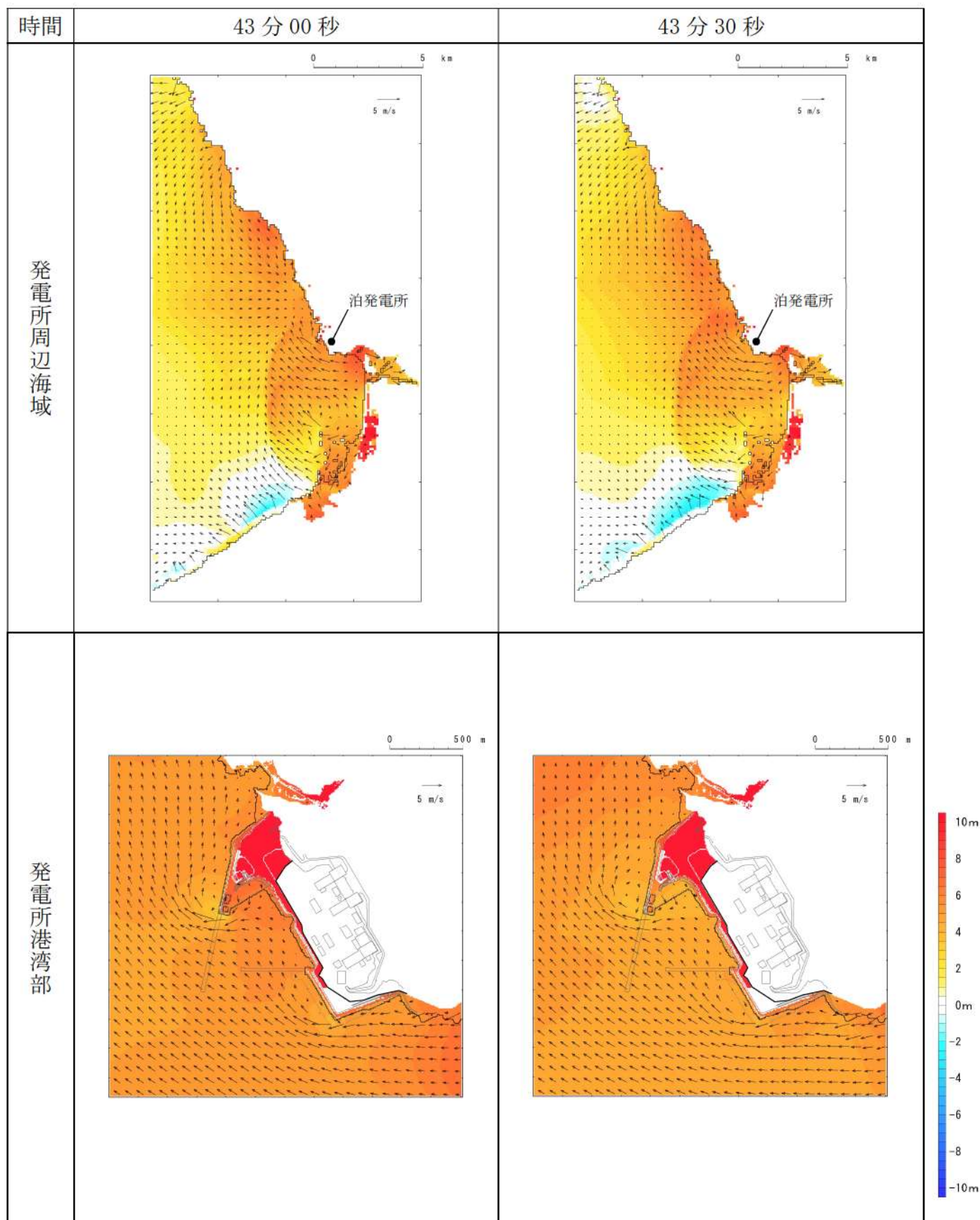
第 6 図-36 基準津波 D（北及び南防波堤損傷）の水位変動・流向ベクトル(36/53)
