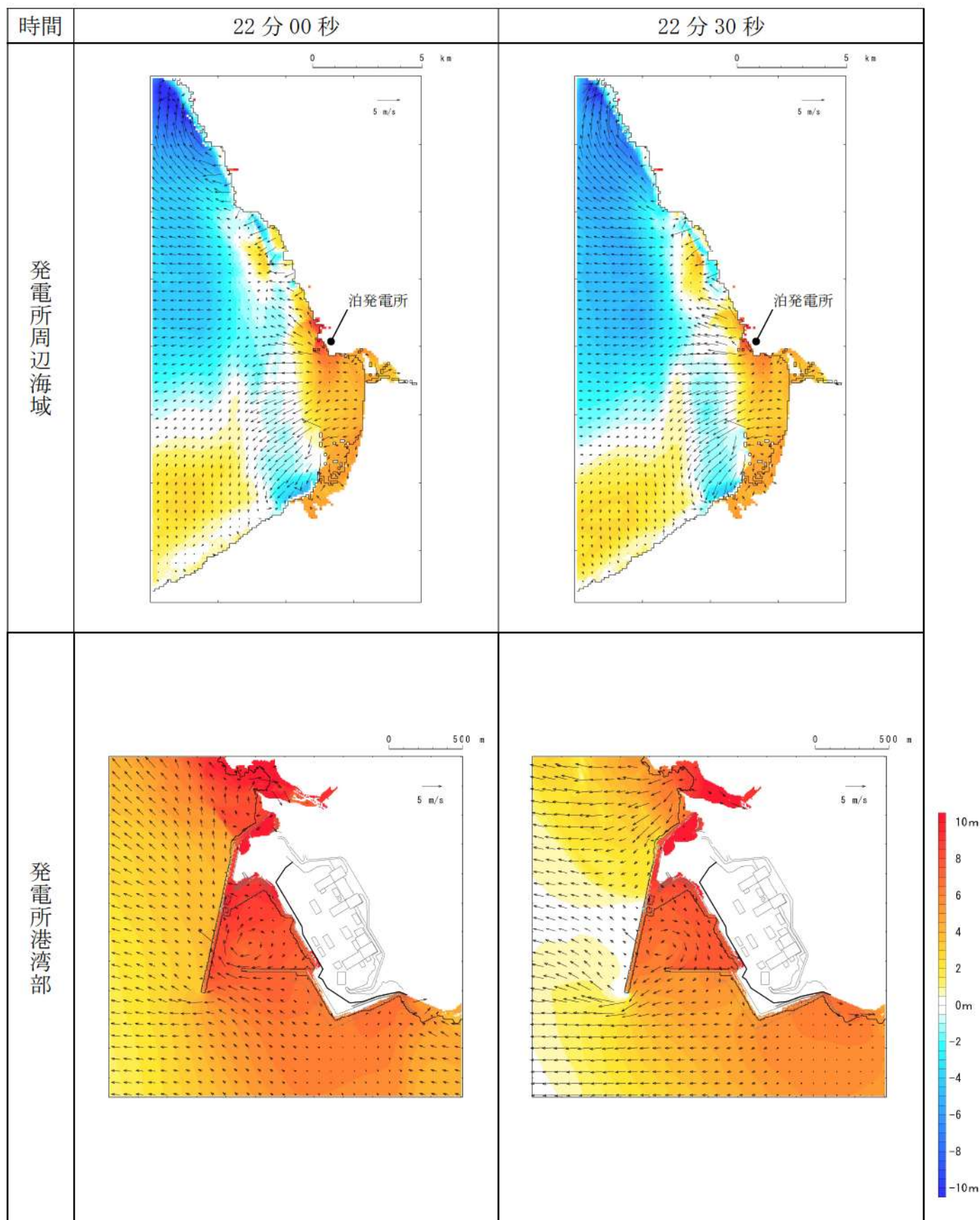
第 5 図-15 基準津波 D（防波堤損傷なし）の水位変動・流向ベクトル(15/53)
