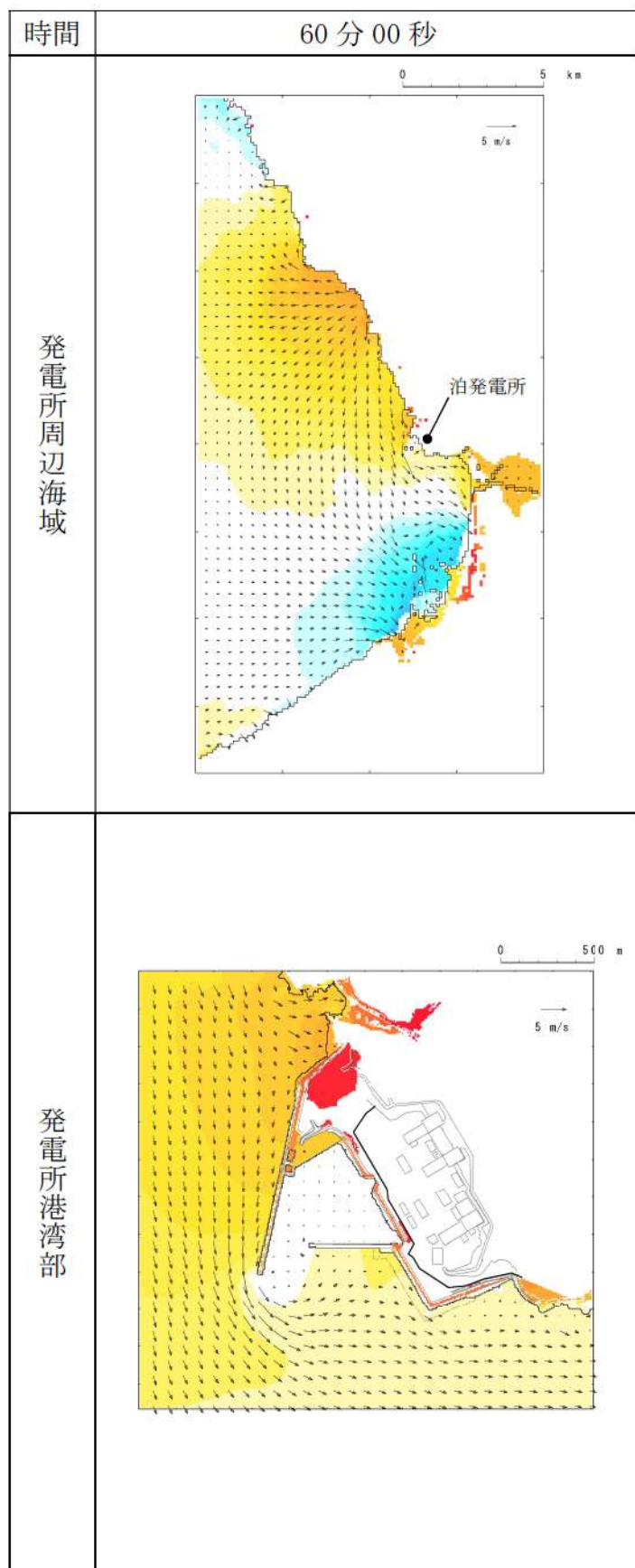
第 5 図-53 基準津波 D（防波堤損傷なし）の水位変動・流向ベクトル (53/53)
