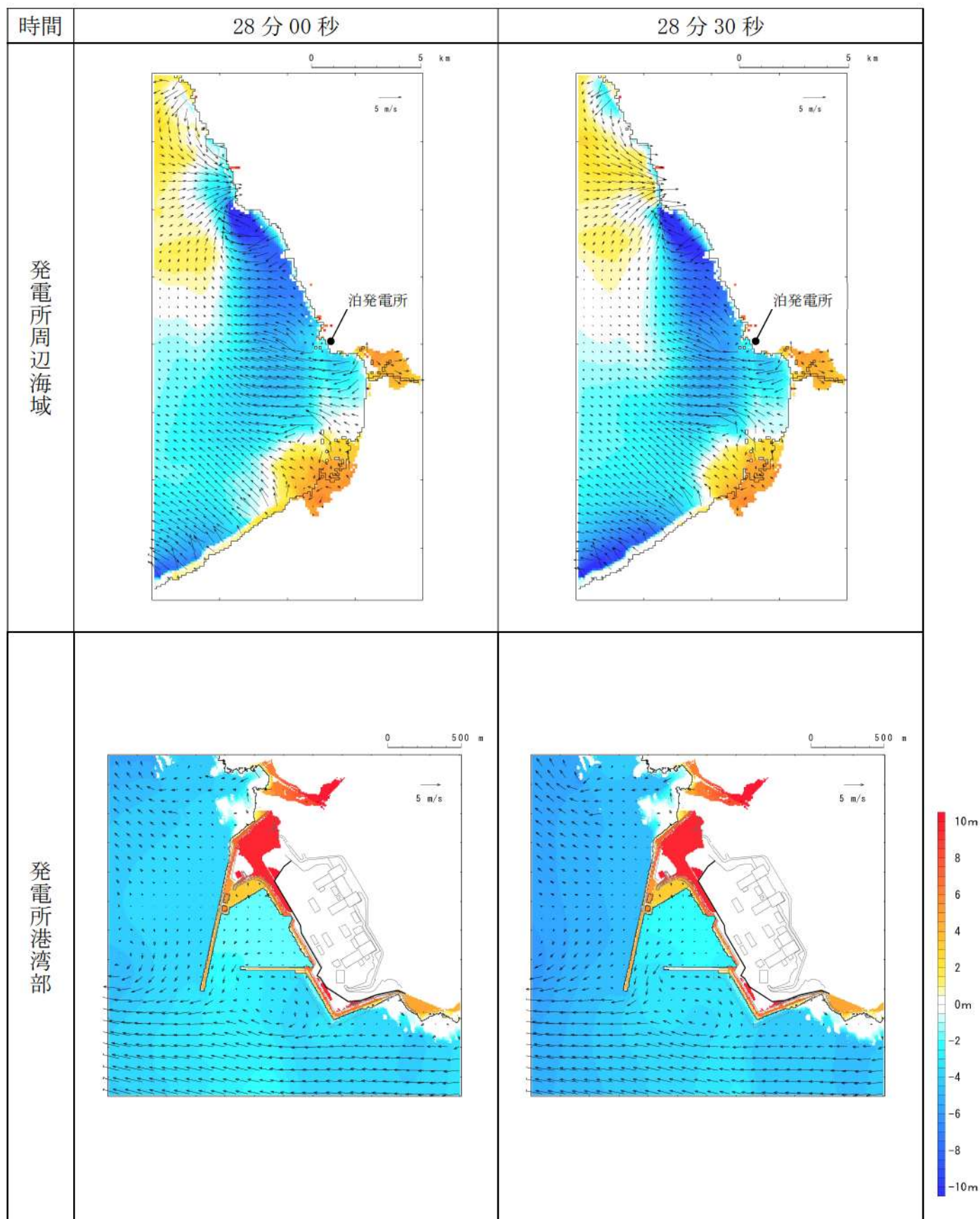
第 4 図-22 基準津波 C（防波堤損傷なし）の水位変動・流向ベクトル (22/54)
