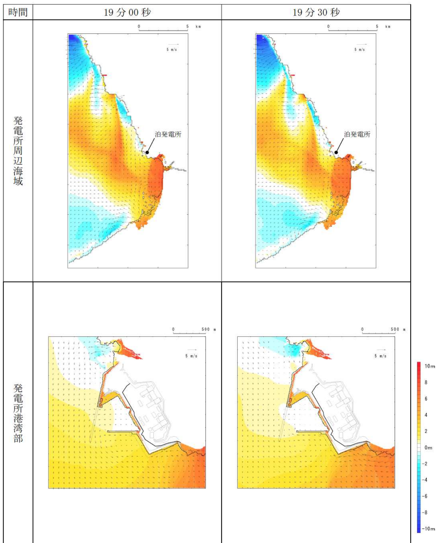
第3図-12 基準津波B（北防波堤損傷）の水位変動・流向ベクトル(12/53)
