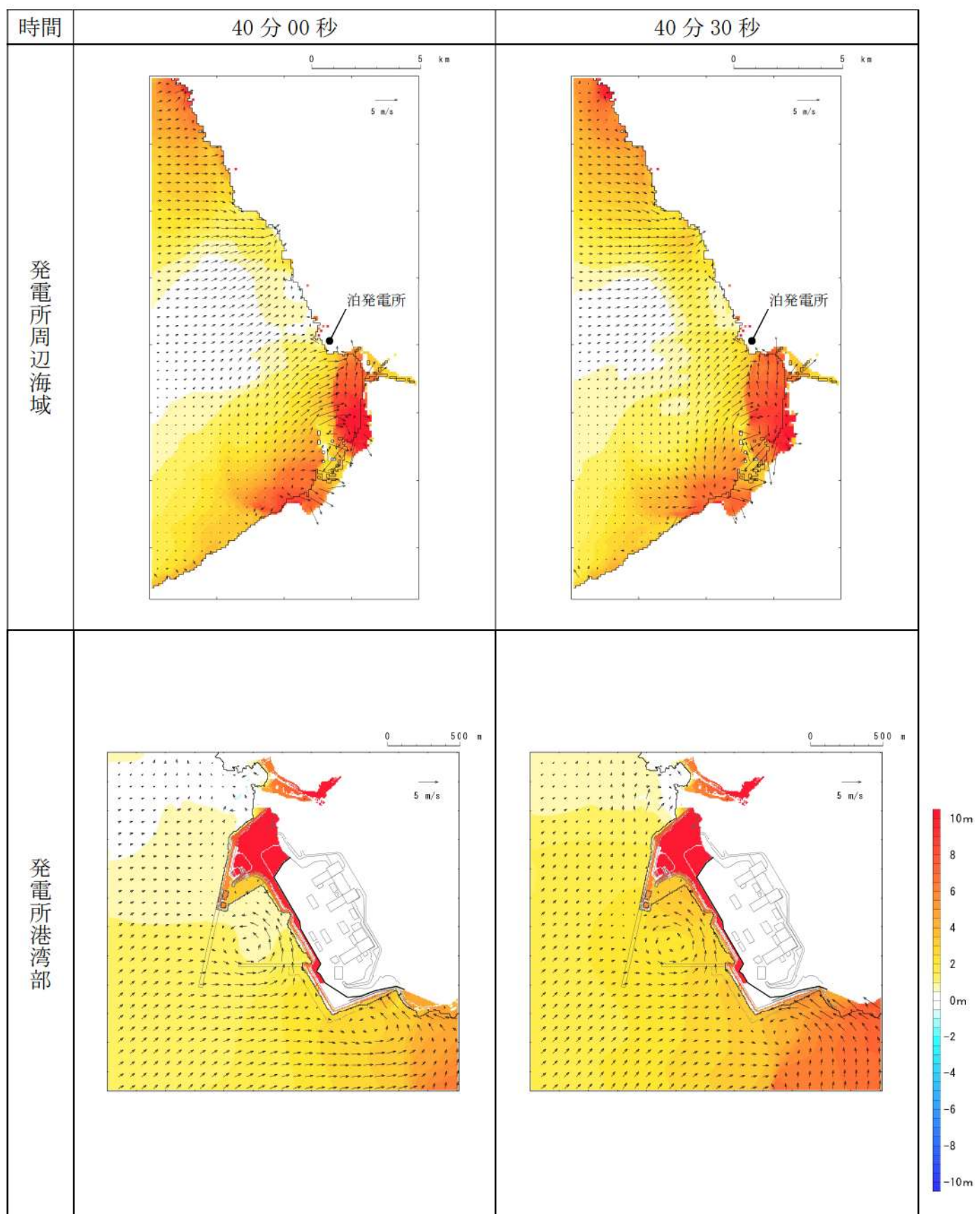
第 6 図-33 基準津波 D（北及び南防波堤損傷）の水位変動・流向ベクトル(33/53)
