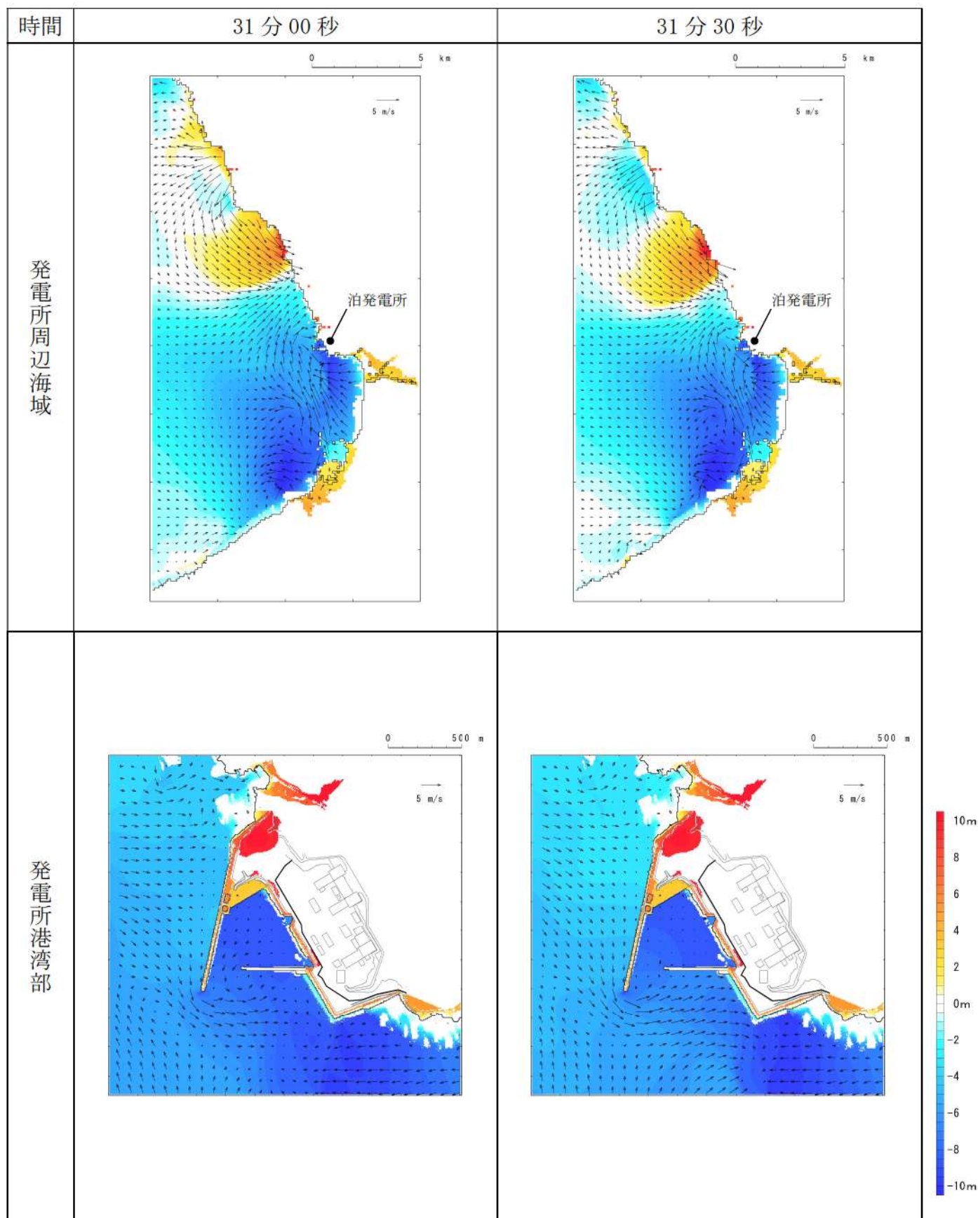
第 5 図-24 基準津波 D (防波堤損傷なし) の水位変動・流向ベクトル (24/53)
