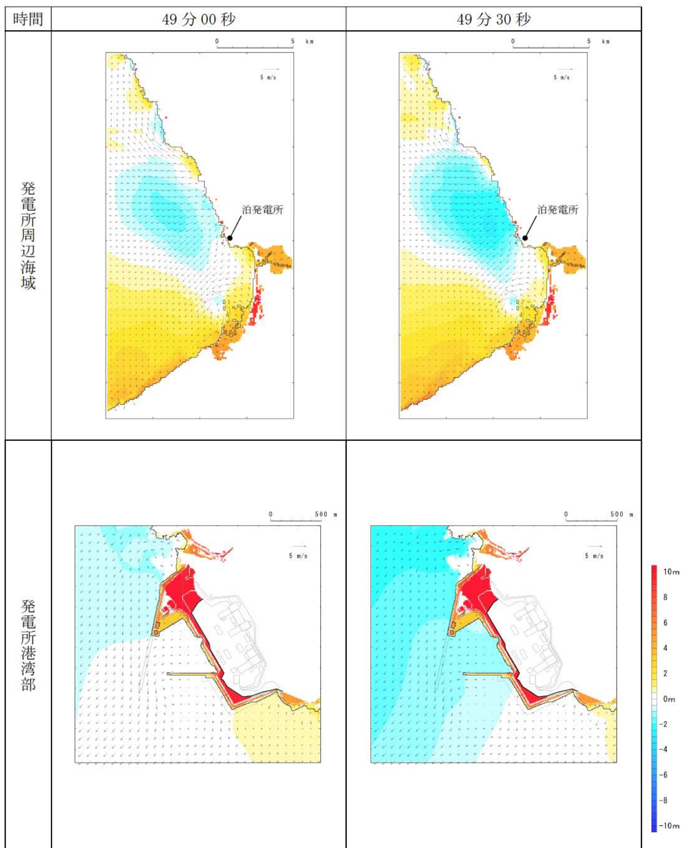
第3図-42 基準津波B（北防波堤損傷）の水位変動・流向ベクトル(42/53)
