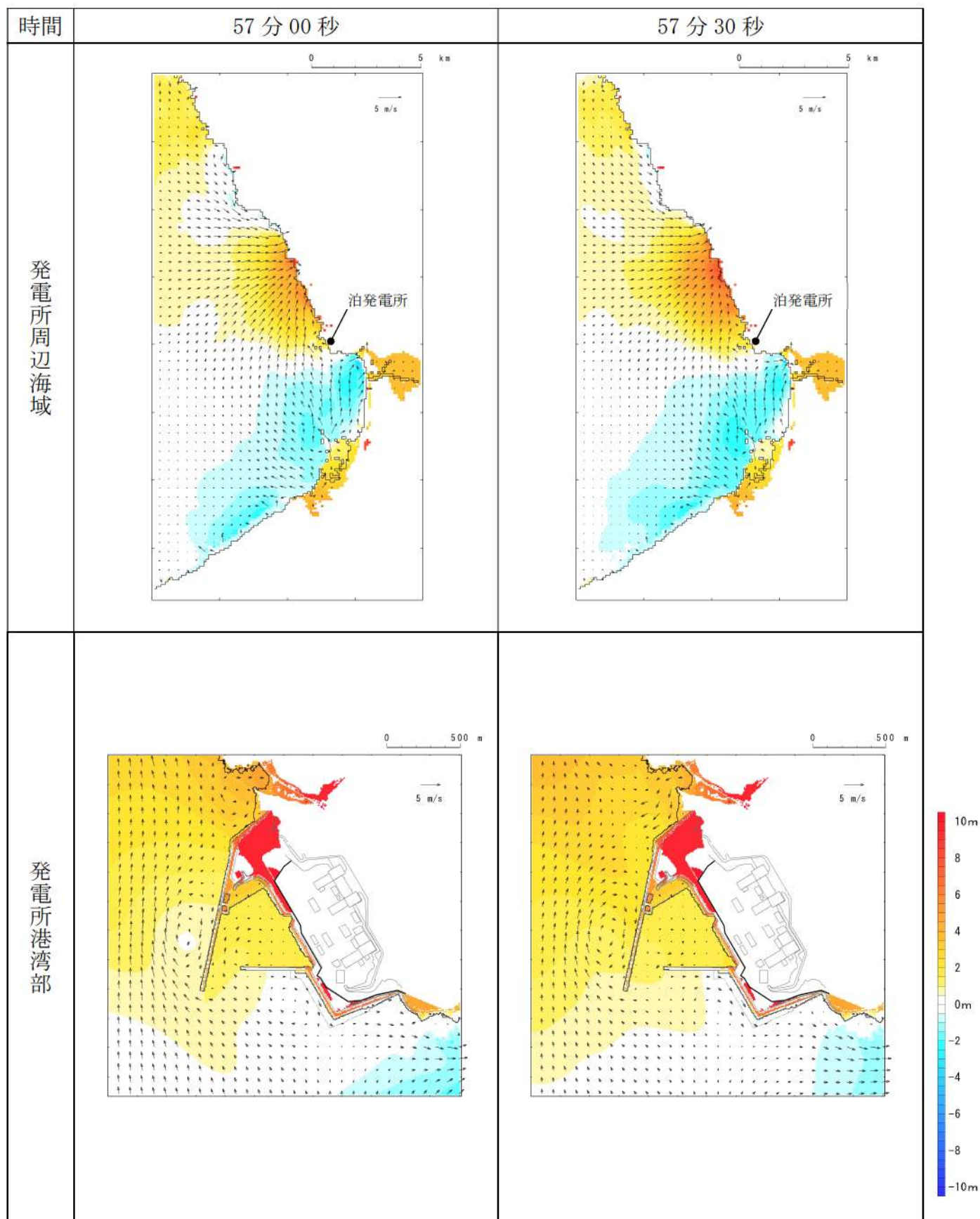
第4図-51 基準津波C（防波堤損傷なし）の水位変動・流向ベクトル(51/54)
