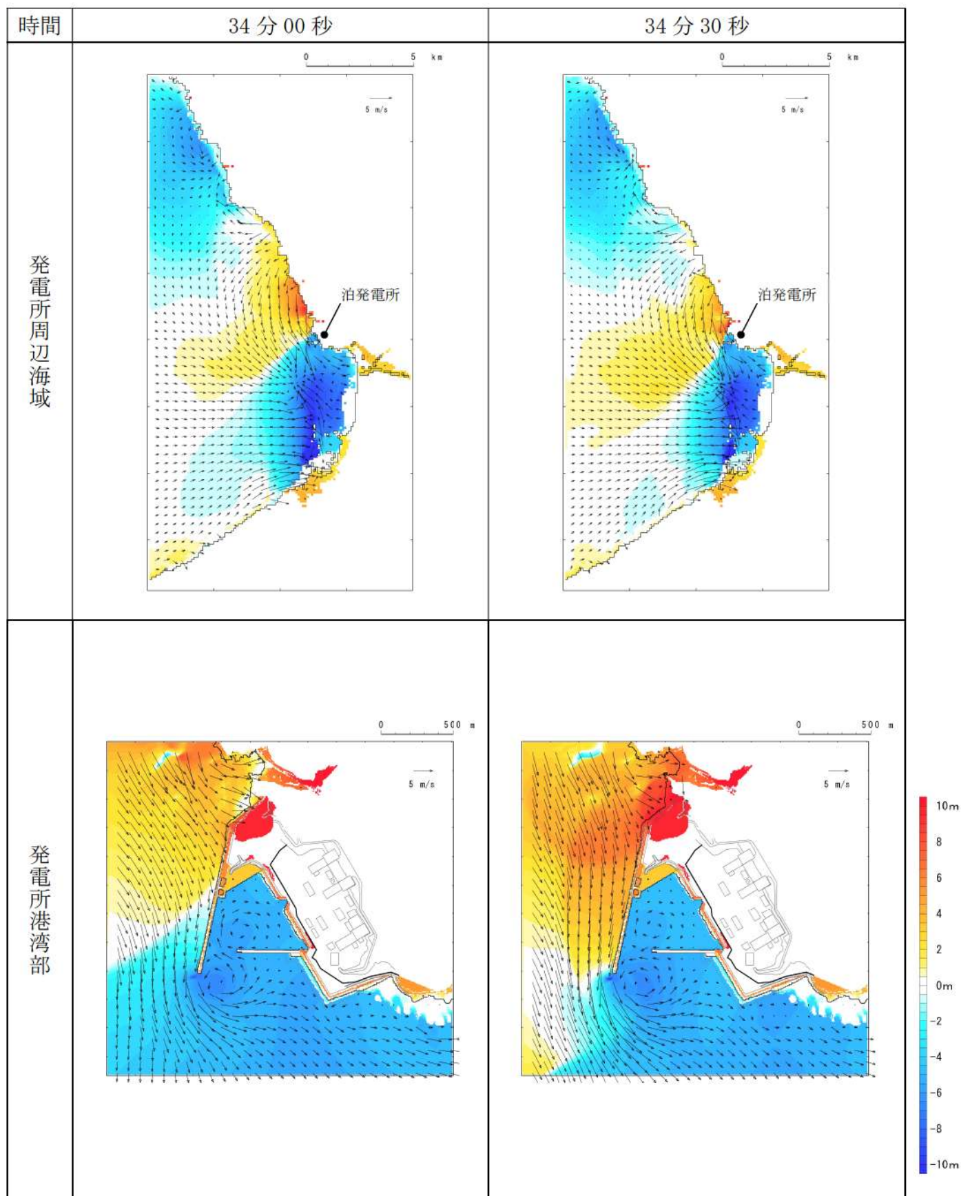
第 5 図-27 基準津波 D（防波堤損傷なし）の水位変動・流向ベクトル (27/53)
