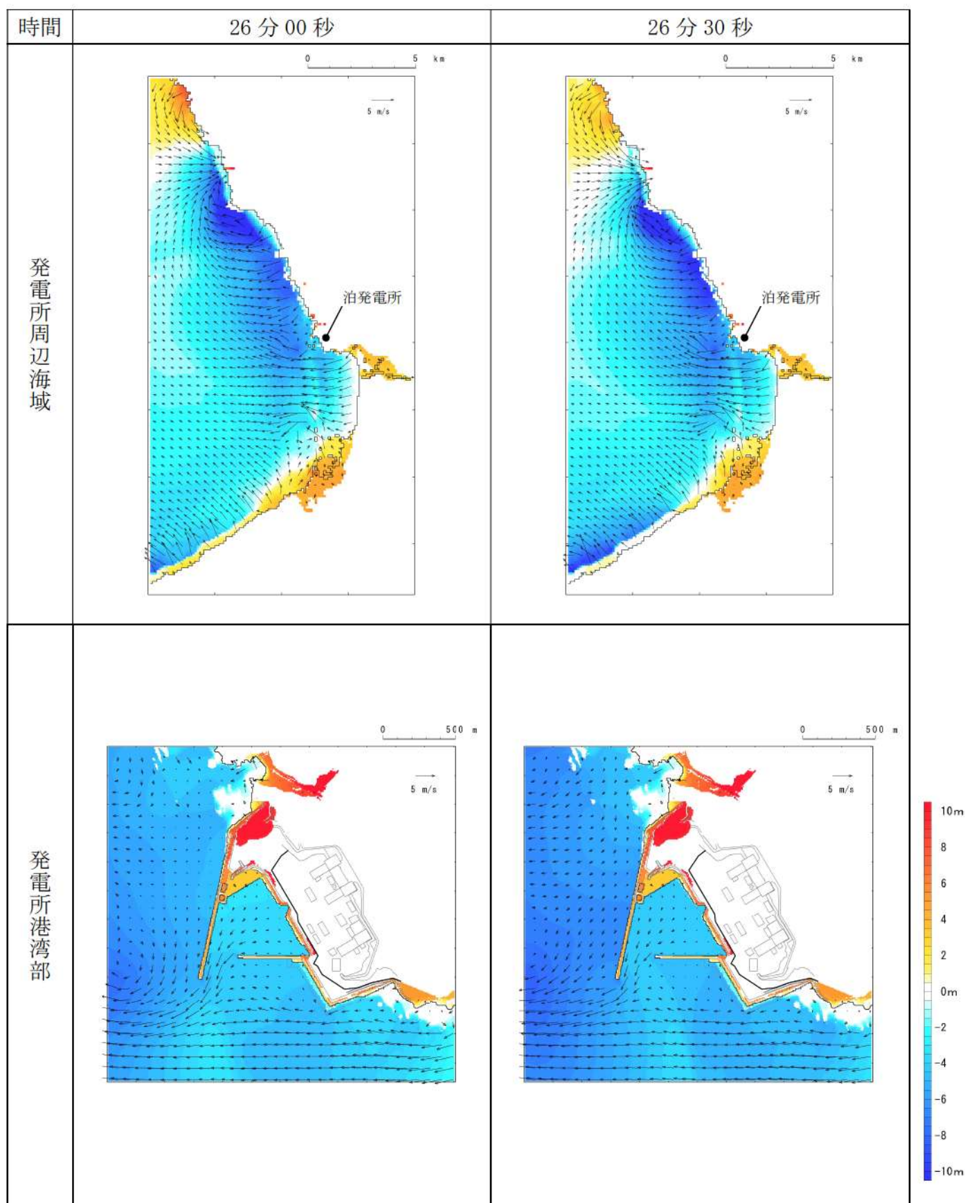
第 5 図-19 基準津波 D（防波堤損傷なし）の水位変動・流向ベクトル(19/53)
