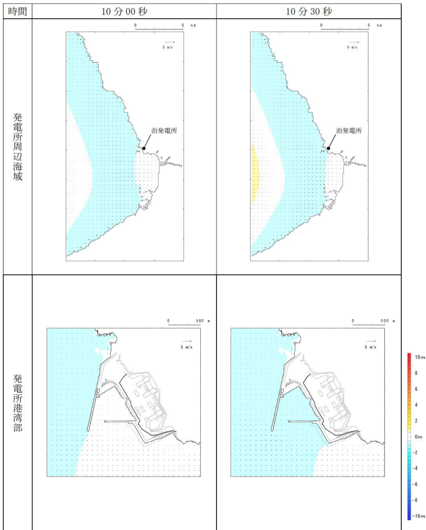
第4図-4 基準津波C（防波堤損傷なし）の水位変動・流向ベクトル(4/54)
