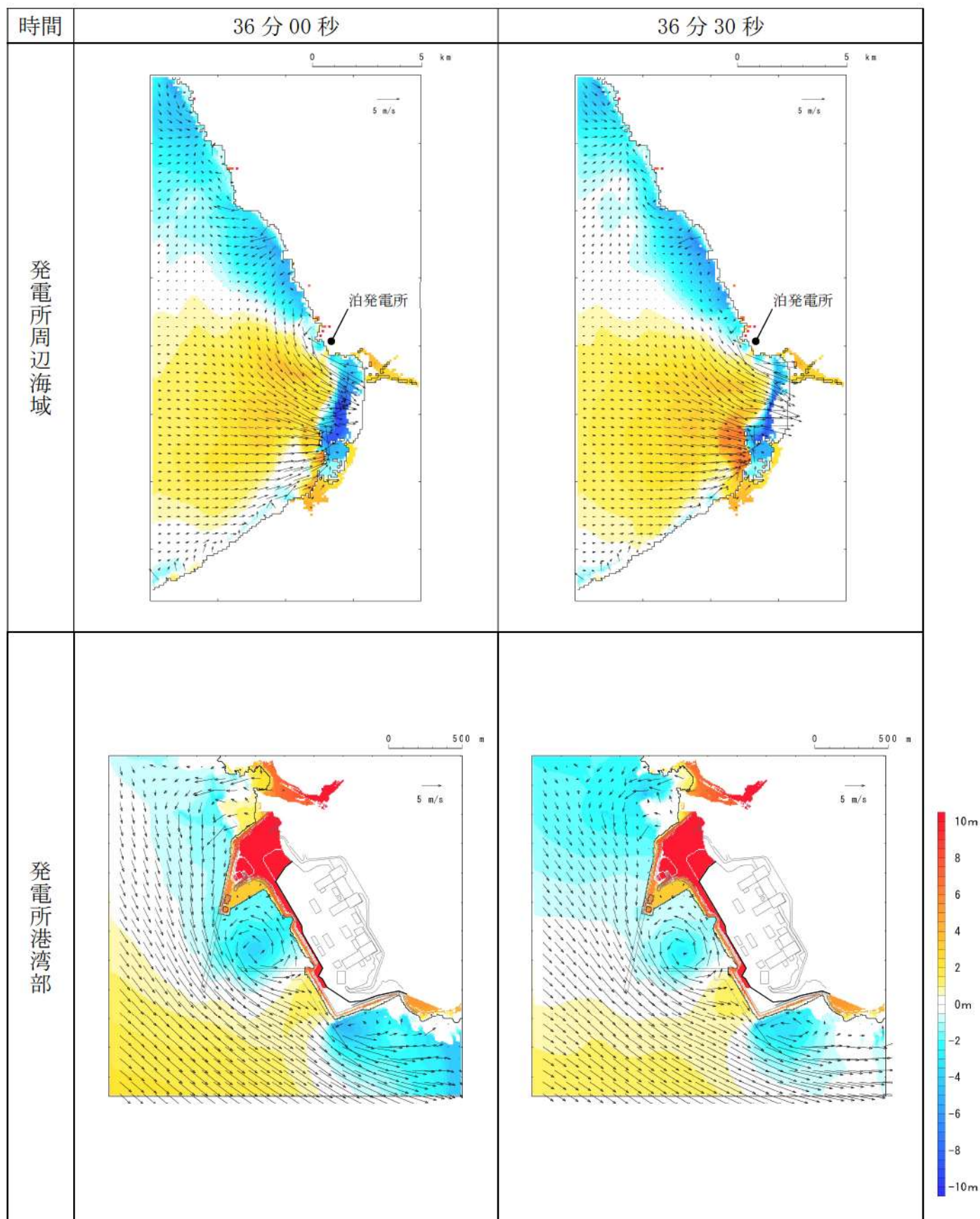
第 6 図-29 基準津波 D（北及び南防波堤損傷）の水位変動・流向ベクトル (29/53)
