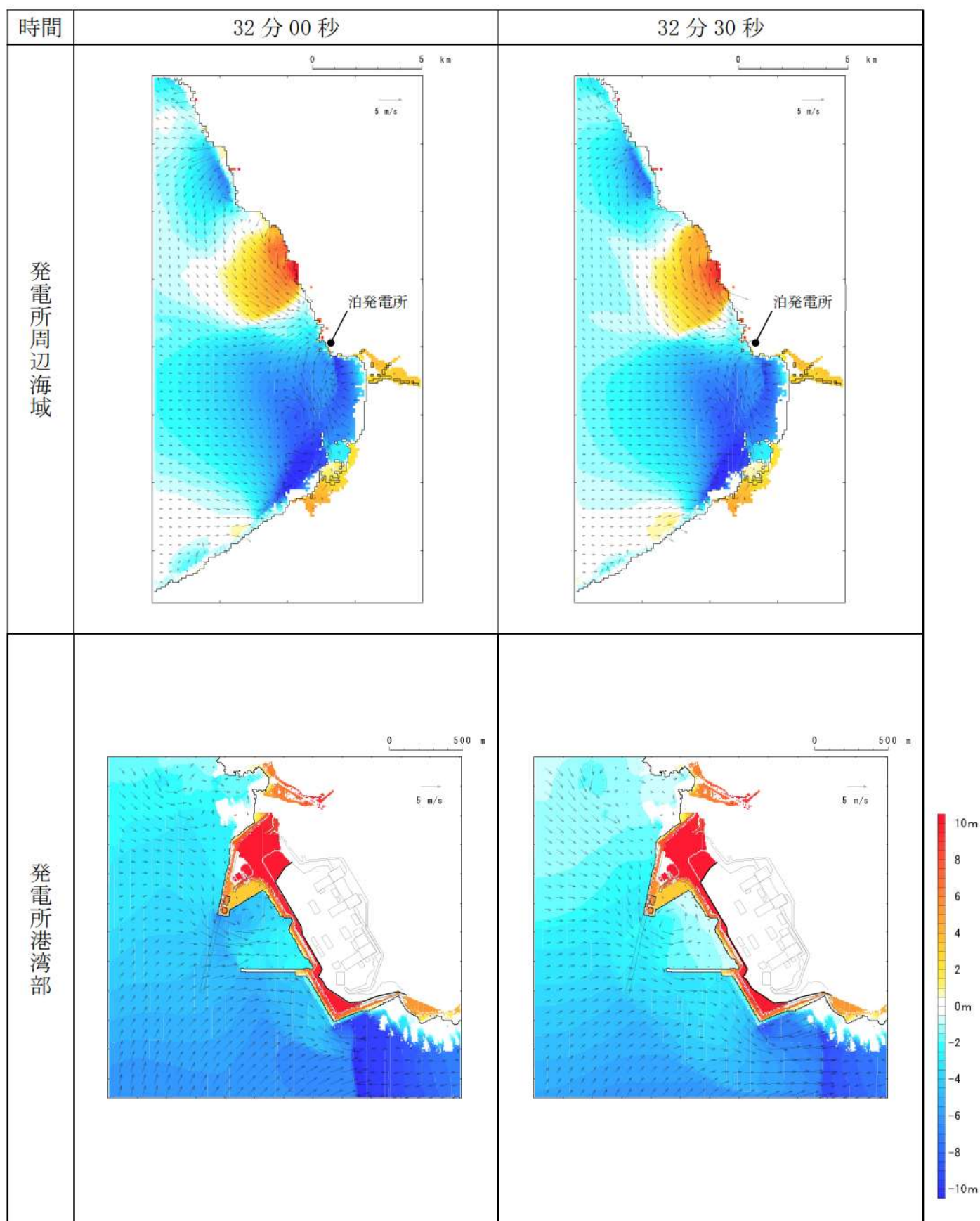
第3図-25 基準津波B（北防波堤損傷）の水位変動・流向ベクトル(25/53)
