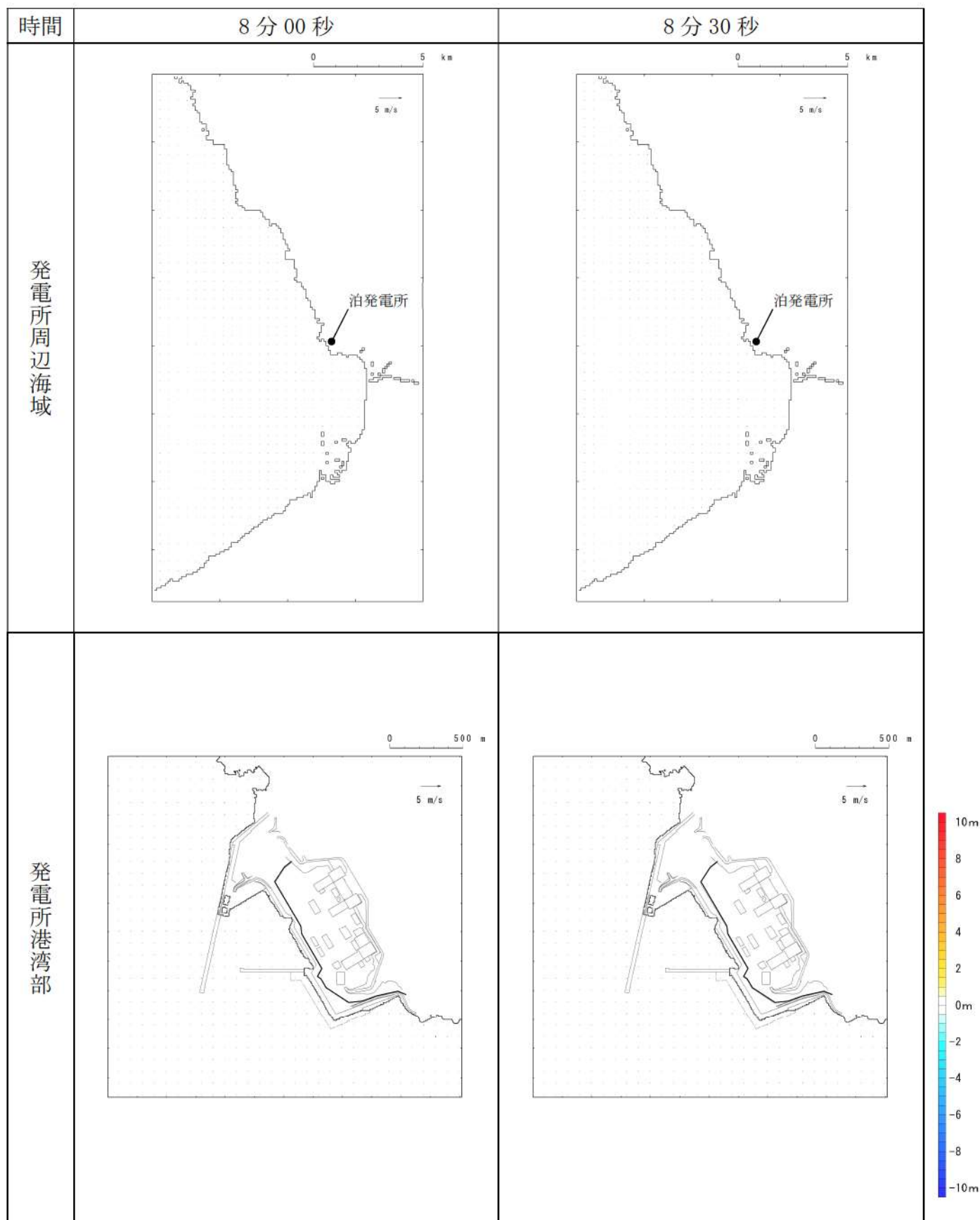
第 6 図- 1 基準津波 D（北及び南防波堤損傷）の水位変動・流向ベクトル(1/53)
