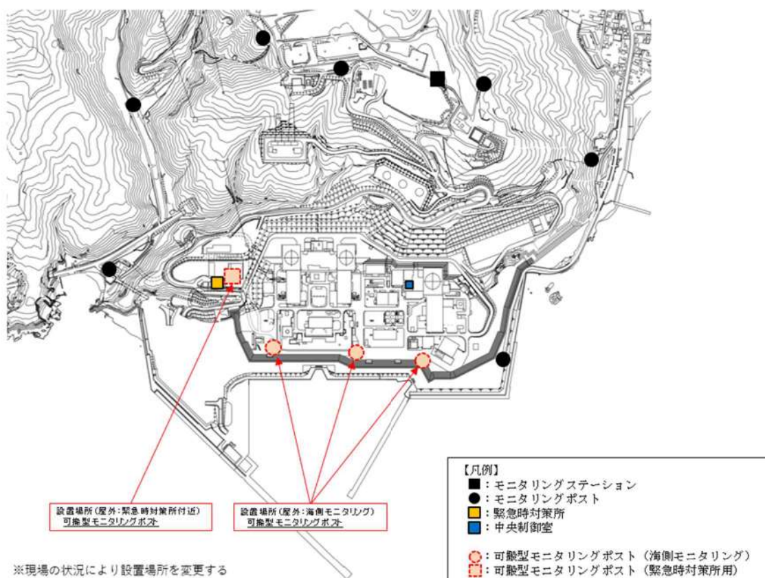
第1.17.4図 可搬型モニタリングポスト設置場所 (発電所海側及び緊急時対策所付近への設置)
