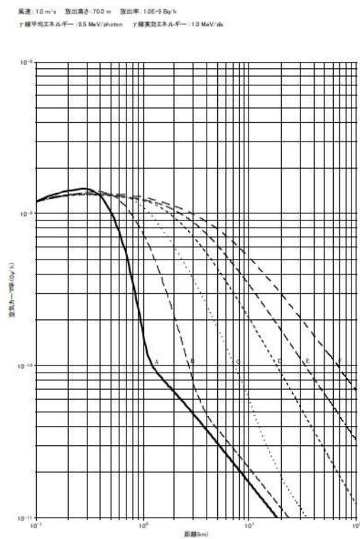
第 1 図 風下軸上空気カーマ率
