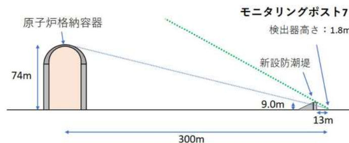
第2図 モニタリングポスト7から3号炉の原子炉方向を見たときの新設防潮堤との位置関係
