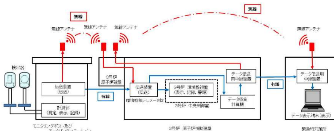
第 1.1.3 図 モニタリングポスト及びモニタリングステーション設備の伝送概略図
