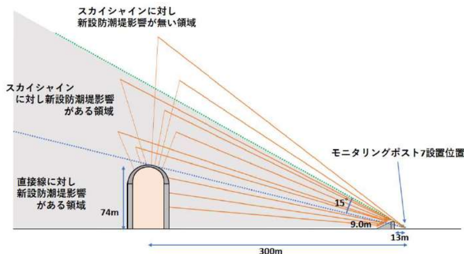
第6図 直接線及びスカイシャイン線の経路
