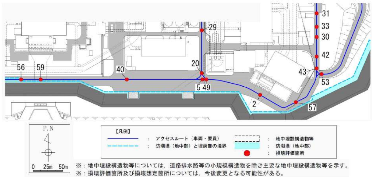
第 6-44 図 構造物損壊による段差発生想定箇所（5/5）（D エリア）
