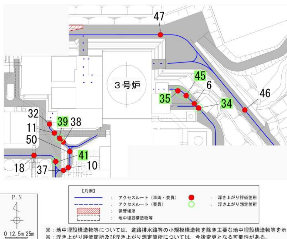
第 6-42 図 液状化による浮き上がりの評価結果（4/5）（C エリア）
