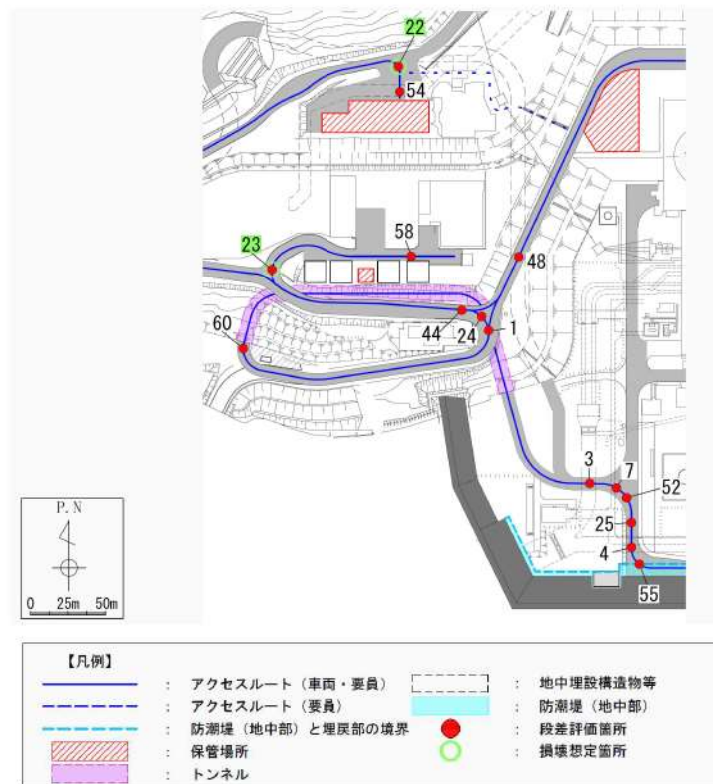
第 6-44 図 構造物損壊による段差発生想定箇所（2/5）（A エリア）
