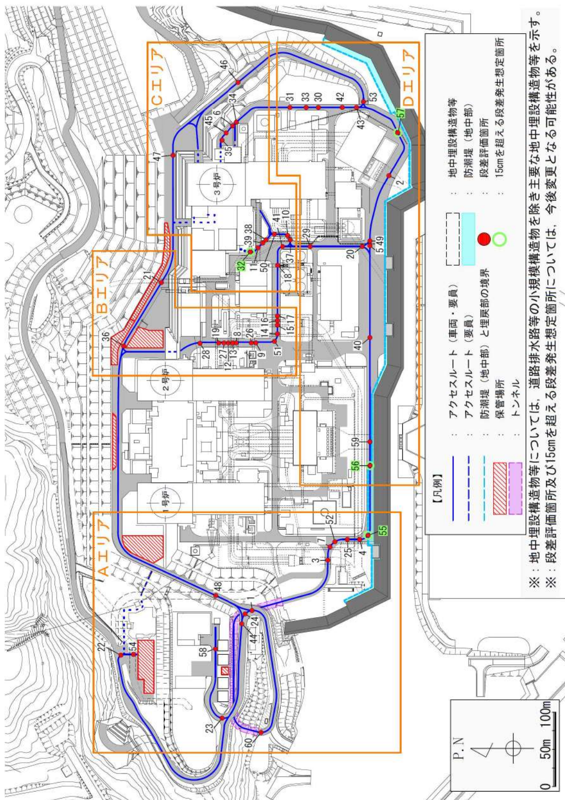
第6-20図 地中埋設構造物等と埋戻部との境界部における段差評価結果 (1/5) (全体)
