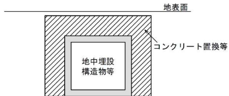
第 6-43 図 浮き上がり対策工概念図
