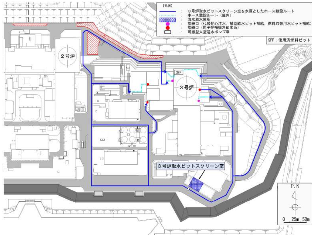
第9図 海水取水ホースの敷設ルート図(1/2)
