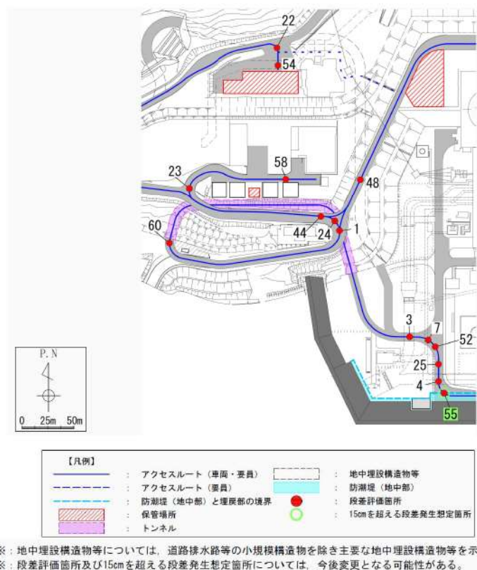
第 6-20 図 地中埋設構造物等と埋戻部との境界部における 段差評価結果（2/5）（A エリア）
