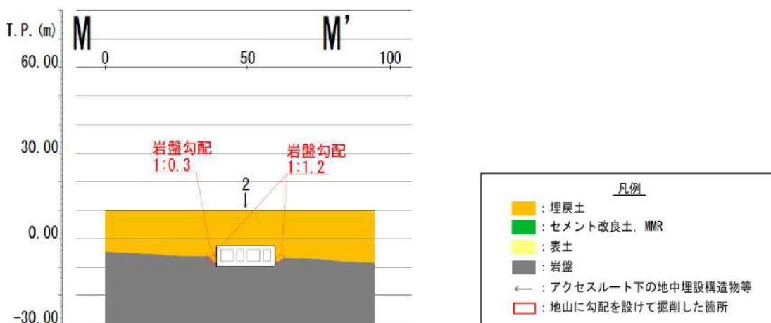
第2図 アクセスルート地盤構造概要(7/8)
