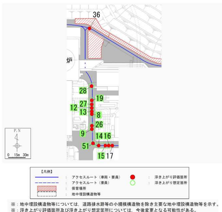
第 6-42 図 液状化による浮き上がりの評価結果（3/5）（B エリア）
