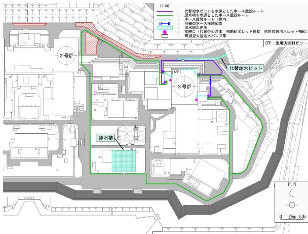
第8図 淡水取水ホースの敷設ルート図
