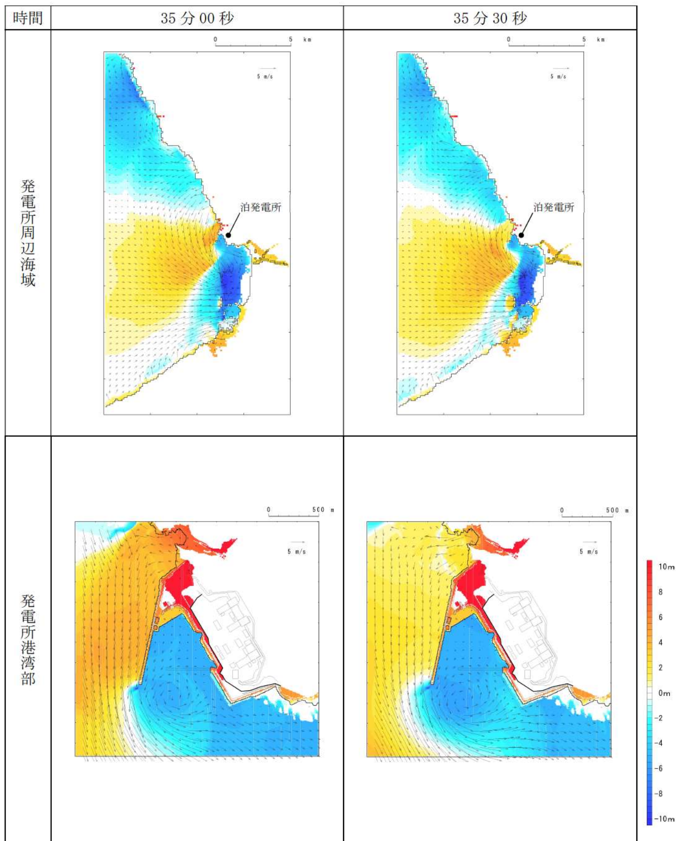
第 17 図-28 基準津波（波源K，南防波堤損傷）の水位変動・流向ベクトル(28/53)
