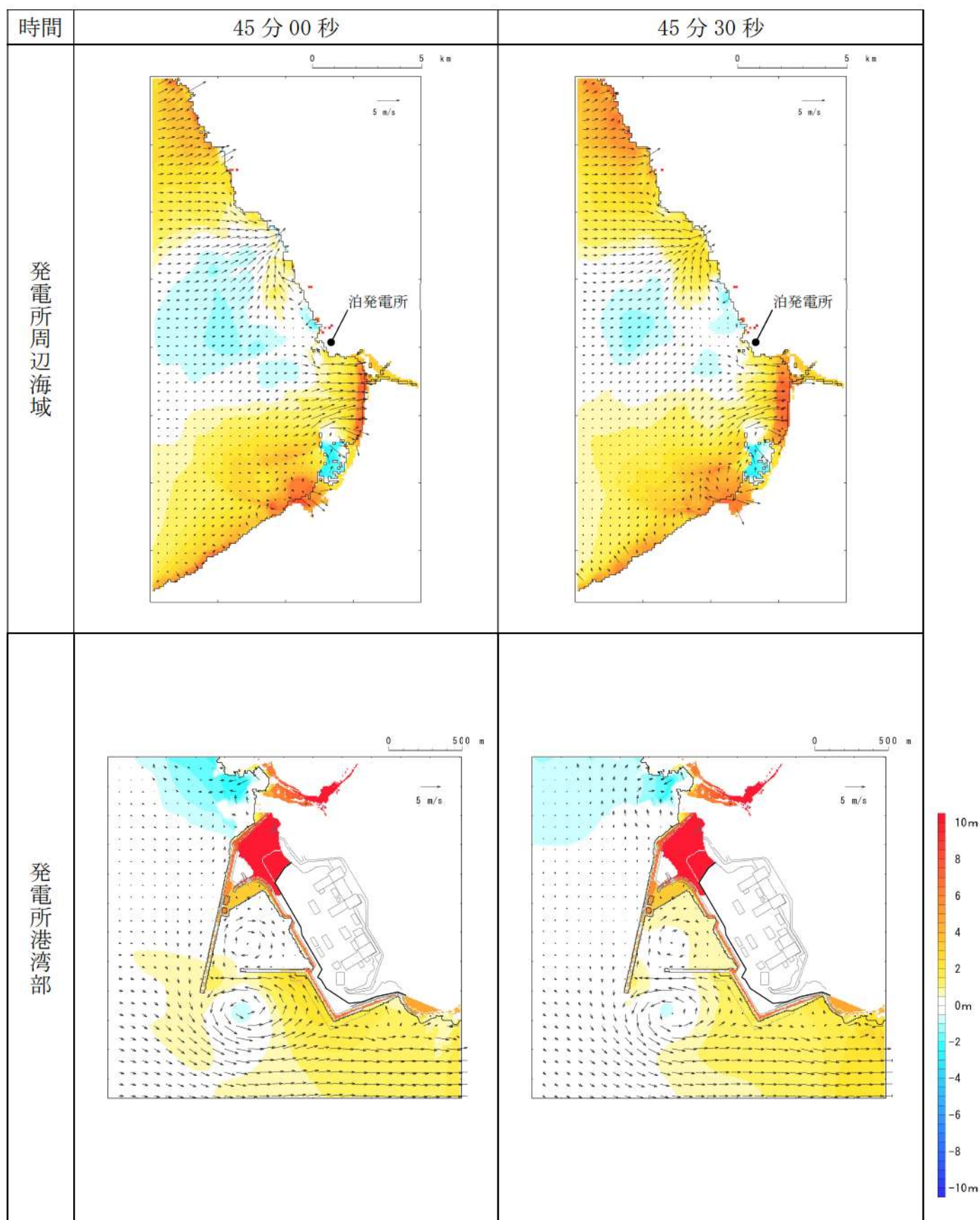
第 15 図-35 基準津波（波源 I，防波堤損傷なし）の水位変動・流向ベクトル(35/50)
