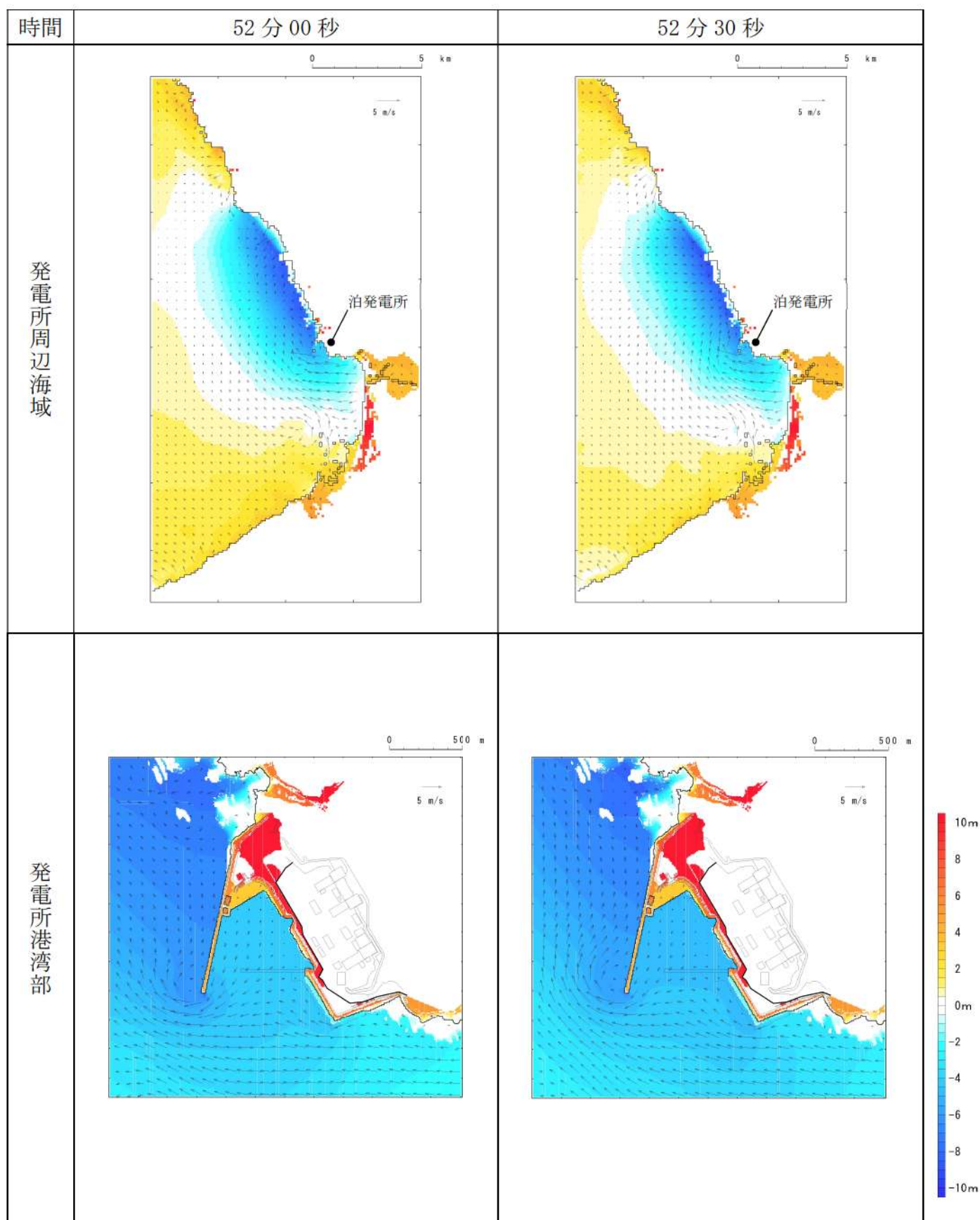
第 17 図-45 基準津波（波源K，南防波堤損傷）の水位変動・流向ベクトル(45/53)
