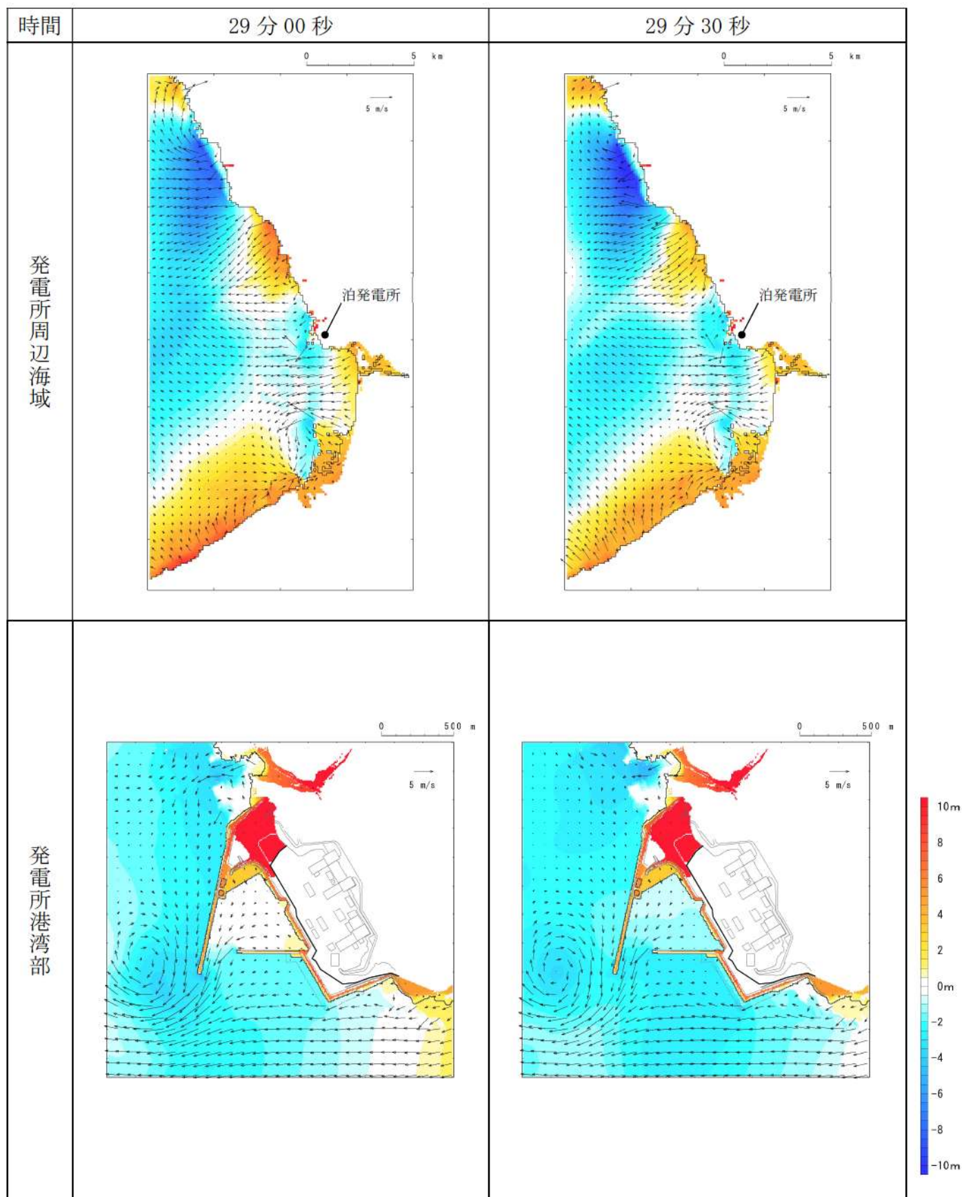
第 15 図-19 基準津波（波源 I，防波堤損傷なし）の水位変動・流向ベクトル(19/50)
