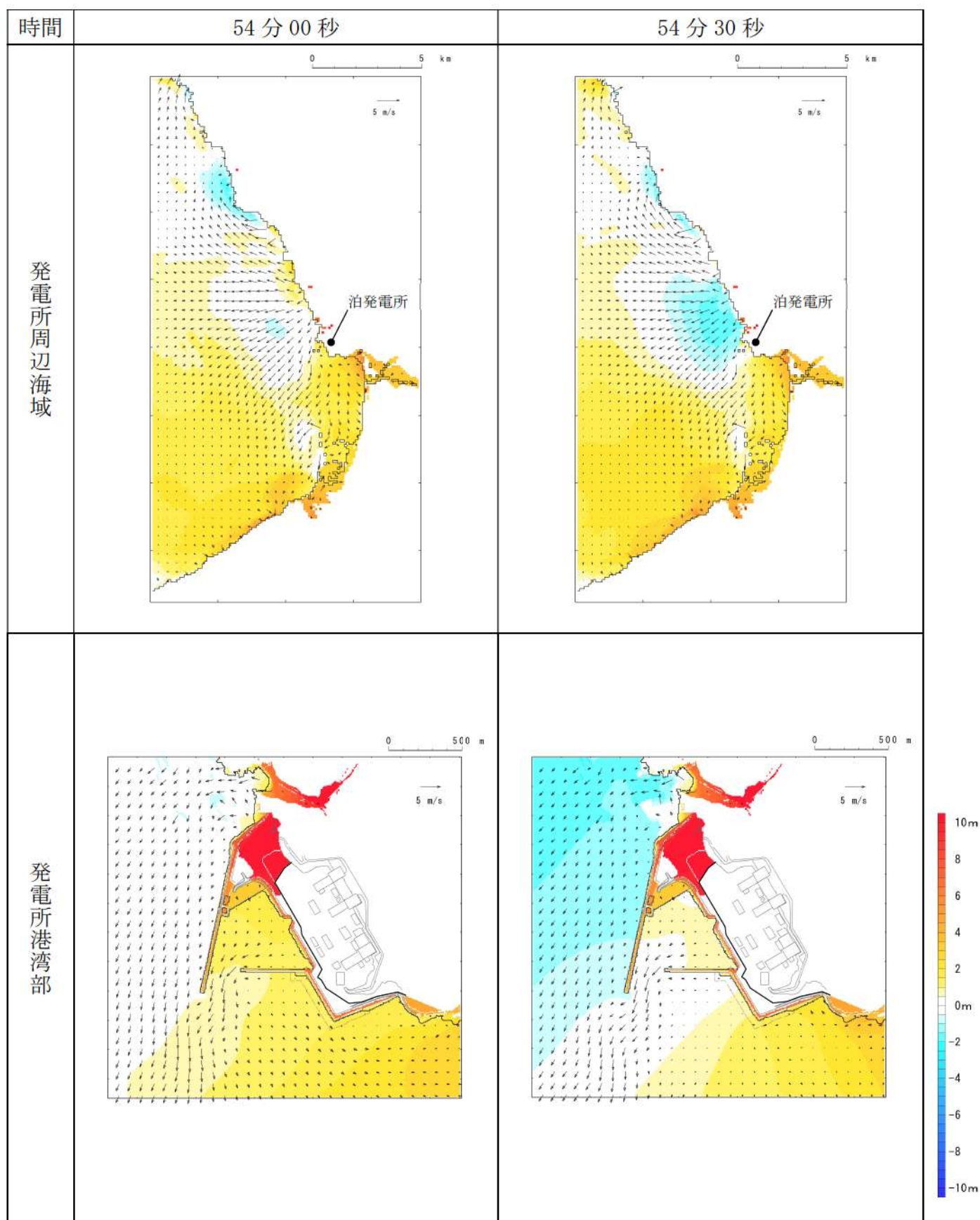
第 15 図-44 基準津波（波源 I，防波堤損傷なし）の水位変動・流向ベクトル(44/50)
