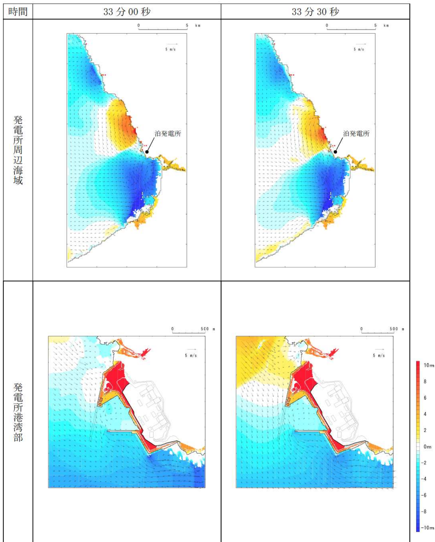
第 14 図-26 基準津波（波源H，北防波堤損傷）の水位変動・流向ベクトル(26/53)
