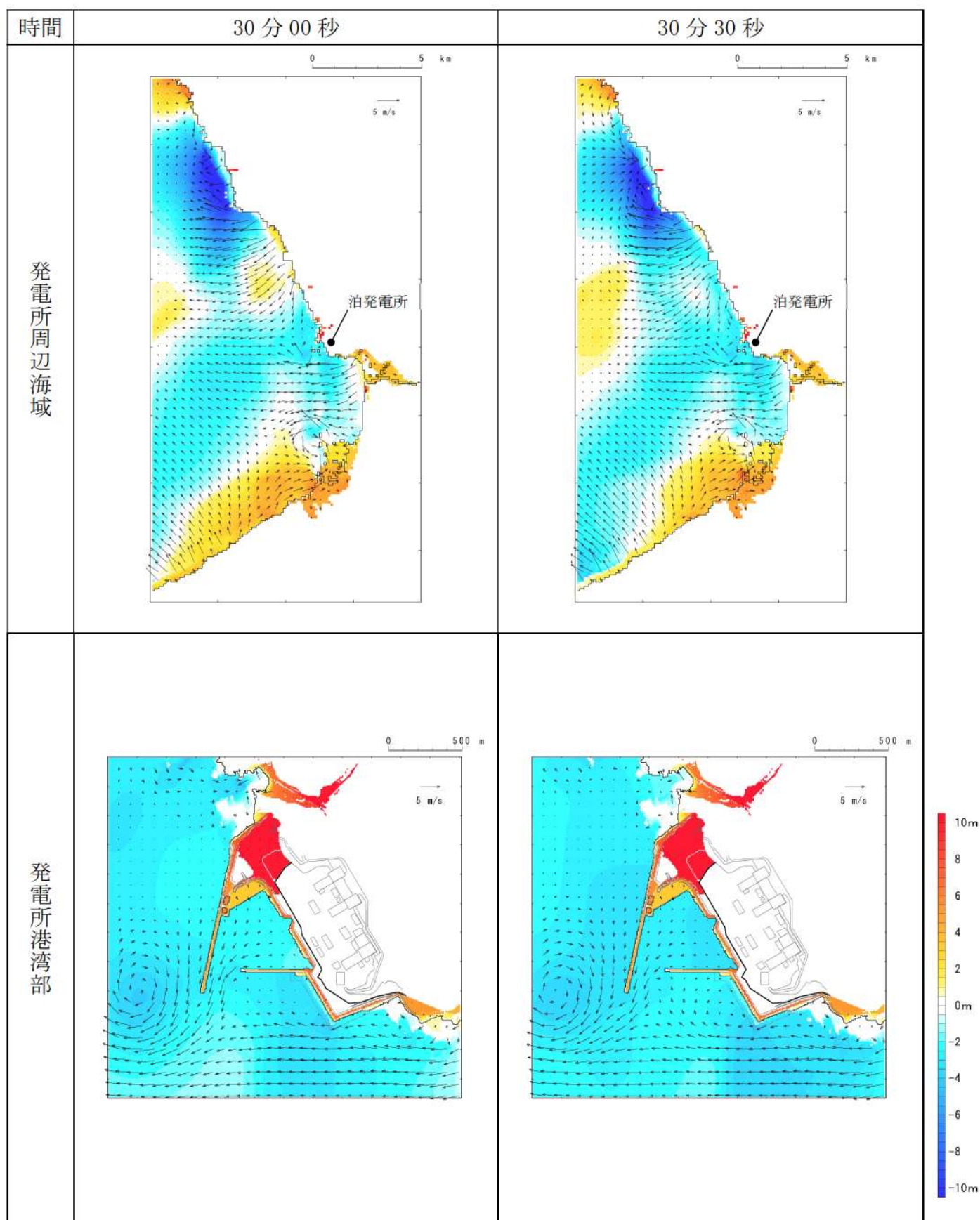
第 15 図-20 基準津波（波源 I，防波堤損傷なし）の水位変動・流向ベクトル(20/50)
