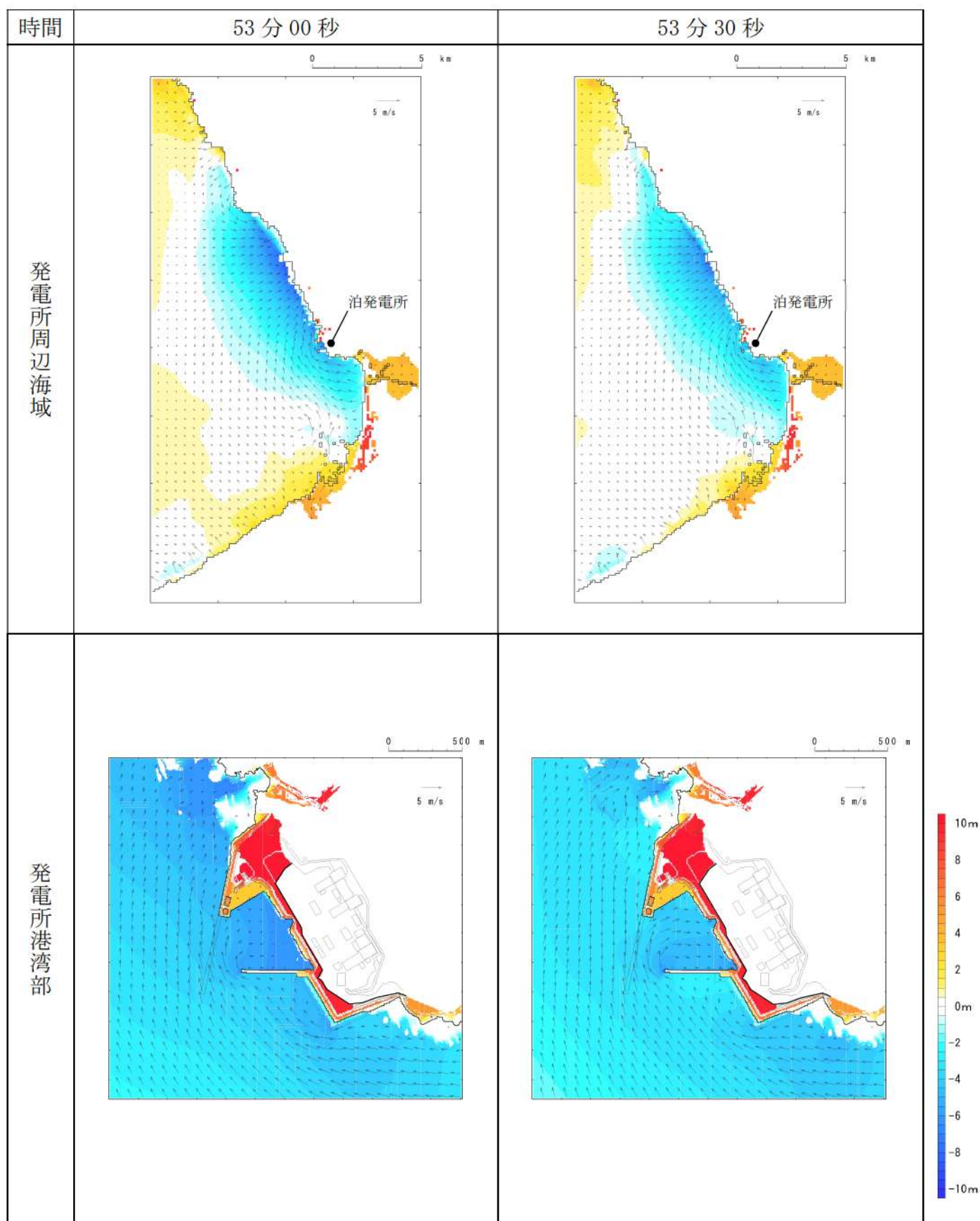
第 14 図-46 基準津波（波源H，北防波堤損傷）の水位変動・流向ベクトル(46/53)
