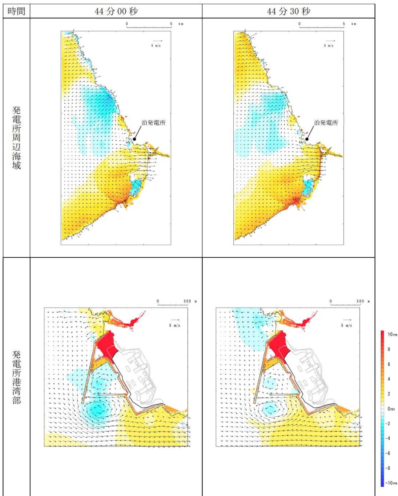
第 15 図-34 基準津波（波源 I，防波堤損傷なし）の水位変動・流向ベクトル(34/50)
