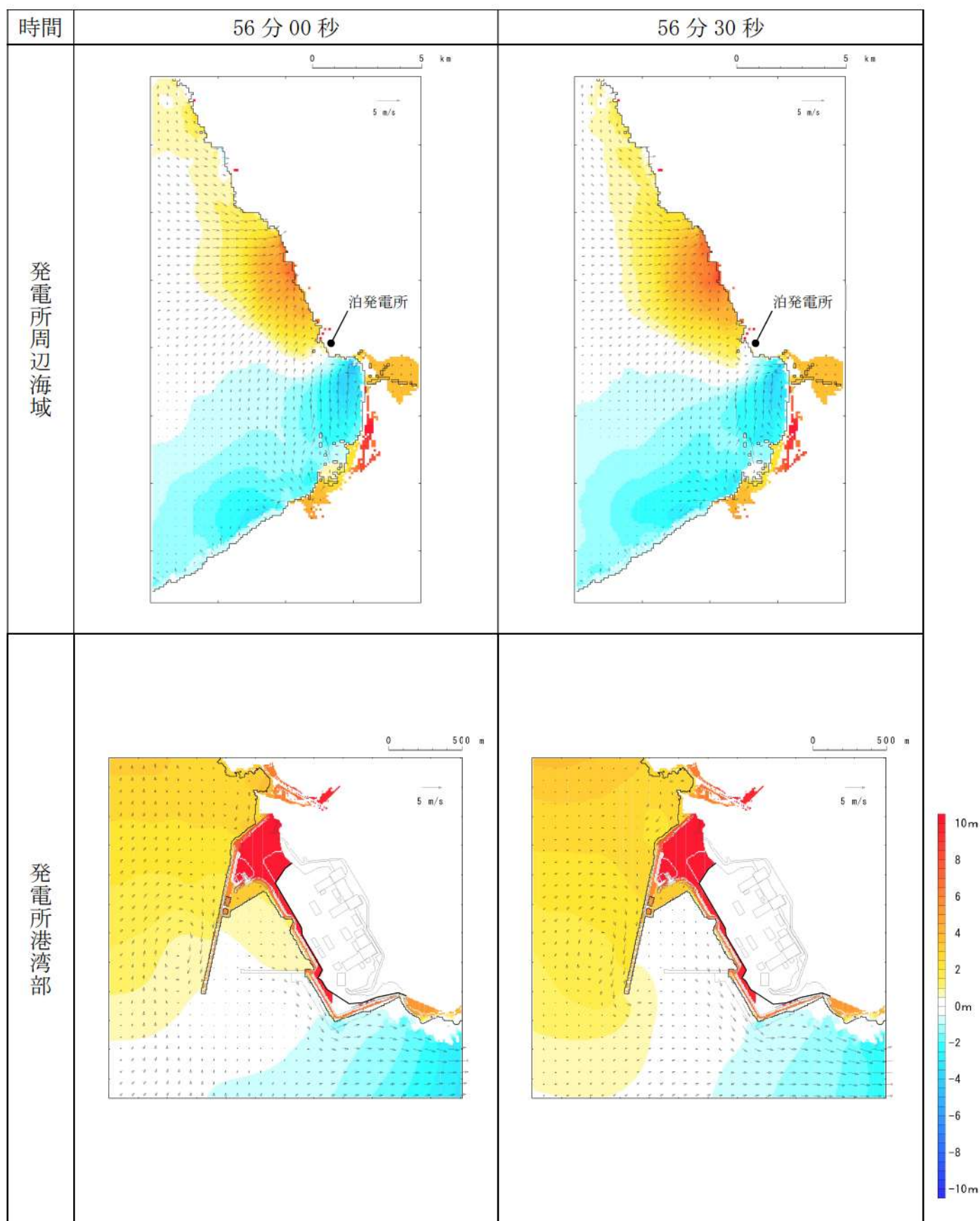
第 13 図-49 基準津波（波源 G，南防波堤損傷）の水位変動・流向ベクトル(49/53)
