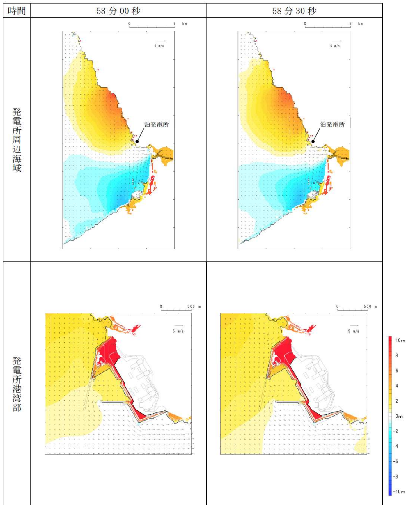
第 14 図-51 基準津波（波源H，北防波堤損傷）の水位変動・流向ベクトル(51/53)
