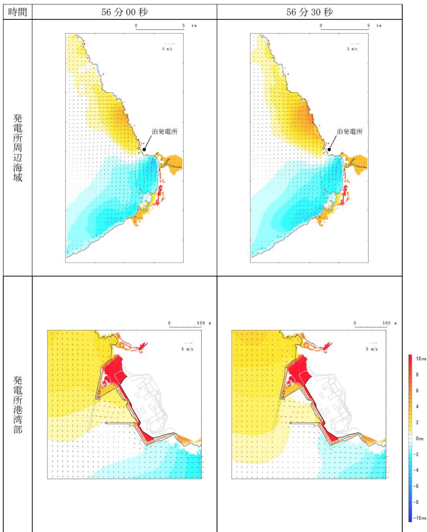
第 14 図-49 基準津波（波源H，北防波堤損傷）の水位変動・流向ベクトル(49/53)
