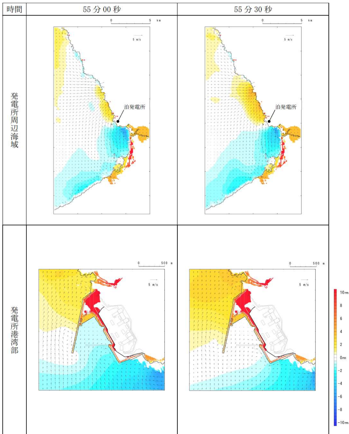
第 17 図-48 基準津波（波源K，南防波堤損傷）の水位変動・流向ベクトル(48/53)
