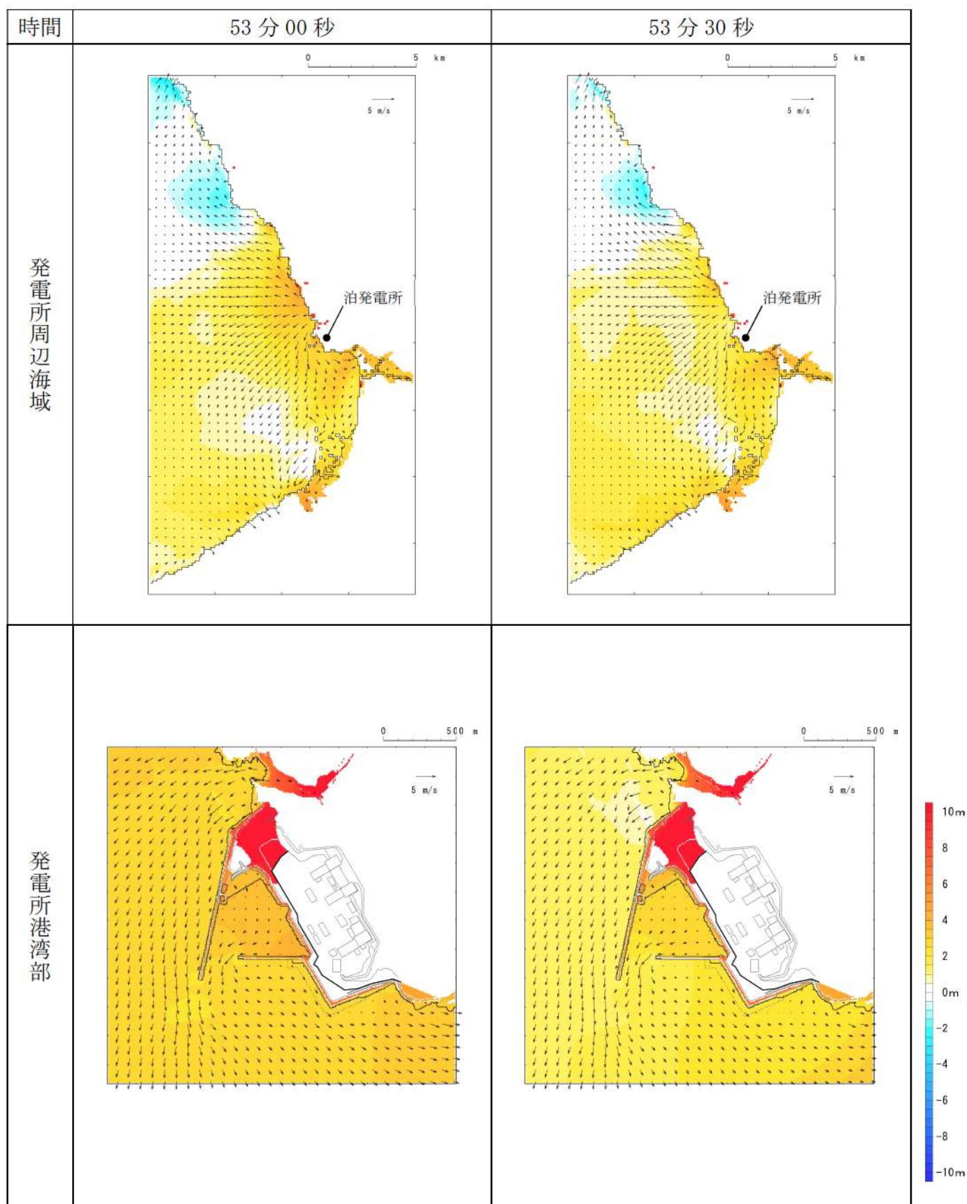
第 15 図-43 基準津波（波源 I，防波堤損傷なし）の水位変動・流向ベクトル(43/50)
