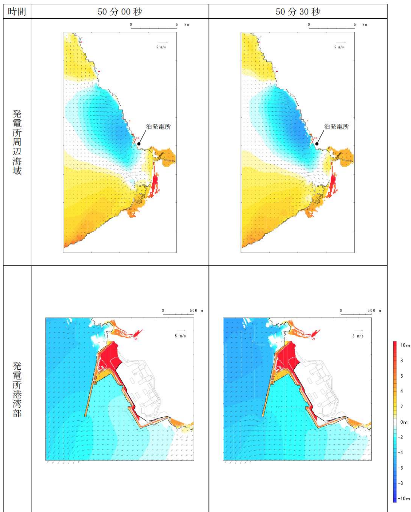
第 13 図-43 基準津波（波源 G，南防波堤損傷）の水位変動・流向ベクトル(43/53)
