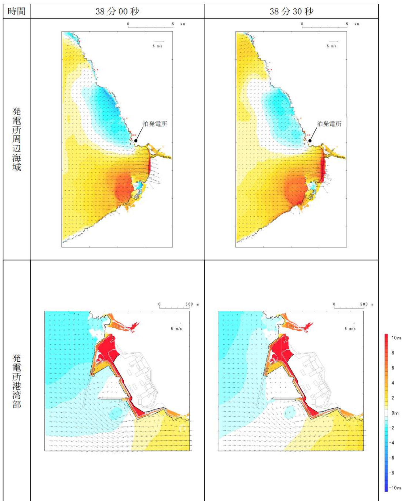
第 14 図-31 基準津波（波源H，北防波堤損傷）の水位変動・流向ベクトル(31/53)
