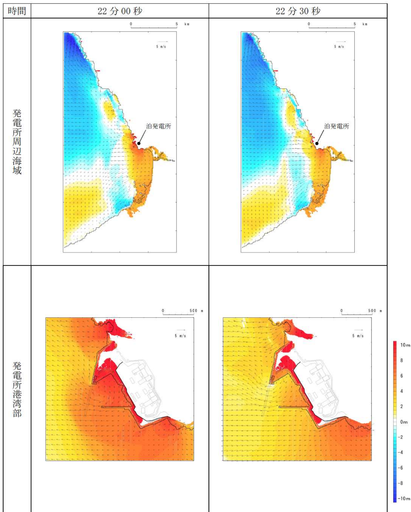
第 14 図-15 基準津波（波源H，北防波堤損傷）の水位変動・流向ベクトル(15/53)
