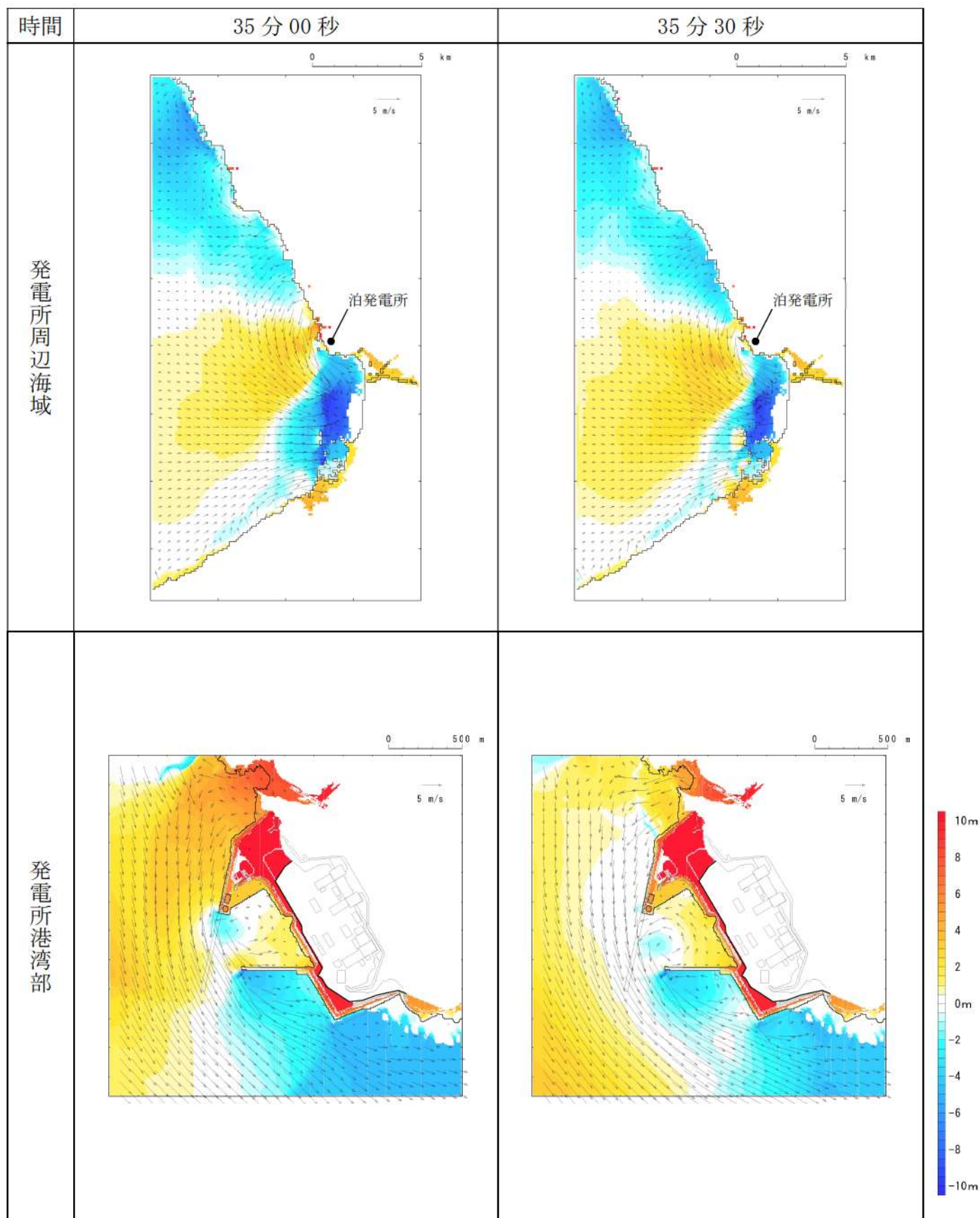
第 14 図-28 基準津波（波源H，北防波堤損傷）の水位変動・流向ベクトル(28/53)
