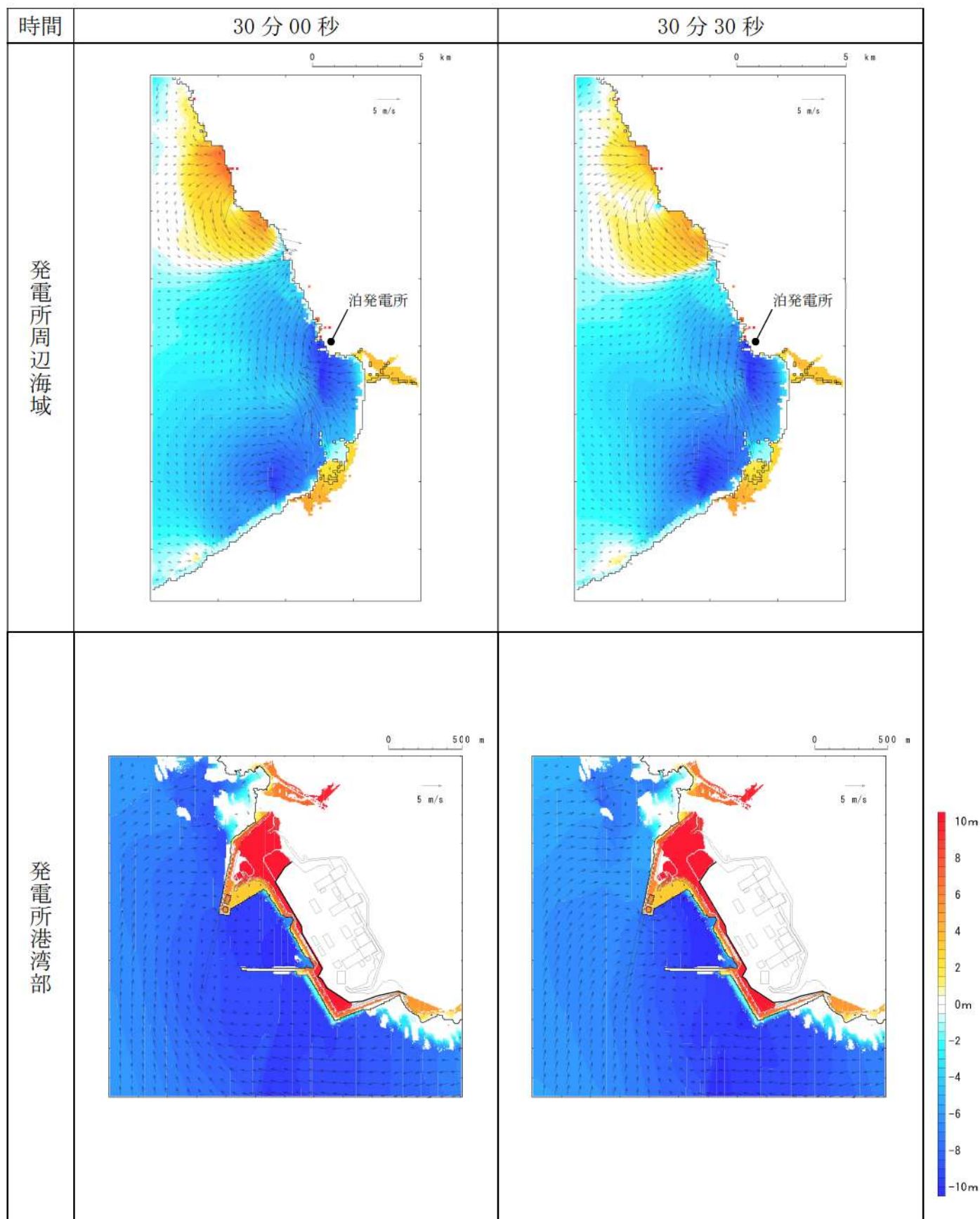
第 14 図-23 基準津波（波源H，北防波堤損傷）の水位変動・流向ベクトル(23/53)
