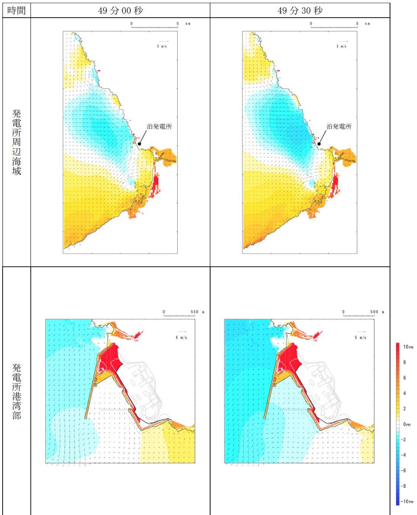
第 13 図-42 基準津波（波源 G，南防波堤損傷）の水位変動・流向ベクトル(42/53)
