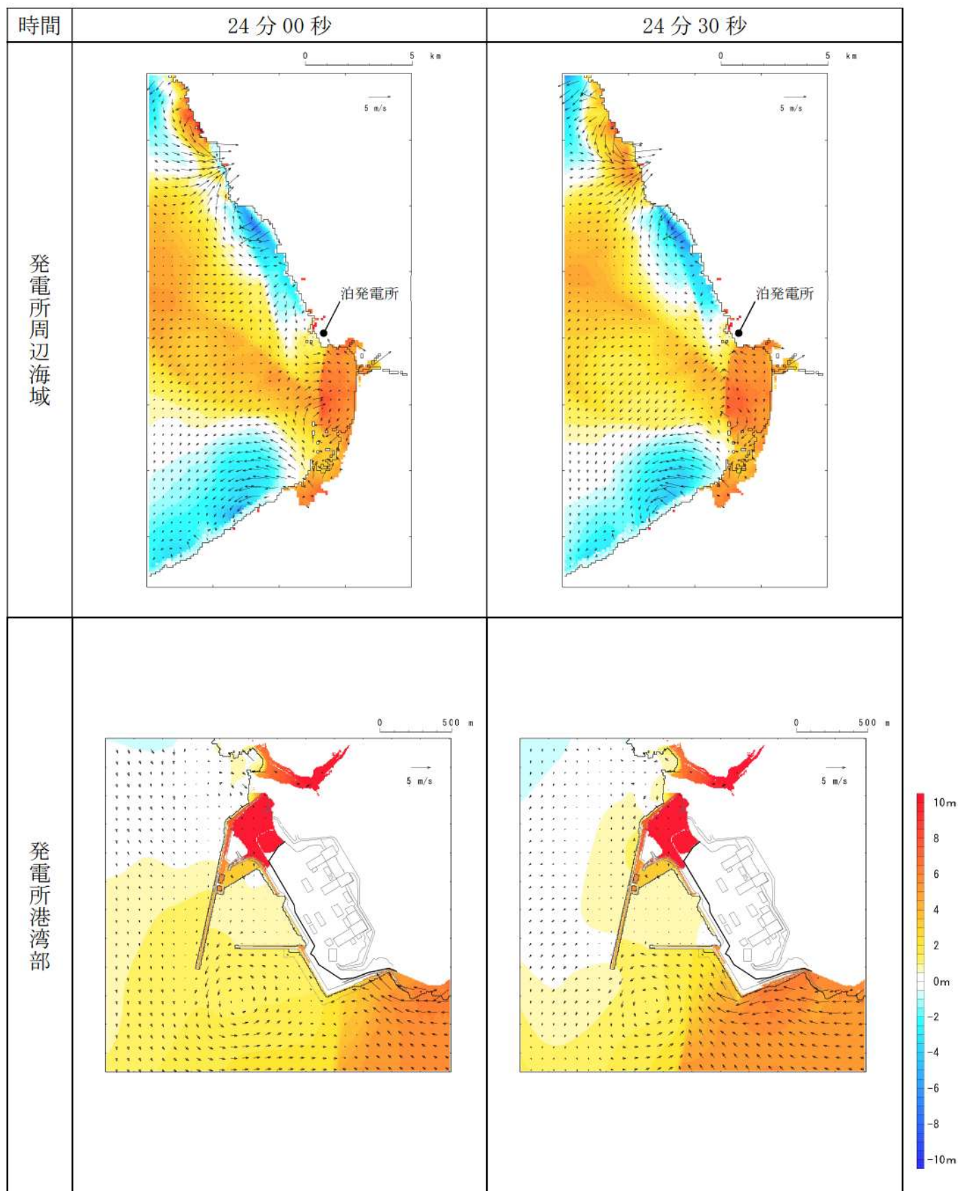
第 15 図-14 基準津波（波源 I，防波堤損傷なし）の水位変動・流向ベクトル(14/50)
