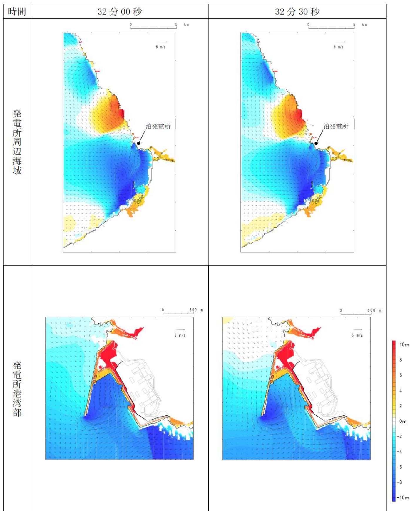
第 17 図-25 基準津波（波源K，南防波堤損傷）の水位変動・流向ベクトル(25/53)
