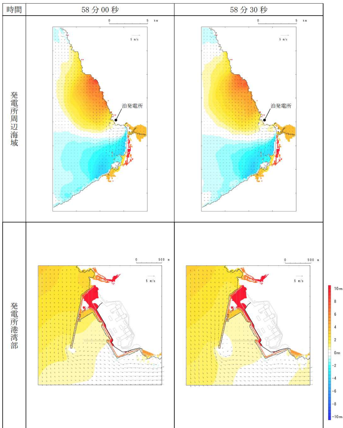
第 17 図-51 基準津波（波源K，南防波堤損傷）の水位変動・流向ベクトル(51/53)
