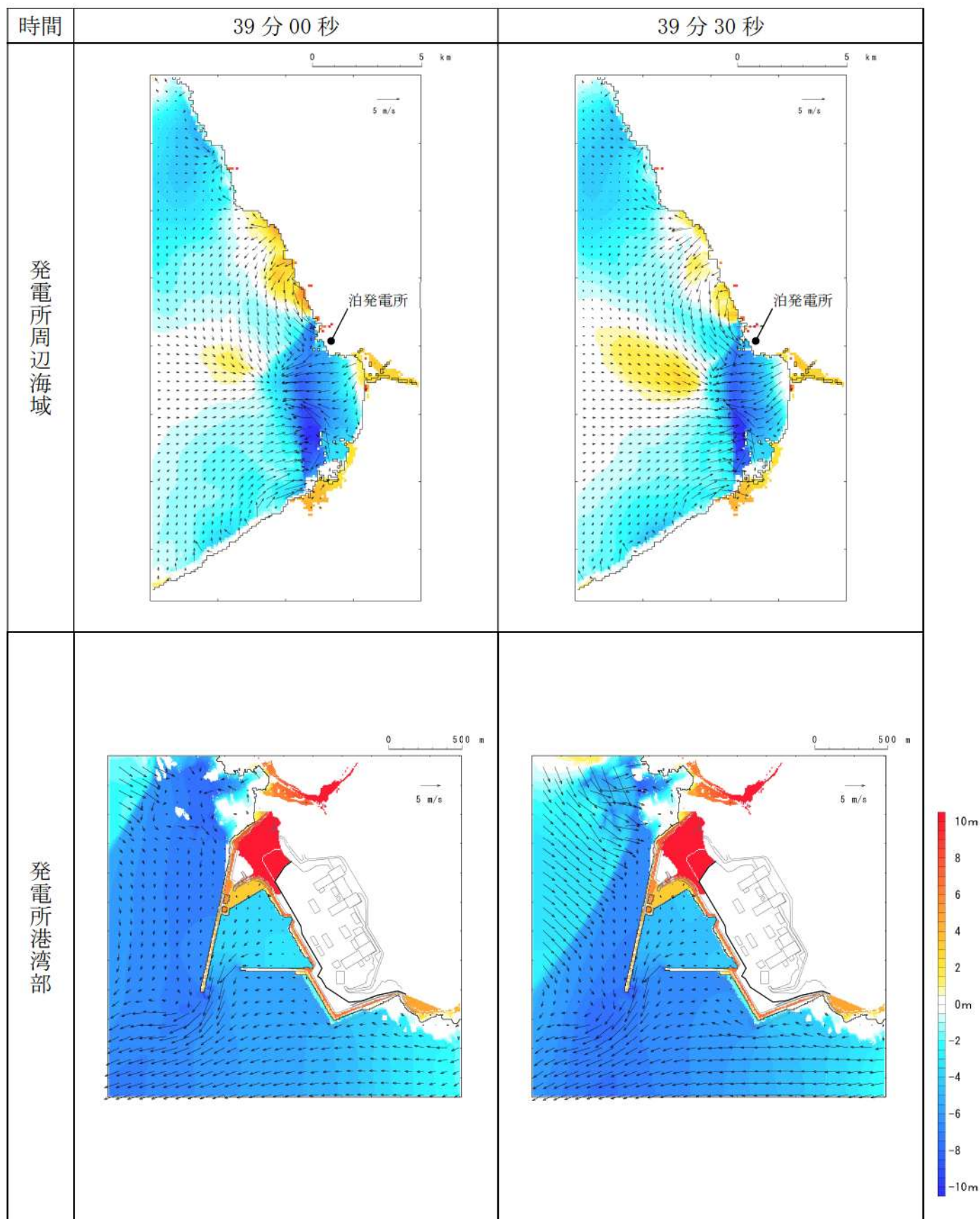
第 15 図-29 基準津波（波源 I，防波堤損傷なし）の水位変動・流向ベクトル(29/50)
