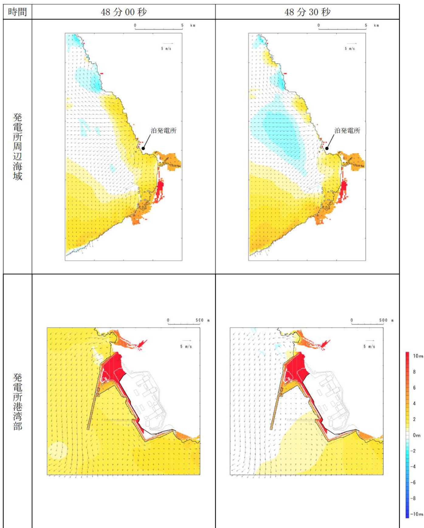
第 13 図-41 基準津波（波源 G，南防波堤損傷）の水位変動・流向ベクトル(41/53)
