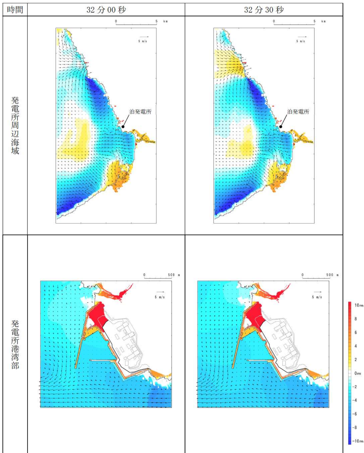
第 15 図-22 基準津波（波源 I，防波堤損傷なし）の水位変動・流向ベクトル(22/50)
