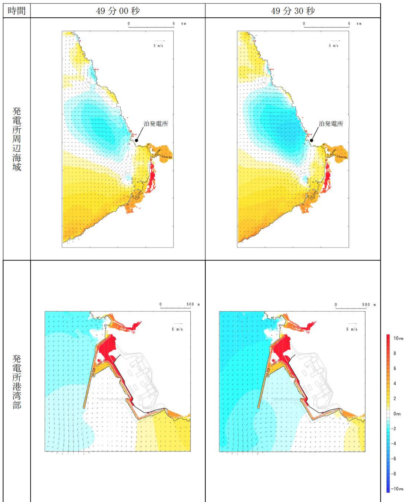
第 17 図-42 基準津波（波源K，南防波堤損傷）の水位変動・流向ベクトル(42/53)
