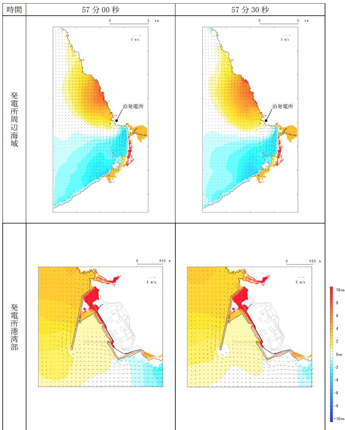
第 17 図-50 基準津波（波源K，南防波堤損傷）の水位変動・流向ベクトル(50/53)
