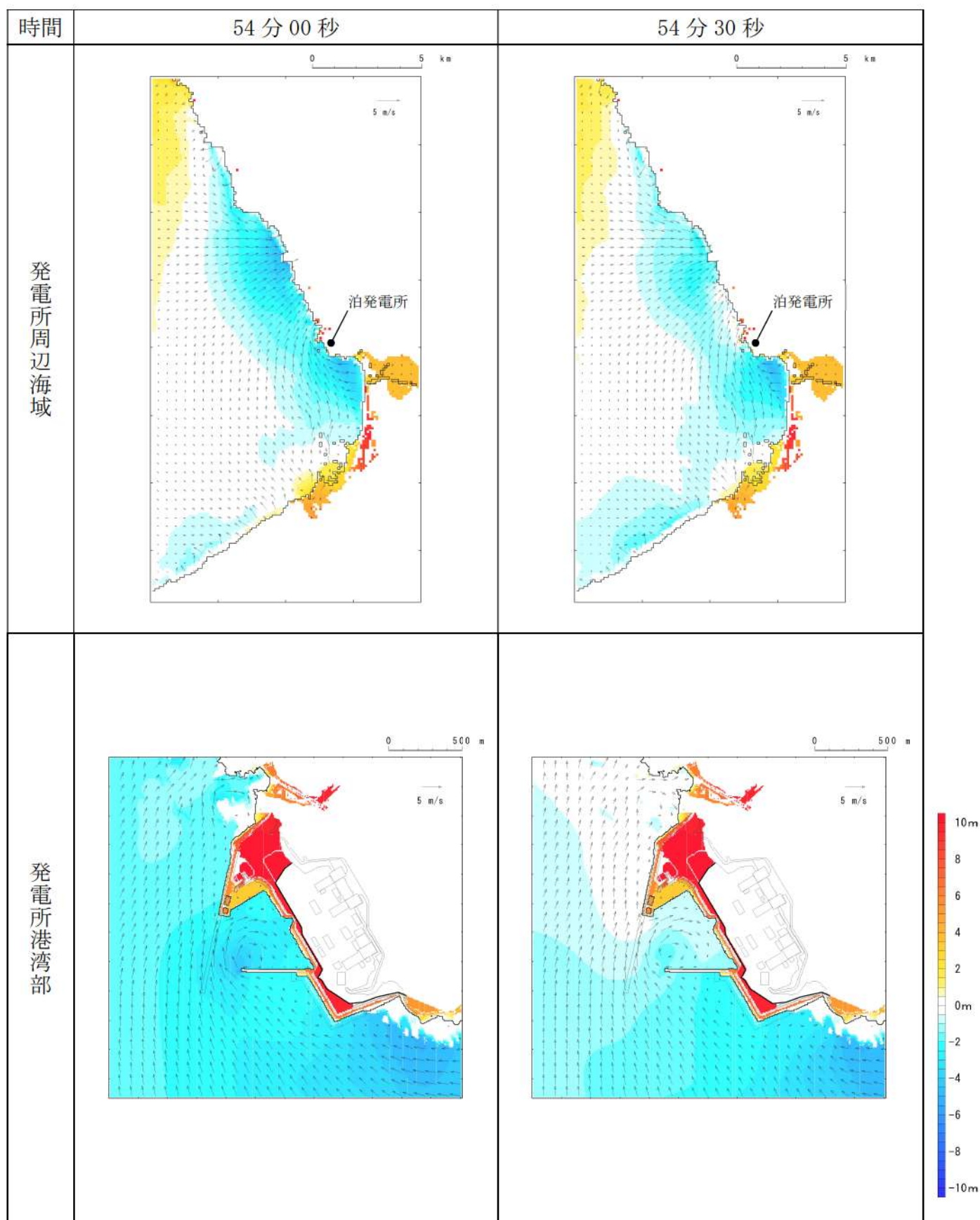
第 14 図-47 基準津波（波源H，北防波堤損傷）の水位変動・流向ベクトル(47/53)
