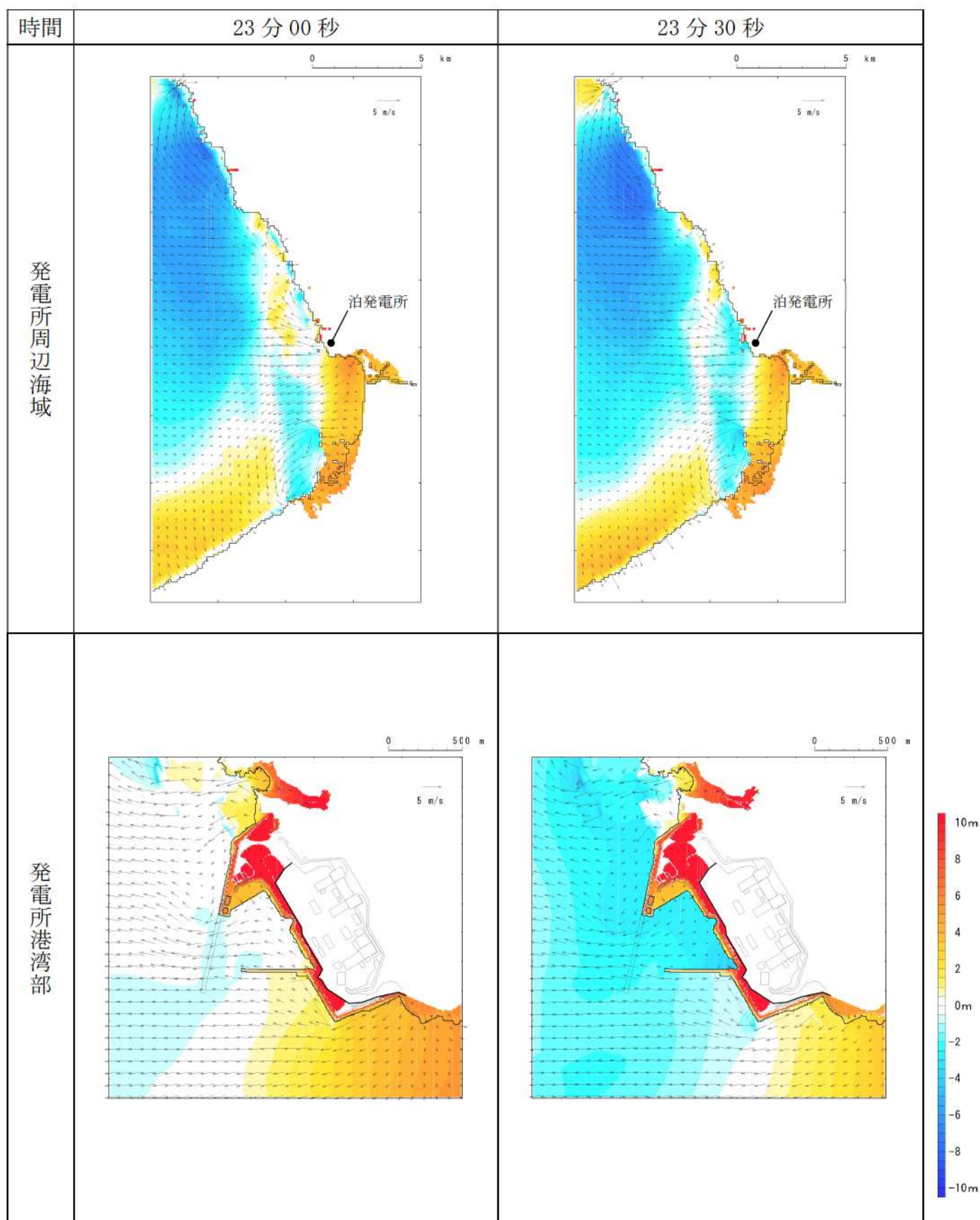
第 14 図-16 基準津波（波源H，北防波堤損傷）の水位変動・流向ベクトル(16/53)
