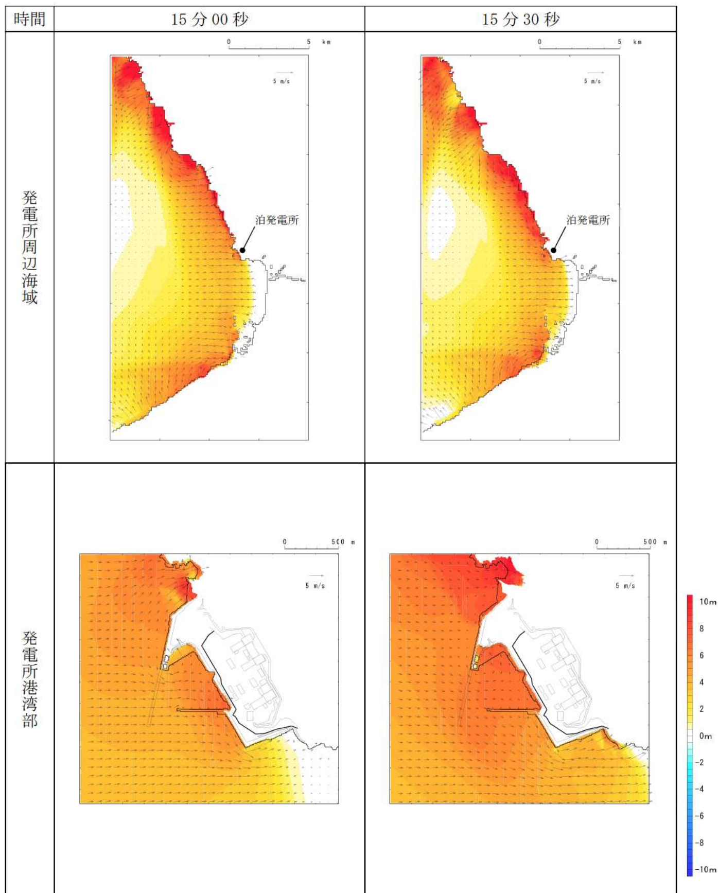
第 14 図-8 基準津波（波源H，北防波堤損傷）の水位変動・流向ベクトル(8/53)
