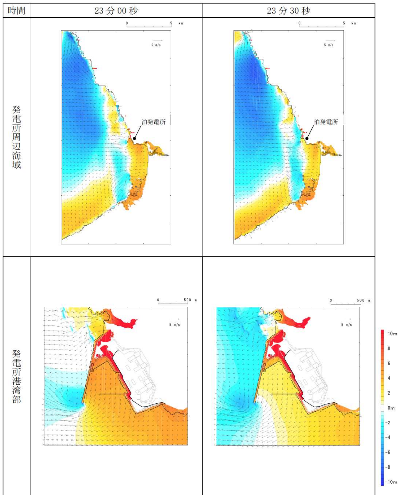
第 17 図-16 基準津波（波源K，南防波堤損傷）の水位変動・流向ベクトル(16/53)
