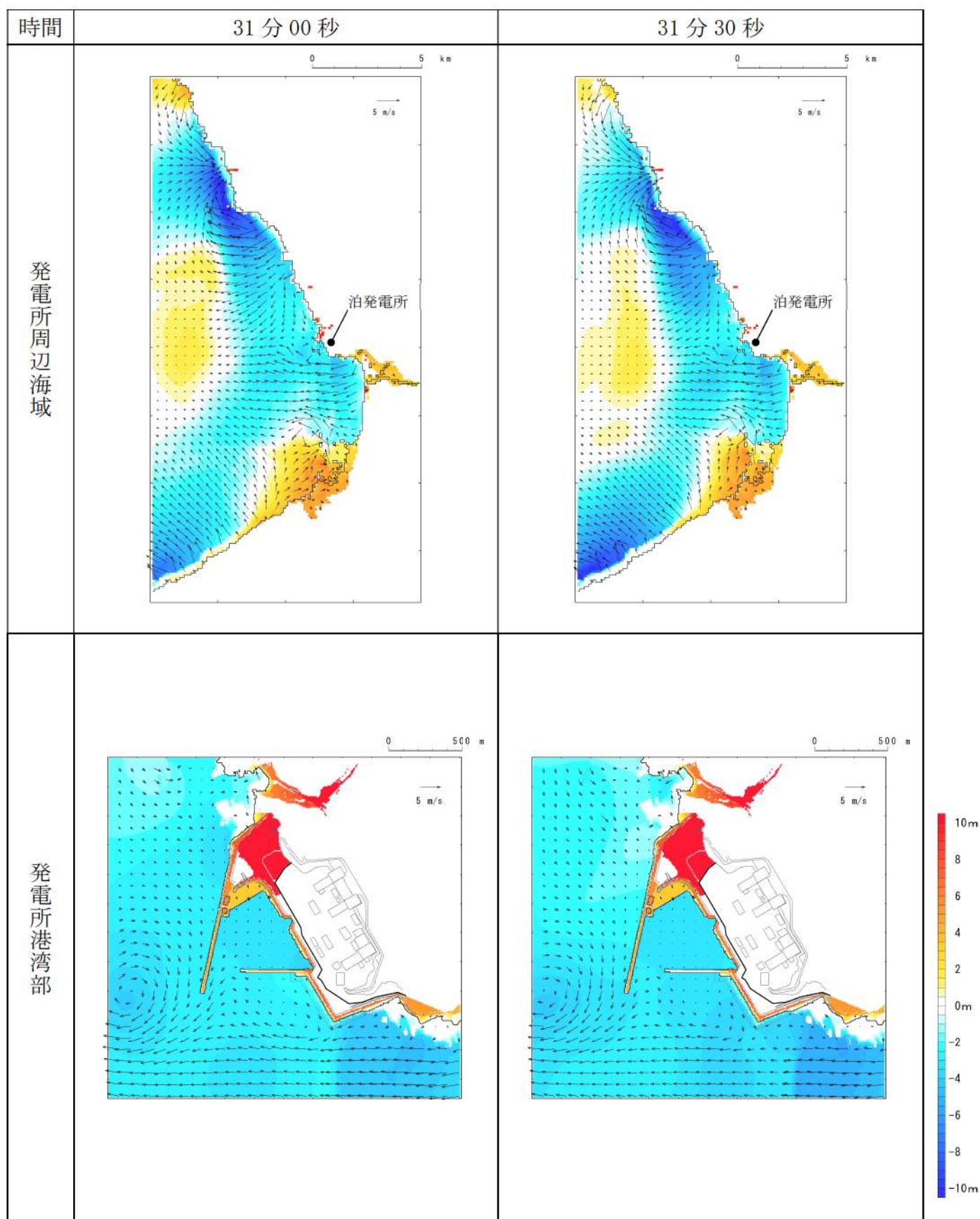
第 15 図-21 基準津波（波源 I，防波堤損傷なし）の水位変動・流向ベクトル(21/50)
