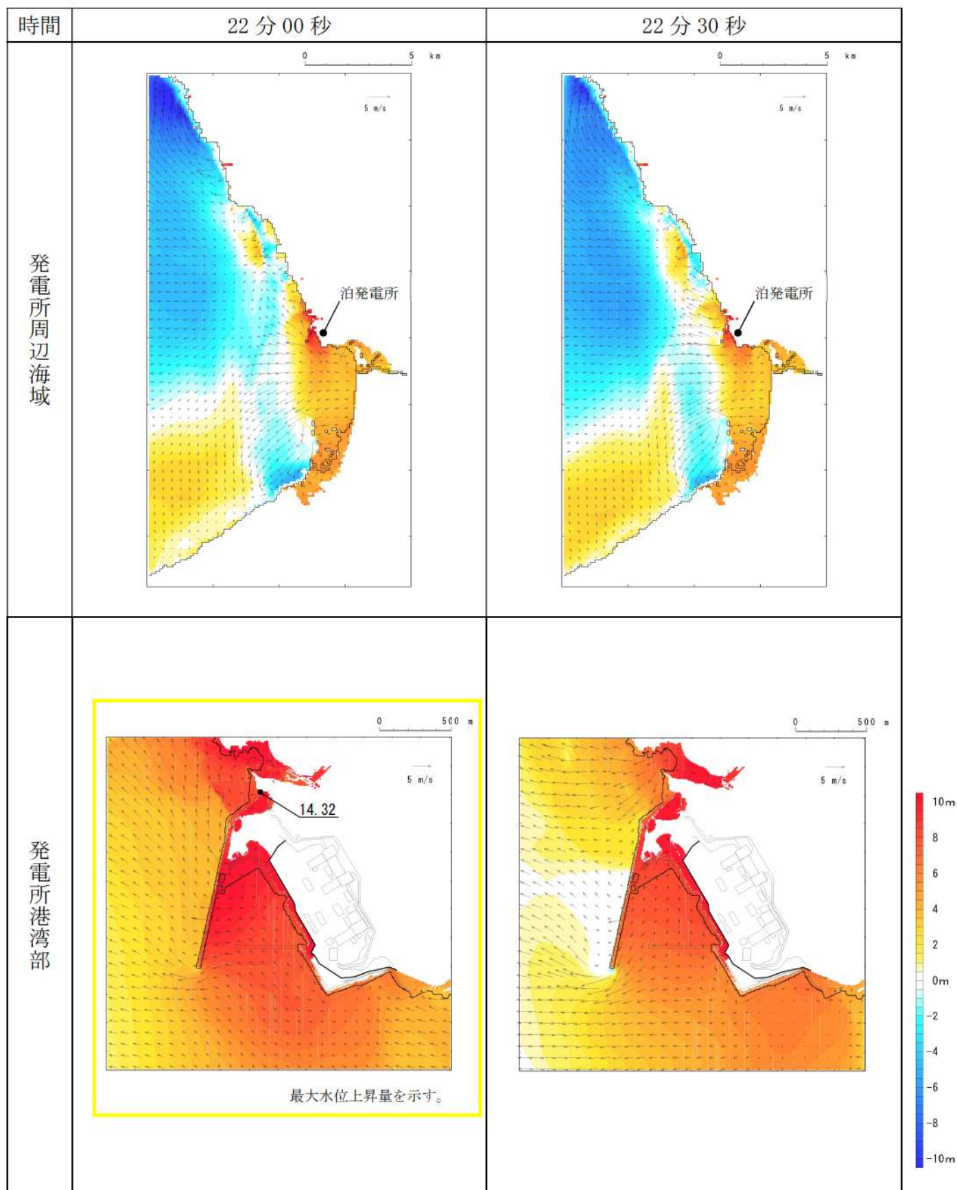
第 17 図-15 基準津波（波源K，南防波堤損傷）の水位変動・流向ベクトル(15/53)
