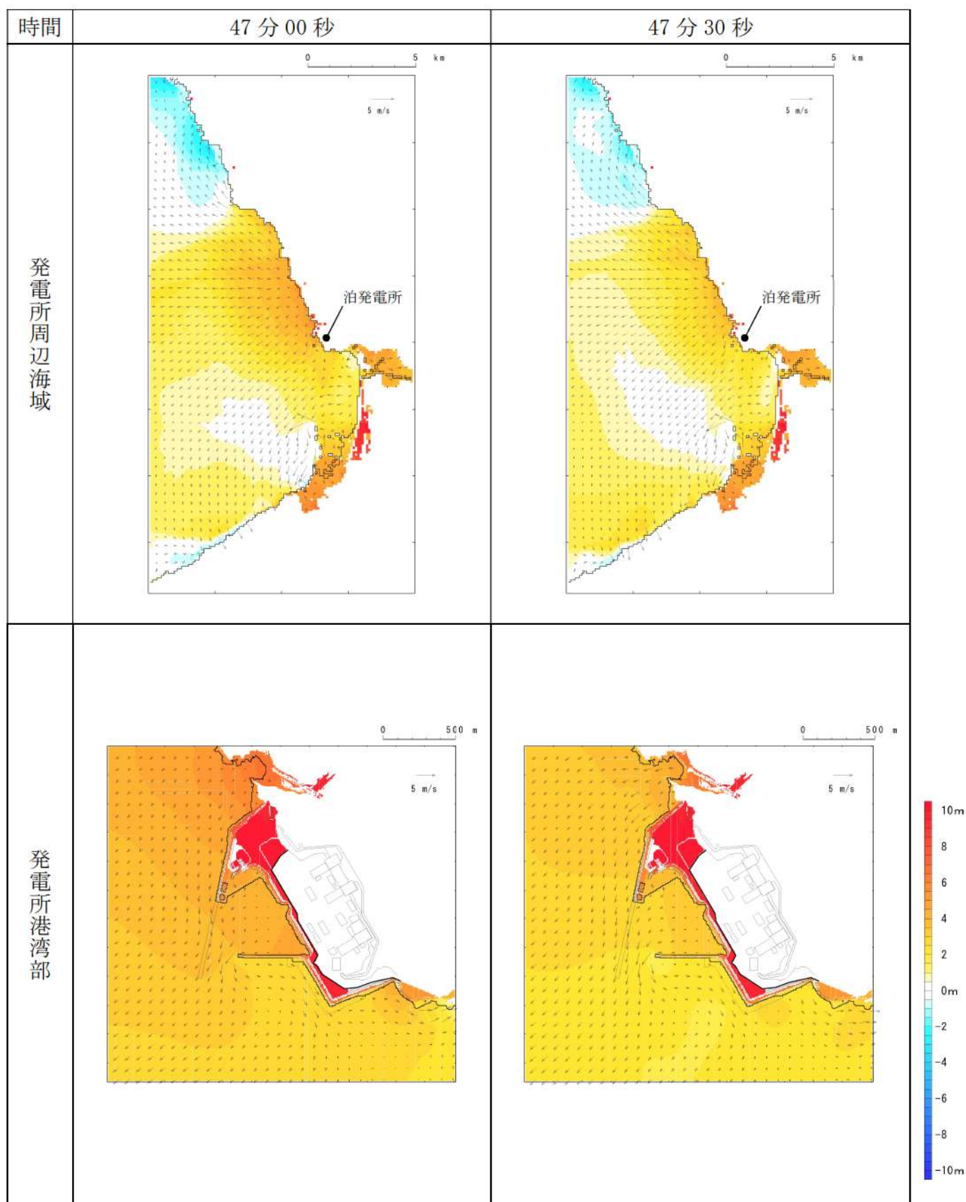
第 14 図-40 基準津波（波源H，北防波堤損傷）の水位変動・流向ベクトル(40/53)
