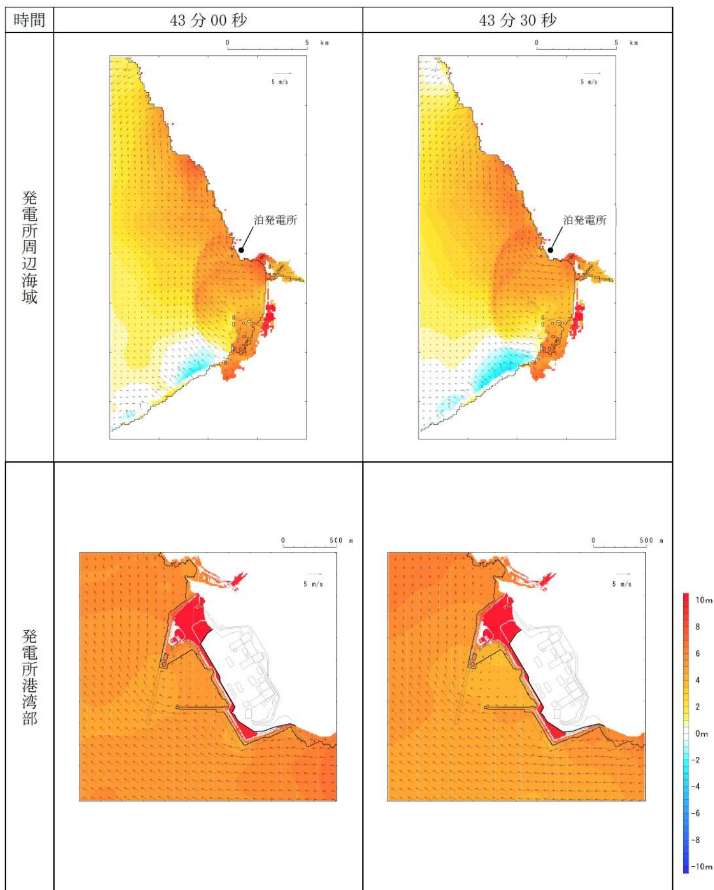
第 14 図-36 基準津波（波源H，北防波堤損傷）の水位変動・流向ベクトル(36/53)
