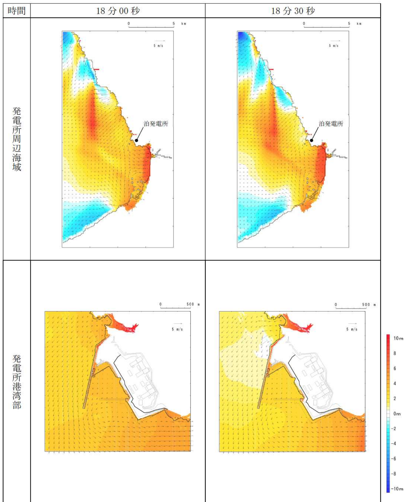
第 17 図-11 基準津波（波源K，南防波堤損傷）の水位変動・流向ベクトル(11/53)
