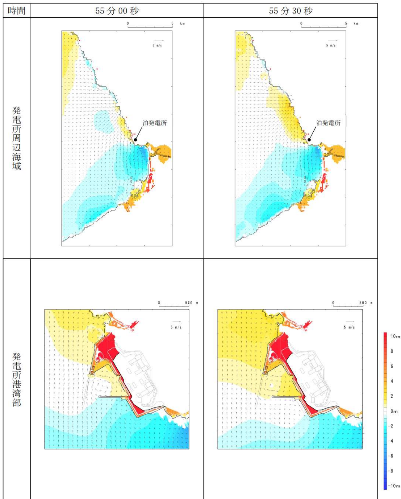
第 14 図-48 基準津波（波源H，北防波堤損傷）の水位変動・流向ベクトル(48/53)
