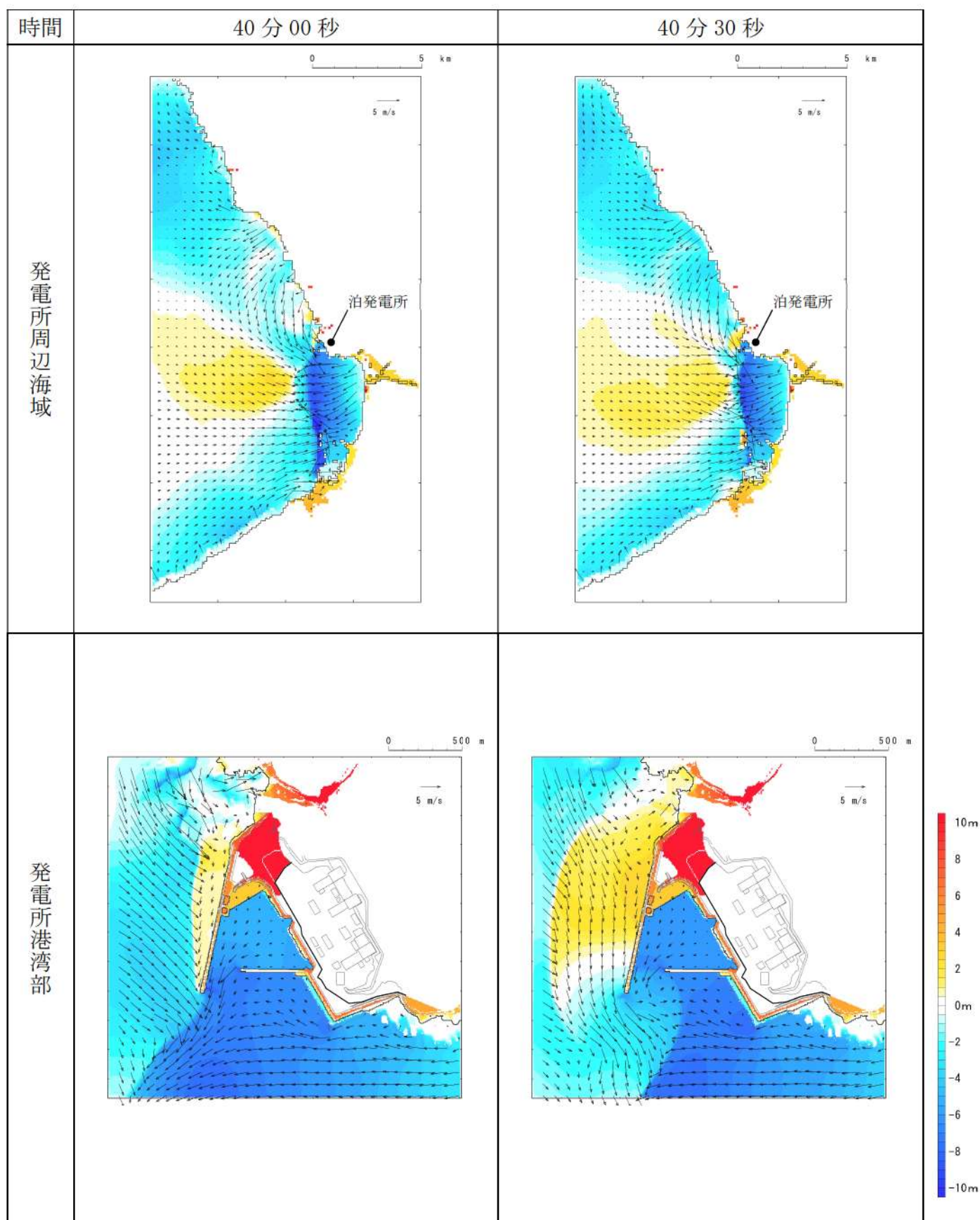
第 15 図-30 基準津波（波源 I，防波堤損傷なし）の水位変動・流向ベクトル(30/50)
