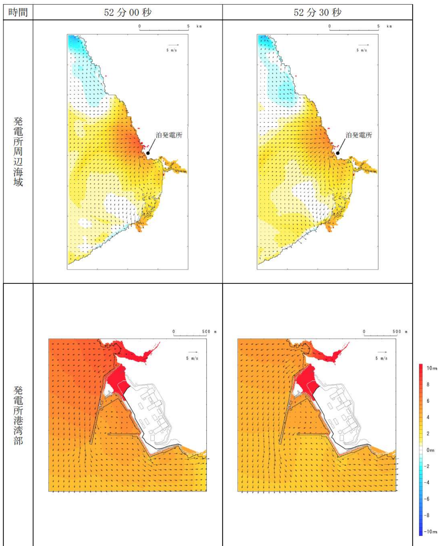
第 15 図-42 基準津波（波源 I，防波堤損傷なし）の水位変動・流向ベクトル(42/50)
