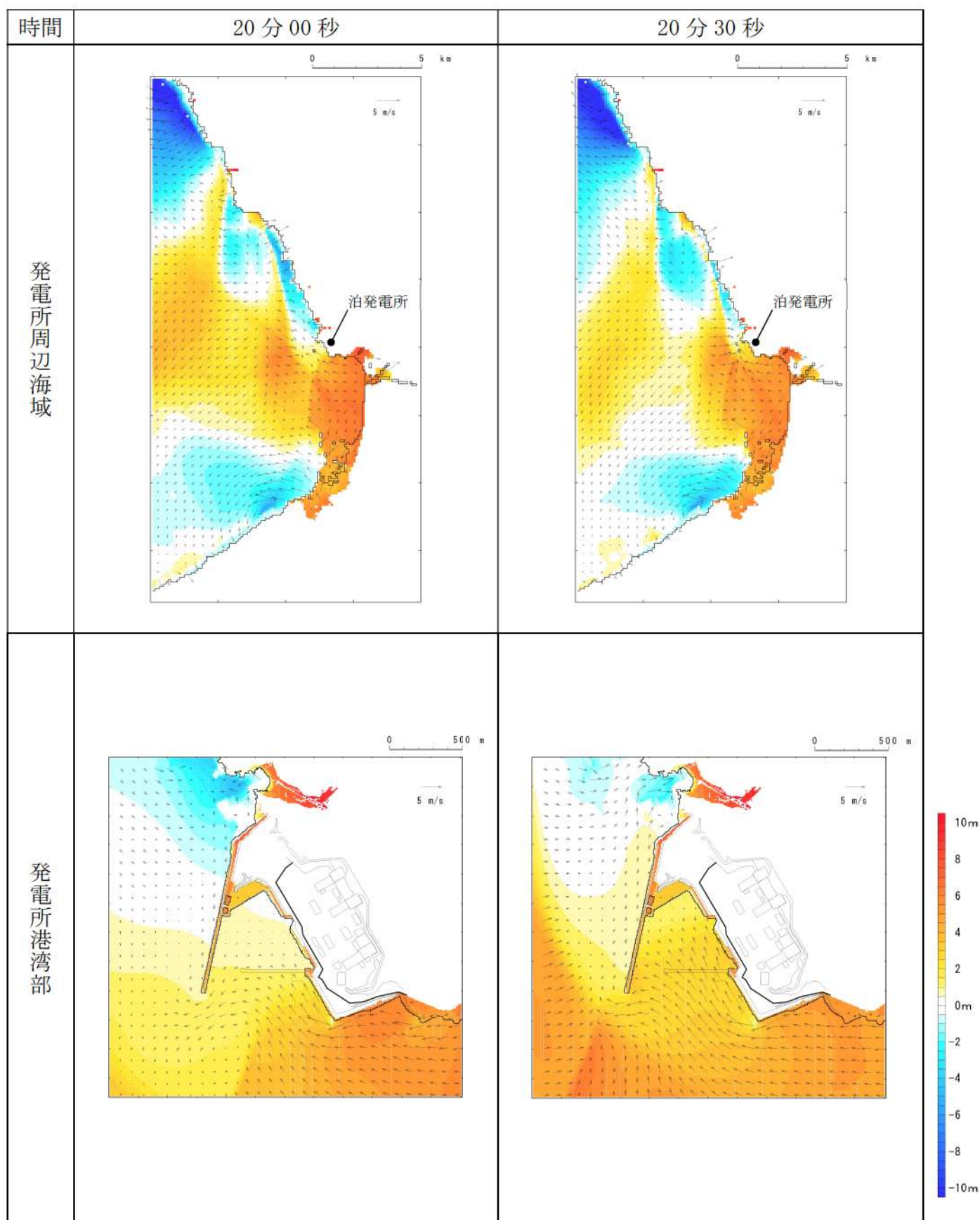
第 17 図-13 基準津波（波源K，南防波堤損傷）の水位変動・流向ベクトル(13/53)
