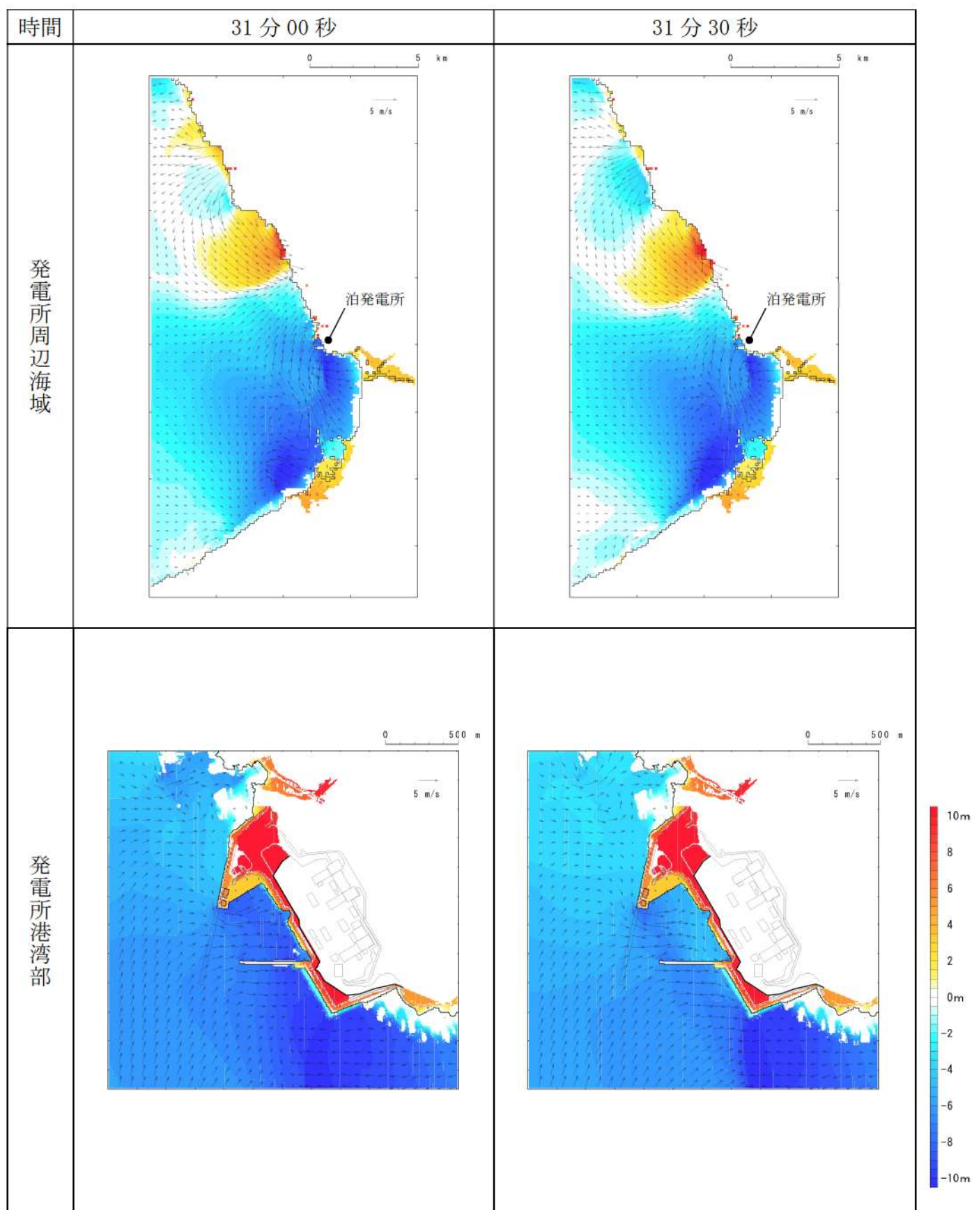
第 14 図-24 基準津波（波源H，北防波堤損傷）の水位変動・流向ベクトル(24/53)
