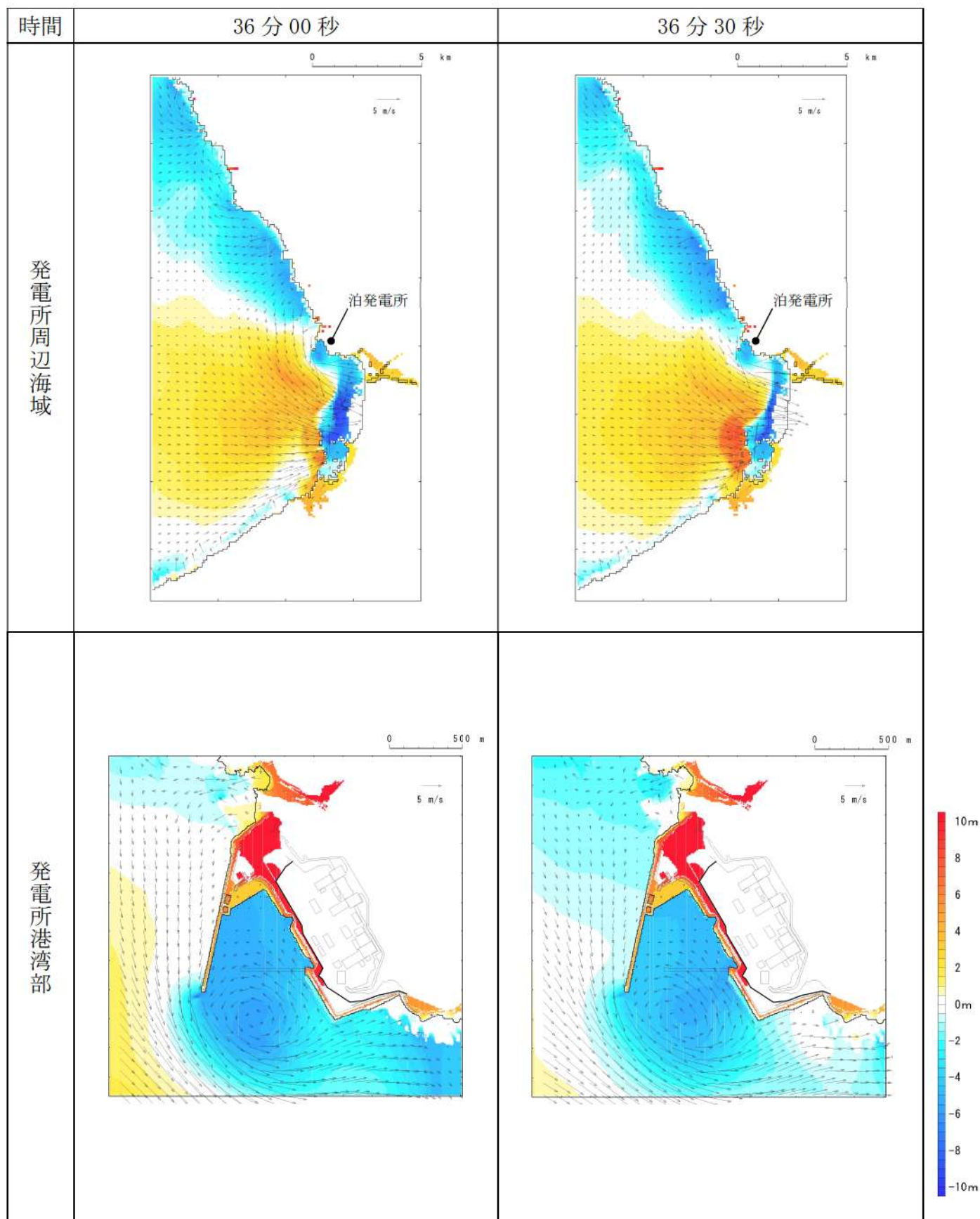
第 17 図-29 基準津波（波源K，南防波堤損傷）の水位変動・流向ベクトル(29/53)
