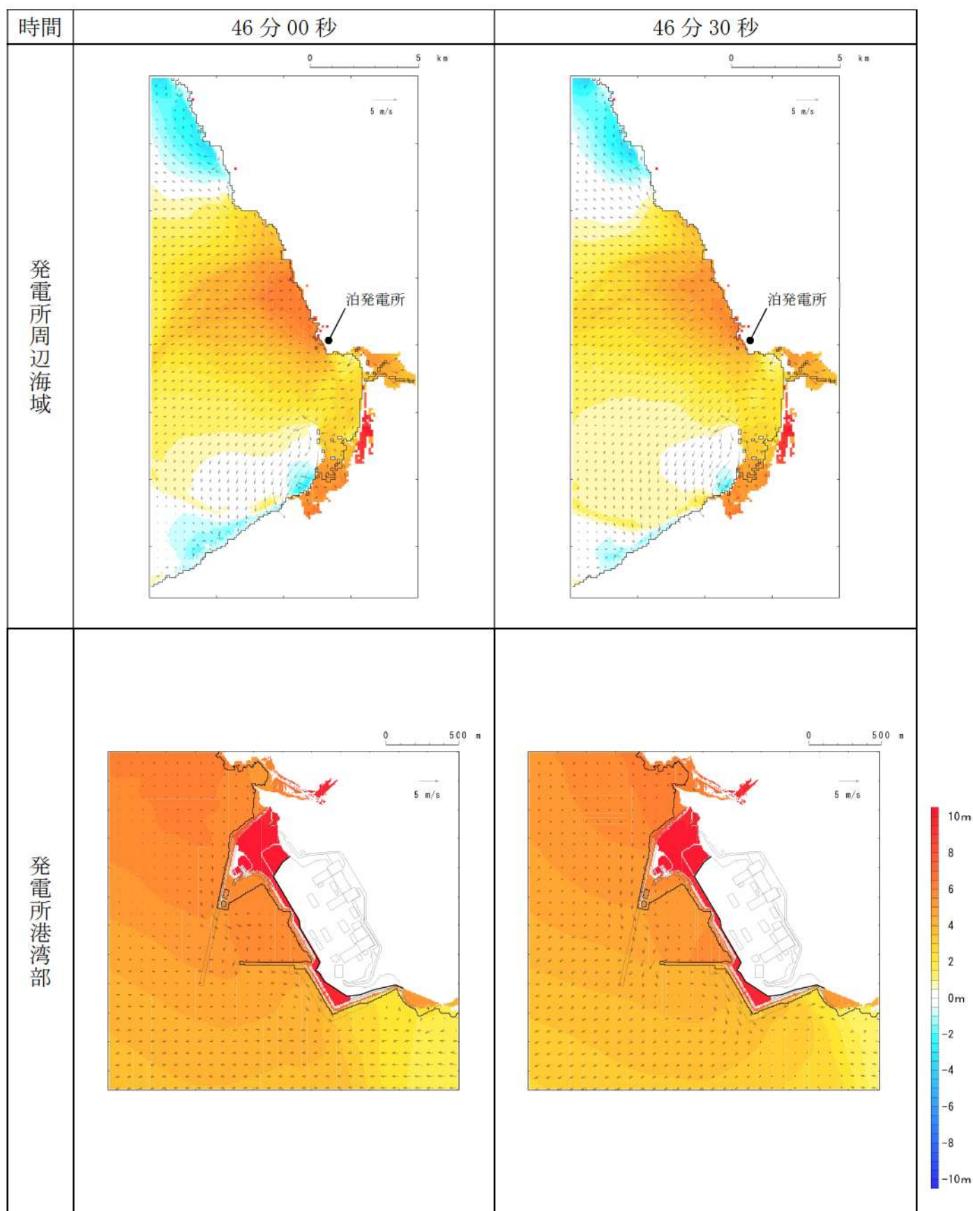
第 14 図-39 基準津波（波源H，北防波堤損傷）の水位変動・流向ベクトル(39/53)
