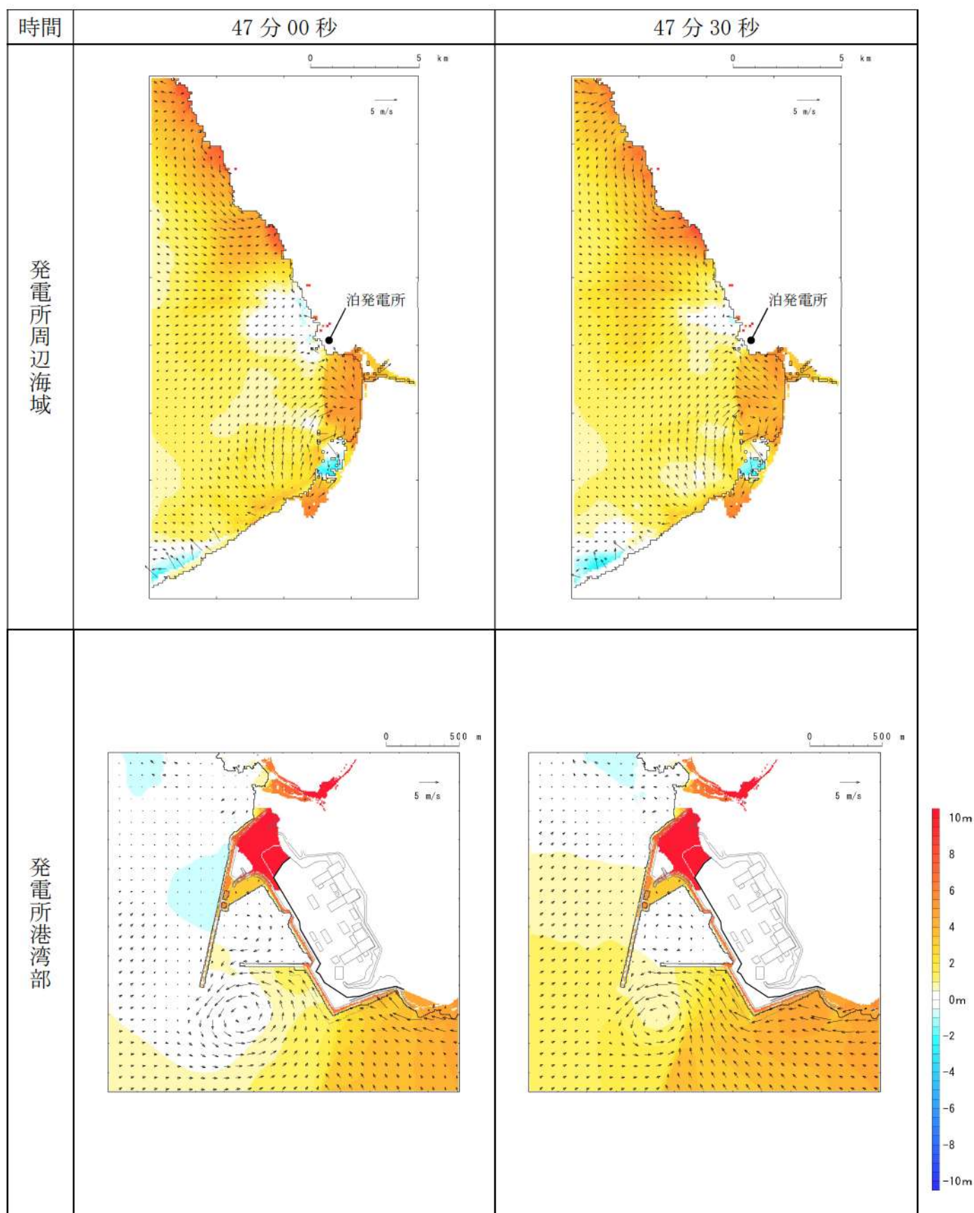
第 15 図-37 基準津波（波源 I，防波堤損傷なし）の水位変動・流向ベクトル(37/50)
