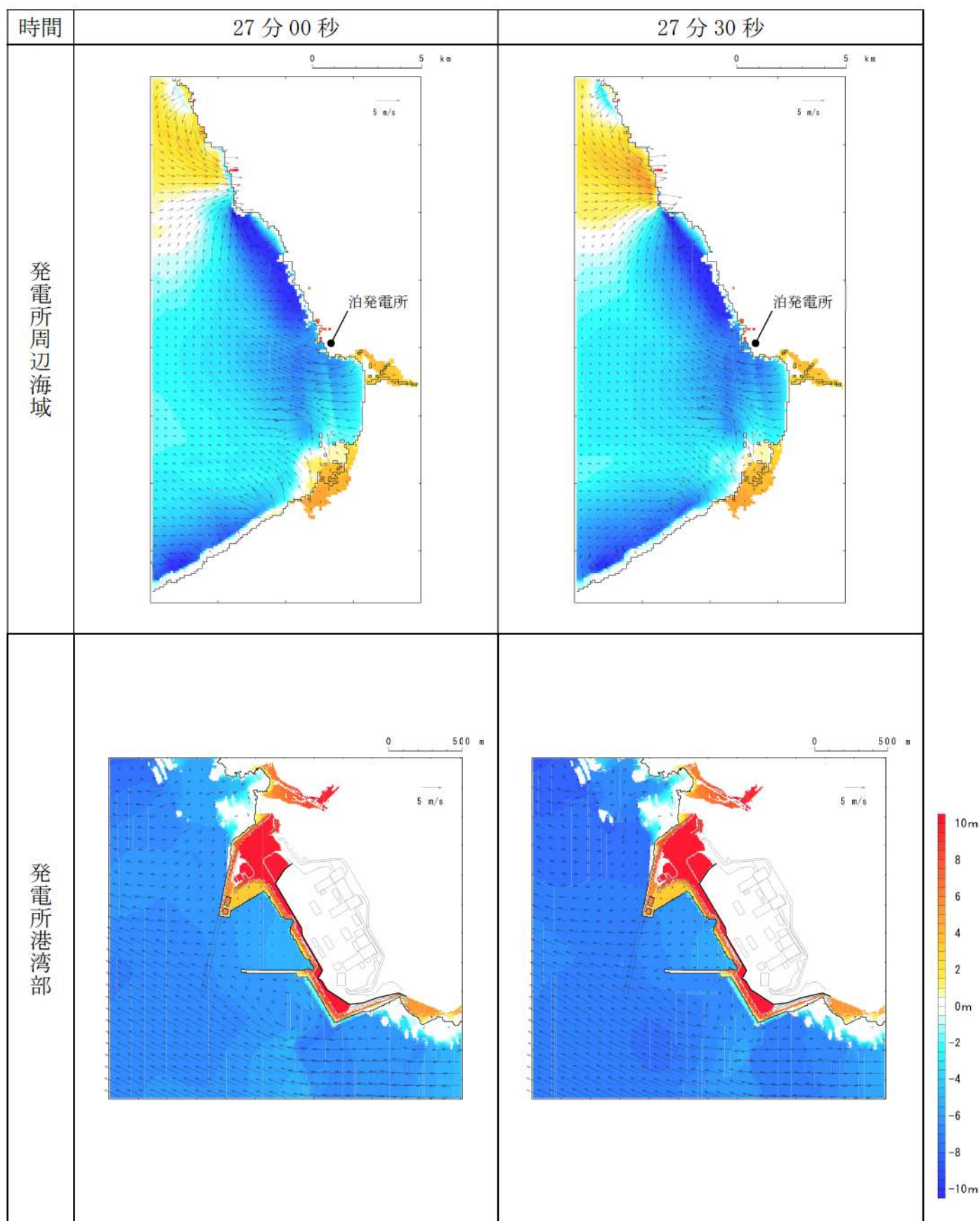
第 14 図-20 基準津波（波源H，北防波堤損傷）の水位変動・流向ベクトル(20/53)
