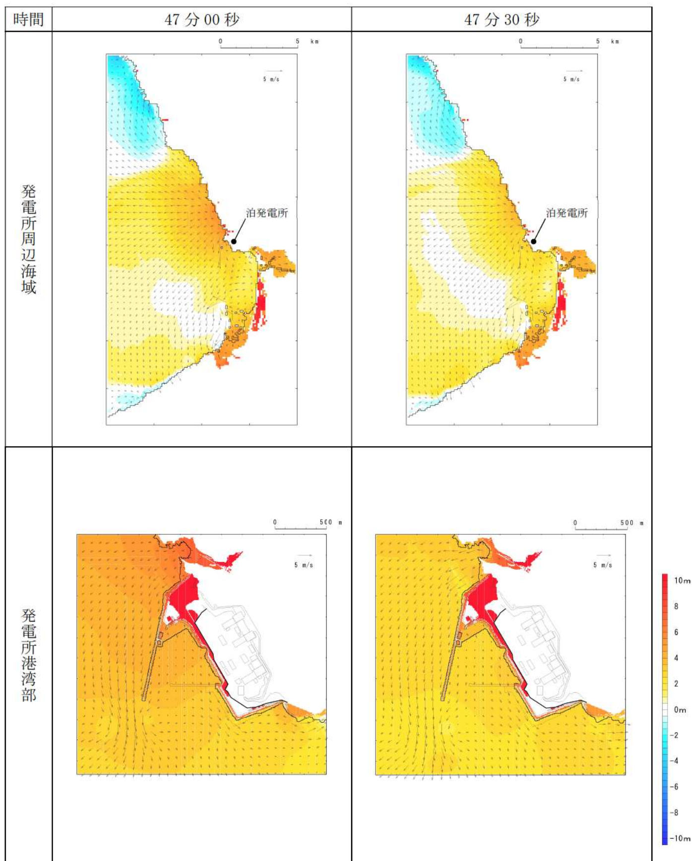
第 17 図-40 基準津波（波源K，南防波堤損傷）の水位変動・流向ベクトル(40/53)
