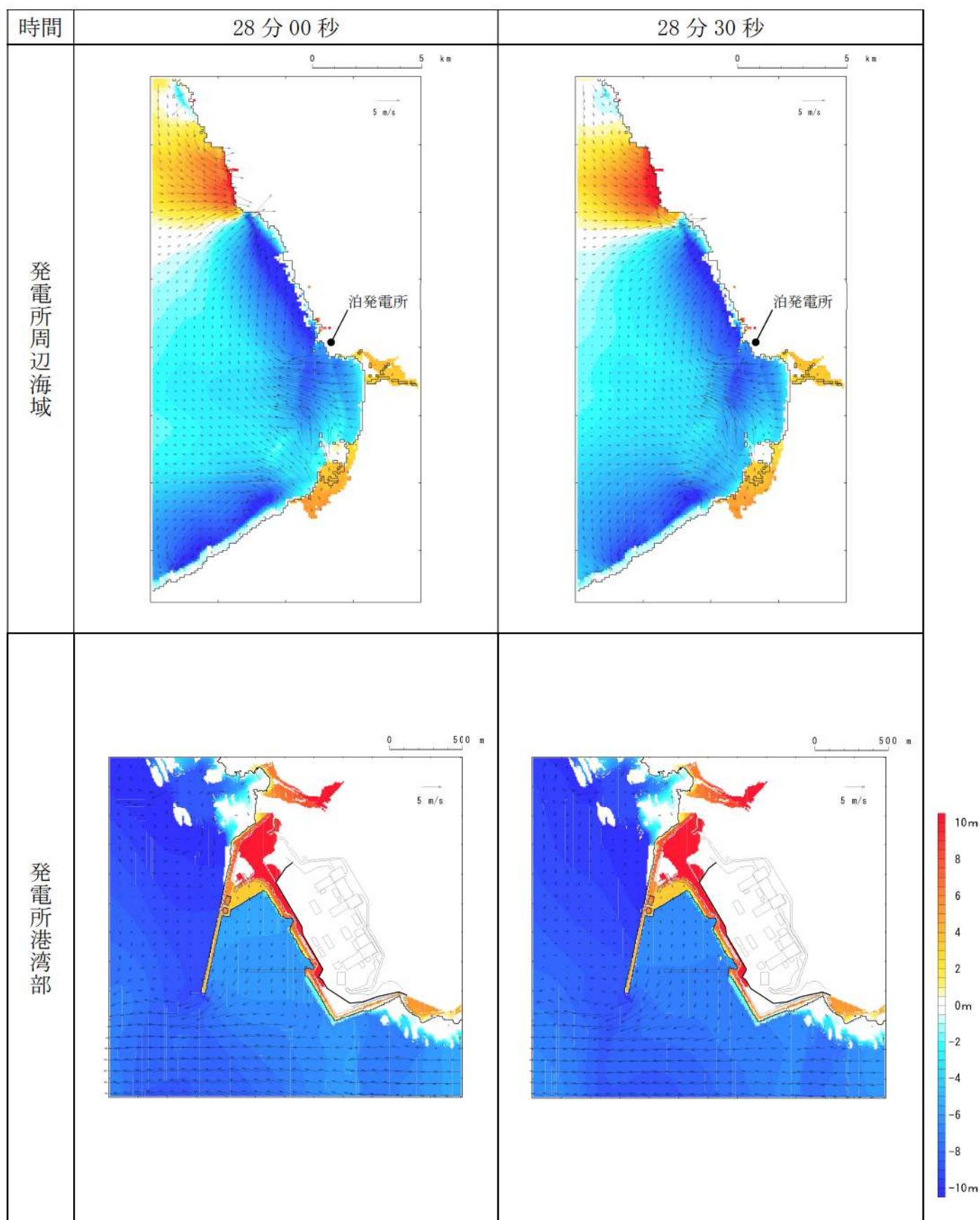
第 17 図-21 基準津波（波源K，南防波堤損傷）の水位変動・流向ベクトル(21/53)
