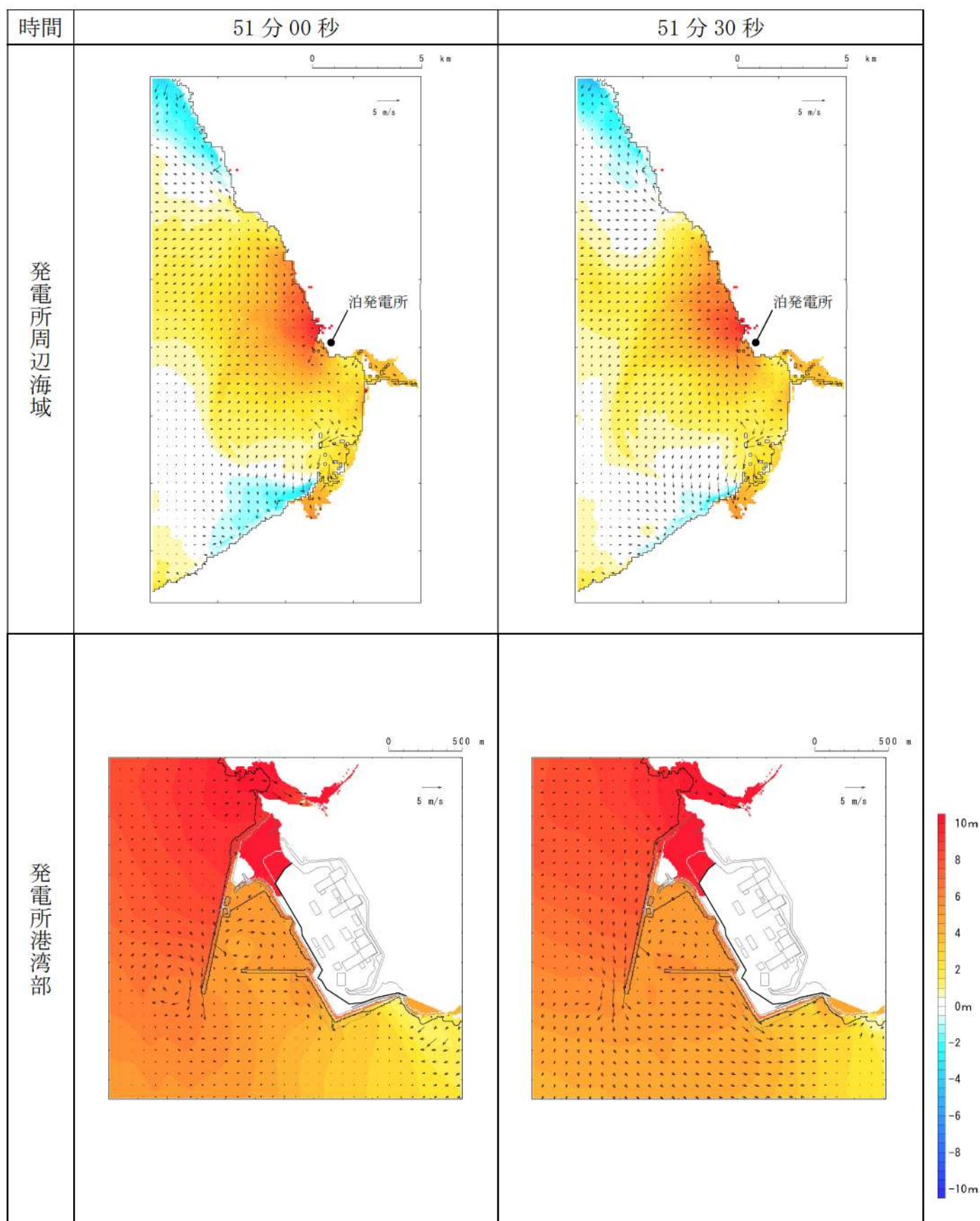
第 15 図-41 基準津波（波源 I，防波堤損傷なし）の水位変動・流向ベクトル(41/50)
