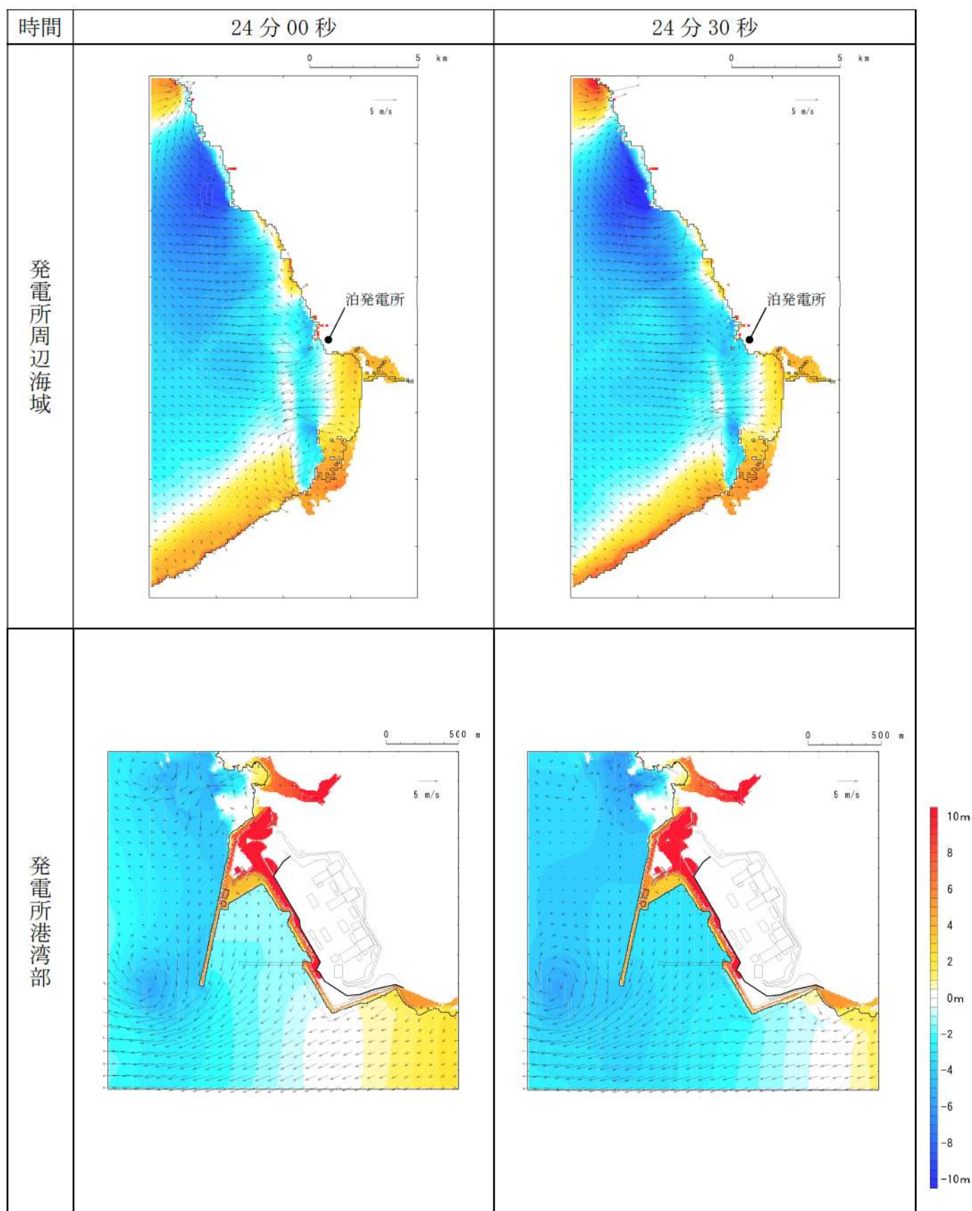
第 17 図-17 基準津波（波源K，南防波堤損傷）の水位変動・流向ベクトル(17/53)
