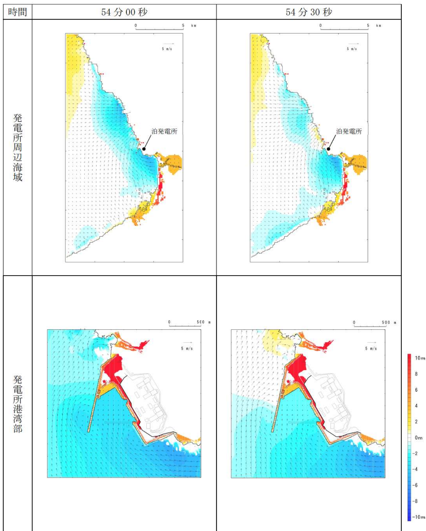
第 17 図-47 基準津波（波源K，南防波堤損傷）の水位変動・流向ベクトル(47/53)
