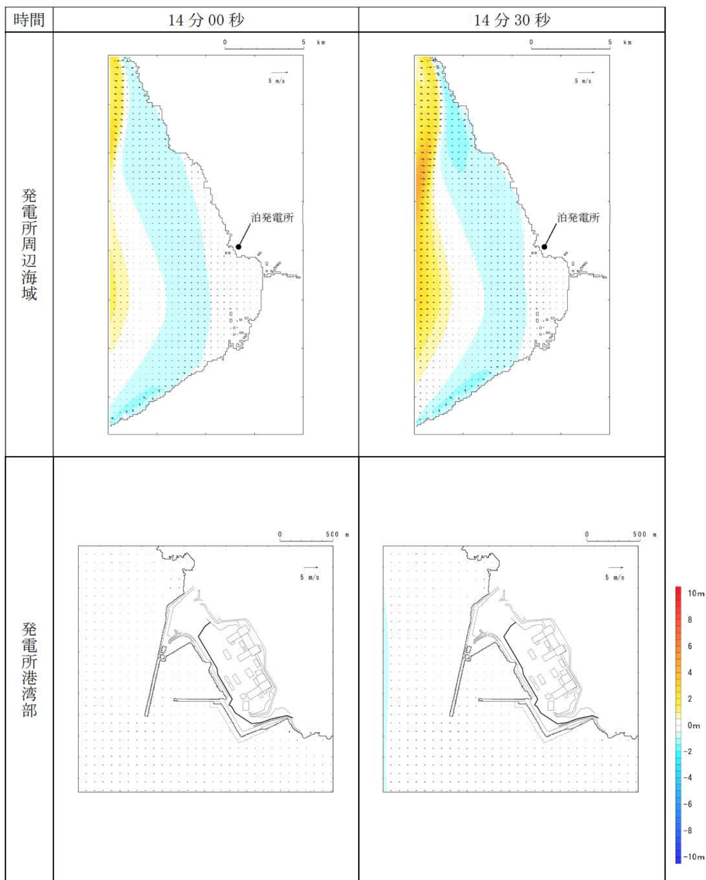
第 15 図-4 基準津波（波源 I，防波堤損傷なし）の水位変動・流向ベクトル(4/50)
