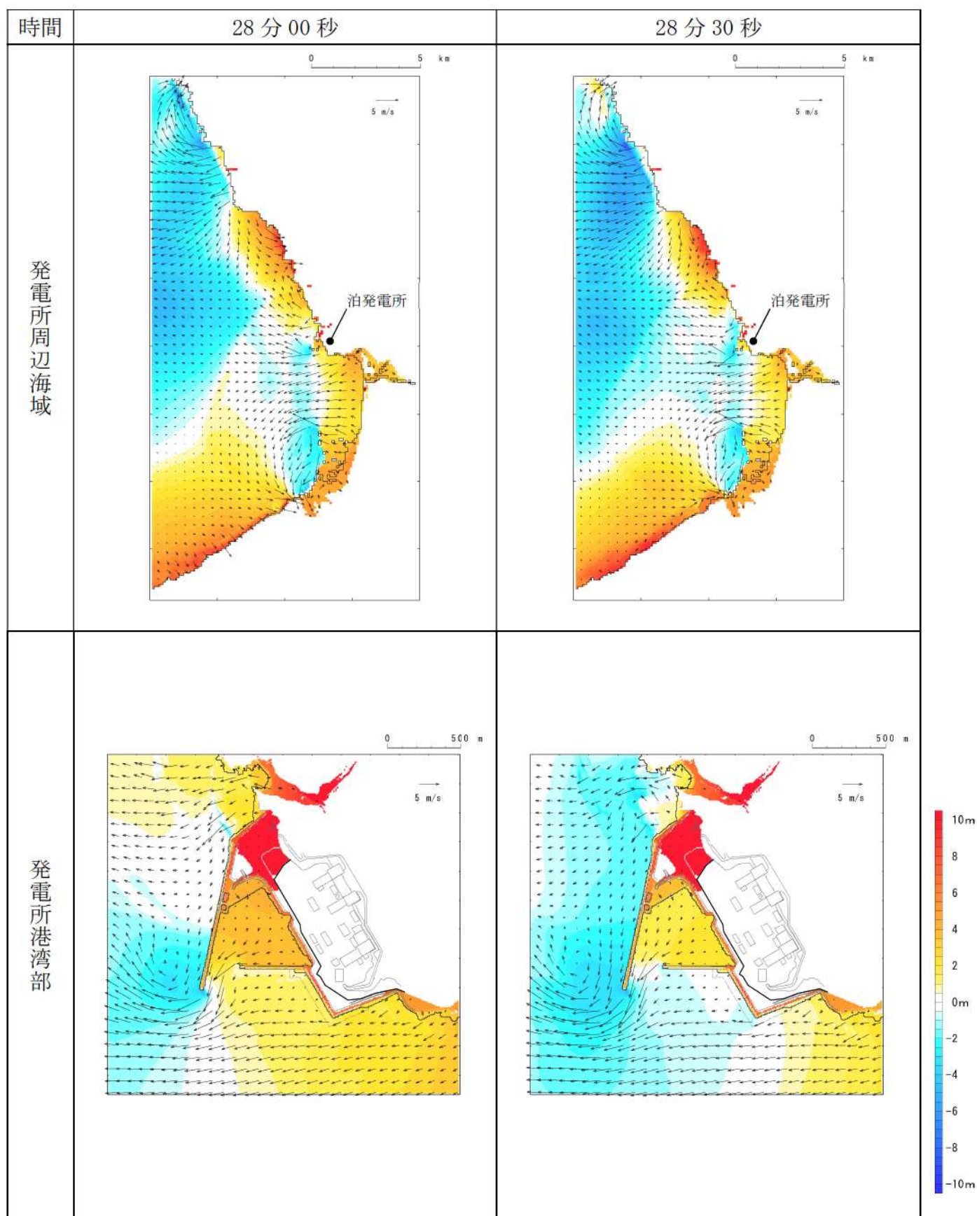
第 15 図-18 基準津波（波源 I，防波堤損傷なし）の水位変動・流向ベクトル(18/50)
