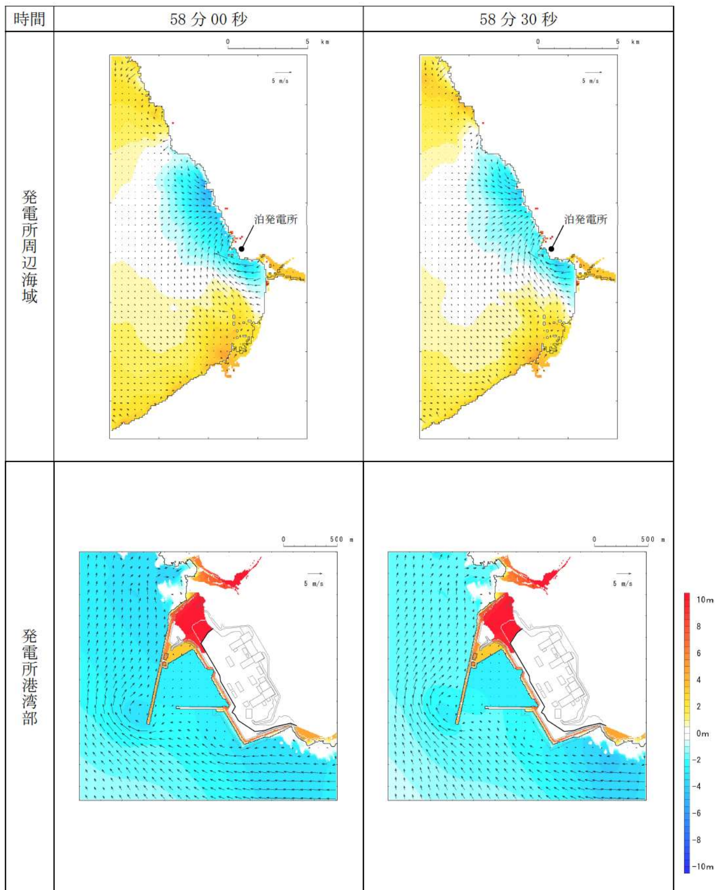
第 15 図-48 基準津波（波源 I，防波堤損傷なし）の水位変動・流向ベクトル(48/50)
