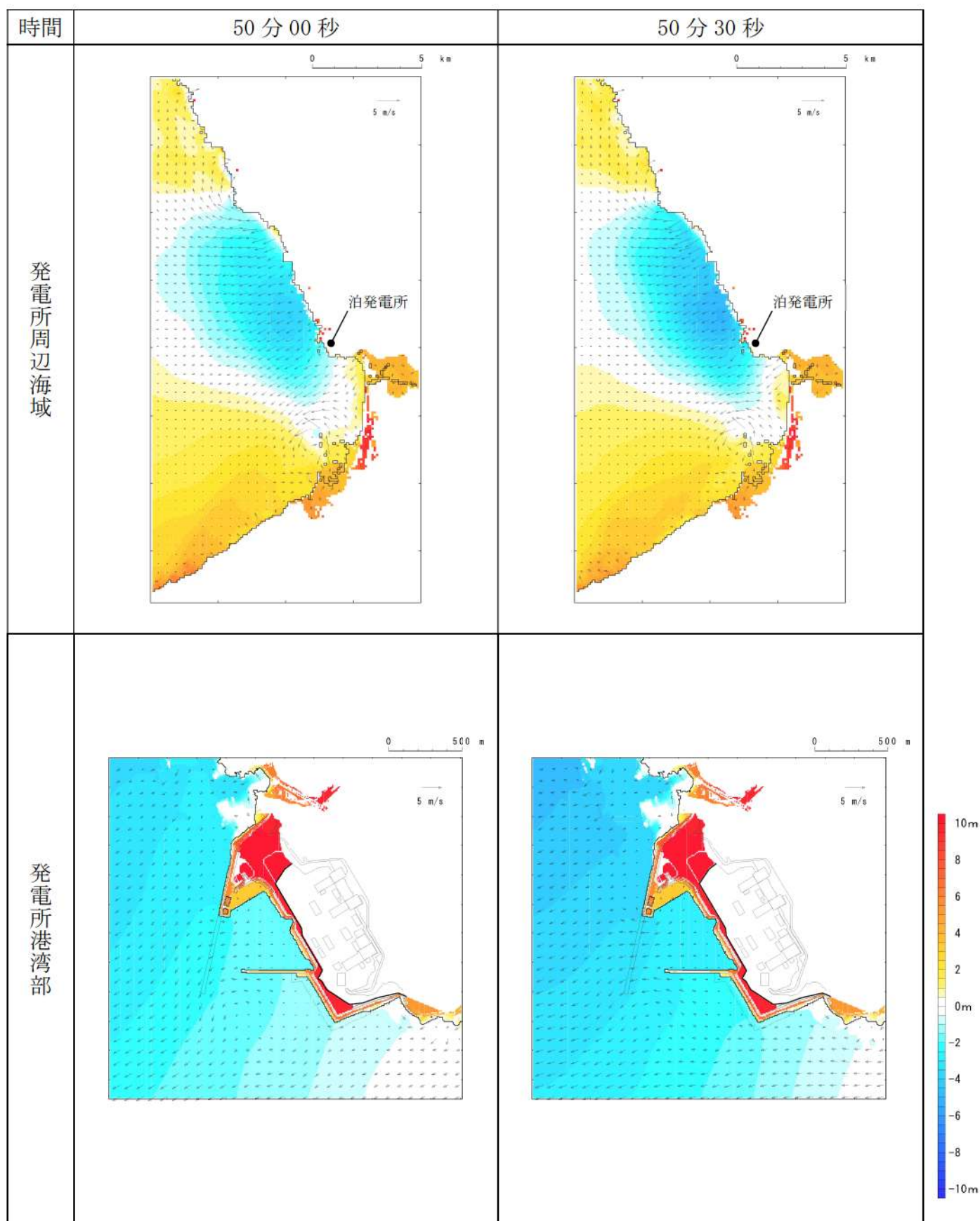
第 14 図-43 基準津波（波源H，北防波堤損傷）の水位変動・流向ベクトル(43/53)
