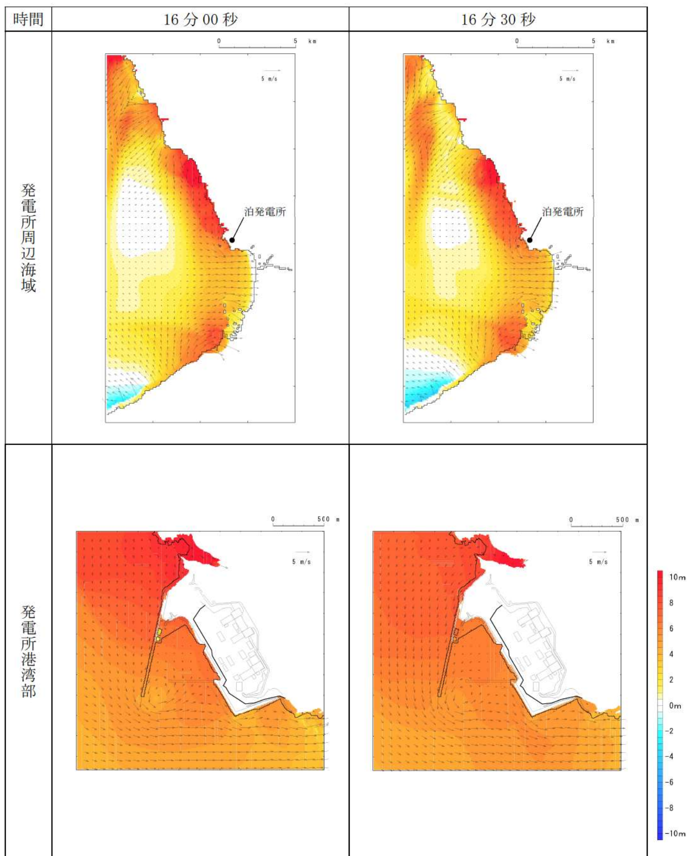
第 17 図-9 基準津波（波源K，南防波堤損傷）の水位変動・流向ベクトル(9/53)
