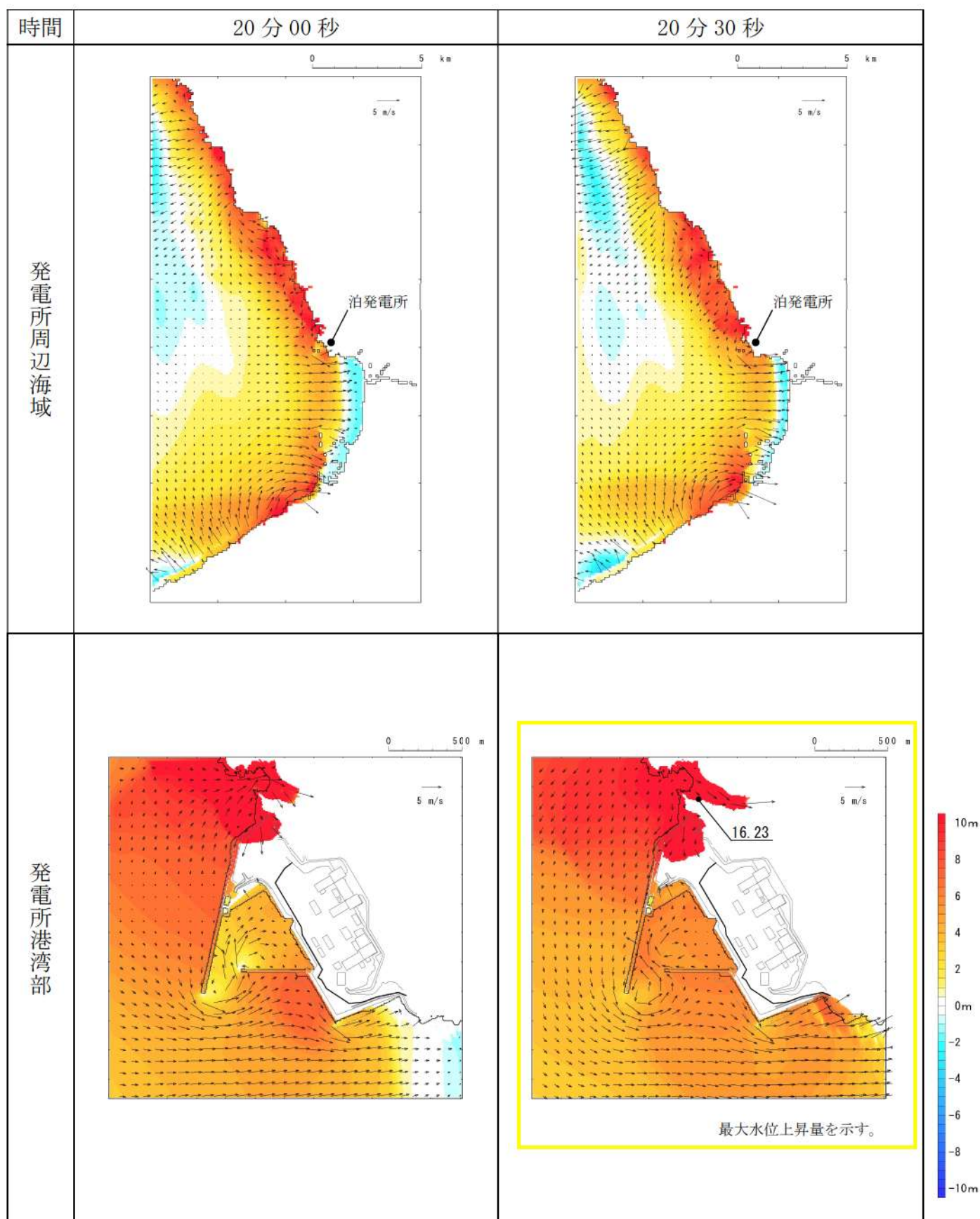
第 15 図-10 基準津波（波源 I，防波堤損傷なし）の水位変動・流向ベクトル(10/50)
