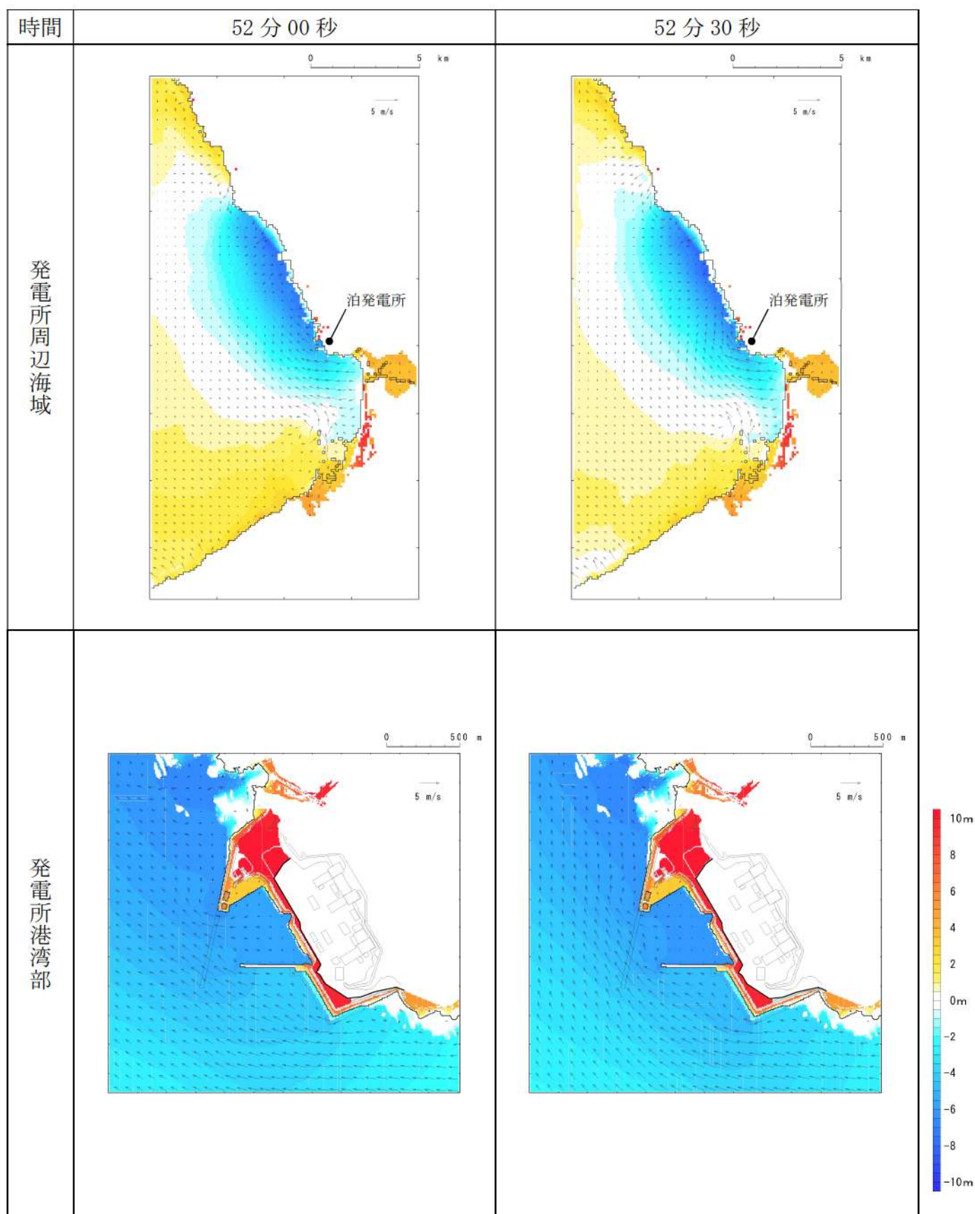
第 14 図-45 基準津波（波源H，北防波堤損傷）の水位変動・流向ベクトル(45/53)
