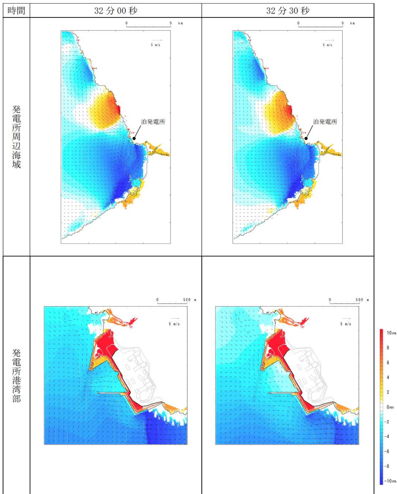
第 14 図-25 基準津波（波源H，北防波堤損傷）の水位変動・流向ベクトル(25/53)
