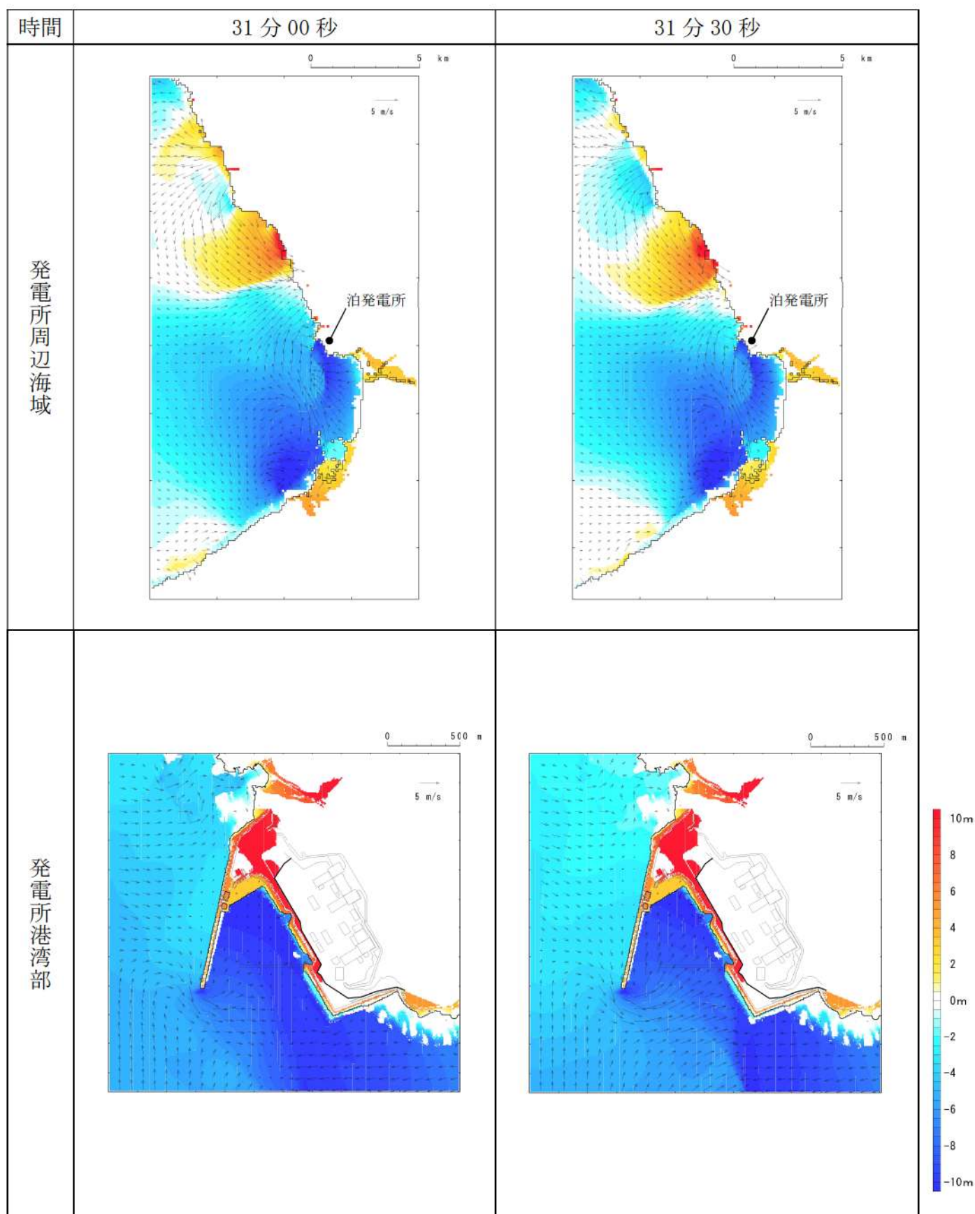
第 17 図-24 基準津波（波源K，南防波堤損傷）の水位変動・流向ベクトル(24/53)
