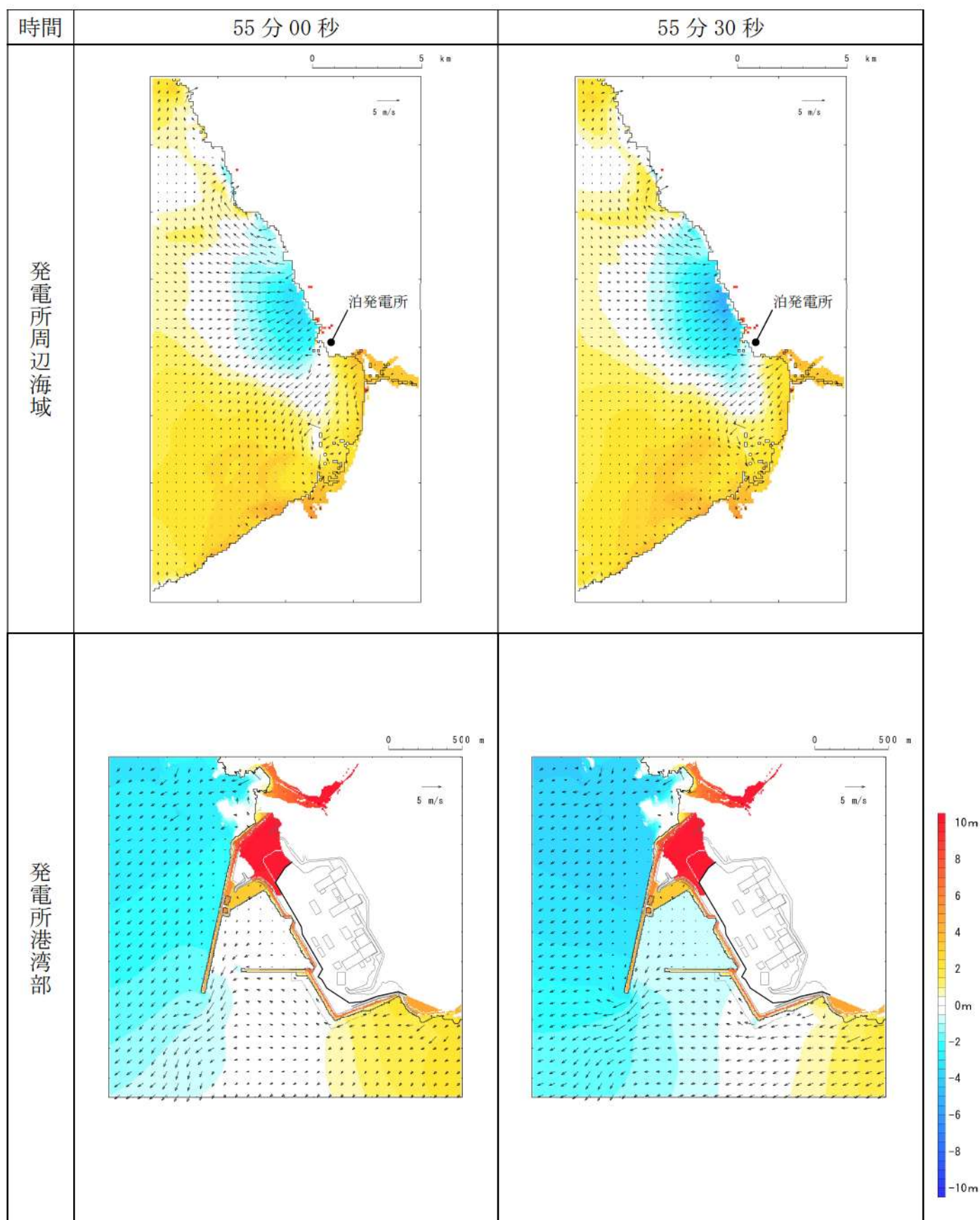
第 15 図-45 基準津波（波源 I，防波堤損傷なし）の水位変動・流向ベクトル(45/50)
