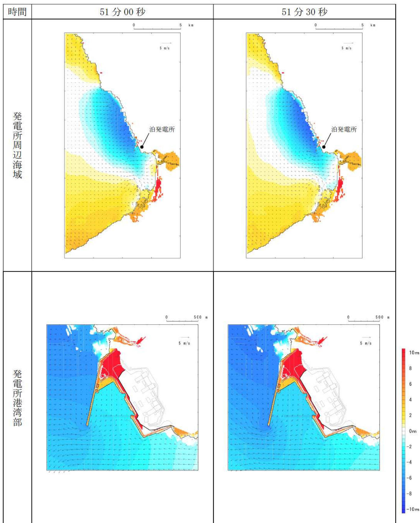
第 13 図-44 基準津波（波源 G，南防波堤損傷）の水位変動・流向ベクトル(44/53)
