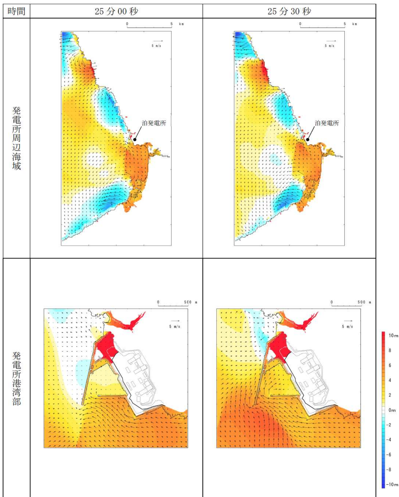
第 15 図-15 基準津波（波源 I，防波堤損傷なし）の水位変動・流向ベクトル(15/50)
