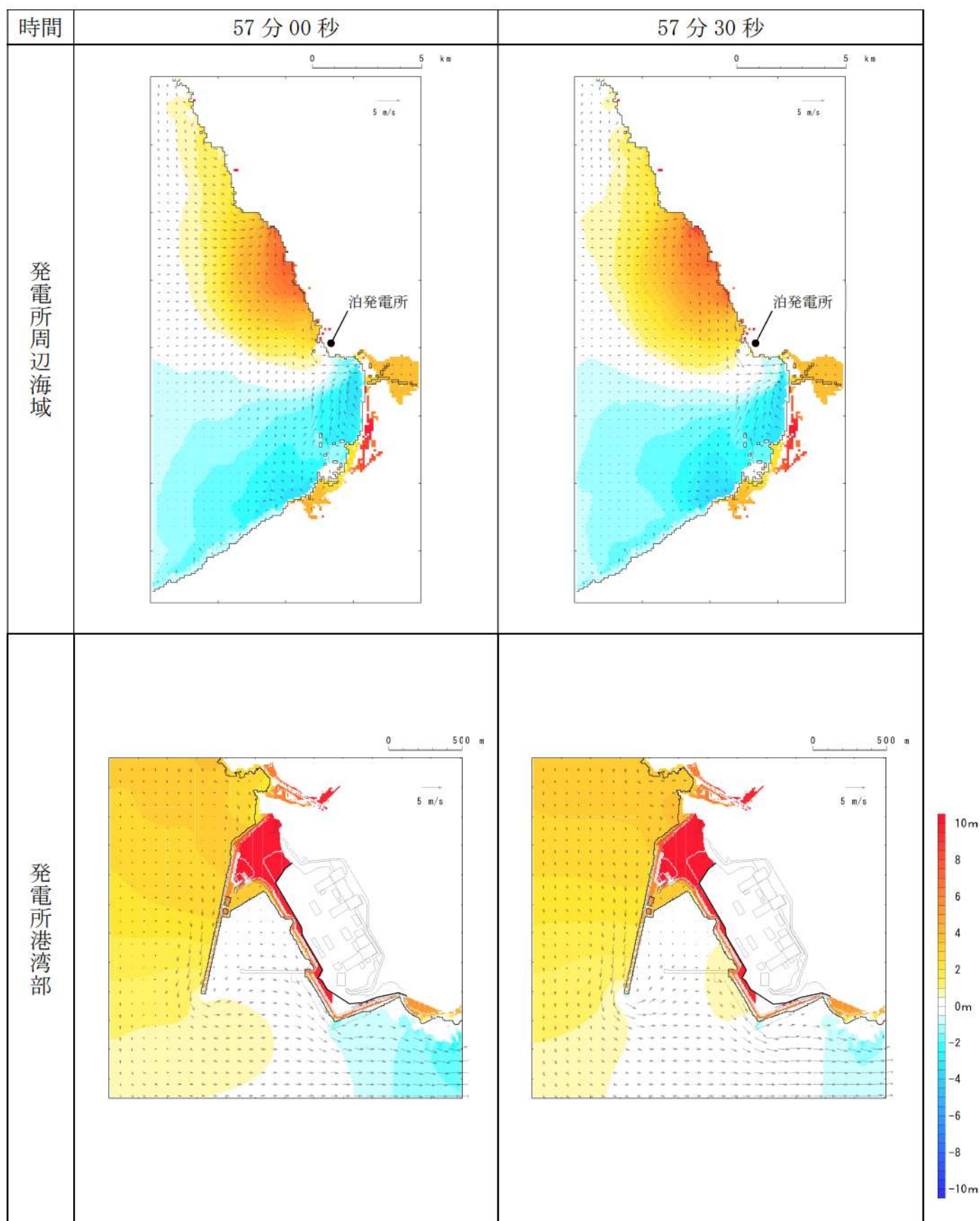
第 13 図-50 基準津波（波源G，南防波堤損傷）の水位変動・流向ベクトル(50/53)
