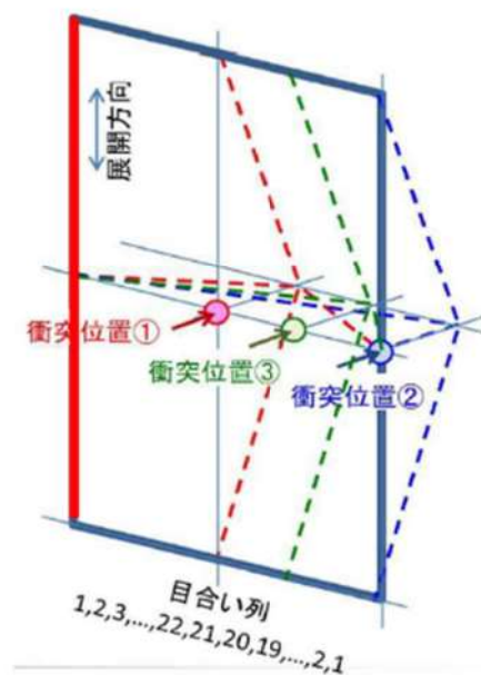
図5 衝突位置と金網固定位置の関係
