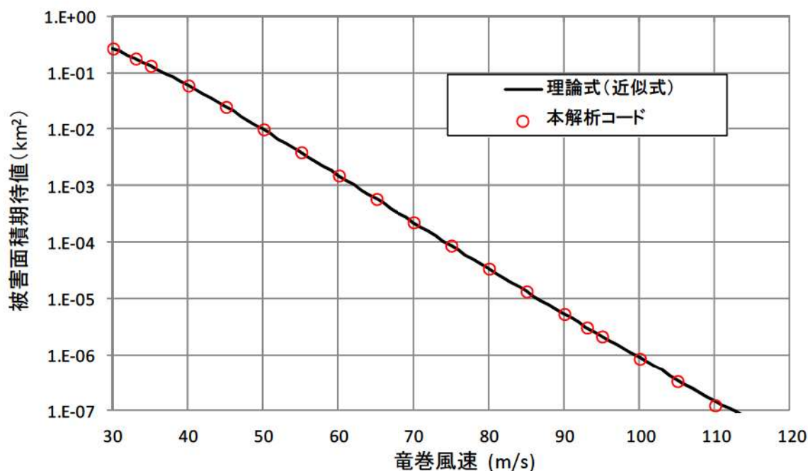
図6 被害面積の期待値の比較
