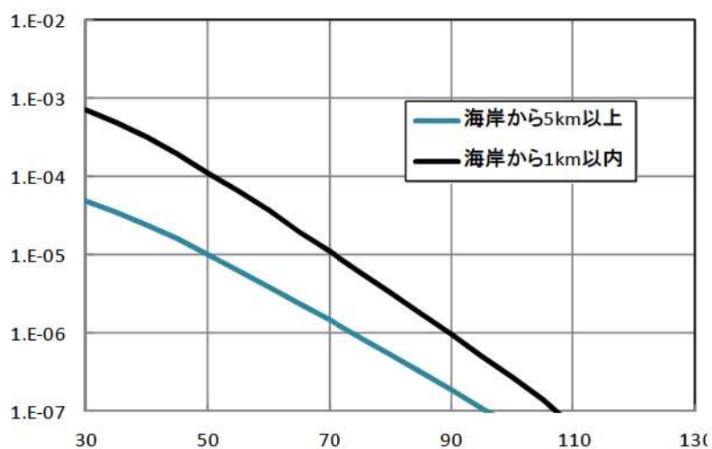
図8 ハザード算定結果（本解析コード）
