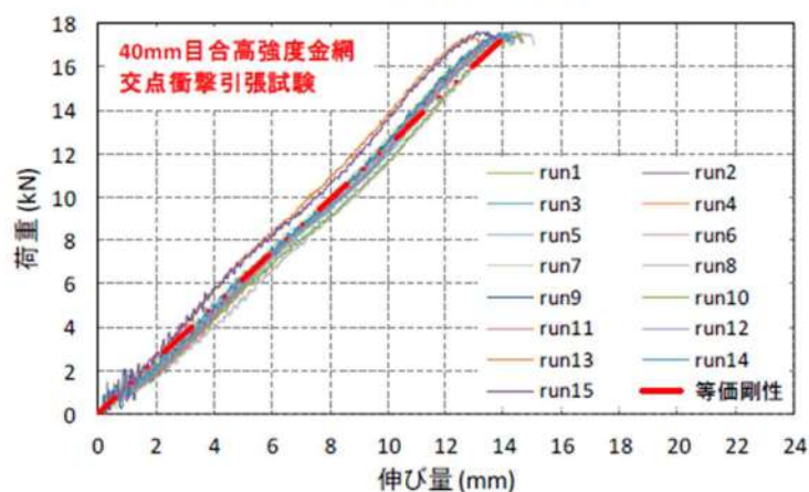
図 1 金網の荷重—伸び曲線
