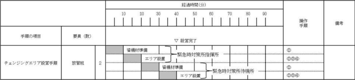
図3.3-2 チェンジングエリアの設置のタイムチャート
