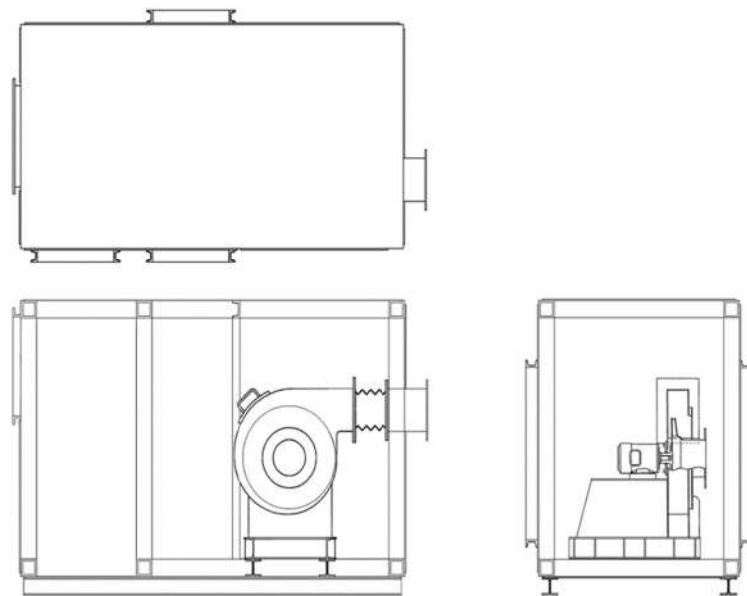
図 4-3 可搬型新設緊急時対策所用空気浄化ファン・原動機概要図
