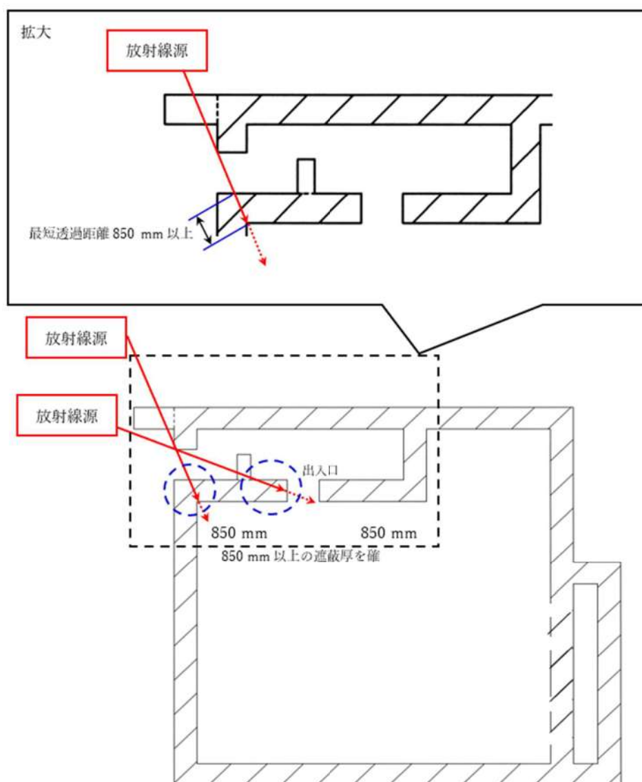
図5.11-1 出入口開口に関する遮蔽概要
