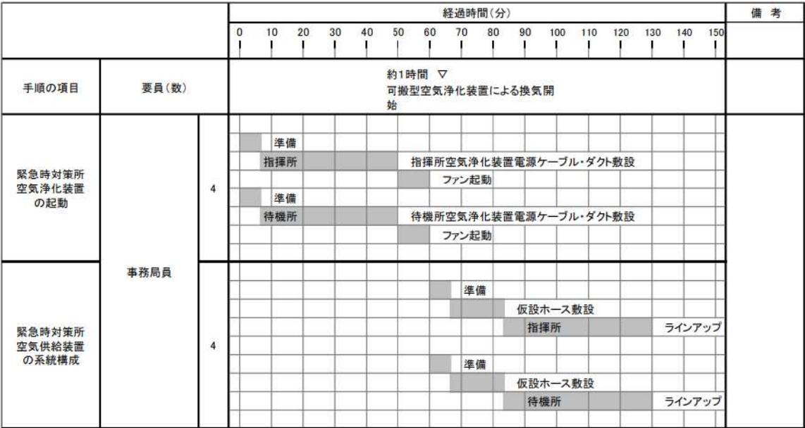
第 2 図 緊急時対策所空気浄化装置タイムチャート
