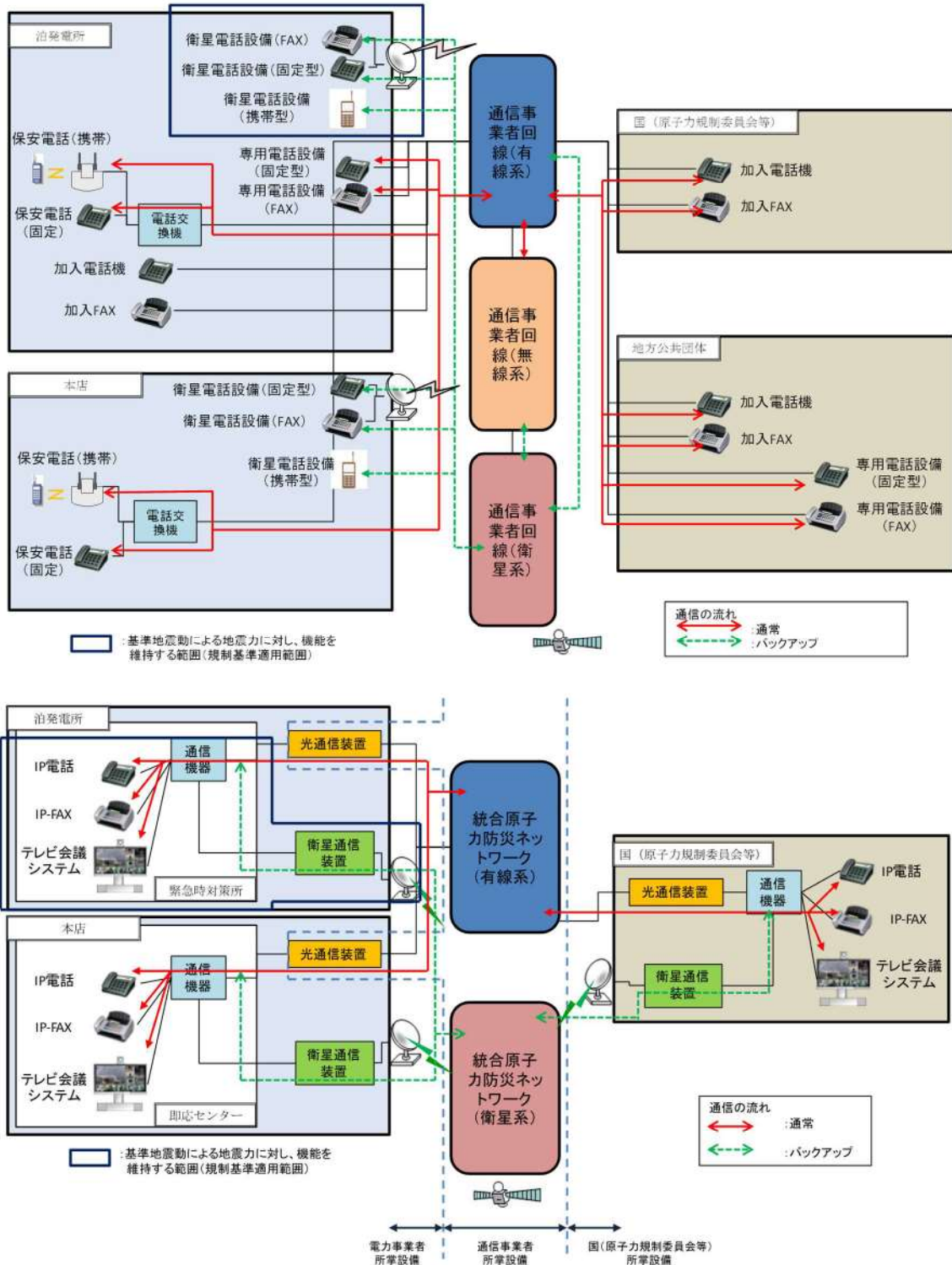
図 4-8 通信連絡設備の耐震設計範囲
