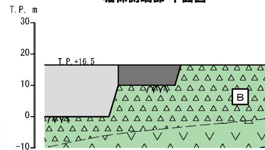
堀株側端部 地質縦断面図
