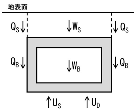
地下構造物の浮き上がりの評価
