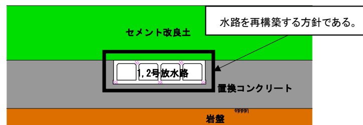
1,2号放水路正面イメージ図
