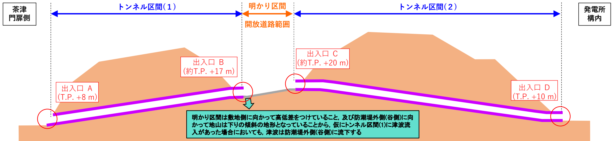
茶津入構トンネル 縦断面図
