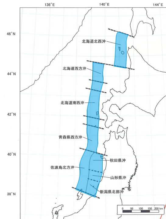
想定される日本海東縁部の範囲 (地震本部(2003)に一部加筆)
