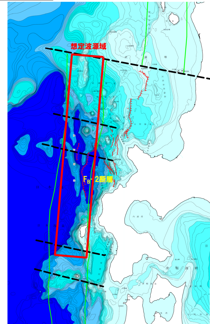
想定波源域と F_B -2断層の位置比較
