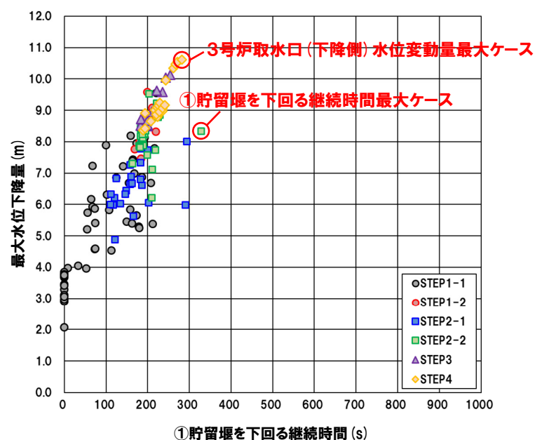
【①貯留堰を下回る継続時間】
