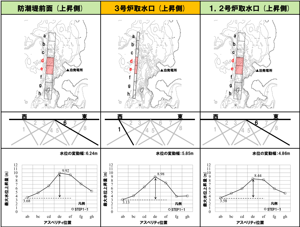
パラメータスタディ評価因子（防波堤の損傷を考慮した地形モデル①（北防波堤なし-南防波堤なし）） STEP1-1 東西方向位置・傾斜角及び傾斜方向 8通り（西傾斜，東傾斜）※東西幅50km，傾斜角30°，60° アスベリティ位置 隣接するアスベリティ位置（40kmピッチ） STEP1-2 アスベリティ詳細位置 隣接するアスベリティ位置（10kmピッチ） STEP2-1 アスベリティ数及び位置 隣接しないアスベリティ位置（40kmピッチ） STEP2-2 アスベリティ詳細位置 隣接しないアスベリティ位置（10kmピッチ） STEP3 波源位置 矩形モデル（基準），くの字モデル（基準）， 矩形モデル（東へ移動），くの字モデル（東へ移動） STEP4 断層面上縁深さ 0km，1km（基準），2km，3km，4km，5km
