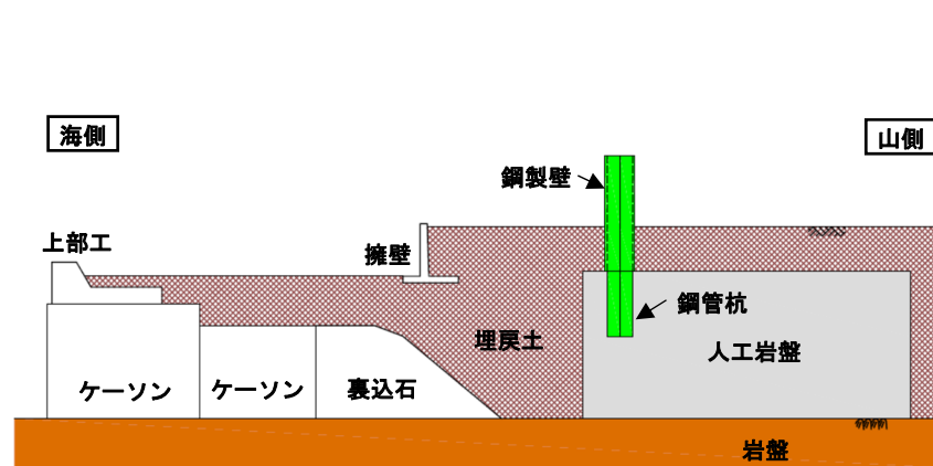
鋼製壁部(取合部) 断面図
