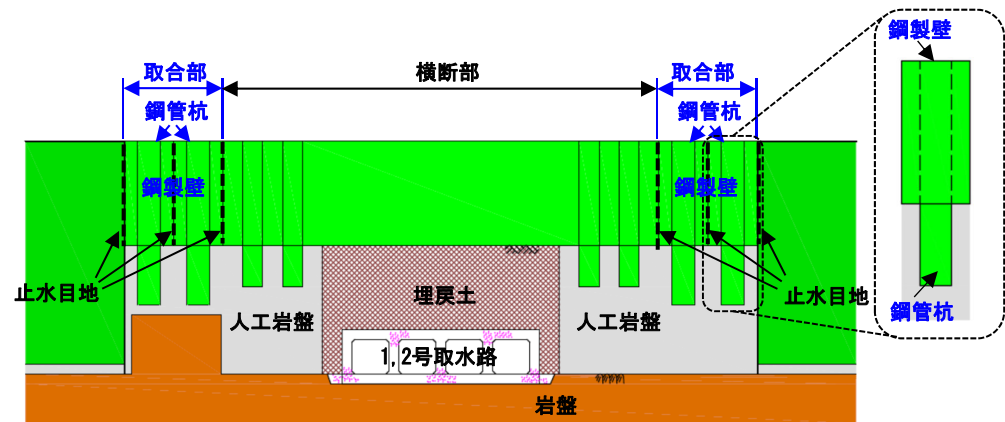
鋼製壁部(取合部) 正面図
