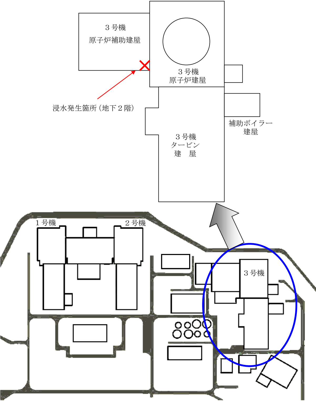
泊発電所 3 号機 配置図
