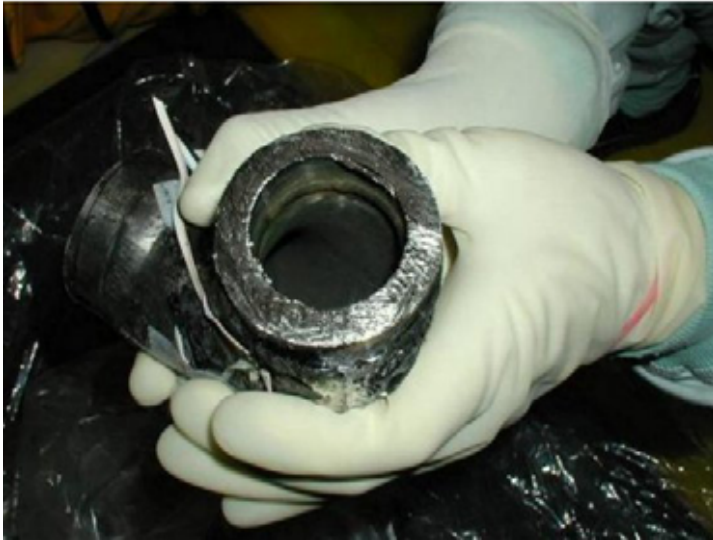
再生熱交換器 管台部
