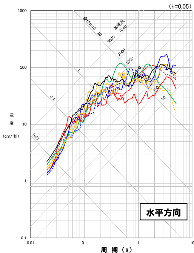
応答スペクトル図
