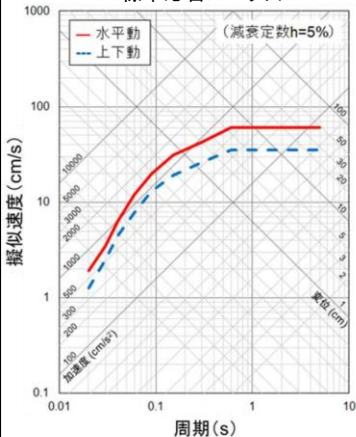
標準応答スペクトル
