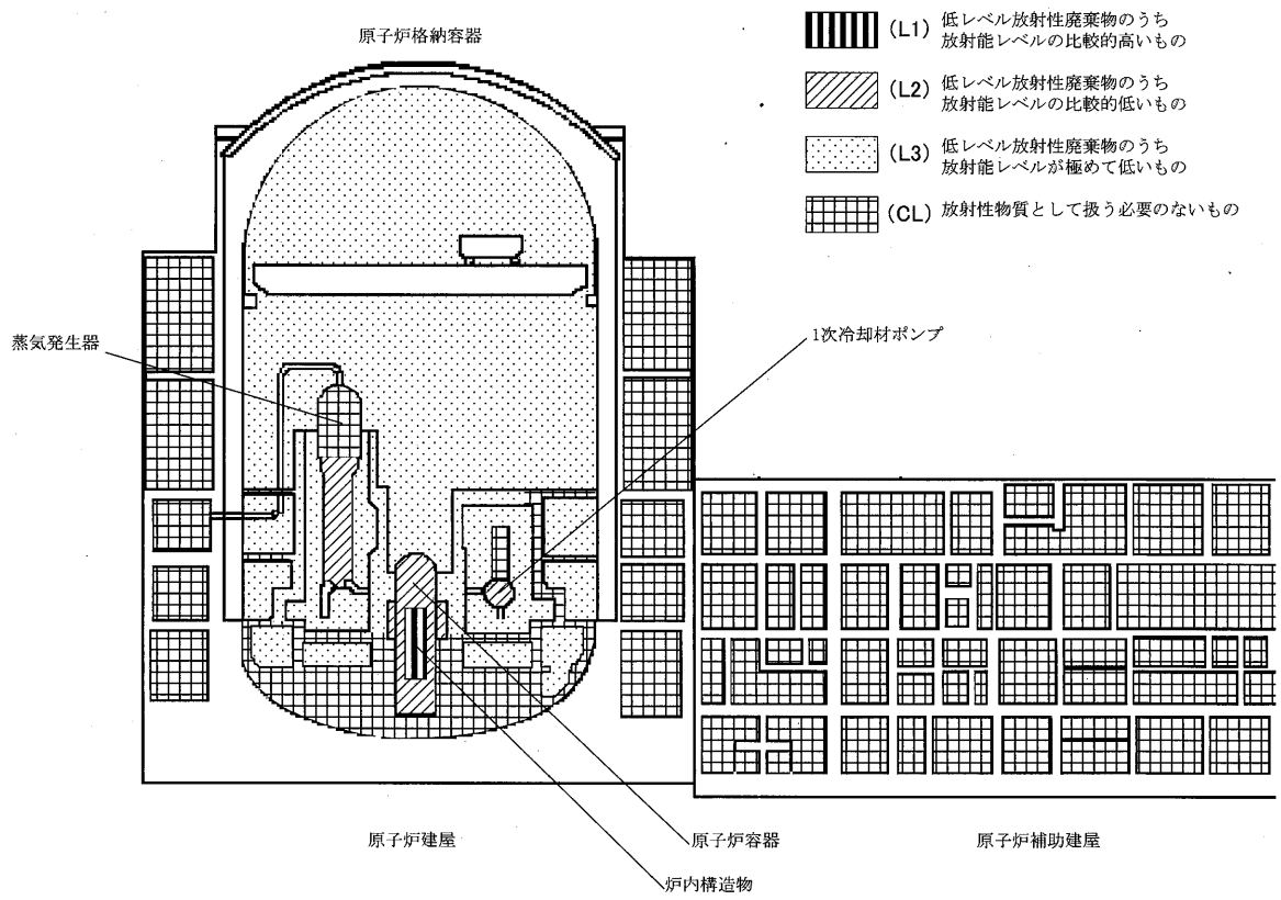
図 7 - 1 主な廃止措置対象施設の推定汚染分布
