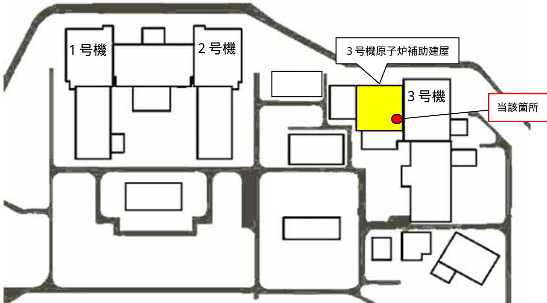
< 全体配置図 >
