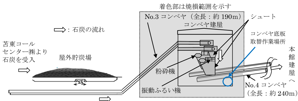
図2 運炭装置 概略図
