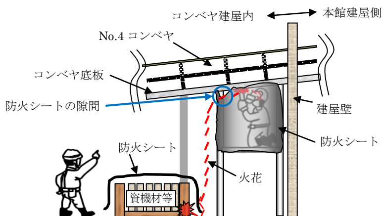
図3 コンベヤ底板取替作業(溶接作業) 概略図
