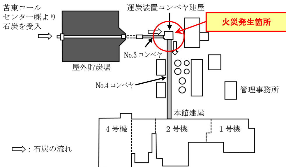
図1 運炭装置コンベヤ建屋配置図
