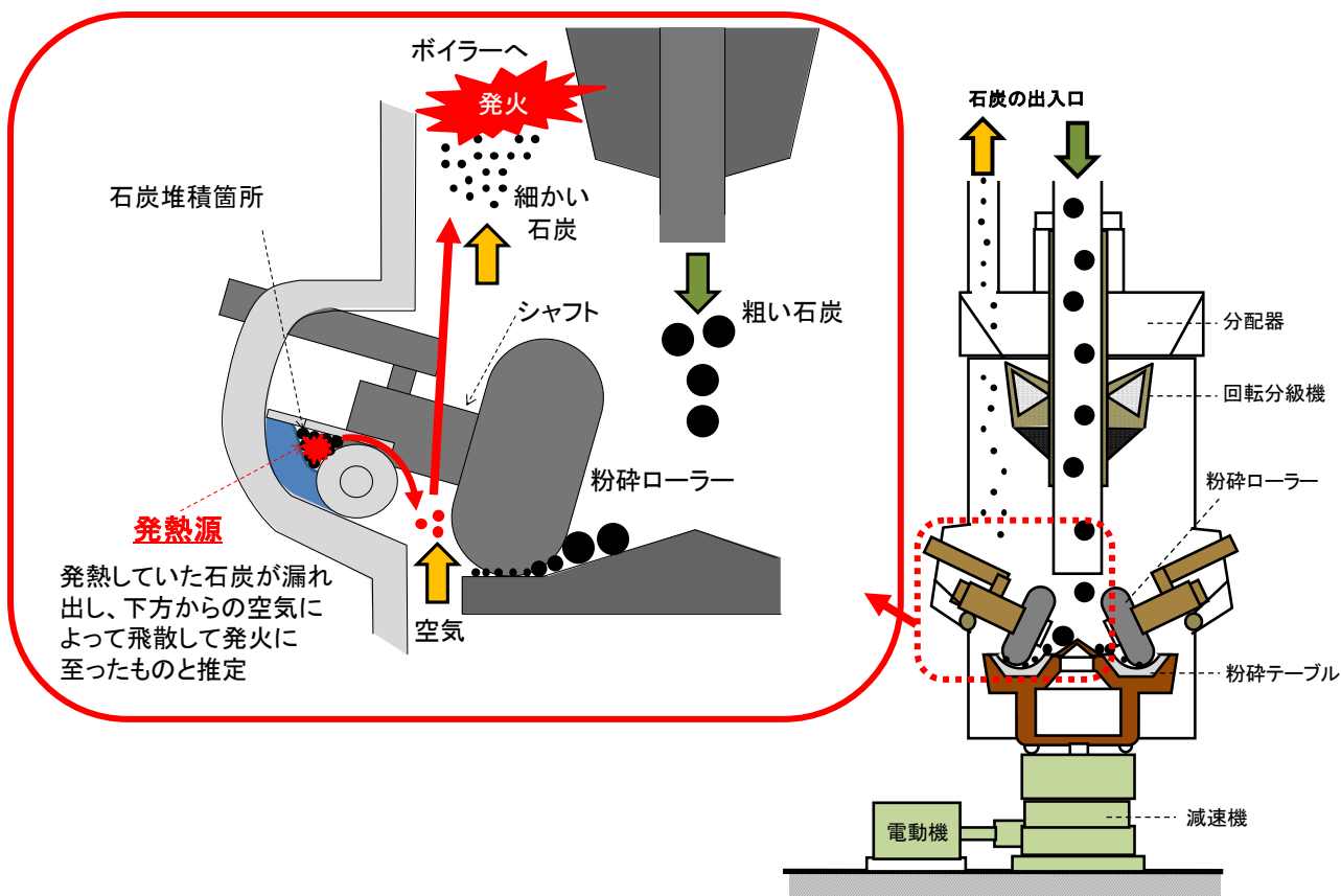
微粉炭機の概要図
