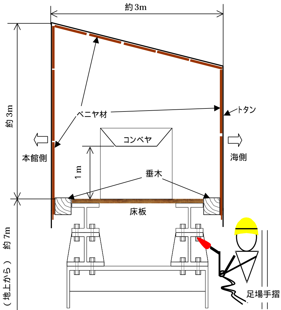
図2 火災発生時の作業状況 (No.2-1 コンベヤ建屋断面図)
