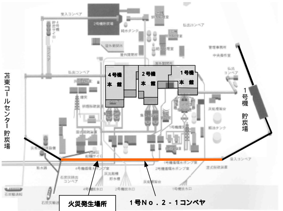
図1 構内配置図
