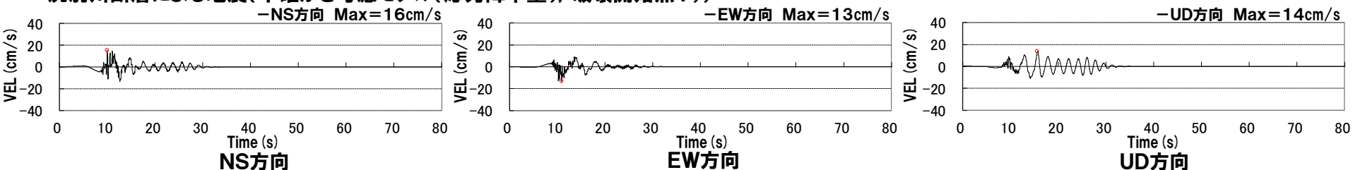
尻別川断層による地震(不確かさ考慮モデル(応力降下量), 破壊開始点2))
