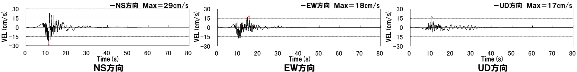
積丹半島北西沖の断層による地震(走向0° ケース, 不確かさ考慮モデル(断層の傾斜角), 破壊開始点3))
