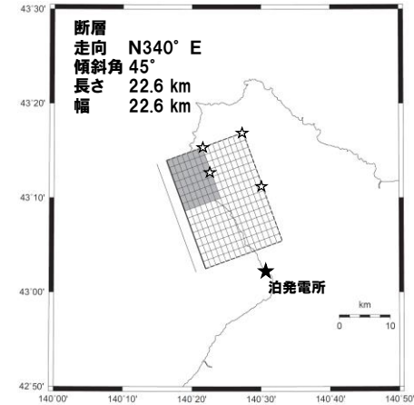
N340° E(走向20° )
