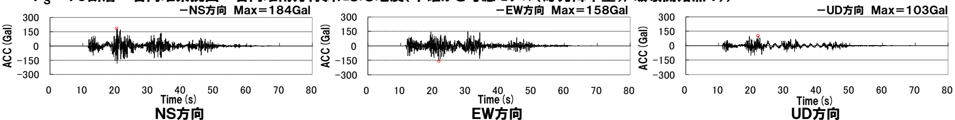
F_S-10 断層～岩内堆東撓曲～岩内堆南方背斜による地震(不確かさ考慮モデル(応力降下量), 破壊開始点4))
