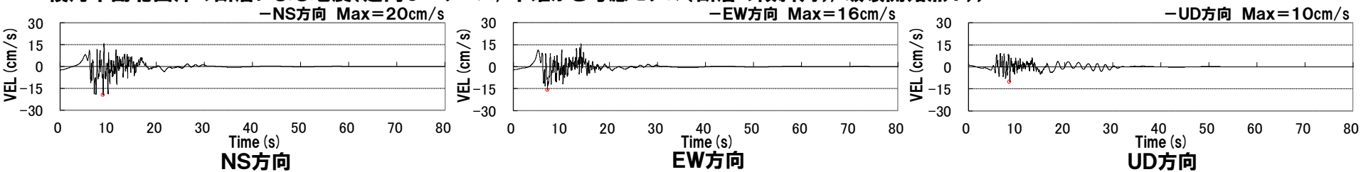
積丹半島北西沖の断層による地震(走向0° ケース, 不確かさ考慮モデル(断層の傾斜角), 破壊開始点2))
