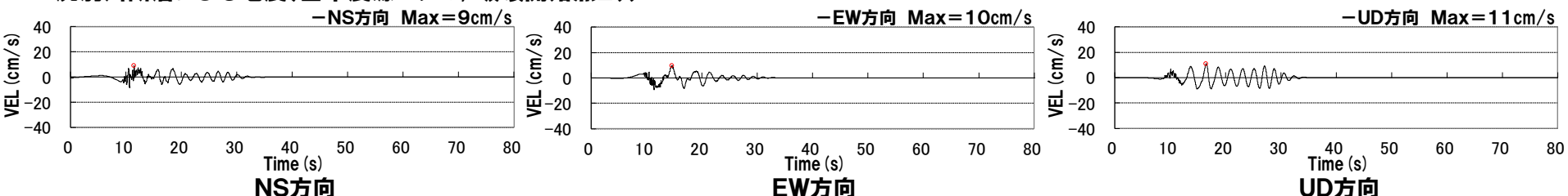
尻別川断層による地震(基本震源モデル, 破壊開始点3))
