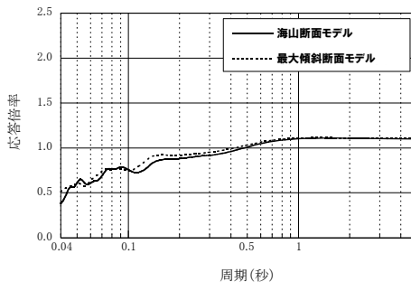
3号炉心直下 伝達関数(+25度)
