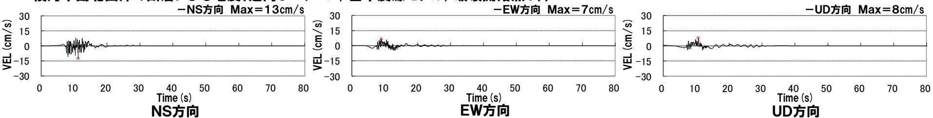
積丹半島北西沖の断層による地震(走向0° ケース, 基本震源モデル, 破壊開始点2))
