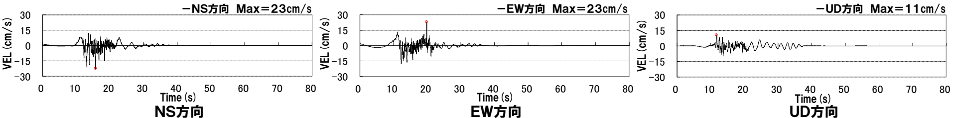
積丹半島北西沖の断層による地震(走向0° ケース, 不確かさ考慮モデル(断層の傾斜角), 破壊開始点4))
