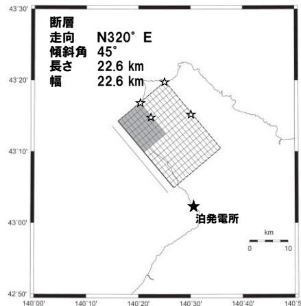
N320° E(走向40° )
