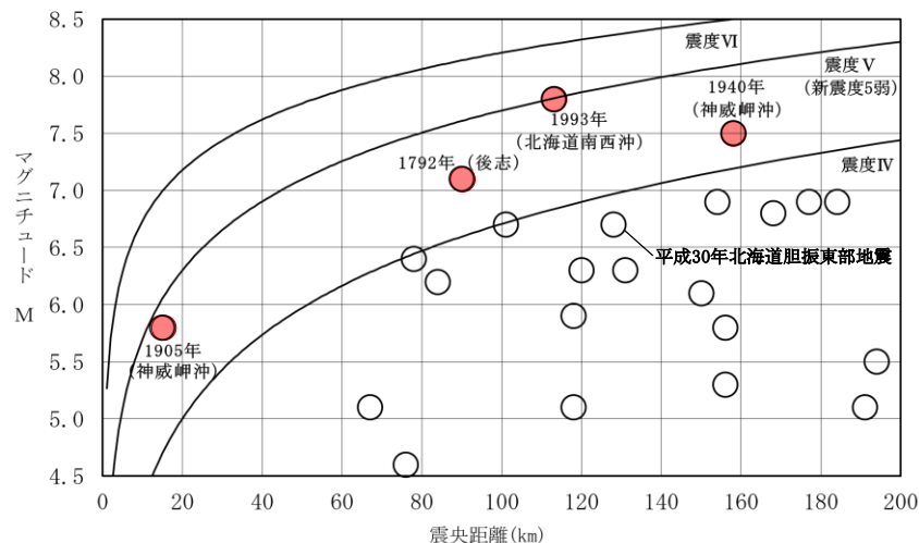
敷地周辺の被害地震のマグニチュードー震央距離図
