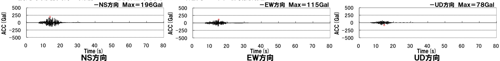
積丹半島北西沖の断層による地震(基本震源モデル(走向 0^{\circ} ),破壊開始点4))
