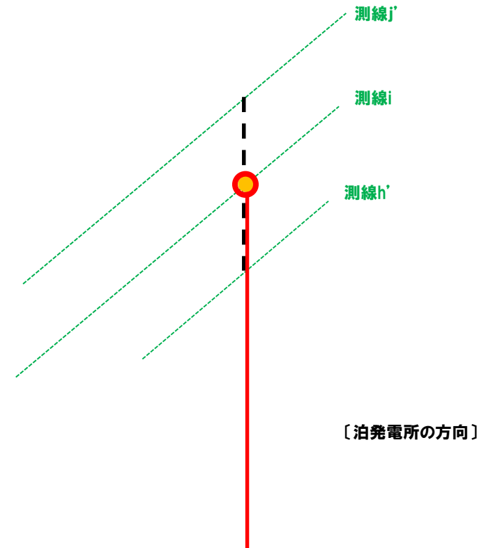
断層位置のイメージ
