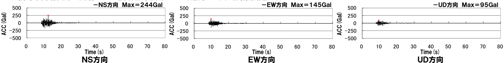
積丹半島北西沖の断層による地震(基本震源モデル(走向 0^{\circ} ),破壊開始点3))
