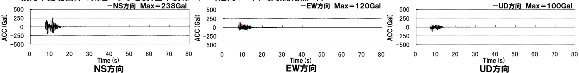
積丹半島北西沖の断層による地震(基本震源モデル(走向 0^{\circ} ),破壊開始点2))
