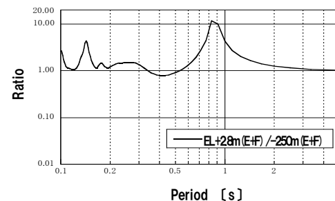
3号炉地盤モデル(後背斜面モデル)伝達関数
