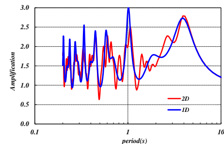
伝達関数
