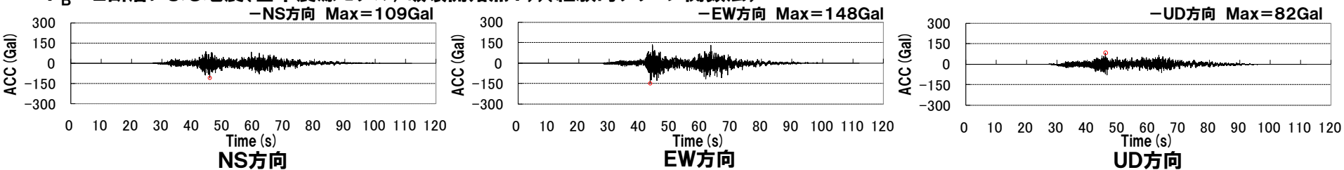
F_B-2 断層による地震(基本震源モデル, 破壊開始点2)(経験的グリーン関数法)
