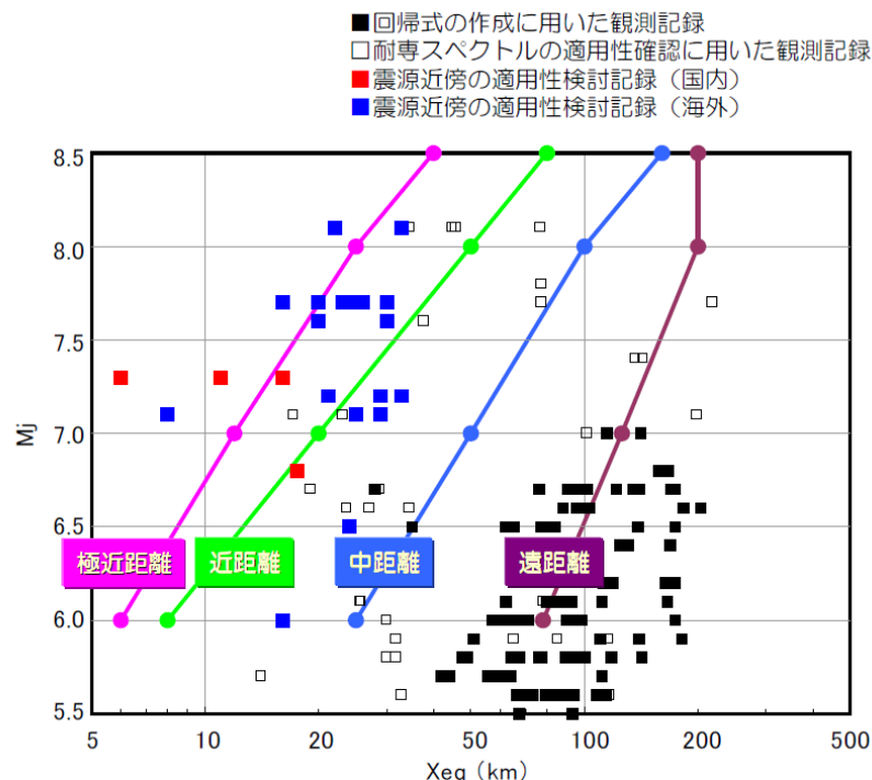
Noda et al. (2002)の地震データの比較 (東京電力(2009))
