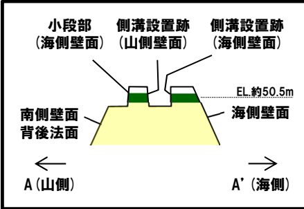
平面模式図 南側壁面の背後法面 天端付近 断面模式図(A-A'断面)
