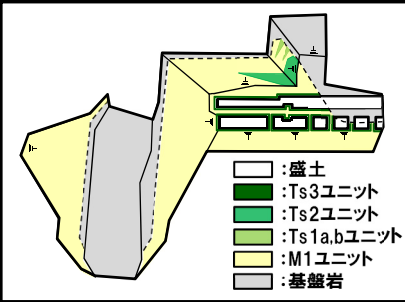
平面模式図 南側壁面の背後法面 天端付近 断面模式図(A-A'断面)
