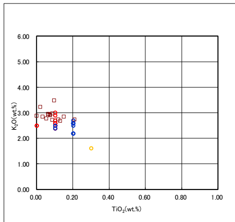
A-2-b 火山ガラスのK 2 O-TiO 2 図(左図), K 2 O-Na 2 O図(右図)
