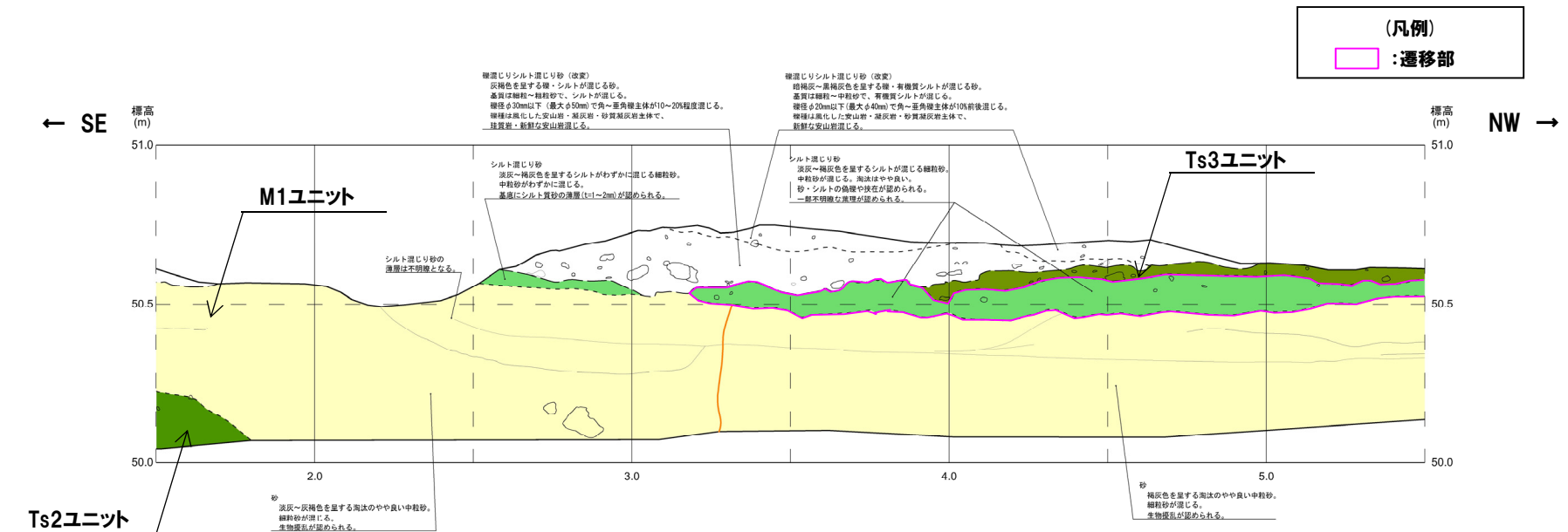
開削調査箇所(南側)小段部(海側壁面) スケッチ(範囲B)
