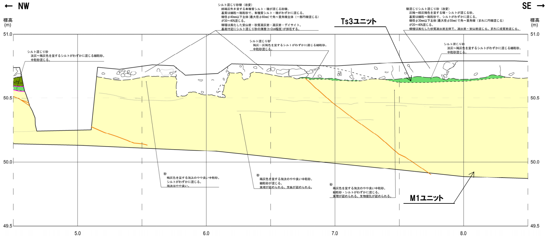
開削調査箇所(南側)海側壁面 スケッチ(範囲C)
