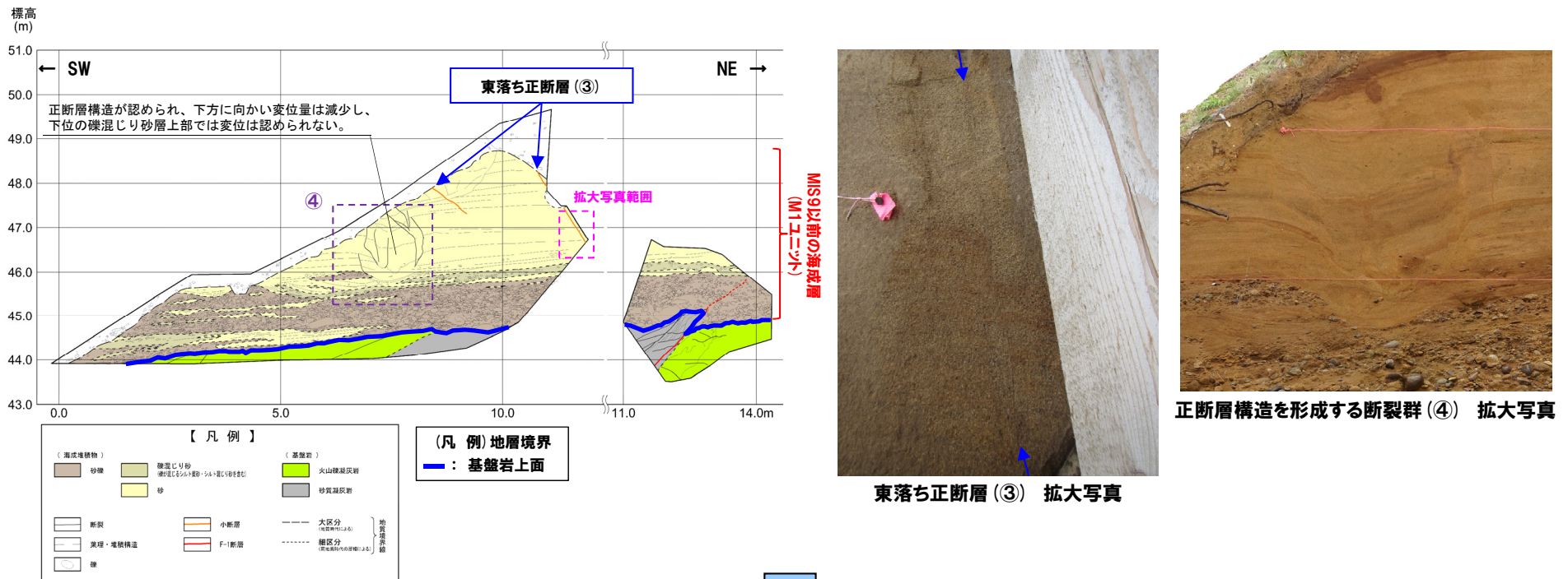
開削調査箇所(南側) 北側壁面スケッチ
