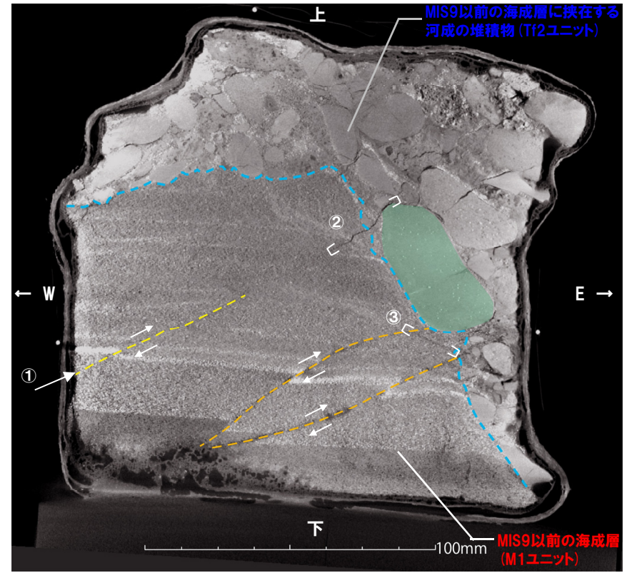
マイクロフォーカスX線CT画像(解釈線あり) (断面(A):ブロック試料中央断面から約2cm手前方向, P371断面再掲)
