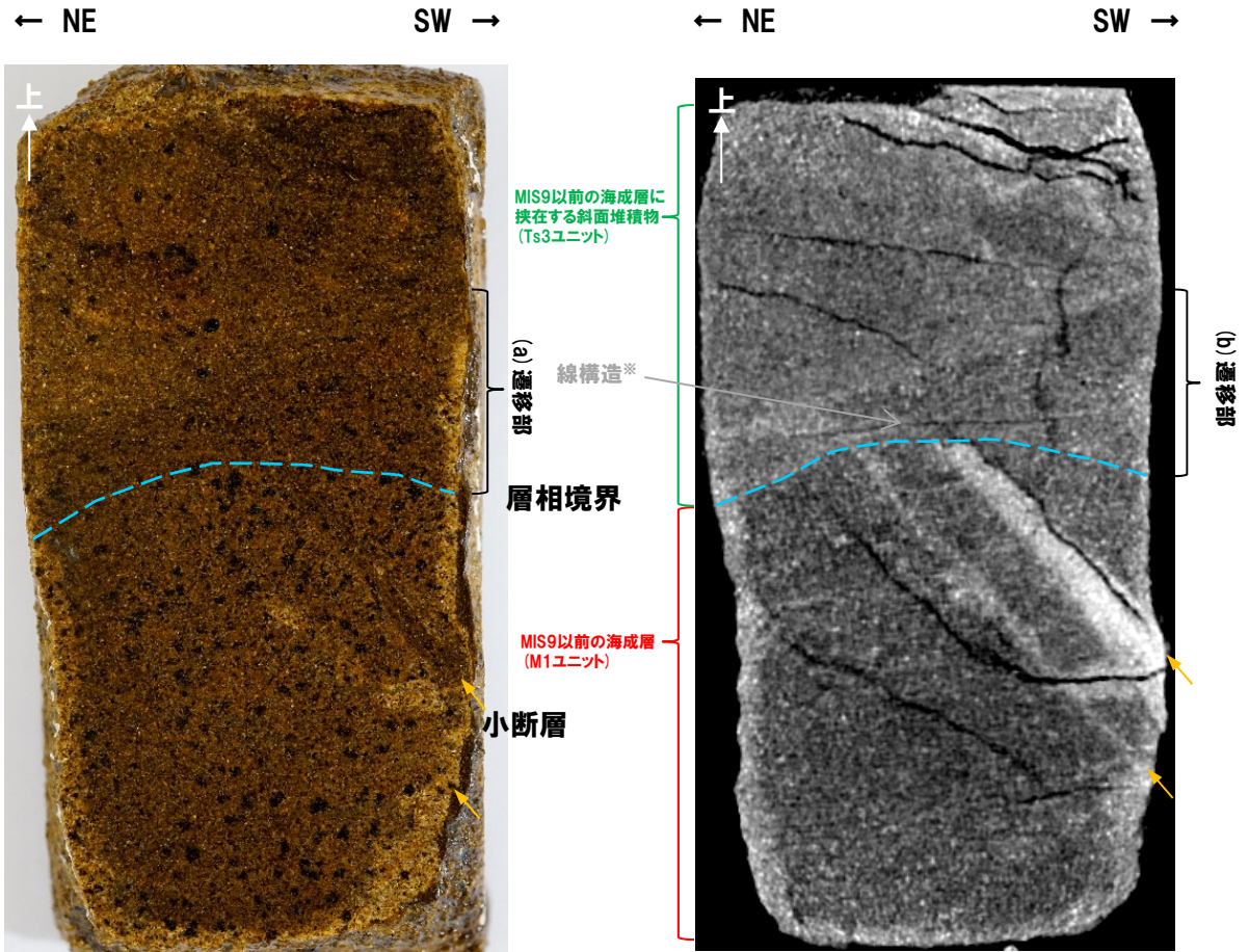
傾斜方向研磨片 (解釈線あり) 5cm
