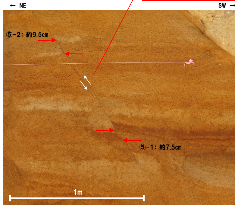
⑤ 見かけ鉛直変位量計測箇所
