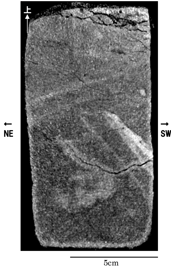
X線CT画像(傾斜方向断面, 解釈線なし) (断面(D): 研磨片作成位置断面から奥行き方向に約10mmの位置)
