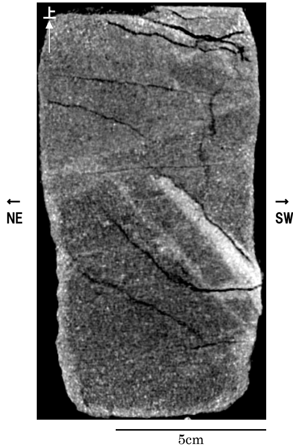
X線CT画像(傾斜方向断面, 解釈線なし) (断面(B): 研磨片作成位置断面, P429断面再掲)
