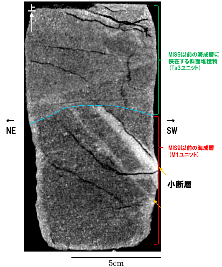
X線CT画像(傾斜方向断面, 解釈線あり) (断面(B): 研磨片作成位置断面, P427断面再掲)
