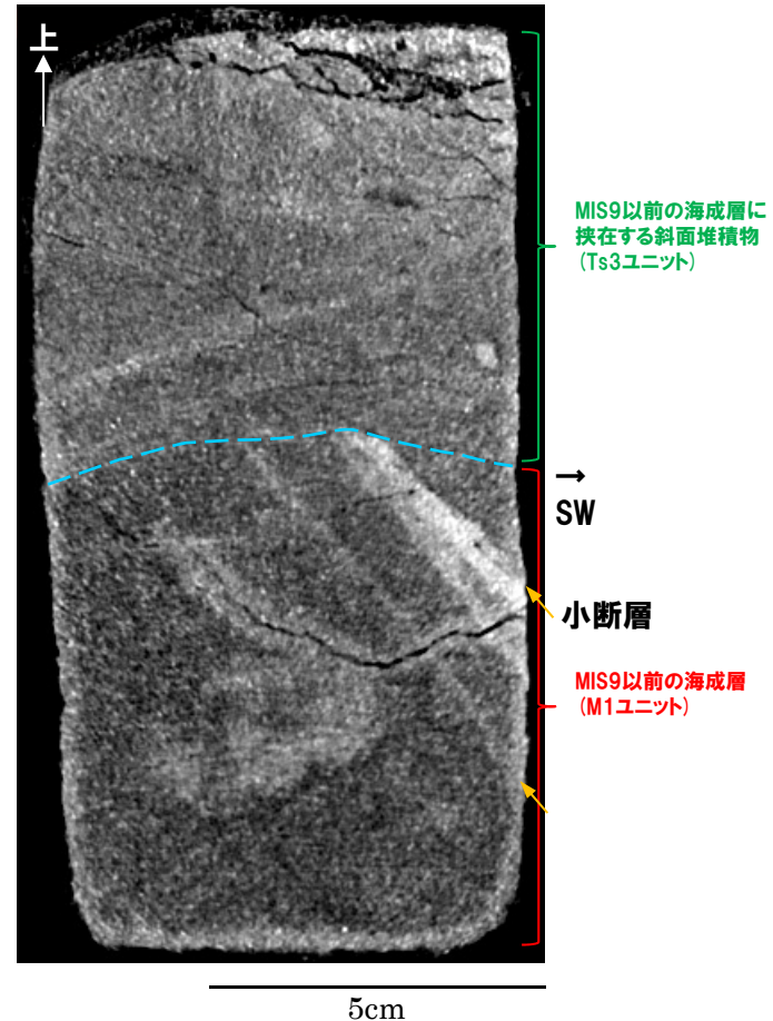
X線CT画像(傾斜方向断面, 解釈線あり) (断面(D): 研磨片作成位置断面から奥行き方向に約10mmの位置)
