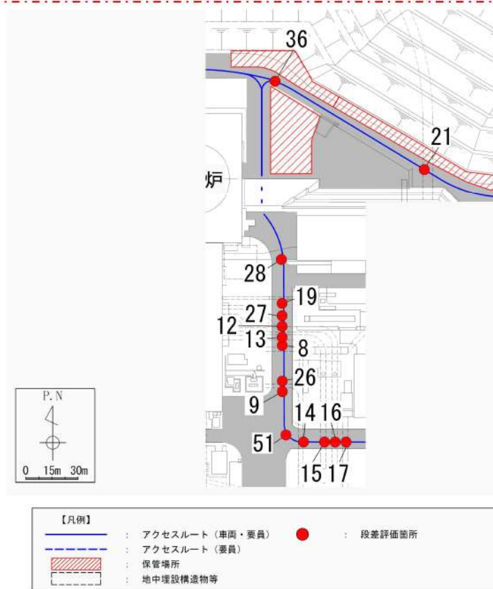
第 6-20 図 地中埋設構造物等と埋戻部との境界部における 段差評価結果 (3/5) (Bエリア)
