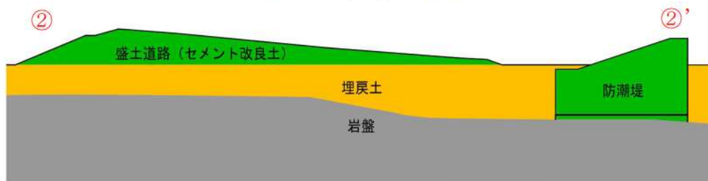
Cエリア②-②' 地点
