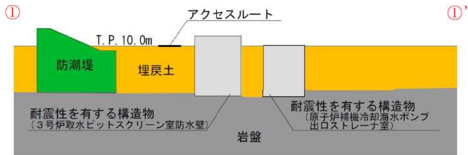
Bエリア①-①' 地点
