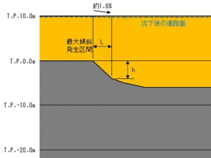
A エリア縦断図
