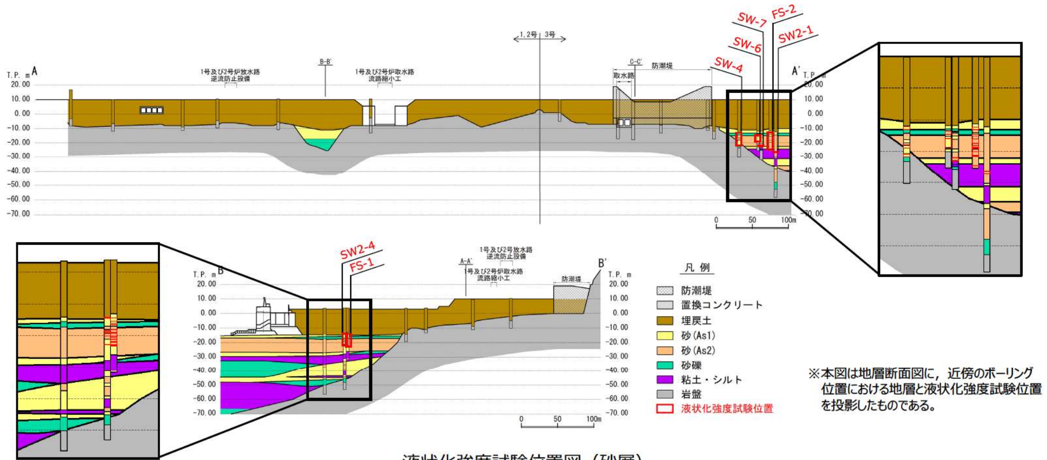
液状化強度試験位置図 (砂層)
