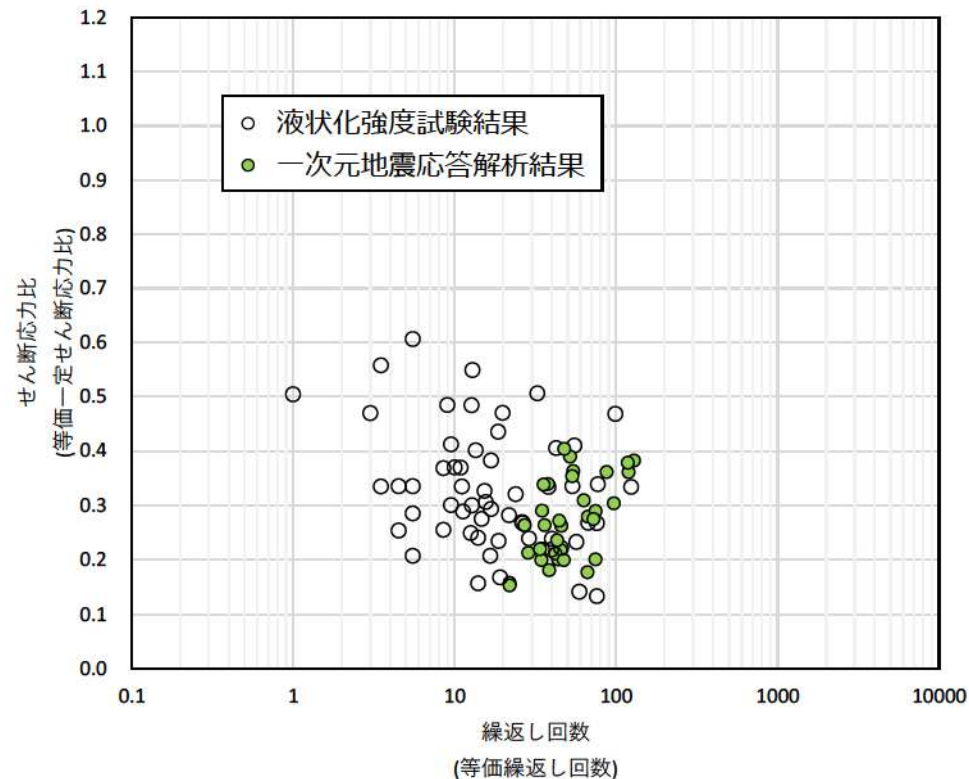
(例) 液状化強度試験結果と一次元地震応答解析結果の比較
