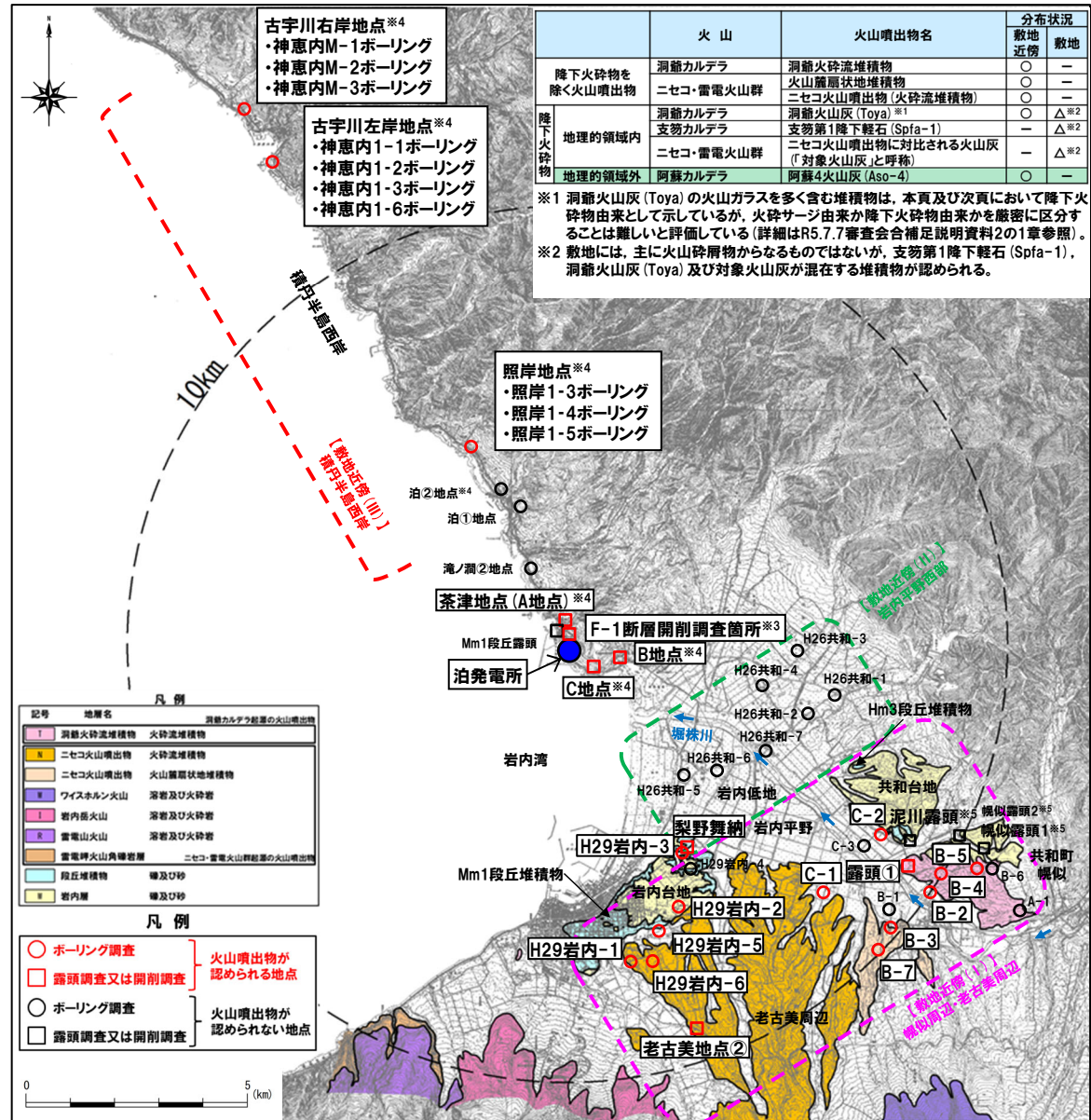
③ 文献及び当社地質調査結果を踏まえた敷地周辺における支笏火砕流堆積物の分布状況確認 (4/5)
