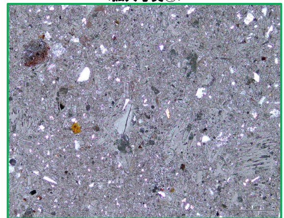
クロスニコル (左方向に45° 回転)
