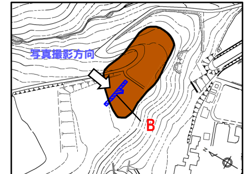
凡例 Hm2段丘面
