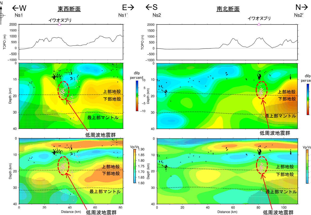
地震波速度構造(鉛直断面)
