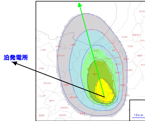
n.En-b (分布主軸上で給源～敷地と同程度の距離における 層厚:0cm)
