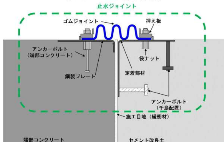
止水ジョイント設置概要（A-A' 断面）
