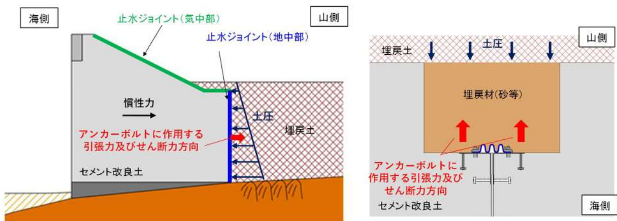
第 7-49 図 埋戻材の土圧及び止水ジョイントのうちアンカーボルトに作用する荷重方向
