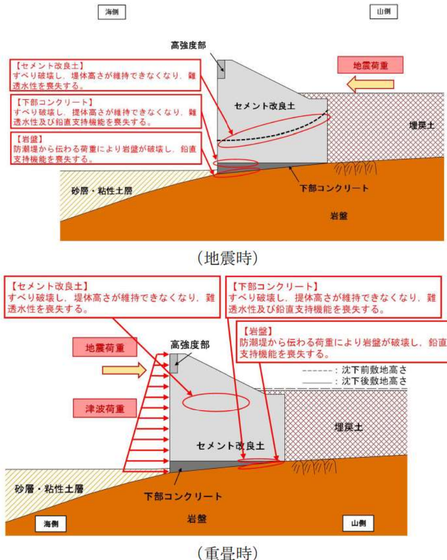
第 5-37 図 防潮堤（標準部）の構造上の弱部（地震時，重畳時）
