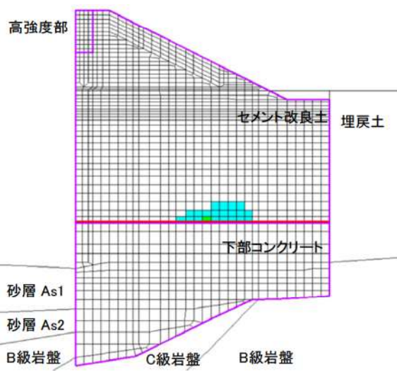
セメント改良土及び高強度部における すべり安全率最小時刻時の局所安全係数分布
