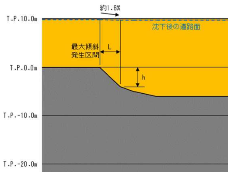
A-A' エリア縦断図
