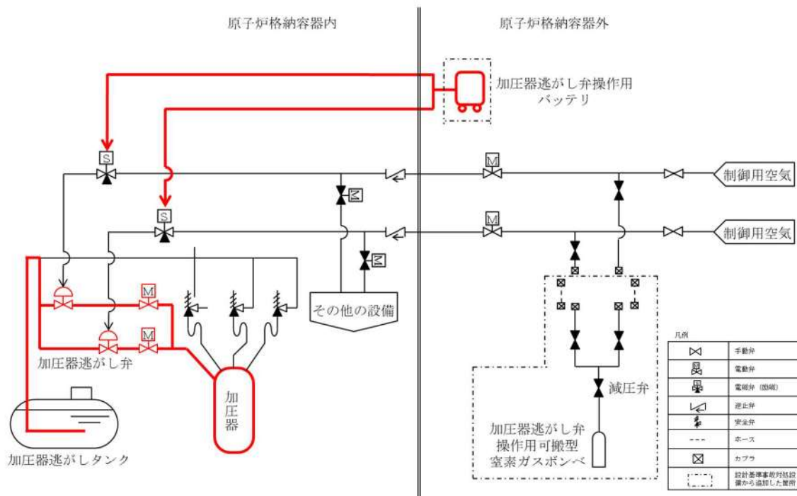
第 60 図 燃料冷却機能の系統概要図 (5 / 6)
