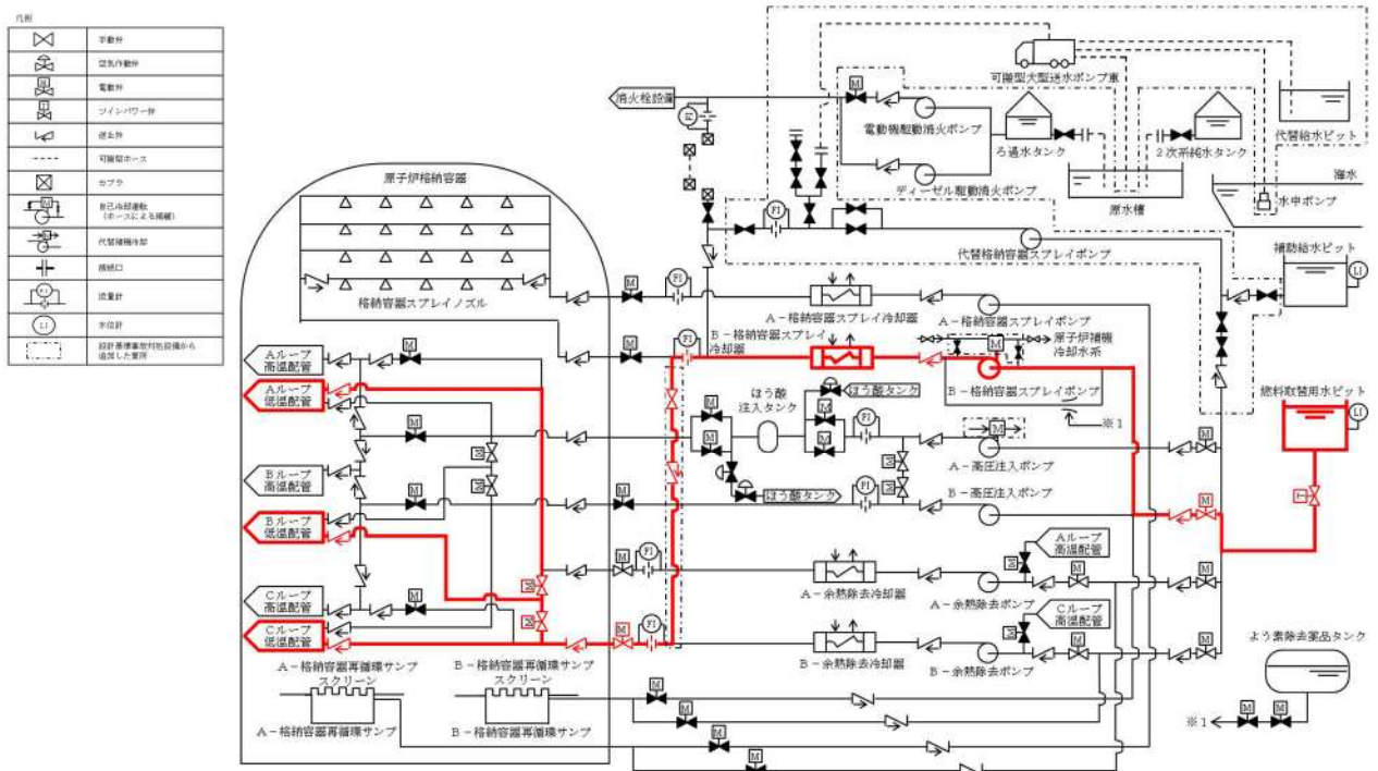
第18-1図 代替炉心注水 (B-格納容器スプレイポンプ) 系統概要図
