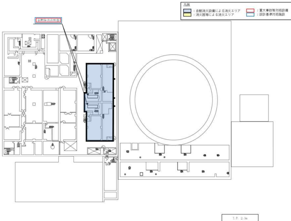
第 2 1 図 代替炉心注水（代替格納容器スプレイポンプ）に関する機器の配置（1 / 2）
