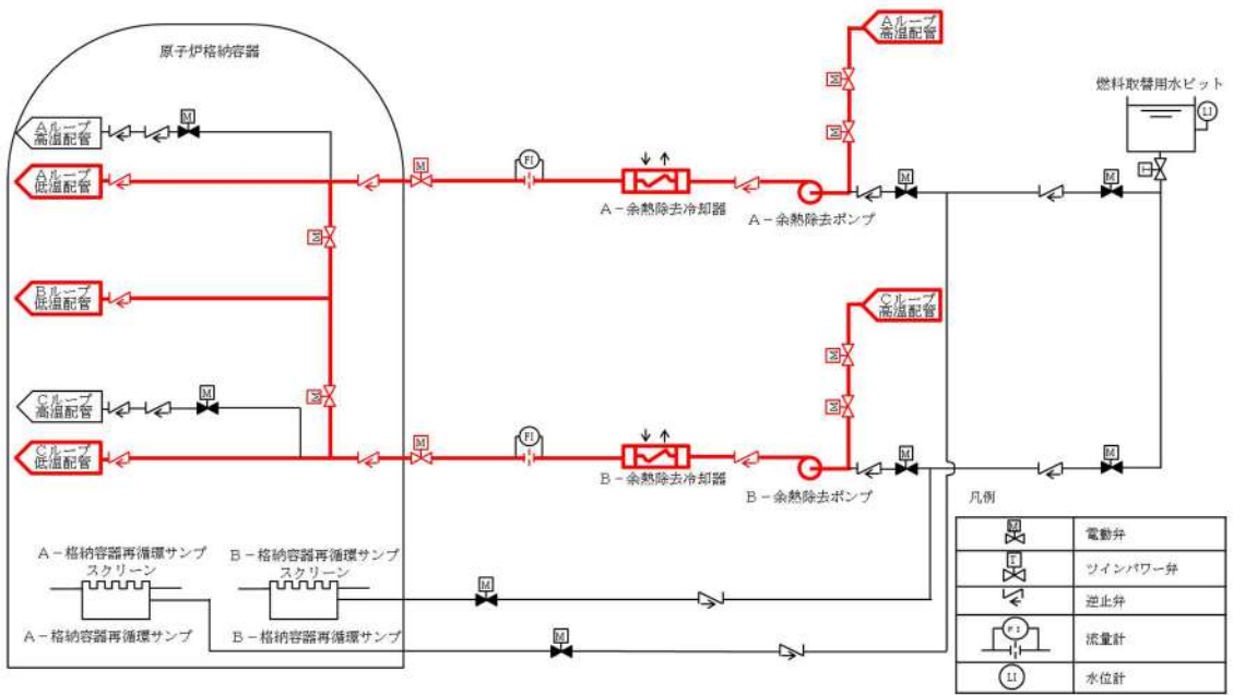
第 2 4 - 3 図 余熱除去運転（余熱除去設備による崩壊熱除去）系統概要図
