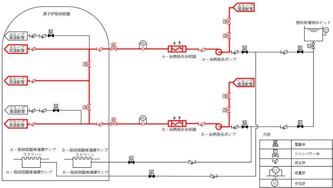
第 2 2 - 3 図 余熱除去運転（余熱除去設備による崩壊熱除去）系統概要図
