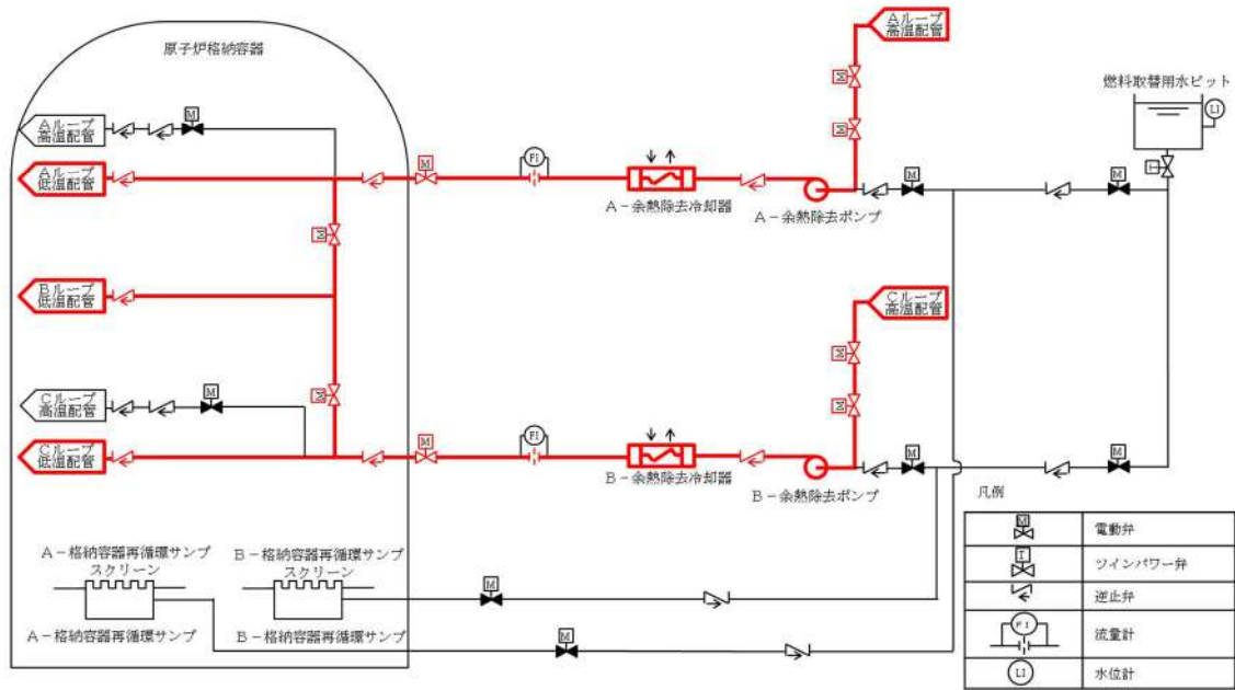
第20-6図 余熱除去運転（余熱除去設備による崩壊熱除去）系統概要図
