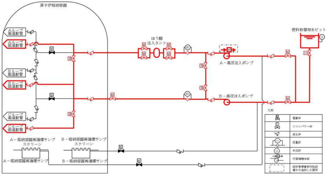
第20-3図 高圧注入ポンプによる炉心注水 系統概要図
