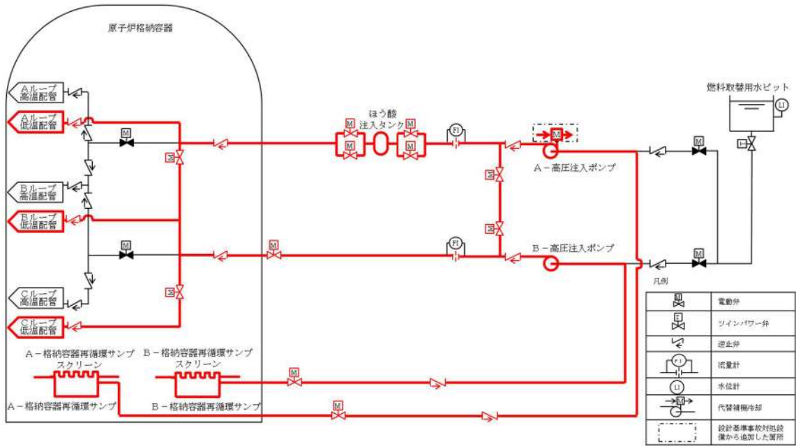
第20-5図 高圧注入ポンプによる再循環運転 系統概要図
