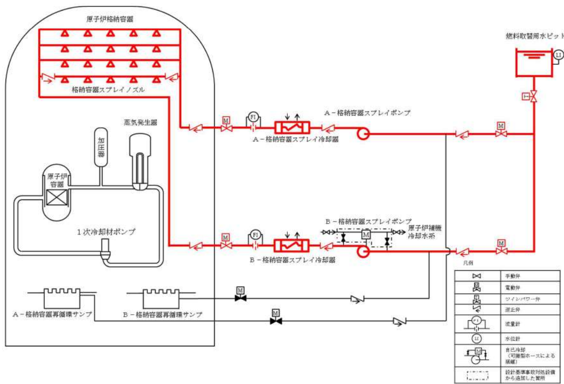
第4 2 - 2 図 格納容器スプレイ 系統概要図
