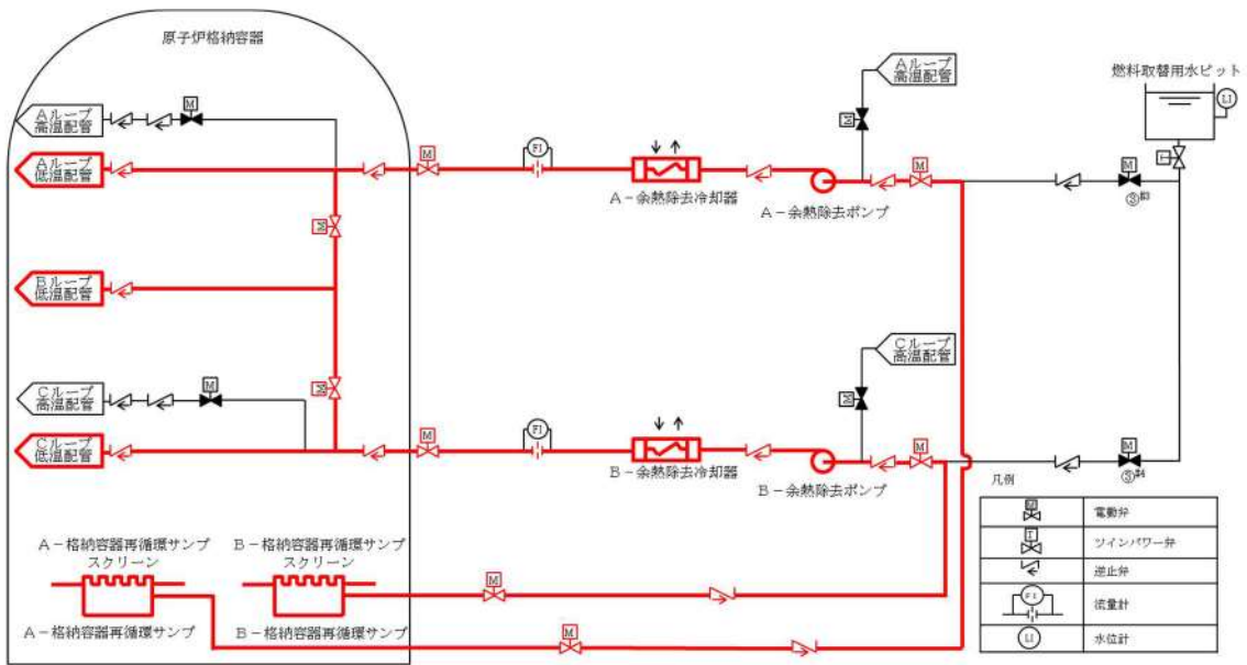
第 18-4 図 余熱除去ポンプによる再循環運転 系統概要図
